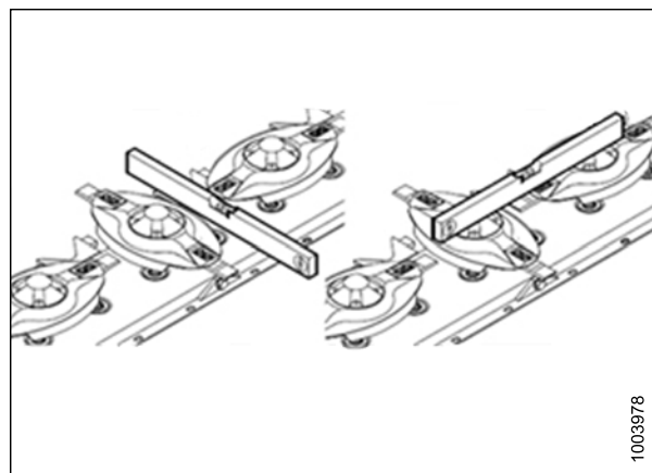
Figure 6.17: Niveau à bulle sur la barre de coupe
