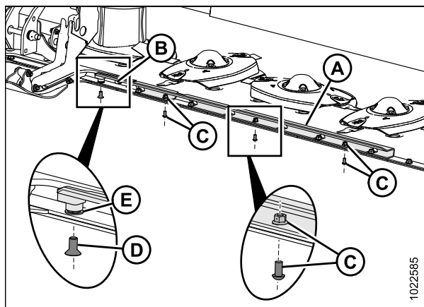
Figure 8.16: Déflecteurs gauche de la barre de coupe
