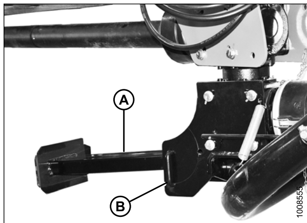
Figure 3.125: Chandelle d'attelage
