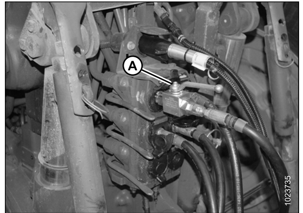
Figure 7.10: Vanne de verrouillage de la direction en position ouverte
