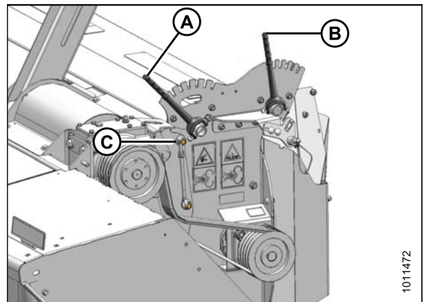
Figure 8.11: Côté gauche de la conditionneuse à peignes
