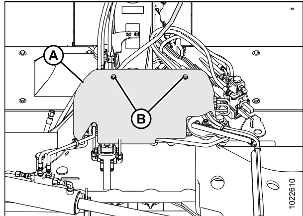
Figure 4.54: Capot (vue de dessus)
