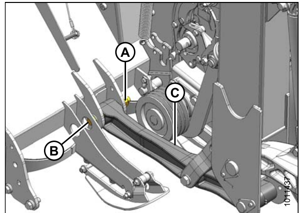
Figure 8.6: Côté gauche de la conditionneuse
