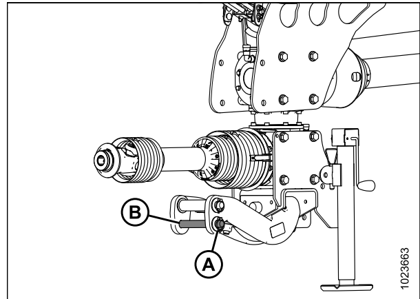
Figure 3.115: Attelage de la faucheuse à disques
