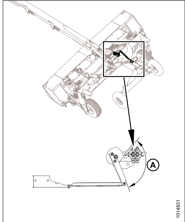
Figure 6.39: Ensemble du mécanisme de déploiement/rotation du transport
