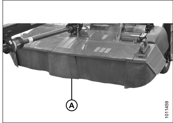
Figure 3.154: Rideaux de porte de la barre de coupe
