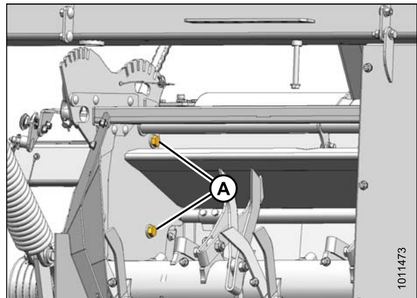
Figure 8.13: Côté gauche de la conditionneuse à peignes – Côté droit similaire
