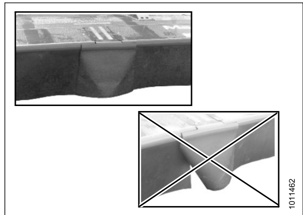
Figure 4.122: Rideaux de porte de la barre de coupe
