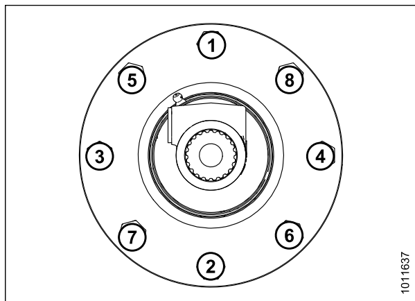
Figure 6.37: Séquence de serrage
