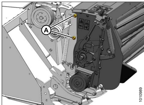
Figure 8.19: Côté gauche de la conditionneuse – Côté droit similaire
