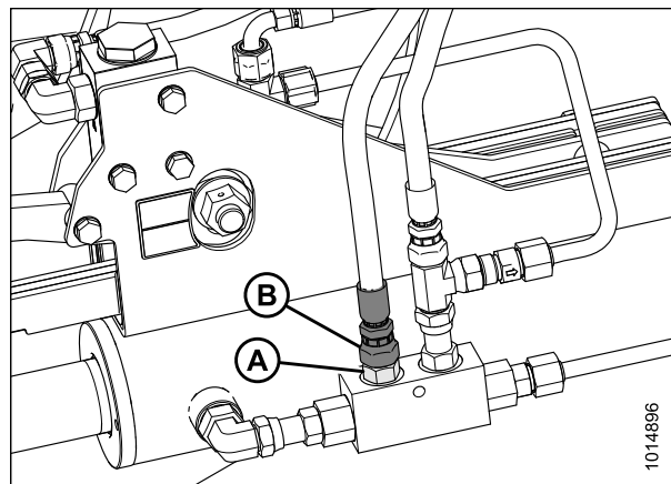
Figure 4.60: Alignement du raccord de vanne
