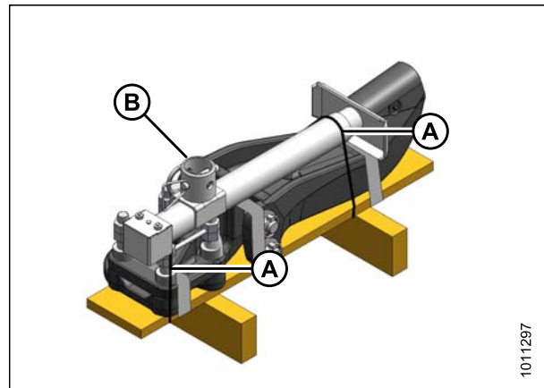
Figure 3.19: Emballage du cric et du crochet d'attelage
