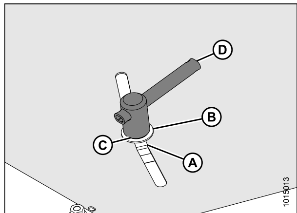
Figure 4.112: Réglage du déflecteur
