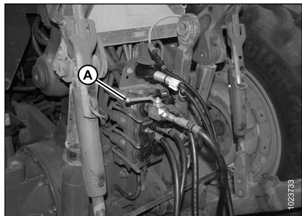
Figure 7.3: Clapet de verrouillage de rotation d'attelage montré en position fermée
