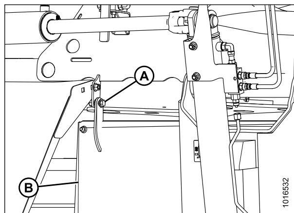
Figure 4.2: Blindage central (conditionneuses à peignes seulement)
