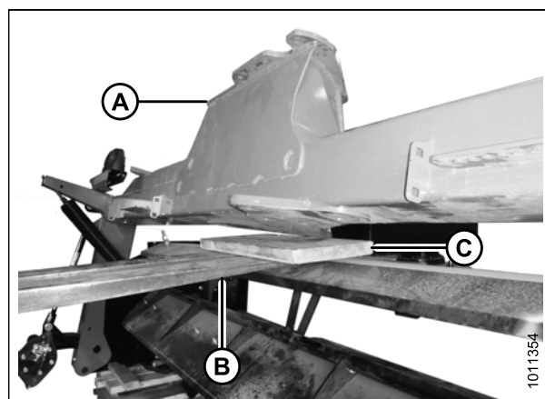
Figure 3.1: Châssis porteur
