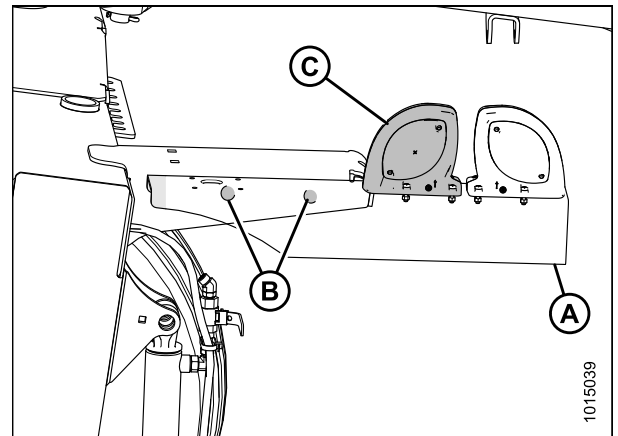
Figure 3.98: Côté gauche du véhicule
