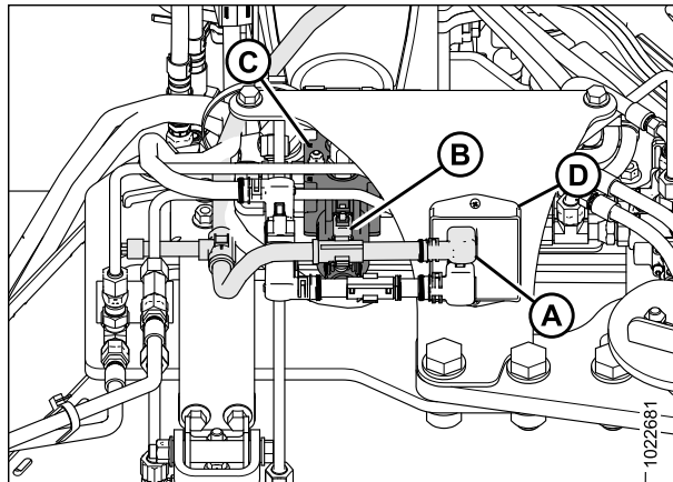
Figure 3.105: Alimentation de la vanne sélectrice
