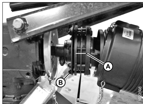
Figure 6.31: Transmission et boîte de vitesses
