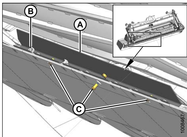
Figure 8.20: Déflecteur gauche de la barre de coupe vu du dessous de la barre de coupe
