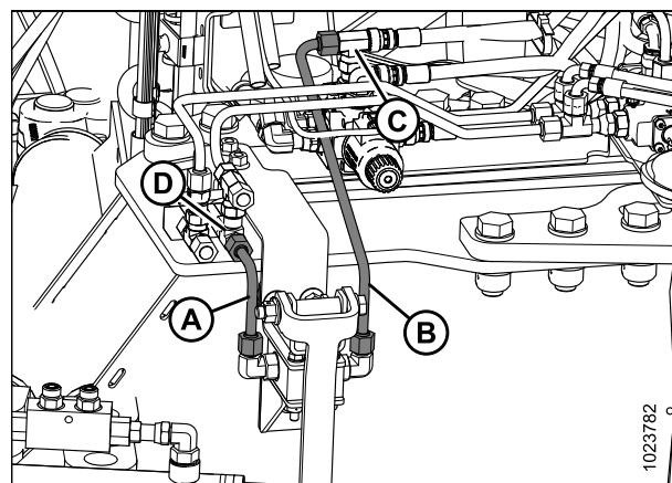
Figure 3.87: Tuyauterie du système d'assemblage final
