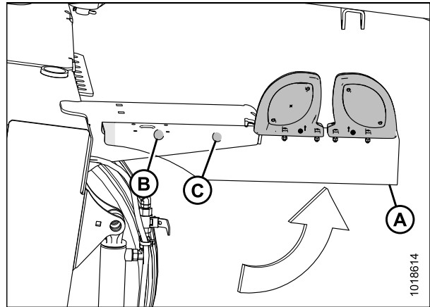
Figure 4.68: Gauche, extrémité arrière de la faucheuse
