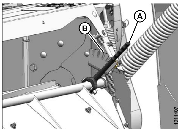
Figure 6.26: Dispositif de réglage de chicane (conditionneuses à rouleaux)
