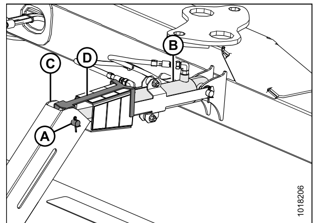
Figure 8.31: Vérin d'inclinaison et bielles de l'indicateur
