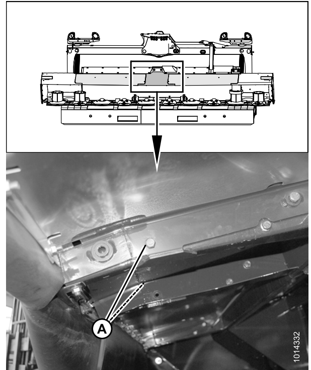
Figure 3.152: Dessous des portes de la barre de coupe
