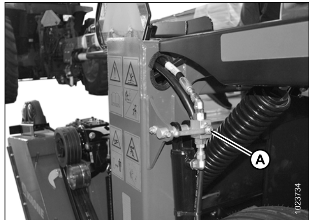
Figure 7.13: Clapet de verrouillage du vérin de levage
