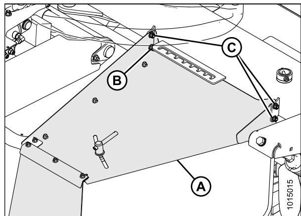
Figure 3.140: Blindages de formage (côté droit)
