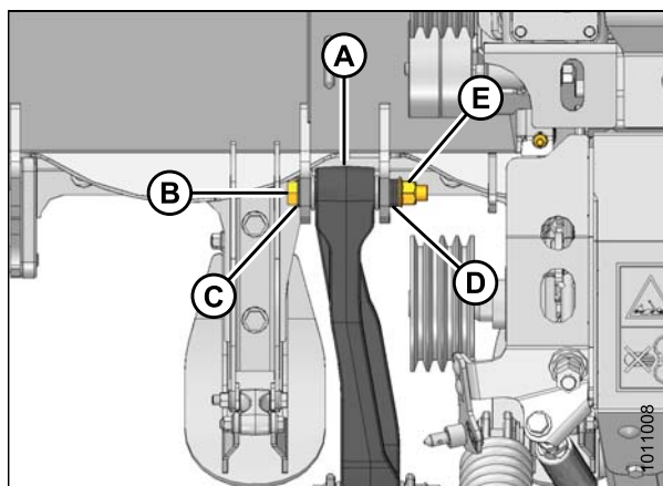
Figure 8.28: Montant gauche
