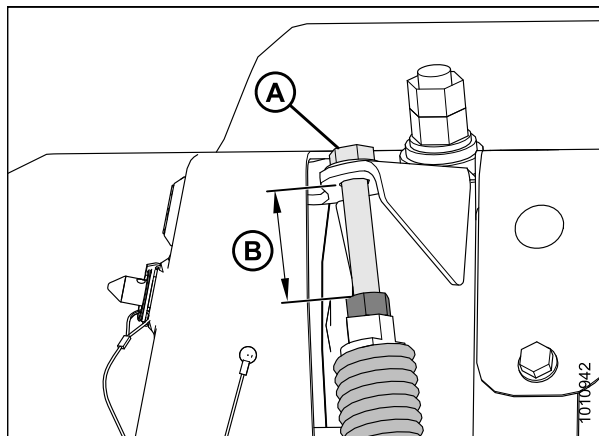
Figure 6.23: Dispositif de réglage de la tension des rouleaux
