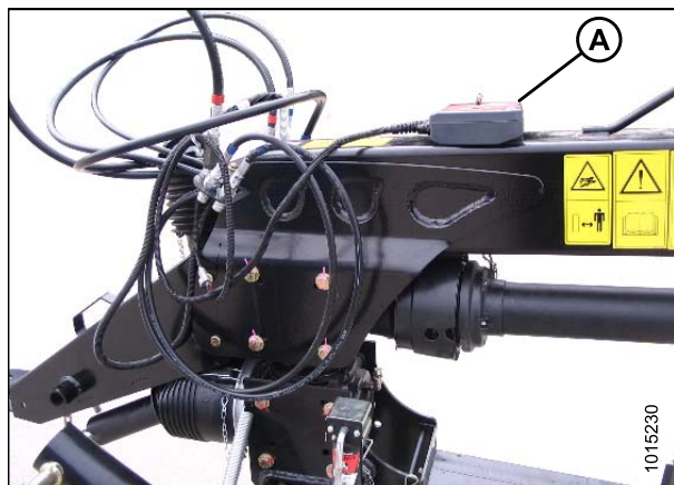
Figure 3.106: Contrôle à distance au-dessus de l'attelage
