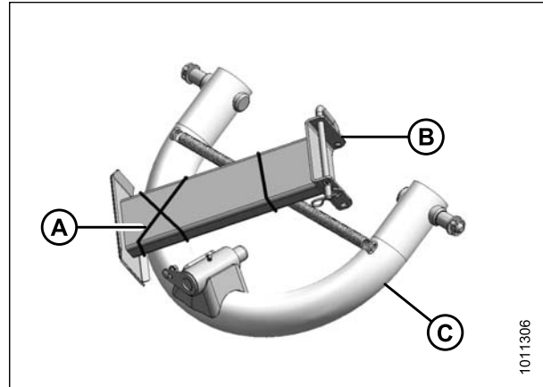
Figure 3.29: Emballage de l'attelage deux points
