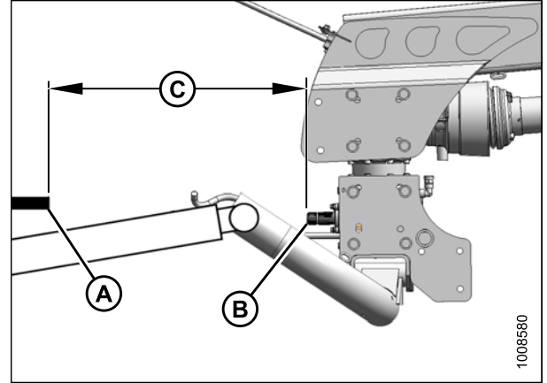
Figure 3.122: Longueur admissible de la transmission
