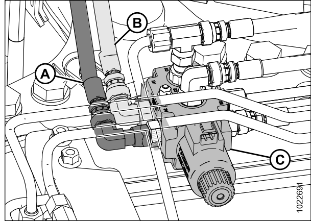
Figure 3.90: Alimentation de la vanne sélectrice
