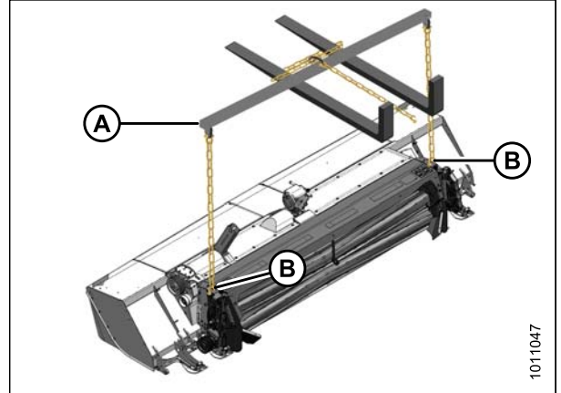
Figure 8.9: Barre d'écartement
