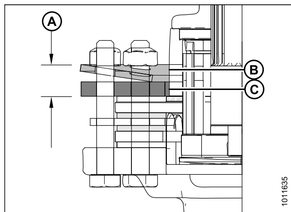
Figure 6.36: Mesure de réglage initiale
