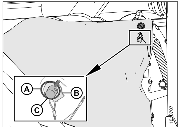
Figure 5.11: Blindage de la transmission de gauche
