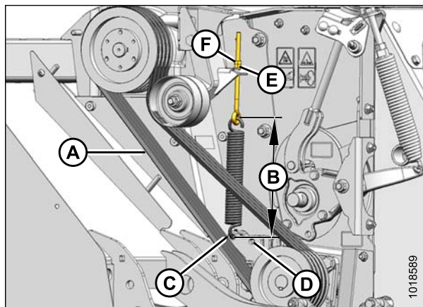
Figure 6.5: Courroie d'entraînement de la conditionneuse
