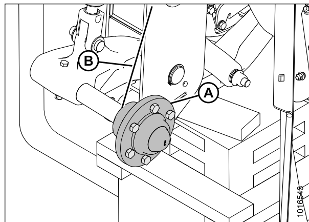
Figure 4.91: Fusée de la roue
