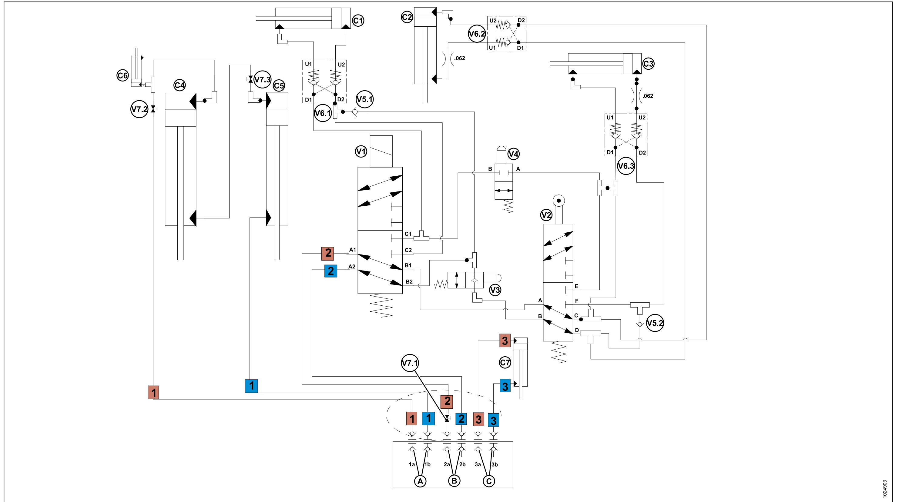
Figure 9.1: Schéma hydraulique – avec transport
