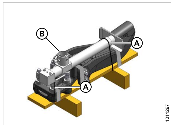
Figure 4.22: Emballage du cric et du crochet d'attelage
