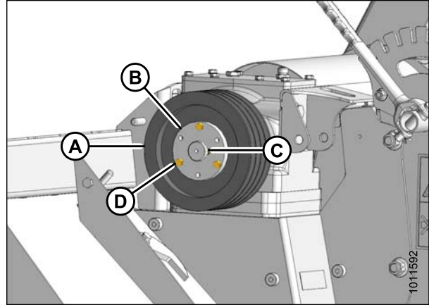
Figure 8.23: Poulie d'entraînement
