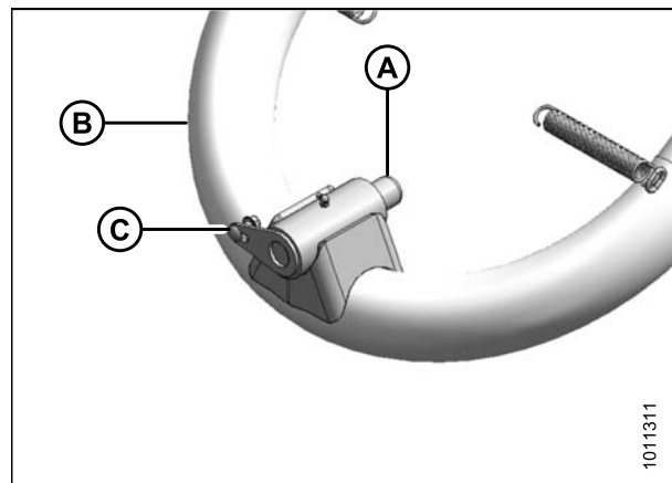
Figure 3.30: Adaptateur d'attelage deux points
