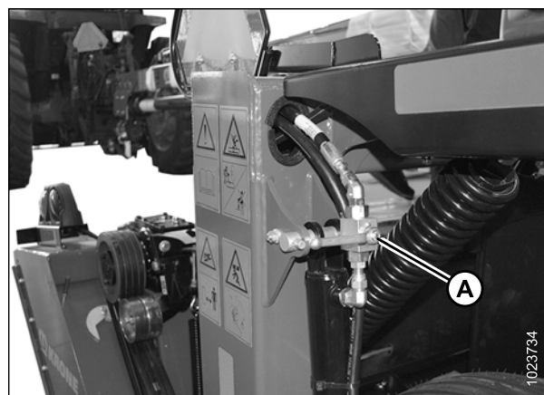
Figure 4.124: Clapets de verrouillage des vérins de levage
