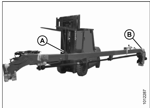
Figure 4.14: Levage de l'attelage
