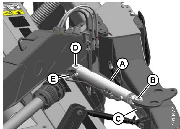
Figure 3.40: Vérin de rotation d'attelage
