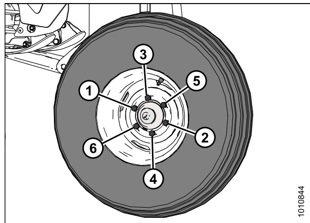
Figure 6.1: Séquence de serrage
