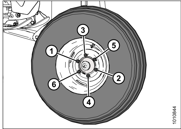
Figure 4.94: Séquence de serrage
