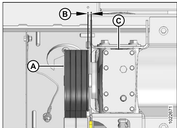
Figure 8.24: Poulie d'entraînement
