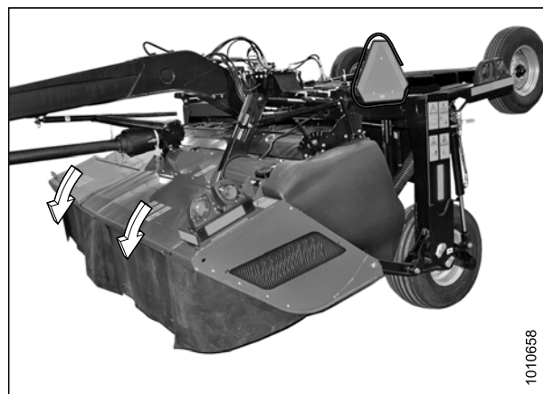
Figure 10.5: Faucheuse à disques de type tracté R113
