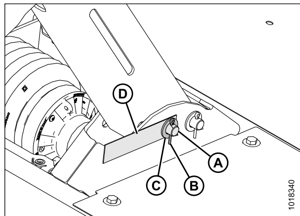
Figure 4.6: Ancre du vérin d'inclinaison (côté droit du vérin d'inclinaison)
