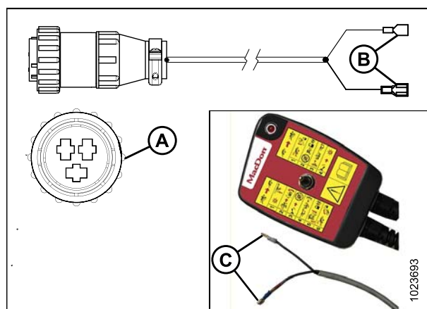
Figure 4.72: Connecteur auxiliaire à trois broches
