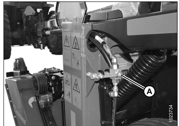
Figure 3.158: Clapets de verrouillage des vérins de levage
