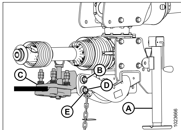
Figure 4.79: Attelage de la faucheuse à disques
