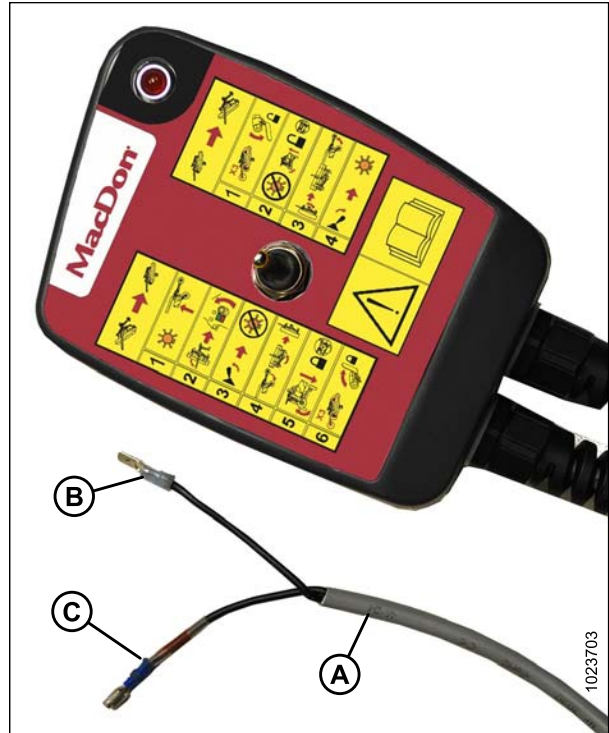
Figure 4.73: Commande à distance
