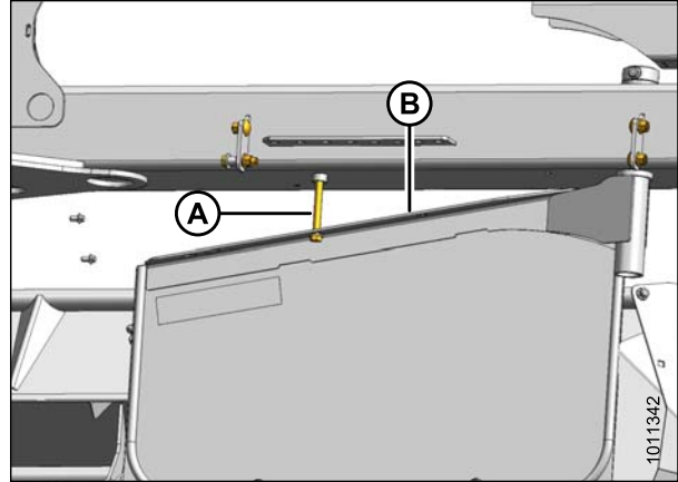
Figure 3.144: Ensemble du déflecteur latéral
