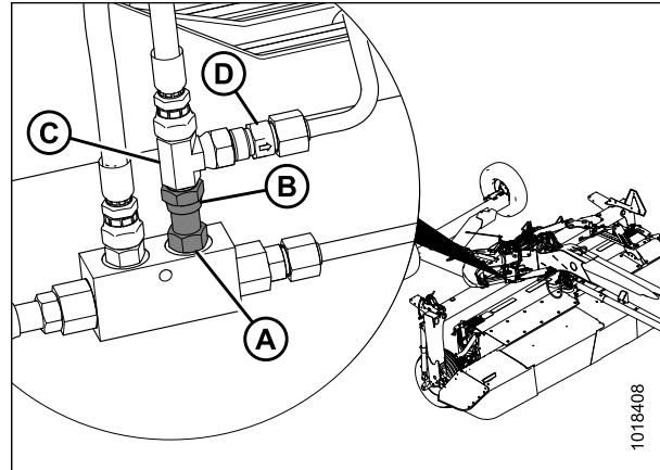
Figure 3.85: Alignement du raccord de vanne
