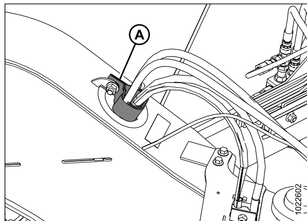
Figure 4.65: Arrière de l'attelage
