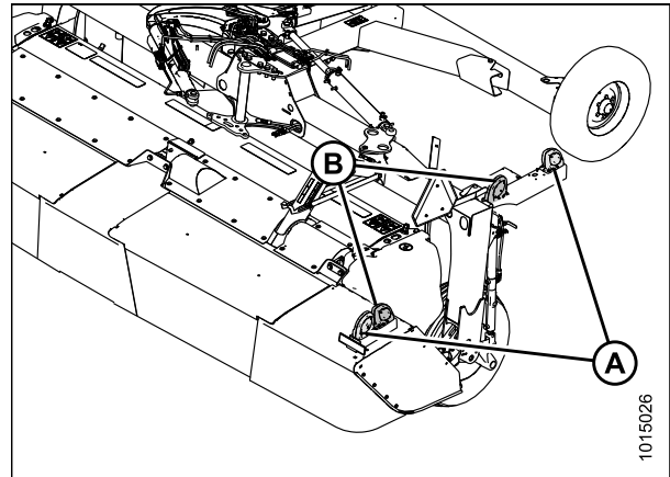
Figure 7.8: Emplacements d'éclairage (avec le Road Friendly Transport™ [système de transport routier])
