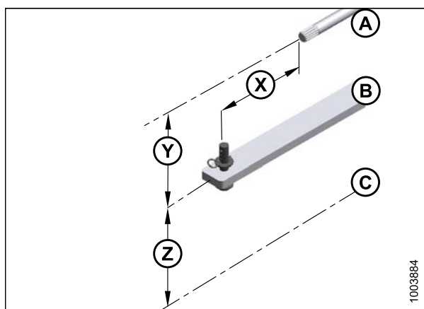
Figure 4.75: Réglages de la barre d'attelage du tracteur
