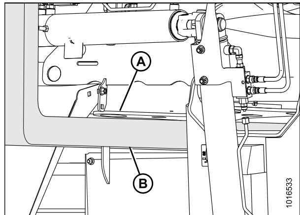
Figure 4.4: Châssis porteur
