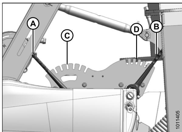
Figure 6.25: Dispositifs de réglage de chicane (conditionneuses à peignes)
