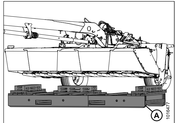
Figure 3.169: Retrait de la palette d'expédition
