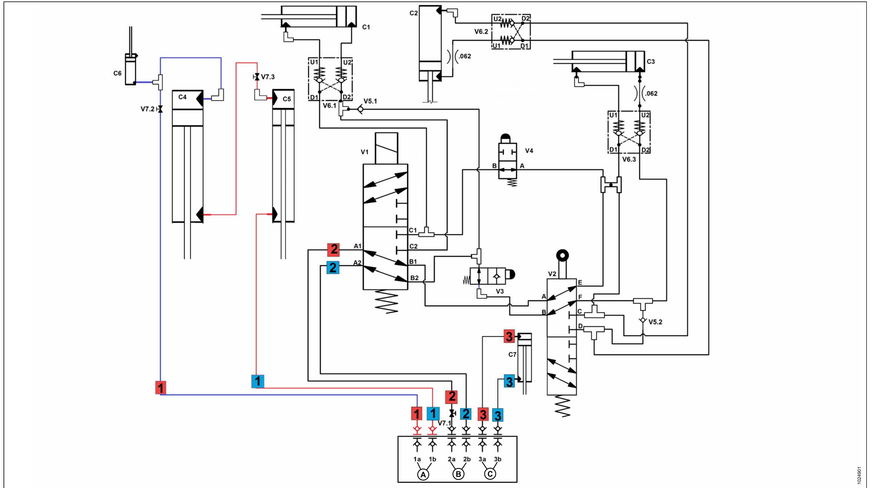
Figure 9.7: Schéma hydraulique – Verrouillage pour le transport de la plateforme
