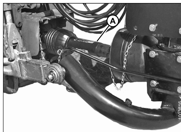
Figure 4.85: Transmission de la faucheuse à disques fixée à la PF du tracteur
