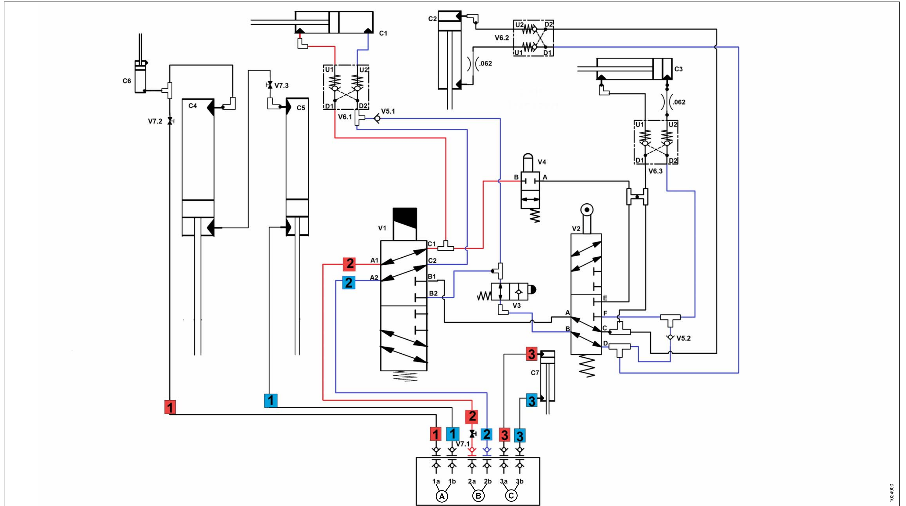
Figure 9.3: Schéma hydraulique – Rotation de plateforme
