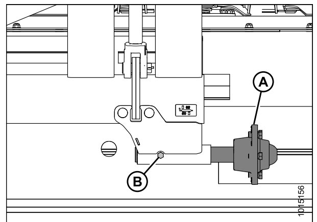
Figure 4.100: Relocalisation de l'ensemble de l'essieu
