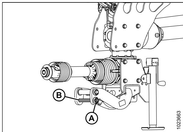
Figure 4.77: Attelage de la faucheuse à disques
