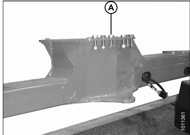
Figure 3.8: Châssis porteur
