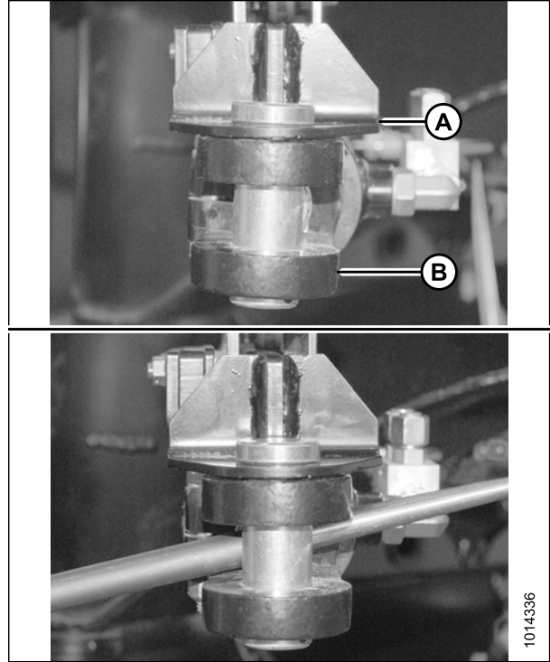
Figure 4.58: Alignement du bras de came
