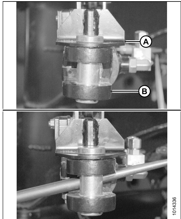
Figure 3.82: Alignement du bras de came
