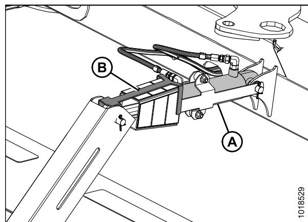
Figure 6.6: Vérin d'inclinaison hydraulique
