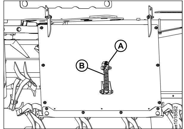
Figure 3.141: Ressort sur le blindage central
