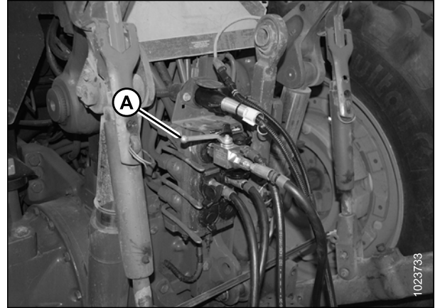
Figure 7.23: Vanne de verrouillage de la direction
