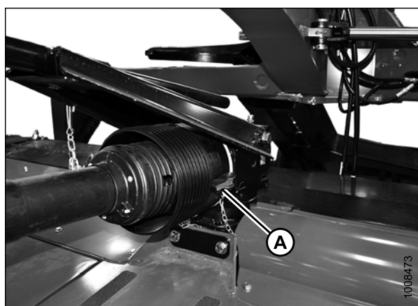
Figure 6.33: Cône de protection de la transmission
