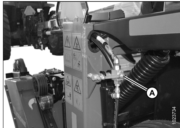
Figure 10.3: Clapet de verrouillage du vérin de levage
