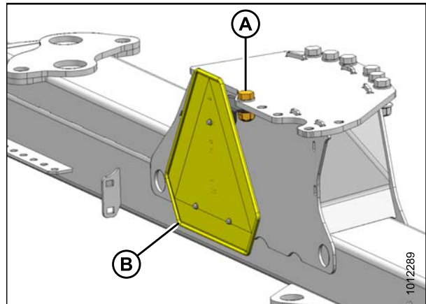
Figure 3.58: Panneau VLM fixé au châssis porteur
