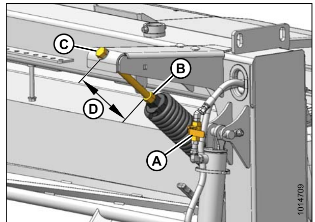
Figure 3.7: Clapet de verrouillage du vérin de levage, contre-écrou et boulon de réglage
