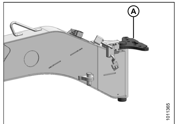
Figure 3.12: Broche d'attelage
