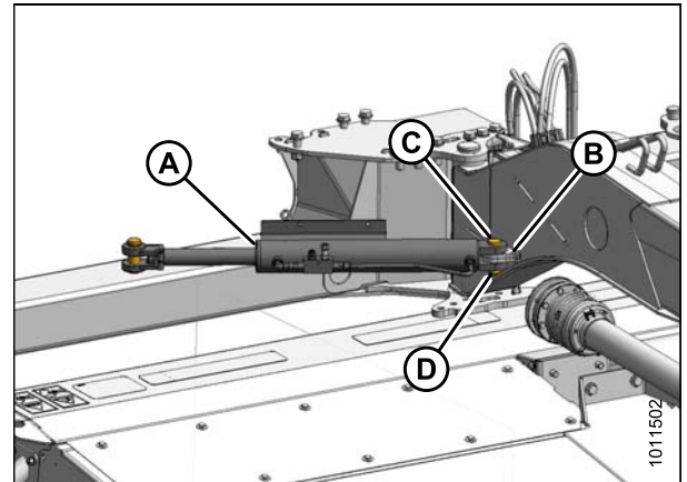
Figure 3.41: Vérin de rotation d'attelage
