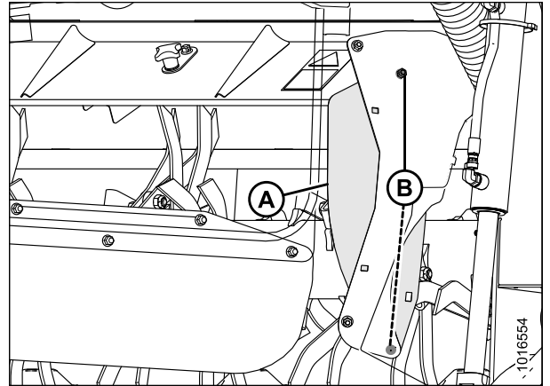
Figure 3.147: Blindage du déflecteur de droite illustré – Blindage du déflecteur de gauche opposé
