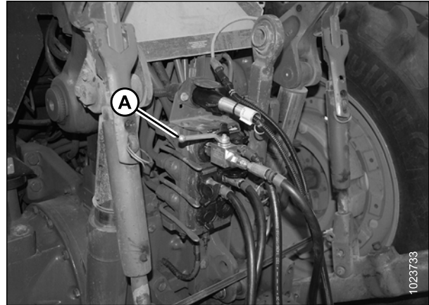
Figure 7.12: Vanne de verrouillage de la direction
