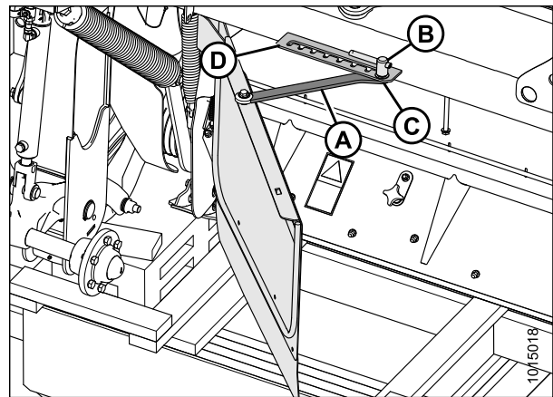
Figure 3.151: Barre de réglage
