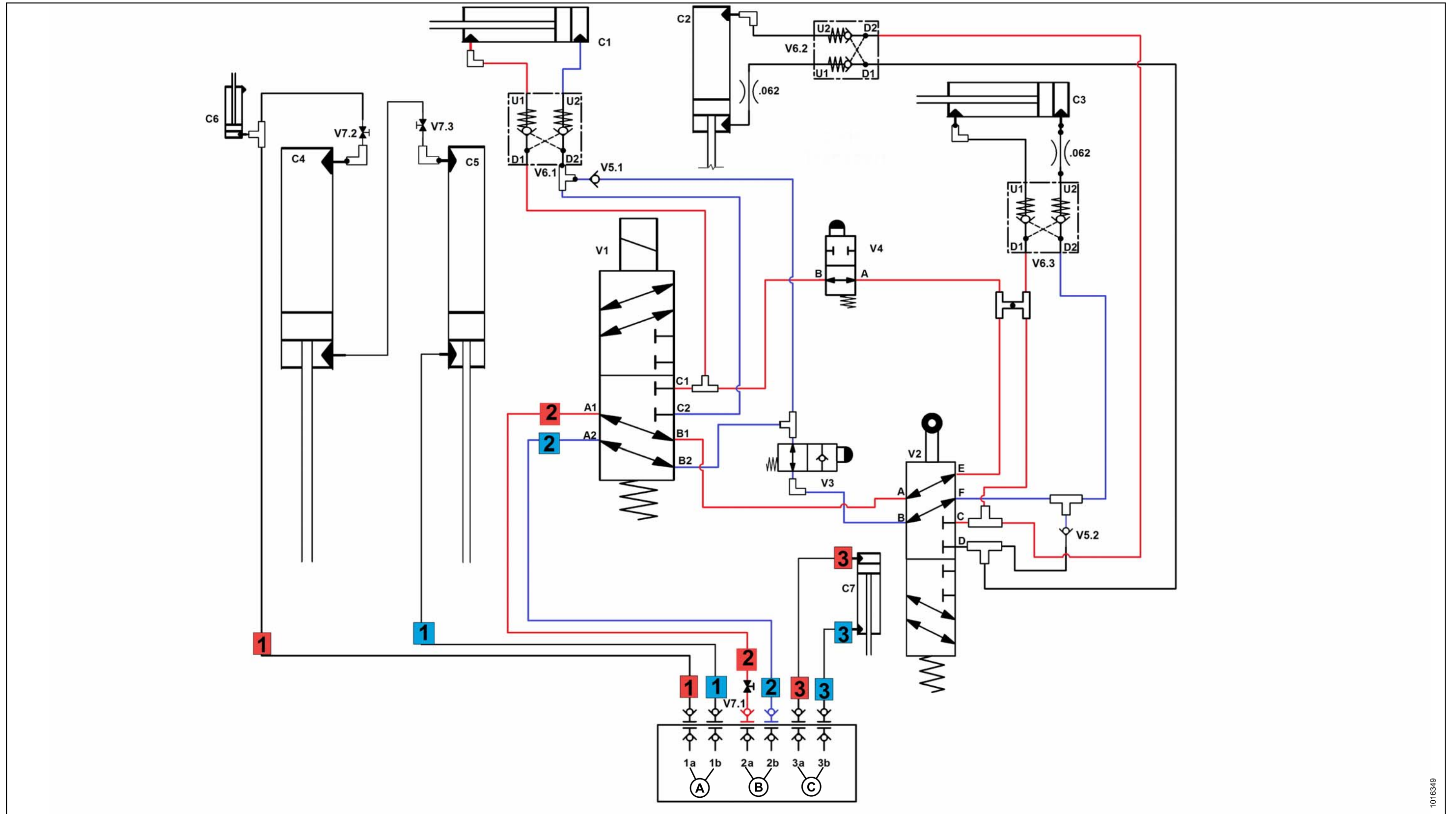
Figure 9.6: Schéma hydraulique – Rotation complète pour le transport de la plateforme
