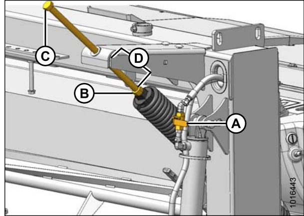
Figure 8.2: Régleur de flottement du côté droit – Côté gauche similaire
