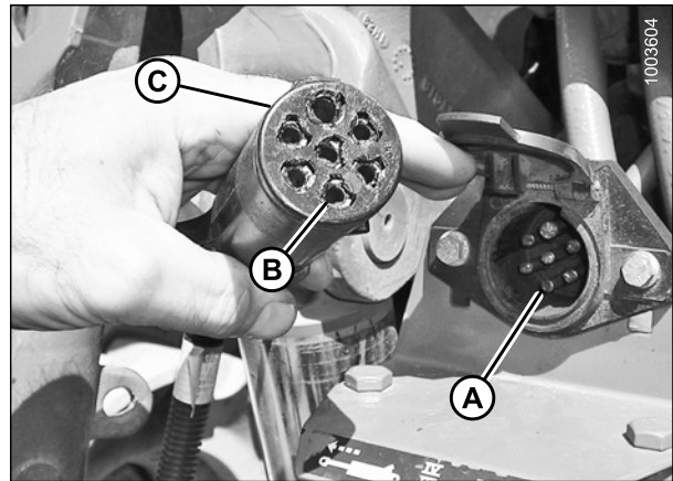
Figure 4.90: Faisceau de câblage électrique et prise femelle
