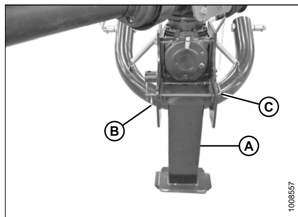
Figure 4.86: Chandelle d'attelage
