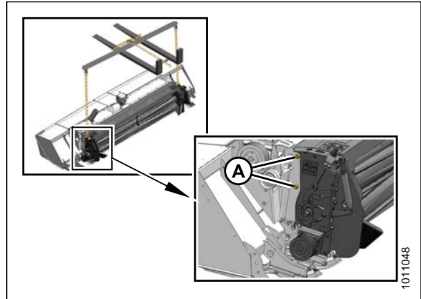
Figure 8.12: Côté gauche de la conditionneuse – Côté droit similaire
