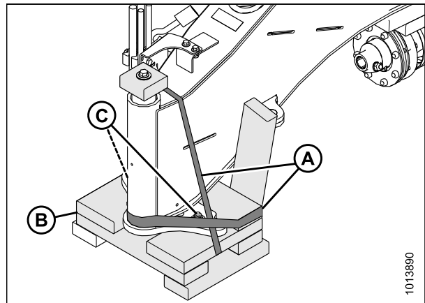
Figure 3.9: Emballage de l'attelage
