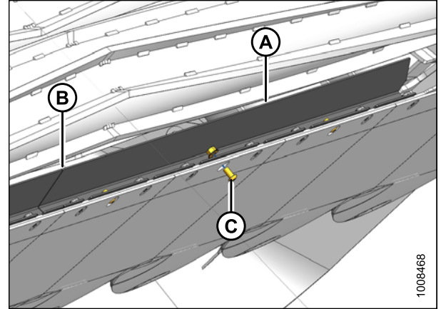
Figure 8.21: Déflecteur droit de la barre de coupe vu du dessous de la barre de coupe
