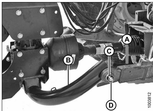
Figure 4.83: Configuration de l'attelage deux points
