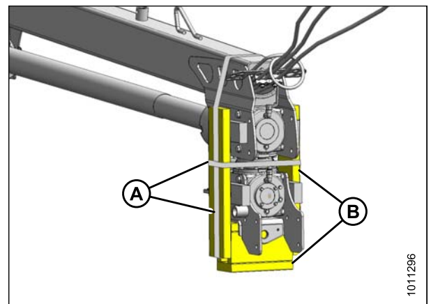
Figure 3.28: Emballage de l'attelage
