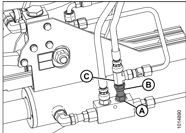
Figure 4.59: Alignement du raccord de vanne
