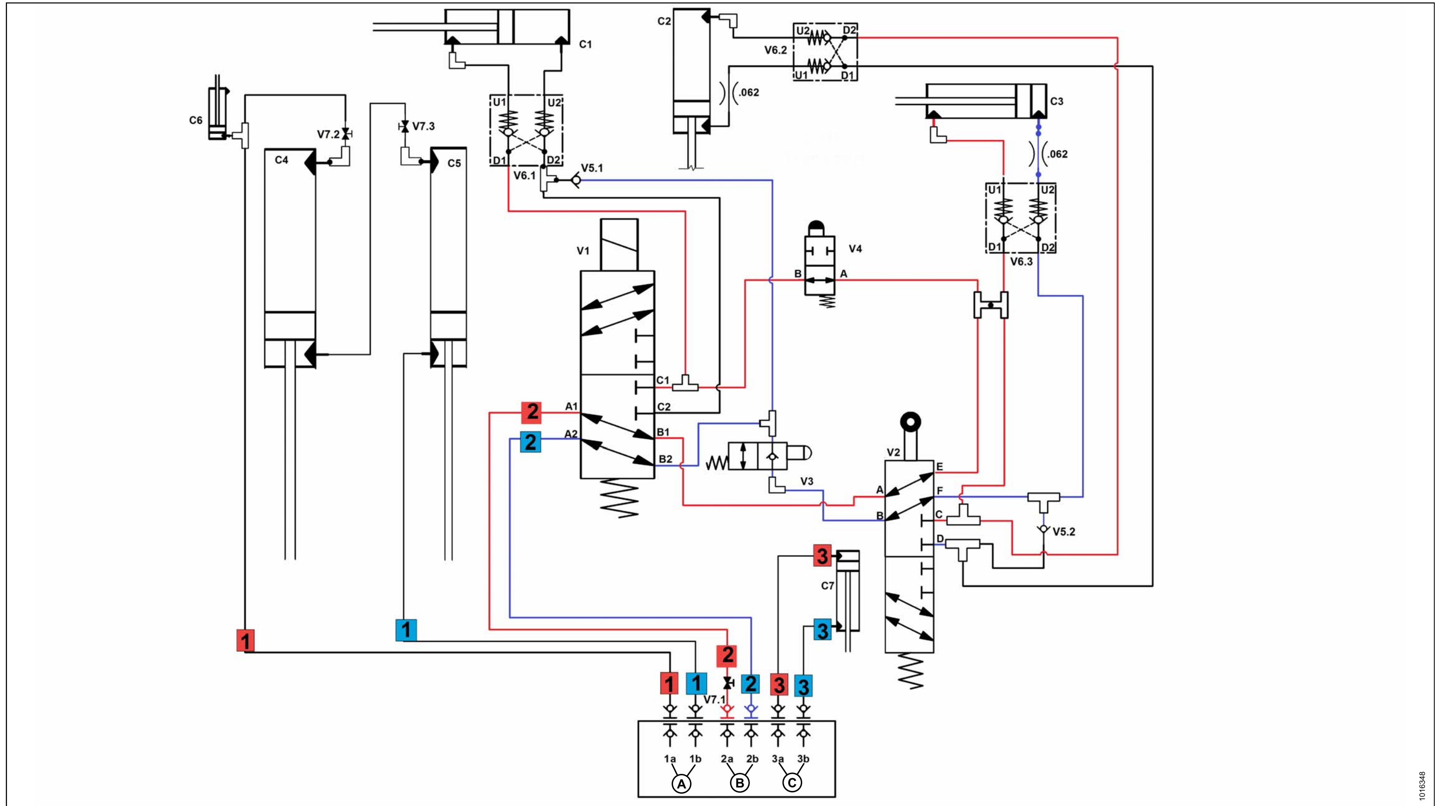
Figure 9.5: Schéma hydraulique – Rotation pour le transport de la plateforme
