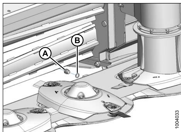
Figure 6.18: Barre de coupe
