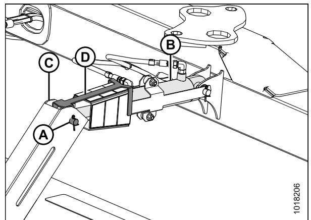
Figure 8.7: Vérin d'inclinaison et indicateur
