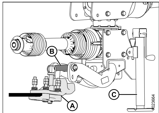
Figure 3.116: Attelage de la faucheuse à disques
