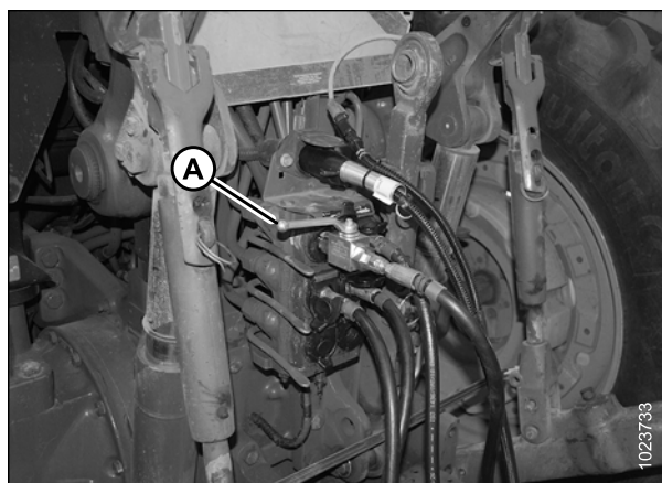
Figure 6.49: Vanne de verrouillage de la direction
