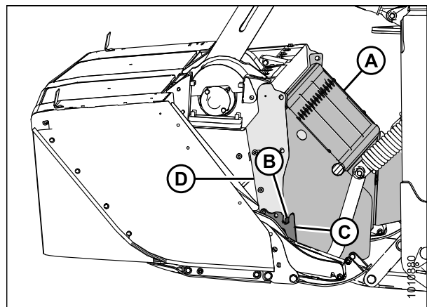
Figure 3.160: Vue latérale de la plateforme
