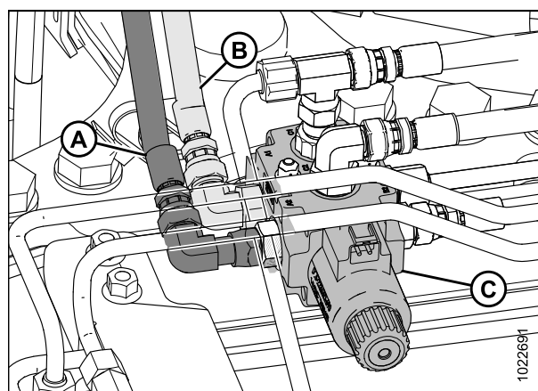
Figure 4.61: Alimentation de la vanne sélectrice
