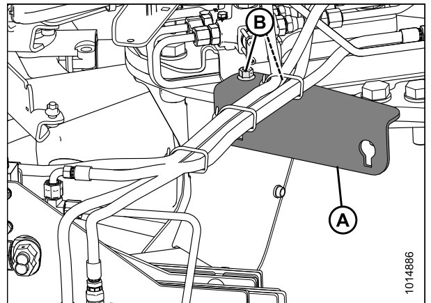
Figure 4.11: Support d'expédition (vue de face, à droite)
