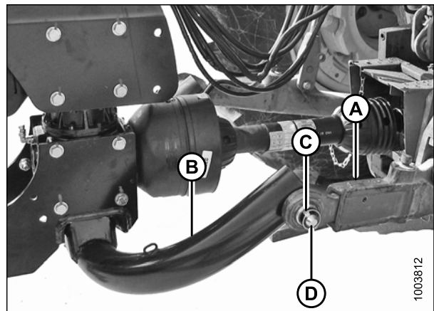
Figure 3.121: Configuration de l'attelage deux points
