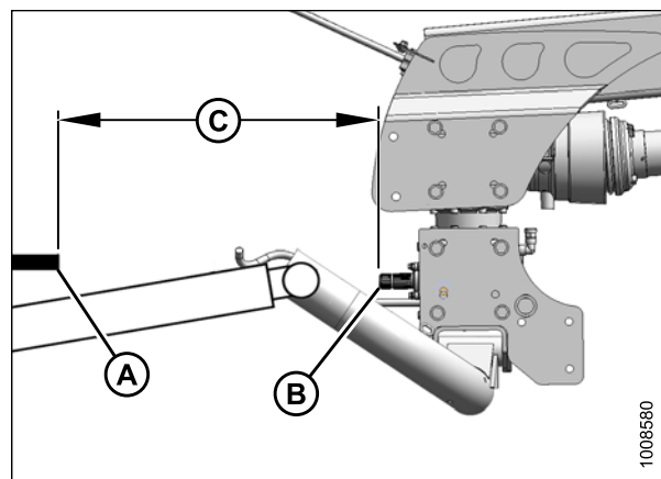
Figure 4.84: Longueur admissible de la transmission
