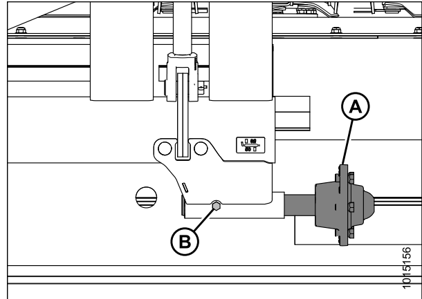
Figure 3.75: Relocalisation de l'ensemble de l'essieu
