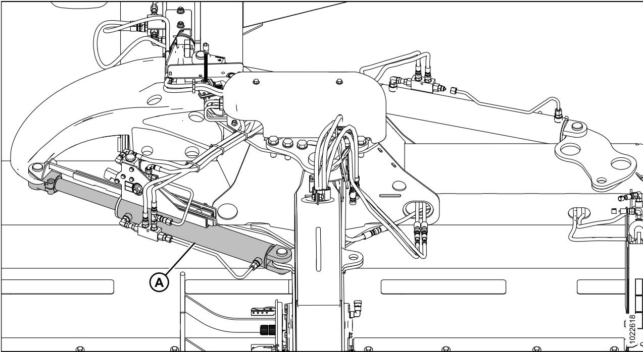
Figure 4.96: Système hydraulique
