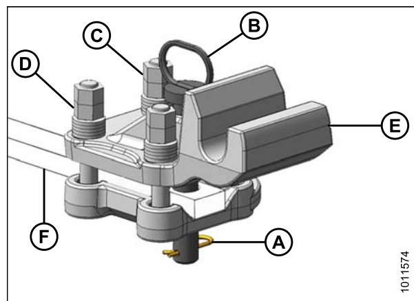
Figure 4.76: Adaptateur du crochet d'attelage
