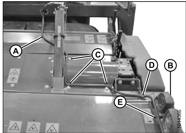
Figure 8.33: Faisceau électrique
