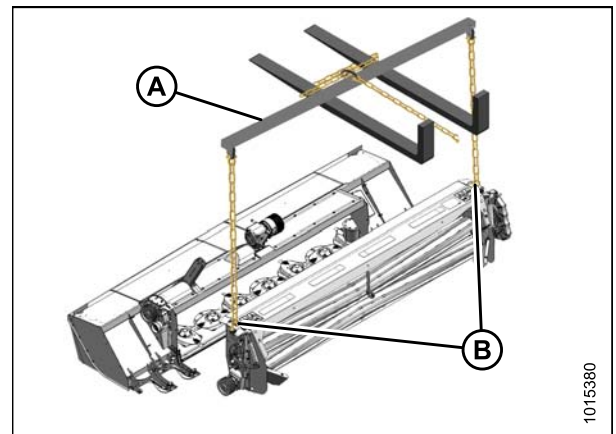
Figure 8.17: Levage de la conditionneuse
