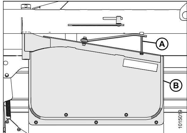
Figure 4.116: Blindage de formage du côté gauche
