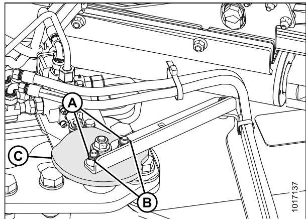
Figure 6.40: Ensemble du mécanisme de déploiement/rotation du transport
