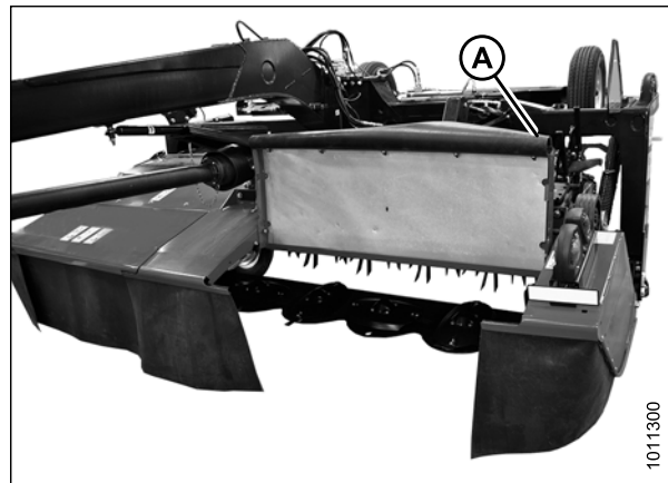
Figure 10.4: Côté gauche de la porte de la barre de coupe en position ouverte
