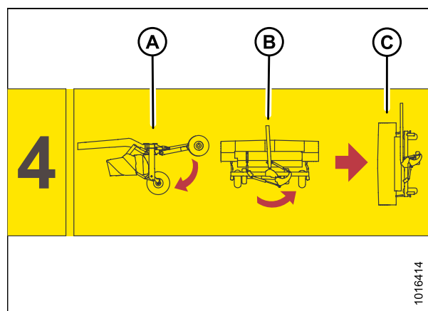
Figure 6.46: Rotation de l'ensemble de transport
