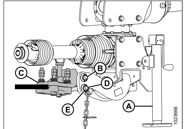
Figure 3.117: Attelage de la faucheuse à disques
