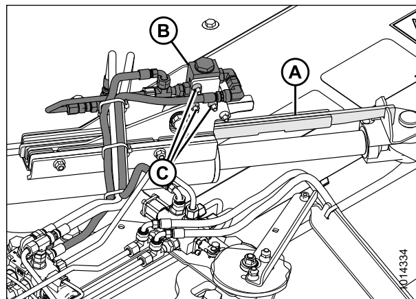
Figure 4.56: Contrôle d'alignement (vue de l'arrière, à droite)
