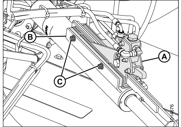
Figure 3.78: Contrôle d'alignement (vue de l'arrière, à droite)
