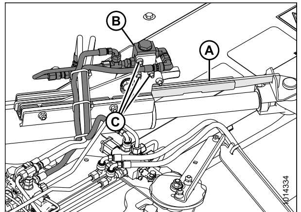
Figure 3.80: Contrôle d'alignement (vue de l'arrière, à droite)
