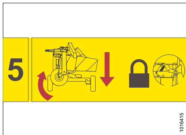
Figure 6.47: Abaissement de l'ensemble de transport
