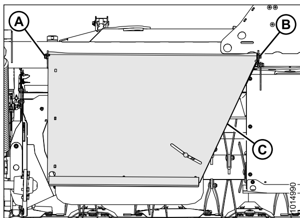
Figure 4.104: Capot supérieur extérieur
