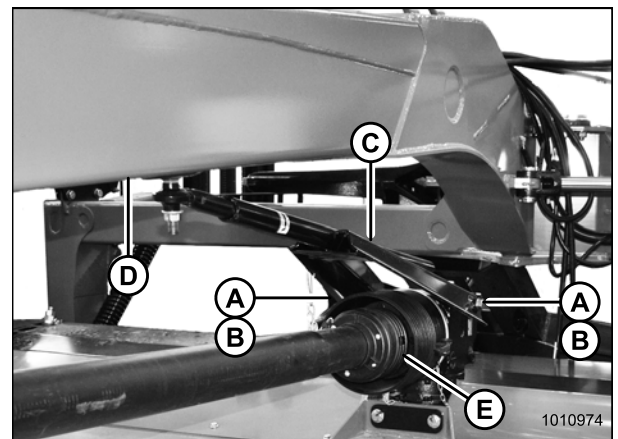
Figure 8.30: Transmission arrière et bras de direction
