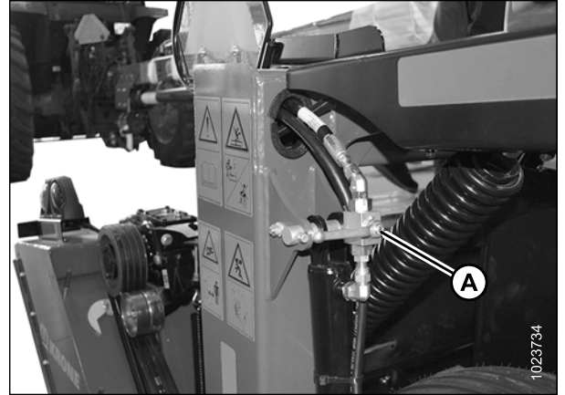
Figure 7.4: Clapet de verrouillage du vérin
