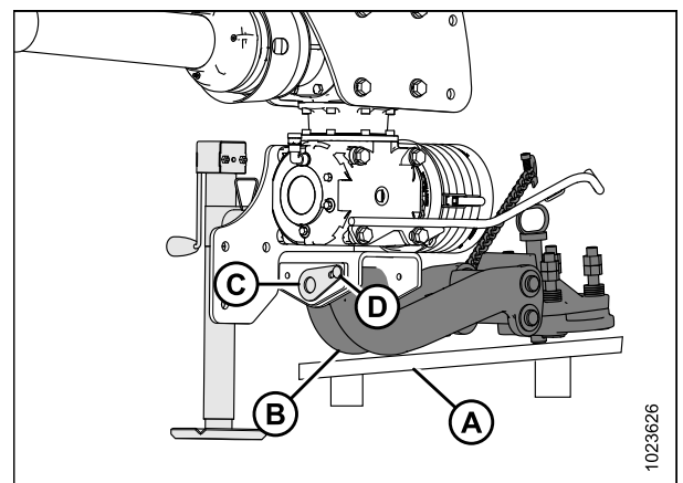
Figure 3.22: Crochet d'attelage
