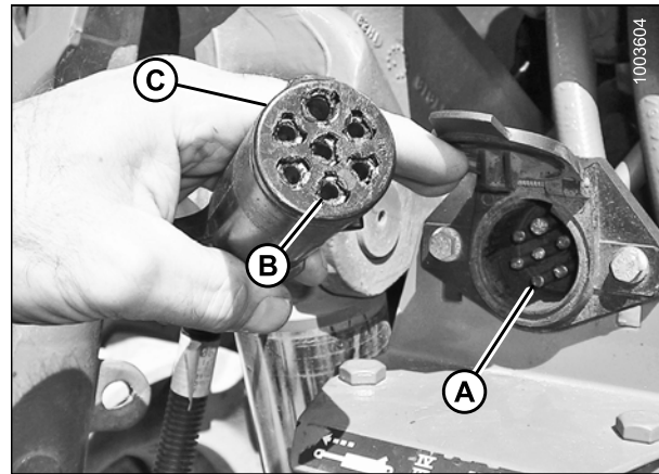
Figure 3.128: Faisceau de câblage électrique et prise femelle
