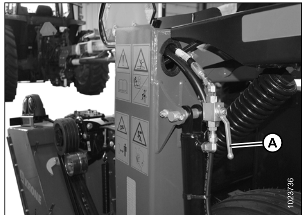
Figure 3.167: Clapets de verrouillage des vérins de levage
