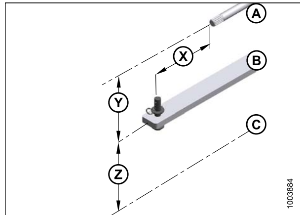
Figure 3.113: Réglages de la barre d'attelage du tracteur
