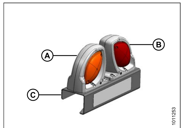
Figure 3.99: Système d'éclairage
