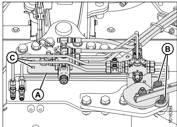
Figure 3.65: Valve sélectrice
