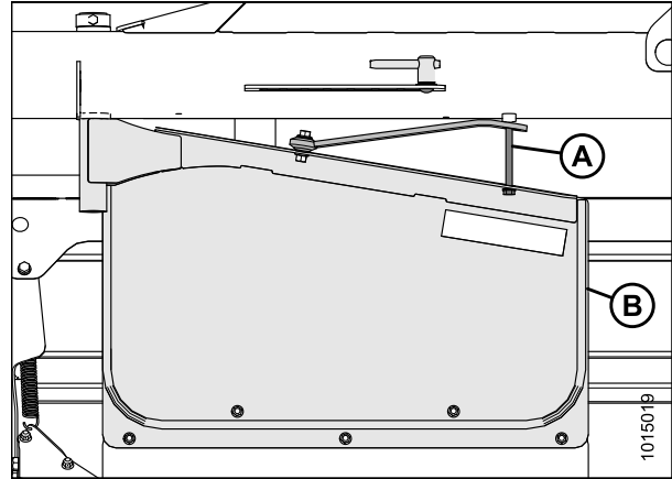
Figure 3.150: Blindage de formage du côté gauche
