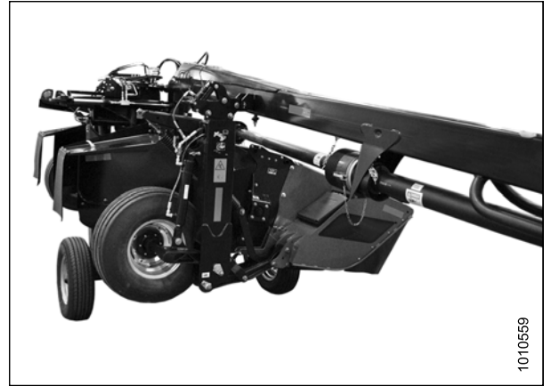
Figure 7.14: Road Friendly Transport™ (système de transport routier) Système
