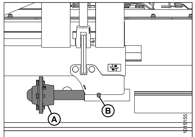
Figure 3.74: Relocalisation de l'ensemble de l'essieu
