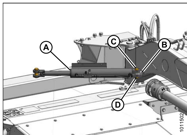
Figure 4.43: Vérin de rotation d'attelage
