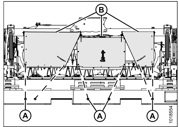
Figure 3.136: Blindages de formage cerclés à la palette
