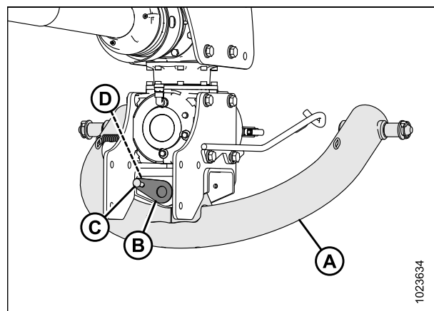
Figure 3.31: Adaptateur d'attelage deux points
