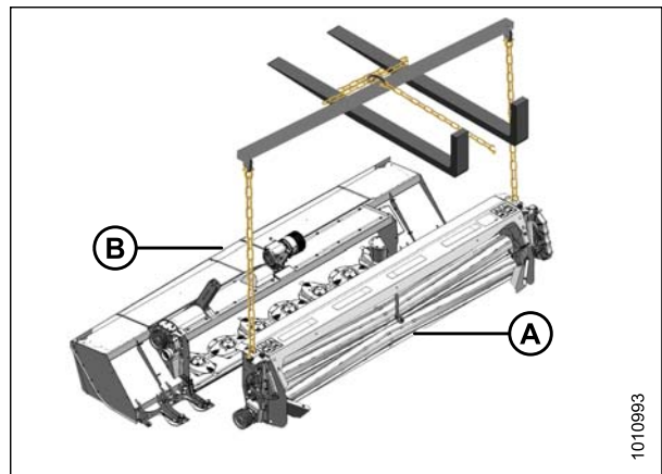
Figure 8.14: Levage de la conditionneuse
