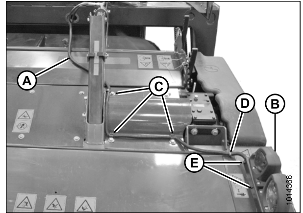
Figure 3.103: Routage du faisceau R113 représenté (identique à R116)
