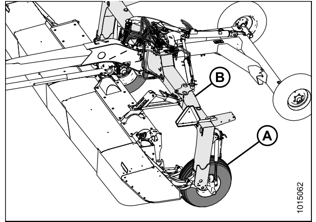
Figure 4.128: Faucheuse à disques avec transport
