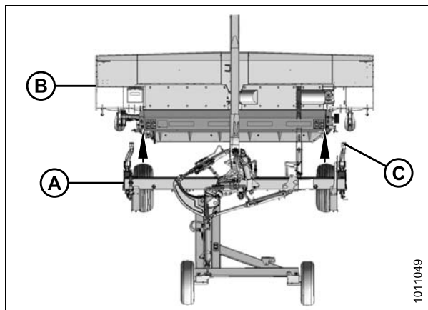
Figure 8.27: Châssis porteur aligné avec la plateforme
