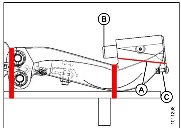
Figure 3.21: Moulage de l'attelage
