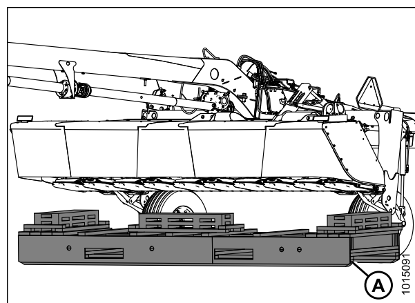
Figure 4.135: Retrait de la palette d'expédition
