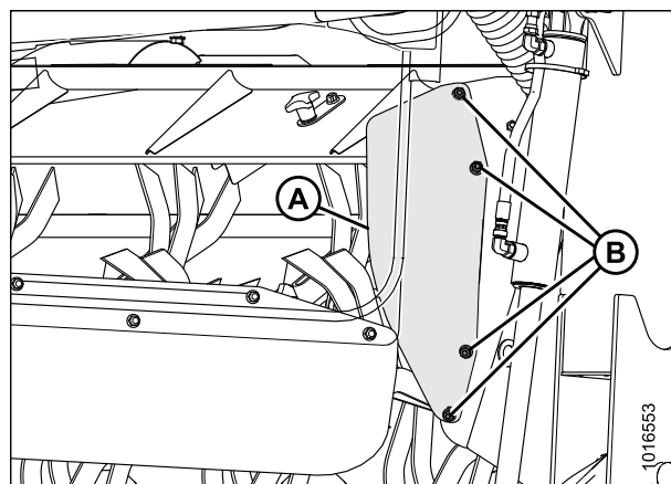
Figure 4.114: Blindage du déflecteur de droite illustré – Blindage du déflecteur de gauche opposé
