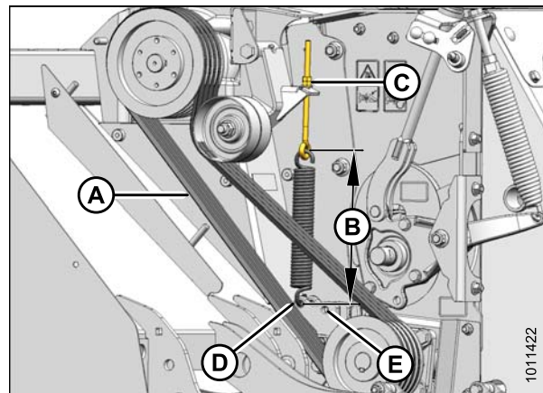
Figure 6.4: Courroie d'entraînement de la conditionneuse
