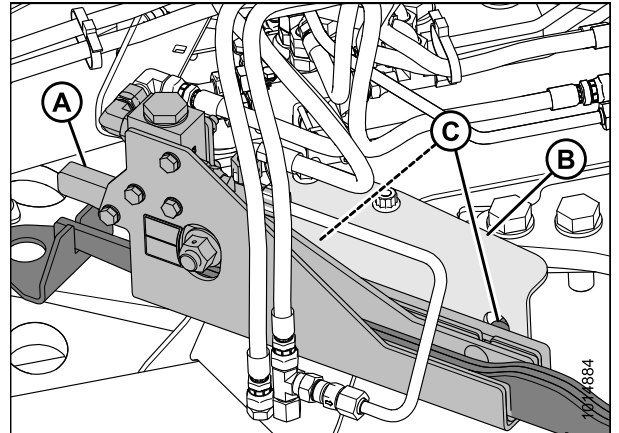
Figure 4.10: Contrôles d'alignement (vue de face, à droite)
