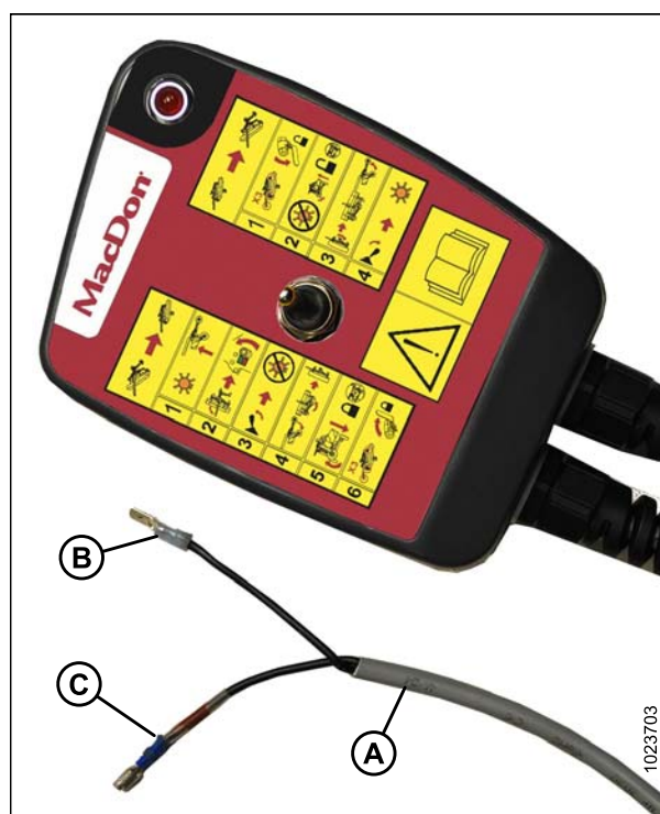
Figure 3.109: Commande à distance
