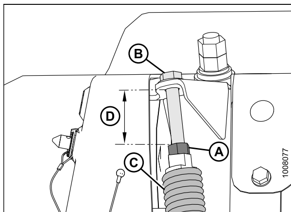
Figure 6.24: Côté gauche visible – Côté droit à l'opposé
