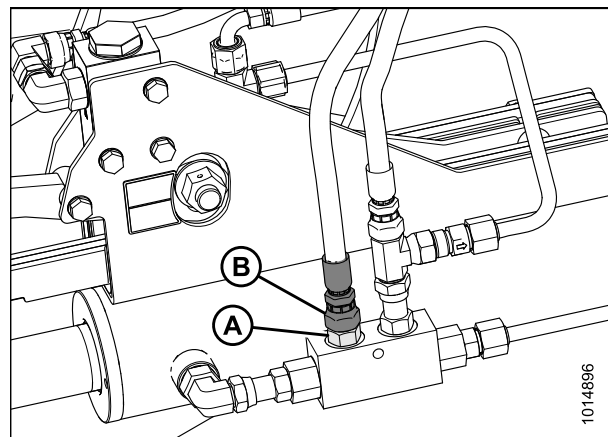
Figure 3.86: Alignement du raccord de vanne
