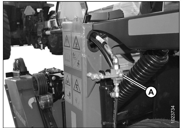
Figure 4.129: Clapets de verrouillage des vérins de levage
