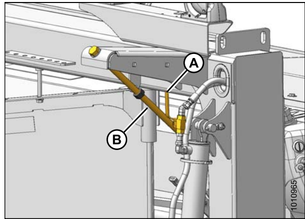
Figure 8.3: Régleur de flottement côté droit – Côté gauche similaire
