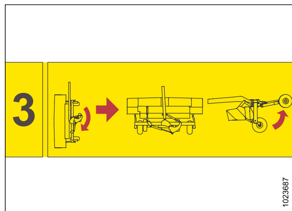
Figure 6.59: Rotation de la faucheuse à disques
