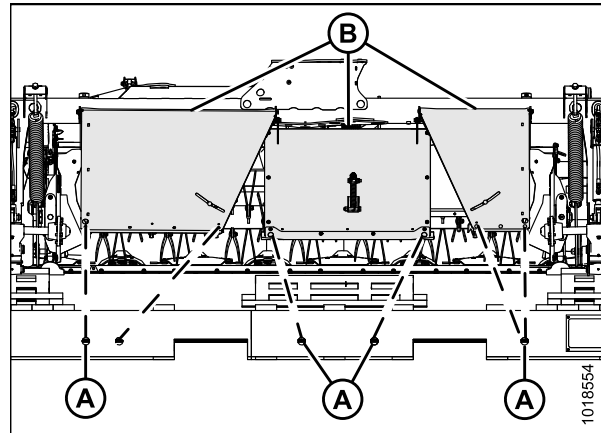
Figure 4.103: Cerclage de la plateforme
