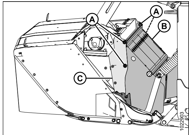
Figure 4.132: Côté gauche de la plateforme (côté droit opposé)
