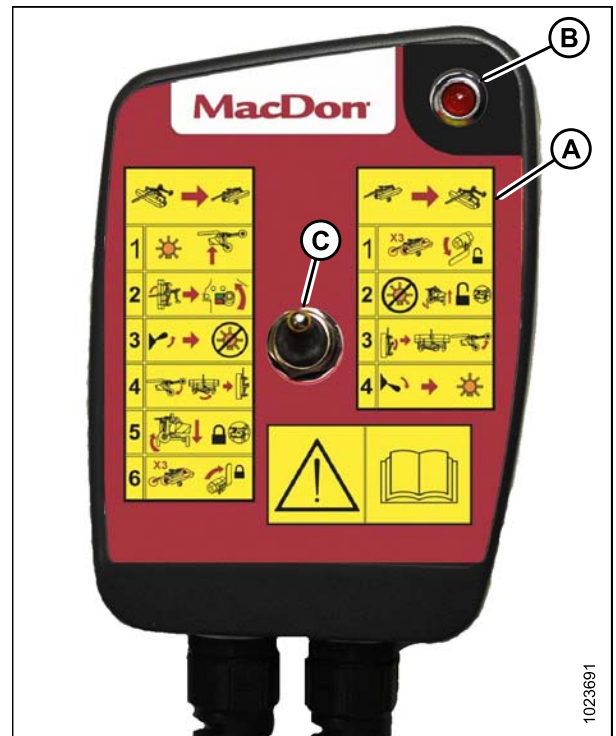
Figure 7.28: Commande à distance
