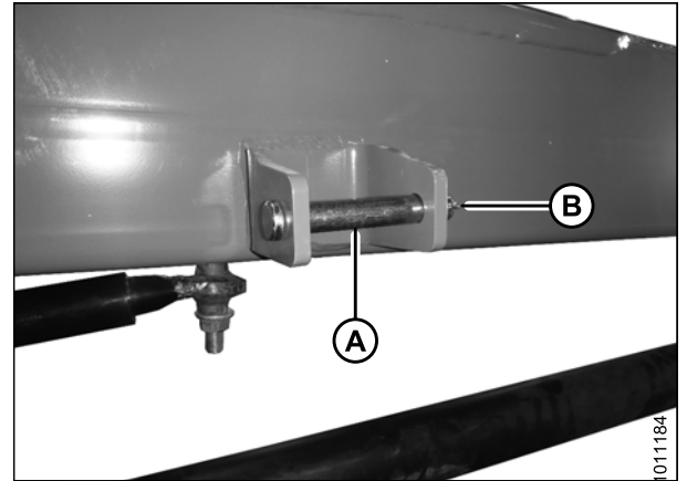
Figure 4.98: Axe de verrouillage
