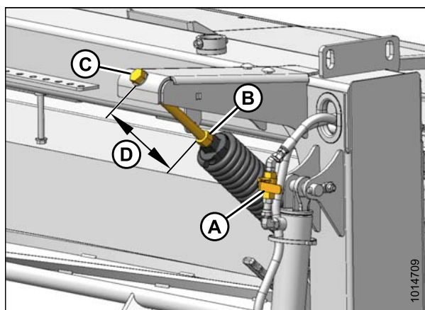
Figure 6.11: Clapet de verrouillage du vérin de levage, contre-écrou et boulon de réglage
