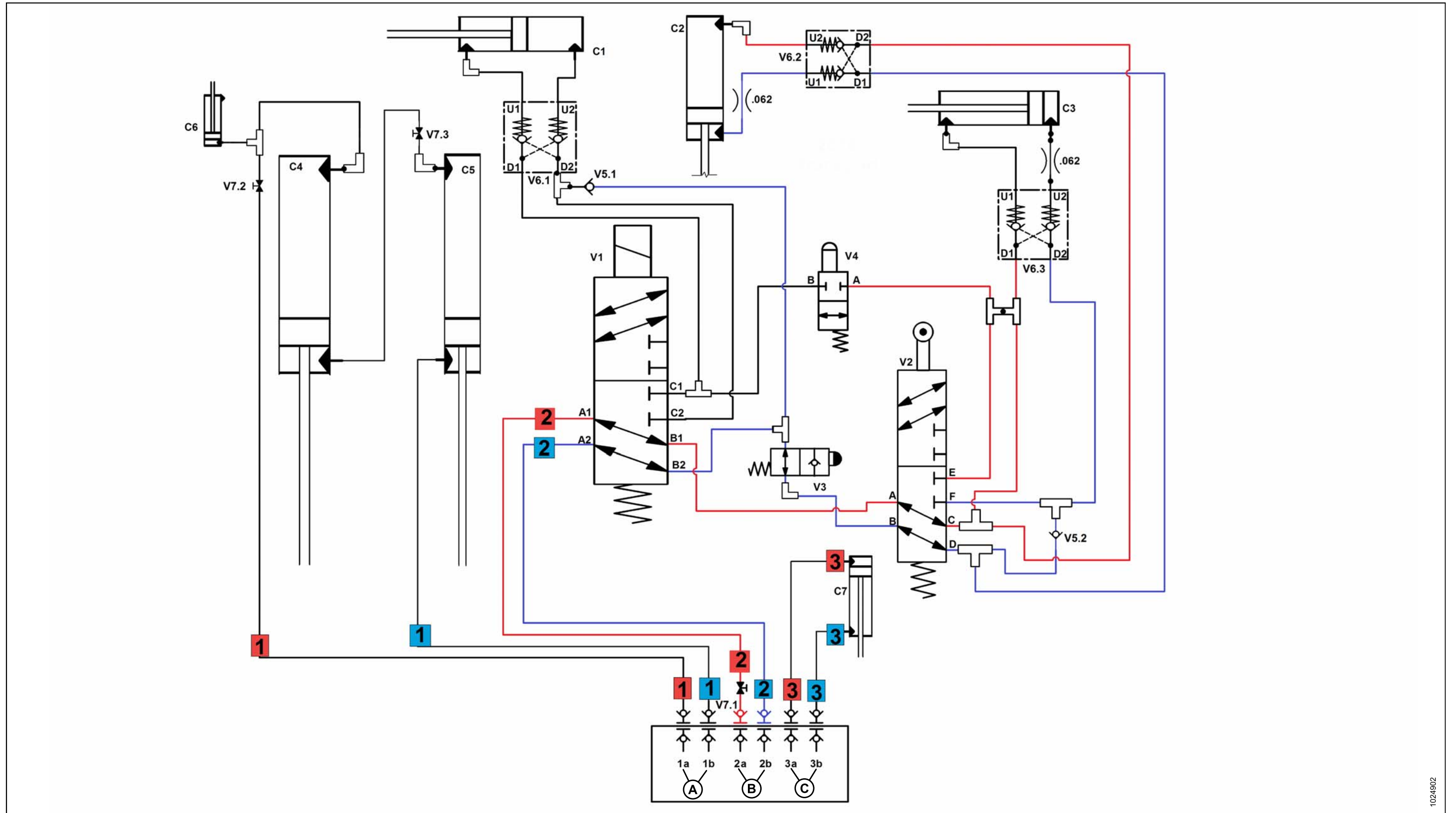
Figure 9.4: Schéma hydraulique – Déploiement pour le transport de la plateforme
