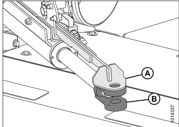
Figure 3.81: Contrôle d'alignement (vue de l'arrière, à droite)
