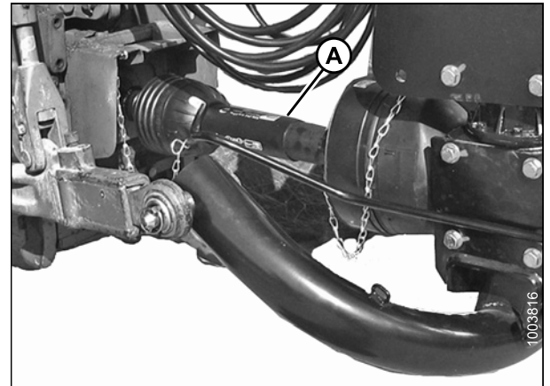
Figure 3.123: Transmission de la faucheuse à disques fixée à la PF du tracteur
