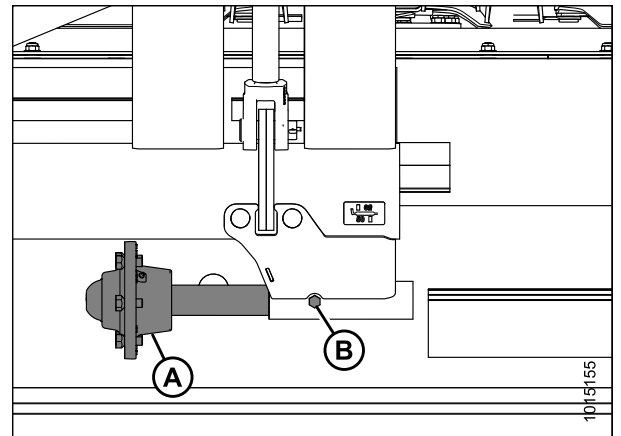
Figure 4.99: Relocalisation de l'ensemble de l'essieu
