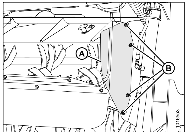
Figure 3.148: Blindage du déflecteur de droite illustré – Blindage du déflecteur de gauche opposé
