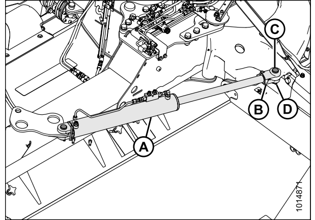
Figure 3.72: Vérin de rotation (vue arrière gauche)
