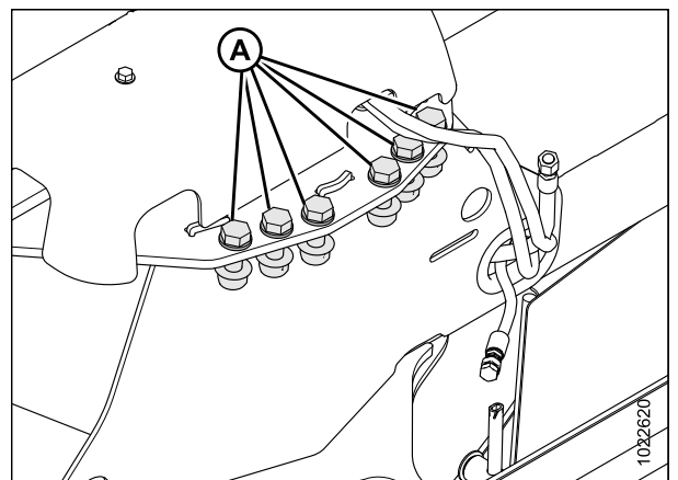
Figure 4.12: Châssis porteur
