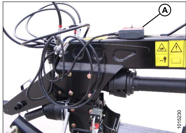
Figure 4.70: Contrôle à distance au-dessus de l'attelage
