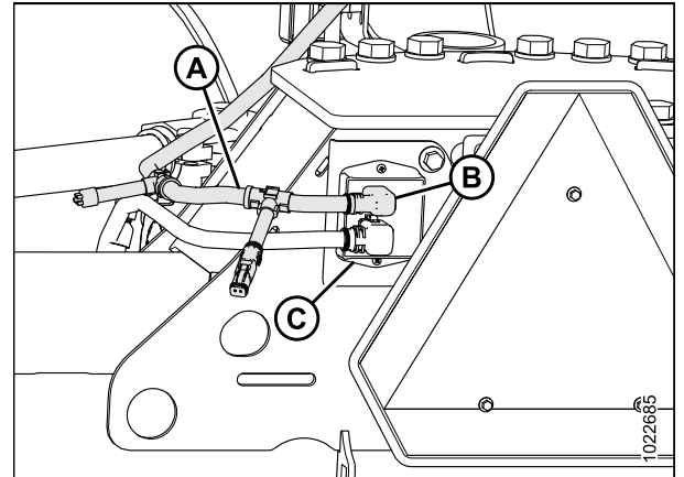
Figure 3.51: Faisceau de remorque
