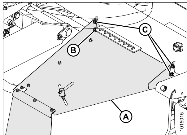
Figure 4.107: Capot supérieur extérieur (côté droit)
