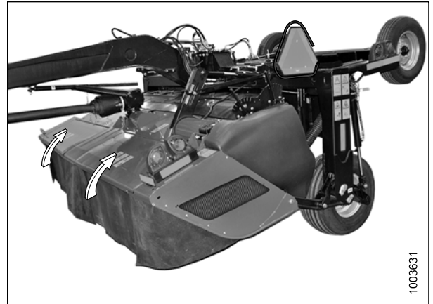
Figure 10.1: Faucheuse à disques de type tracté R113
