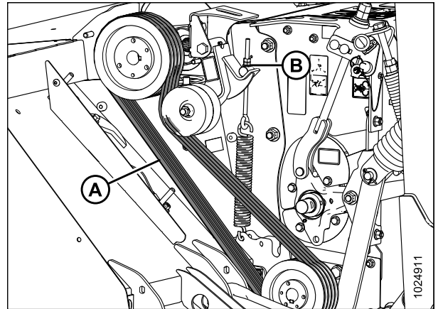
Figure 8.10: Entraînement de la conditionneuse
