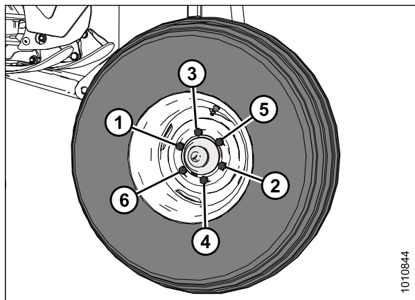
Figure 3.132: Séquence de serrage
