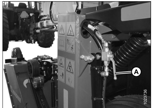
Figure 7.11: Clapet de verrouillage du vérin de levage
