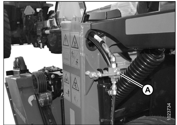
Figure 3.163: Clapets de verrouillage des vérins de levage
