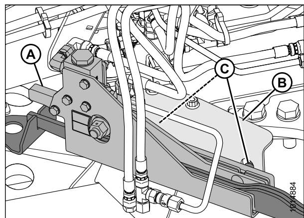
Figure 3.77: Contrôles d'alignement (vue de face, à droite)
