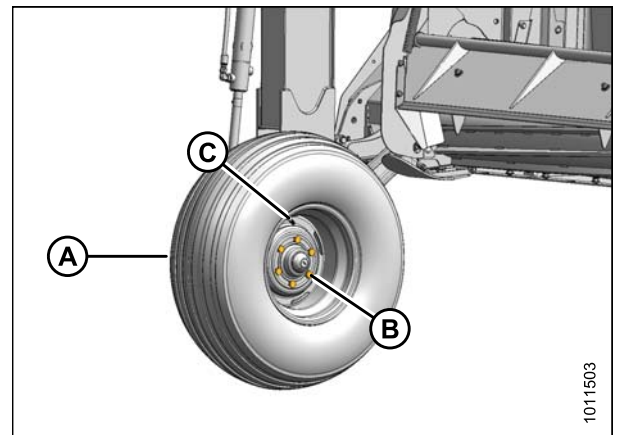
Figure 3.131: Installation des boulons de roue
