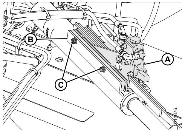
Figure 4.55: Contrôle d'alignement (vue de l'arrière, à droite)
