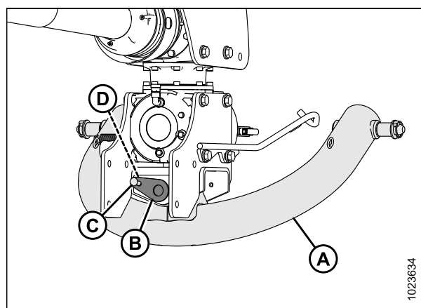
Figure 4.34: Adaptateur d'attelage deux points
