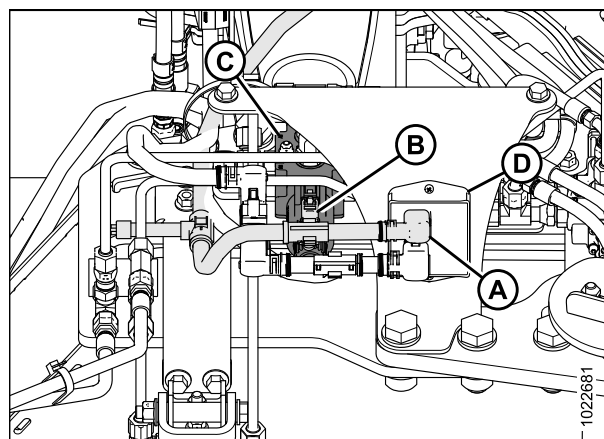
Figure 4.67: Alimentation de la vanne sélectrice
