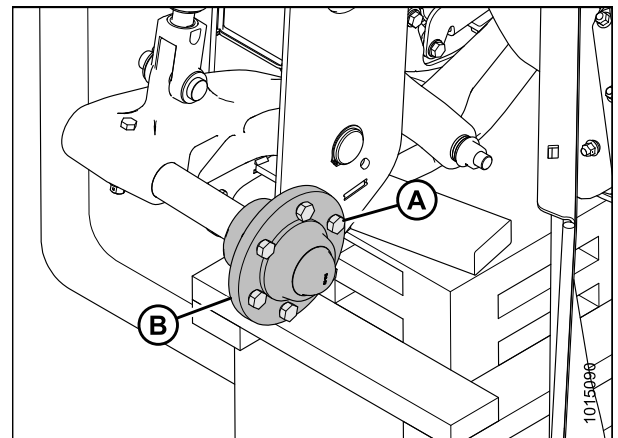
Figure 3.130: Fusée de la roue
