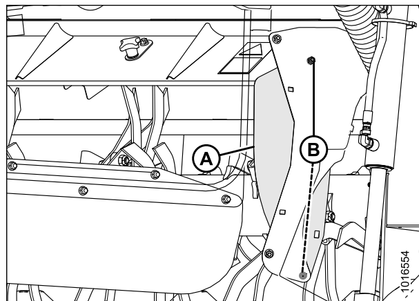
Figure 4.113: Blindage du déflecteur de droite illustré – Blindage du déflecteur de gauche opposé
