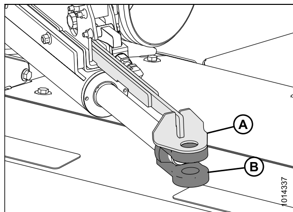
Figure 4.57: Contrôle d'alignement (vue de l'arrière, à droite)
