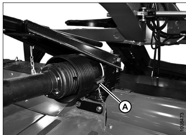
Figure 6.34: Cône de protection de la transmission
