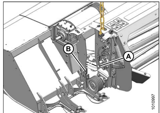
Figure 8.18: Goupilles de la conditionneuse
