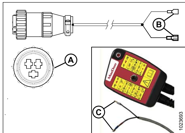
Figure 3.108: Connecteur auxiliaire à trois broches
