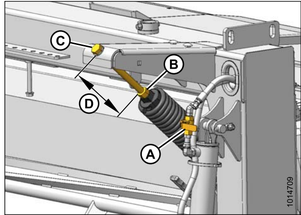
Figure 4.9: Clapet de verrouillage du vérin de levage, contre-écrou et boulon de réglage
