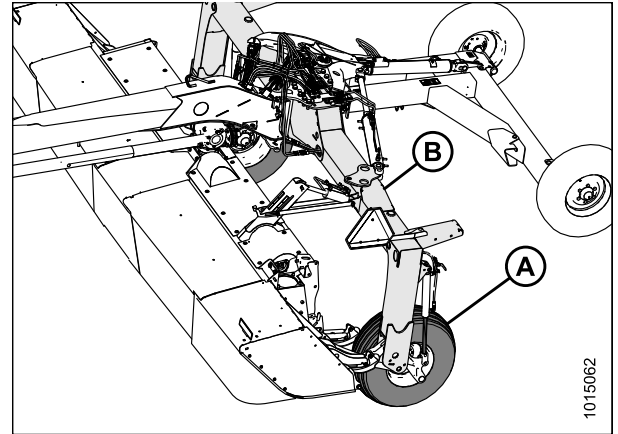
Figure 3.162: Faucheuse à disques avec transport
