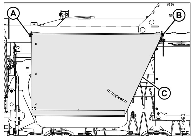
Figure 3.137: Capot supérieur extérieur
