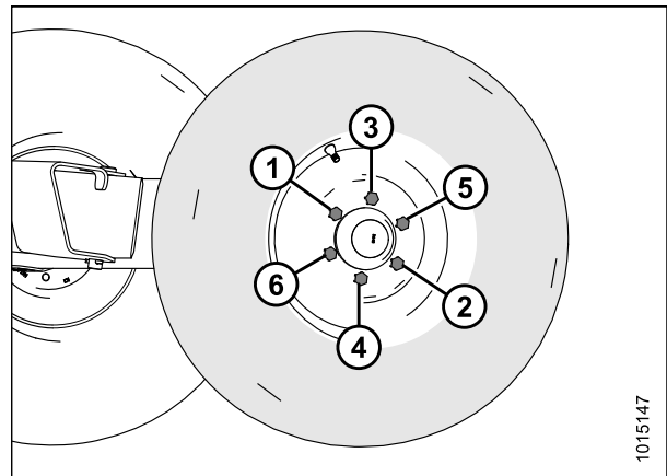
Figure 3.76: Séquence de serrage
