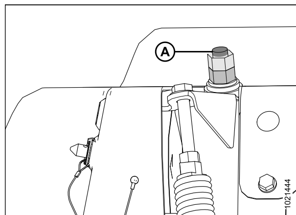
Figure 6.20: Réglage de l'écartement des rouleaux
