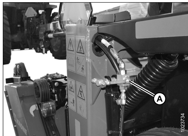
Figure 6.50: Clapet de verrouillage du vérin de levage
