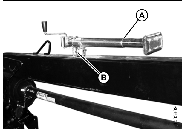
Figure 7.5: Cric rangé à sa place
