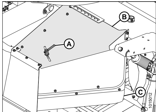
Figure 4.111: Ensemble du déflecteur latéral
