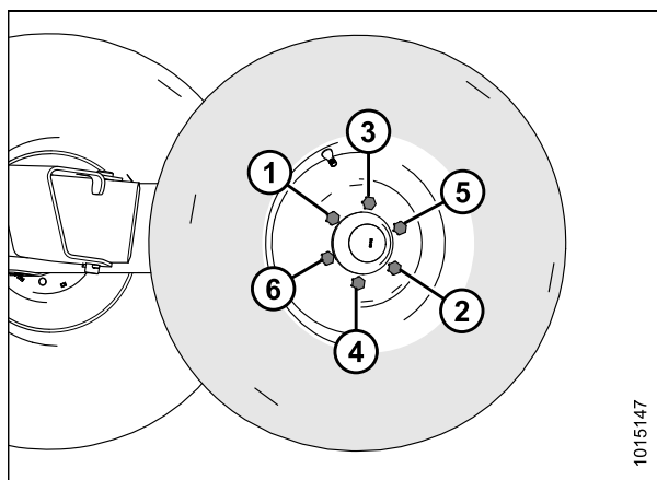
Figure 4.102: Séquence de serrage
