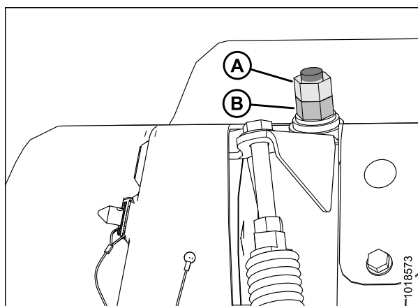
Figure 6.22: Réglage de l'écartement des rouleaux
