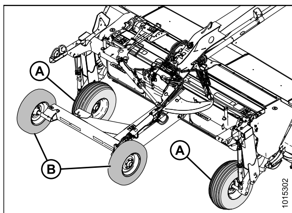
Figure 6.3: Roues de travail et roues de transport
