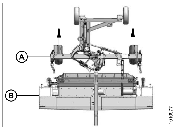
Figure 8.8: Châssis retiré de la plateforme
