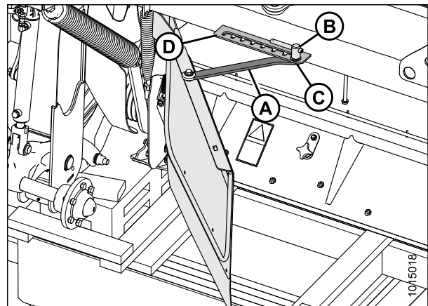
Figure 4.117: Barre de réglage
