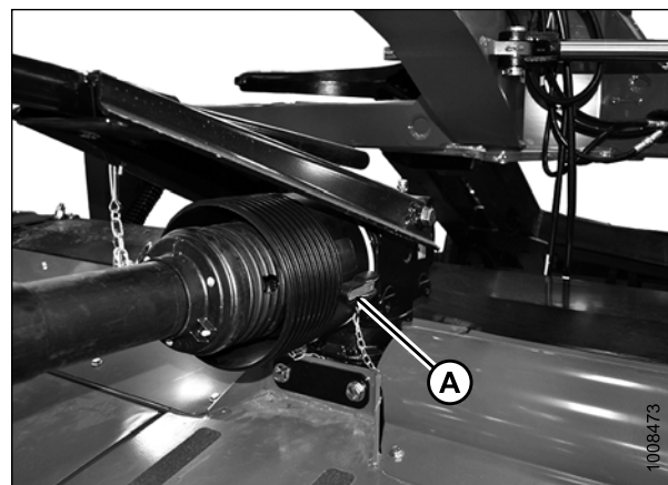
Figure 6.30: Cône de protection de la transmission
