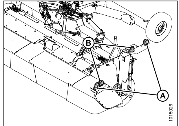
Figure 7.6: Emplacements des feux (avec le Road Friendly Transport™)
