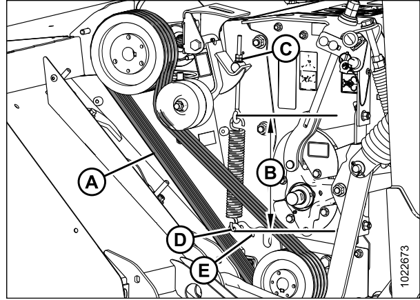
Figure 8.32: Entraînement de la conditionneuse
