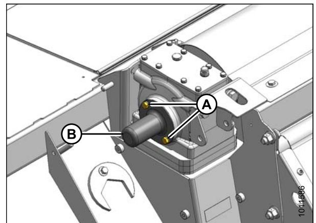
Figure 8.22: Protection de l'arbre
