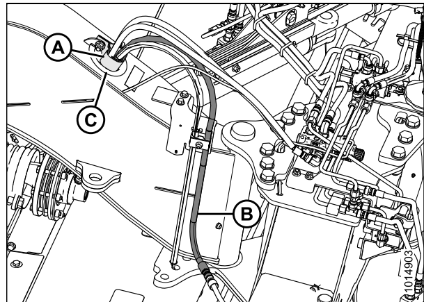
Figure 3.91: Flexibles de levage
