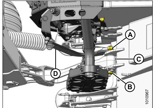
Figure 8.5: Côté droit du châssis (vue de dessus)
