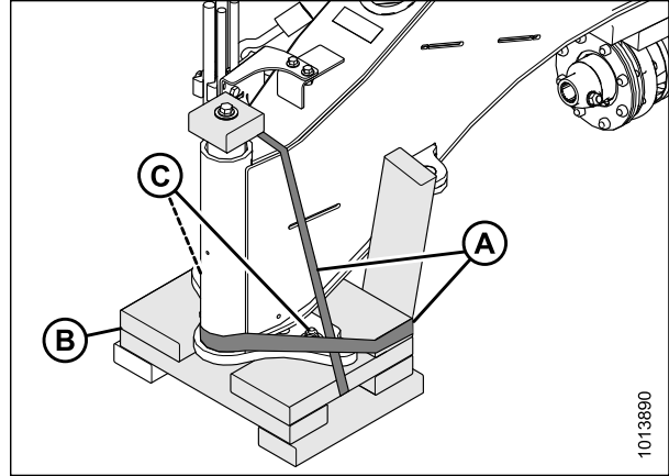
Figure 4.13: Emballage de l'attelage
