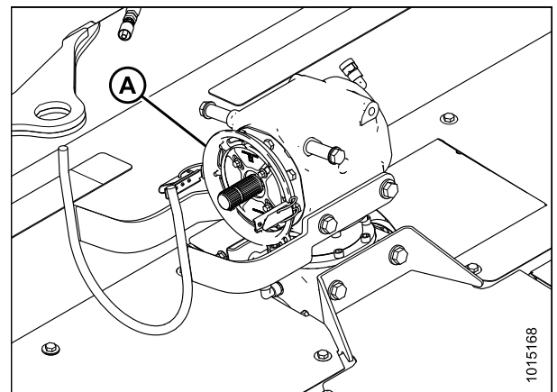
Figure 3.13: Boîte de vitesses
