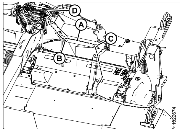
Figure 3.101: Passage du faisceau
