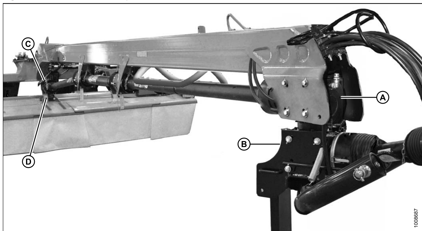
Figure 6.15: Boîtes de vitesses pivotantes avant et arrière
