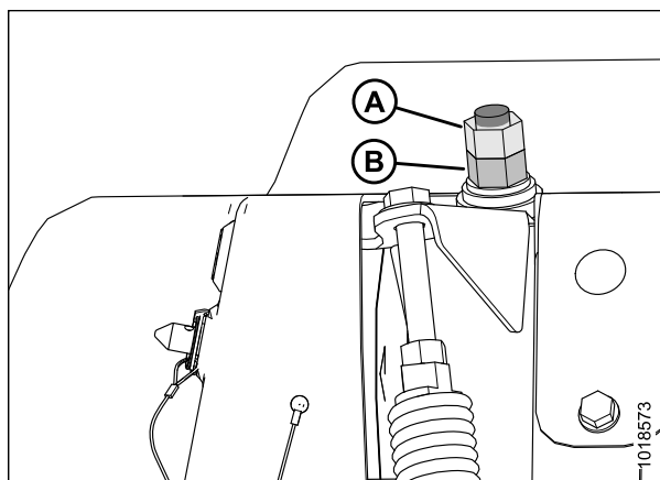
Figure 6.21: Réglage de l'écartement des rouleaux
