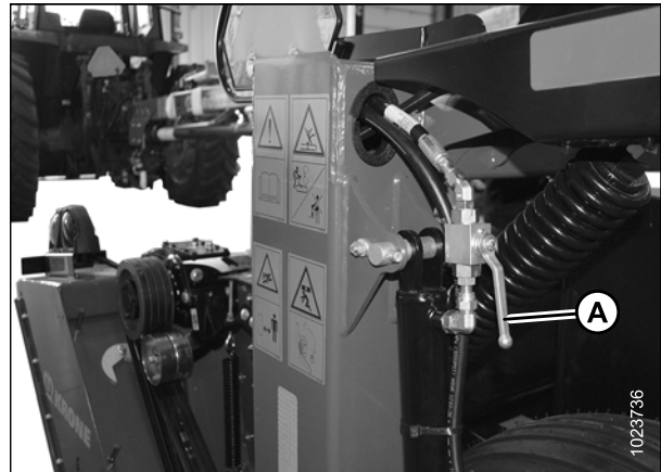
Figure 6.57: Clapet de verrouillage du vérin de levage
