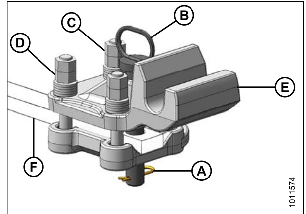
Figure 3.114: Adaptateur du crochet d'attelage
