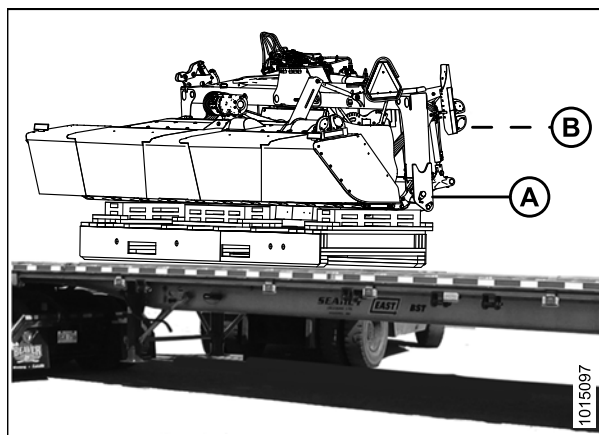
Figure 2.2: Déchargement de la de la faucheuse à disques
