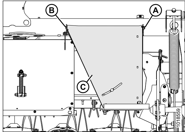
Figure 3.138: Capot supérieur extérieur
