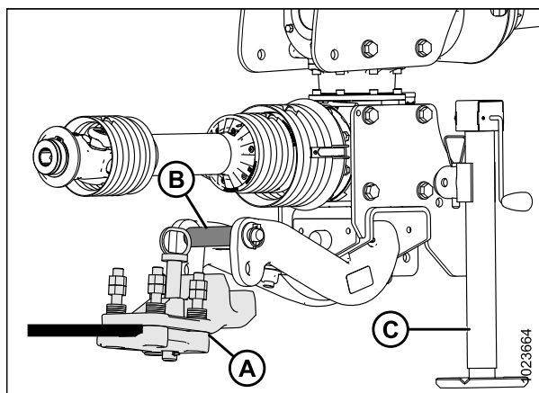
Figure 4.78: Attelage de la faucheuse à disques
