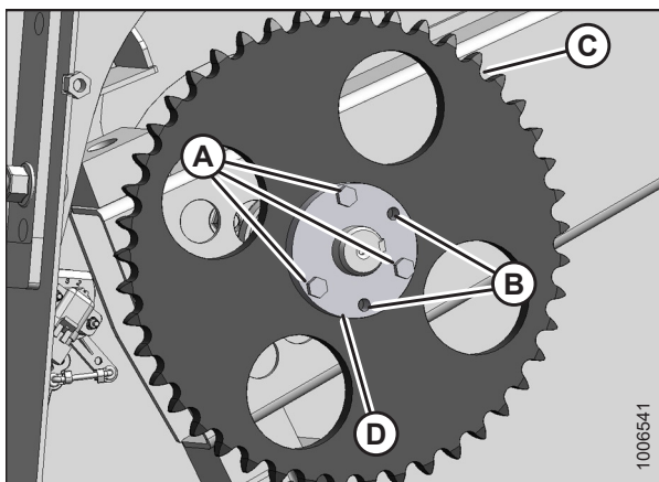
Figura 5.56: Piñón de mando
