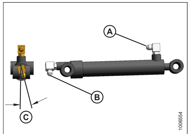
Figura 5.178: Cilindro maestro
