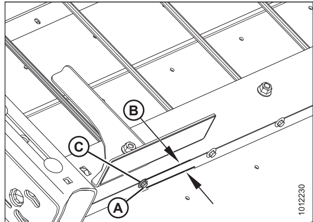
Figura 5.171: Varilla de fibra de vidrio externa
