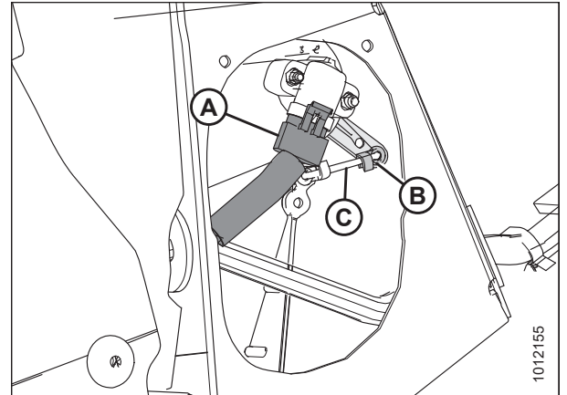
Figura 4.15: Ensamblaje del sensor de altura de la plataforma; lado derecho
