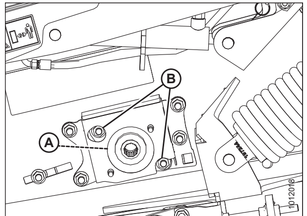
Figura 5.161: Rodillo de mando de la cama frontal del lado izquierdo
