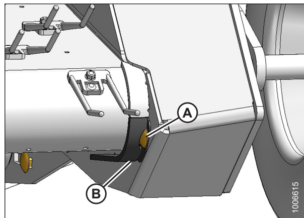
Figura 5.150: Cama delantera de lado izquierdo; lado derecho opuesto.
