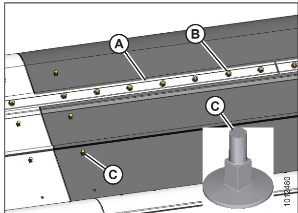
Figura 5.103: Correa de lona delantera
