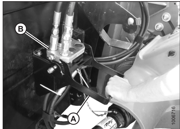
Figura 3.46: Reemplazo del acoplador
