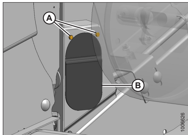
Figura 5.122: Cama trasera del lado derecho
