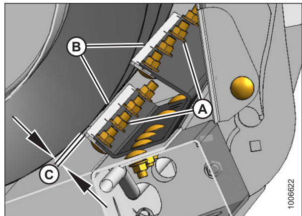
Figura 3.101: Separación de la placa de alimentación
