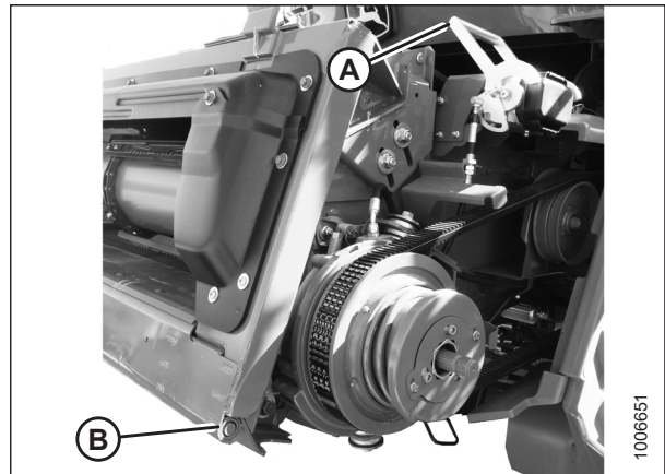
Figura 3.35: Trabas del embocador
