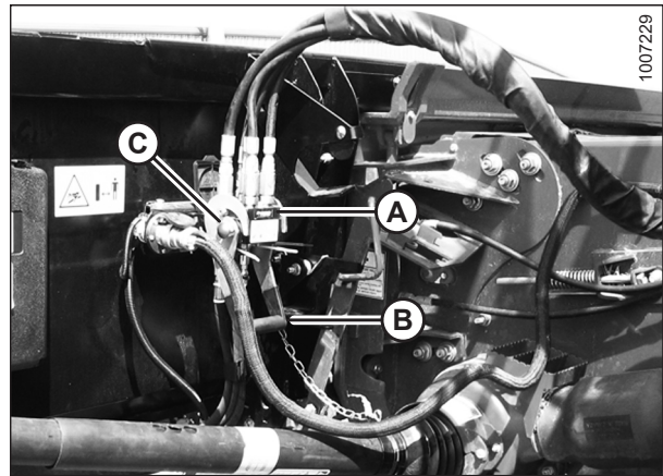
Figura 3.59: Liberación del acoplador
