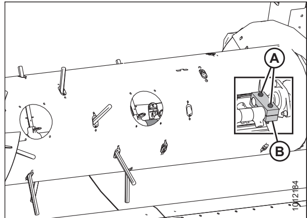
Figura 5.82: Abrazadera de soporte de dedos de sinfín del lado izquierdo - Se muestra la imagen del corte
