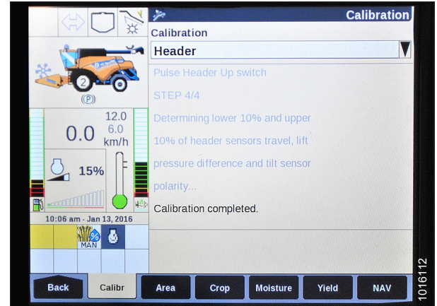
Figura 4.130: Pantalla de la cosechadora New Holland
