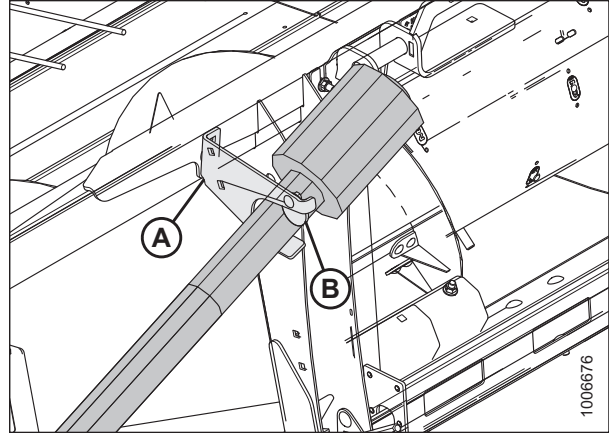
Figura 3.73: Mando en posición de almacenamiento
