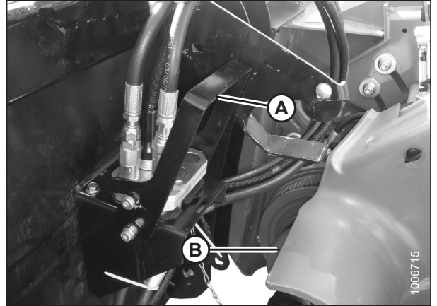
Figura 3.47: Bloqueo del acoplador
