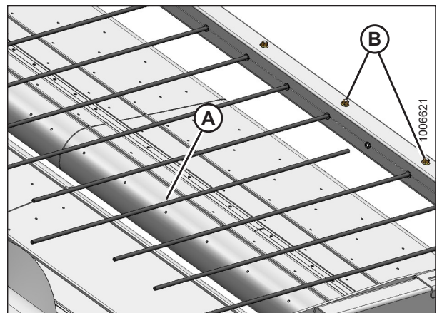
Figura 5.173: Varillas de fibra de vidrio
