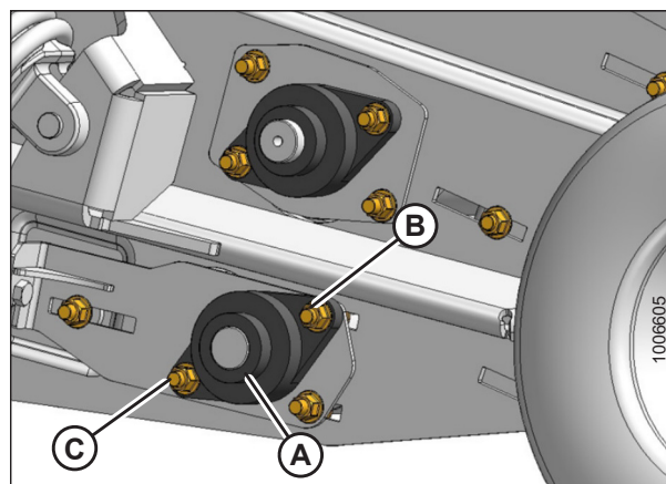
Figura 5.133: Rodamiento de tensor del lado derecho
