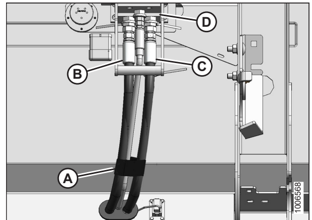
Figura 5.38: Multiacoplador en la parte posterior de la plataforma
