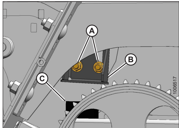
Figura 3.96: Tope izquierdo
