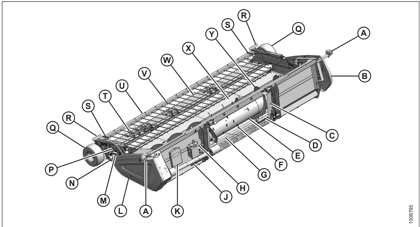
Figura 2.3: Plataforma recolectoraPW8
