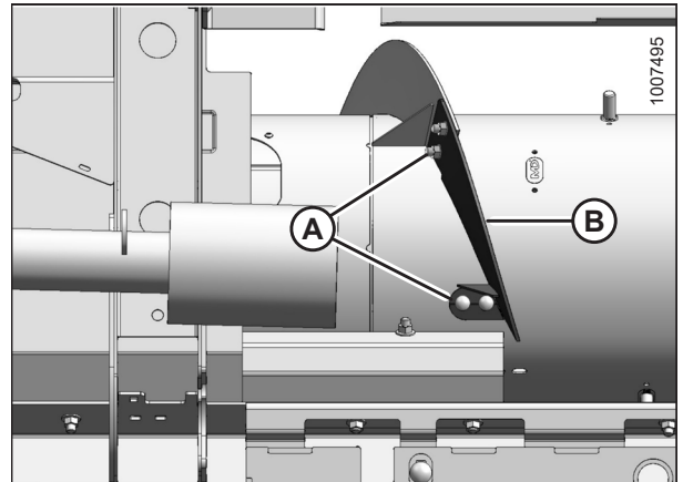
Figura 5.87: Extensión de las alas
