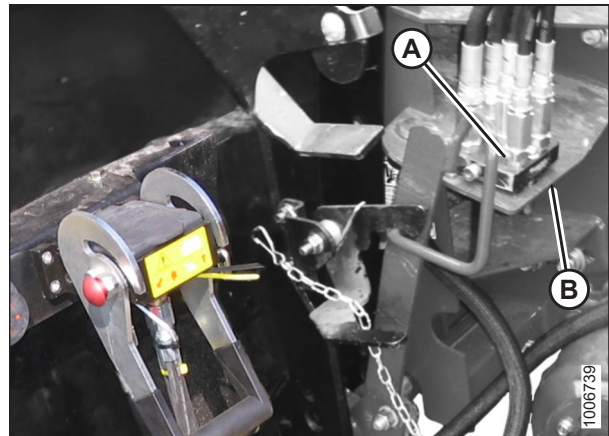
Figura 3.27: Ubicación de almacenamiento del acoplador
