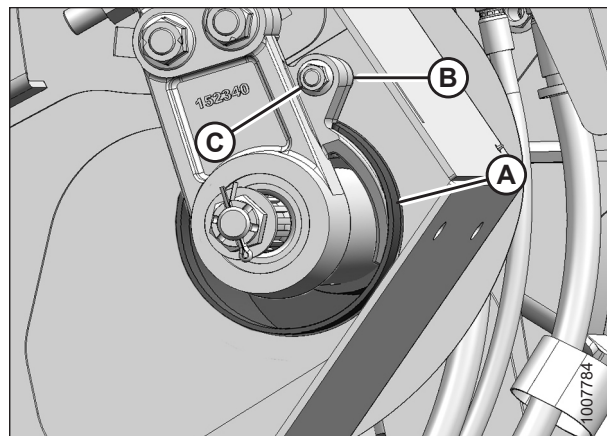
Figura 5.10: Escudo del cardán para cosechadora
