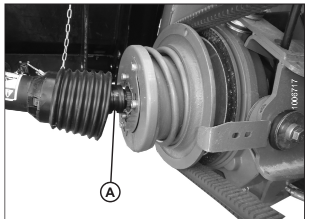
Figura 3.48: Desacoplamiento del cardán para cosechadora
