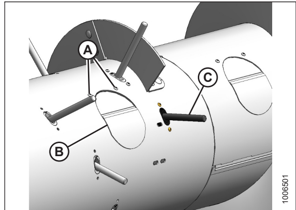
Figura 5.71: Cubierta de acceso
