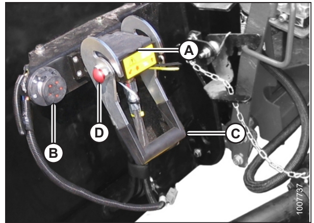
Figura 3.61: Bloqueo del multiacoplador
