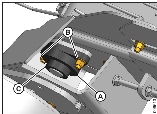
Figura 5.151: Cama delantera de lado izquierdo; lado derecho opuesto.
