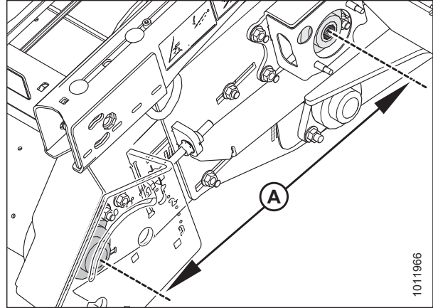
Figura 5.157: Cama delantera de lado izquierdo; lado derecho opuesto
