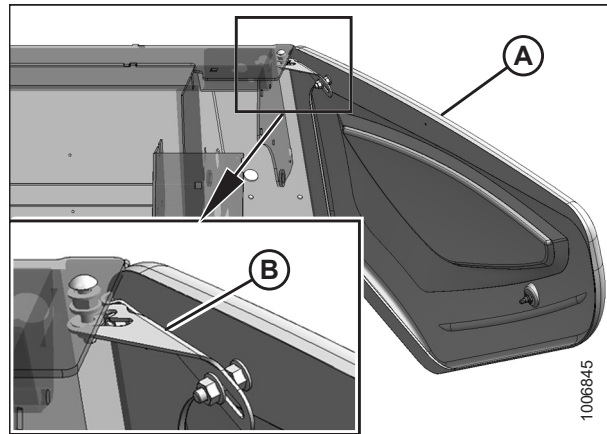
Figura 3.3: Soporte de tapa lateral
