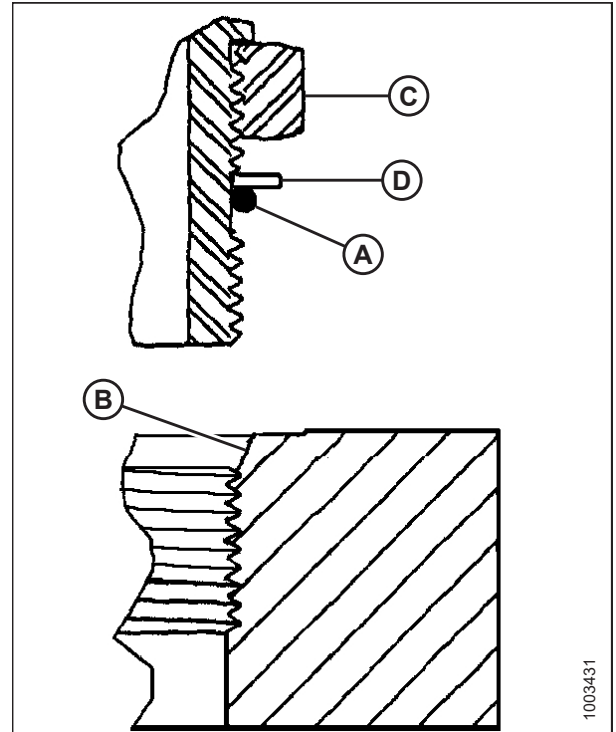
Figura 8.7: Accesorio hidráulico
