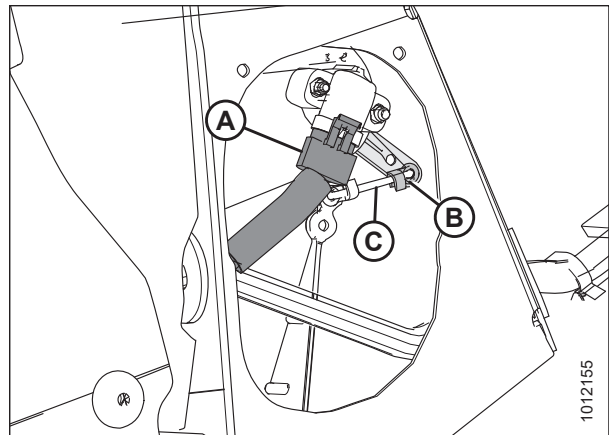
Figura 4.8: Ensamblaje del sensor de altura de la plataforma; lado derecho
