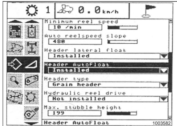
Figura 4.106: Pantalla de la cosechadora New Holland
