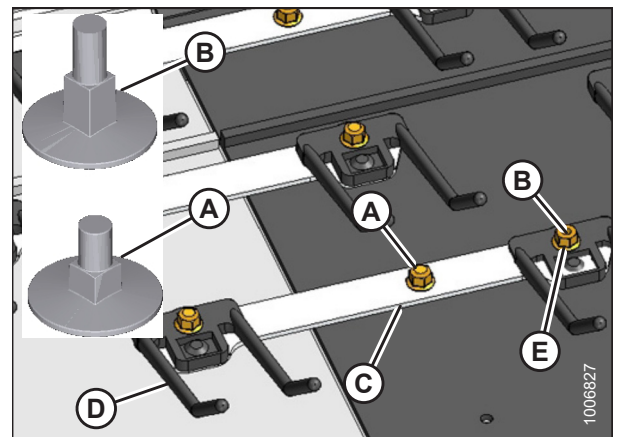
Figura 5.97: Correa de lona delantera
