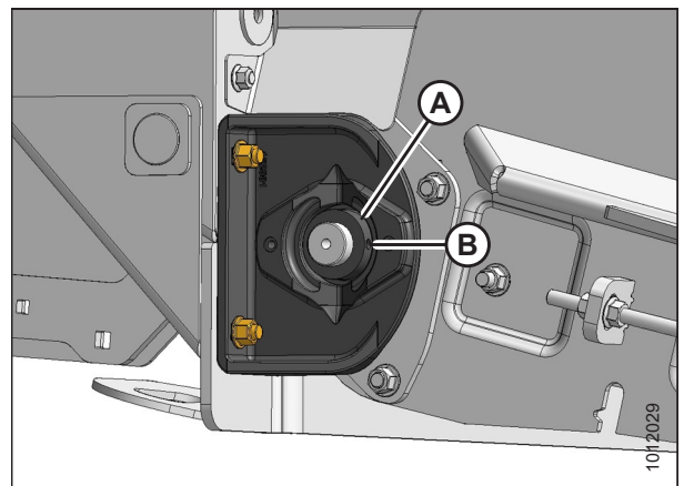
Figura 5.130: Cama trasera del lado derecho
