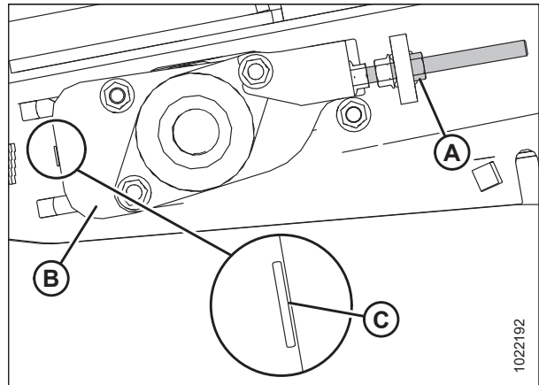
Figura 5.137: Se muestra la cama frontal de lado izquierdo; lado derecho opuesto.
