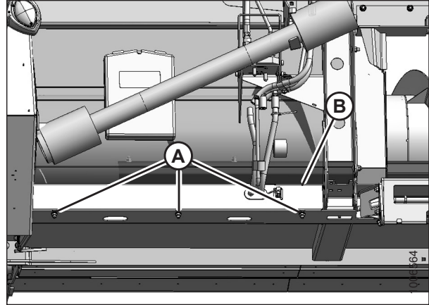
Figura 5.39: Cubierta de viga inferior
