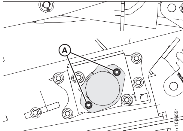
Figura 5.27: Motor hidráulico delantero; lado izquierdo
