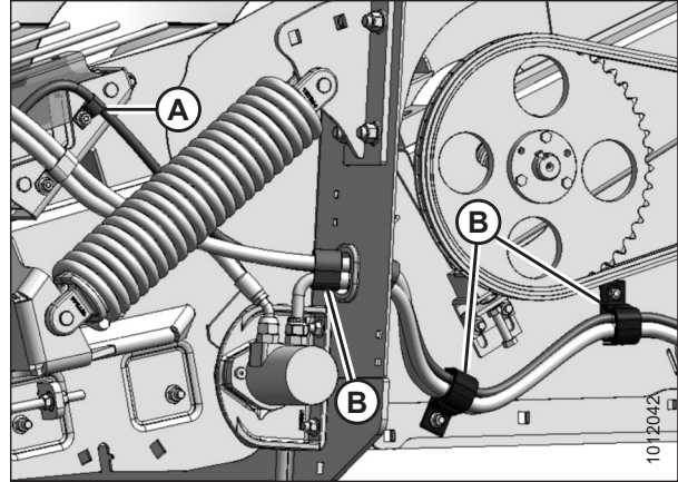
Figura 5.202: Lado izquierdo de la plataforma
