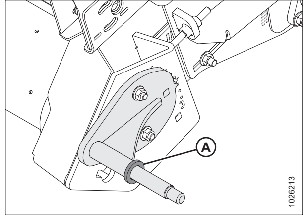
Figura 5.209: Husillo de las ruedas: lado izquierdo de la plataforma
