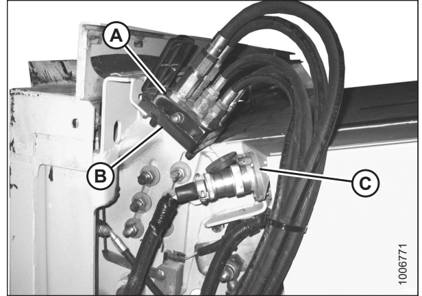
Figura 3.60: Ubicación de almacenamiento del acoplador y del conector eléctrico
