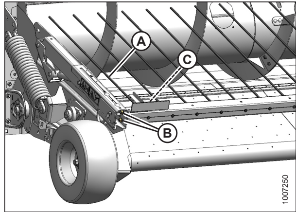
Figura 5.170: Varilla de fibra de vidrio externa
