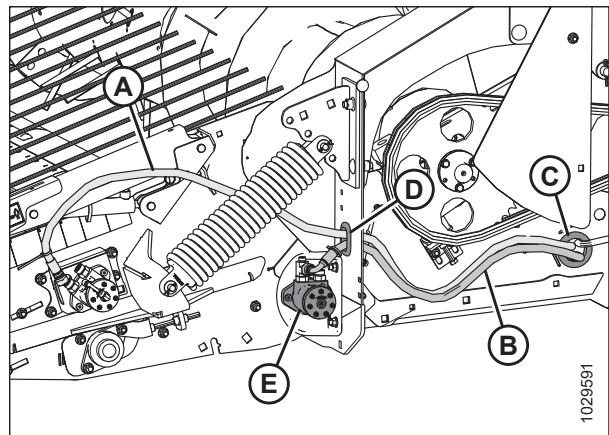
Figura 5.41: Lado izquierdo de la plataforma:
