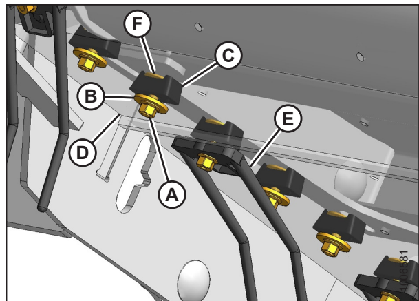
Figura 5.106: Guías de la lona
