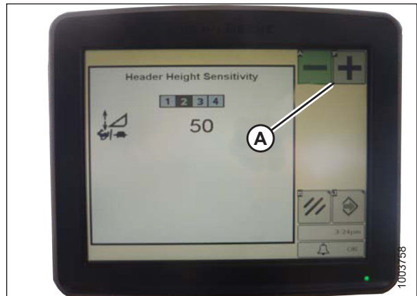
Figura 4.92: Pantalla de la cosechadora John Deere
