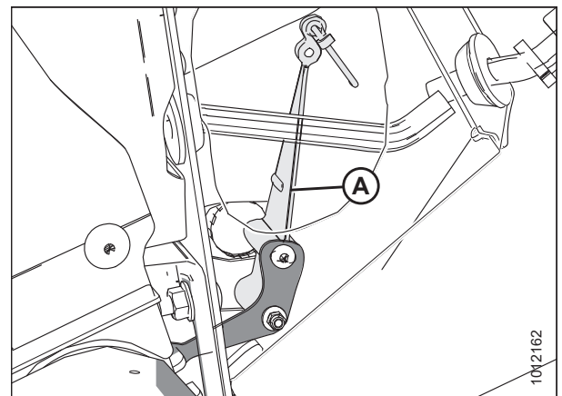
Figura 4.11: Ensamble del sensor de altura de la plataforma; lado derecho
