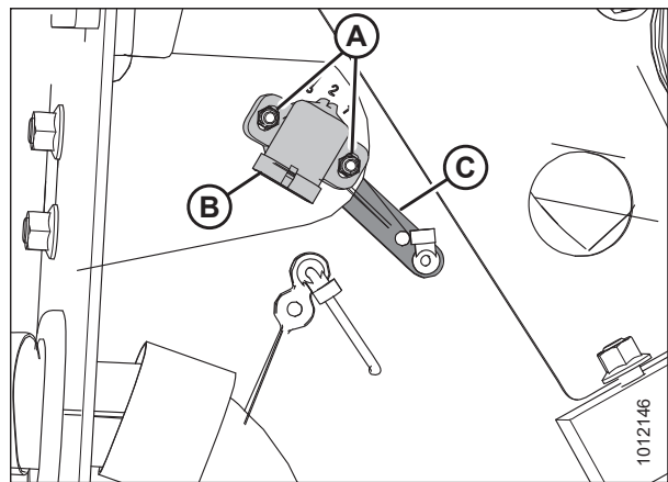
Figura 4.4: Ensamblaje del sensor de altura de la plataforma; lado izquierdo
