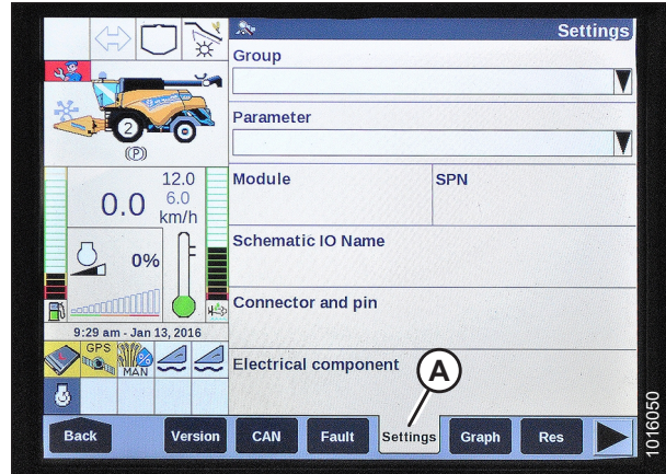
Figura 4.123: Pantalla de la cosechadora New Holland
