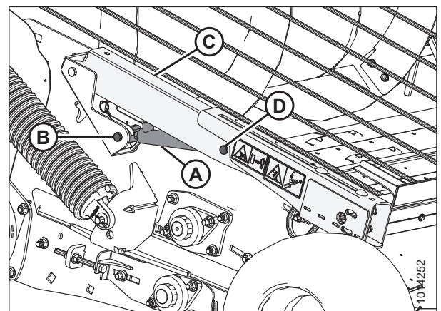
Figura 5.187: Cilindro secundario: lado derecho de la plataforma
