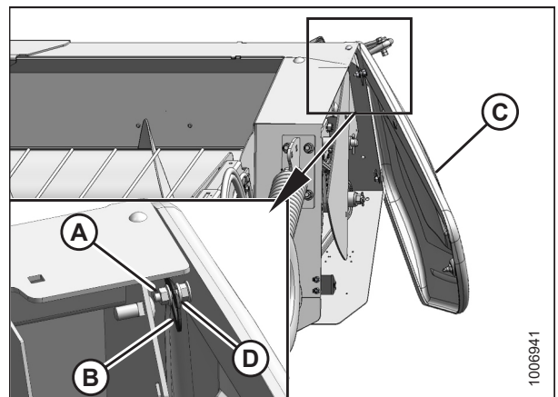
Figura 3.11: Acoplamiento del soporte
