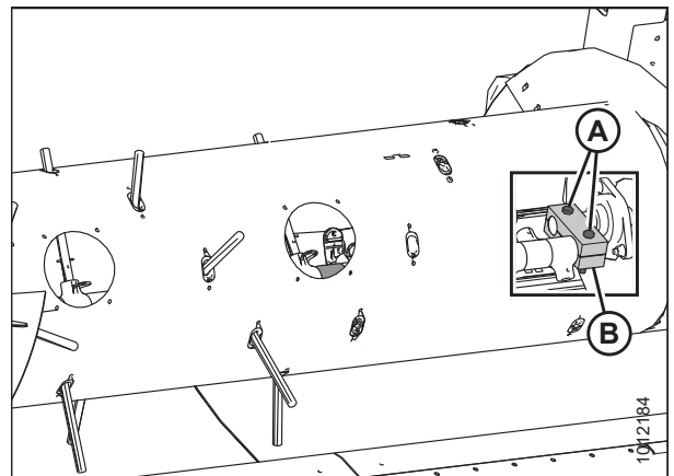
Figura 5.79: Abrazadera de soporte de dedos del sinfín del lado izquierdo - Se muestra la imagen del corte
