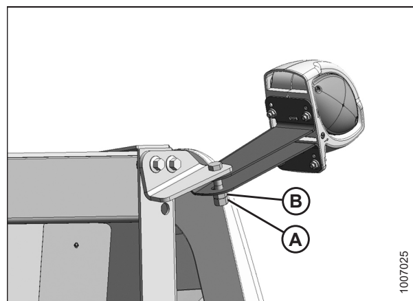
Figura 5.212: Luces de transporte
