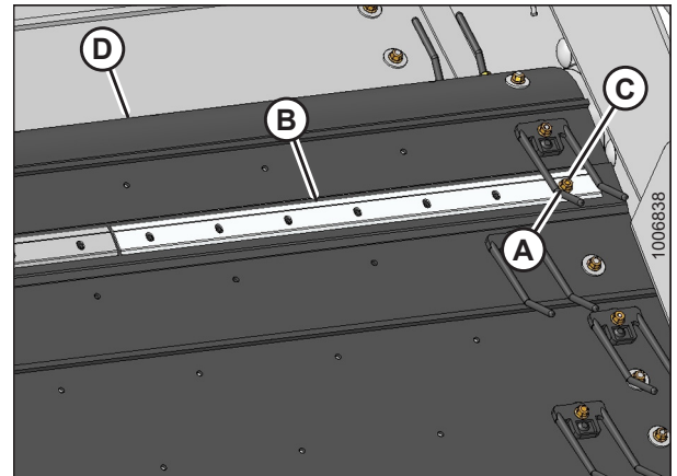
Figura 5.91: Correa de la lona trasera
