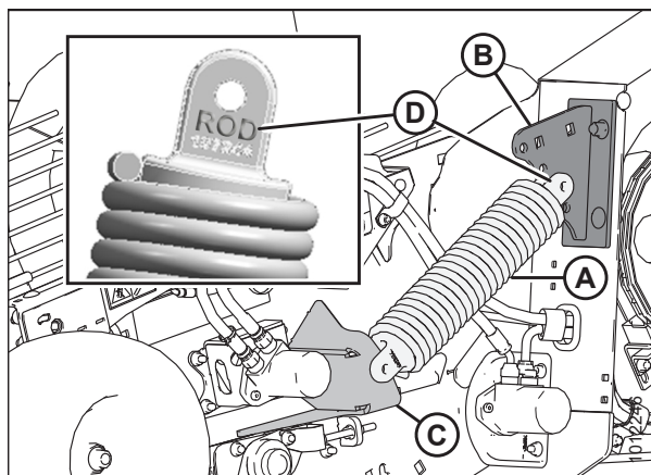
Figura 5.165: Se muestran los anclajes del lado izquierdo; lado derecho opuesto
