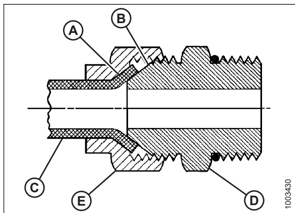
Figura 8.6: Accesorio hidráulico
