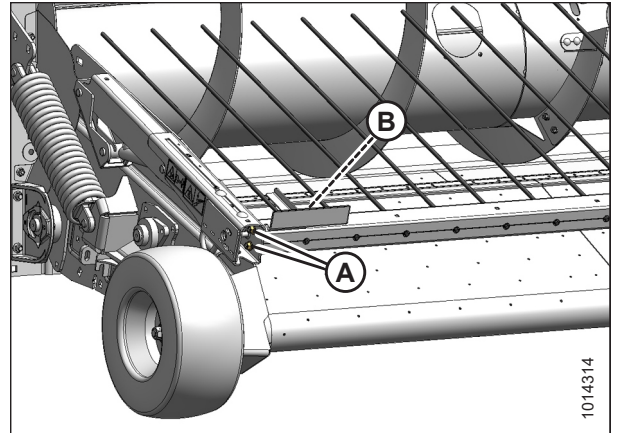
Figura 5.172: Varilla de fibra de vidrio externa
