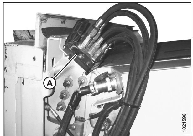
Figura 3.57: Acoplador/conector de la cosechadora
