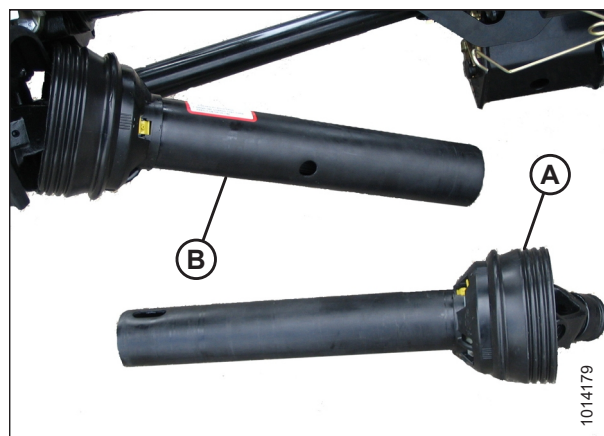
Figura 5.15: Mando separado
