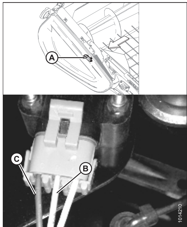
Figura 4.20: Sensor de altura derecho
