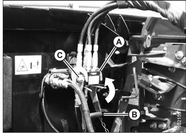
Figura 3.26: Liberación del acoplador
