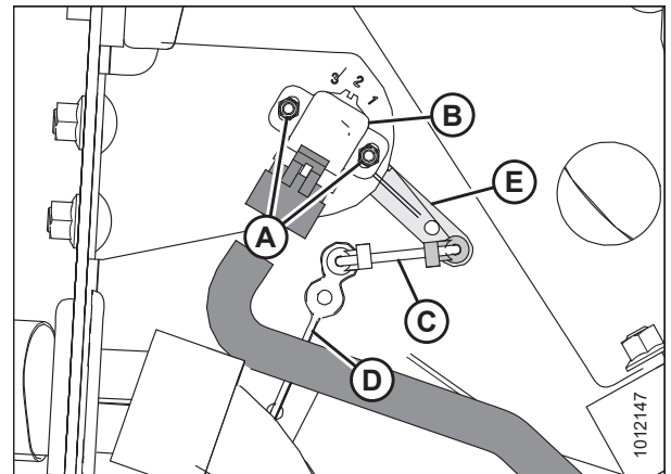
Figura 4.21: Ensamblaje del sensor de altura de la plataforma; lado izquierdo
