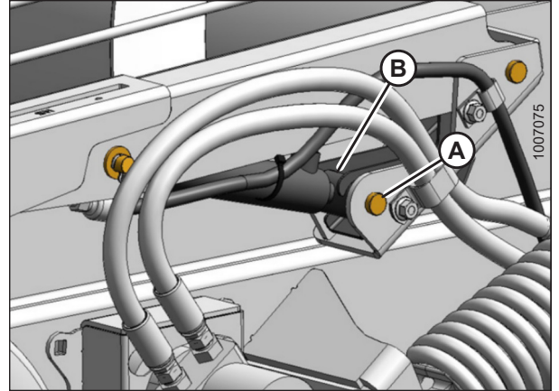
Figura 5.176: Cilindro maestro: lado izquierdo de la plataforma
