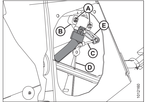
Figura 4.24: Ensamblaje del sensor de altura de la plataforma; lado derecho
