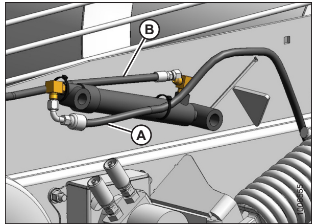
Figura 5.177: Cilindro maestro: lado izquierdo de la plataforma
