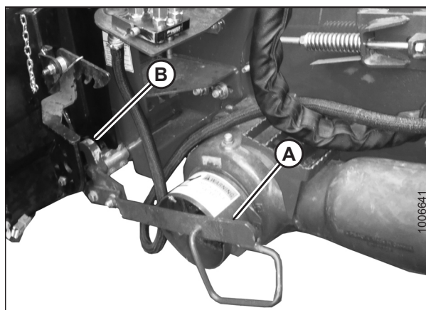
Figura 3.19: Trabas del embocador
