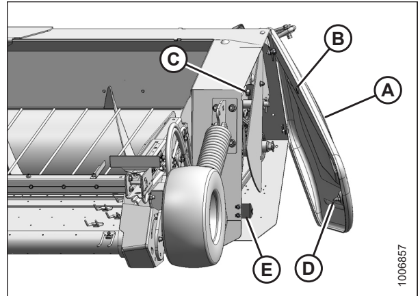
Figura 3.10: Alineación de la tapa lateral
