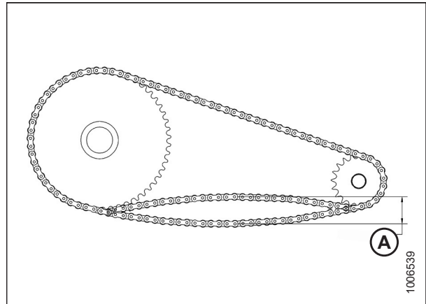
Figura 5.51: Desviación de cadena
