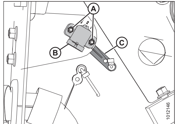
Figura 4.5: Ensamble del sensor de altura de la plataforma; lado izquierdo
