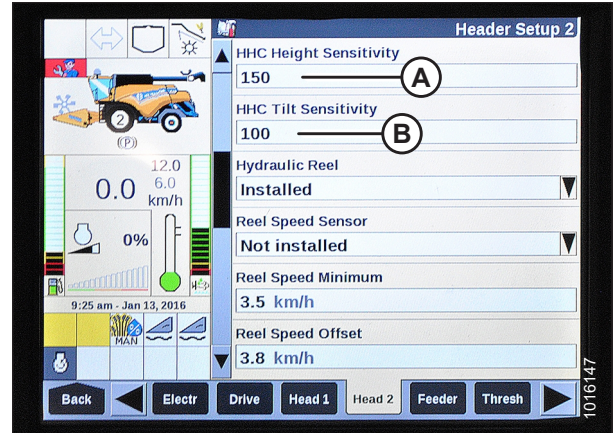
Figura 4.121: Pantalla de la cosechadora New Holland
