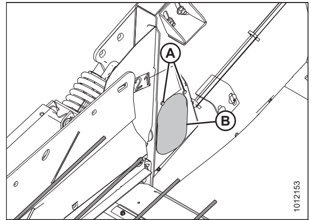
Figura 4.25: Panel de acceso: lado derecho
