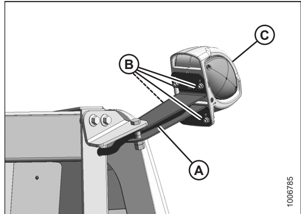
Figura 5.215: Luces de transporte
