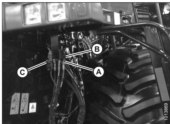
Figura 3.79: Ubicación de almacenamiento del acoplador y del conector eléctrico
