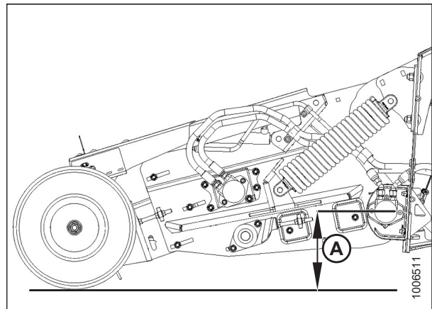
Figura 3.105: Altura de funcionamiento
