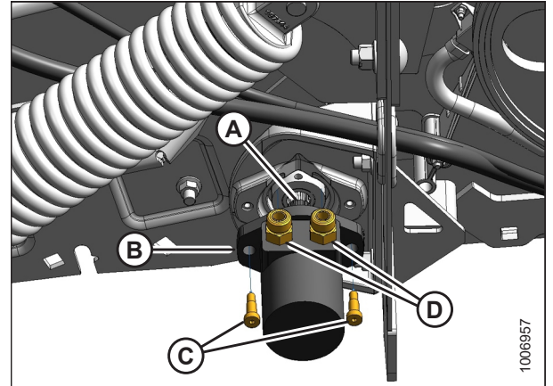
Figura 5.32: Motor hidráulico trasero; lado izquierdo
