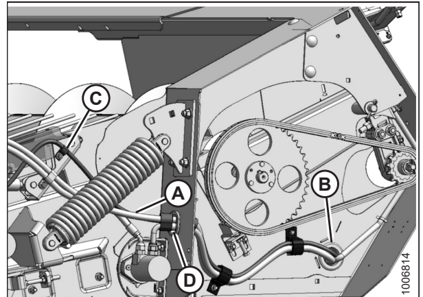
Figura 5.199: Parte final izquierda
