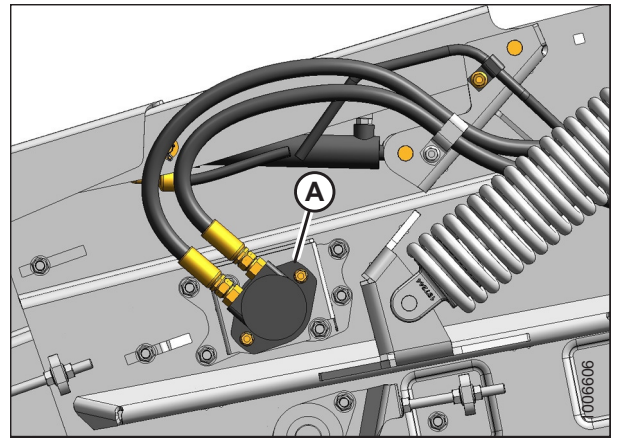
Figura 5.134: Motores hidráulicos delanteros
