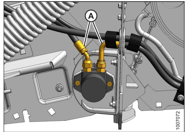
Figura 5.33: Motor hidráulico trasero; lado izquierdo
