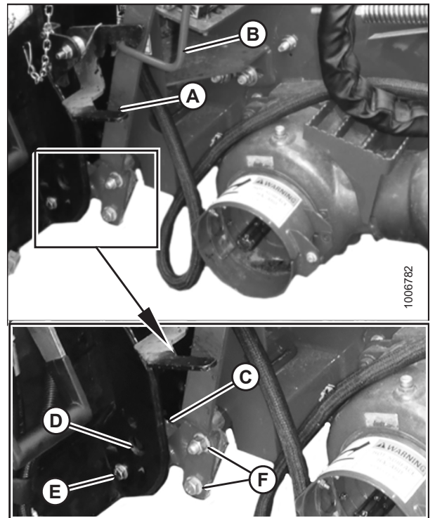
Figura 3.21: Activación de bloqueos
