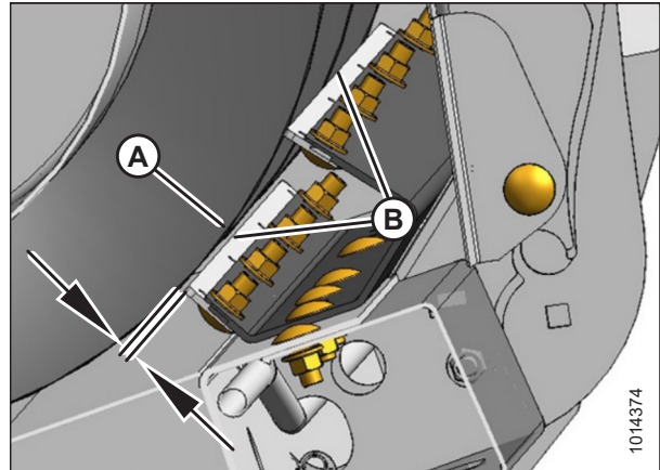
Figura 3.100: Separación de la placa de alimentación
