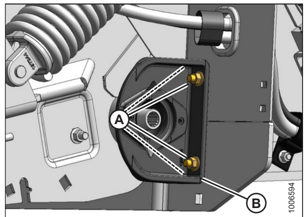
Figura 5.113: Cama trasera del lado izquierdo
