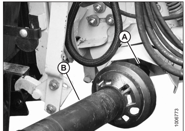
Figura 3.62: Desacoplamiento del cardán para cosechadora
