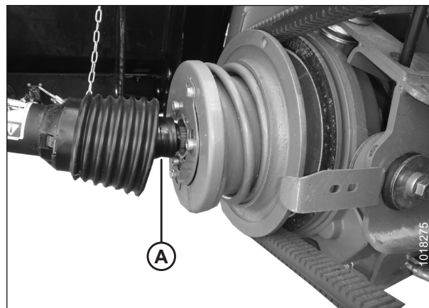
Figura 5.14: Extremo de la cosechadora del cardán conectado a la cosechadora
