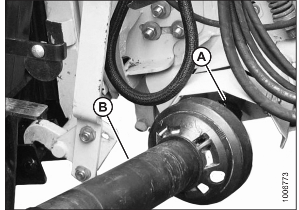
Figura 3.55: Acoplamiento del cardán para cosechadora
