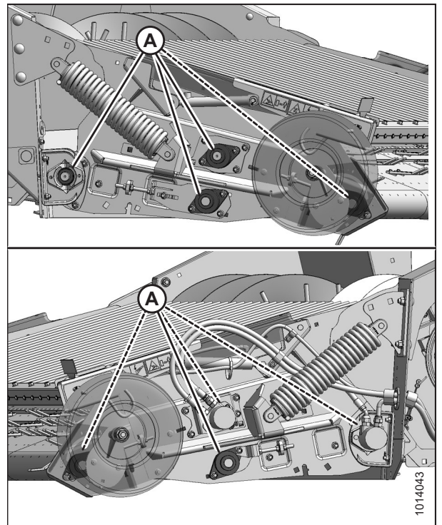
Figura 5.108: Rodamientos del rodillo de lona
