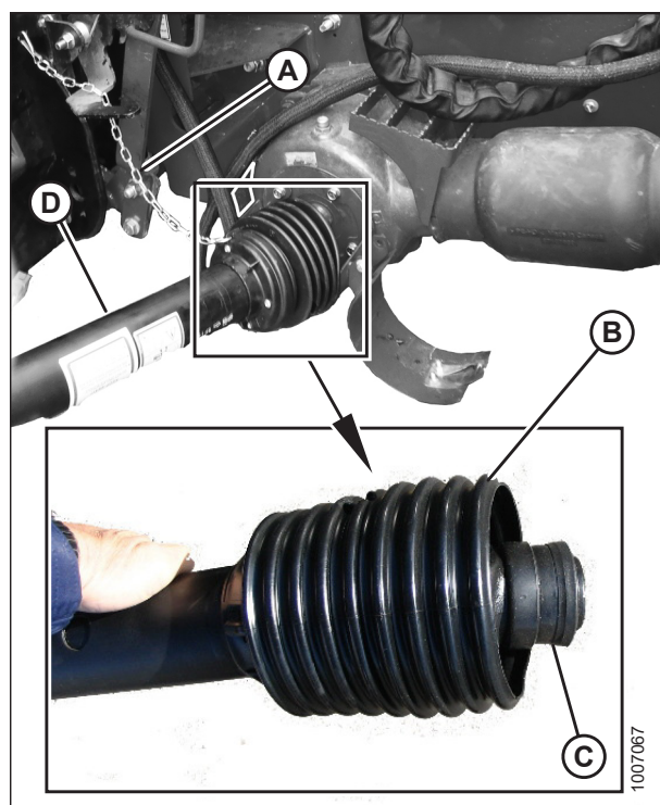
Figura 5.11: Mando
