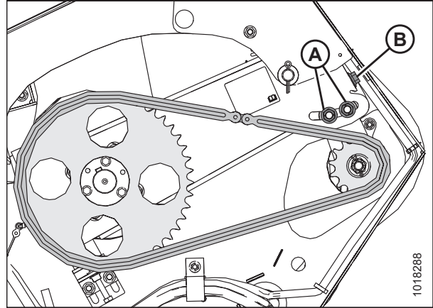
Figura 5.50: Cadena de mando del sinfín
