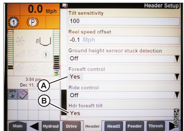
Figura 4.53: Pantalla de la cosechadora Case IH
