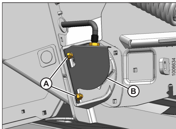
Figura 5.121: Cama trasera del lado derecho
