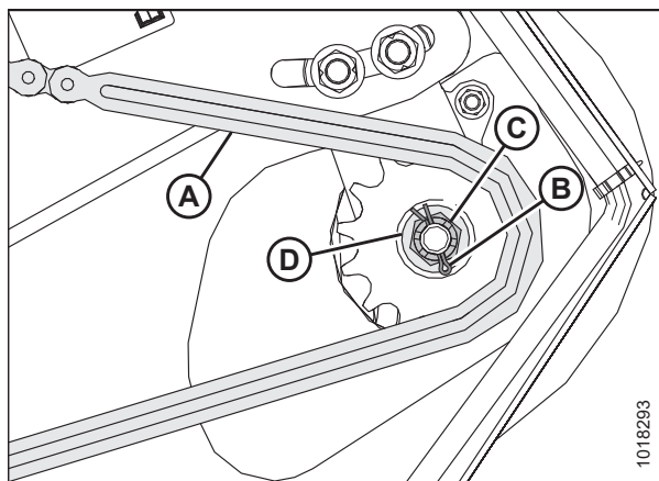
Figura 5.62: Piñón de mando
