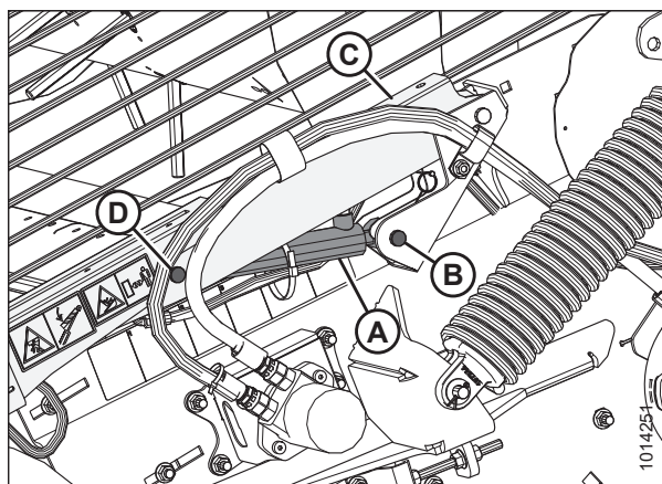
Figura 5.174: Cilindro maestro: lado izquierdo de la plataforma
