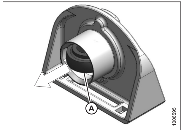
Figura 5.126: Soporte de rodamiento
