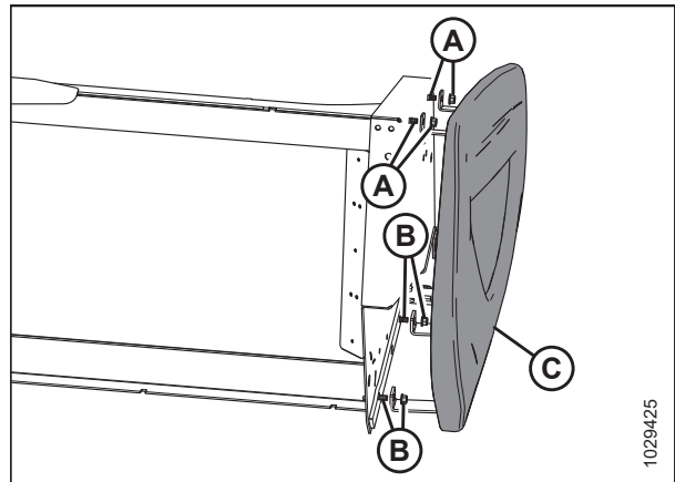
Figura 3.14: Tapa lateral derecha
