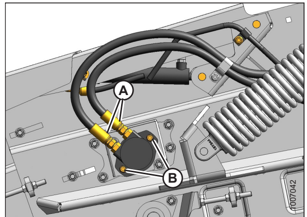
Figura 5.24: Motor hidráulico delantero; lado izquierdo
