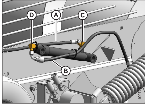
Figura 5.179: Cilindro maestro: lado izquierdo de la plataforma
