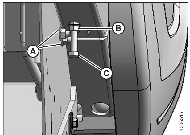
Figura 3.90: Tope derecho del sinfín
