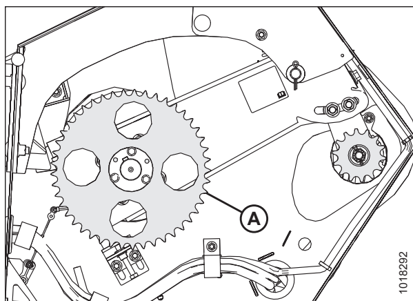
Figura 5.61: Piñón accionado
