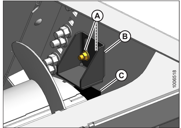
Figura 3.93: Tope derecho
