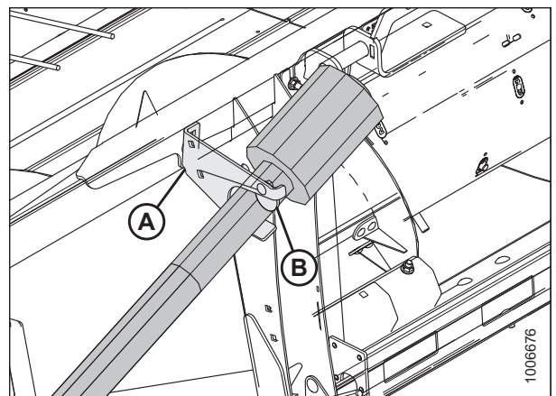
Figura 3.82: Mando
