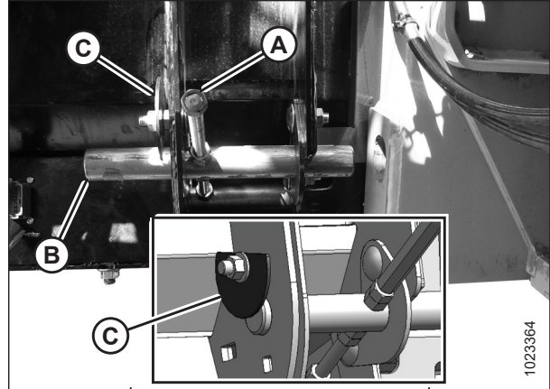
Figura 3.83: Bloqueo del embocador
