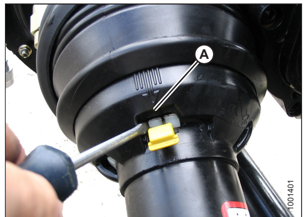
Figura 5.20: Protección del mando
