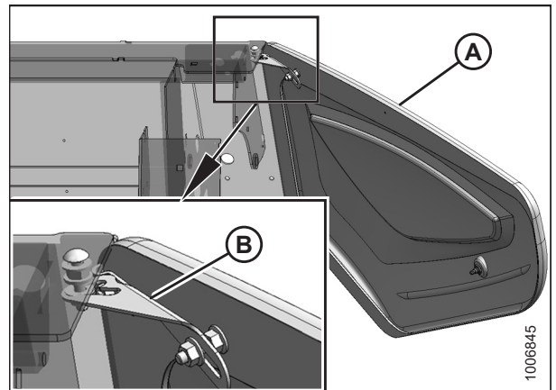
Figura 3.2: Tapa lateral abierta
