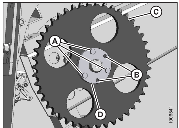
Figura 5.59: Piñón de mando
