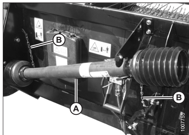
Figura 3.117: Protección del mando
