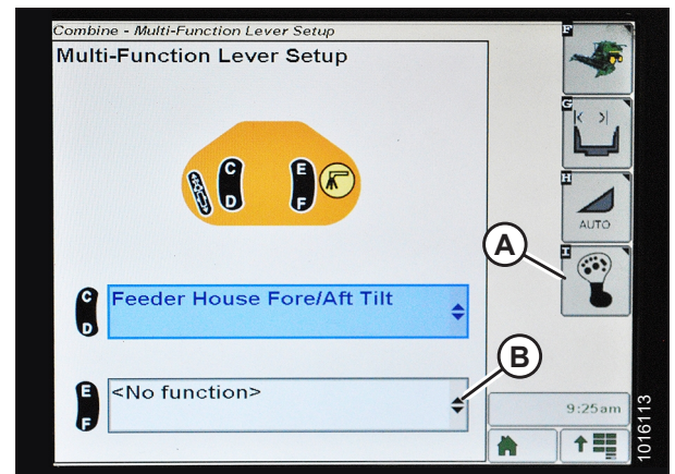
Figura 4.80: Pantalla de la cosechadora John Deere
