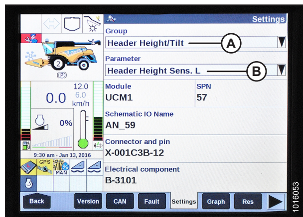
Figura 4.124: Pantalla de la cosechadora New Holland
