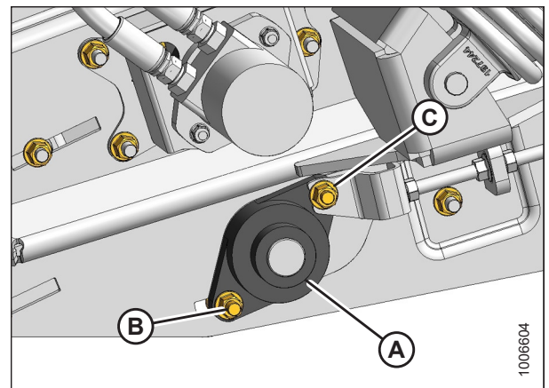
Figura 5.132: Rodamiento de tensor del lado izquierdo
