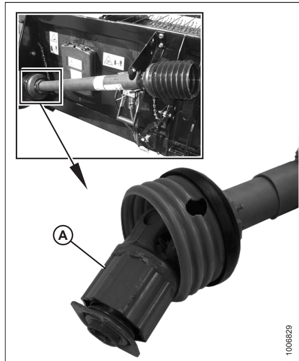
Figura 3.116: Embrague de clavija radial
