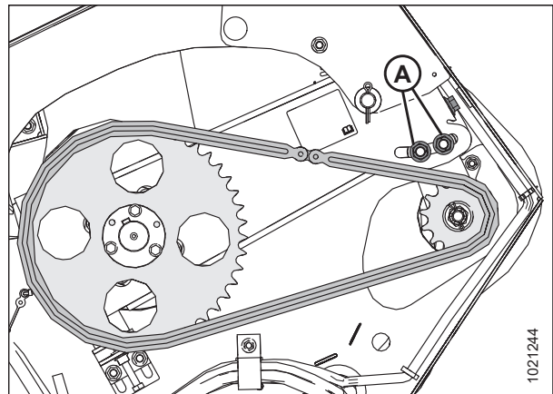
Figura 5.52: Cadena de mando del sinfín
