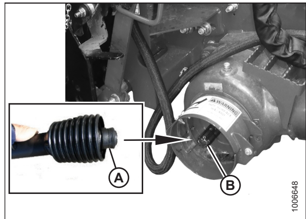
Figura 3.23: Acoplamiento del cardán para cosechadora
