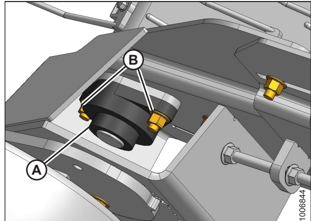
Figura 5.148: Cama delantera de lado izquierdo; lado derecho opuesto.
