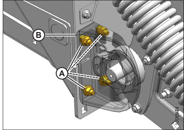
Figura 5.125: Cama trasera del lado derecho
