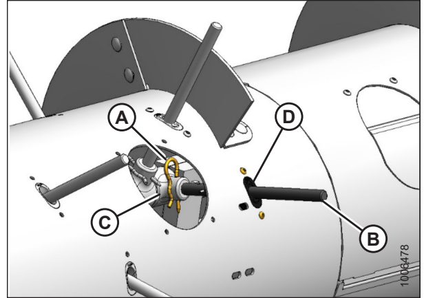
Figura 5.77: Dedos del sinfín
