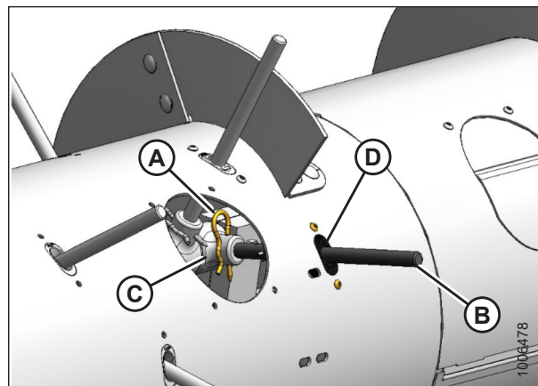
Figura 5.83: Dedos del sinfín
