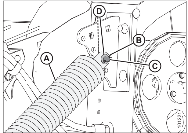
Figura 3.109: Se muestra el ensamble del resorte de flotación del lado izquierdo; lado derecho opuesto.
