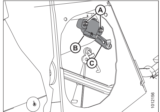
Figura 4.9: Ensamble del sensor de altura de la plataforma; lado derecho
