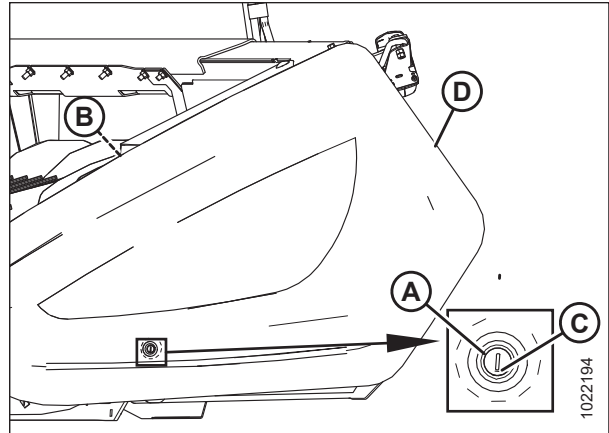
Figura 3.13: Tapa lateral cerrada
