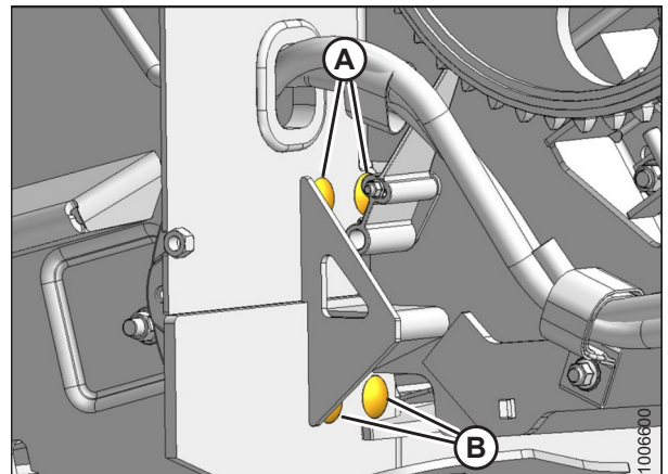
Figura 5.118: Cama trasera del lado izquierdo
