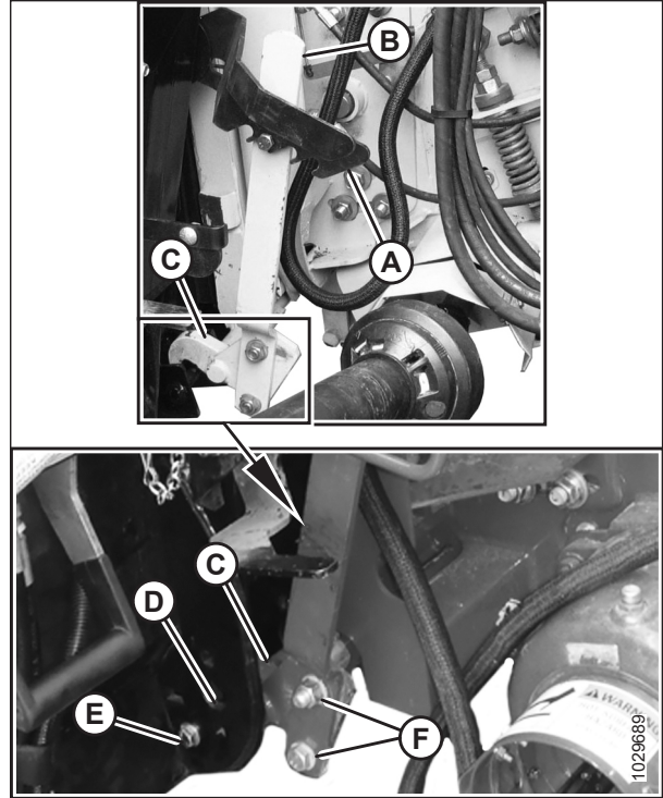
Figura 3.53: Activación de bloqueos
