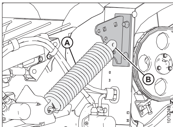
Figura 5.167: Se muestra el anclaje del lado izquierdo; lado derecho opuesto.
