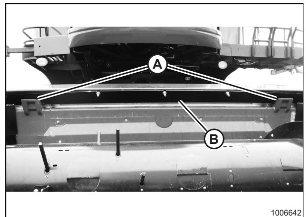
Figura 3.52: Plataforma en la cosechadora
