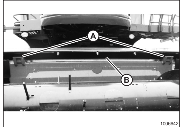
Figura 3.20: Plataforma en la cosechadora
