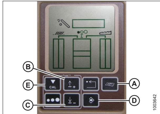
Figura 4.69: Pantalla de la cosechadora John Deere
