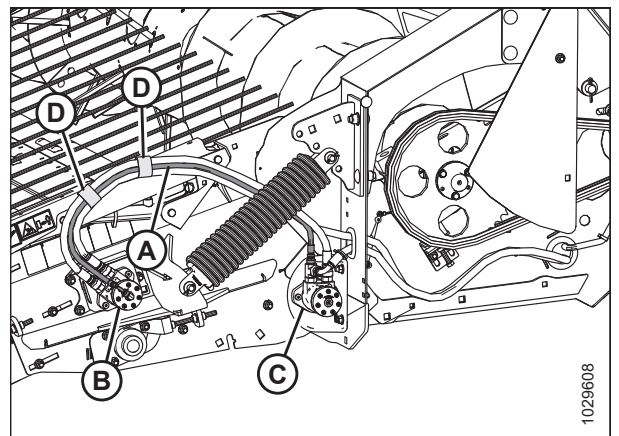
Figura 5.44: Lado izquierdo de la plataforma:
