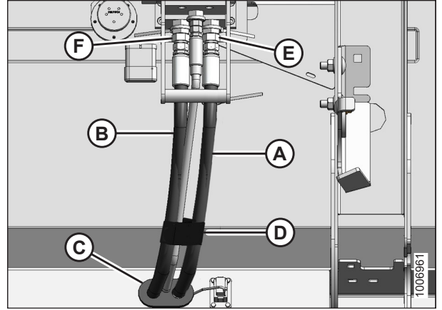
Figura 5.42: Multiacoplador en la parte posterior de la plataforma
