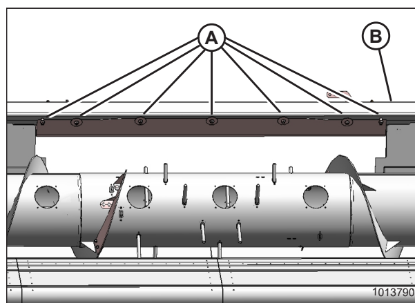
Figura 3.69: Viga superior - Vista frontal
