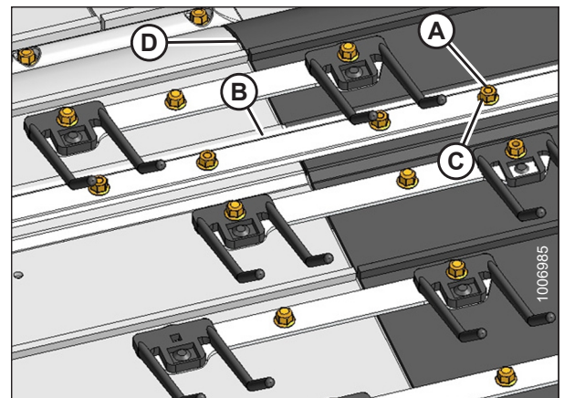
Figura 5.92: Correa de lona delantera
