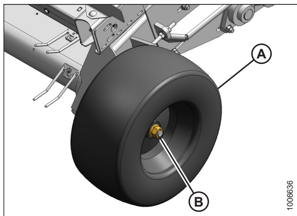
Figura 5.208: Rueda: lado izquierdo de la plataforma
