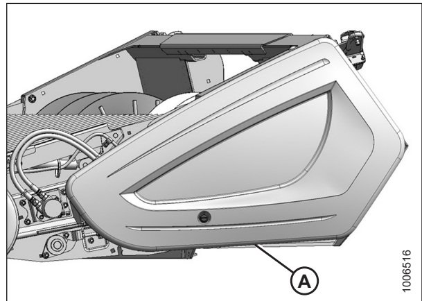
Figura 3.108: Tapa lateral izquierda
