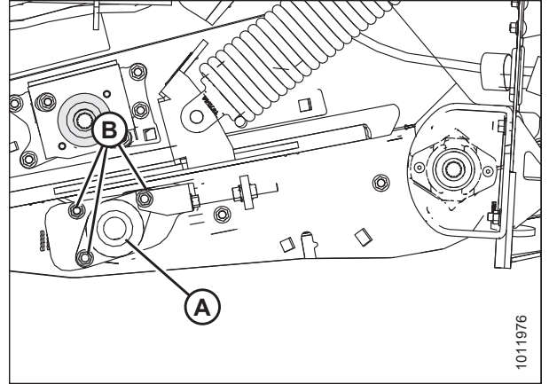
Figura 5.139: Rodillo tensor de la cama frontal del lado izquierdo
