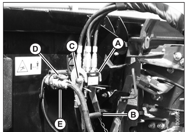
Figura 3.77: Acoplamiento del acoplador
