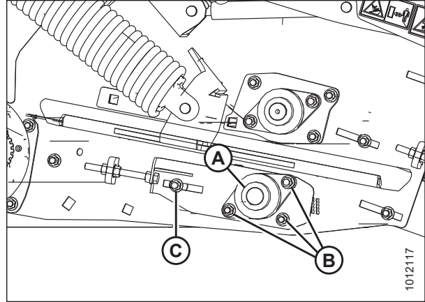
Figura 5.136: Rodillo tensor de la cama frontal del lado derecho
