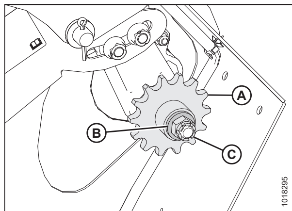
Figura 5.65: Piñón de mando
