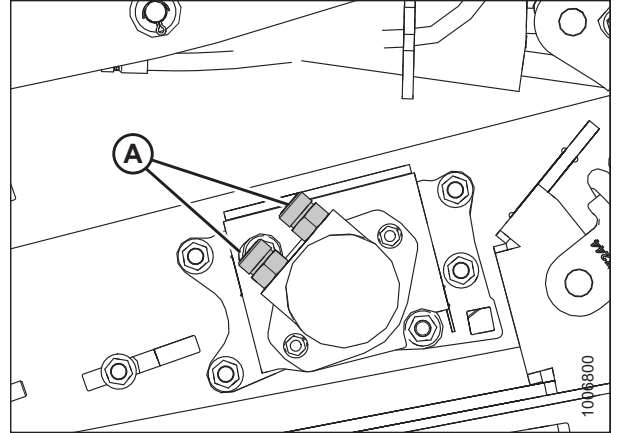
Figura 5.28: Accesorios hidráulicos
