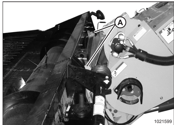
Figura 3.84: Desacoplamiento de la plataforma
