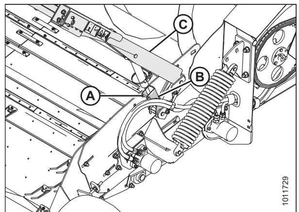
Figura 3.17: Traba de seguridad acoplada
