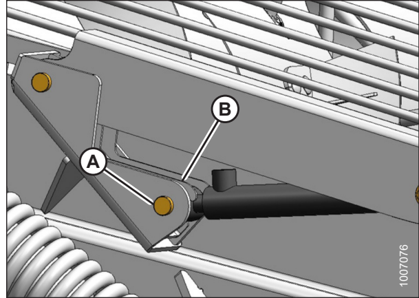
Figura 5.183: Cilindro secundario: lado derecho de la plataforma
