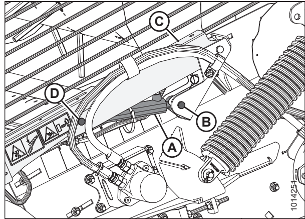
Figura 5.180: Cilindro maestro: lado izquierdo de la plataforma
