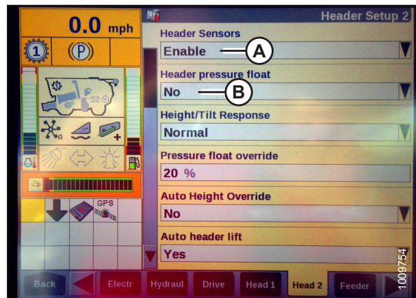
Figura 4.56: Pantalla de la cosechadora Case IH
