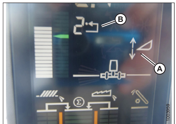
Figura 4.100: Pantalla de la cosechadora
