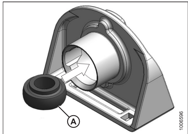
Figura 5.115: Soporte de rodamiento
