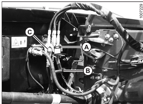
Figura 3.78: Liberación del acoplador
