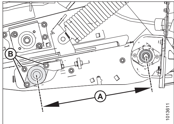
Figura 5.138: Se muestra la cama frontal de lado izquierdo; lado derecho opuesto.
