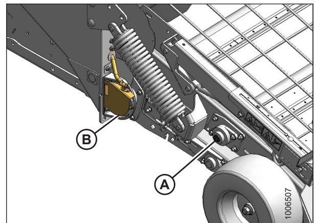
Figura 3.86: Rodillo de la lona y sensor de velocidad
