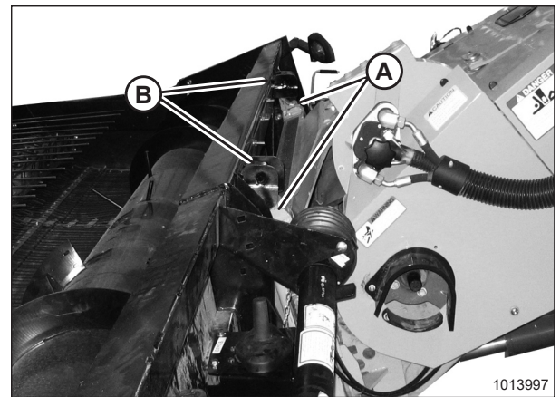
Figura 3.66: Plataforma de recolección
