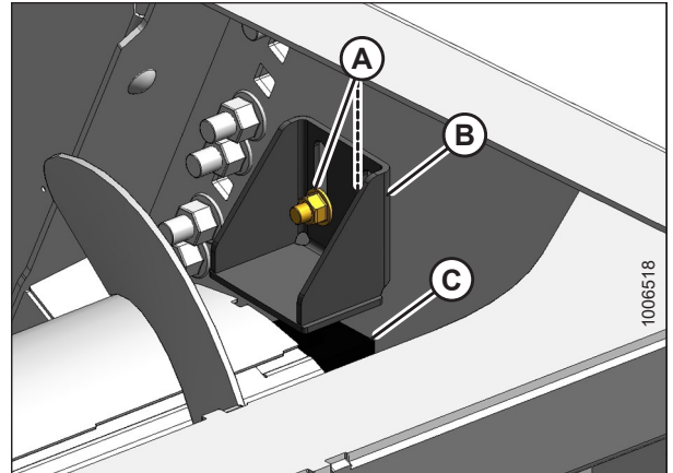
Figura 3.97: Tope derecho
