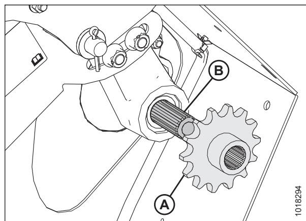
Figura 5.64: Piñón de mando
