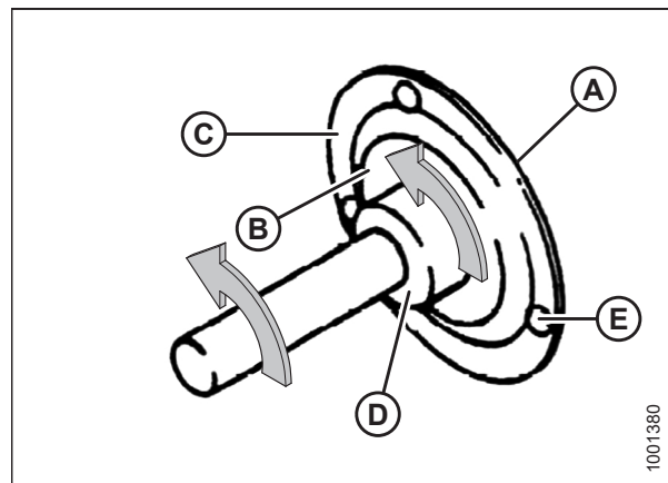
Figura 5.4: Rodamiento sellado
