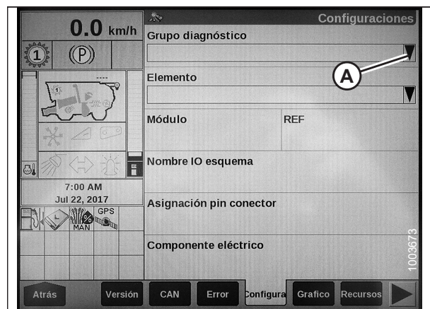
Figura 4.102: Pantalla de la cosechadora New Holland
