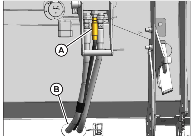
Figura 5.200: Hoja posterior izquierda
