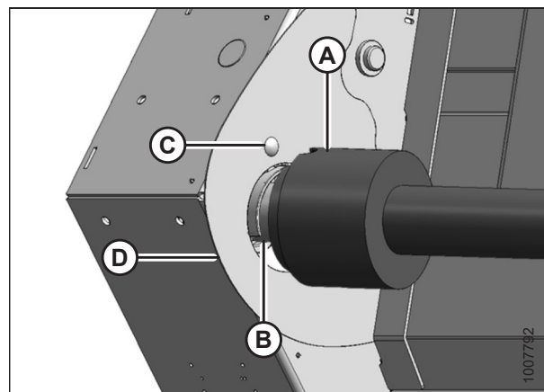
Figura 5.7: Extremo de la plataforma del cardán
