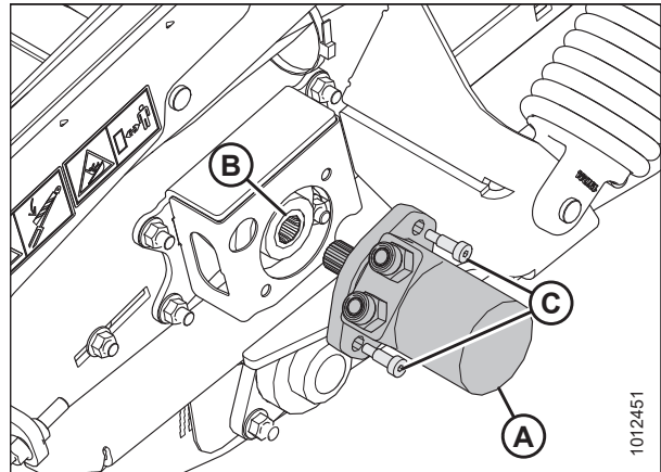
Figura 5.26: Motor hidráulico delantero; lado izquierdo
