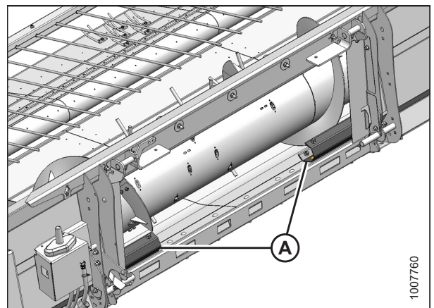
Figura 3.99: Placas de alimentación
