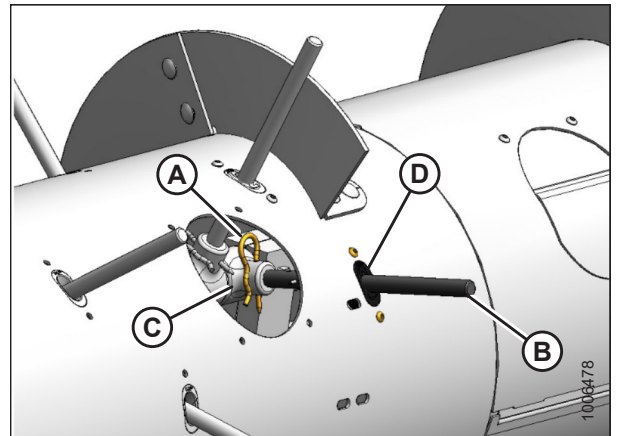
Figura 5.69: Dedos del sinfín
