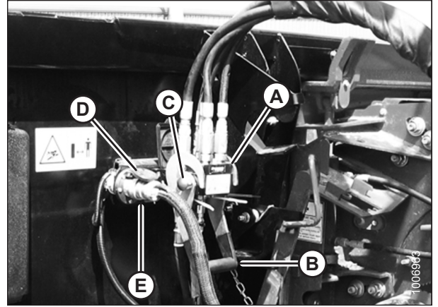
Figura 3.25: Acoplamiento del acoplador
