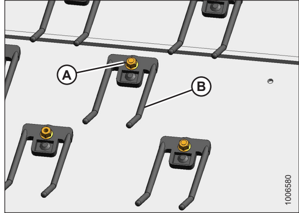
Figura 5.105: Dedos de la lona
