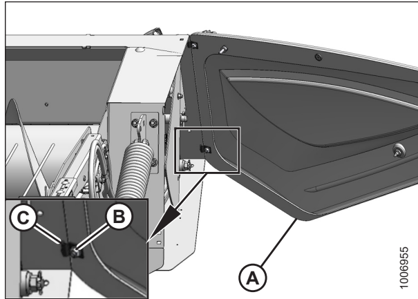
Figura 3.8: Extracción de la tapa lateral
