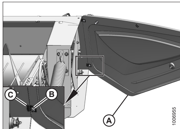
Figura 3.5: Ajuste de la tapa lateral
