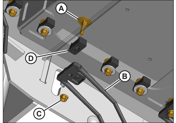
Figura 5.107: Guías de la lona
