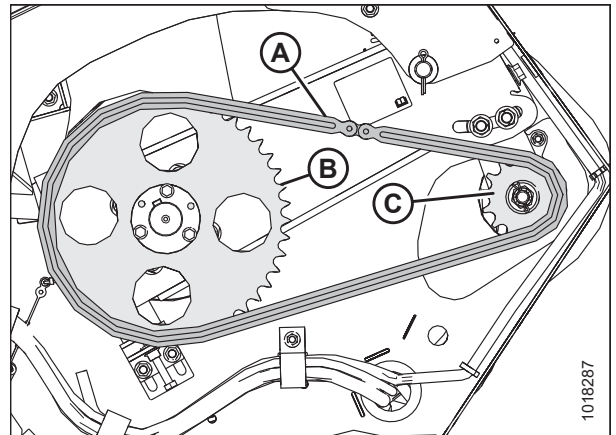
Figura 5.49: Cadena de mando del sinfín
