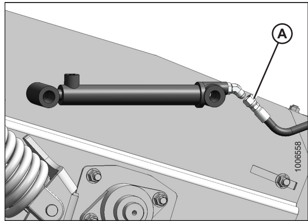
Figura 5.184: Cilindro secundario: lado derecho de la plataforma
