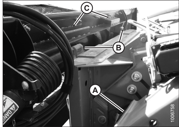
Figura 3.50: Desacoplamiento de la plataforma
