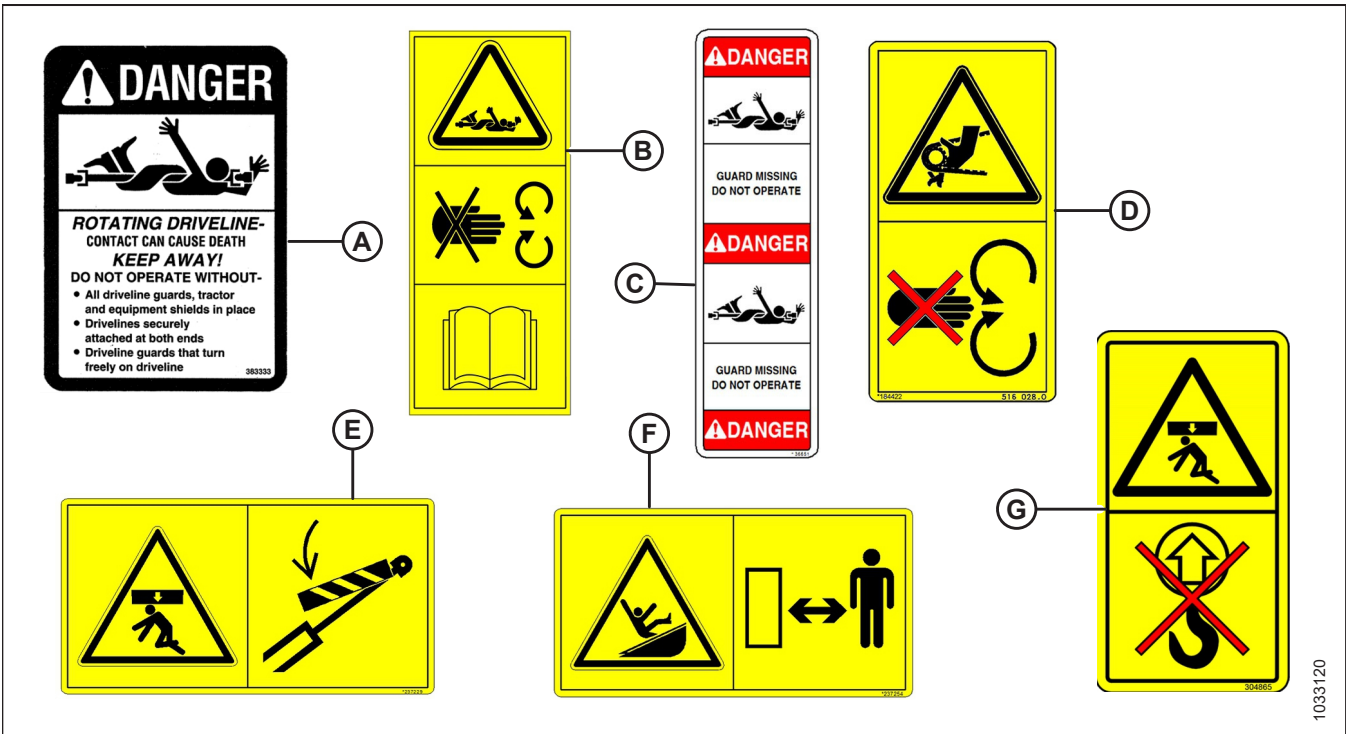
Figura 1.26: Calcomanías del cardán para cosechadora y del sujetador
