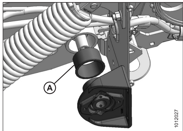
Figura 5.116: Cama trasera del lado izquierdo
