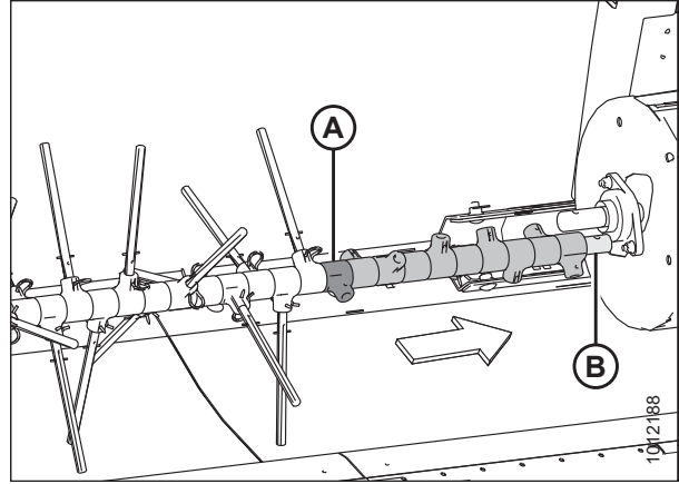
Figura 5.80: Sujetadores de dedos de sinfín del lado izquierdo
