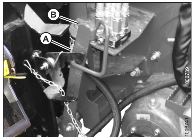
Figura 3.29: Almacenamiento del conector eléctrico
