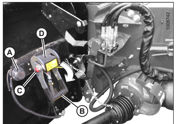
Figura 3.30: Bloqueo del multiacoplador
