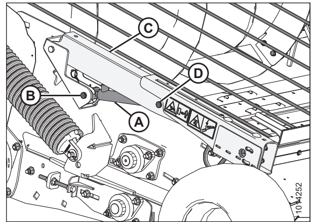
Figura 5.181: Cilindro secundario: lado derecho de la plataforma
