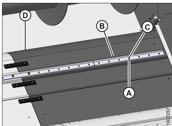
Figura 5.98: Correa de la lona trasera
