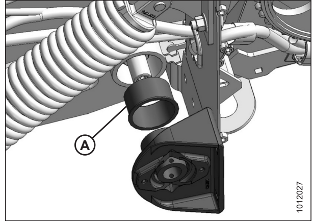
Figura 5.128: Se muestra el lado izquierdo; lado derecho opuesto.
