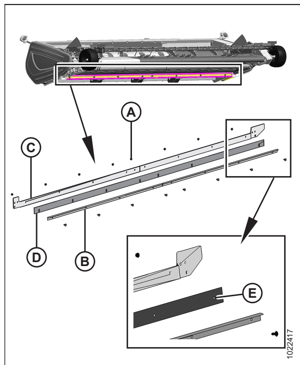
Figura 3.118: Ensamble del sello
