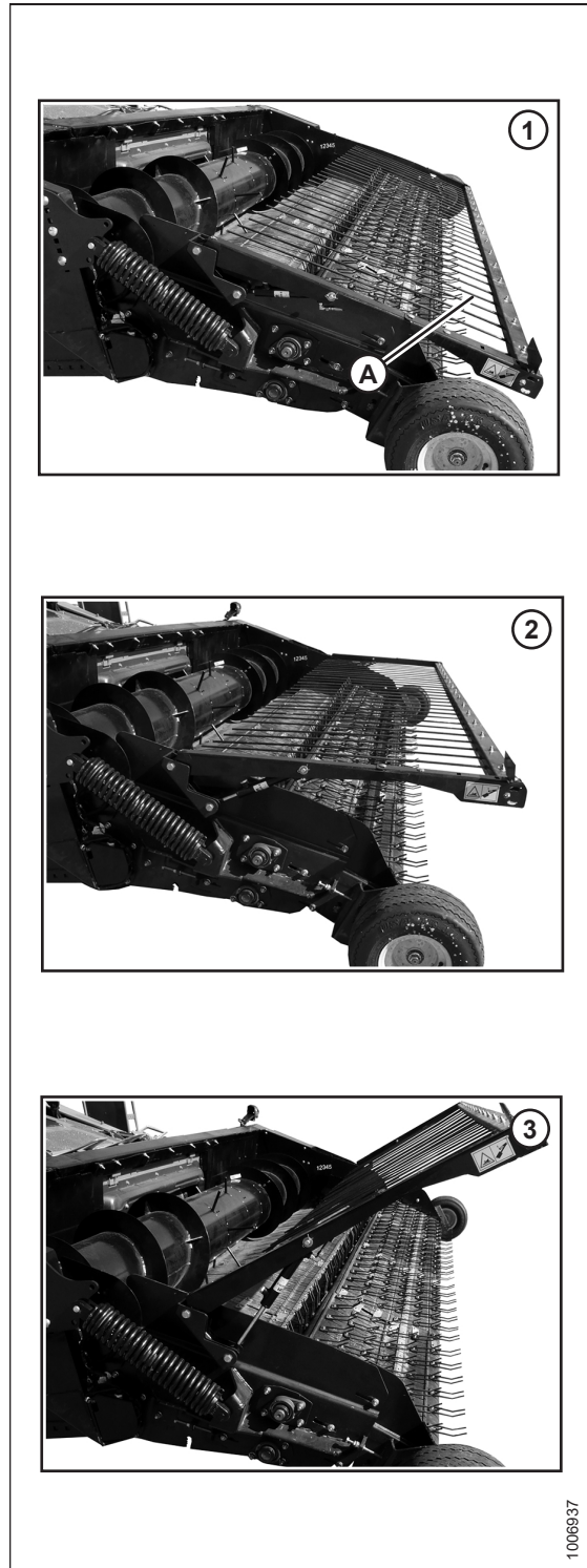
Figura 3.112: Posiciones del sujetador
