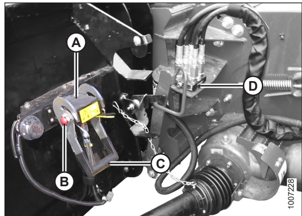
Figura 3.24: Bloqueo del acoplador
