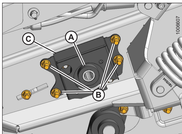
Figura 5.142: Cama delantera del lado izquierdo
