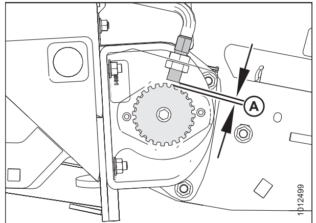
Figura 5.204: Separación de disco
