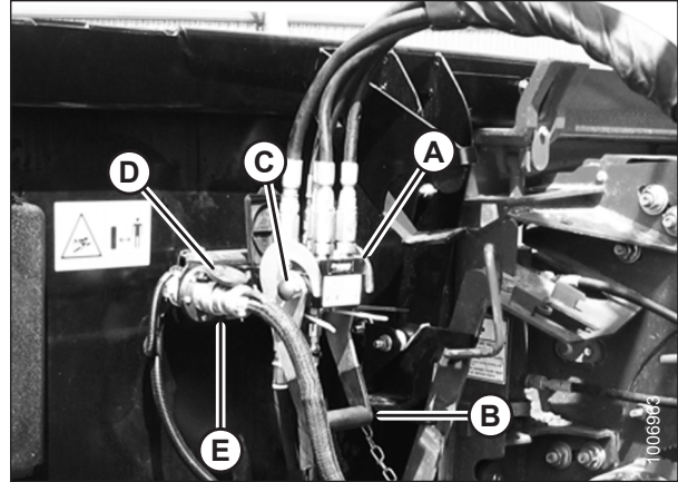
Figura 3.58: Acoplamiento del acoplador
