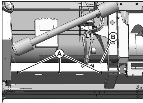
Figura 5.46: Cubierta de viga inferior
