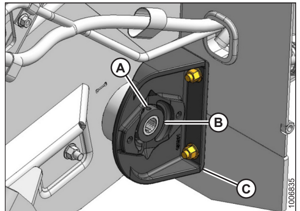
Figura 5.112: Cama trasera del lado izquierdo
