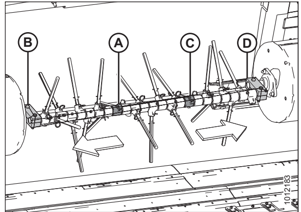
Figura 5.78: Dedos del sinfín
