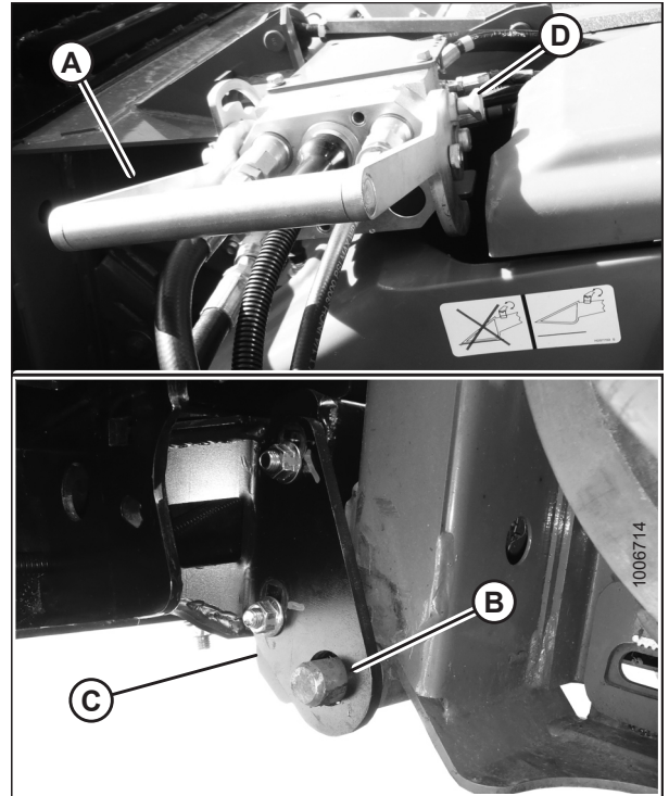
Figura 3.43: Bloqueo de embocador
