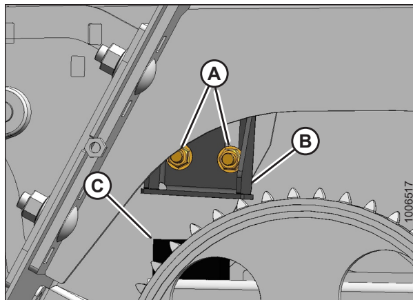
Figura 3.92: Tope izquierdo
