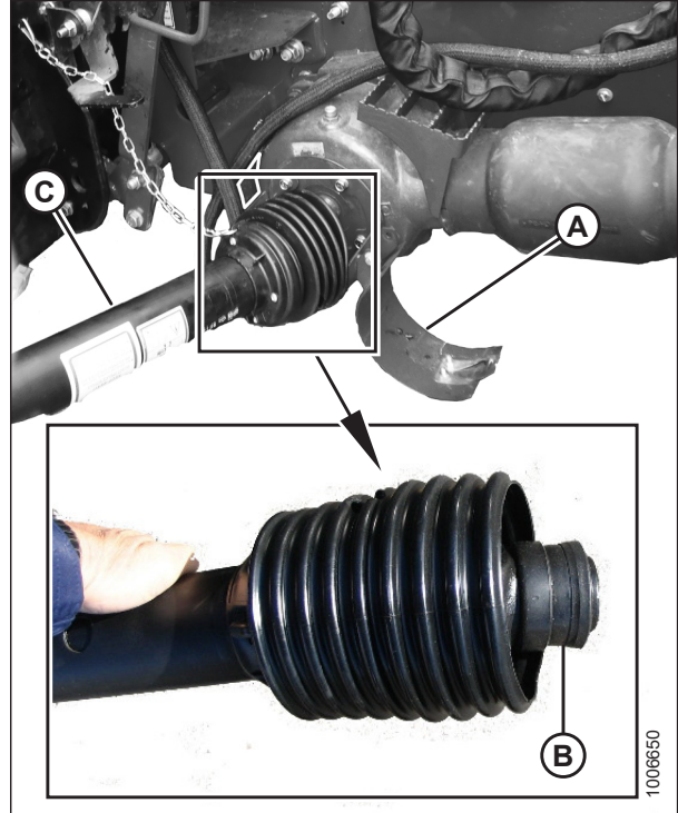
Figura 3.31: Desacoplamiento del cardán para cosechadora
