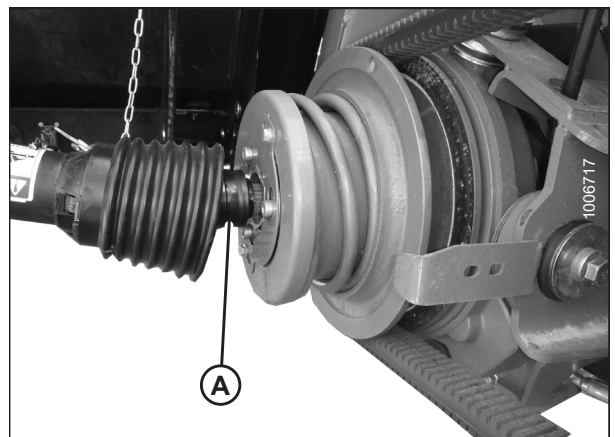
Figura 3.39: Acoplamiento del cardán a la cosechadora
