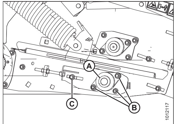
Figura 5.140: Rodillo tensor de la cama frontal del lado derecho
