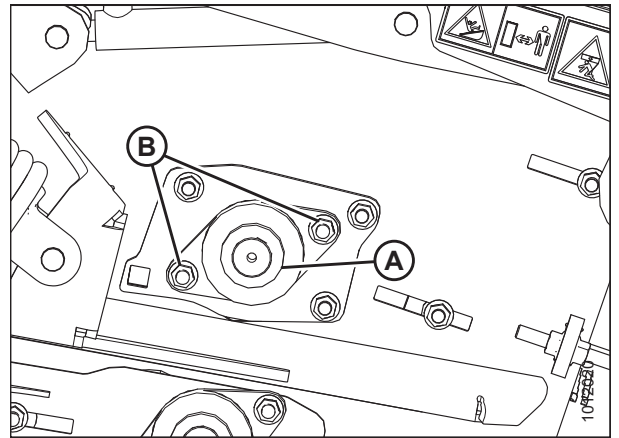
Figura 5.155: Rodillo de mando de la cama frontal del lado derecho
