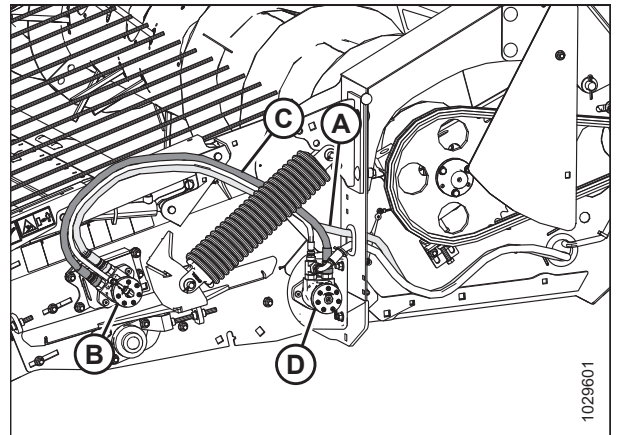
Figura 5.43: Lado izquierdo de la plataforma:
