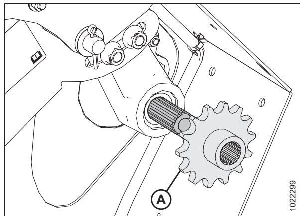
Figura 5.63: Piñón de mando
