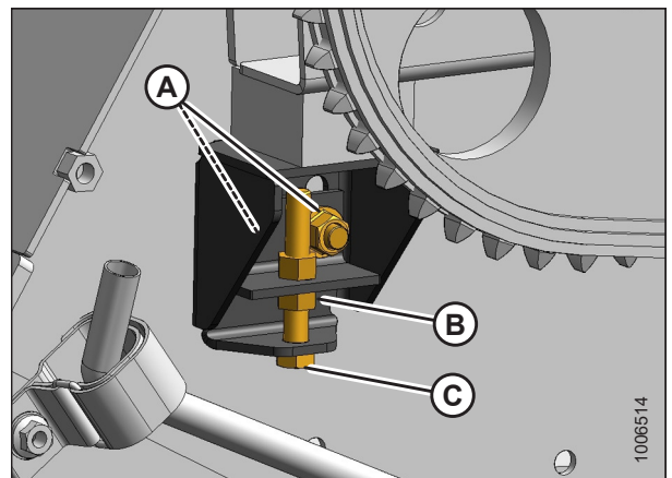
Figura 3.89: Tope izquierdo del sinfín
