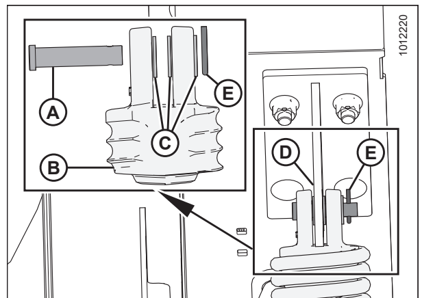
Figura 3.111: Se muestra el ensamble del resorte de flotación del lado izquierdo; lado derecho opuesto.
