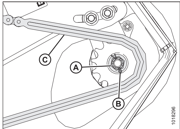
Figura 5.67: Piñón de mando
