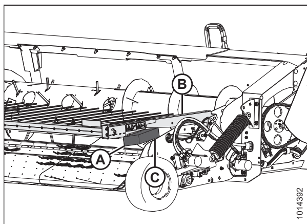
Figura 5.175: Ubicación de bloques
