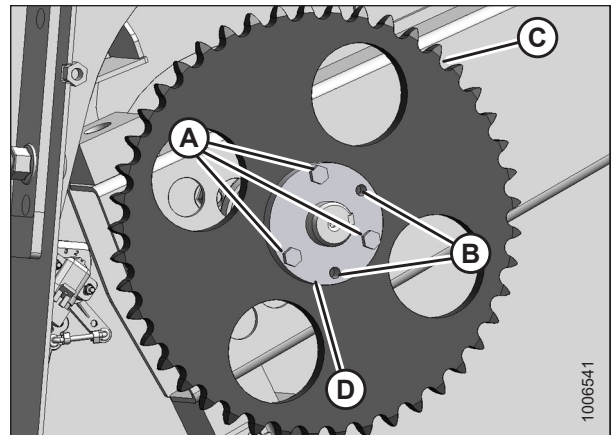
Figura 5.54: Piñón de mando
