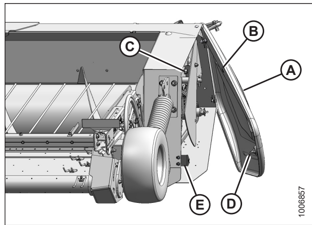
Figura 3.4: Tapa lateral
