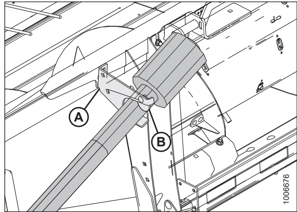
Figura 3.54: Mando en posición de almacenamiento
