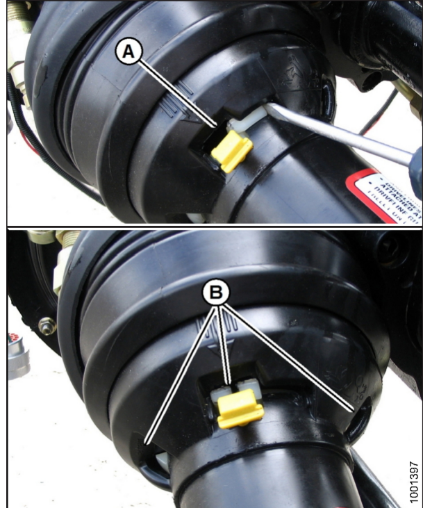
Figura 5.17: Protección del mando
