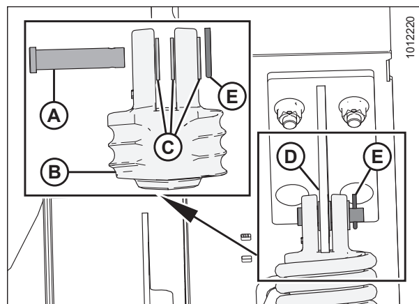
Figura 5.168: Se muestra el ensamble del resorte de flotación del lado izquierdo; lado derecho opuesto.
