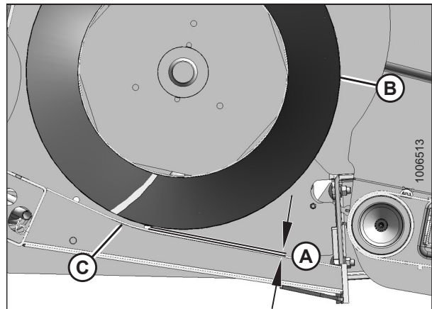
Figura 3.87: Separación entre el sinfín y la bandeja
