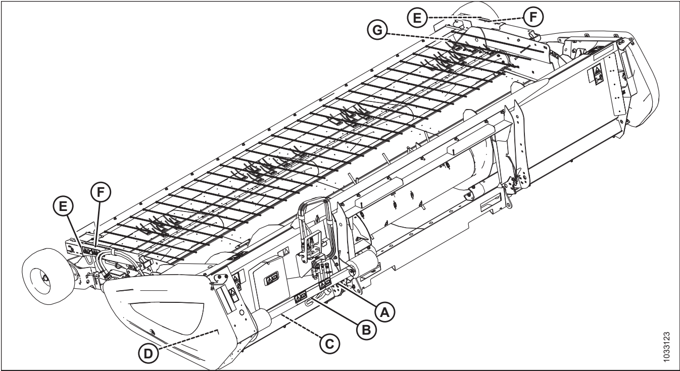
Figura 1.25: Calcomanías del cardán para cosechadora y del sujetador – John Deere
