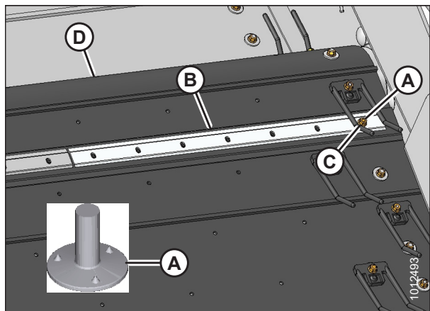
Figura 5.95: Correa de la lona trasera
