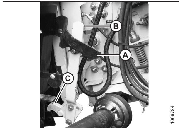
Figura 3.64: Desacoplamiento de la plataforma
