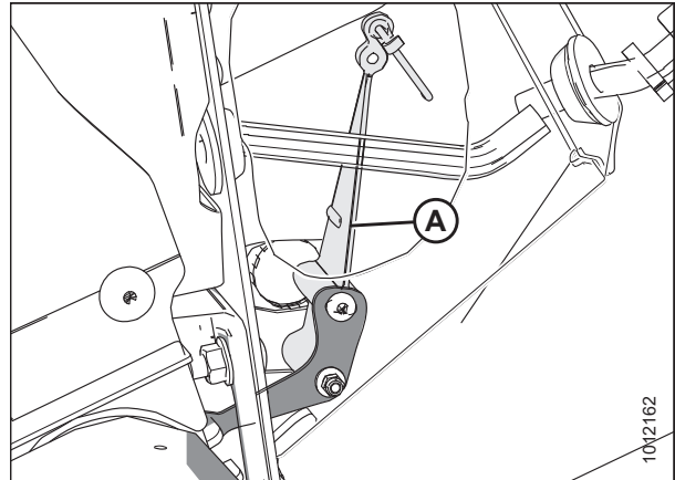
Figura 4.12: Ensamble del sensor de altura de la plataforma; lado derecho
