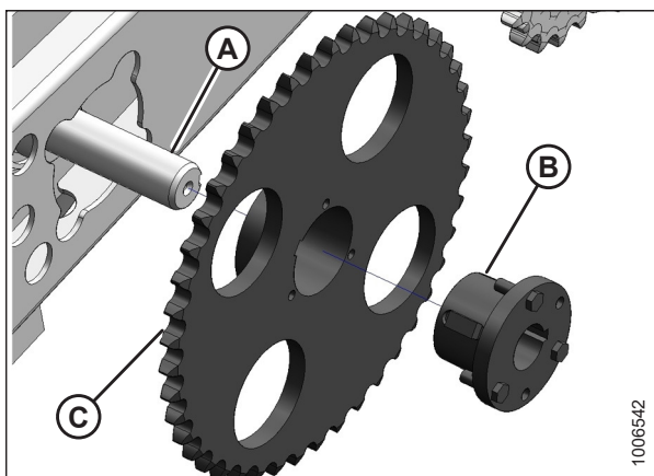
Figura 5.55: Piñón de mando
