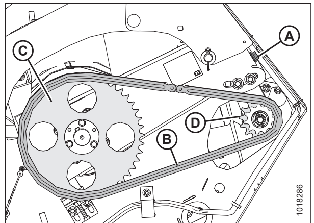
Figura 5.48: Cadena de mando del sinfín
