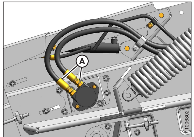
Figura 5.29: Mangueras hidráulicas
