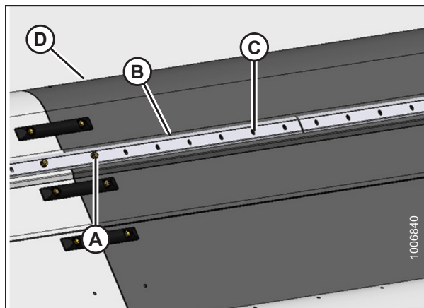
Figura 5.99: Correa de lona trasera
