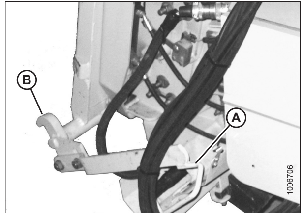
Figura 3.51: Trabas del embocador
