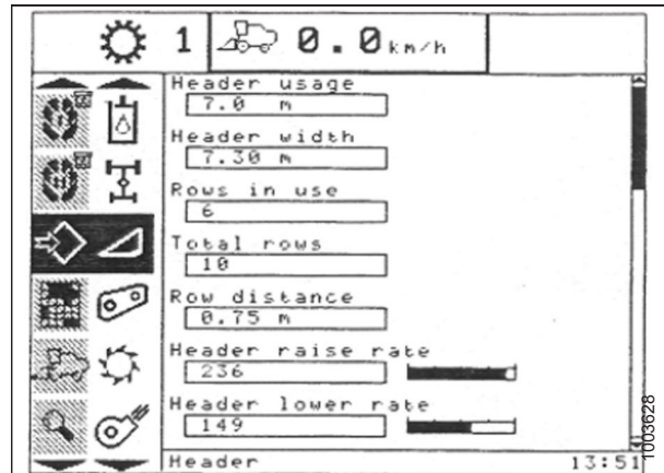
Figura 4.111: Pantalla de la cosechadora New Holland
