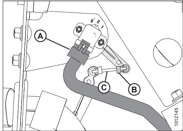
Figura 4.3: Ensamblaje del sensor de altura de la plataforma; lado izquierdo
