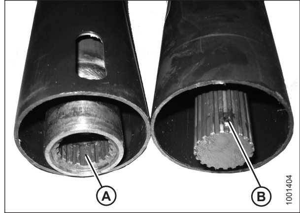
Figura 5.22: Ranuras del cardán para cosechadora
