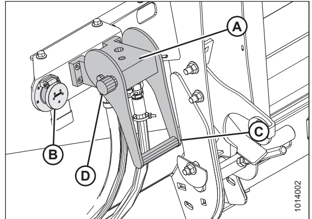
Figura 3.80: Bloqueo del multiacoplador
