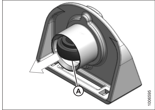
Figura 5.114: Soporte de rodamiento
