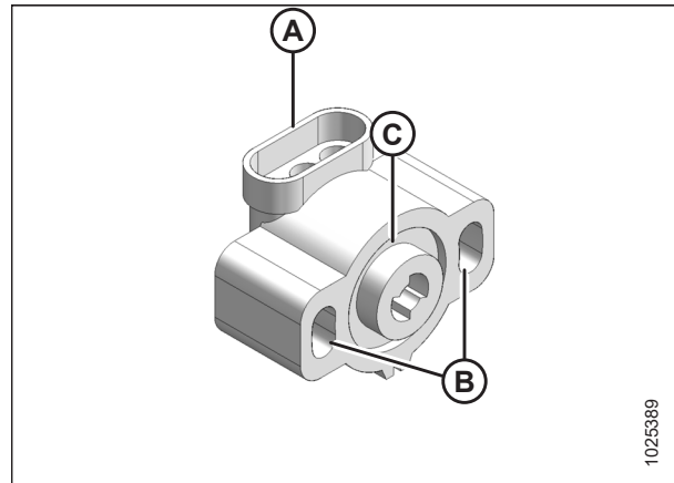
Figura 4.1: Sensor de tipo de resistencia variable
