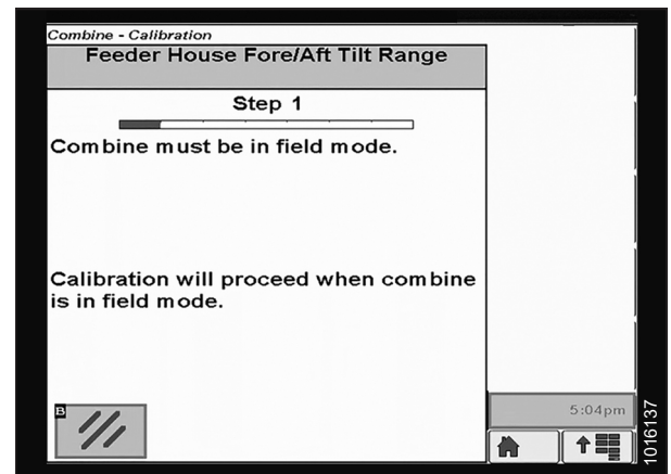
Figura 4.85: Pantalla de la cosechadora John Deere
