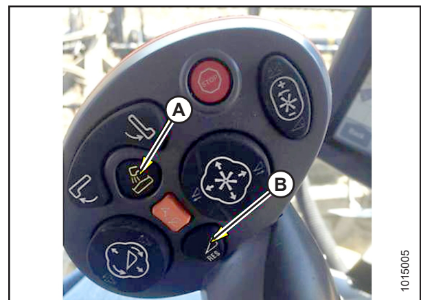
Figura 4.117: Controles de la cosechadora New Holland
