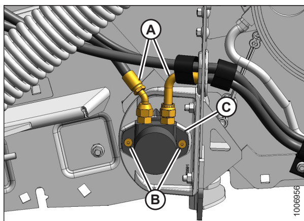
Figura 5.31: Motor hidráulico trasero; lado izquierdo
