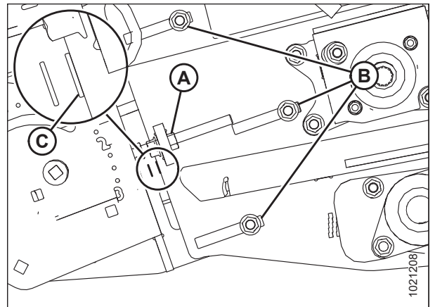
Figura 5.156: Cama delantera de lado izquierdo; lado derecho opuesto
