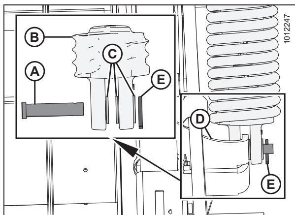
Figura 5.166: Se muestra el ensamble del resorte de flotación del lado izquierdo; lado derecho opuesto.
