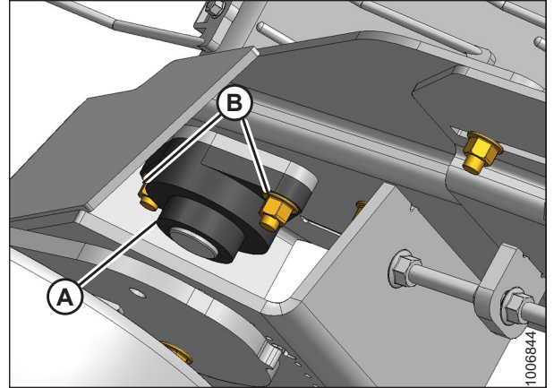
Figura 5.159: Rodillo tensor de la cama frontal
