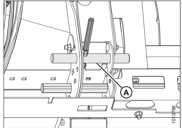
Figura 3.65: Clavijas de bloqueo replegadas
