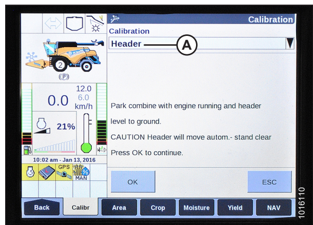
Figura 4.128: Pantalla de la cosechadora New Holland
