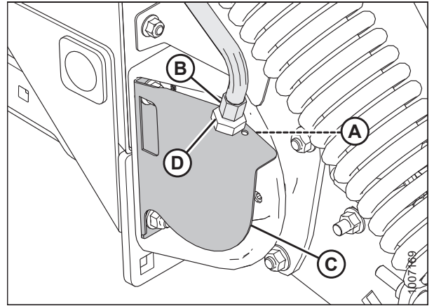
Figura 5.207: Sensor de velocidad de lonas
