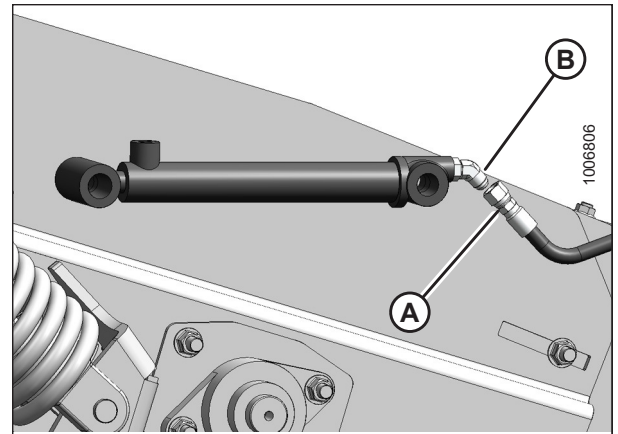
Figura 5.186: Cilindro secundario: lado derecho de la plataforma
