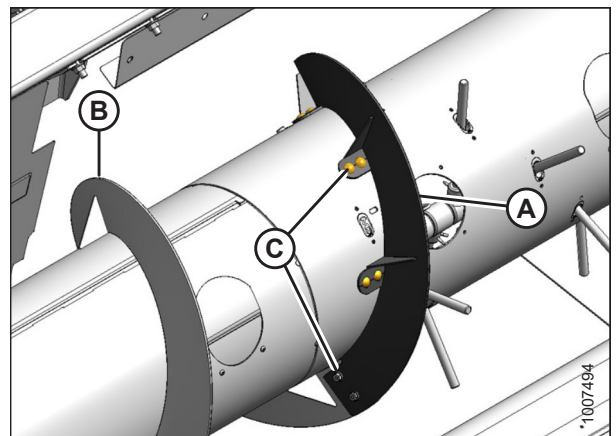
Figura 5.88: Extensión de las alas
