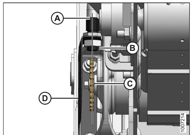
Figura 5.205: Alineación de sensor y disco
