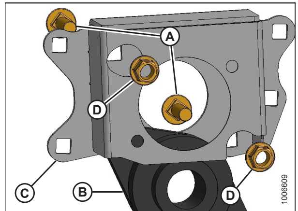
Figura 5.144: Cama delantera del lado izquierdo
