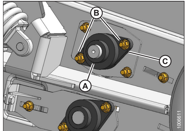
Figura 5.147: Cama delantera del lado derecho
