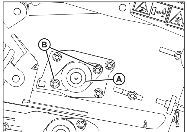
Figura 5.160: Rodillo de mando de la cama frontal del lado derecho
