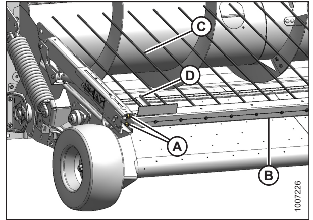
Figura 3.113: Barras del sujetador
