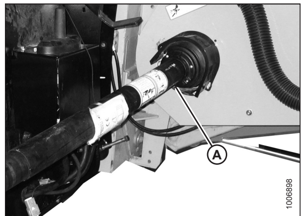
Figura 3.81: Desacoplamiento del cardán para cosechadora
