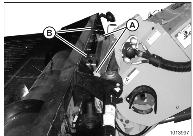
Figura 3.72: Plataforma de recolección
