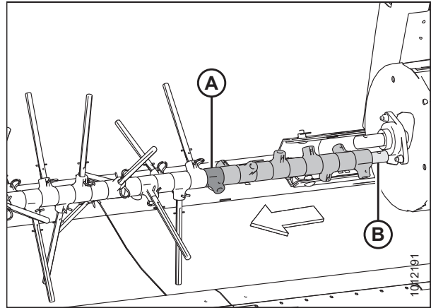
Figura 5.81: Sujetadores de dedos de sinfín del lado izquierdo
