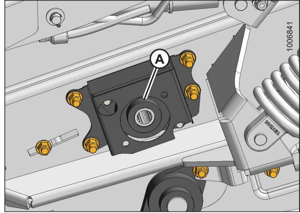
Figura 5.146: Cama delantera del lado izquierdo
