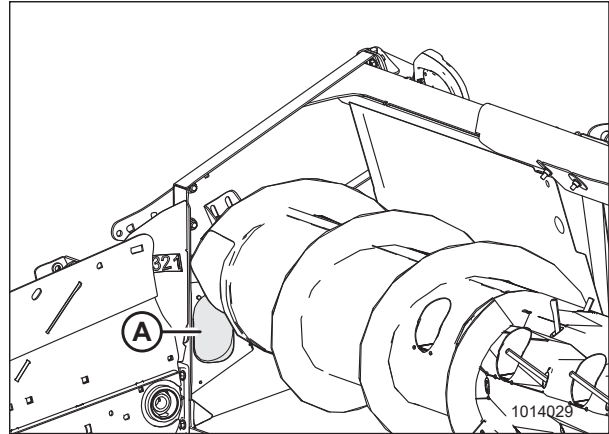
Figura 4.22: Panel de acceso: lado derecho
