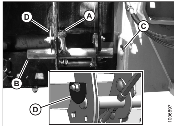
Figura 3.67: Bloqueo del embocador
