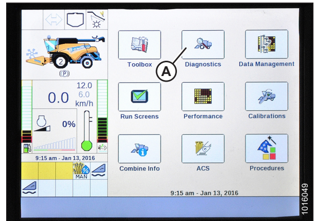
Figura 4.122: Pantalla de la cosechadora New Holland
