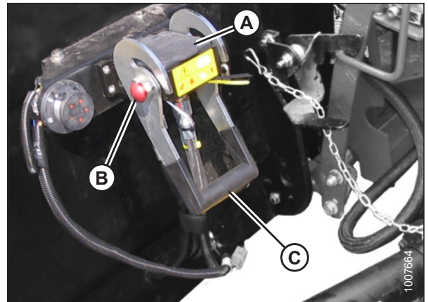
Figura 3.56: Receptáculo de la plataforma
