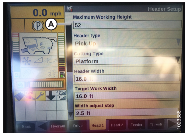
Figura 4.39: Pantalla de la cosechadora Case - Página de configuración de la plataforma
