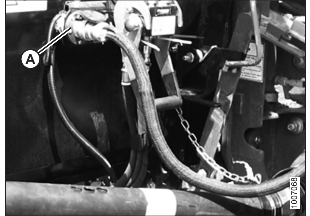
Figura 3.28: Conector eléctrico
