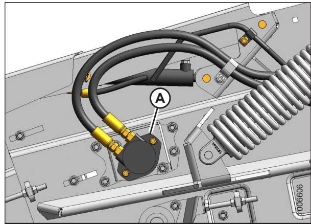
Figura 5.152: Motores hidráulicos delanteros
