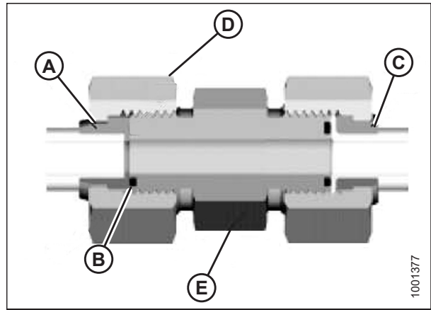
Figura 8.11: Accesorio hidráulico
