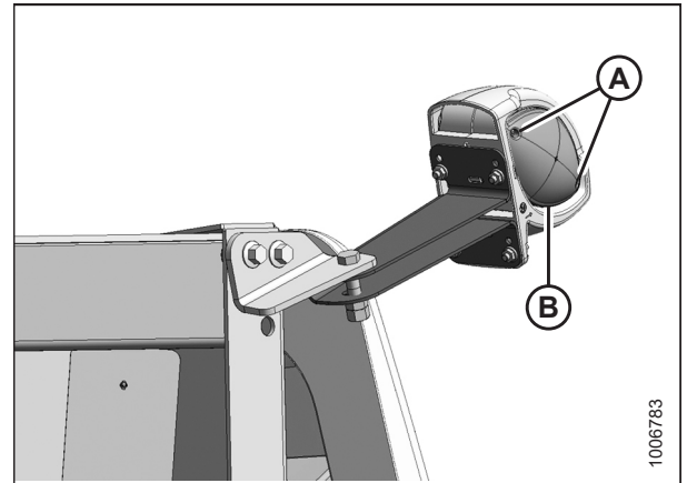
Figura 5.214: Luces de transporte
