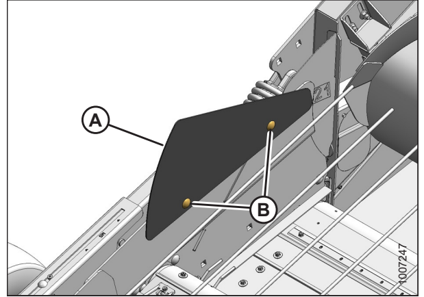
Figura 3.115: Deflector de cultivos
