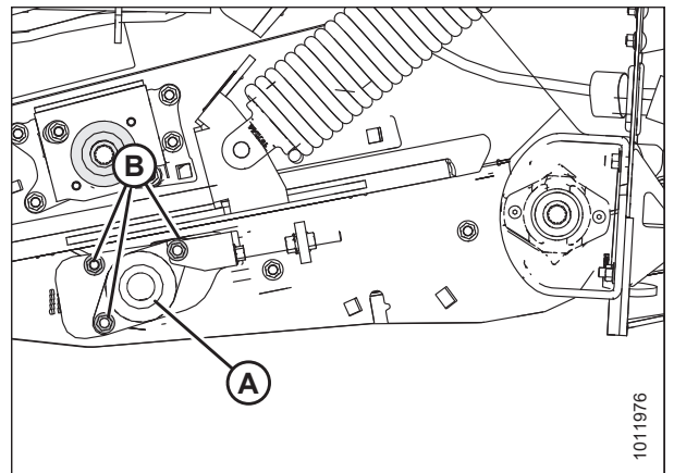
Figura 5.135: Rodillo tensor de la cama frontal del lado izquierdo
