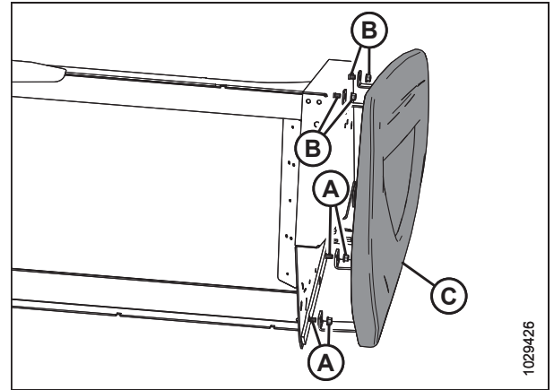
Figura 3.15: Tapa lateral derecha
