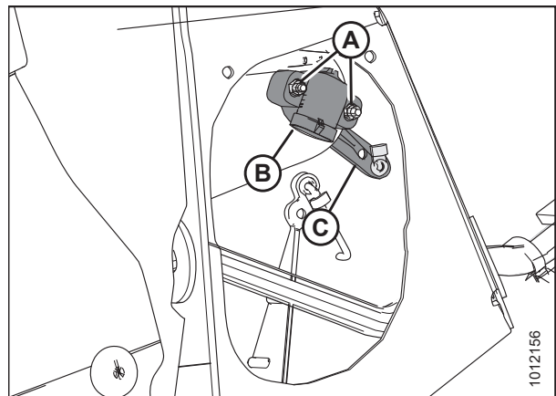
Figura 4.14: Ensamble del sensor de altura de la plataforma; lado derecho
