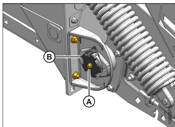
Figura 5.123: Cama trasera del lado derecho
