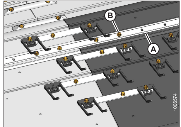
Figura 5.96: Correa de lona delantera
