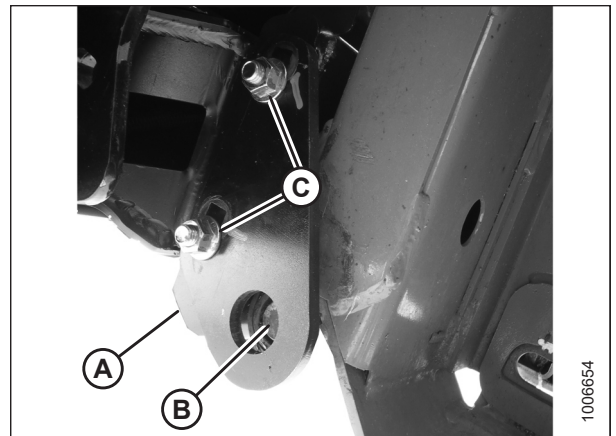
Figura 3.44: Alineación de placas de bloqueo
