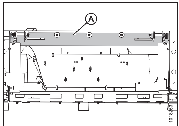
Figura 3.71: Viga superior - Vista posterior
