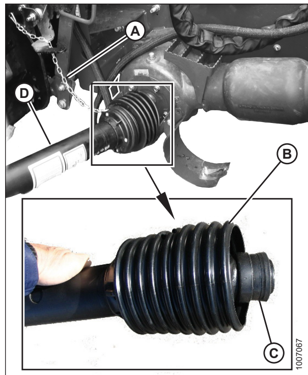
Figura 5.6: Extremo del mando de la cosechadora
