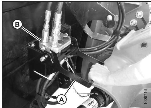
Figura 3.41: Liberación del acoplador
