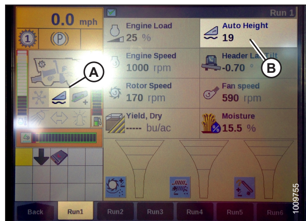
Figura 4.57: Pantalla de la cosechadora Case IH
