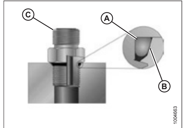
Figura 8.9: Accesorio hidráulico
