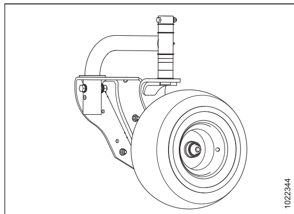
Figura 6.7: Kit de ruedas giratorias
