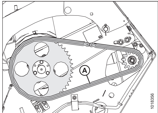
Figura 5.3: Cadena de mando del sinfín
