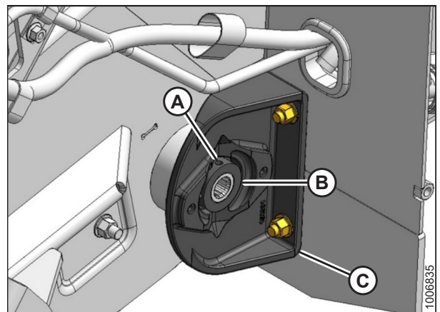
Figura 5.119: Cama trasera del lado izquierdo
