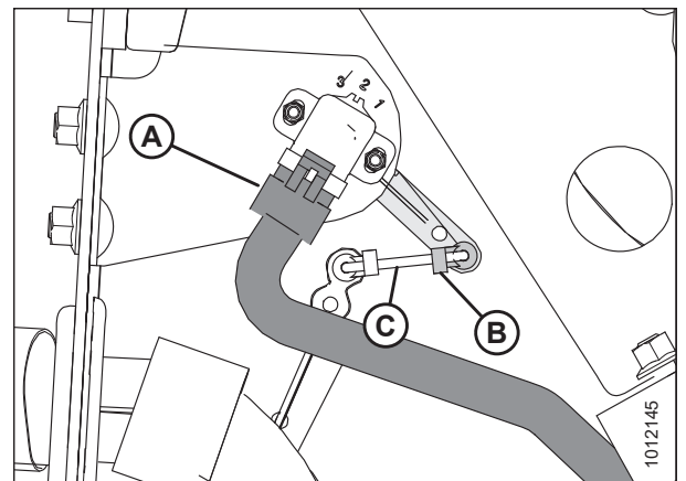
Figura 4.6: Ensamble del sensor de altura de la plataforma; lado izquierdo
