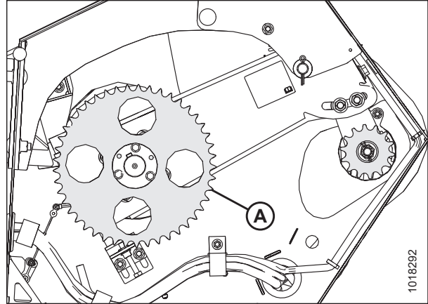
Figura 5.66: Piñón accionado
