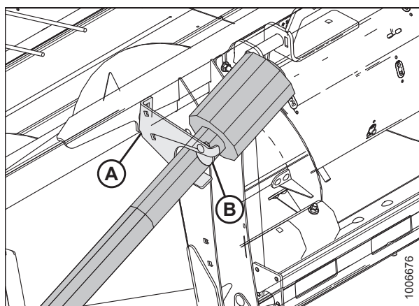
Figura 5.13: Extremo de la cosechadora del cardán en posición de almacenamiento
