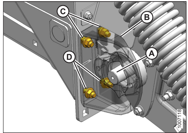
Figura 5.129: Cama trasera del lado derecho
