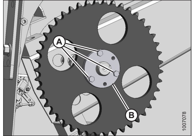
Figura 5.58: Piñón de mando
