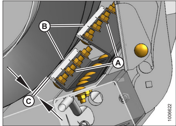
Figura 5.85: Separación de la placa de alimentación
