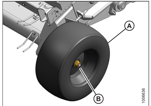
Figura 5.211: Rueda: lado izquierdo de la plataforma
