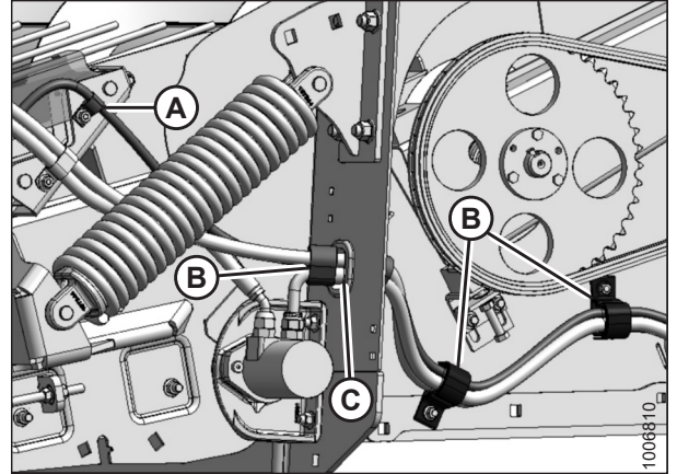
Figura 5.194: Cilindro maestro: lado izquierdo de la plataforma
