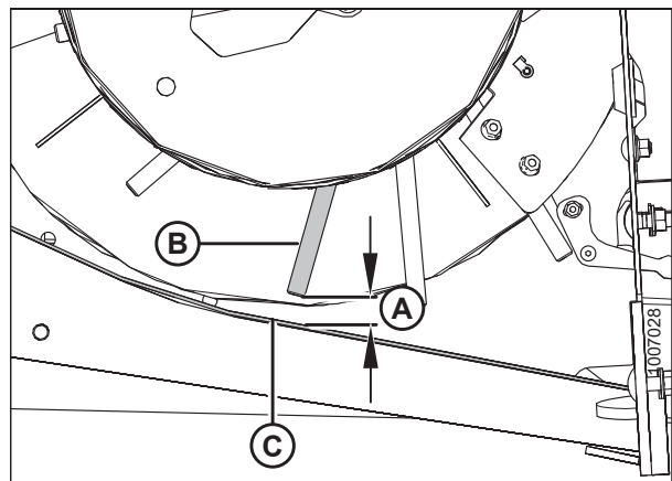
Figura 3.88: Separación entre el dedo y la bandeja
