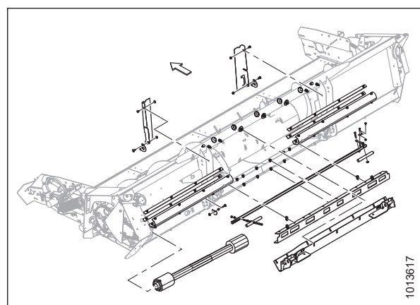
Figura 6.5: Kit de la cosechadora: Versatile
