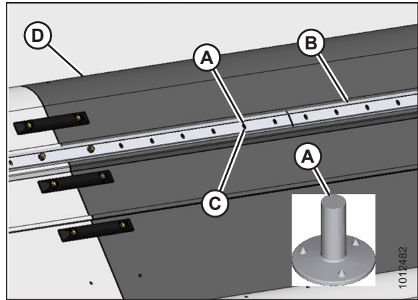
Figura 5.102: Correa de la lona trasera
