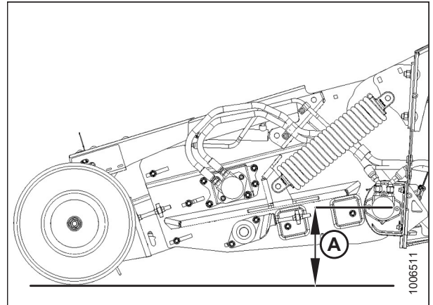
Figura 3.102: Altura de funcionamiento
