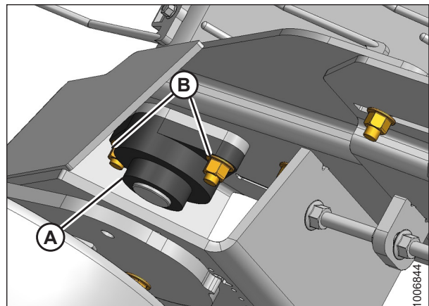
Figura 5.153: Rodillo tensor de la cama frontal
