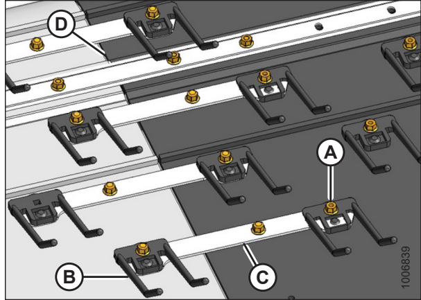
Figura 5.93: Correa de lona delantera
