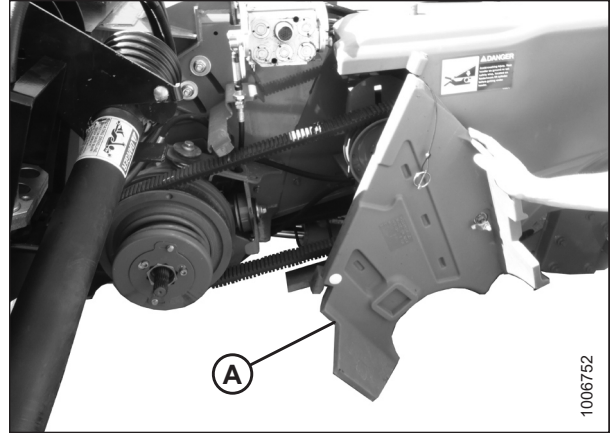
Figura 3.37: Protección del mando de la cosechadora
