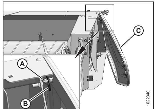
Figura 3.7: Extracción del soporte
