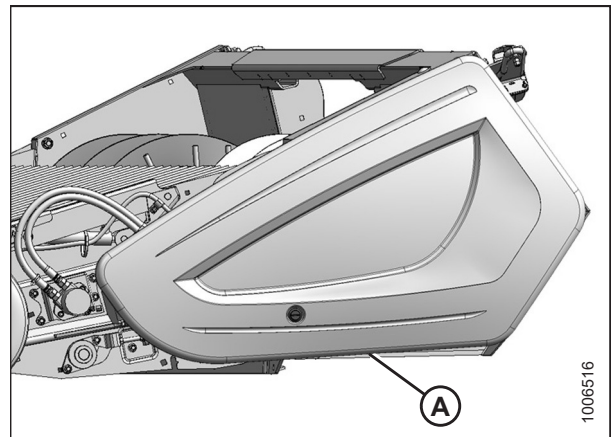
Figura 3.94: Tapa lateral izquierda
