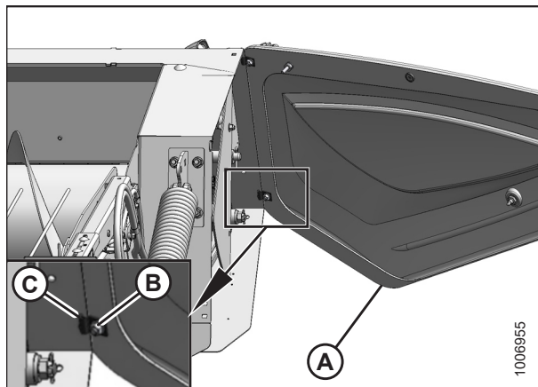
Figura 3.9: Acoplamiento de la tapa lateral
