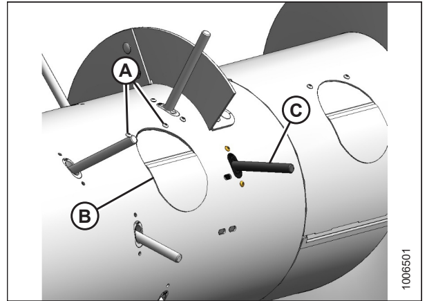
Figura 5.68: Cubierta de acceso
