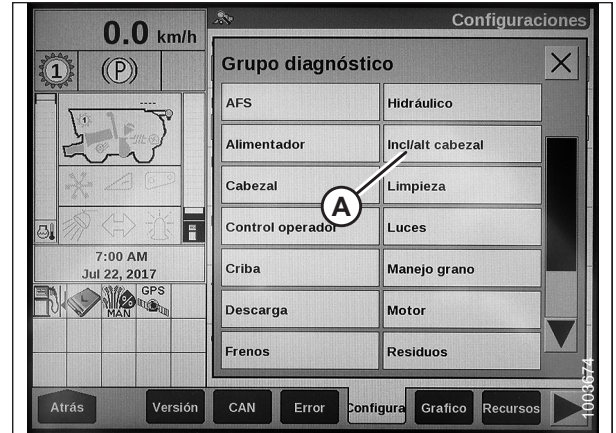
Figura 4.48: Pantalla de la cosechadora Case IH
