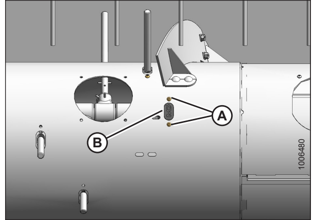
Figura 5.72: Guía de dedos del sinfín
