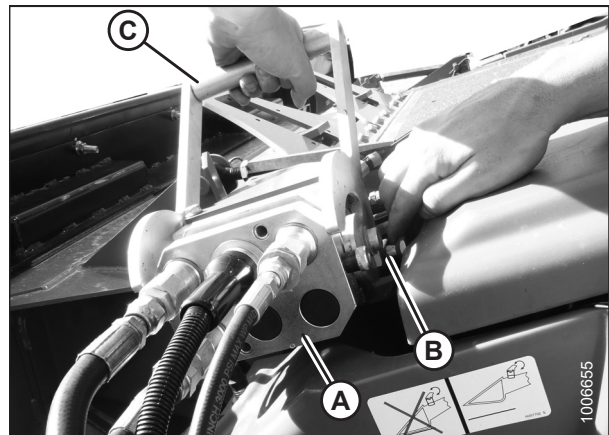
Figura 3.42: Acoplamiento del acoplador
