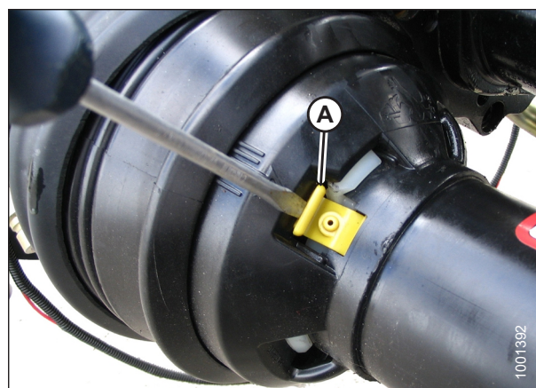
Figura 5.16: Protección del mando
