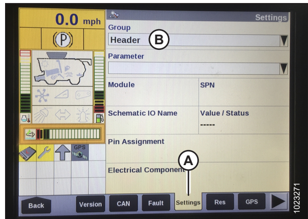
Figura 4.31: Pantalla de la cosechadora Case IH
