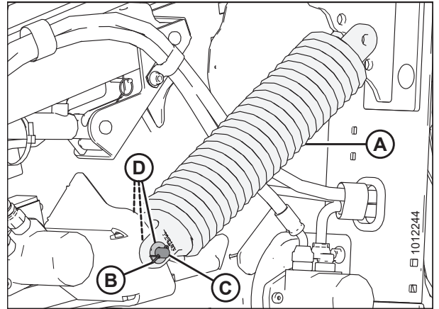
Figura 5.164: Se muestra el anclaje delantero del lado izquierdo; lado derecho opuesto.
