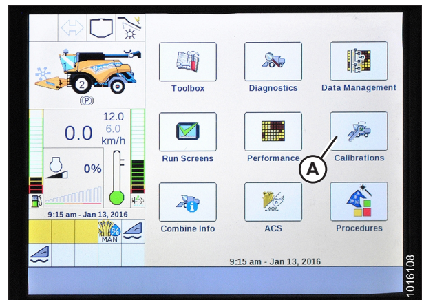
Figura 4.126: Pantalla de la cosechadora New Holland
