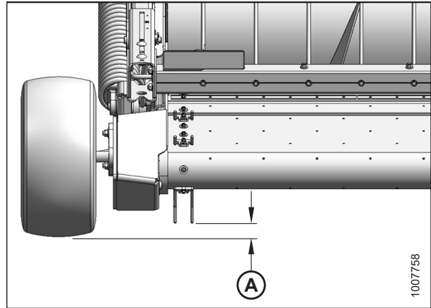
Figura 3.104: Altura de recolección
