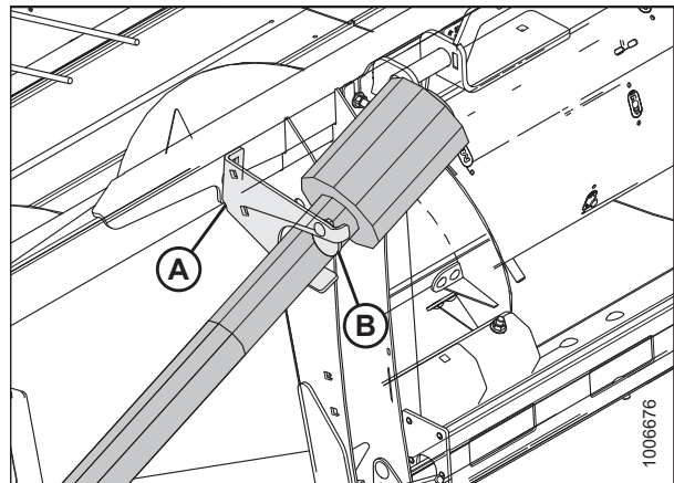
Figura 5.23: Extremo de la cosechadora del cardán en posición de almacenamiento
