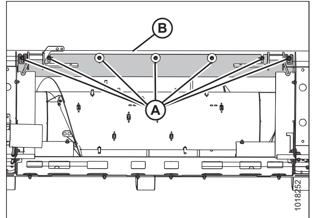
Figura 3.70: Viga superior - Vista posterior
