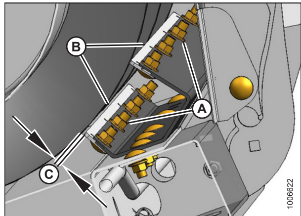
Figura 5.90: Separación de la placa de alimentación
