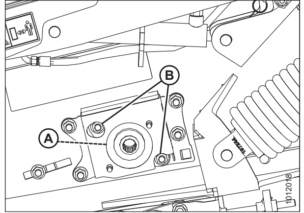
Figura 5.154: Rodillo de mando de la cama frontal del lado izquierdo
