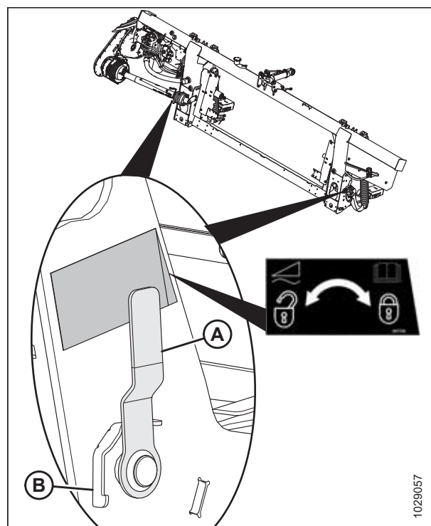
Figura 3.68: Traba de flotación de la plataforma en posición de bloqueo
