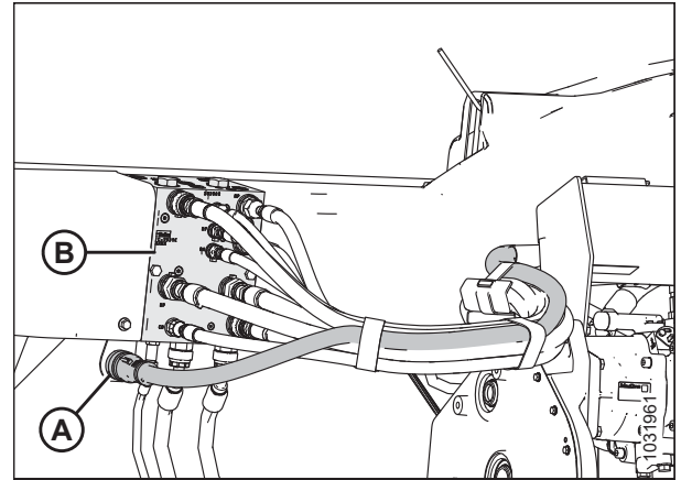
Figura 4.174: Conexiones de plataforma
