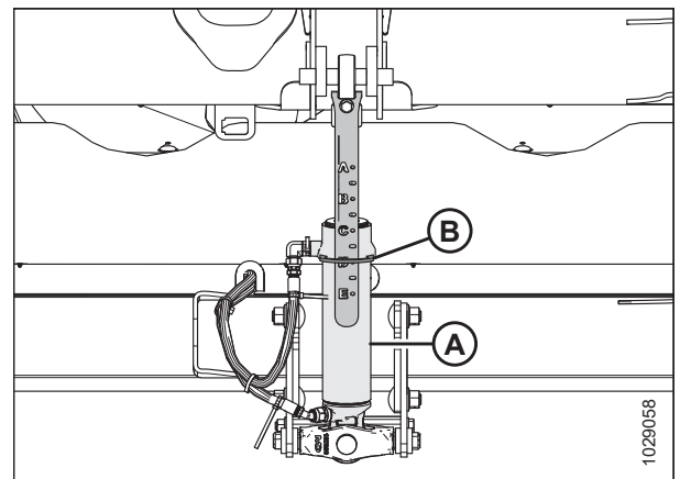
Figura 3.95: Unión central
