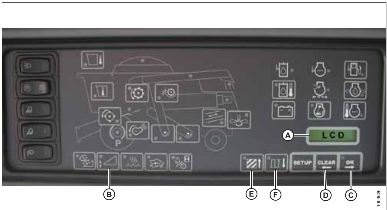
Figura 3.381: Panel de instrumentos electrónicos (EIP) de la cosechadora
