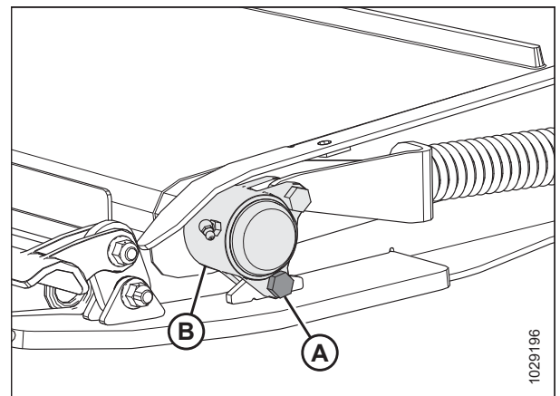
Figura 5.179: Rodillo tensor
