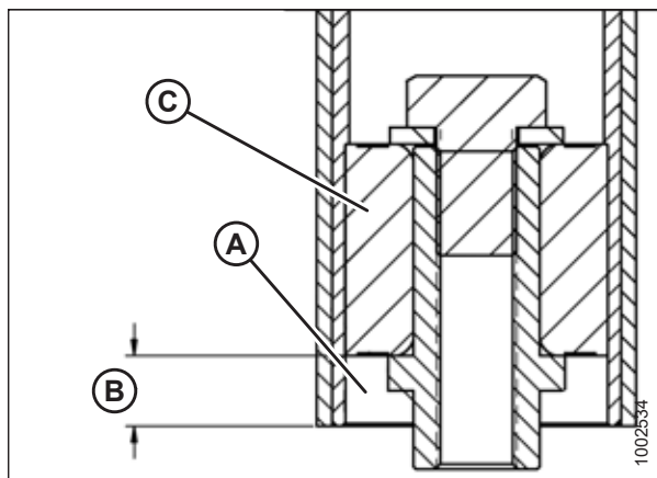
Figura 5.251: Rodamiento del rodillo tensor
