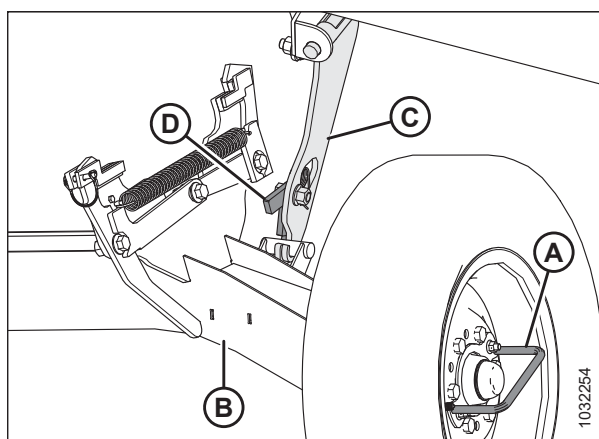
Figura 3.595: Eje de transporte derecho enganchedo en la posición de trabajo
