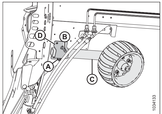
Figura 3.598: Ensamble de la rueda izquierda
