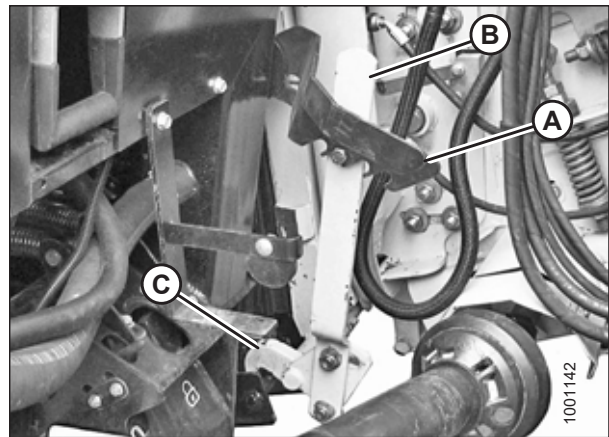
Figura 4.150: Trabas del embocador
