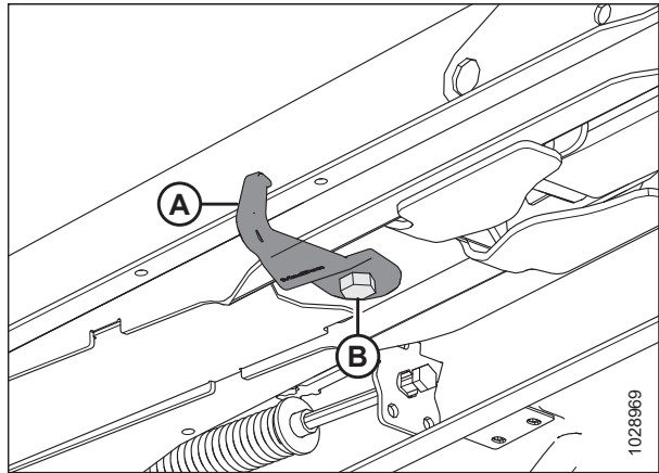
Figura 5.231: Gancho del soporte de unión en posición de almacenamiento
