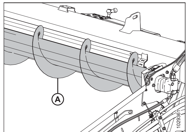
Figura 6.6: Sinfín superior
