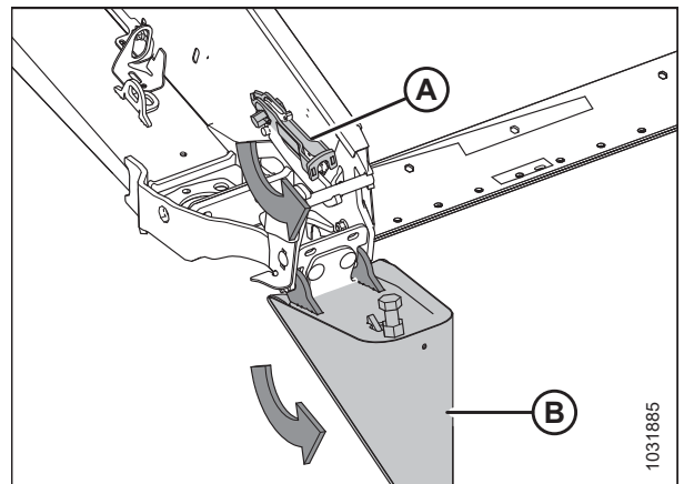
Figura 3.178: Divisor de cosecha con pestillo
