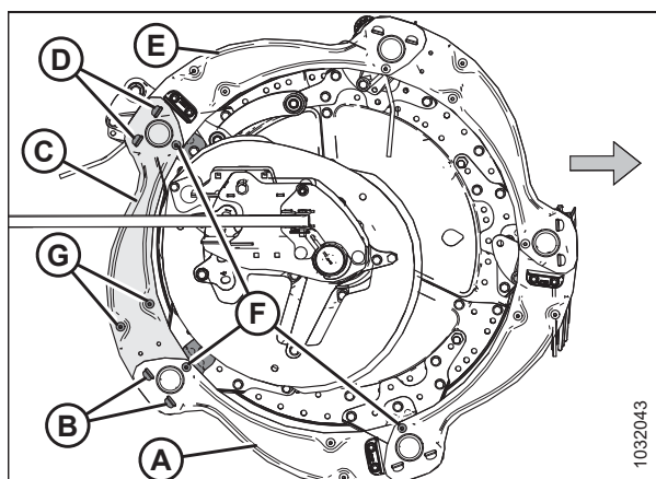
Figura 5.325: Tapas laterales del molinete: extremo de leva exterior
