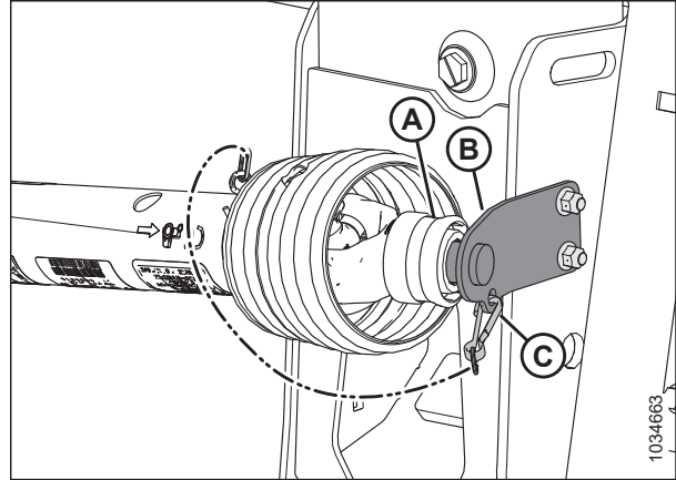
Figura 4.121: Cardán en posición de almacenamiento: Cardán MD n.º B7038 o MD n.º B7039
