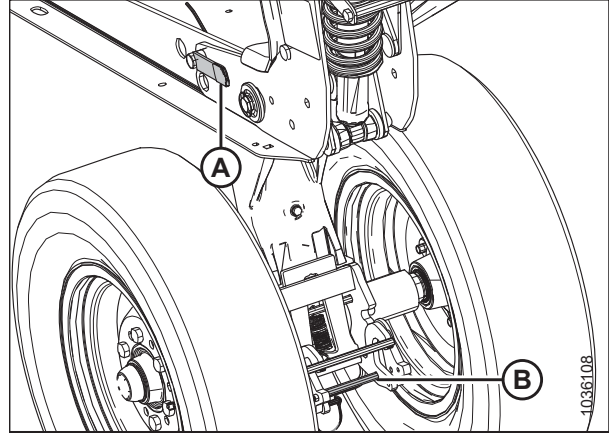
Figura 3.590: Ruedas de transporte izquierdas: pivote suelto
