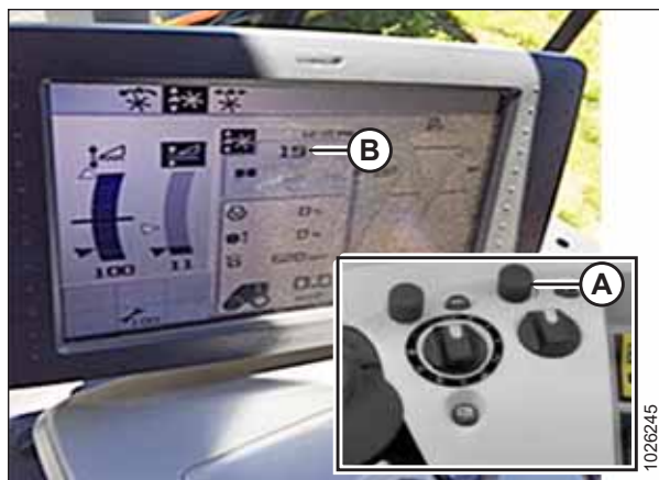
Figura 3.346: Pantalla y consola de la cosechadora CLAAS
