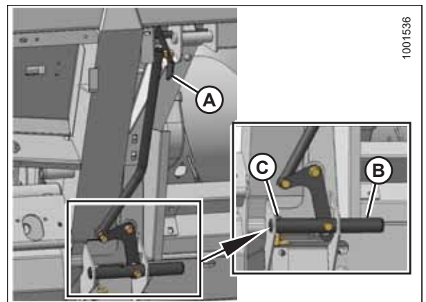
Figura 4.100: Enganche de las clavijas
