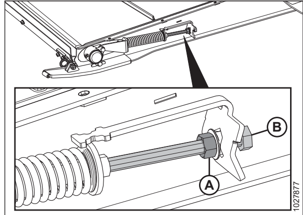
Figura 5.199: Tensor de la lona de alimentación
