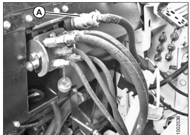
Figura 4.147: Conexiones del módulo de flotación
