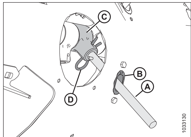
Figura 4.54: Dedo del sinfín
