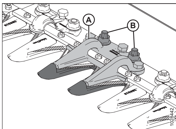
Figura 5.146: Puntón de cuchilla central puntiagudo
