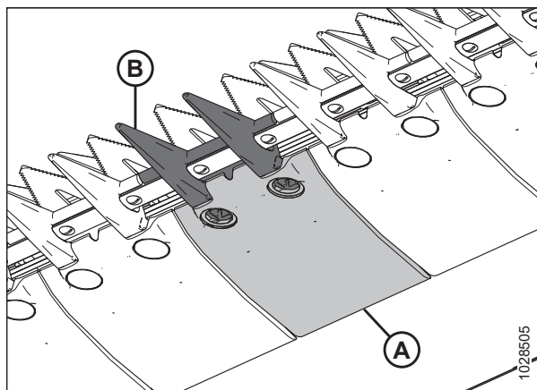
Figura 5.162: Puntón de cuchilla central y placa de desgaste
