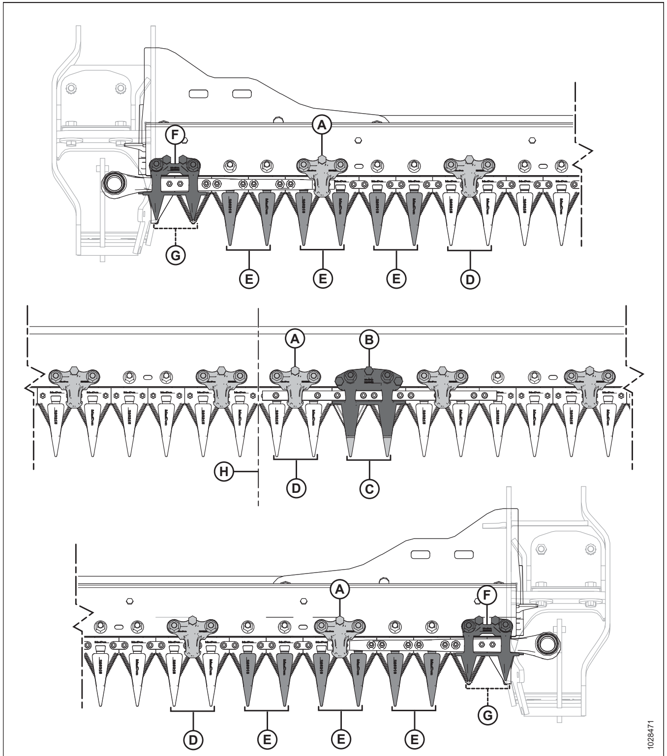
Figura 5.128: Puntón de cuchilla y ubicaciones del sujetador: plataforma de cuchilla doble FD245
