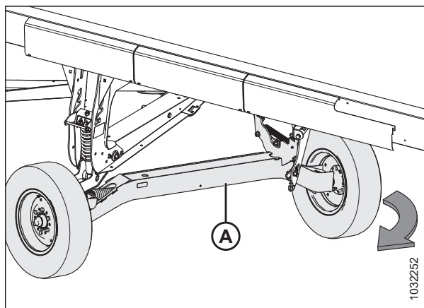
Figura 3.594: Rotación del eje de transporte derecho
