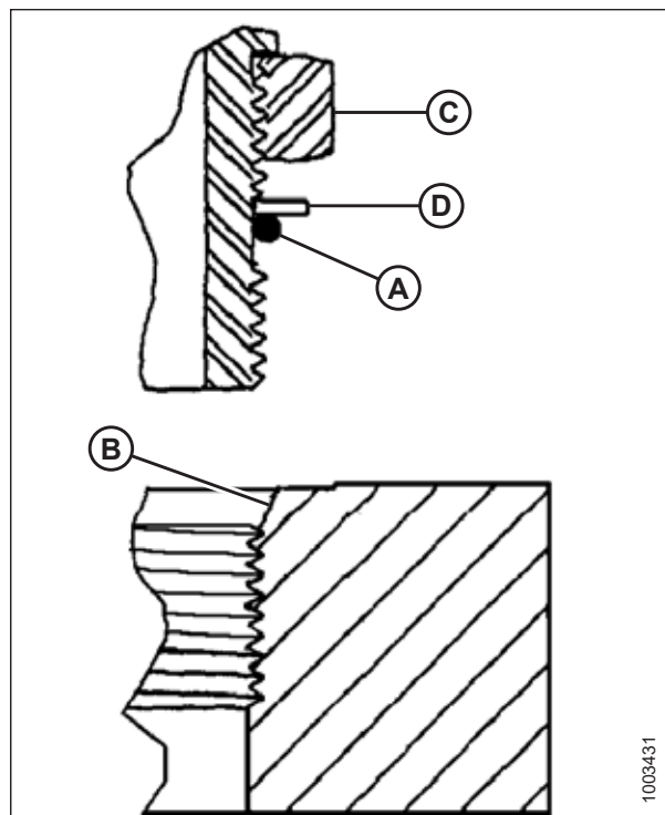
Figura 8.6: Accesorio hidráulico
