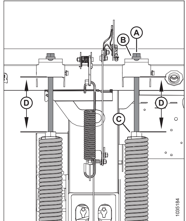
Figura 3.71: Resortes de flotación izquierdos
