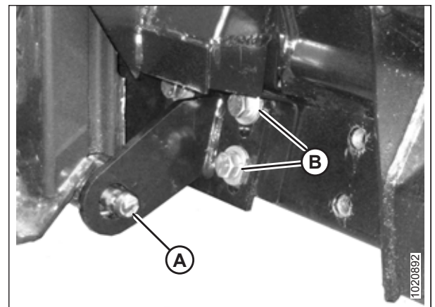
Figura 4.119: Clavija del embocador
