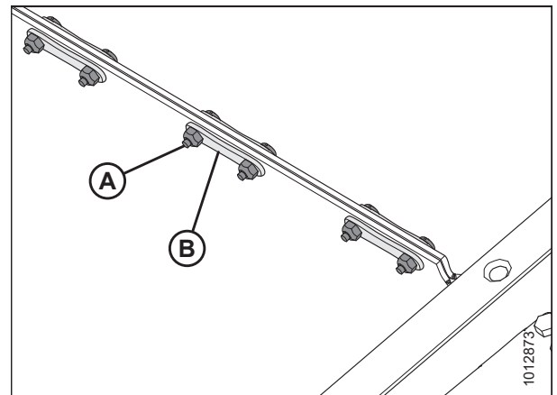
Figura 5.178: Correas del conector de lona
