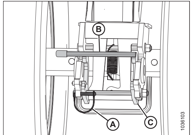
Figura 3.588: Ruedas de transporte izquierdas: pestillo de bloqueo de la rotación desenganchado
