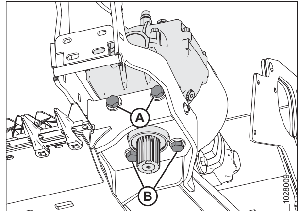
Figura 5.170: Caja de mando de cuchillas: vista desde abajo
