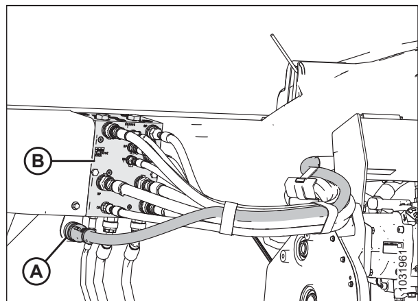
Figura 4.163: Conexiones de la plataforma
