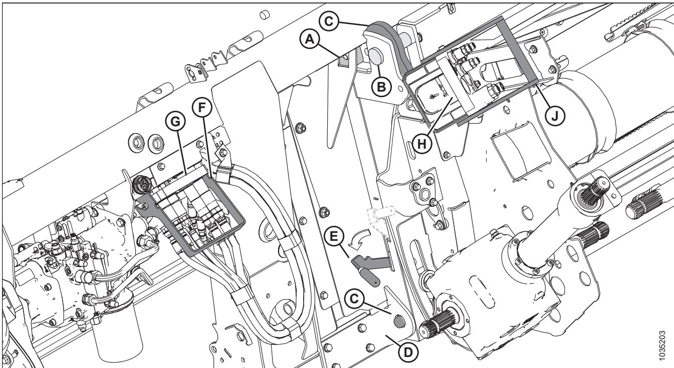
Figura 4.73: Embocador
