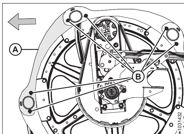
Figura 5.334: Tapas laterales del molinete: sección final interior
