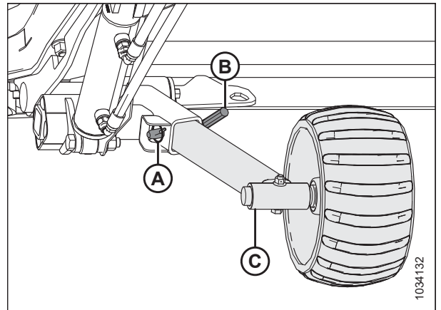
Figura 3.597: Ensamble de la rueda izquierda
