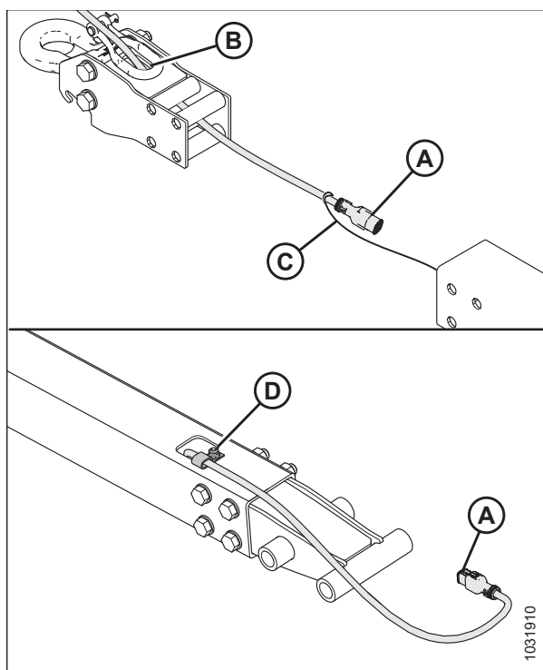
Figura 5.388: Instalación del adaptador de anillo de pivote
