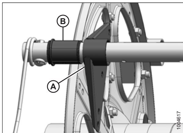
Figura 5.291: Buje
