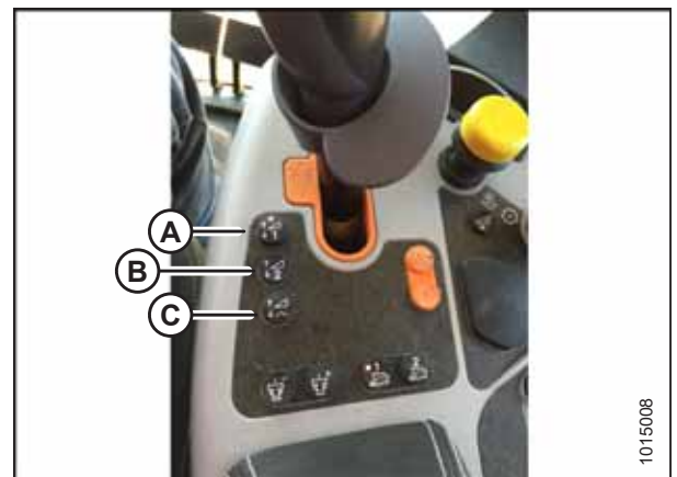
Figura 3.566: Controles de la cosechadora New Holland
