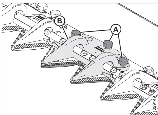
Figura 5.163: Puntón de cuchilla central
