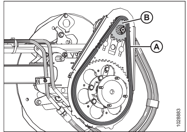
Figura 5.349: Piñón único
