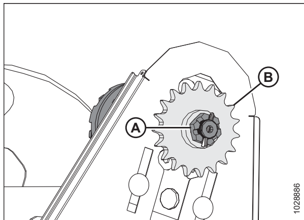
Figura 5.351: Piñón único
