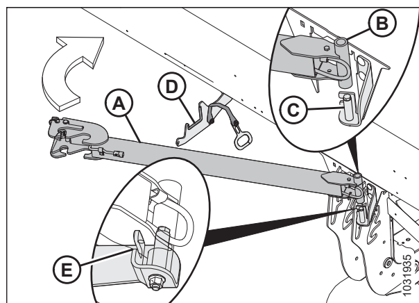
Figura 3.583: Almacenamiento de la extensión de la barra de remolque
