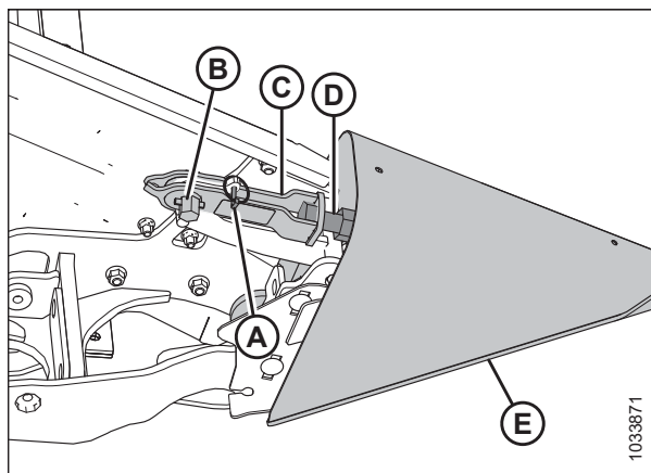
Figura 3.173: Divisor de cosecha con pestillo
