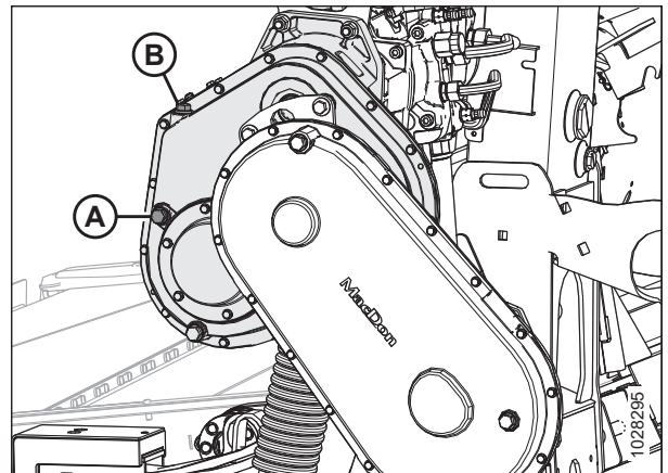
Figura 5.24: Caja de engranajes principal del mando de la plataforma
