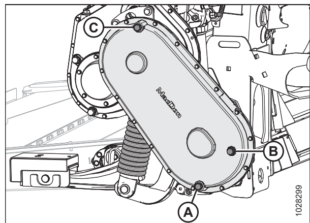
Figura 5.28: Caja de engranajes de completión del mando de la plataforma
