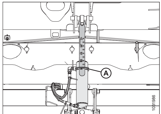
Figura 3.199: Unión central
