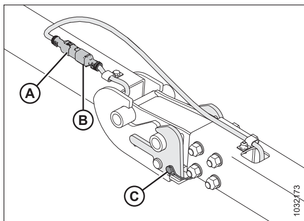
Figura 3.575: Barra de remolque/Arnés de extensión
