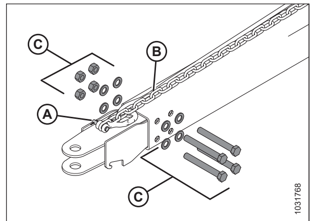
Figura 5.386: Extracción del adaptador de remolque de la horquilla
