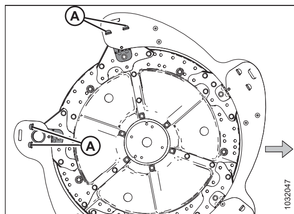
Figura 5.328: Tapa lateral del molinete extraída: extremo de leva interior
