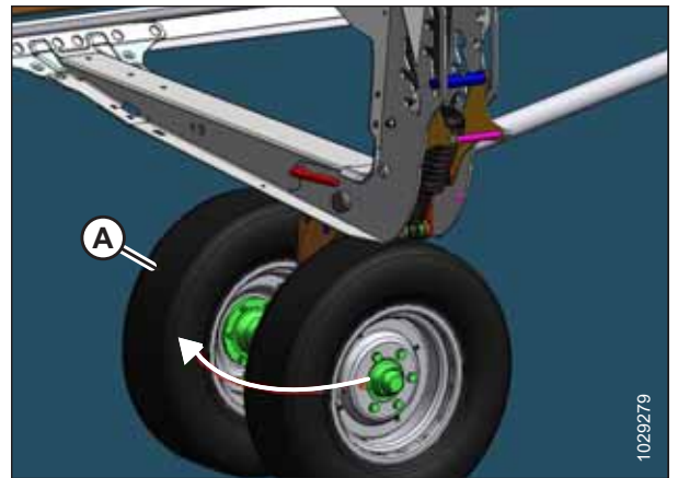
Figura 3.602: Rueda de calibración
