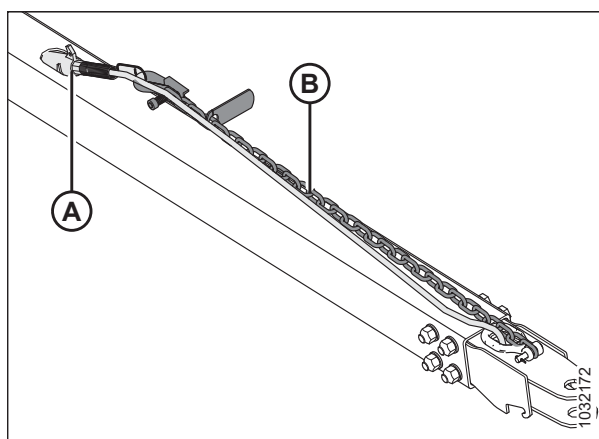
Figura 3.615: Arnés de cableado de la barra de remolque
