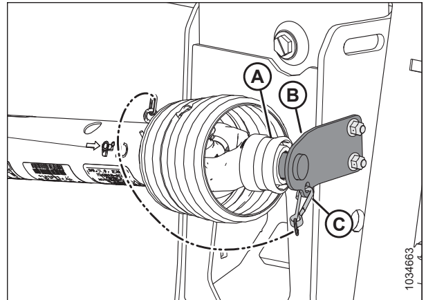
Figura 4.86: Cardán en posición de almacenamiento: Cardán MD n.º B7038 o MD n.º B7039
