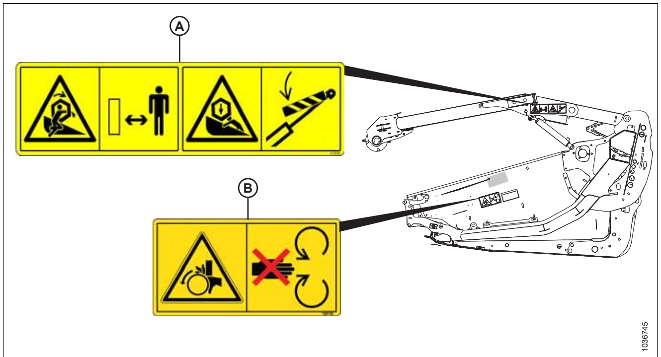
Figura 1.15: Brazos del molinete y chapa posterior
