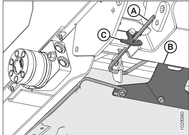
Figura 5.228: Parte inferior de la bandeja de la plataforma de alimentación
