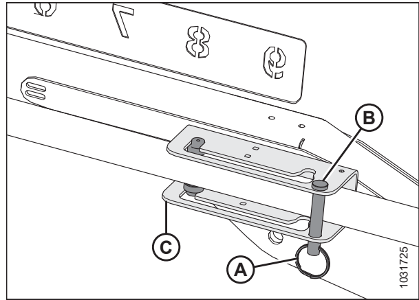
Figura 3.153: Cilindro del brazo izquierdo: Posición de avance
