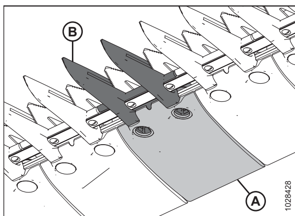
Figura 5.137: Puntón de cuchilla puntiagudo y placa de desgaste
