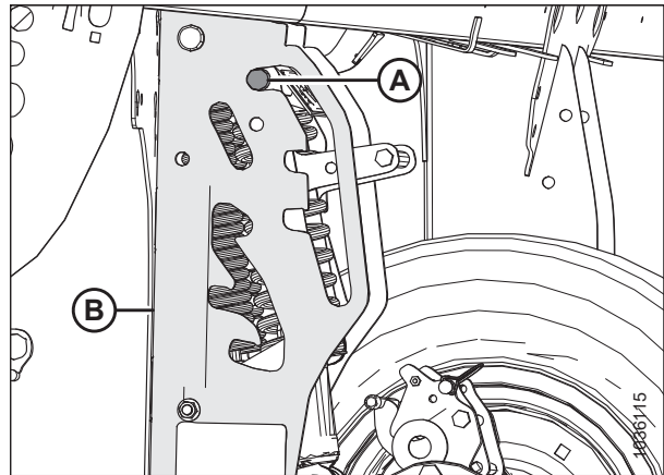
Figura 3.592: Clavija de pivote de las ruedas de transporte izquierdas en la posición de almacenamiento más alta
