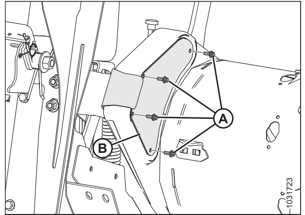
Figura 5.88: Lado izquierdo del mando del sinfín: vista trasera
