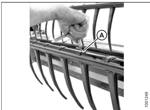
Figura 5.288: Instalación de dientes de plástico
