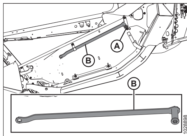
Figura 5.345: Ubicación de almacenamiento de la herramienta múltiple: lado izquierdo
