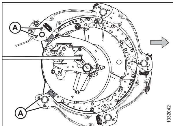
Figura 5.324: Tapas laterales del molinete extraídas: extremo de leva exterior
