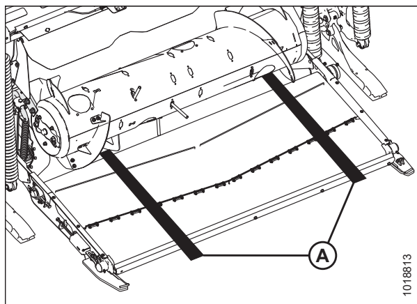
Figura 5.72: Bloques debajo del sinfín
