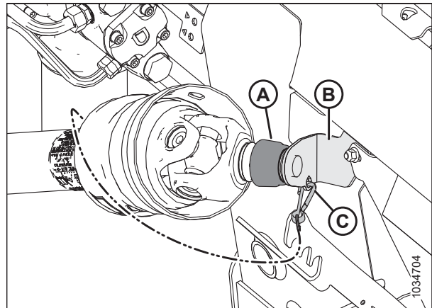
Figura 4.122: Cardán en posición de almacenamiento: cardán Sidehill/Hillside MD n.º B7180, MD n.º B7181, o MD n.º B7182
