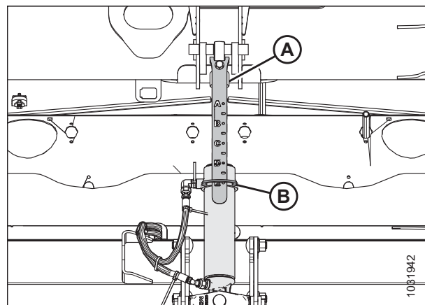
Figura 4.153: Unión central
