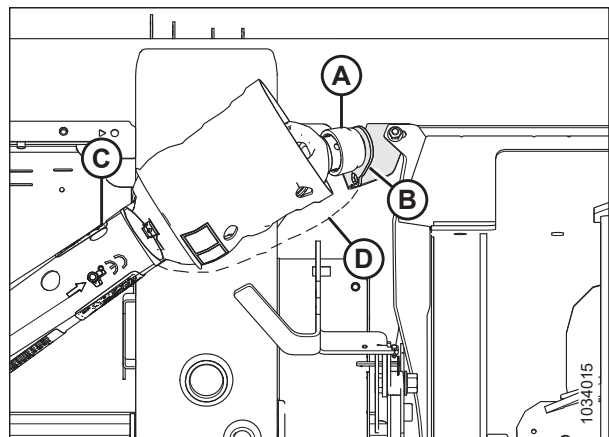
Figura 5.39: Protector del cardán de inclinación lateral opcional
