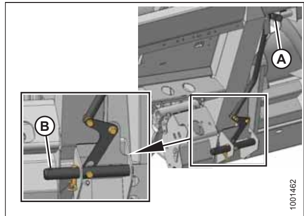
Figura 4.97: Clavijas replegadas
