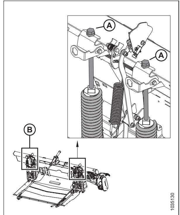
Figura 3.67: Ajuste de flotación: izquierdo
