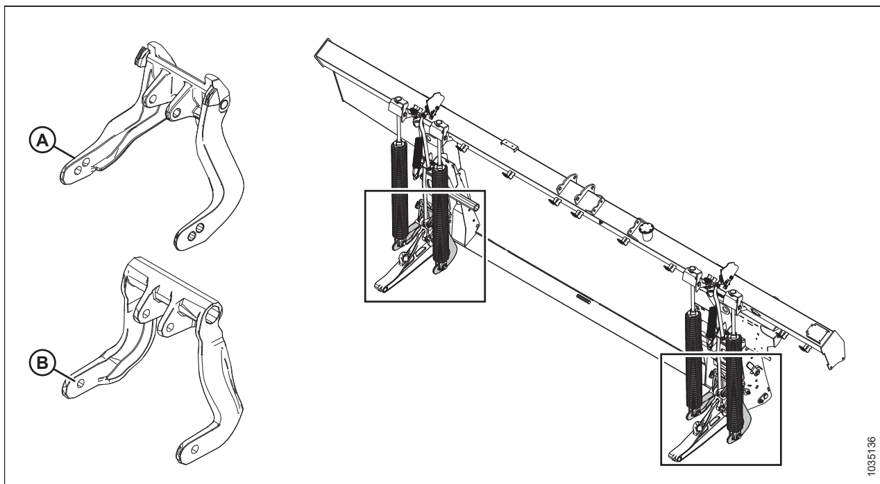
Figura 3.60: Palanca de flotación con un agujero frente a palanca de flotación con dos agujeros
