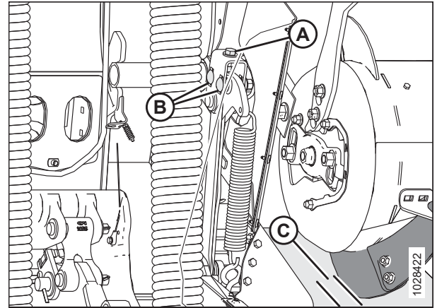
Figura 5.66: Separación del sinfín
