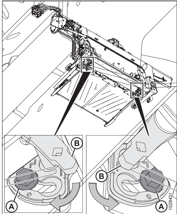
Figura 3.189: Ajuste de flotación del sinfín de alimentación
