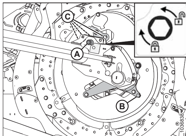
Figura 3.166: Posiciones del disco de leva
