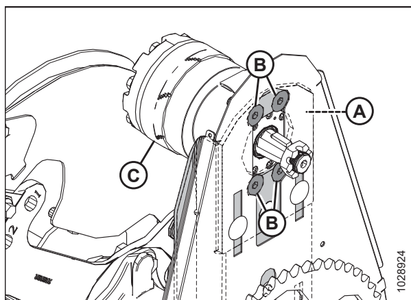
Figura 5.361: Tornillos de montaje del motor del mando del molinete
