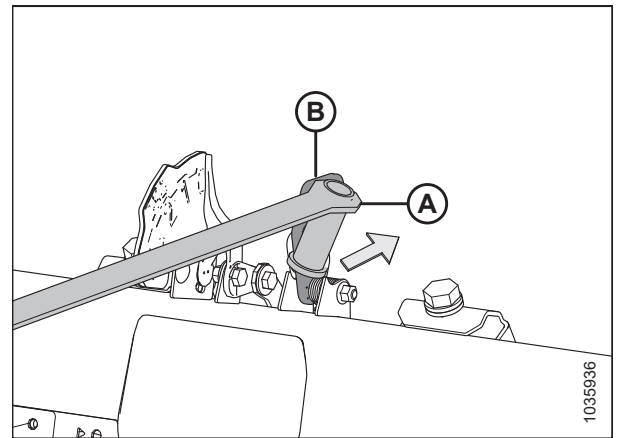
Figura 3.59: Ajuste de flotación: izquierdo
