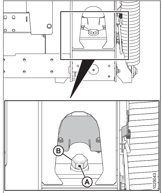
Figura 3.568: Bloqueo de flotación: lado derecho
