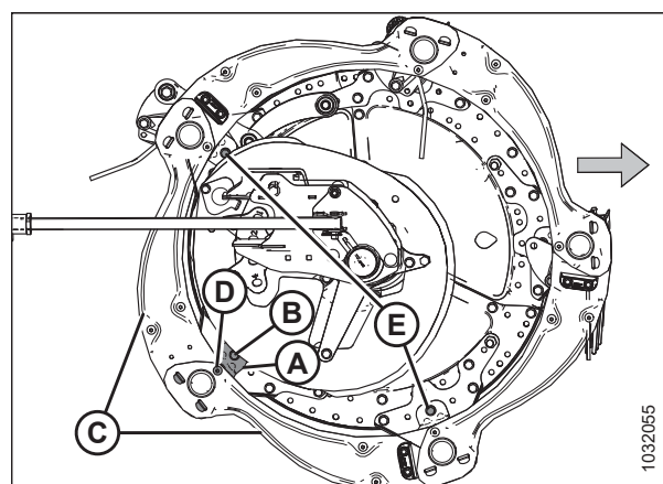
Figura 5.342: Soportes de la tapa lateral del molinete
