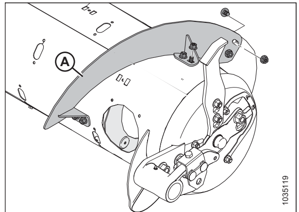
Figura 4.38: Ala larga: lado derecho
