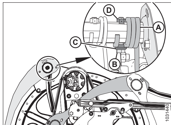
Figura 5.338: Tapas laterales del molinete: sección final interior
