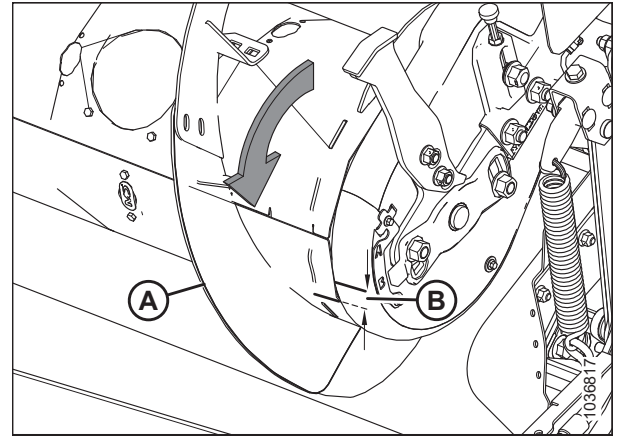
Figura 5.68: Mando del sinfín de alimentación
