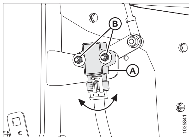
Figura 3.133: Sensor de altura del molinete: brazo derecho del molinete con molinete hacia arriba
