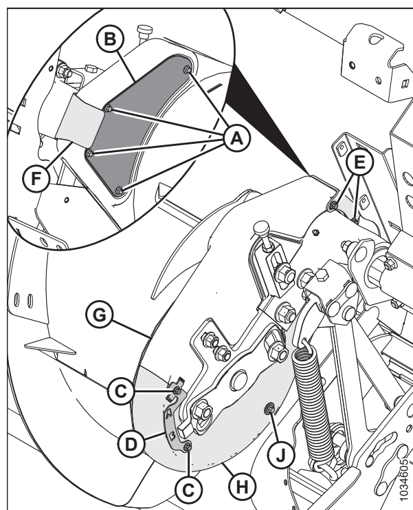
Figura 5.86: Sinfín
