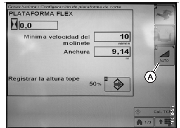
Figura 3.453: Pantalla de la cosechadora
