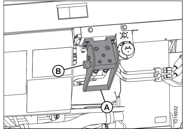
Figura 4.95: Receptáculo del módulo de flotación
