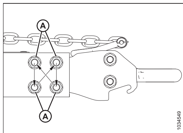
Figura 5.390: Secuencia de par de torsión
