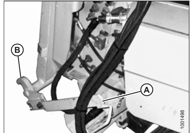
Figura 4.82: Trabas del embocador
