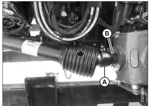
Figura 4.78: Desacoplamiento del cardán para cosechadora
