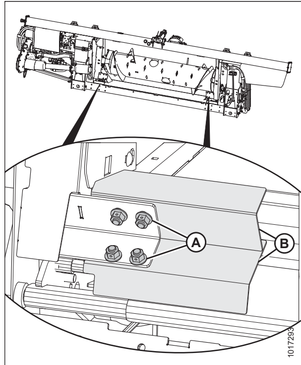
Figura 5.233: Esquinero de alimentación
