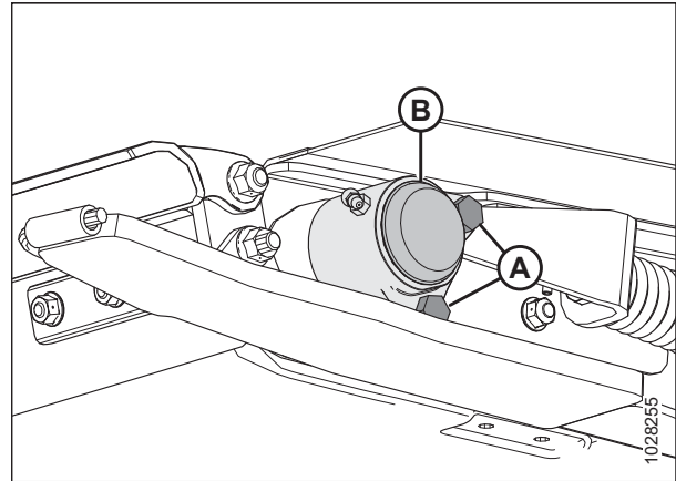
Figura 5.216: Rodamiento de rodillo tensor: lado izquierdo
