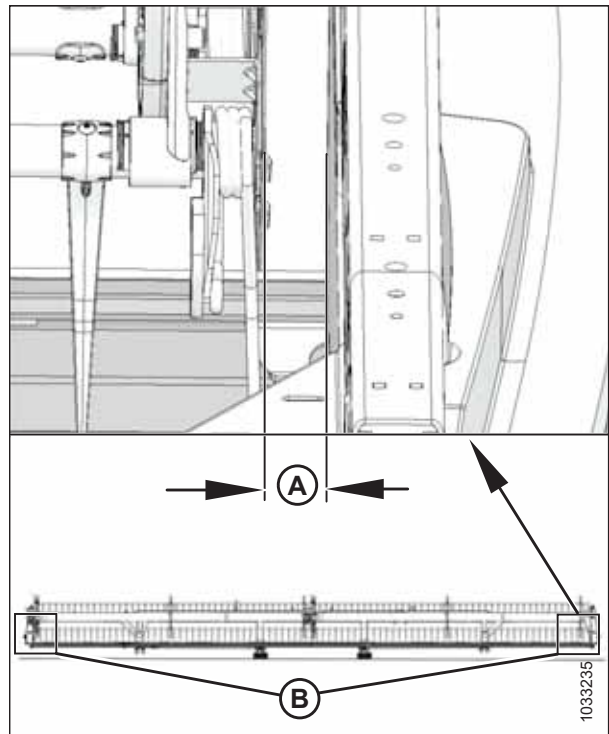
Figura 5.281: Centrar el molinete
