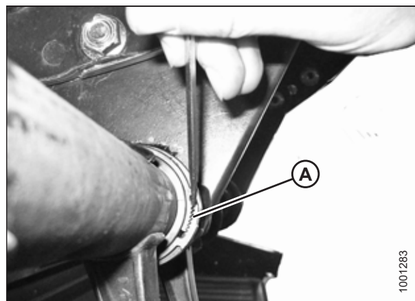
Figura 5.290: Abrazadera del buje
