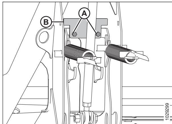
Figura 3.90: Placa limitadora de "cara triste" de flexión
