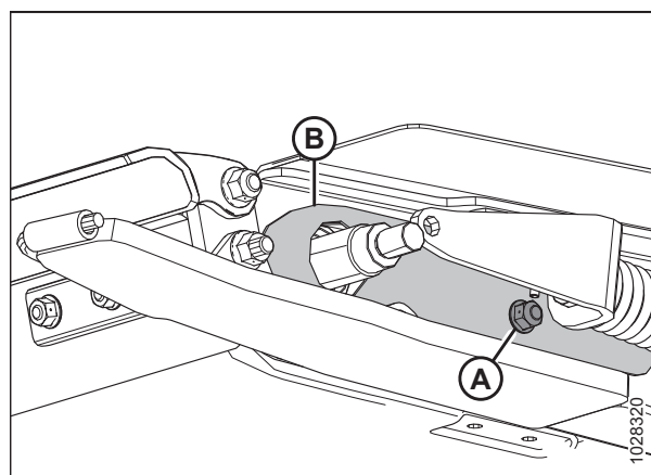
Figura 5.203: Cubierta del rodillo tensor
