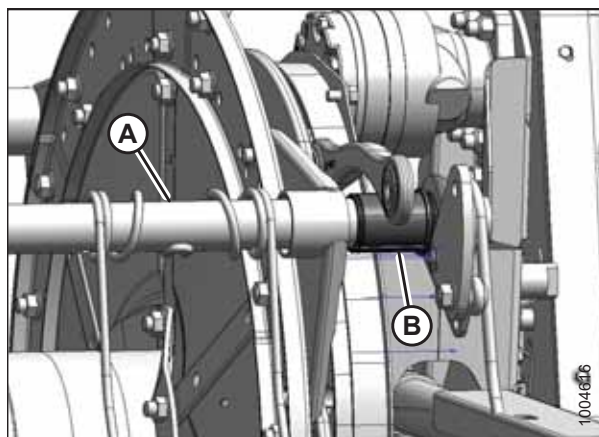
Figura 5.310: Extremo de leva
