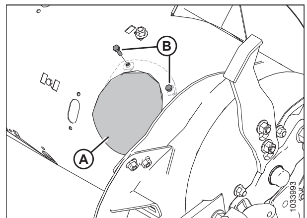
Figura 4.33: Cubierta de acceso: lado derecho
