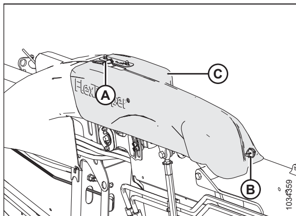
Figura 3.30: Cubierta de conexión de flexión interna: lado izquierdo
