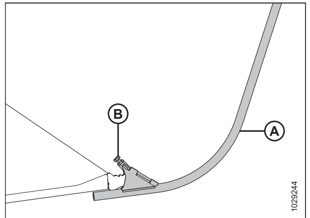
Figura 3.183: Varilla divisora en el divisor de cosecha
