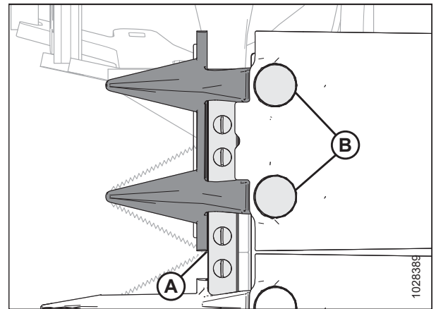
Figura 5.121: Primer puntón de cuchillas: vista desde la cuchilla inferior
