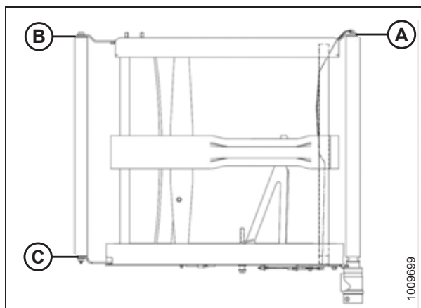
Figura 5.243: Brazos del rodillo
