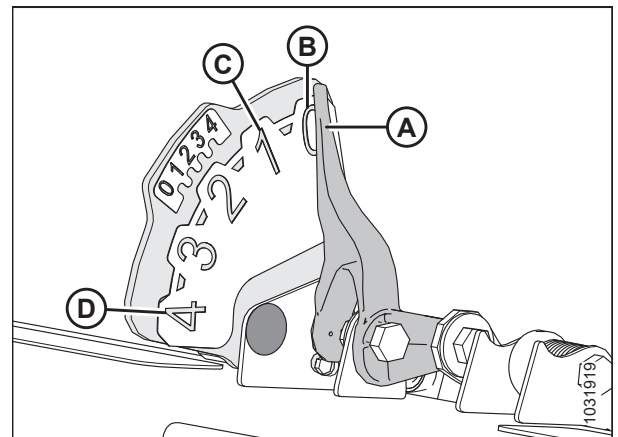
Figura 3.283: Indicador de flotación
