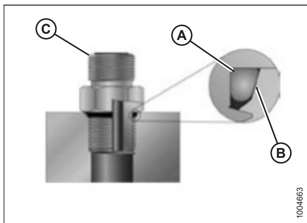
Figura 8.8: Accesorio hidráulico
