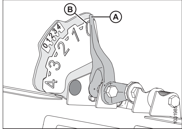
Figura 3.196: Indicador de flotación izquierdo: vista desde atrás
