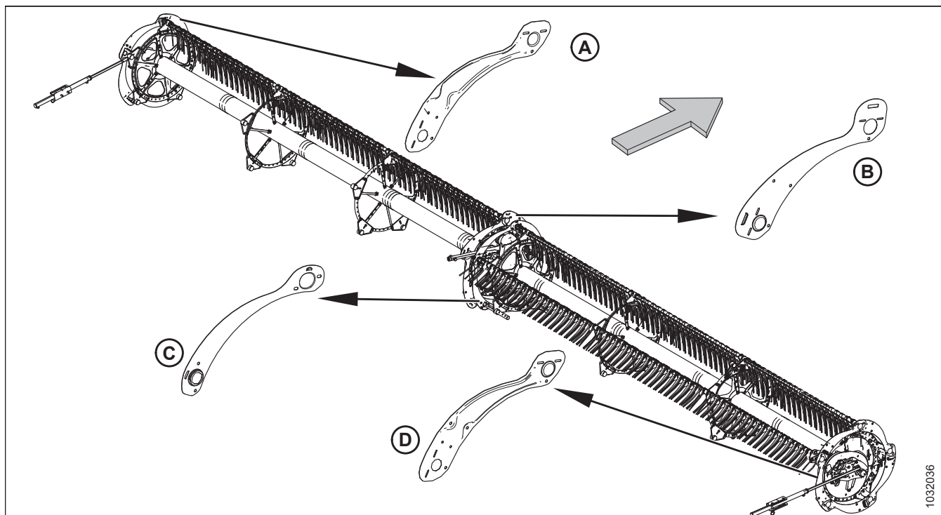
Figura 5.321: Tapas laterales del molinete
