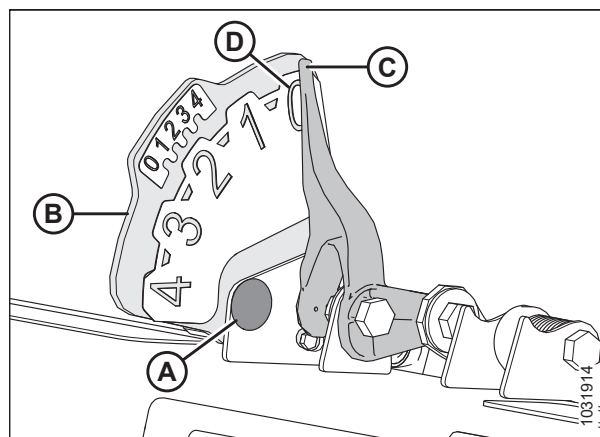
Figura 3.370: Indicador de flotación
