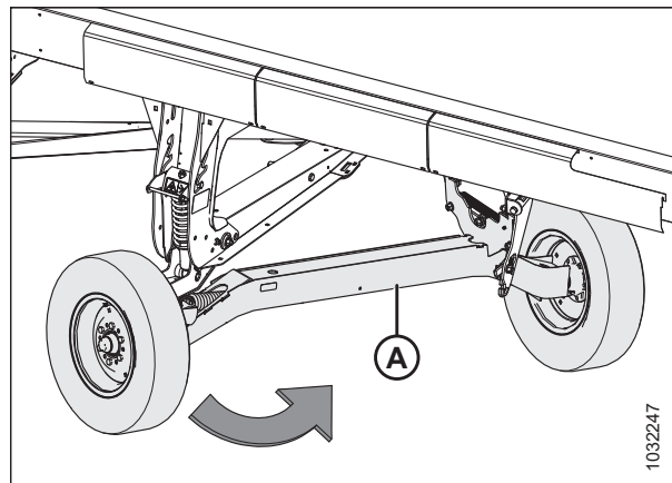
Figura 3.606: Eje de transporte derecho
