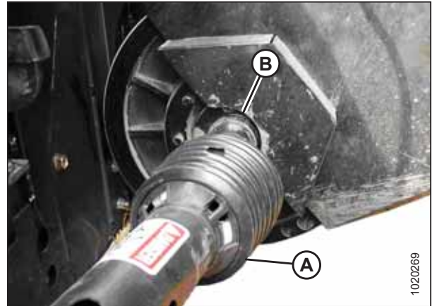
Figura 4.66: Mando
