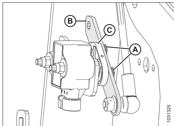
Figura 3.136: Sensor de altura del molinete-Brazo del molinete derecho
