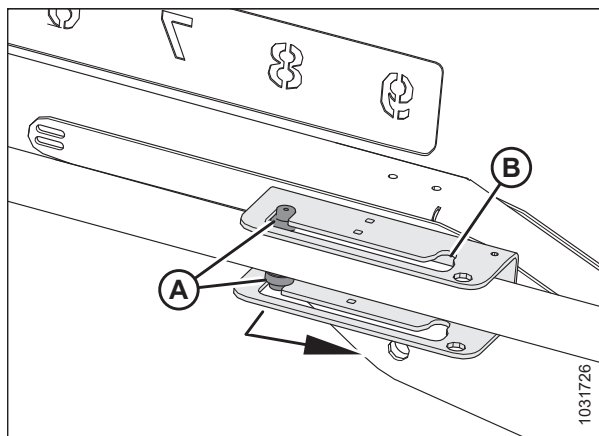
Figura 3.147: Cilindro del brazo izquierdo: Posición de avance
