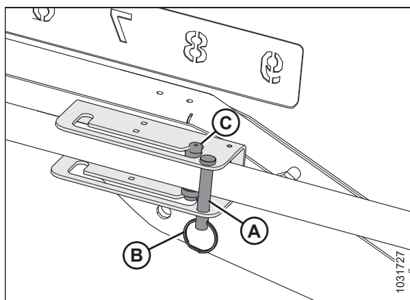
Figura 3.148: Cilindro del brazo izquierdo: Posición de retroceso
