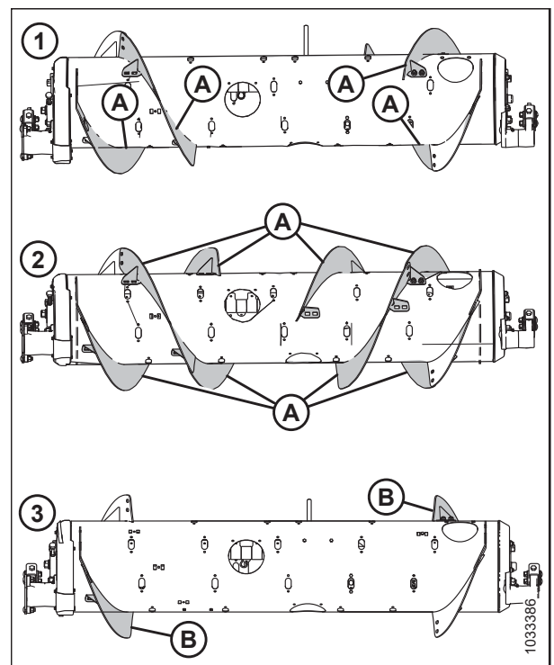
Figura 4.19: Configuraciones de sinfín: vista posterior
