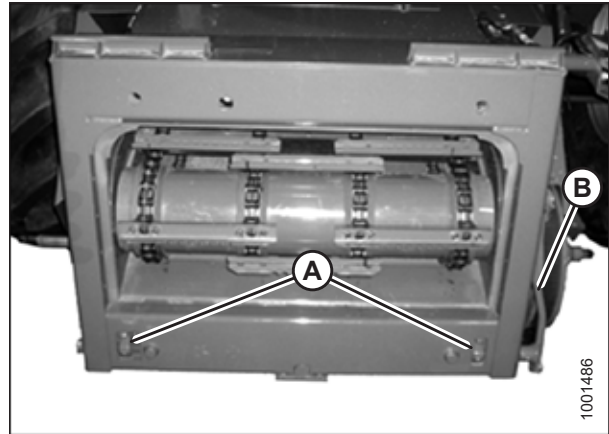
Figura 4.56: Embocador del grupo AGCO
