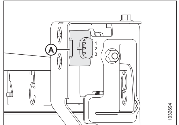
Figura 3.158: Sensor de avance y retroceso
