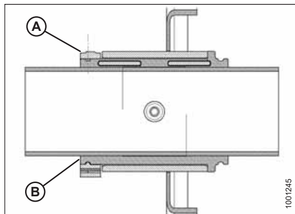
Figura 5.317: Buje
