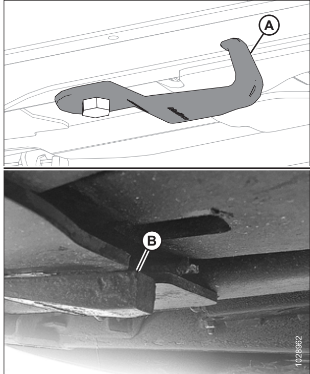
Figura 5.230: Ganchos del soporte de unión
