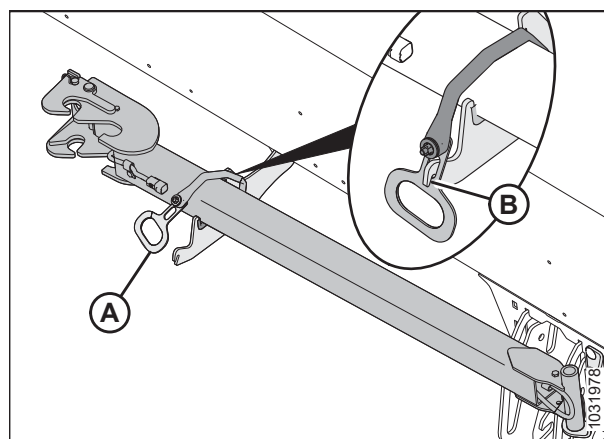
Figura 3.584: Almacenamiento de la extensión de la barra de remolque
