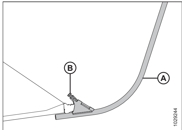
Figura 3.180: Barra abresurcos para cosecha
