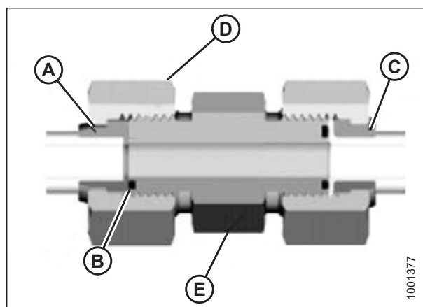
Figura 8.10: Accesorio hidráulico
