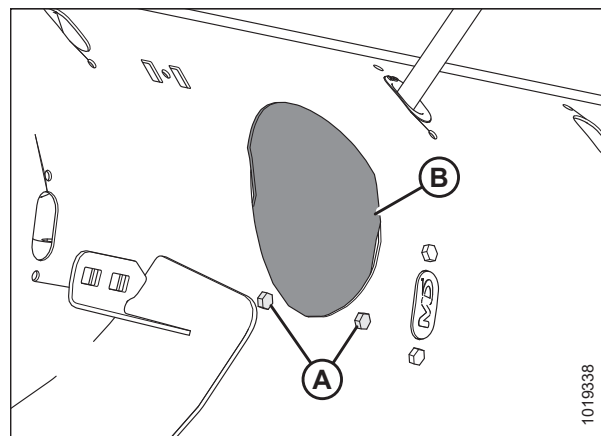
Figura 5.97: Cubierta hueca de acceso del sinfín
