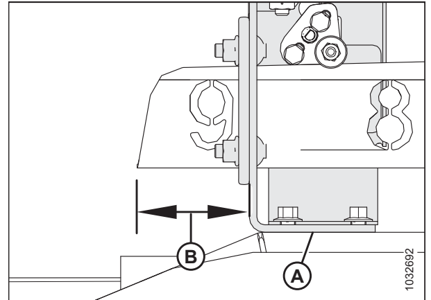
Figura 3.157: Soporte de avance y retroceso
