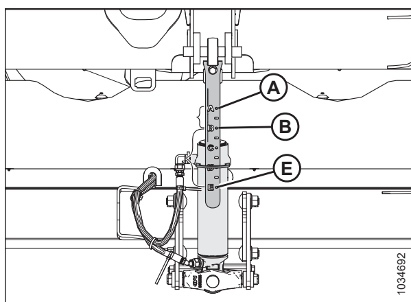
Figura 3.37: Indicador del ángulo de la plataforma
