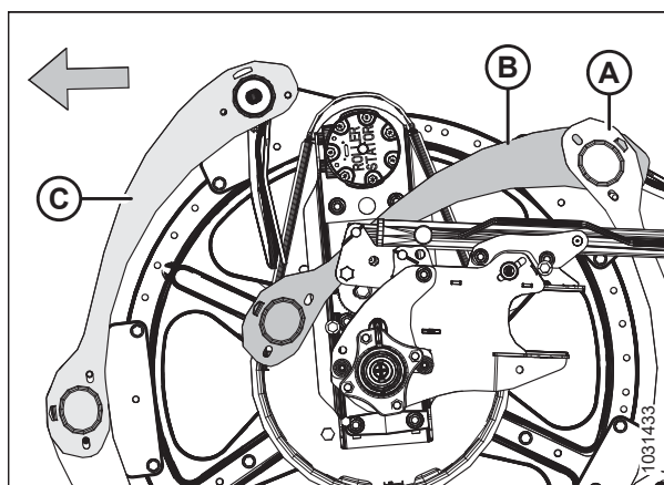
Figura 5.335: Tapas laterales del molinete: sección final interior
