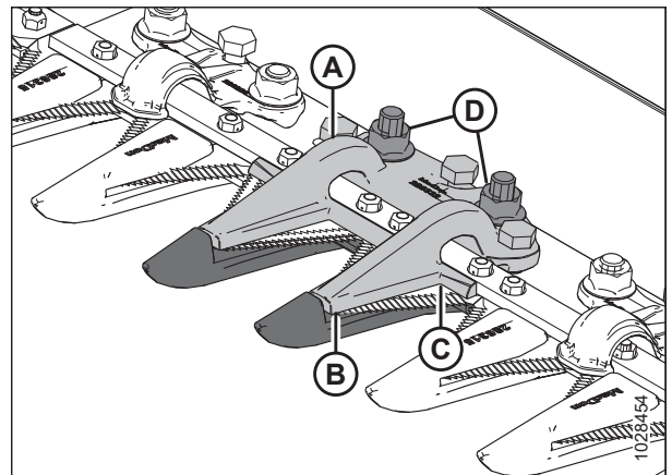
Figura 5.147: Sujetador central puntiagudo
