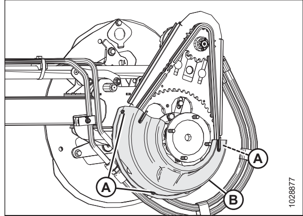
Figura 3.24: Cubierta del mando inferior
