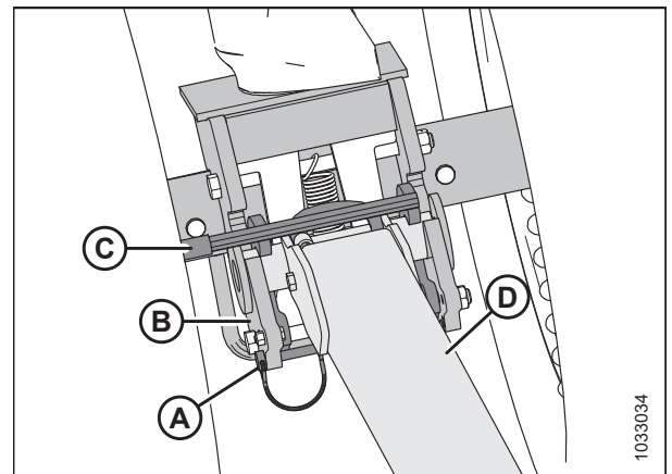
Figura 3.578: Extensión de la barra de remolque y pivote de transporte
