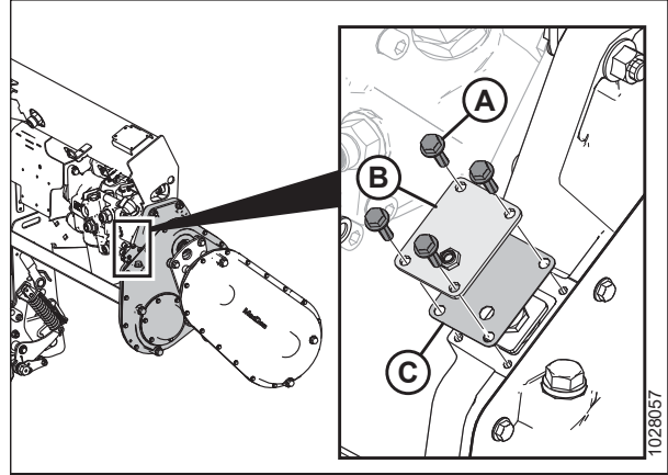
Figura 5.56: Cubierta del tensor de la cadena de la caja de engranajes principal
