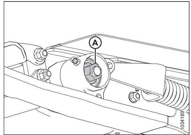
Figura 5.220: Rodamiento de rodillo tensor: lado izquierdo
