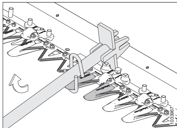
Figura 5.130: Ajuste hacia arriba: puntón puntiagudo
