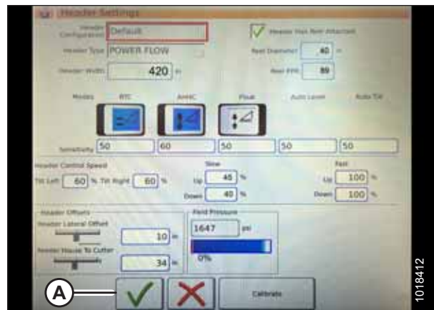
Figura 3.391: Página de configuraciones de la plataforma
