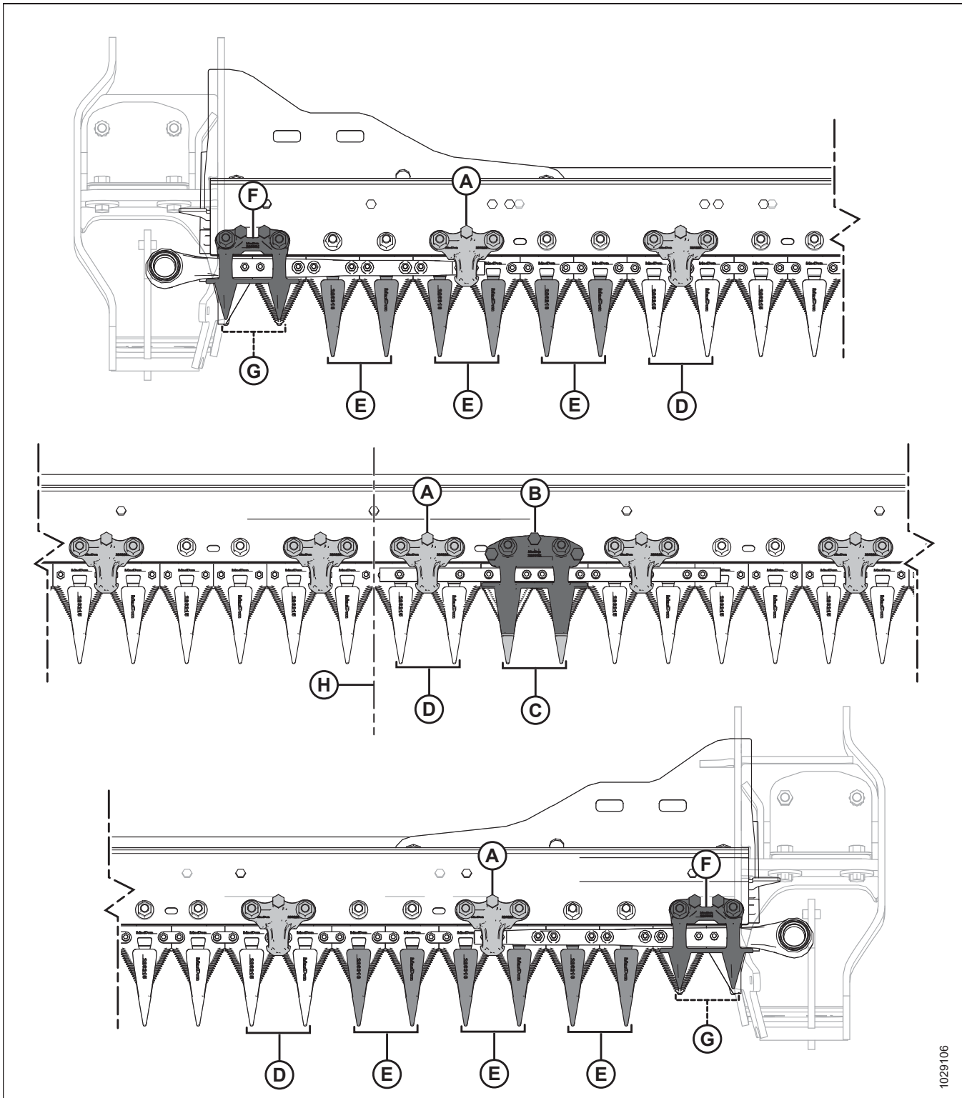
Figura 5.125: Puntón de cuchilla y ubicaciones del sujetador: plataforma de doble cuchilla FD235
