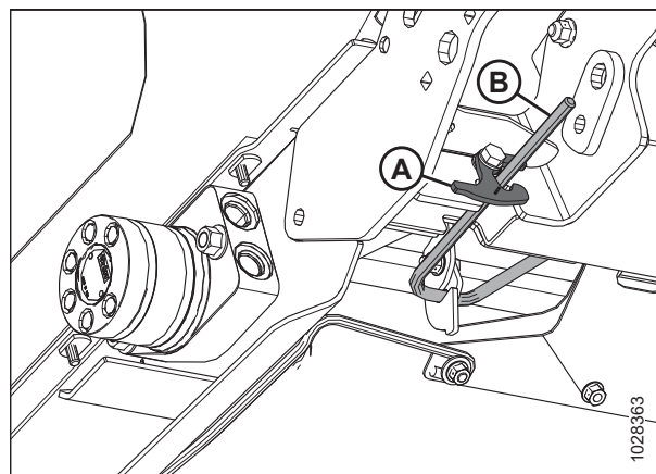
Figura 5.223: Parte inferior de la plataforma de alimentación
