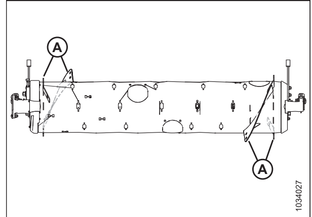
Figura 4.9: Configuración ultraancho
