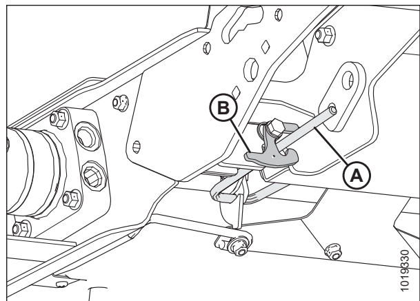
Figura 5.175: Manija de la bandeja de la plataforma de alimentación y pestillo de la manija de la bandeja lateral izquierda
