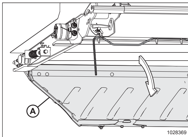
Figura 5.225: Batea de la plataforma de alimentación
