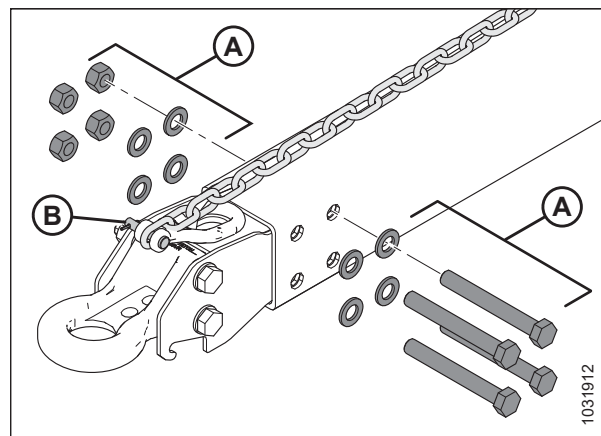
Figura 5.389: Instalación del adaptador de anillo de pivote
