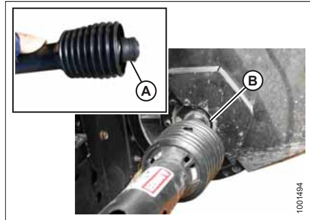
Figura 4.64: Mando
