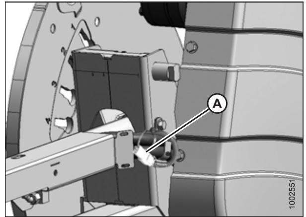
Figura 5.373: Conjunto del mando del molinete: arnés eléctrico
