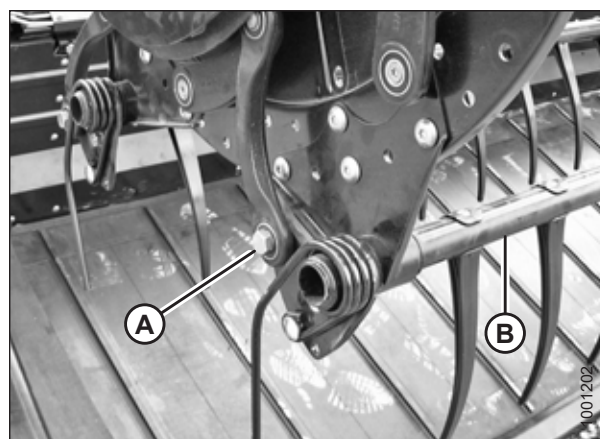
Figura 5.307: Extremo de leva
