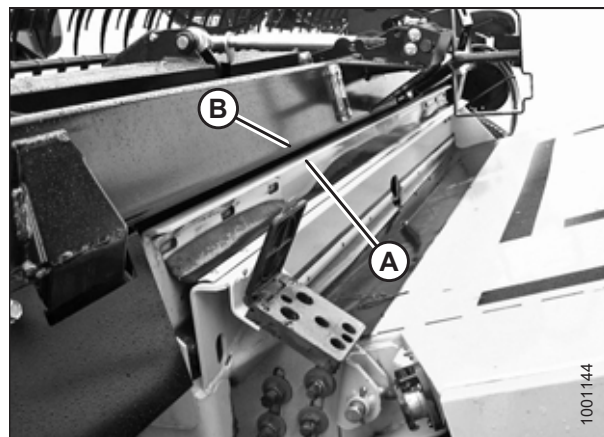
Figura 4.134: Plataforma en la cosechadora
