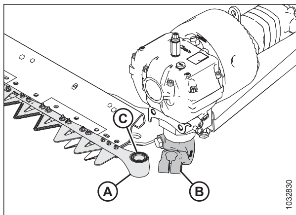
Figura 5.114: Cabeza de la cuchilla izquierda
