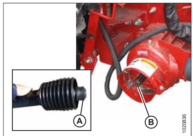
Figura 4.88: Eje de salida de la cosechadora
