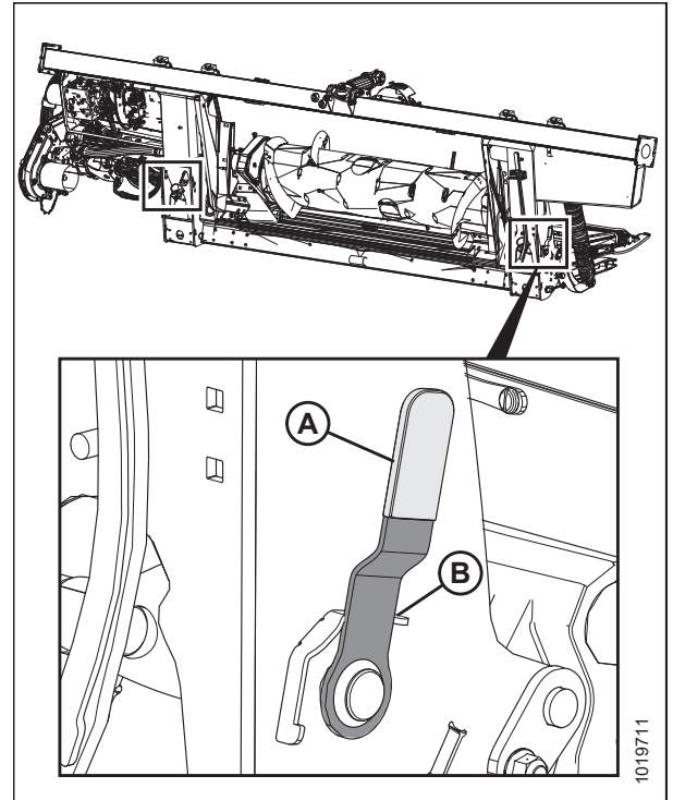
Figura 4.108: Manija de bloqueo de flotación
