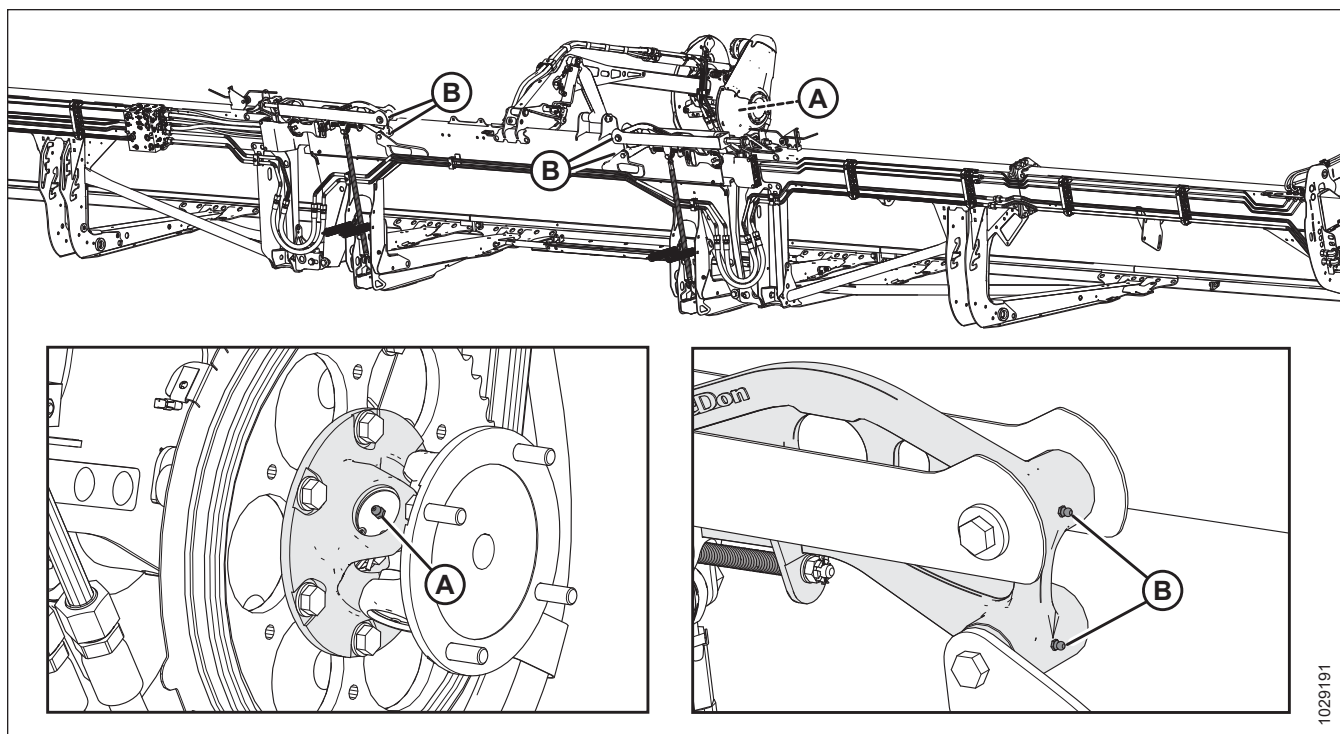
Figura 5.14: Molinete
