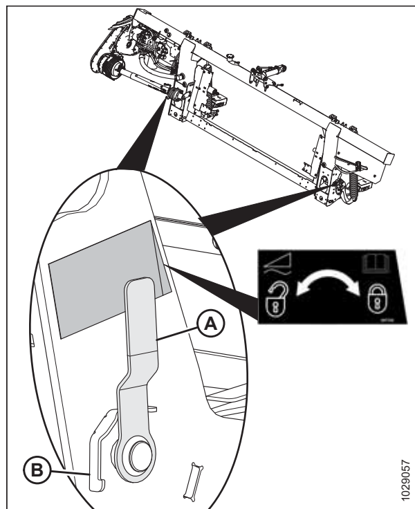
Figura 3.53: Traba de flotación de la plataforma en posición de bloqueo
