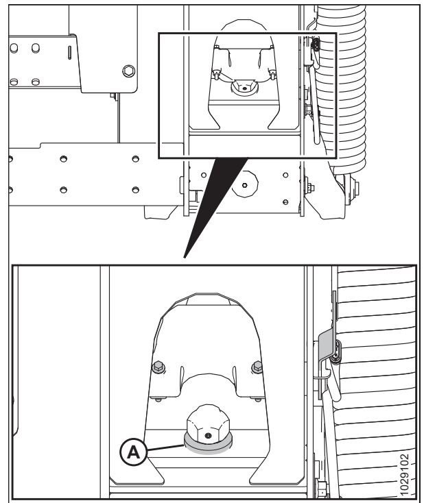
Figura 5.63: Arandela del amortiguador de parada
