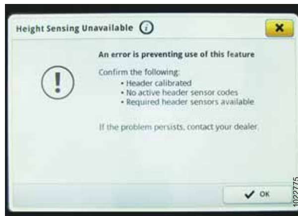
Figura 3.487: Pantalla John Deere S7 - Mensaje de error de detección de altura
