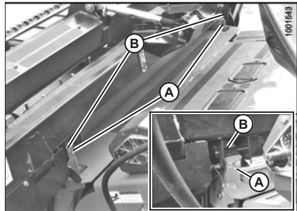
Figura 4.98: Plataforma en la cosechadora
