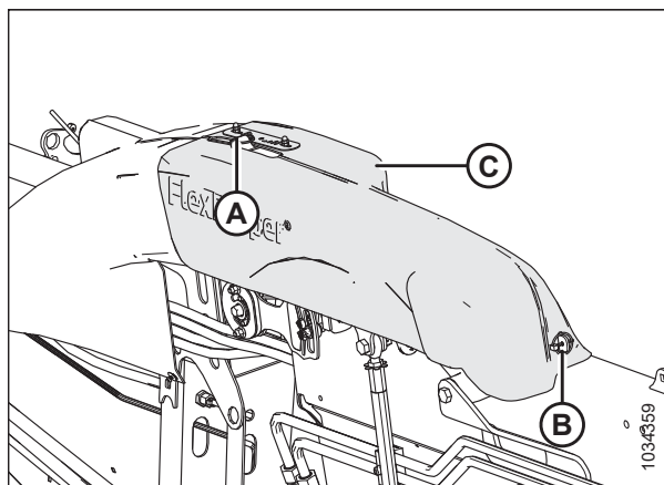
Figura 3.28: Cubierta de conexión de flexión interna: lado izquierdo
