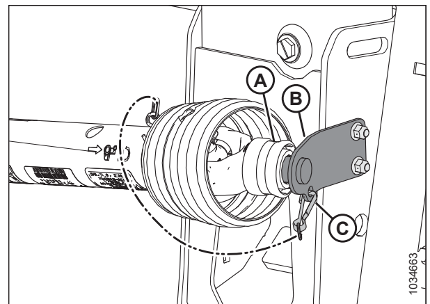
Figura 4.63: Cardán en posición de almacenamiento: Cardán MD n.º B7038 o MD n.º B7039
