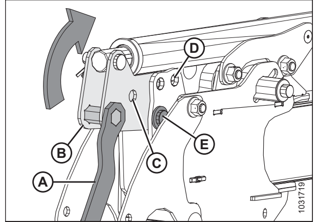
Figura 3.144: Cilindro del brazo derecho – Posición de avance
