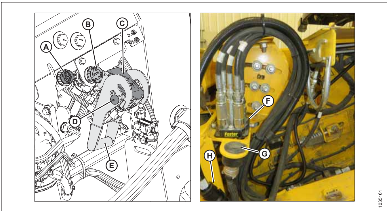
Figura 4.136: Acoplamiento múltiple y conexiones eléctricas
