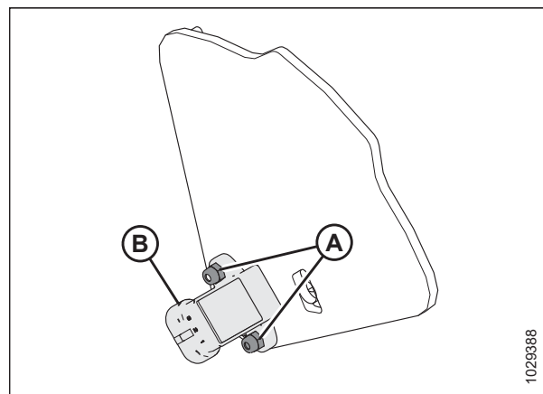
Figura 3.202: Sensor de altura de flotación
