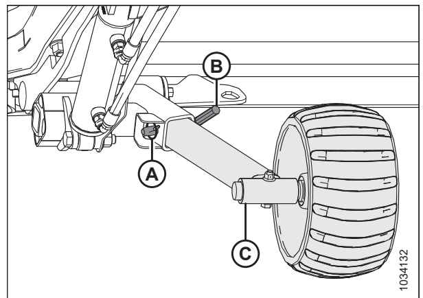
Figura 3.572: Ensamble de la rueda izquierda
