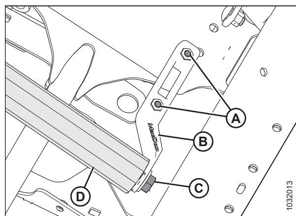
Figura 5.260: Rodillo de mando
