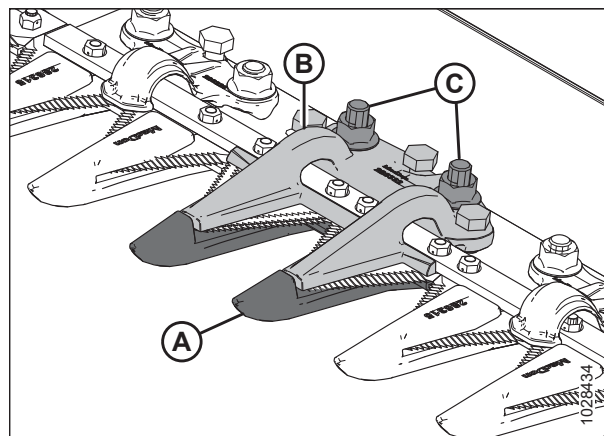
Figura 5.141: Puntón de cuchilla central puntiagudo
