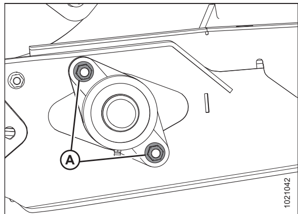
Figura 5.195: Rodamiento del rodillo de mando de la lona de alimentación
