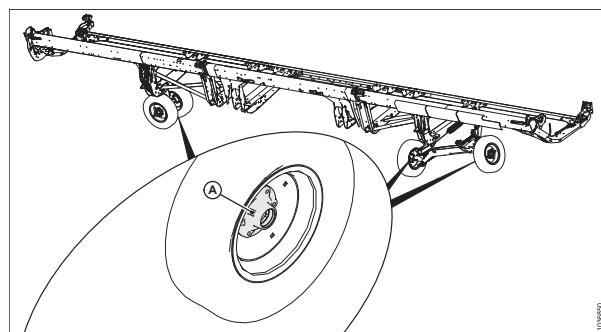
Figura 5.15: Cada 500 horas
