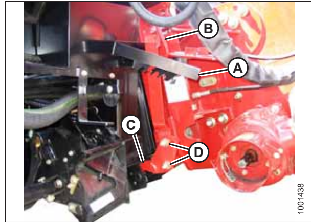
Figura 4.84: Cosechadora y módulo de flotación
