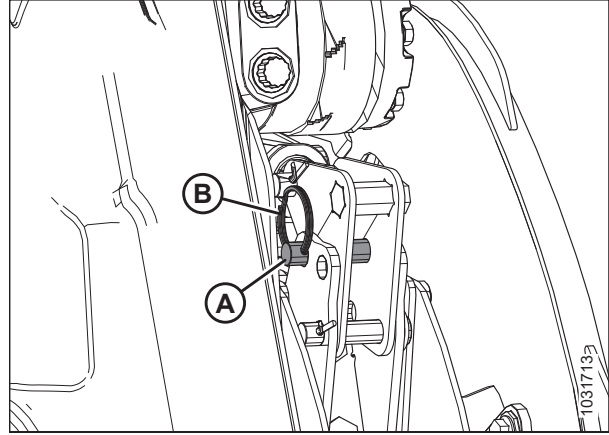
Figura 3.152: Cilindro del brazo central izquierdo: Posición de retroceso
