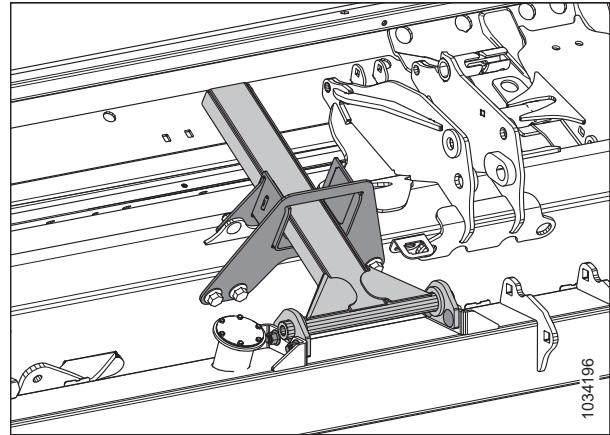
Figura 6.15: Kit estabilizador de montículos
