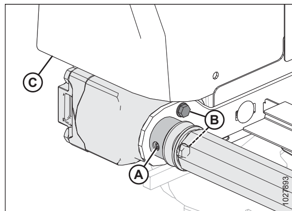
Figura 5.258: Rodillo de mando
