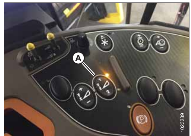
Figura 3.249: Consola de la cosechadora Case
