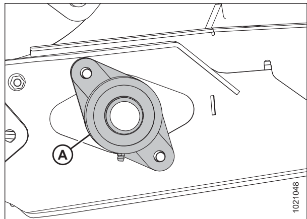
Figura 5.196: Rodamiento del rodillo de mando de la lona de alimentación
