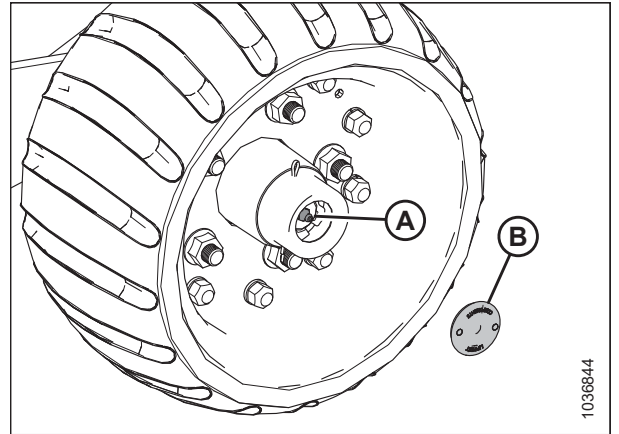
Figura 5.392: Punto de lubricación del eje de la rueda de contorno
