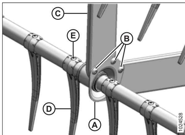
Figura 5.320: Soporte opuesto del kit de refuerzo de la barra de dientes: opcional
