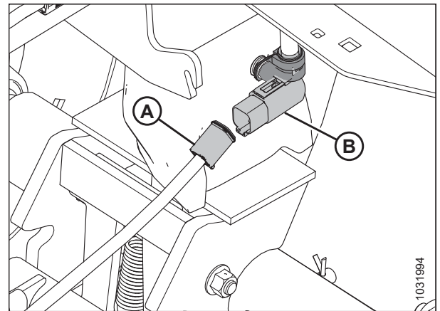
Figura 3.577: Conexión eléctrica de la barra de remolque
