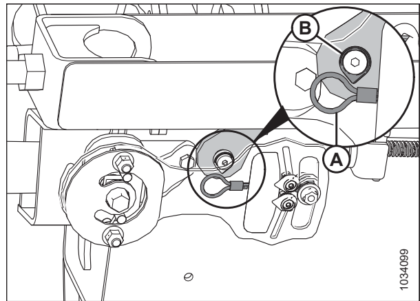
Figura 3.78: Bloqueo de cable verificador de flexión: lado izquierdo
