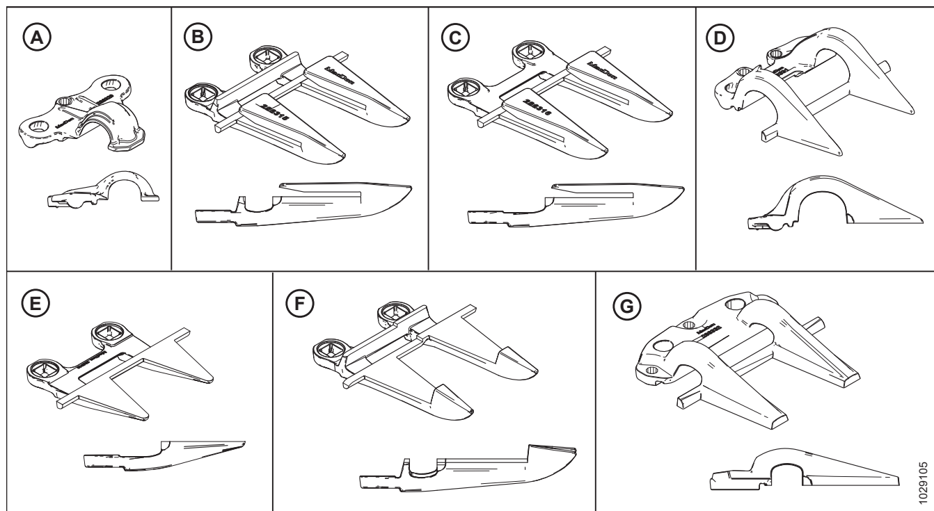
Figura 5.123: Tipos de puntón y sujetador utilizados en las configuraciones de puntón de cuchilla puntiagudo
