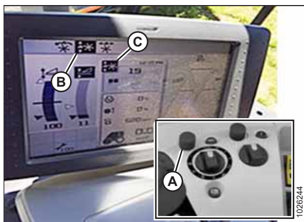
Figura 3.345: Pantalla y consola de la cosechadora CLAAS
