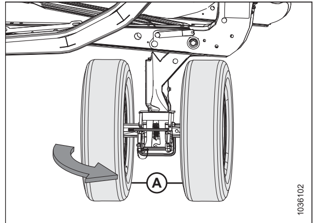
Figura 3.587: Ruedas de transporte izquierdas en modo de transporte
