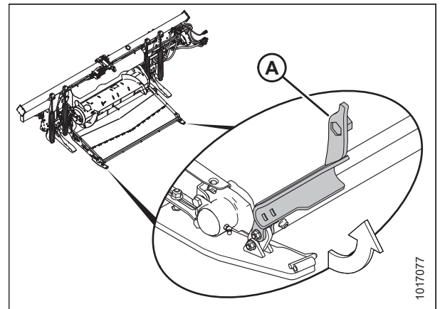
Figura 4.165: Pestillo
