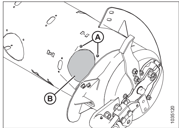
Figura 4.34: Cubierta de acceso del sinfín: lado derecho
