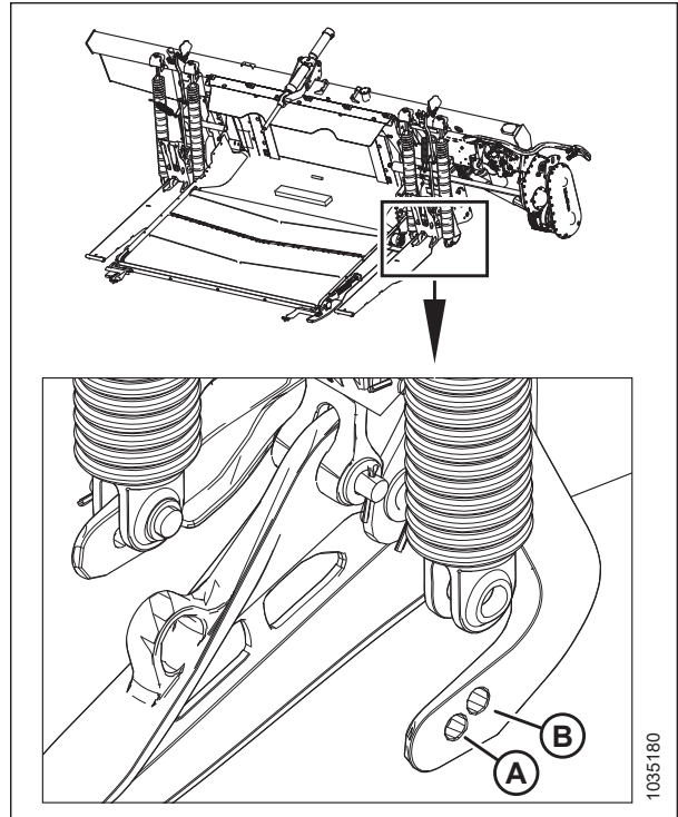
Figura 3.65: Resorte de flotación izquierdo instalado en el agujero de la palanca de flotación trasera
