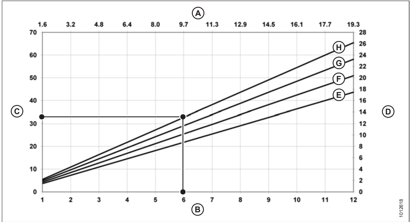
Figura 3.124: Velocidad de avance frente a acres
