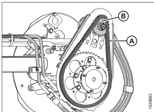
Figura 5.365: Mando del molinete
