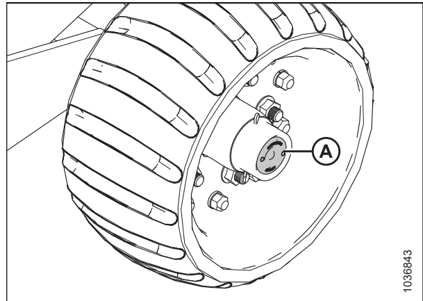
Figura 5.391: Clavija de conexión de goma en el eje de la rueda de contorno
