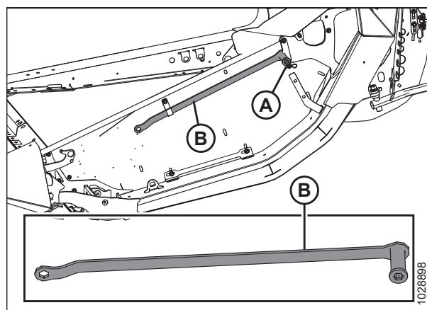
Figura 3.139: Parte final izquierda
