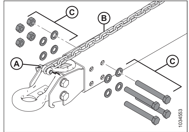
Figura 5.381: Extracción del adaptador de remolque de pivote
