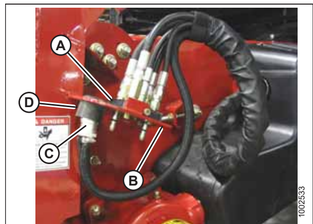
Figura 4.94: Almacenamiento del acoplamiento múltiple
