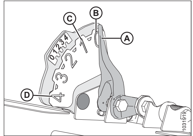
Figura 3.438: Indicador de flotación
