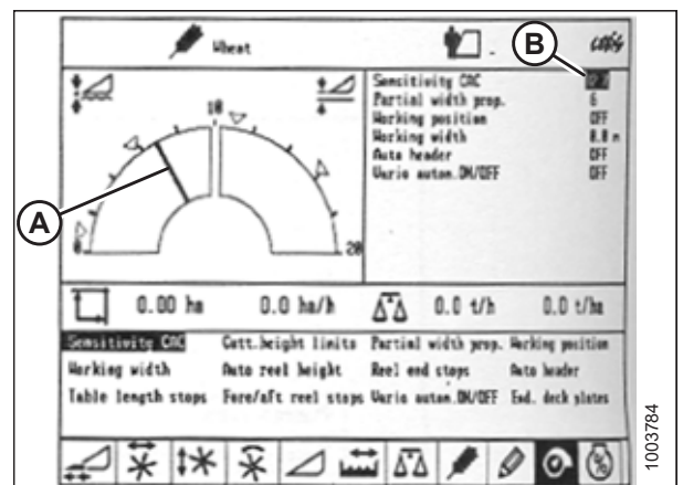
Figura 3.313: Pantalla de la cosechadora CLAAS
