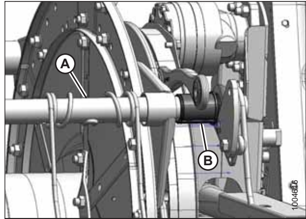
Figura 5.297: Extremo de leva
