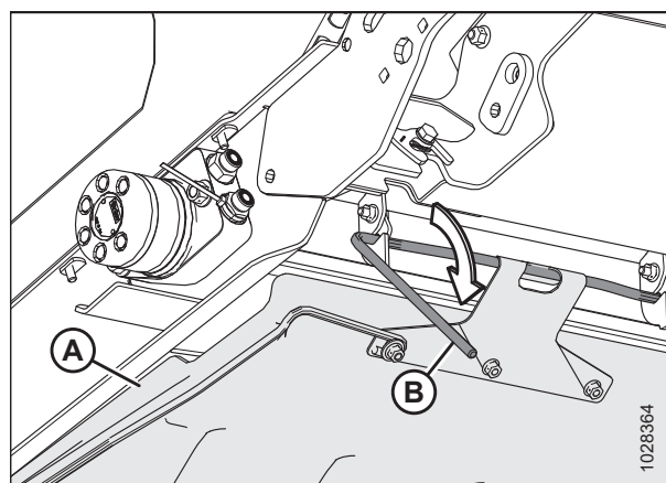
Figura 5.224: Parte inferior de la plataforma de alimentación
