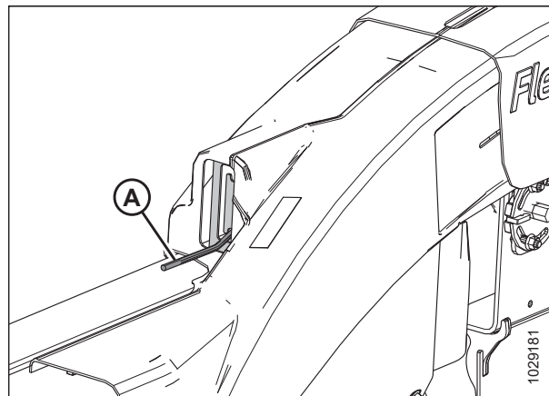
Figura 5.271: Bloqueo de ala en posición de desbloqueo
