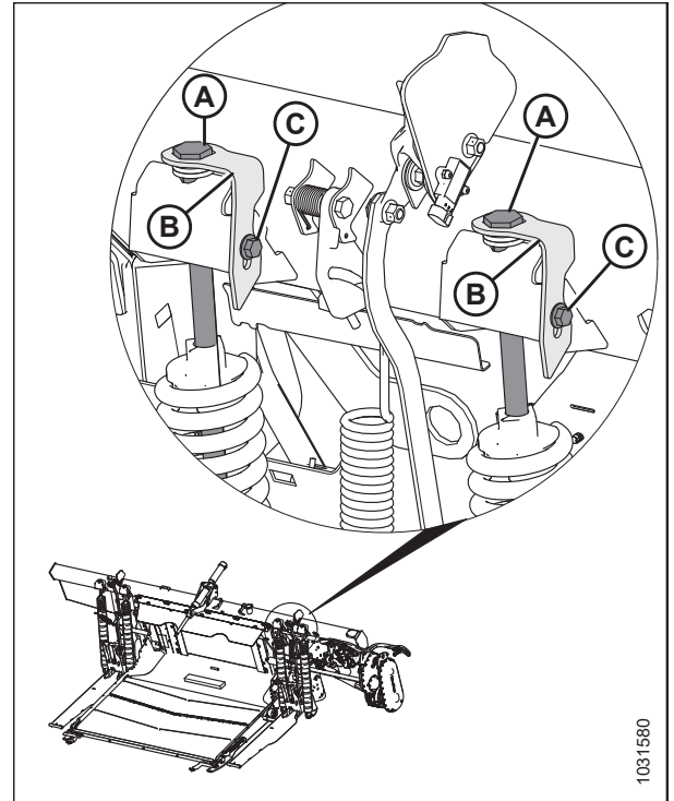
Figura 3.63: Ajuste de flotación: izquierdo
