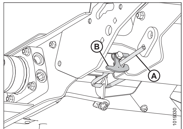
Figura 5.215: Manija de la batea de la plataforma de alimentación y pestillo de la manija de la batea lateral izquierda
