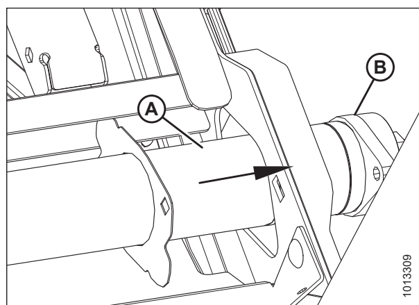
Figura 5.188: Rodillo de mando
