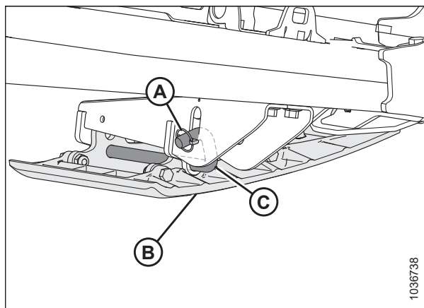
Figura 3.47: Patín externo
