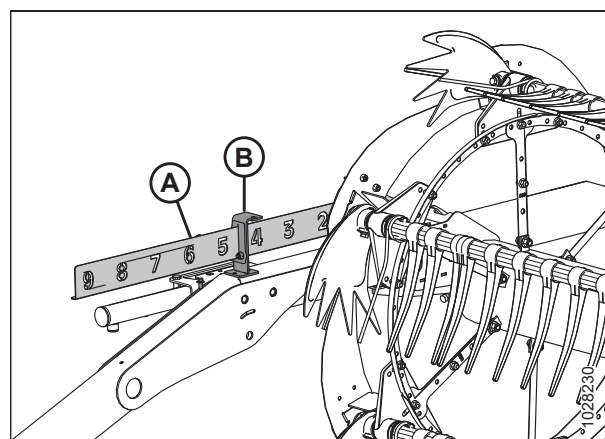
Figura 5.279: Indicador de posición de avance-retroceso
