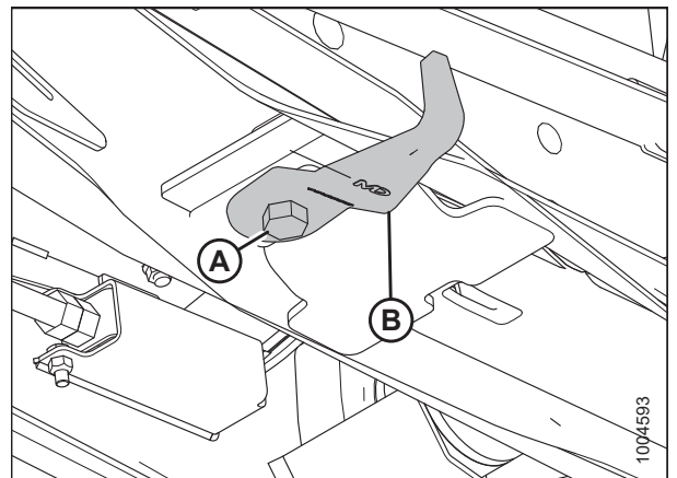
Figura 4.160: Parte inferior del módulo de flotación
