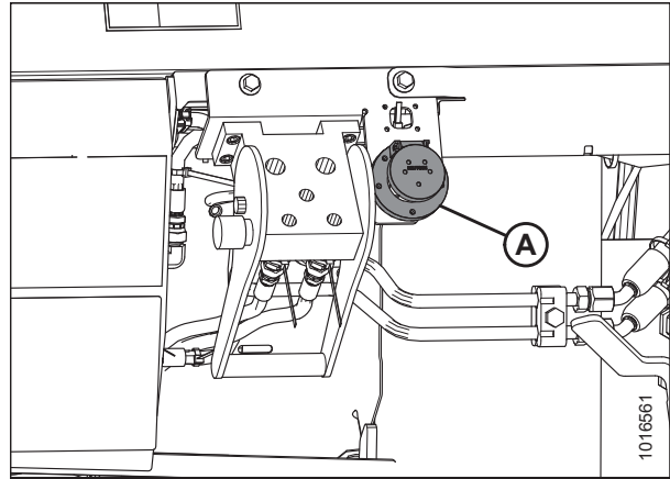
Figura 4.149: Receptáculos del módulo de flotación
