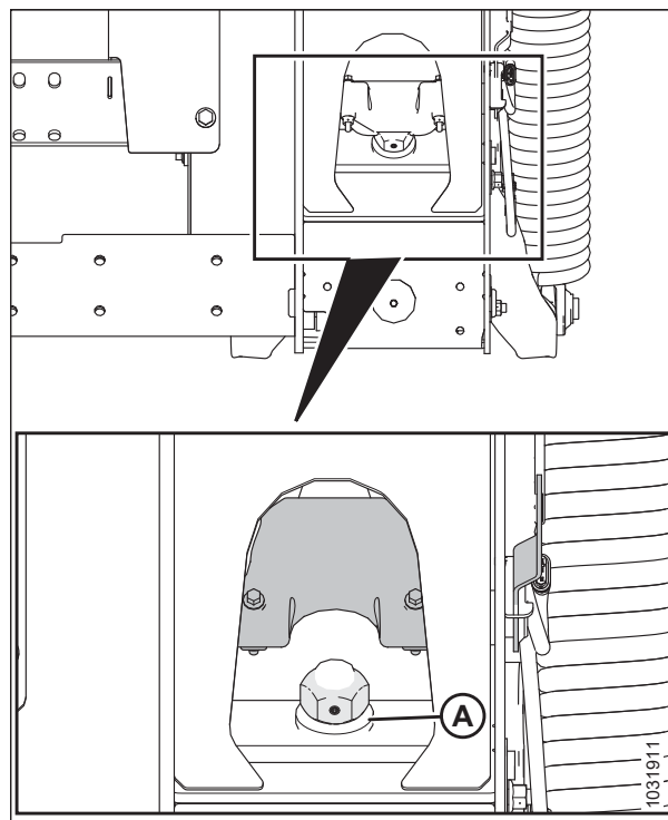
Figura 3.369: Traba de flotación
