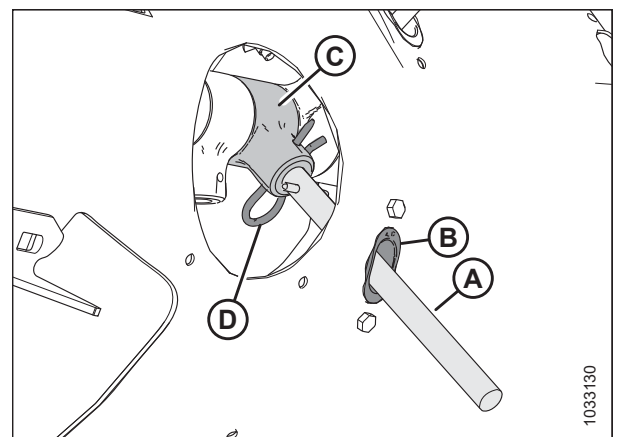
Figura 5.103: Dedo del sinfín
