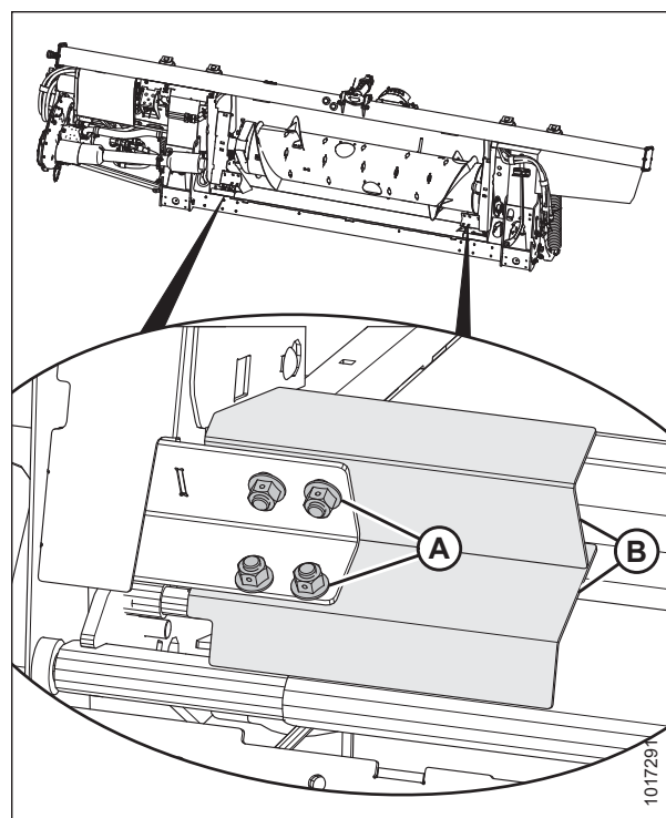
Figura 5.232: Esquinero de alimentación
