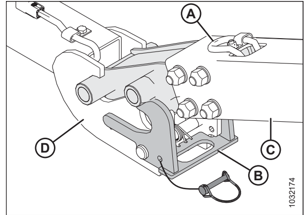
Figura 3.576: Barra de remolque/junta de extensión
