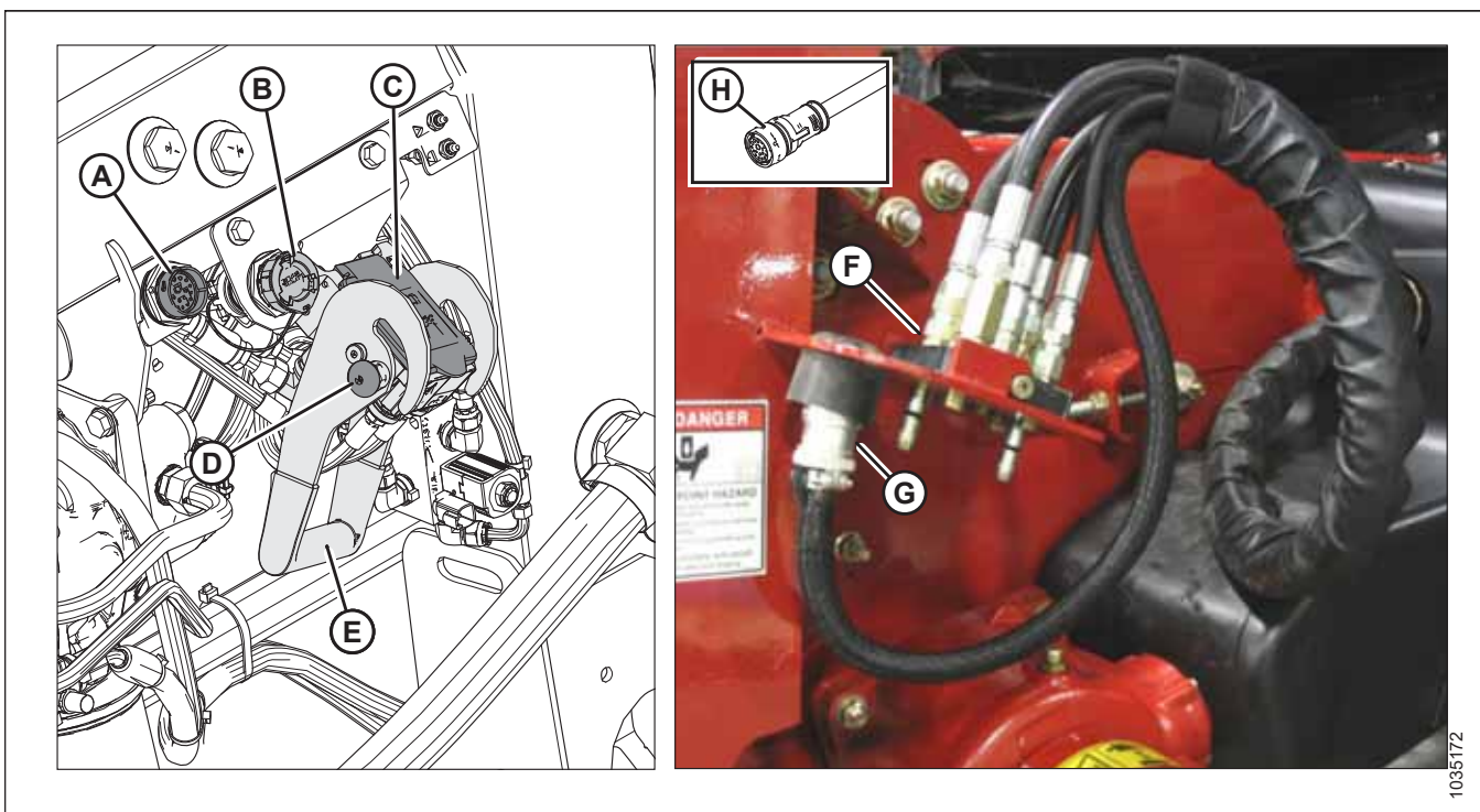
Figura 4.85: Acoplamiento múltiple y conexiones eléctricas
