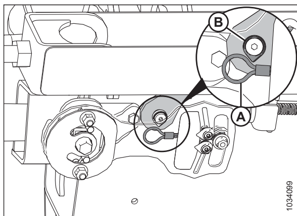
Figura 3.103: Bloqueo de cable verificador de flexión: lado izquierdo
