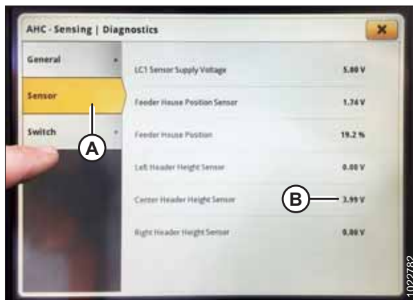
Figura 3.493: Pantalla John Deere S7 - Comprobación de la tensión del sensor
