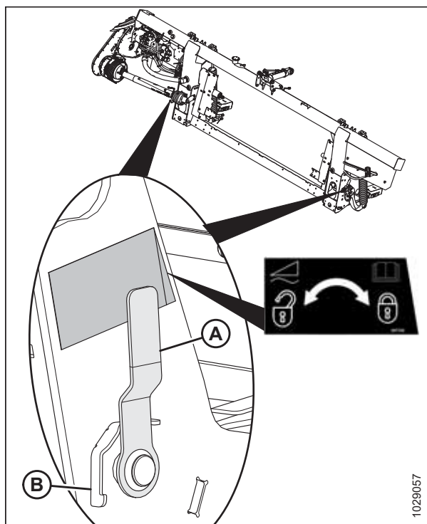
Figura 3.62: Traba de flotación de la plataforma en posición de bloqueo
