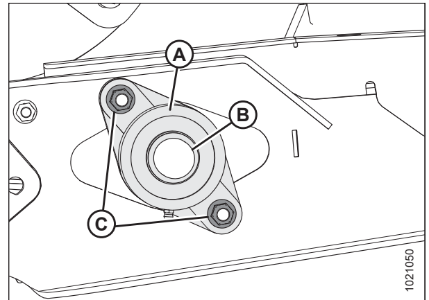
Figura 5.197: Rodamiento del rodillo de mando de la lona de alimentación
