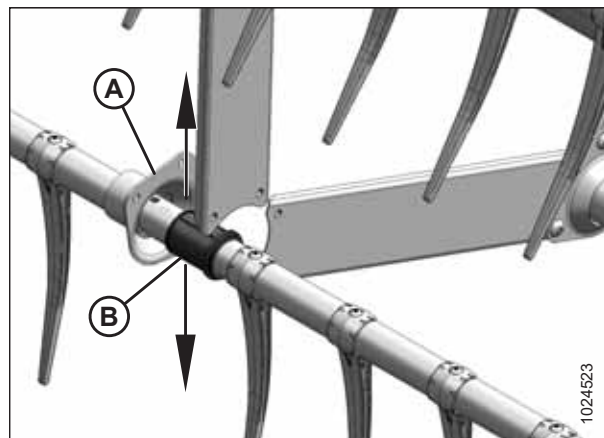
Figura 5.302: Soporte opuesto del kit de refuerzo de la barra de dientes: opcional
