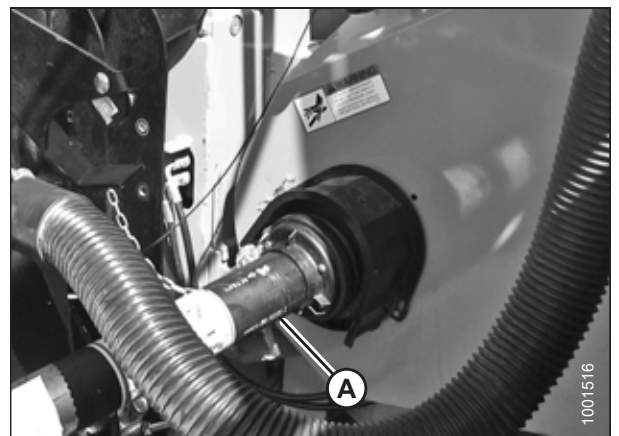
Figura 4.106: Mando y eje de salida
