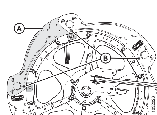
Figura 5.330: Tapas laterales del molinete: sección final exterior
