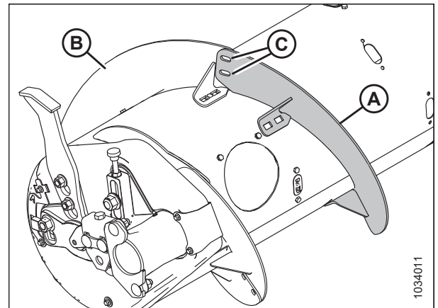
Figura 4.42: Lado izquierdo del sinfín
