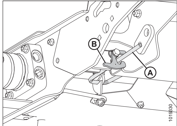
Figura 5.180: Manija de la bandeja de la plataforma de alimentación y pestillo de la manija de la bandeja lateral izquierda
