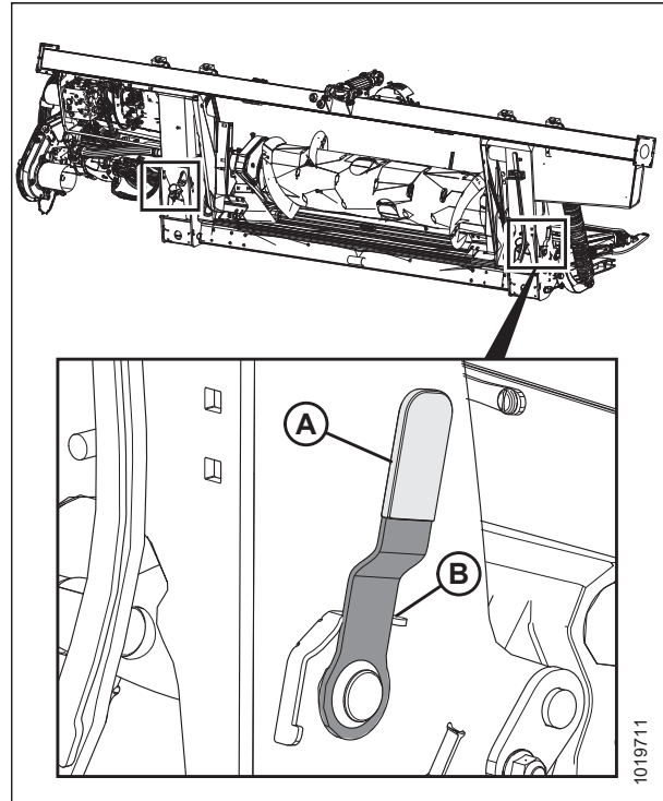
Figura 4.125: Manija de bloqueo de flotación
