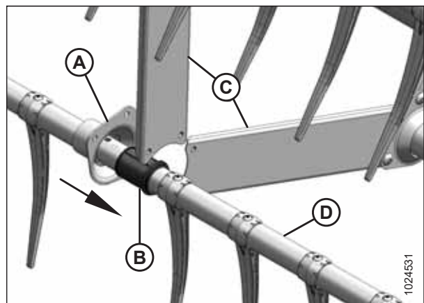
Figura 5.316: Soporte opuesto del kit de refuerzo de la barra de dientes: opcional
