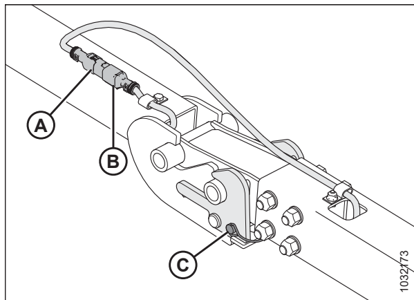
Figura 3.614: Barra de remolque/Arnés de extensión
