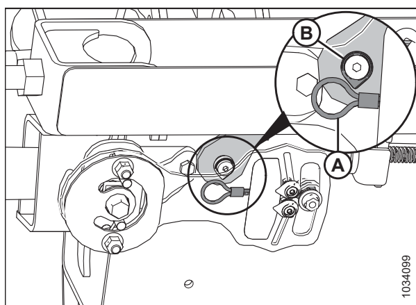
Figura 3.97: Bloqueo de cable verificador de flexión: lado izquierdo
