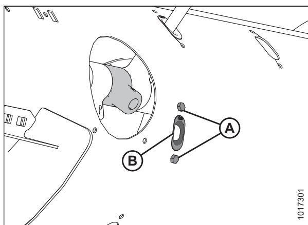
Figura 5.100: Orificio de dedos del sinfín
