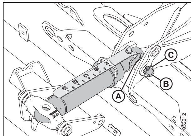
Figura 4.168: Unión central
