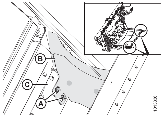
Figura 4.173: Rellenadores
