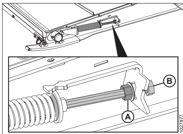
Figura 5.184: Tensor de la lona de alimentación
