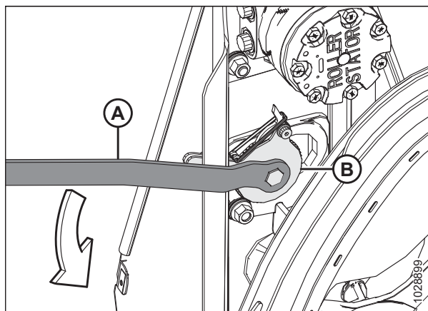
Figura 5.346: Mando del molinete
