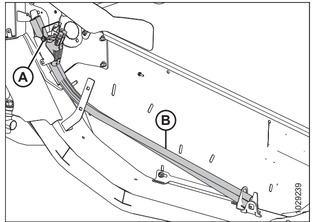
Figura 3.182: Varillas abresurcos en el Ubicación de almacenamiento en la parte final de la plataforma derecha
