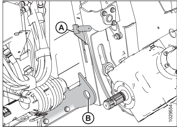
Figura 4.80: Pasadores de bloqueo del embocador
