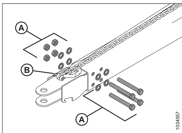
Figura 5.384: Instalación del adaptador de anillo de horquilla
