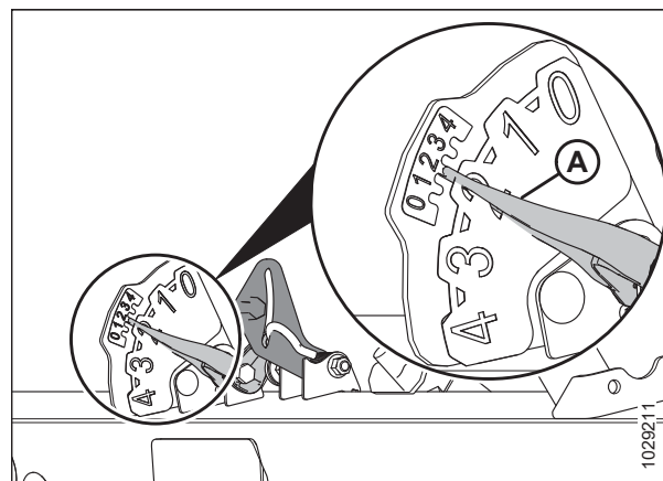
Figura 3.49: Corte al ras del suelo
