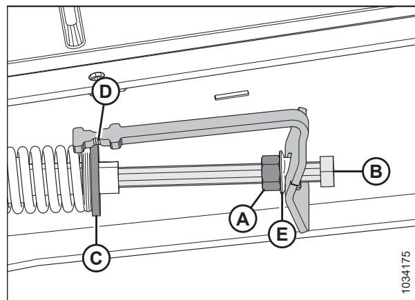
Figura 5.183: Tensionador de la lona de alimentación: lado izquierdo
