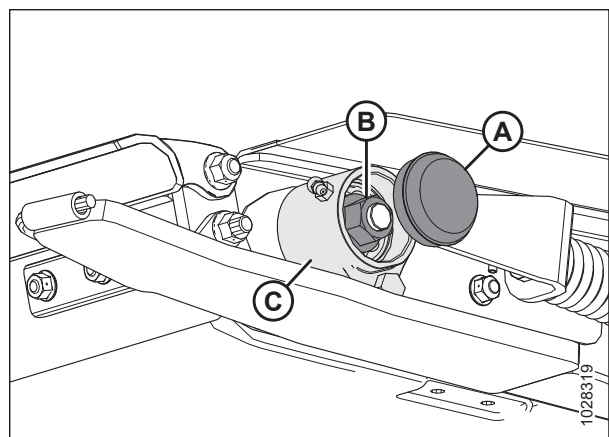
Figura 5.201: Carcasa del rodamiento del rodillo tensor
