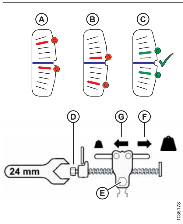
Figura 3.102: Ajuste del balance de alas (se muestra el lado izquierdo)
