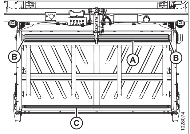
Figura 5.177: Lona de alimentación del módulo de flotación
