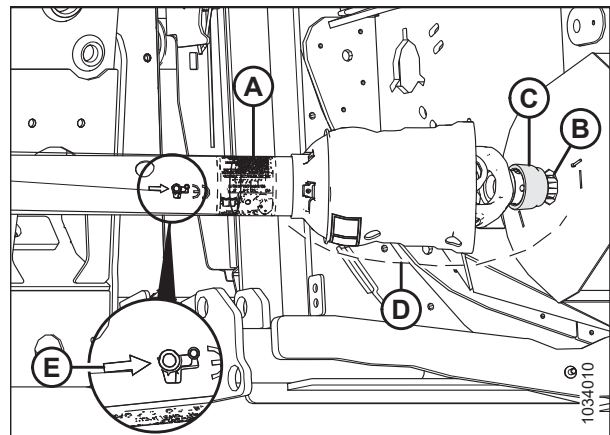
Figura 4.176: Cardán de inclinación lateral
