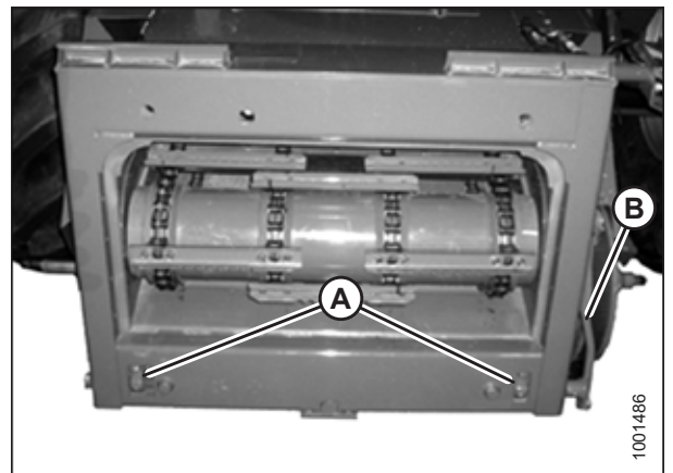
Figura 4.60: Embocador del grupo AGCO
