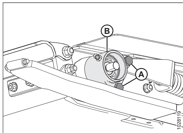
Figura 5.202: Carcasa del rodamiento del rodillo tensor
