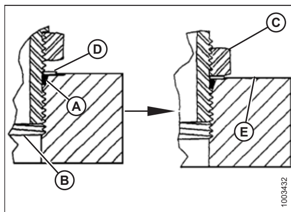
Figura 8.7: Accesorio hidráulico
