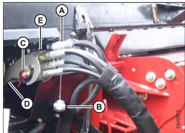
Figura 4.93: Acoplador múltiple
