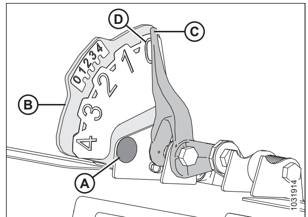
Figura 3.287: Indicador de flotación
