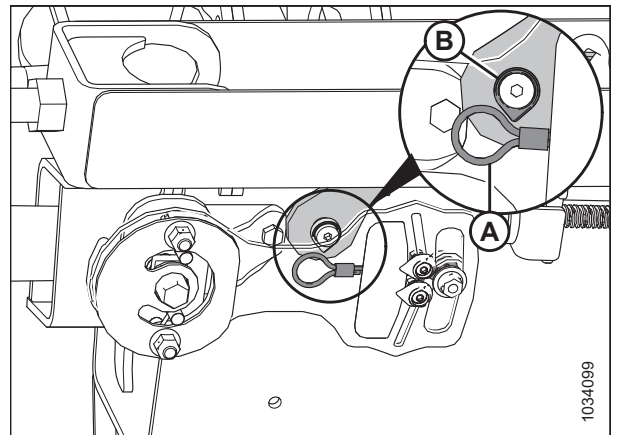
Figura 3.76: Bloqueo de cable verificador de flexión: lado izquierdo
