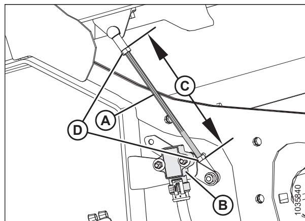
Figura 3.132: Sensor de altura del molinete: brazo derecho del molinete con molinete hacia abajo
