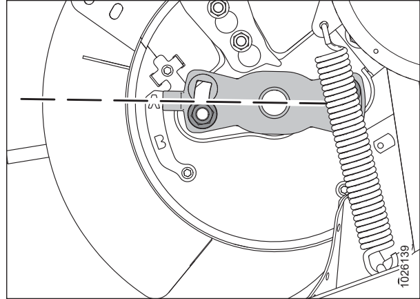
Figura 5.107: Posición A del sinfín
