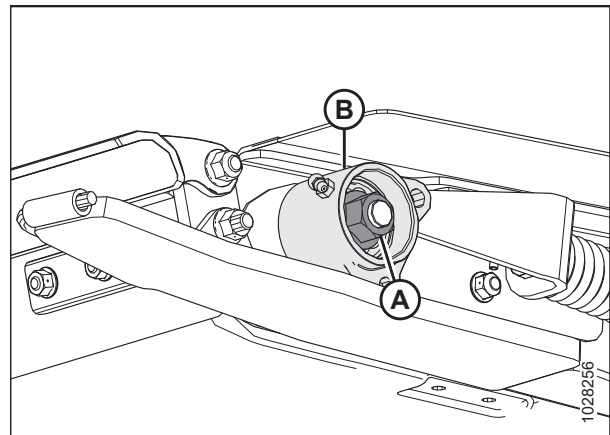
Figura 5.217: Rodamiento de rodillo tensor: lado izquierdo
