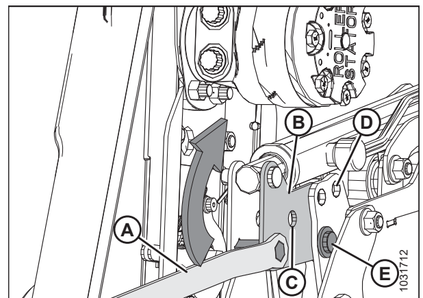
Figura 3.151: Cilindro del brazo central izquierdo: Posición de avance
