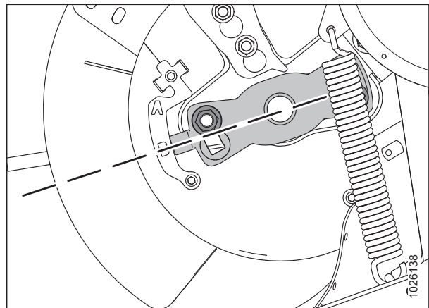
Figura 5.108: Posición B del sinfín
