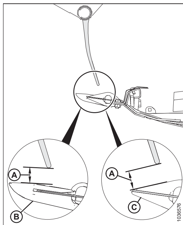
Figura 5.267: Separación de los dientes
