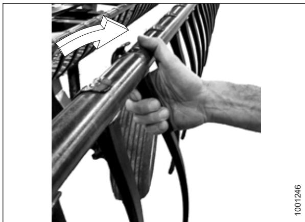
Figura 5.287: Instalación de dientes de plástico
