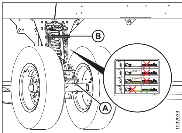
Figura 3.36: Rueda izquierda
