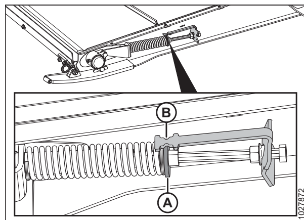
Figura 5.182: Tensor de la lona de alimentación
