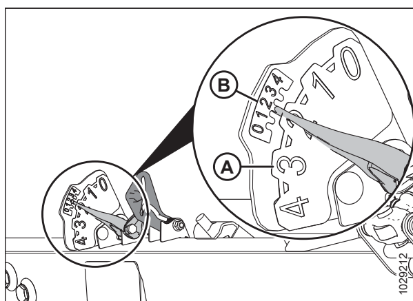
Figura 3.48: Indicador de flotación: lado izquierdo
