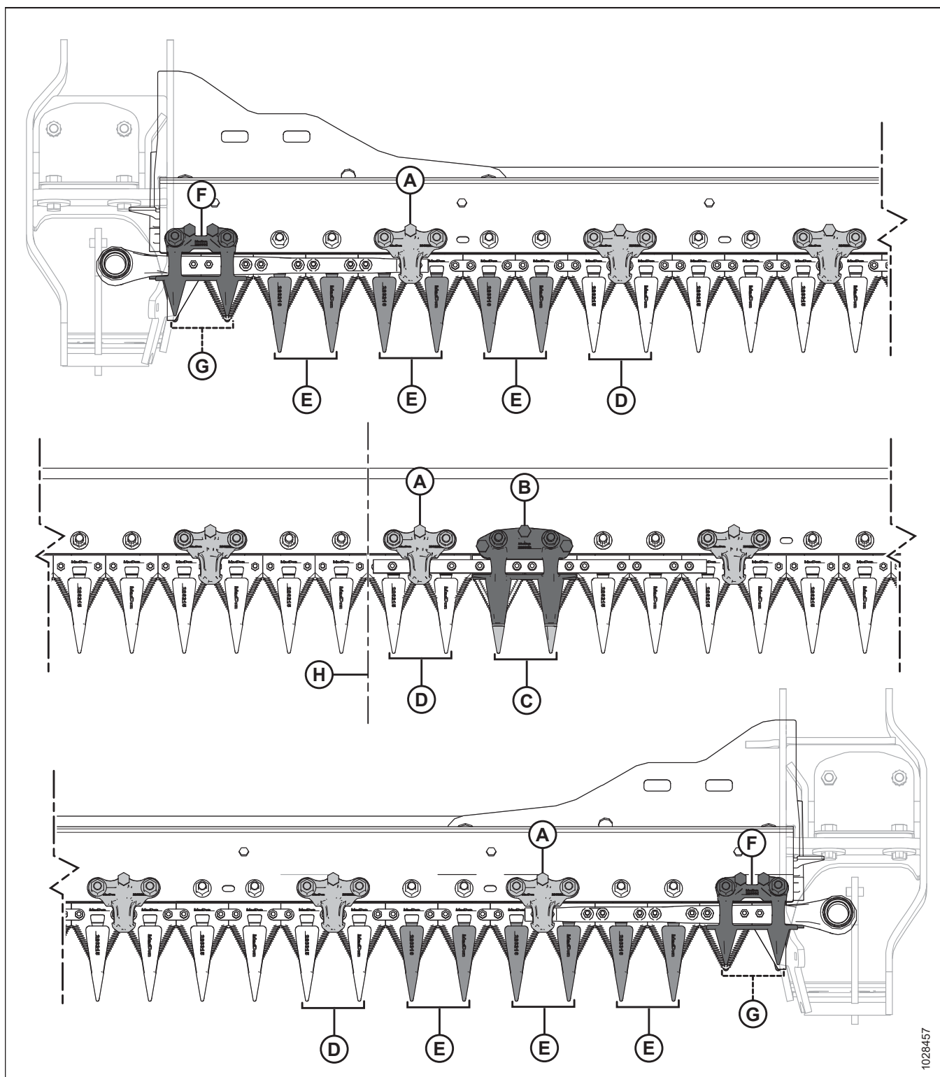
Figura 5.126: Puntón de cuchilla puntiagudo y ubicaciones del sujetador: plataforma de doble cuchilla FD240
