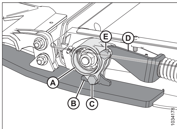
Figura 5.211: Rodamiento de rodillo tensor: lado izquierdo
