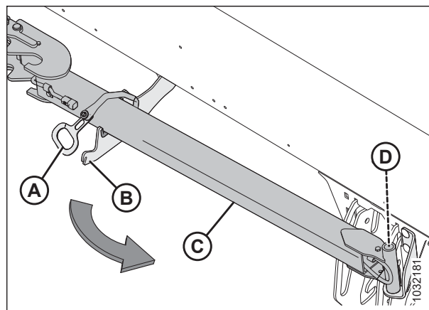
Figura 3.608: Extensión de la barra de remolque en almacenamiento
