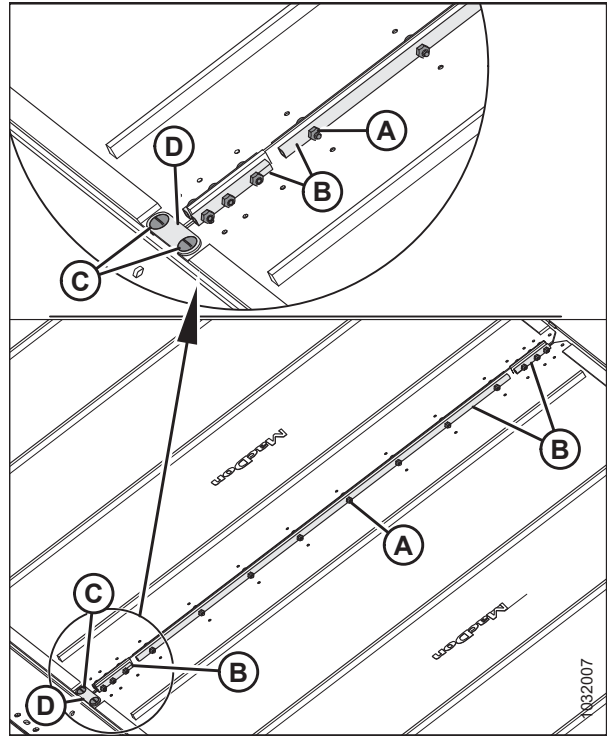
Figura 5.246: Conectores de la lona
