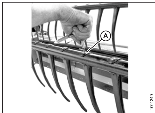
Figura 5.285: Extracción del diente de plástico
