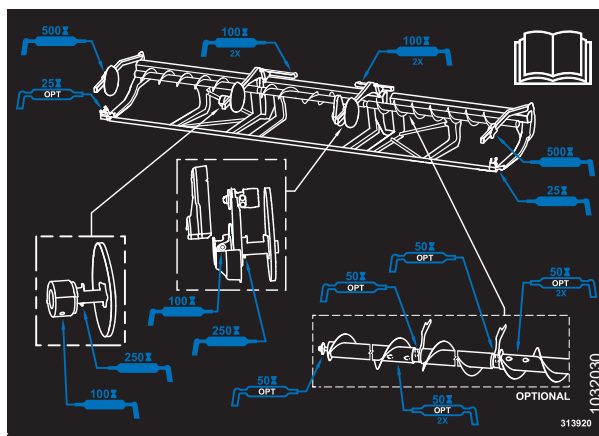
Figura 5.18: Calcomanía de diseño de punto de engrase serie FD2
