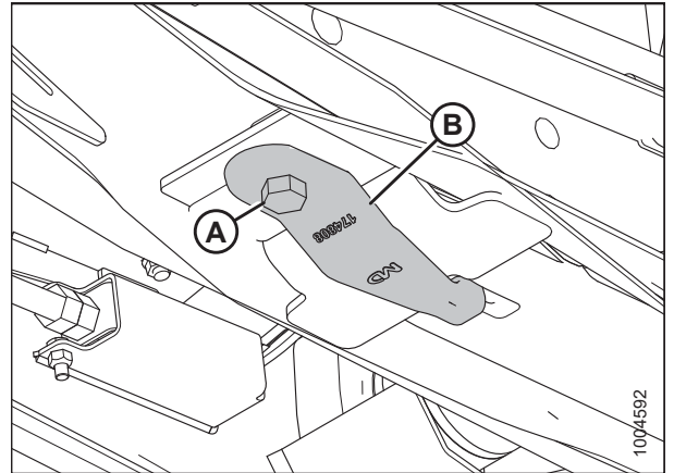
Figura 4.159: Parte inferior del módulo de flotación
