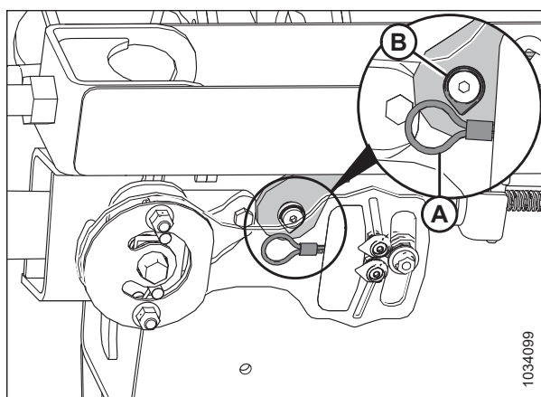
Figura 3.84: Bloqueo de cable verificador de flexión: lado izquierdo
