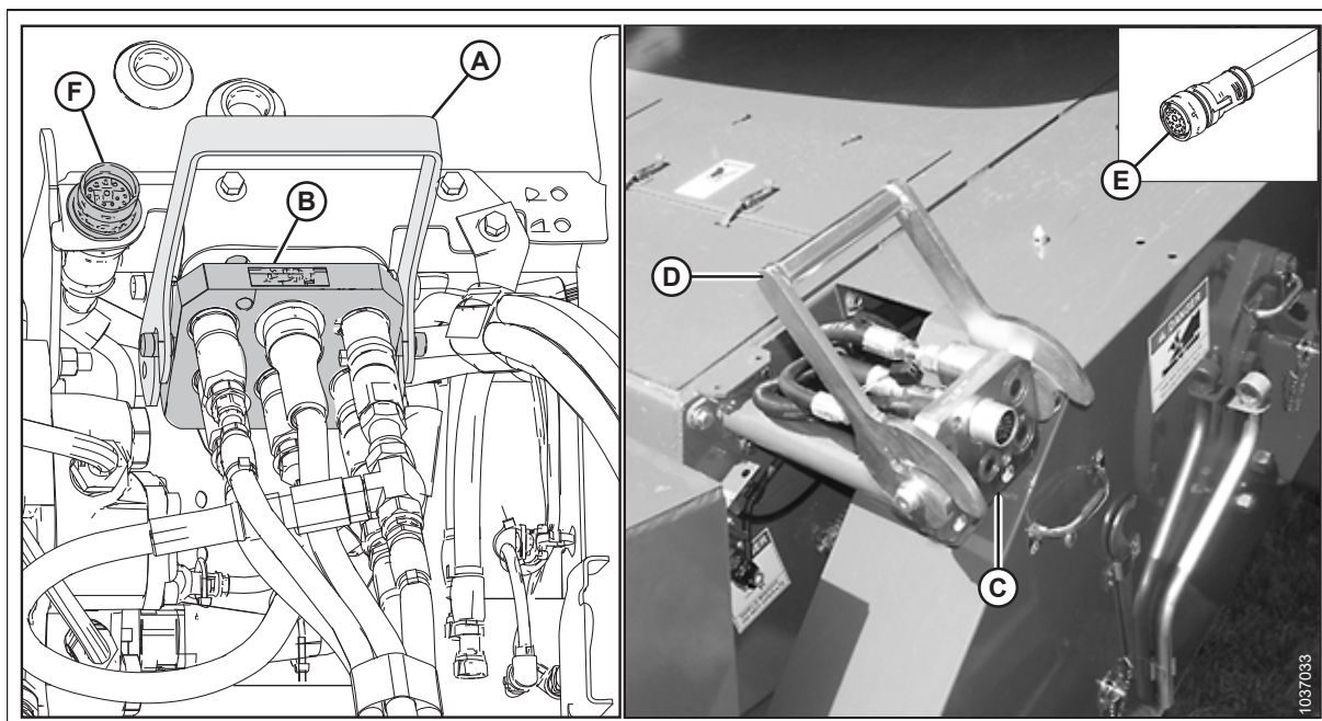
Figura 4.68: Hidráulica y acoplamiento múltiple eléctrico
