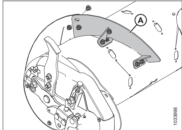
Figura 4.39: Ala corta: lado izquierdo
