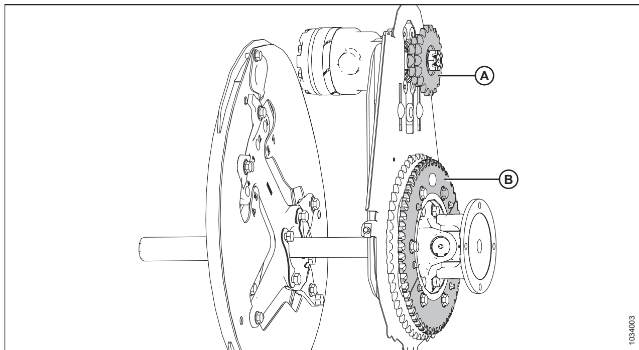
Figura 3.123: Mando del molinete con piñones opcionales
