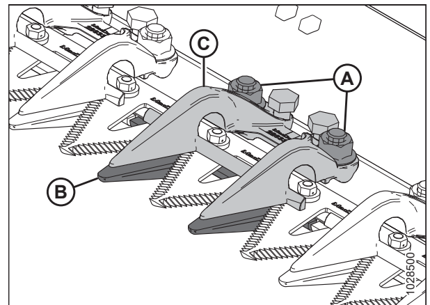
Figura 5.153: Puntones de cuchilla cortos
