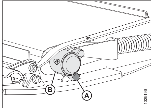
Figura 5.174: Rodillo tensor
