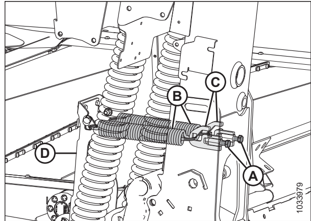
Figura 4.156: Resorte de recorte: lado izquierdo
