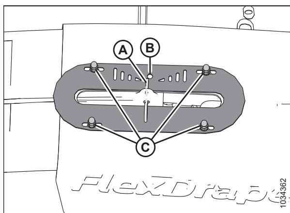
Figura 3.85: Indicador de movimiento del ala en la parte superior de la cubierta de conexión de flexión: se muestra el lado izquierdo
