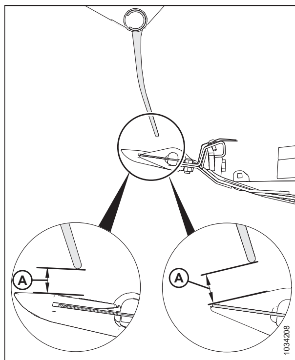
Figura 5.272: Medición desde la punta del dedo hasta el puntón
