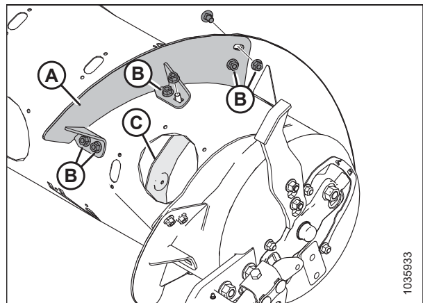
Figura 4.29: Ala corta: lado derecho
