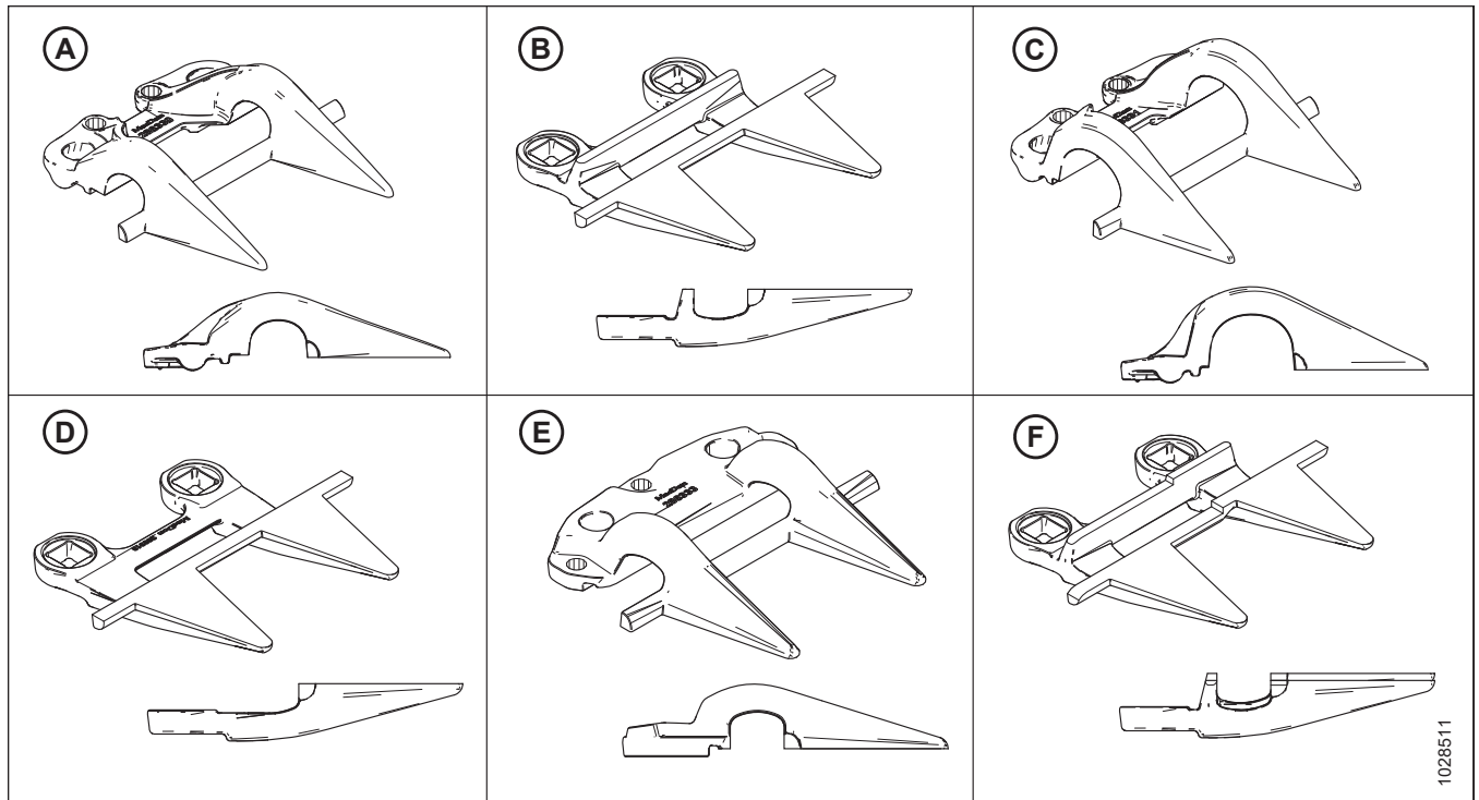
Figura 5.149: Tipos de puntón y sujetador utilizados en las configuraciones de puntón de cuchilla corto
