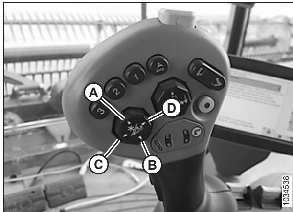
Figura 3.41: Joystick
