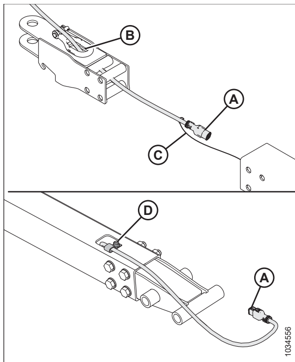
Figura 5.383: Instalación del adaptador de anillo de horquilla
