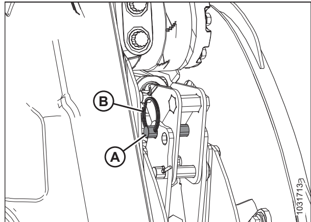
Figura 3.142: Cilindro del brazo central: Posición de retroceso
