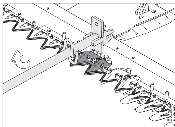
Figura 5.131: Ajuste hacia arriba: puntón de cuchilla corto
