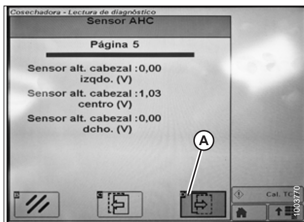
Figura 3.437: Pantalla de la cosechadora John Deere
