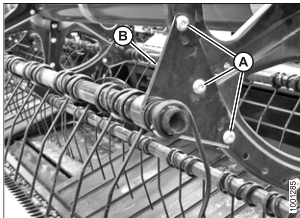
Figura 5.283: Brazo de la barra de dientes
