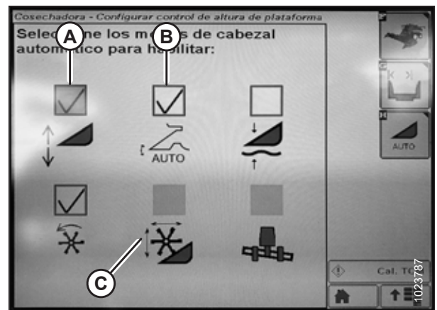
Figura 3.454: Pantalla de la cosechadora
