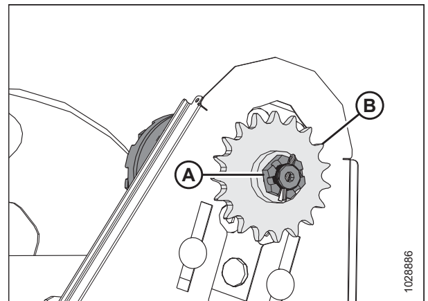
Figura 5.364: Mando del molinete
