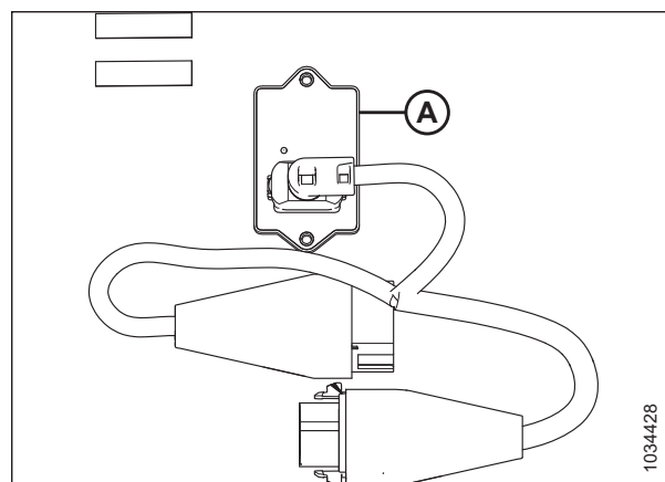
Figura 3.204: Adaptador de 10 V (MD n.º B7241)
