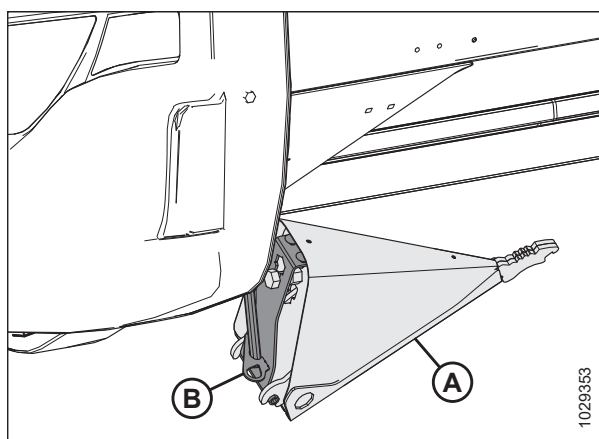
Figura 3.175: Almacenamiento opcional del divisor de cosecha
