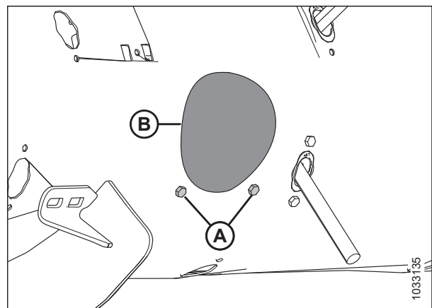
Figura 4.55: Cubierta del orificio de acceso del sinfín
