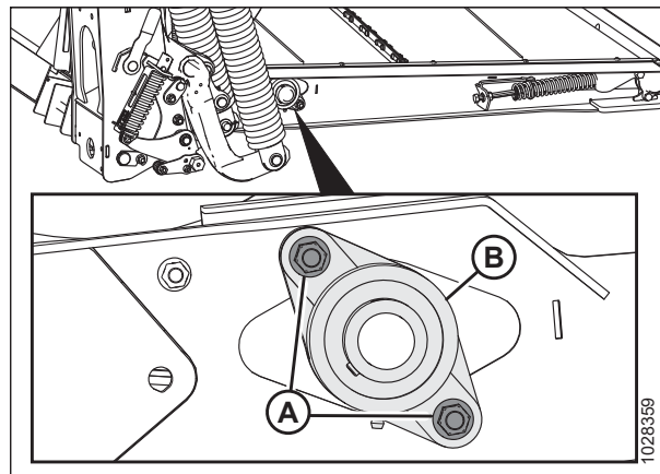
Figura 5.186: Rodamiento del rodillo de mando
