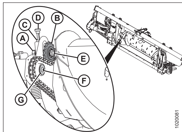
Figura 5.75: Mando del sinfín
