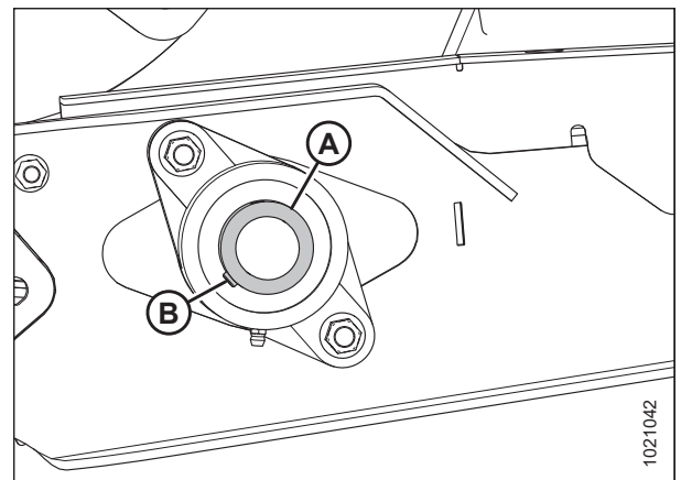
Figura 5.198: Rodamiento del rodillo de mando de la lona de alimentación
