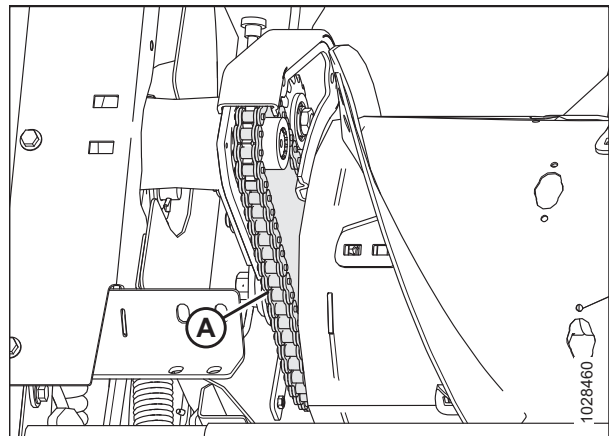
Figura 5.70: Cadena del sinfín de alimentación: vista trasera
