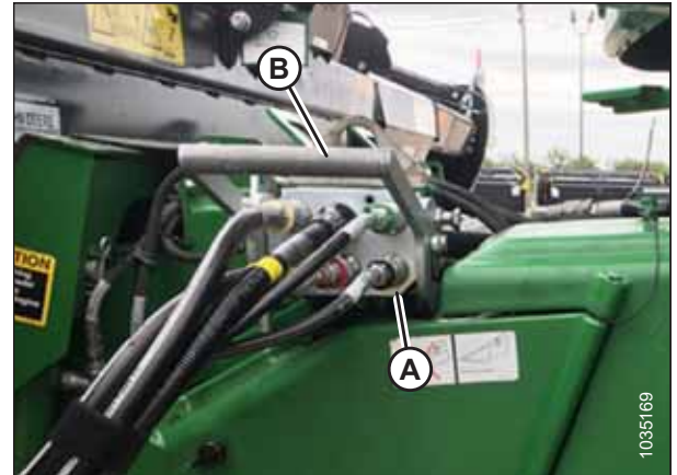
Figura 4.118: Acoplador múltiple
