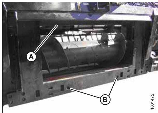
Figura 4.57: Módulo de flotación
