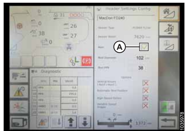
Figura 3.211: Configuraciones de la plataforma
