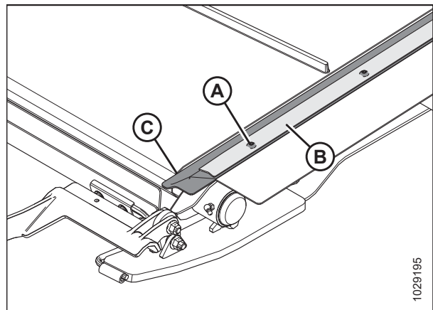
Figura 5.181: Sello de la lona
