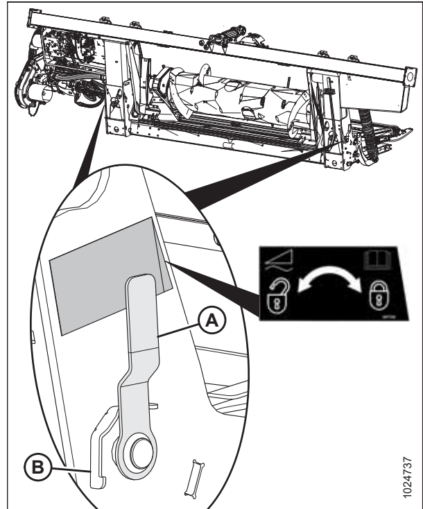
Figura 4.107: Manija de bloqueo de flotación
