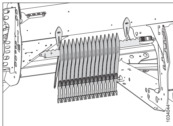
Figura 6.2: Kit de bastidor para elevador de cultivo: lado izquierdo
