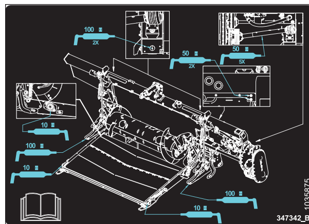
Figura 5.17: Calcomanía de diseño de punto de engrase FM200
