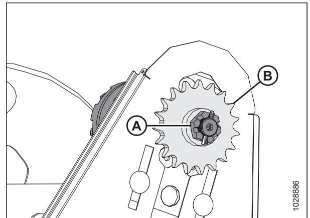
Figura 5.350: Piñón único
