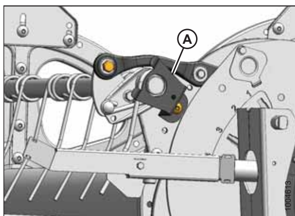
Figura 5.309: Extremo de leva
