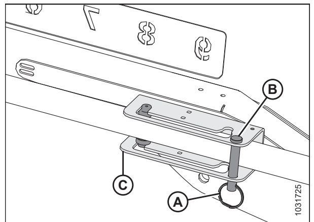
Figura 3.146: Cilindro del brazo izquierdo: Posición de avance
