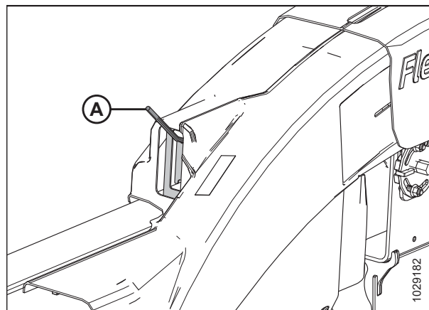
Figura 3.86: Ala en la posición de bloqueo
