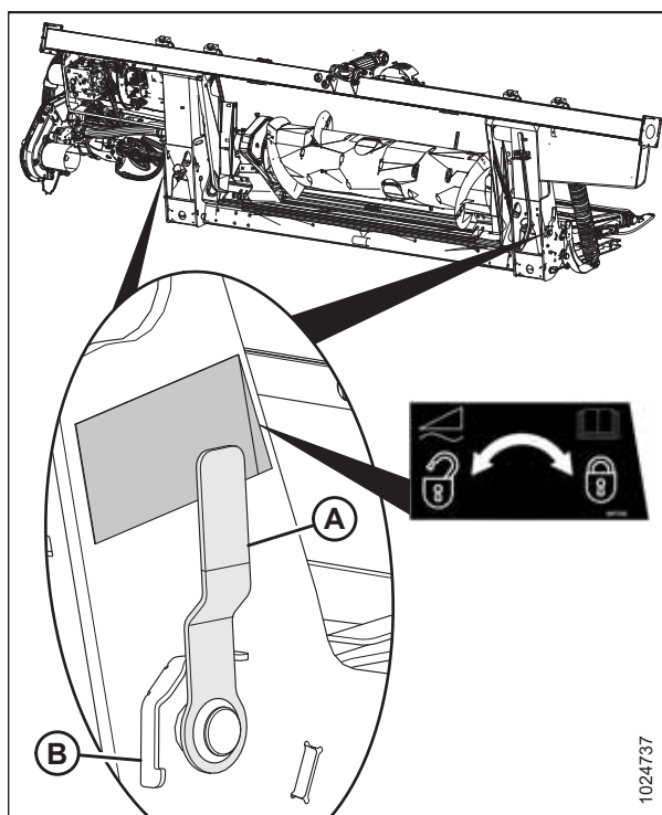
Figura 3.567: Traba de flotación de la plataforma en posición de bloqueo
