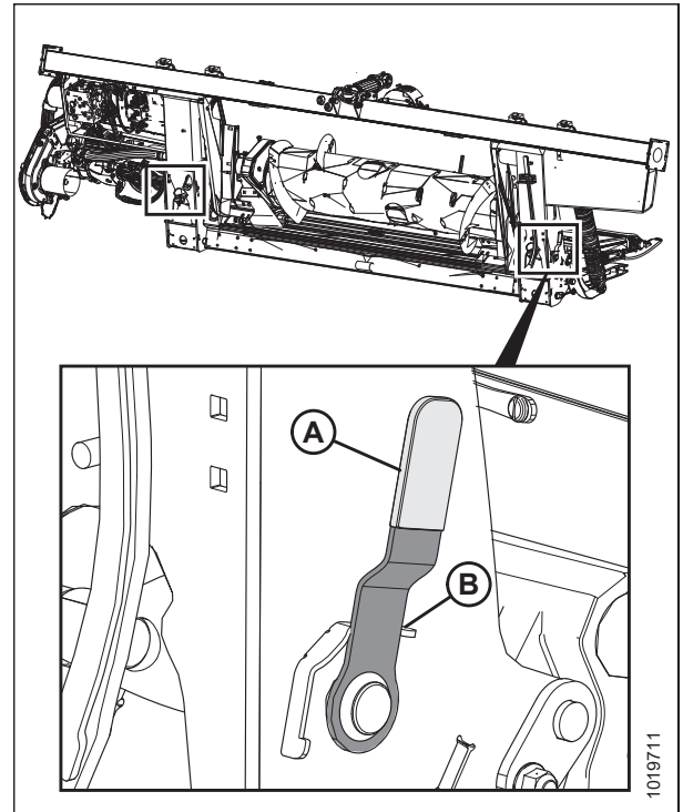
Figura 4.90: Manija de bloqueo de flotación
