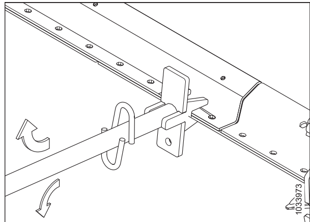
Figura 5.134: Ajuste de la barra de puntón: sin puntones
