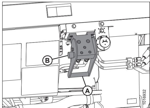
Figura 4.145: Receptáculos del módulo de flotación
