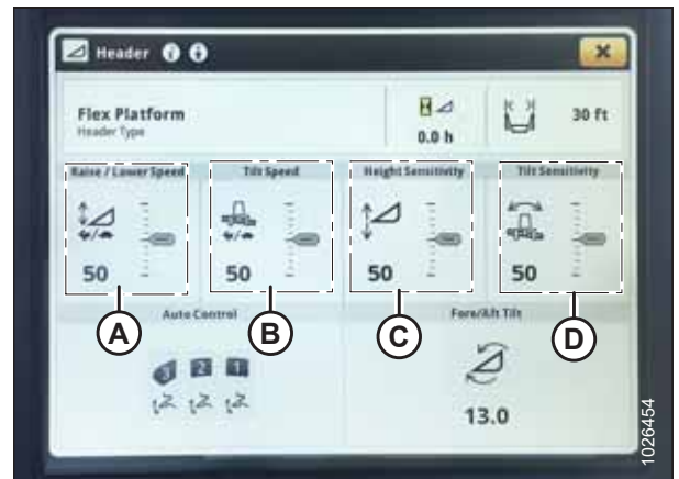
Figura 3.483: Pantalla John Deere S7 - Página de la plataforma
