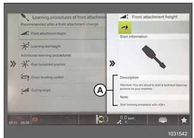
Figura 3.353: Página de altura del accesorio delantero
