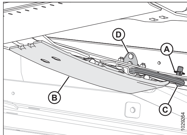
Figura 3.46: Patín interno
