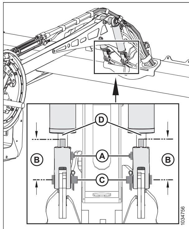
Figura 5.278: Cilindro del brazo central
