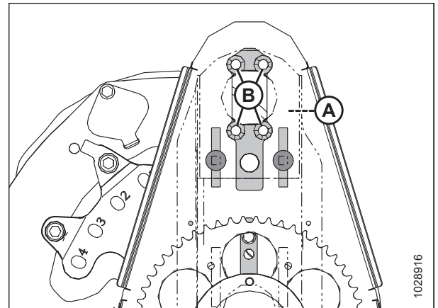
Figura 5.362: Orificios de montaje del motor del mando del molinete
