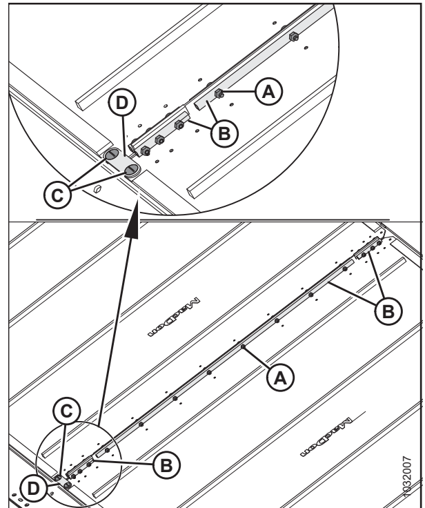
Figura 5.254: Conector de la lona
