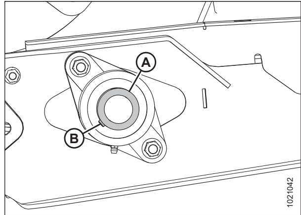
Figura 5.194: Rodamiento del rodillo de mando de la lona de alimentación
