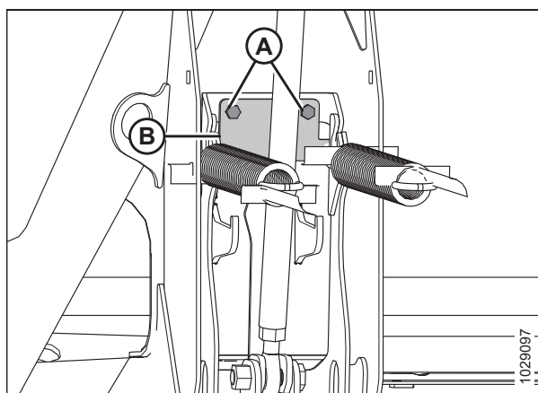
Figura 3.92: Placa limitadora de "cara triste" de flexión
