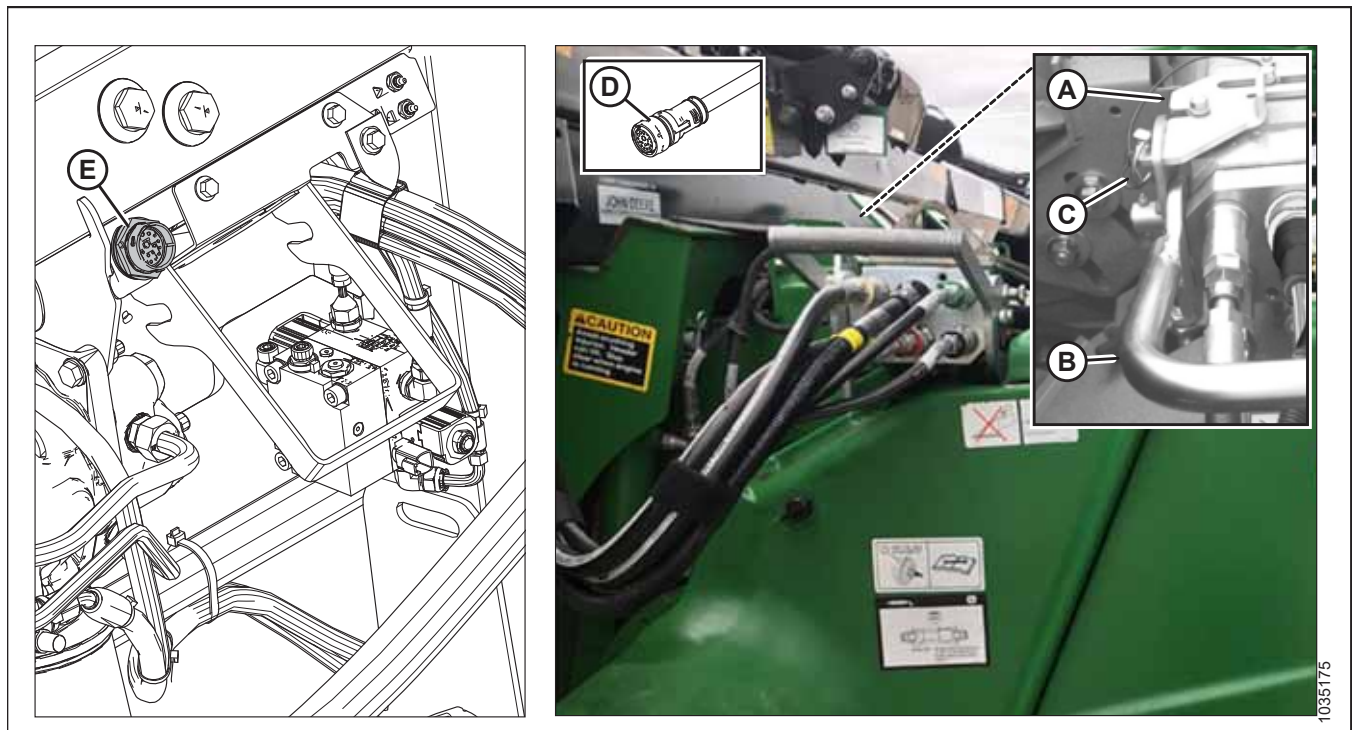
Figura 4.119: Clavija del embocador
