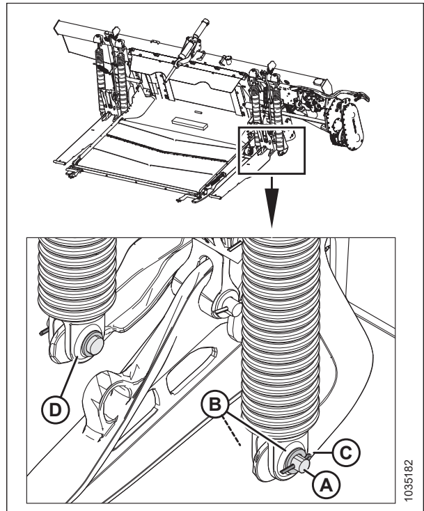
Figura 3.66: Resorte de flotación izquierdo instalado en el agujero de la palanca de flotación trasera
