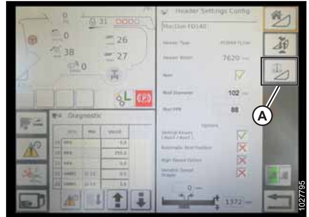
Figura 3.223: Página de configuraciones de la plataforma
