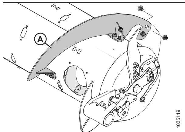
Figura 4.30: Ala larga: lado derecho
