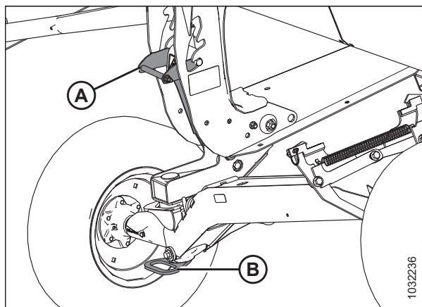
Figura 3.603: Ruedas de calibración
