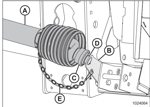
Figura 4.143: Mando
