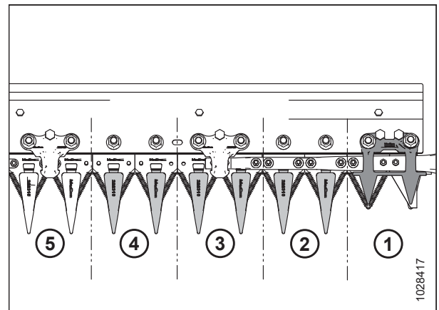
Figura 5.135: Puntones de cuchilla puntiagudos laterales de mando
