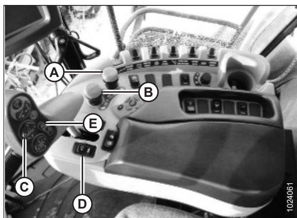
Figura 3.524: Controles de la cosechadora New Holland
