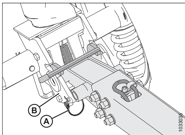
Figura 3.581: Barra de remolque y pivote de transporte
