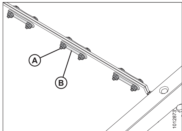
Figura 5.200: Conector de la lona
