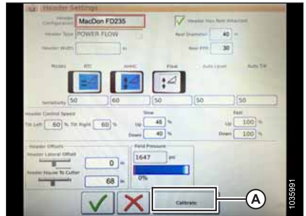
Figura 3.401: Página de configuraciones de la plataforma
