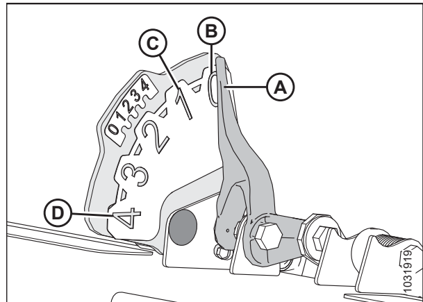
Figura 3.451: Indicador de flotación
