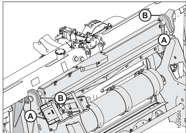
Figura 4.81: Bajar el embocador
