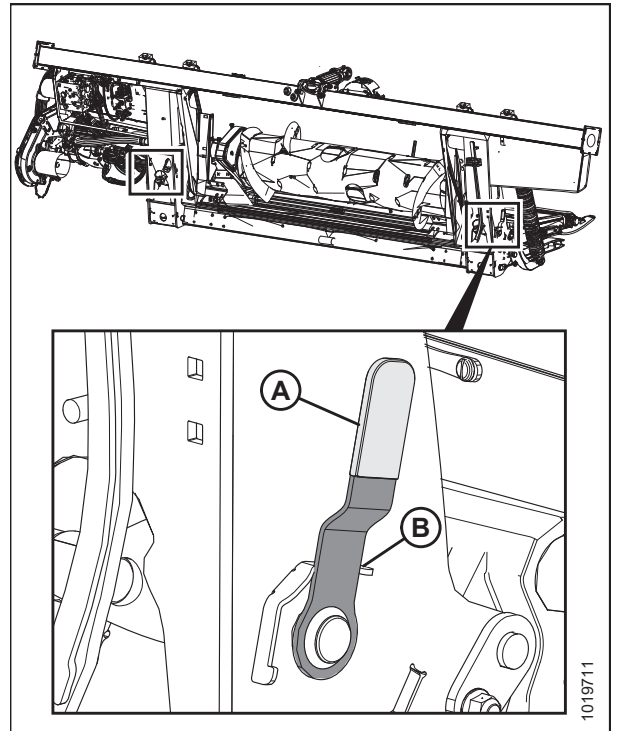
Figura 4.155: Traba de flotación
