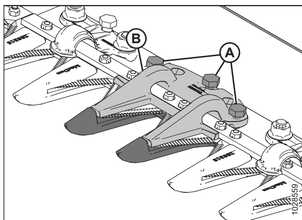
Figura 5.145: Puntón de cuchilla central puntiagudo
