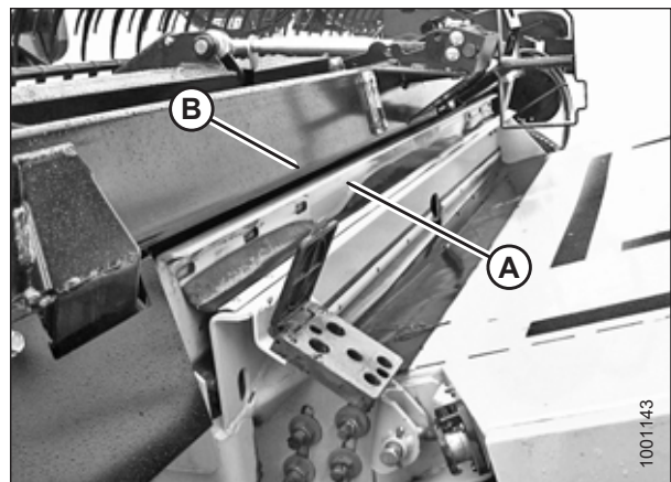
Figura 4.151: Plataforma en la cosechadora
