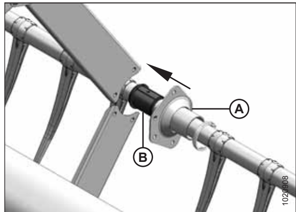
Figura 5.315: Soporte del kit de refuerzo de la barra de dientes: opcional
