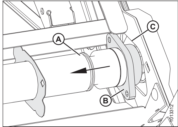
Figura 5.189: Rodillo de mando
