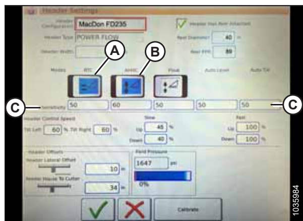
Figura 3.396: Controles automáticos y configuraciones de sensibilidad
