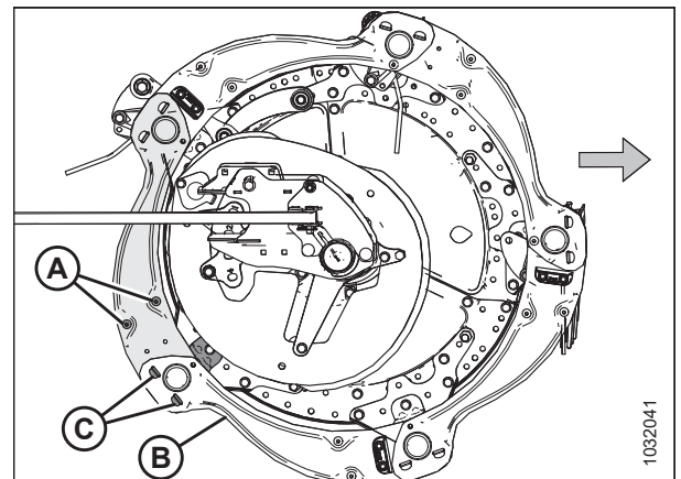
Figura 5.323: Tapas laterales del molinete: extremo de leva exterior
