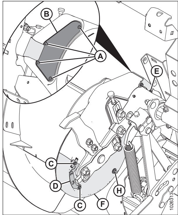
Figura 5.69: Mando del sinfín de alimentación: vista trasera
