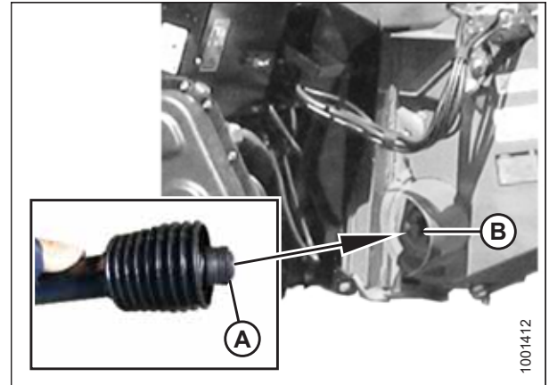
Figura 4.123: Mando
