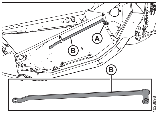
Figura 5.343: Ubicación de almacenamiento de la herramienta múltiple
