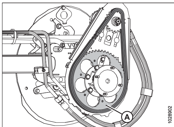
Figura 5.348: Mando del molinete
