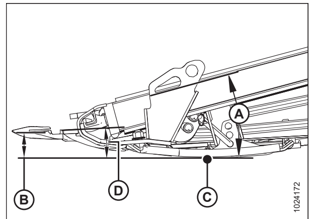
Figura 3.105: Ángulo de la plataforma
