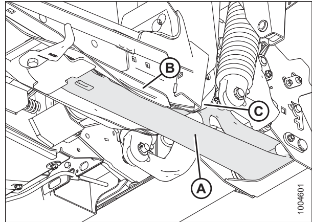
Figura 4.166: Parte inferior del módulo de flotación
