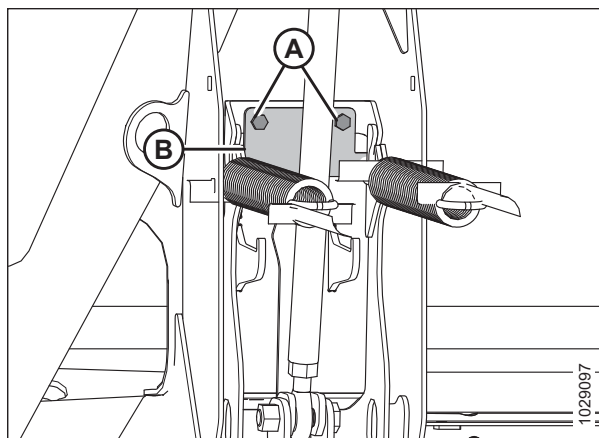
Figura 3.89: Placa limitadora de "cara triste" de flexión
