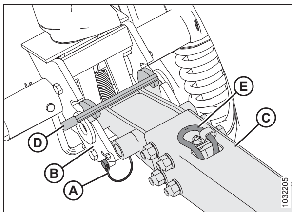
Figura 3.616: Barra de remolque y pivote de transporte
