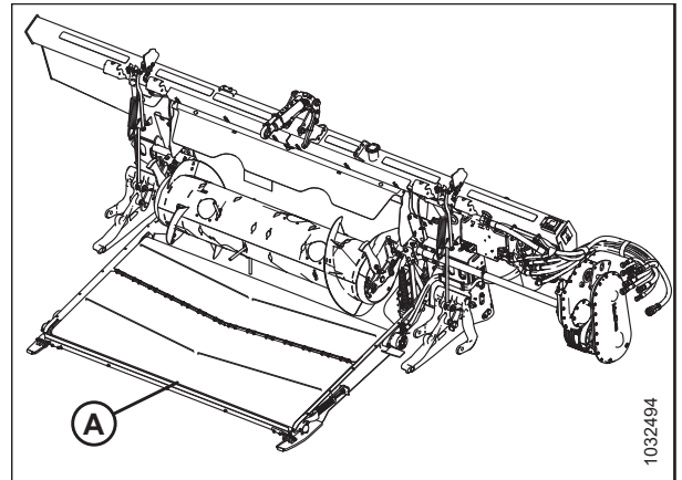
Figura 3.128: Módulo de flotación FM200
