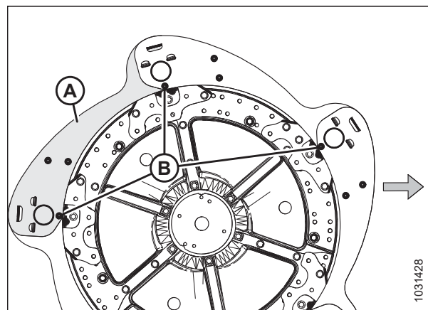
Figura 5.326: Tapas laterales del molinete: extremo de leva interior
