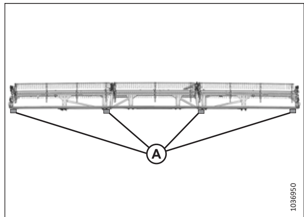
Figura 5.270: Ubicaciones de los bloques de FlexDraper®: molinete triple
