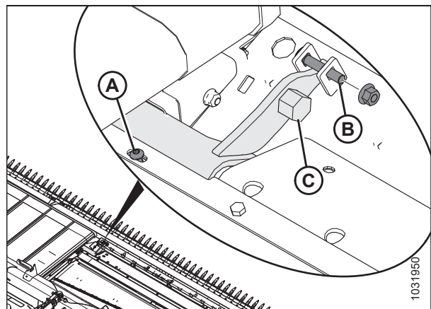
Figura 4.158: Pestillo del módulo de flotación
