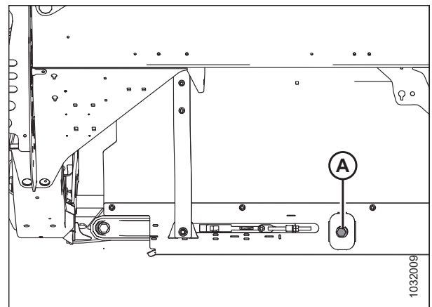
Figura 5.255: Tensor de la lona
