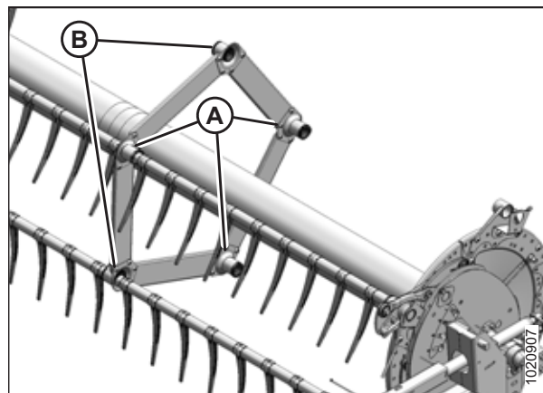
Figura 5.294: Soportes de la barra de dientes
