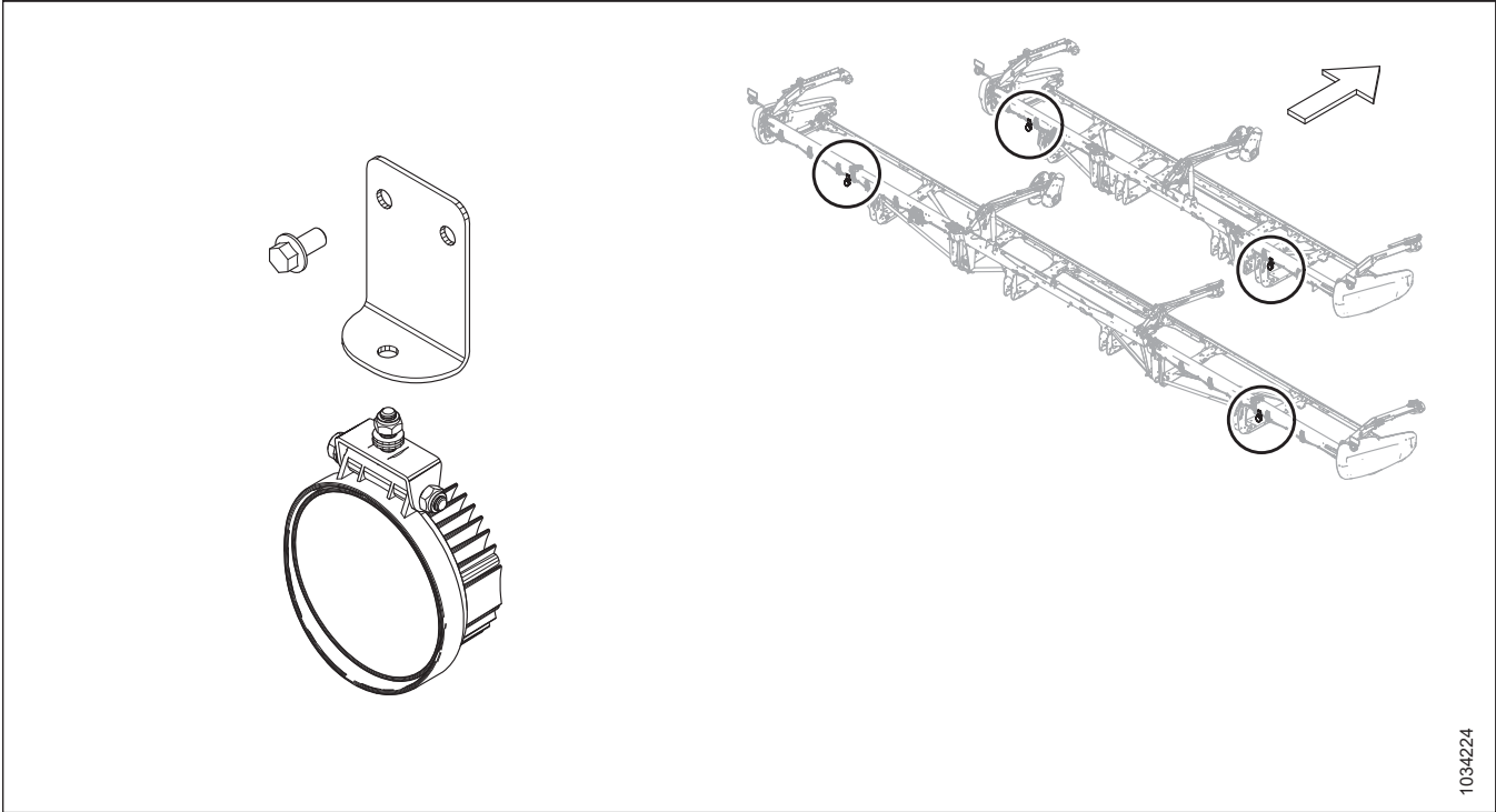
Figura 6.18: Kit de luz de rastreo
