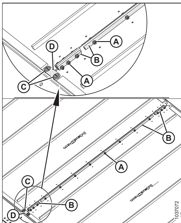
Figura 5.237: Conectores de la lona
