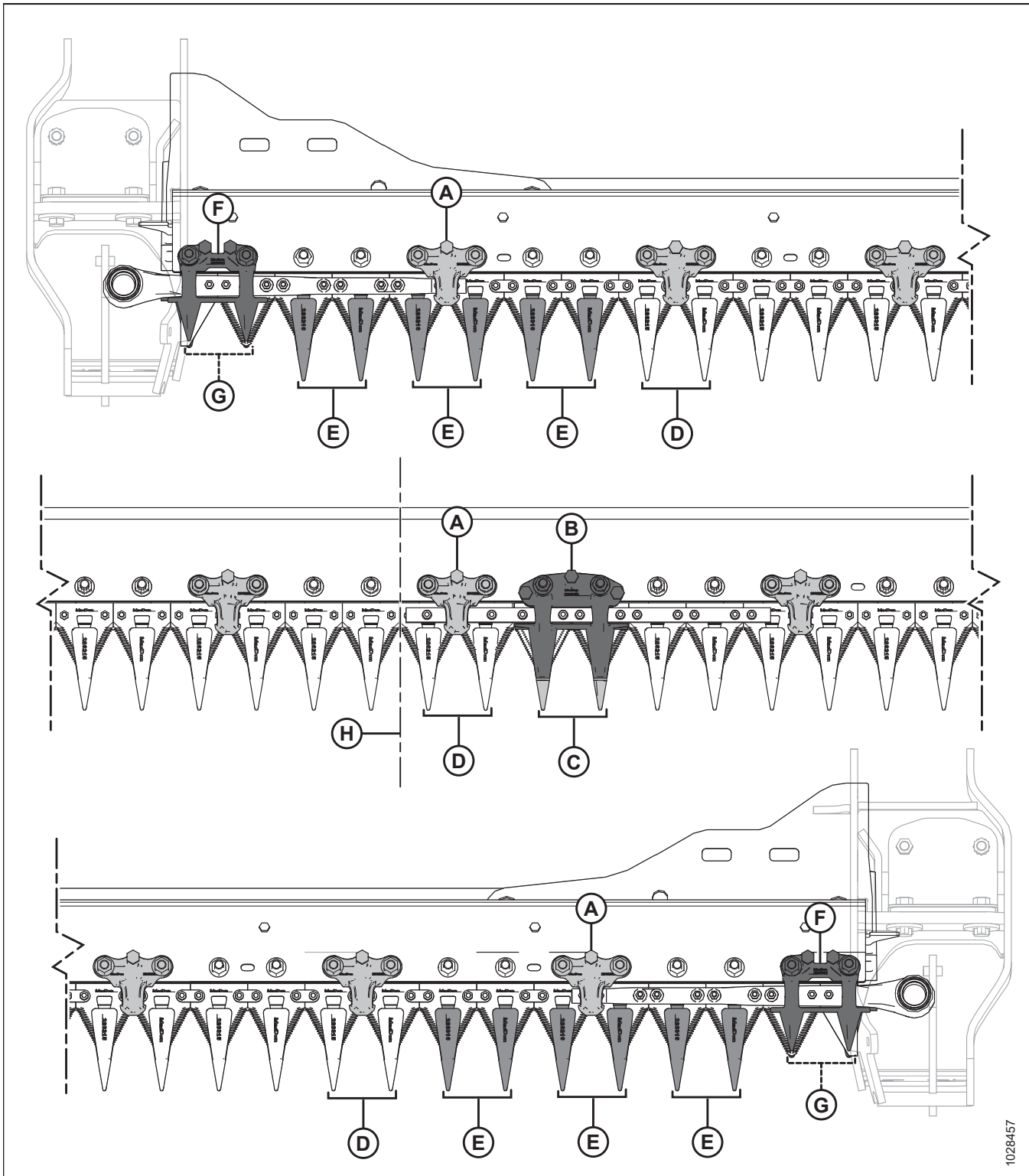
Figura 5.129: Puntón de cuchilla puntiagudo y ubicaciones del sujetador: plataforma de cuchilla doble FD250
