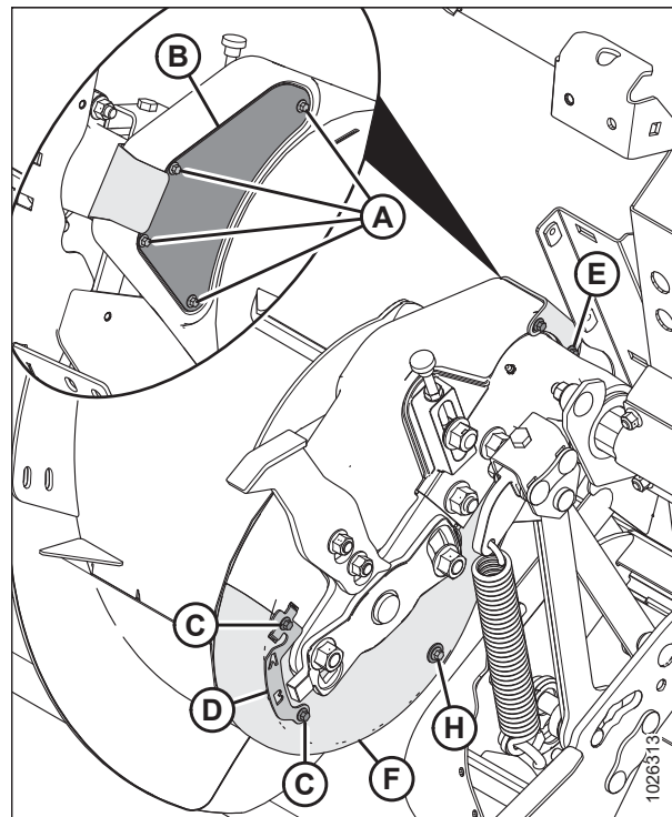
Figura 5.71: Mando del sinfín de alimentación: vista trasera
