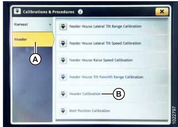
Figura 3.503: Pantalla John Deere S7 - Calibraciones y procedimientos
