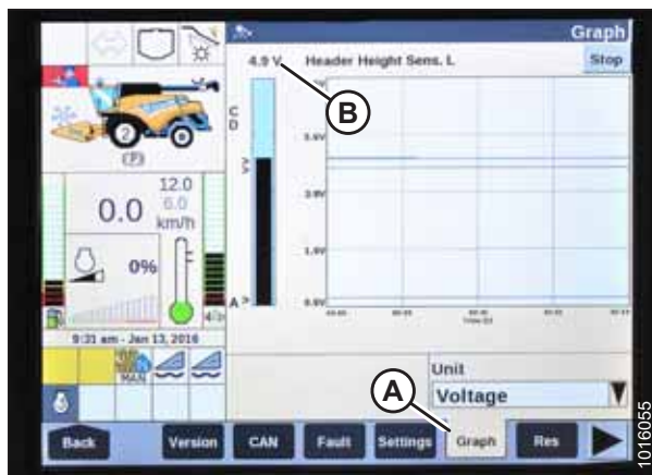
Figura 3.531: Pantalla de la cosechadora New Holland
