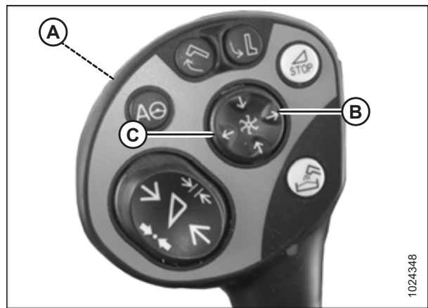
Figura 3.118: Joystick CLAAS 500
