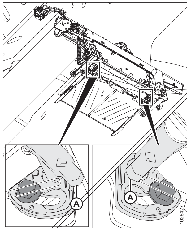
Figura 3.186: Brazos de ajuste de flotación del sinfín
