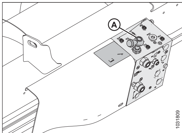
Figura 3.167: Válvula de cierre
