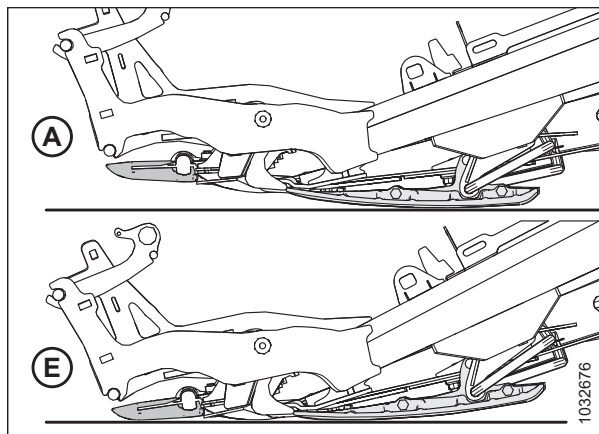
Figura 3.107: Ángulos del puntón
