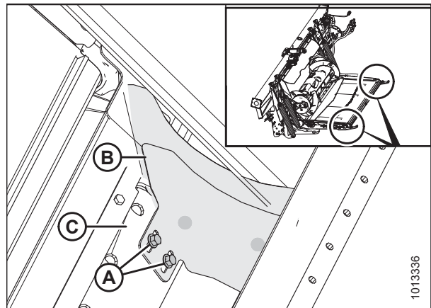
Figura 4.157: Rellenadores
