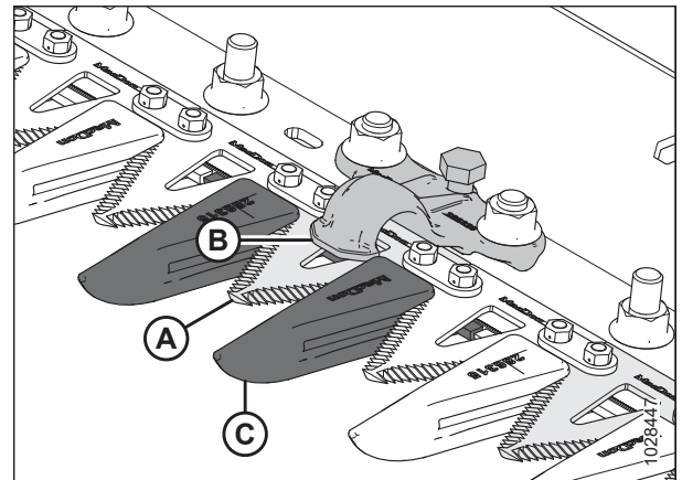
Figura 5.139: Sujetador puntiagudo
