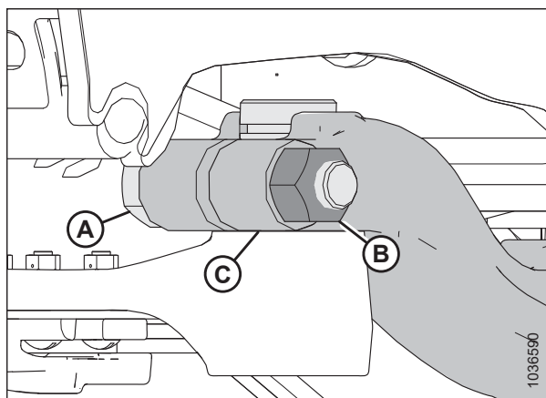
Figura 5.119: Cabeza de la cuchilla
