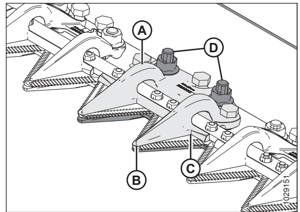
Figura 5.165: Sujetador del puntón de cuchilla central
