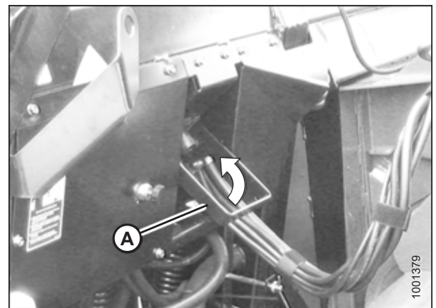
Figura 4.128: Almacenamiento del acoplamiento múltiple
