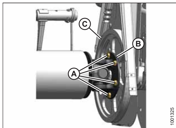
Figura 5.357: Cruceta
