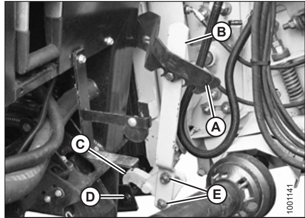
Figura 4.135: Trabas del embocador
