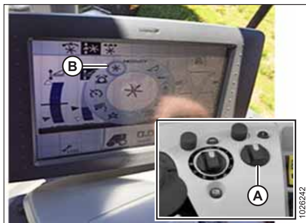
Figura 3.344: Pantalla y consola de la cosechadora CLAAS
