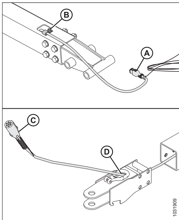
Figura 5.387: Extracción del adaptador de remolque de la horquilla
