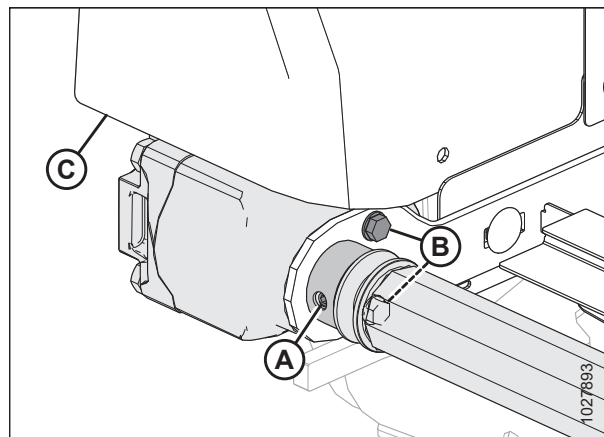
Figura 5.264: Rodillo de mando
