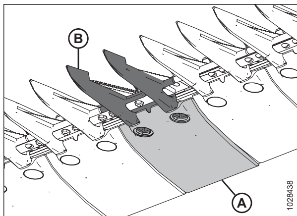
Figura 5.144: Puntón de cuchilla central puntiagudo y placa de desgaste
