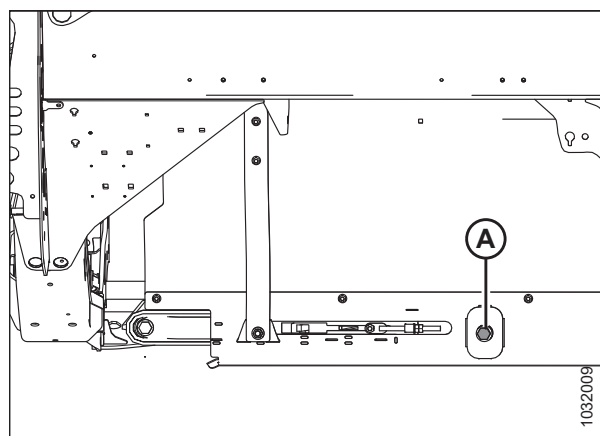
Figura 5.245: Tensionador: se muestra el lado izquierdo
