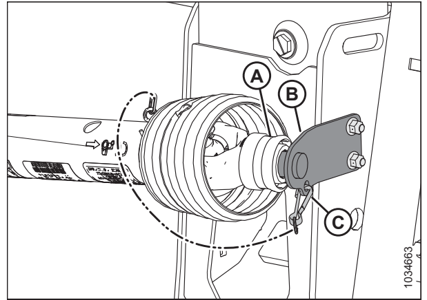
Figura 4.104: Cardán en posición de almacenamiento: Cardán MD n.º B7038 o MD n.º B7039
