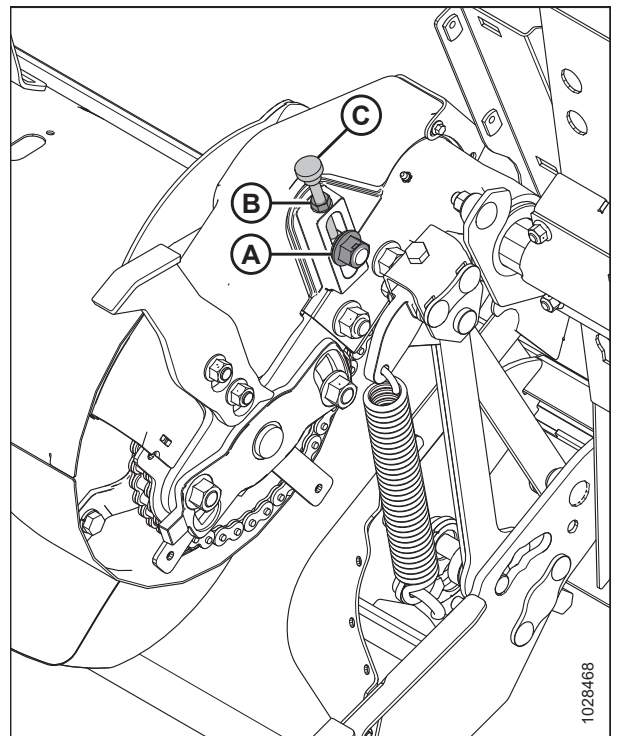
Figura 5.89: Lado izquierdo del mando del sinfín: vista delantera
