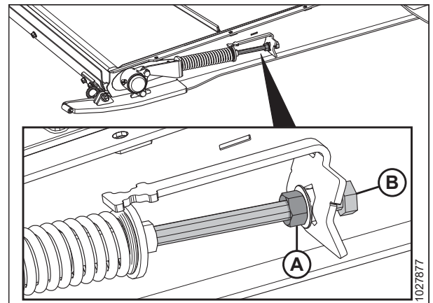
Figura 5.173: Tensor de la lona de alimentación
