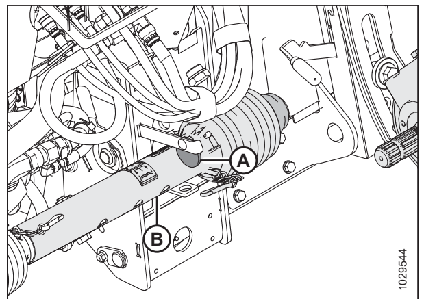
Figura 4.79: Mando en posición de almacenamiento
