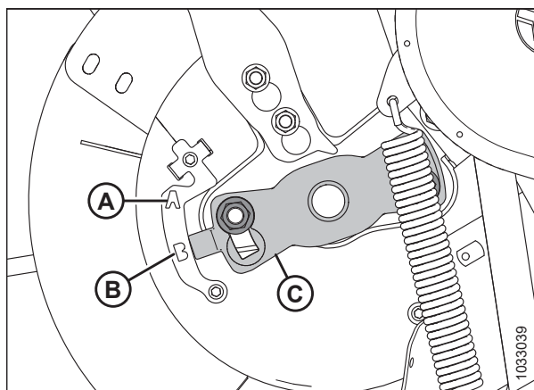
Figura 5.105: Sincronización de los dientes del sinfín: se muestra el lado izquierdo del sinfín
