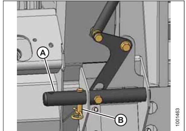
Figura 4.99: Clavijas de bloqueo
