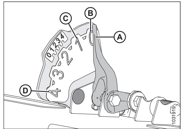
Figura 3.248: Indicador de flotación
