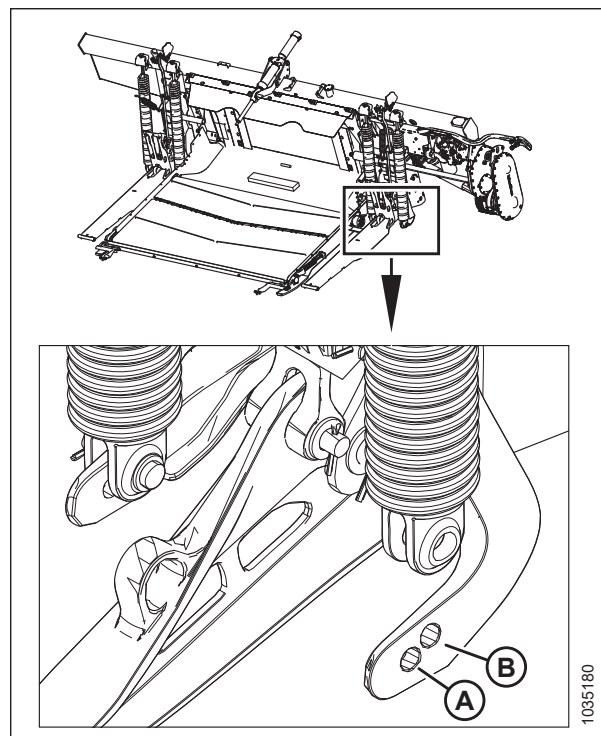
Figura 3.61: Resorte de flotación izquierdo instalado en el agujero de la palanca de flotación trasera
