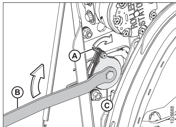
Figura 5.344: Mando del molinete
