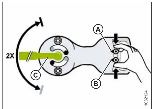
Figura 3.101: Ajuste del balance de alas (se muestra el lado izquierdo)
