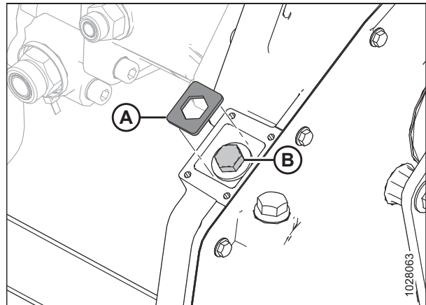
Figura 5.58: Tensor de la cadena de la caja de engranajes principal
