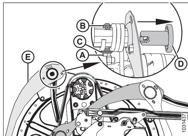
Figura 5.336: Tapas laterales del molinete: sección final interior
