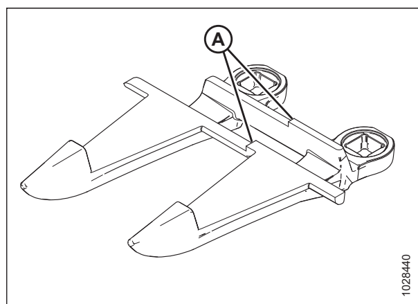
Figura 5.142: Puntón de cuchilla central puntiagudo
