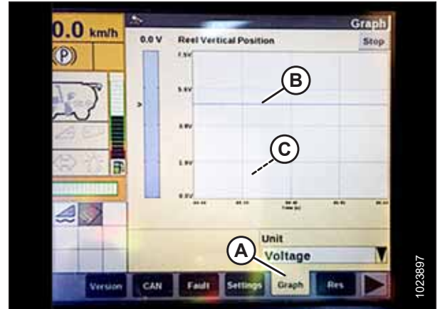
Figura 3.282: Pantalla de la cosechadora Case IH
