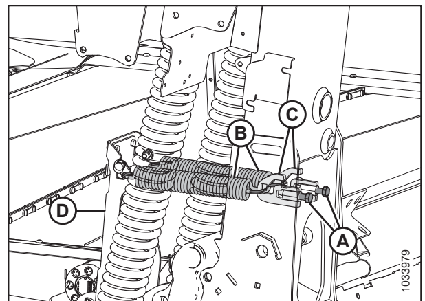
Figura 4.170: Resorte de recorte: lado izquierdo
