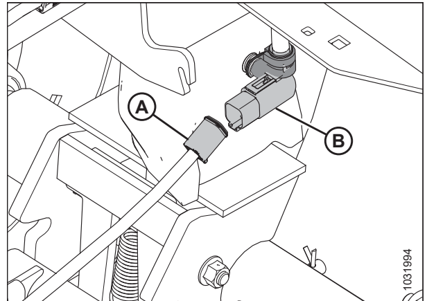
Figura 3.612: Conexión eléctrica de la barra de remolque
