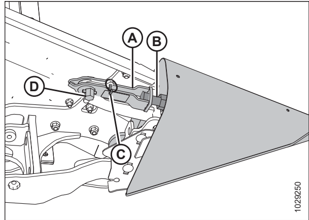
Figura 3.179: Divisor de cosecha con pestillo
