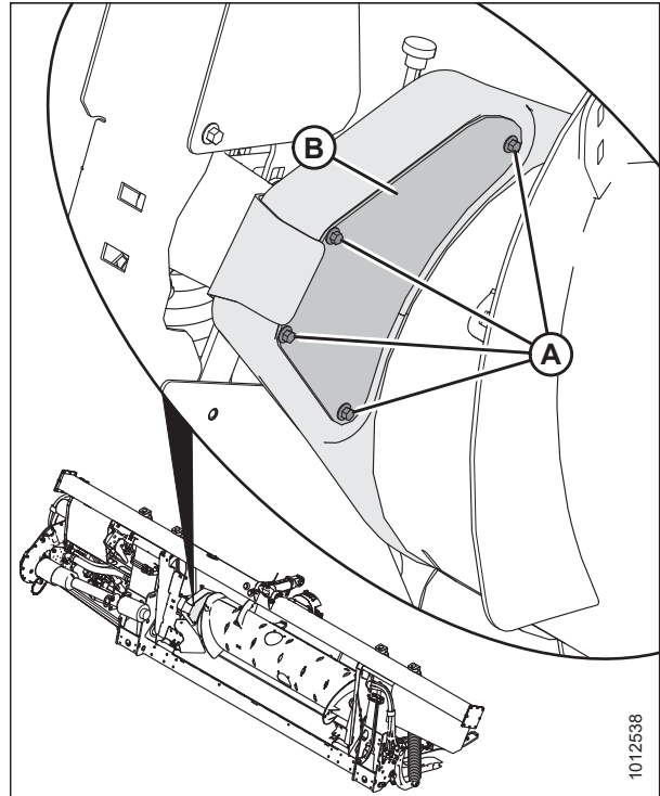
Figura 5.22: Panel de inspección del mando del sinfín
