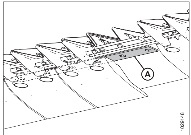
Figura 5.161: Barra de corte
