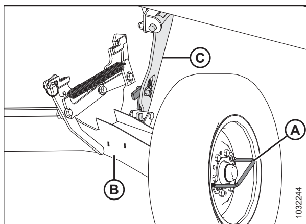
Figura 3.605: Soporte de suelo derecho
