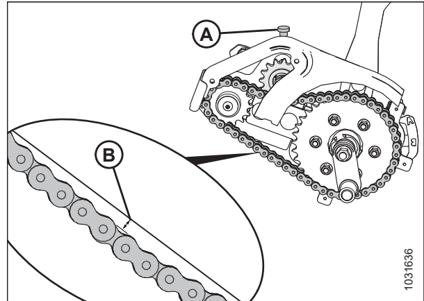
Figura 5.90: Deflexión de la cadena del sinfín de alimentación
