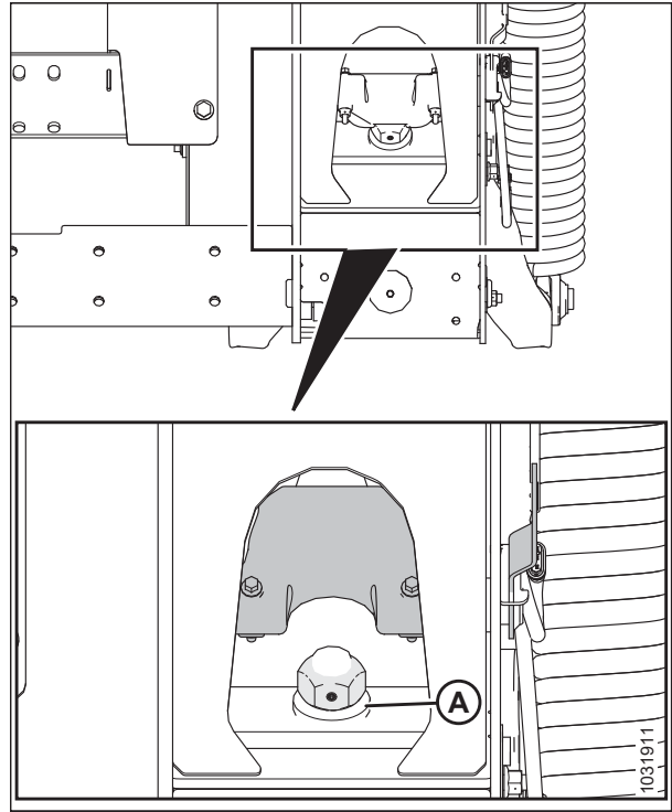
Figura 3.242: Traba de flotación
