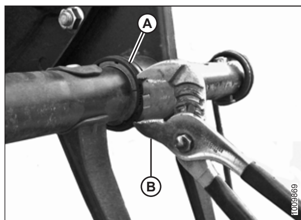
Figura 5.318: Instalación de la abrazadera
