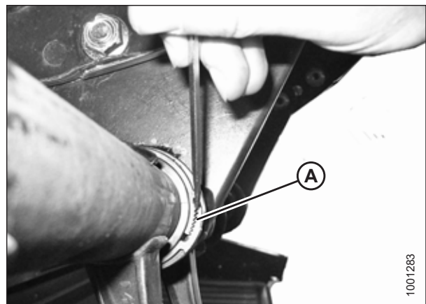
Figura 5.299: Abrazadera del buje
