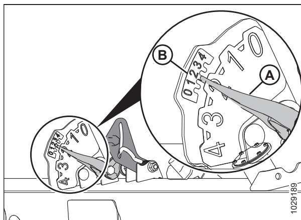
Figura 3.57: Indicador de configuración de flotación: izquierdo
