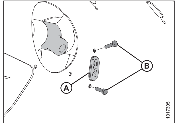
Figura 5.101: Orificio de dedos del sinfín
