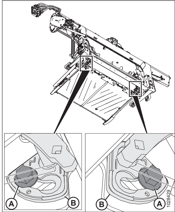
Figura 3.188: Ajuste de flotación del sinfín de alimentación
