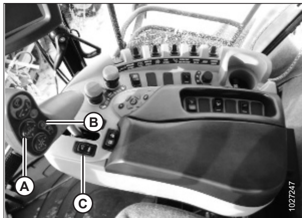
Figura 3.525: Controles de la cosechadora New Holland
