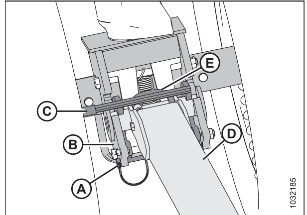
Figura 3.611: Extensión de la barra de remolque al pivote de transporte izquierdo
