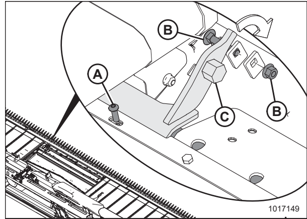
Figura 4.171: Pestillo del módulo de flotación
