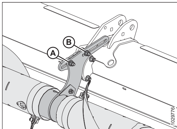
Figura 3.168: Posición inicial de los montajes ajustables: sinfín de dos piezas
