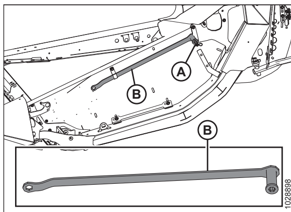
Figura 3.98: Parte final izquierda
