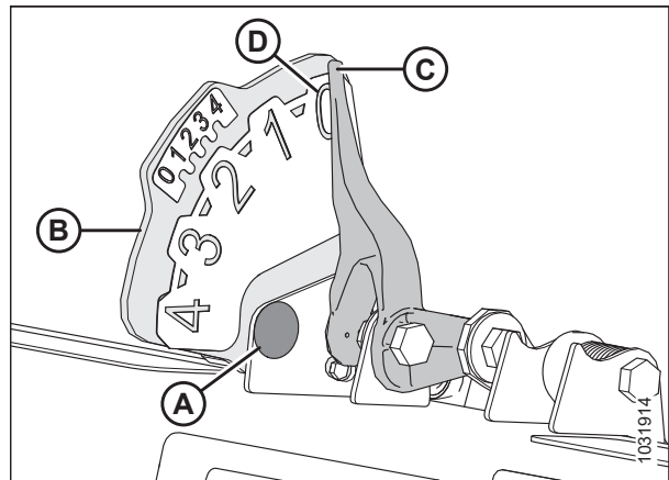
Figura 3.527: Indicador de flotación
