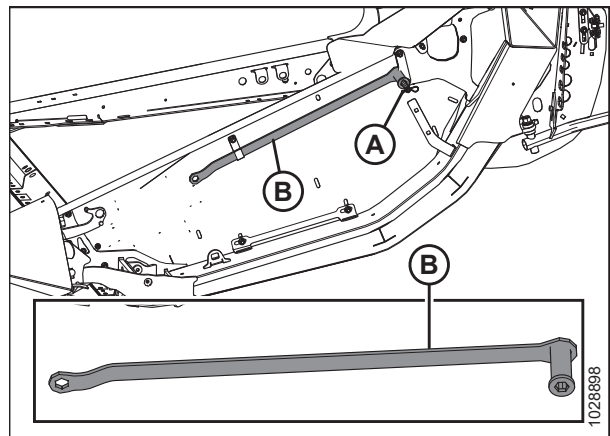
Figura 3.79: Parte final izquierda
