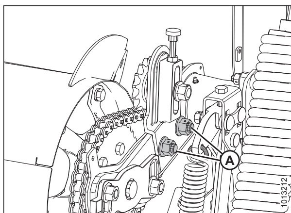
Figura 5.83: Mando del sinfín
