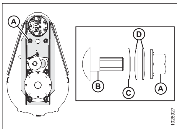
Figura 5.366: Montaje del motor de mando del molinete
