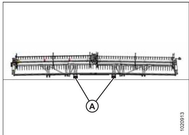
Figura 5.269: Ubicaciones de los bloques de FlexDraper®: molinete doble
