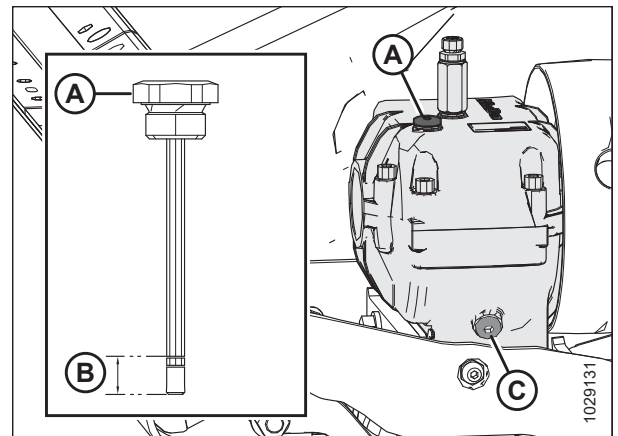
Figura 5.171: Caja de mando de la cuchilla
