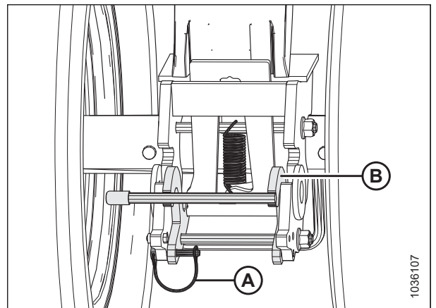
Figura 3.589: Ruedas de transporte izquierdas: pestillo de bloqueo de la rotación enganchado
