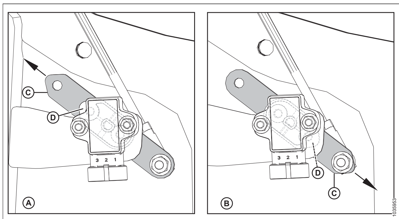
Figura 3.130: Ubicación del sensor de altura del molinete
