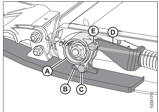
Figura 5.221: Rodamiento de rodillo tensor: lado izquierdo
