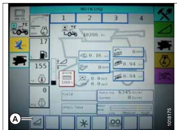
Figura 3.291: Pantalla de la cosechadora Challenger®
