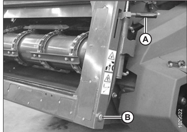
Figura 4.72: Embocador
