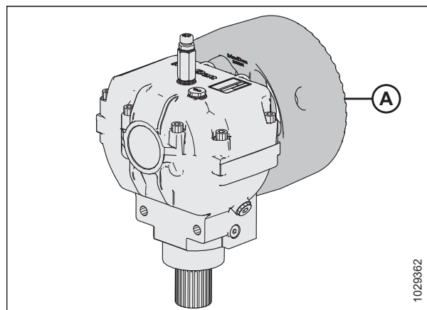
Figura 3.129: Volante
