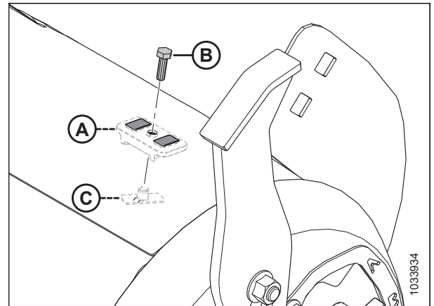
Figura 4.31: Instalación de tapones ranurados
