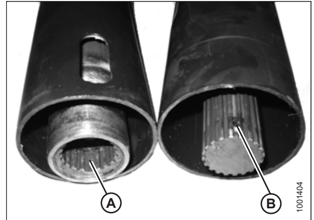
Figura 5.54: Mando
