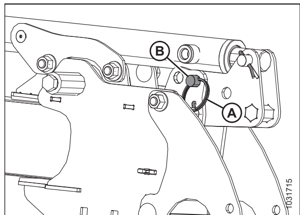
Figura 3.143: Cilindro del brazo derecho – Posición de avance
