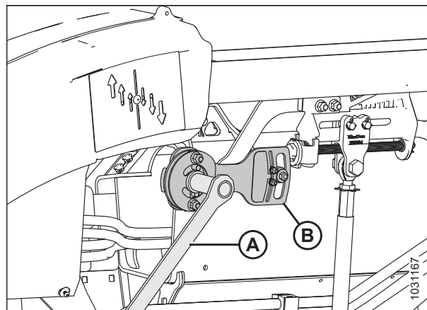
Figura 3.88: Ala en la posición de bloqueo
