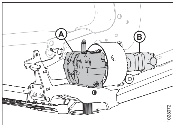
Figura 5.168: Se muestra el lado izquierdo de la caja de mando de cuchillas: lado derecho similar
