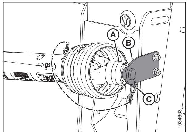
Figura 4.67: Almacenamiento del cardán
