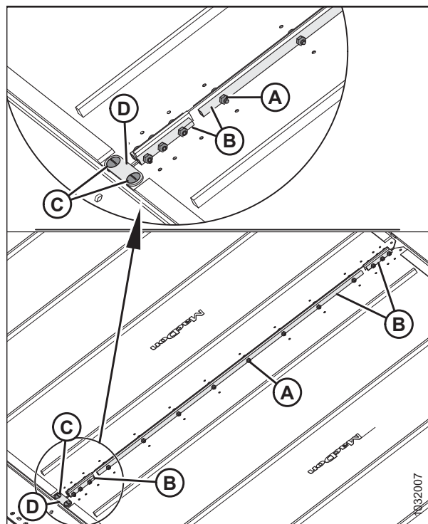
Figura 5.257: Conectores de la lona
