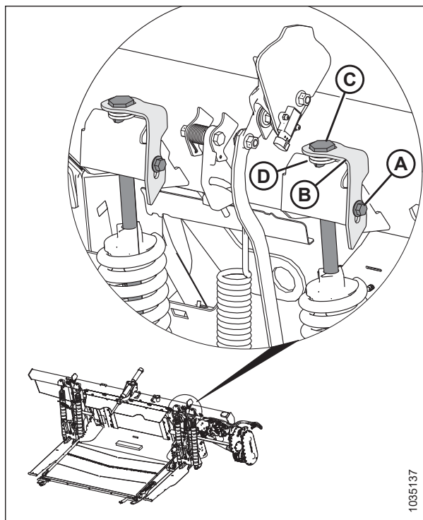
Figura 3.69: Pernos de ajuste de flotación: se muestra el izquierdo; el derecho es similar
