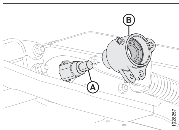
Figura 5.209: Plataforma de alimentación: lado izquierdo
