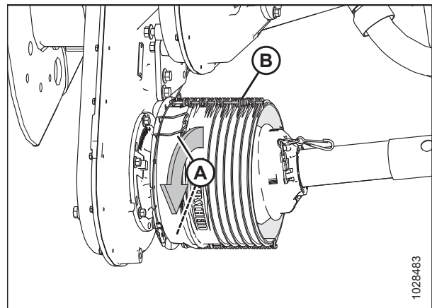
Figura 5.44: Escudo del cardán para cosechadora
