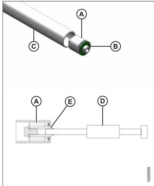
Figura 5.261: Rodamiento del rodillo
