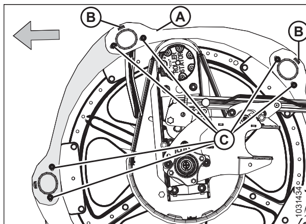
Figura 5.339: Tapas laterales del molinete: sección final interior
