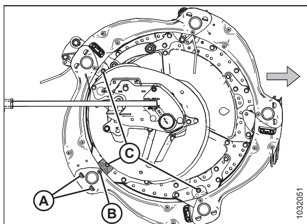
Figura 5.340: Soportes de la tapa lateral del molinete
