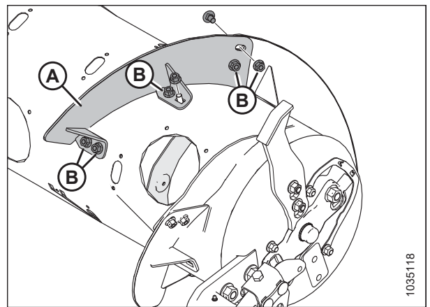
Figura 4.37: Ala corta: lado derecho
