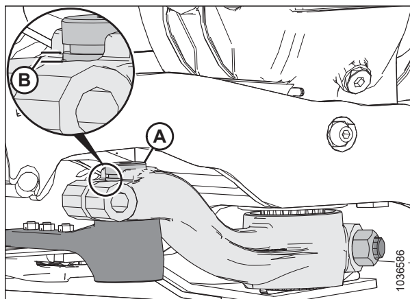
Figura 5.118: Cabeza de la cuchilla
