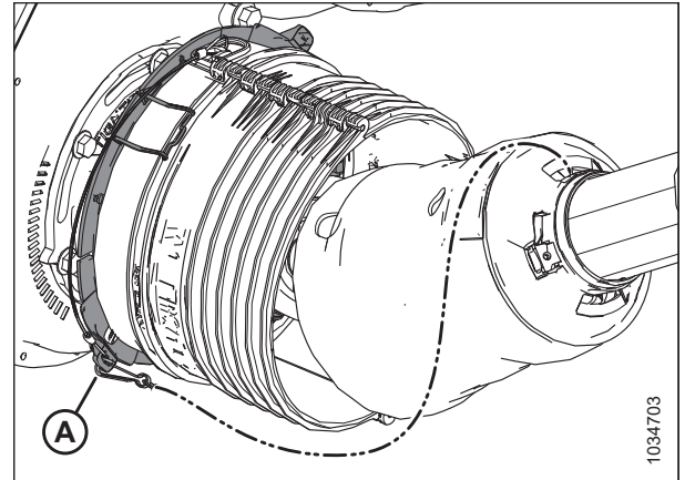
Figura 5.45: Escudo del cardán para cosechadora
