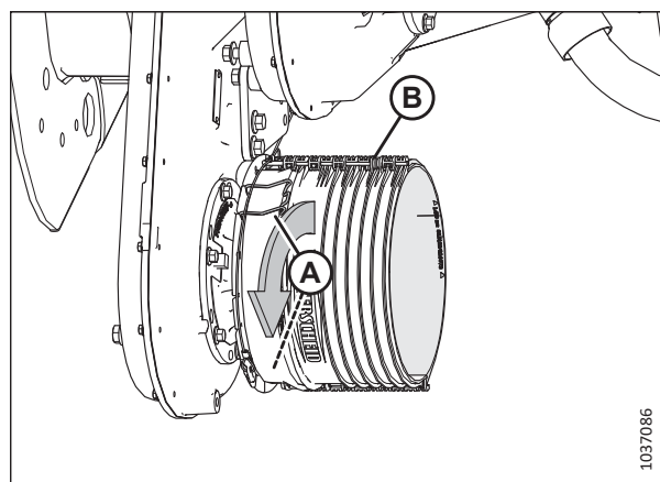
Figura 5.40: Escudo del cardán para cosechadora
