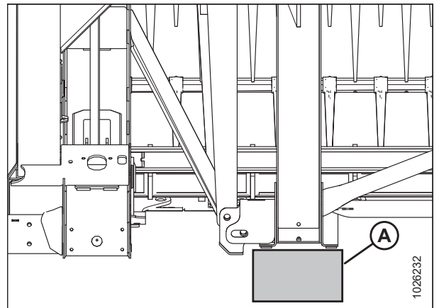
Figura 4.161: Pata de la plataforma en el bloque
