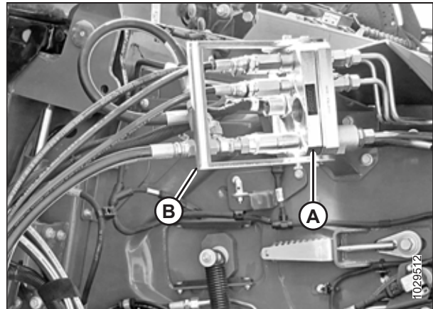
Figura 4.76: Receptáculo de la cosechadora
