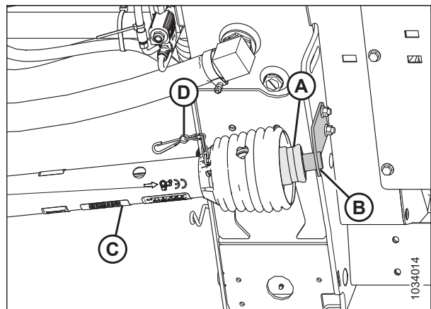
Figura 5.38: Escudo del cardán para cosechadora
