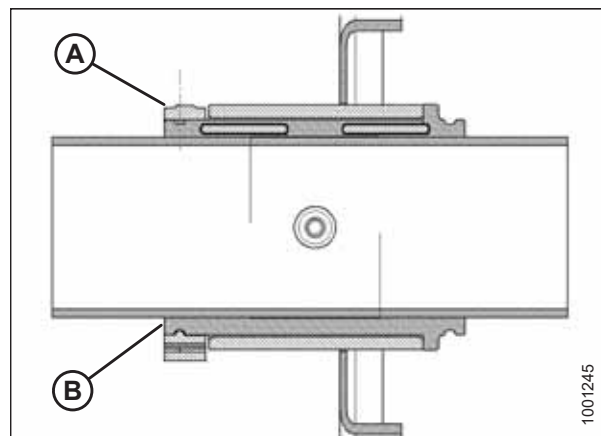
Figura 5.311: Buje
