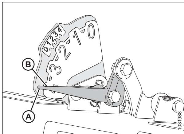
Figura 3.200: Indicador de flotación izquierdo: vista desde atrás
