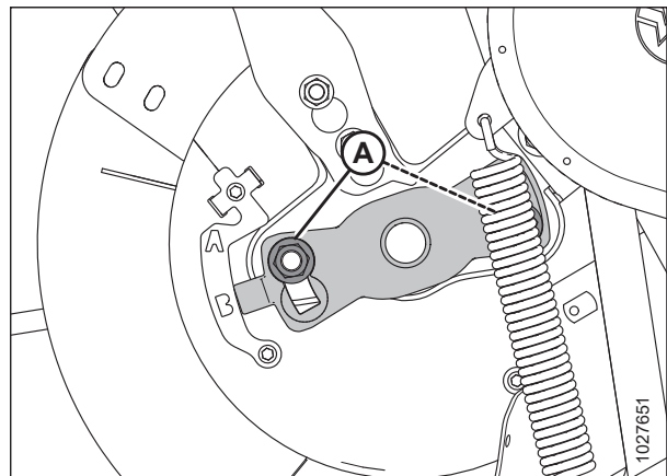
Figura 5.109: Indicador de sincronización de dientes del sinfín
