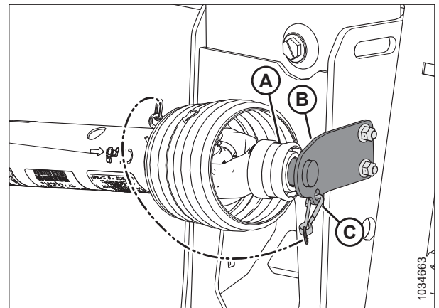
Figura 4.74: Cardán en posición de almacenamiento: Cardán MD n.º B7038 o MD n.º B7039
