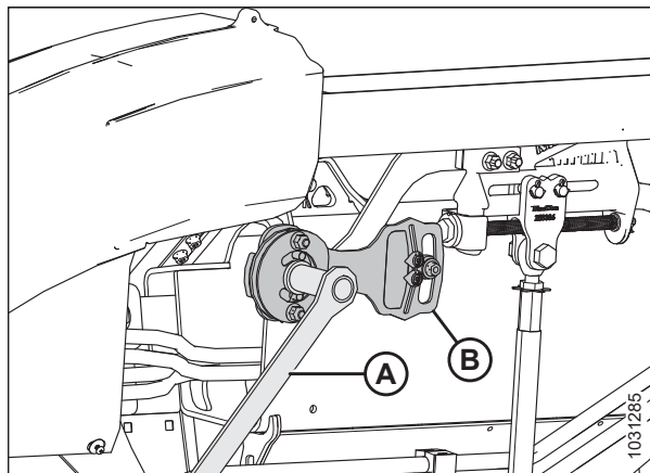
Figura 3.83: Bloqueo de ala en posición desbloqueada
