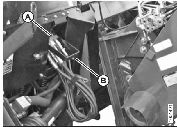
Figura 4.130: Almacenamiento del acoplamiento múltiple
