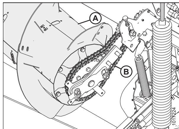
Figura 5.80: Mando del sinfín
