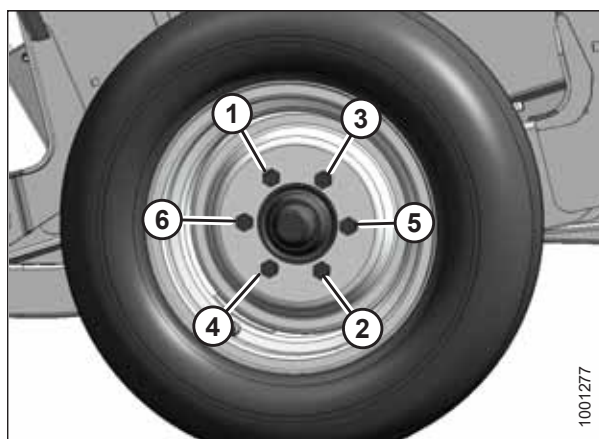
Figura 5.378: Secuencia de ajuste de tornillos
