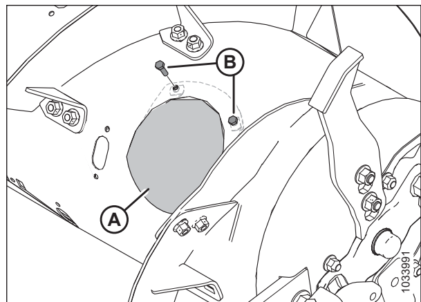
Figura 4.40: Cubierta de acceso: lado derecho
