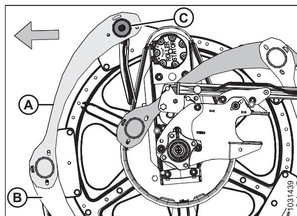
Figura 5.337: Tapas laterales del molinete: sección final interior
