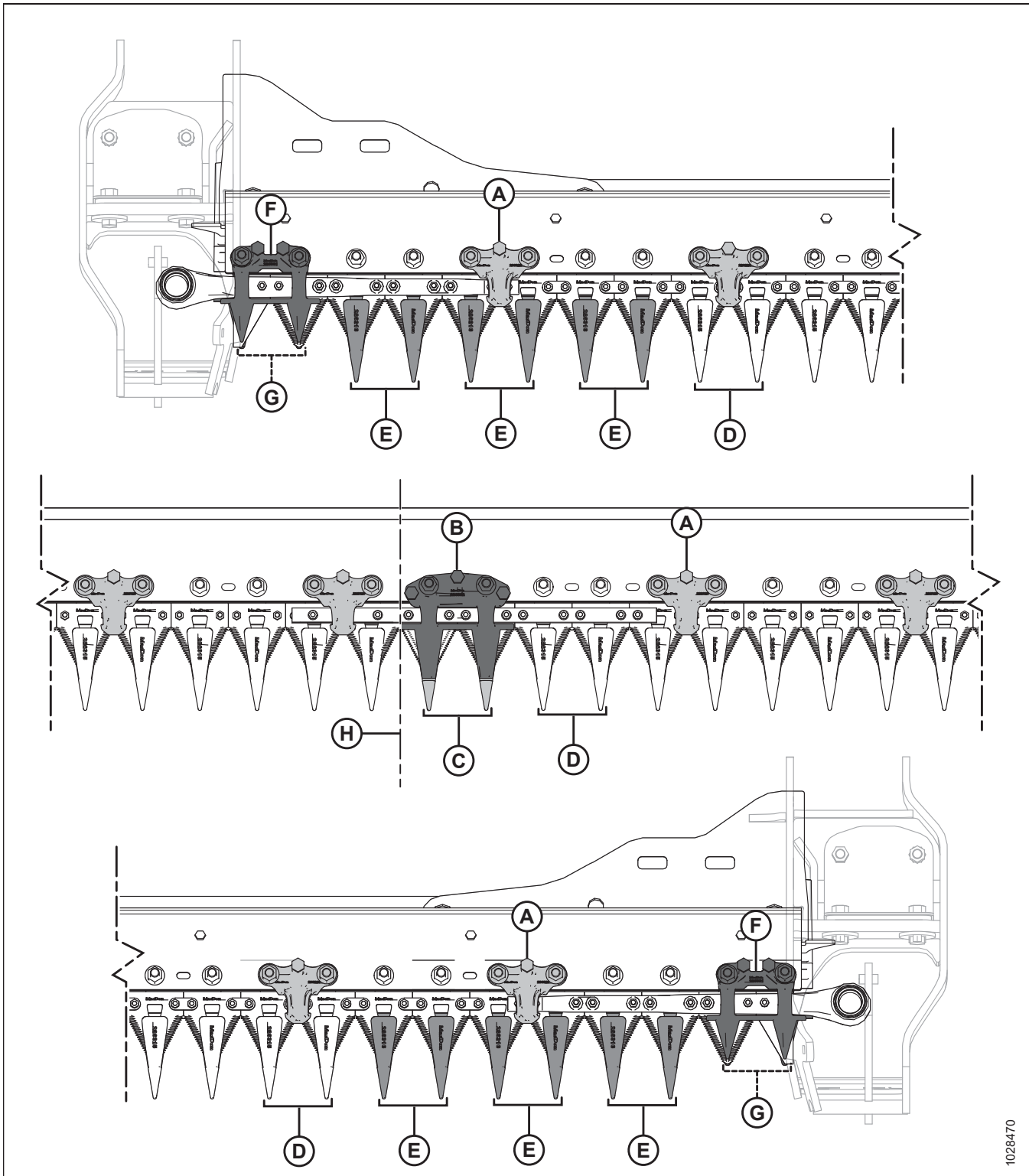
Figura 5.127: Puntón de cuchilla puntiagudo y ubicaciones del sujetador: plataforma de cuchilla doble FD241
