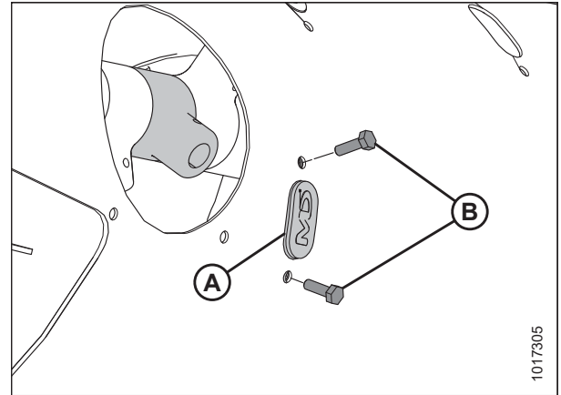
Figura 4.51: Tapón
