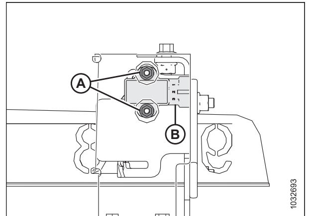
Figura 3.159: Sensor de avance y retroceso
