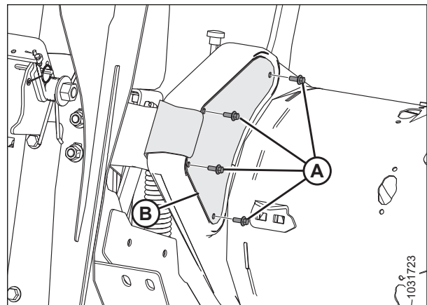
Figura 5.92: Lado izquierdo del mando del sinfín: vista trasera
