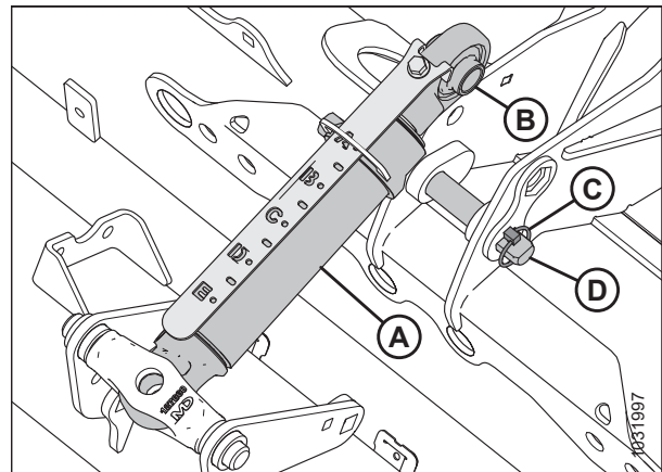
Figura 4.167: Unión central
