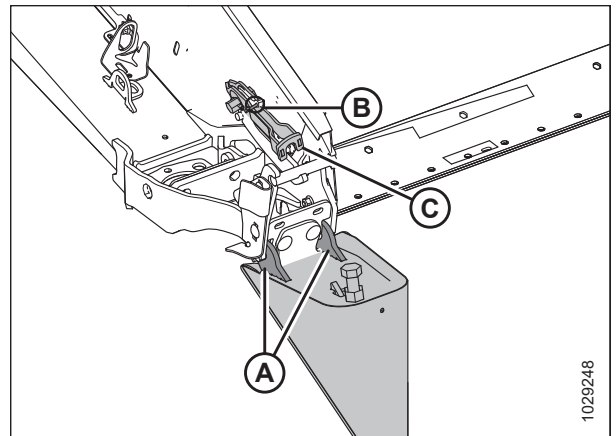
Figura 3.177: Divisor de cosecha con pestillo
