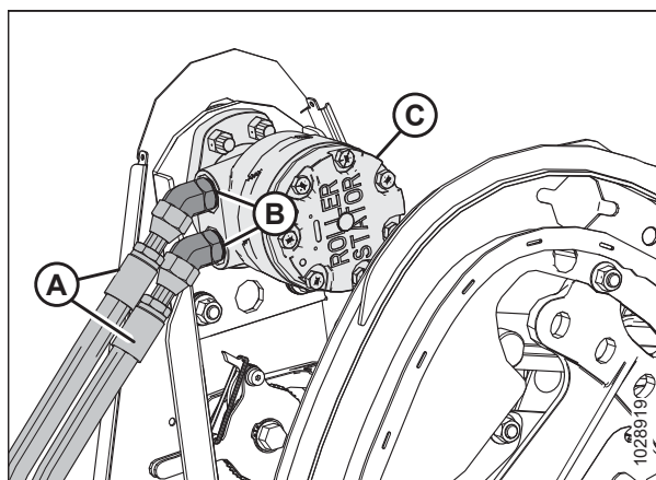
Figura 5.367: Motor de mando y mangueras
