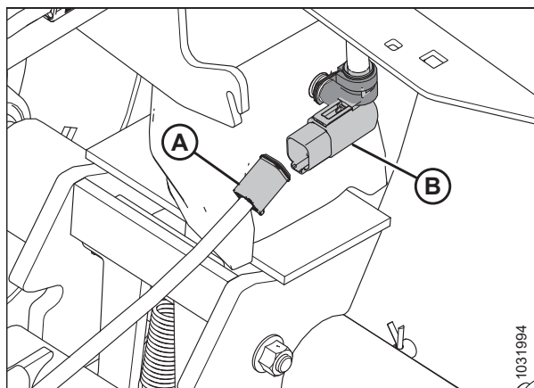
Figura 3.580: Conexión eléctrica de la barra de remolque
