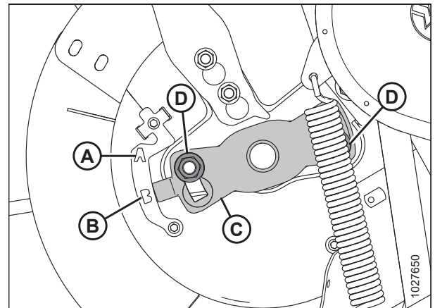
Figura 5.106: Indicador de sincronización de dientes del sinfín
