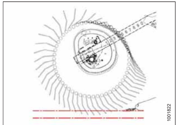
Figura 3.163: Perfil del diente: posición 4
