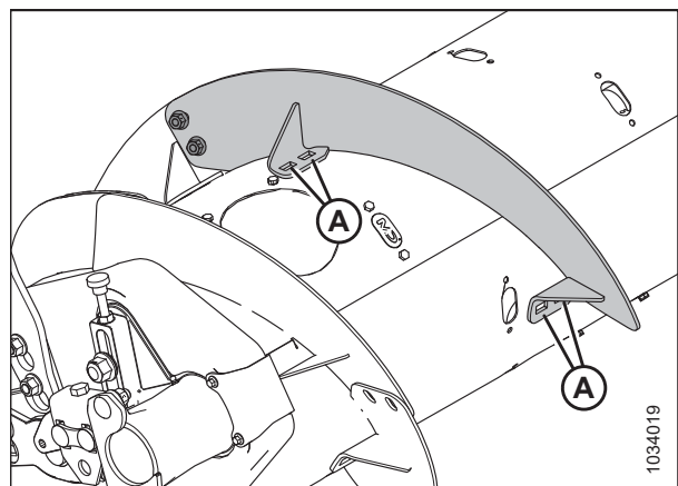
Figura 4.46: Alas en el lado izquierdo del sinfín
