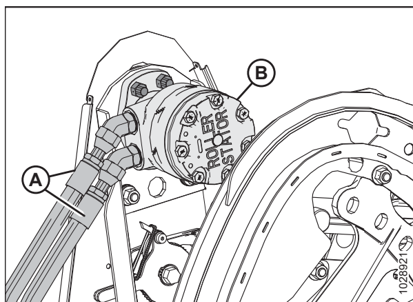
Figura 5.360: Motor de mando y mangueras
