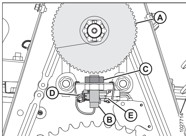
Figura 5.376: Sensor de velocidad
