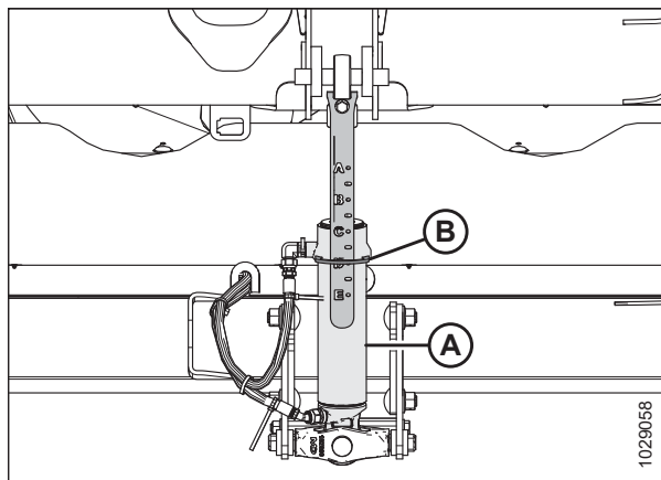
Figura 3.52: Unión central
