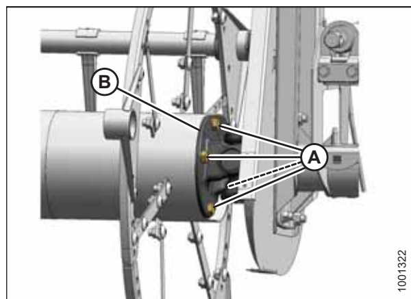
Figura 5.358: Cruceta
