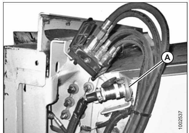
Figura 4.148: Acopladores de la cosechadora
