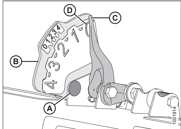
Figura 3.243: Indicador de flotación
