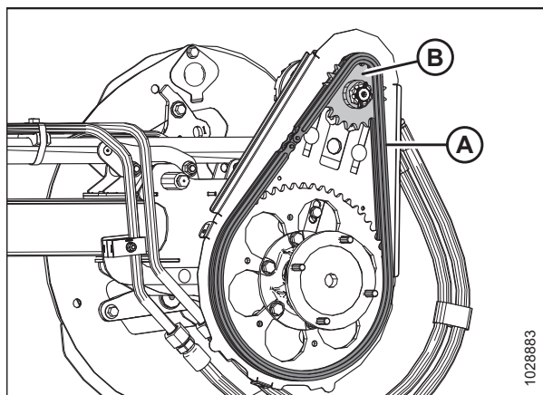
Figura 5.352: Piñón único
