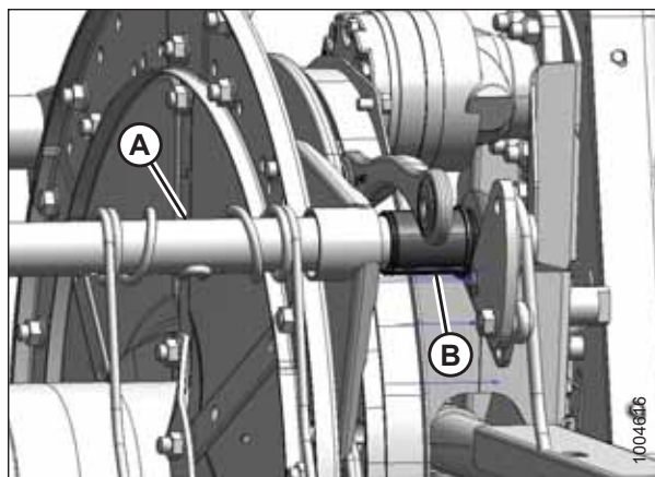
Figura 5.304: Extremo de leva
