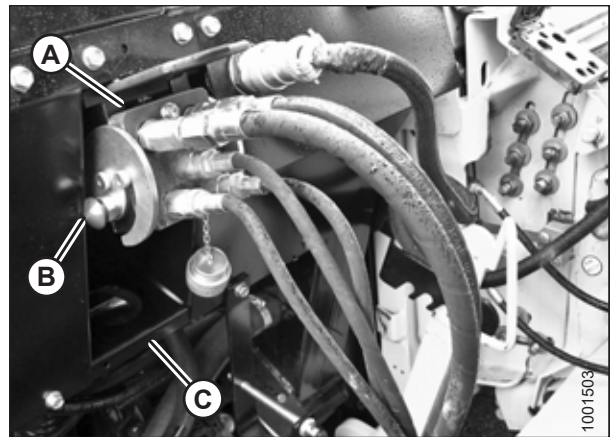
Figura 4.144: Conexiones del módulo de flotación
