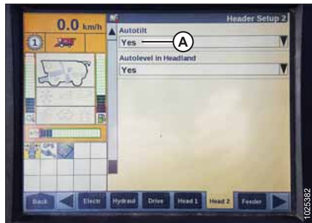
Figura 3.276: Pantalla de la cosechadora Case IH
