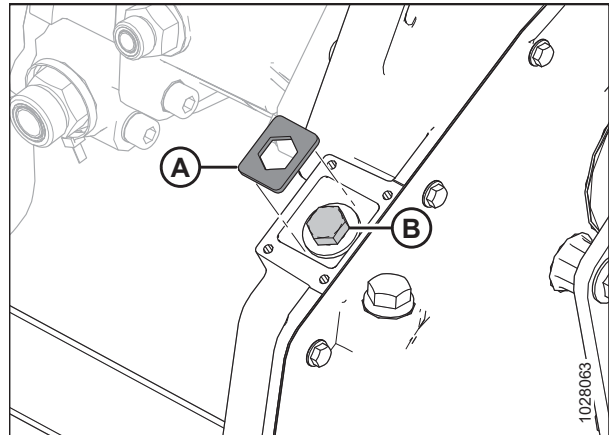
Figura 5.57: Tensor de la cadena de la caja de engranajes principal
