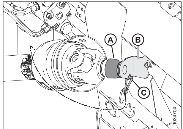
Figura 4.138: Cardán en posición de almacenamiento: cardán Sidehill/Hillside MD n.º B7180, MD n.º B7181, o MD n.º B7182
