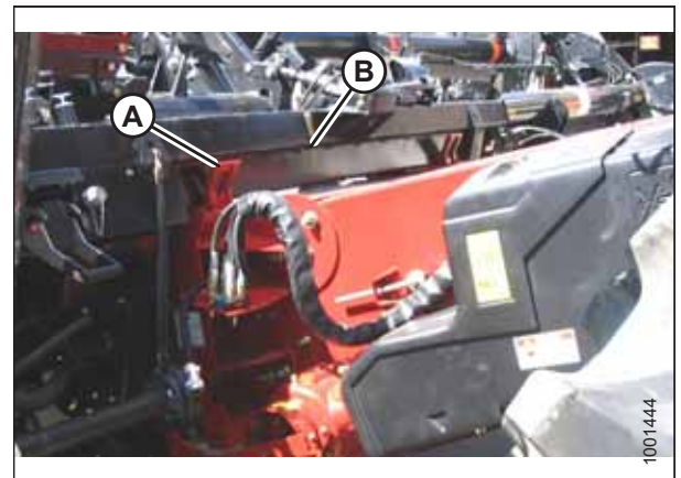
Figura 4.83: Cosechadora y módulo de flotación
