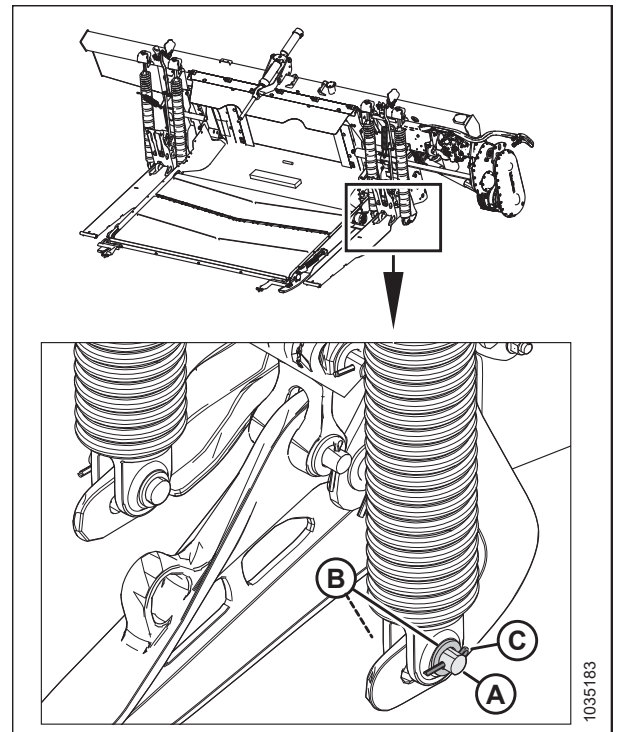
Figura 3.64: Resorte de flotación izquierdo instalado en el agujero de la palanca de flotación trasera
