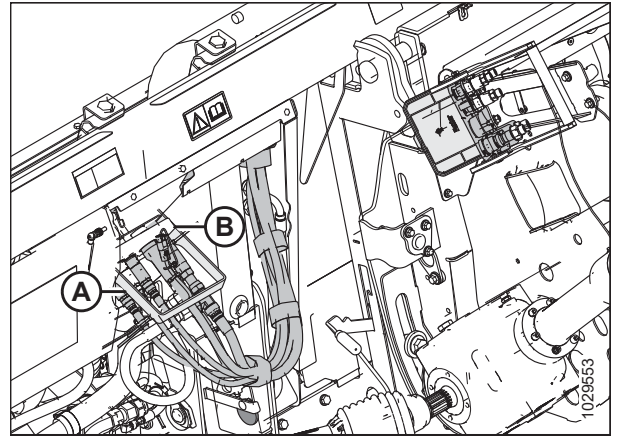
Figura 4.77: Bloqueo del multiacoplador
