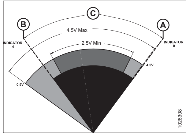
Figura 3.193: AHHC: rango del sensor demasiado cerca del límite de tensión alto
