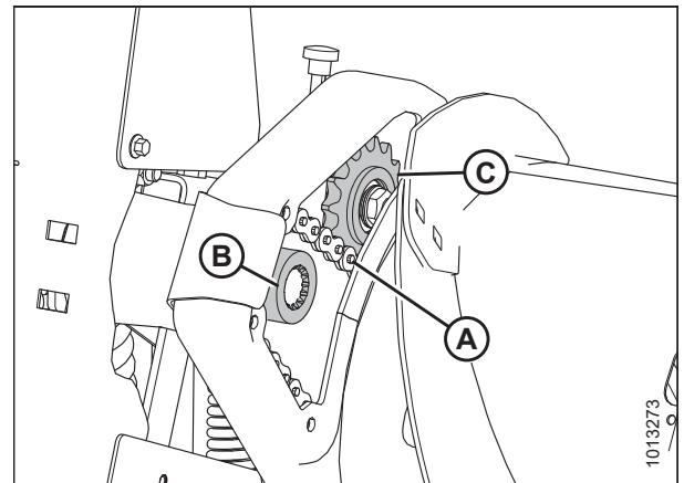
Figura 5.21: Cadena de mando del sinfín
