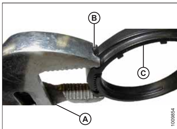
Figura 5.303: Pinza pico de loro modificada
