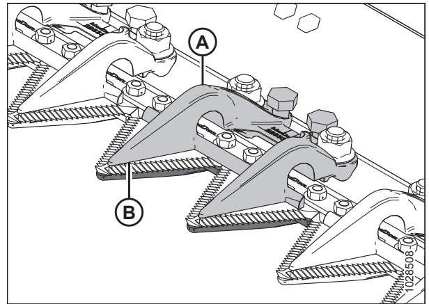
Figura 5.157: Puntones de cuchilla cortos
