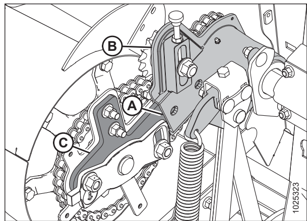
Figura 5.77: Sinfín
