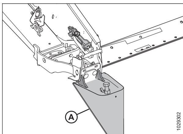
Figura 3.174: Divisor de cosecha con pestillo
