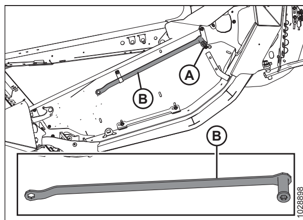
Figura 3.54: Ubicación de la herramienta múltiple
