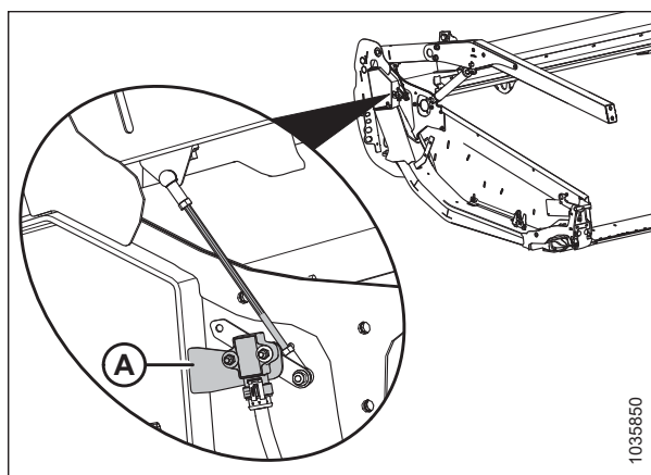
Figura 3.130: Ubicación del sensor de altura del molinete
