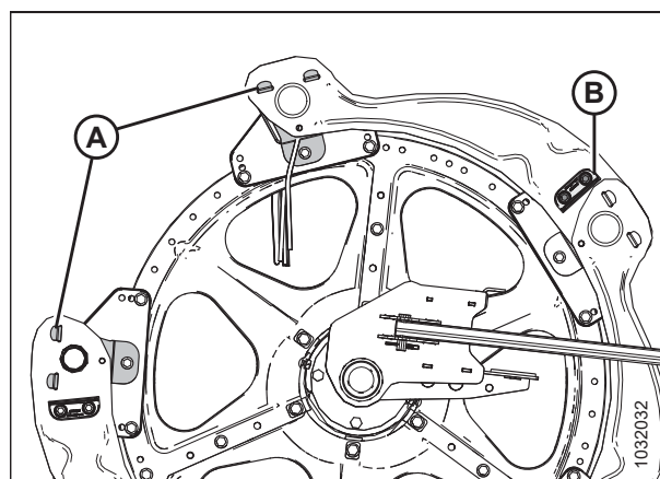
Figura 5.332: Tapa lateral del molinete extraída: sección final exterior
