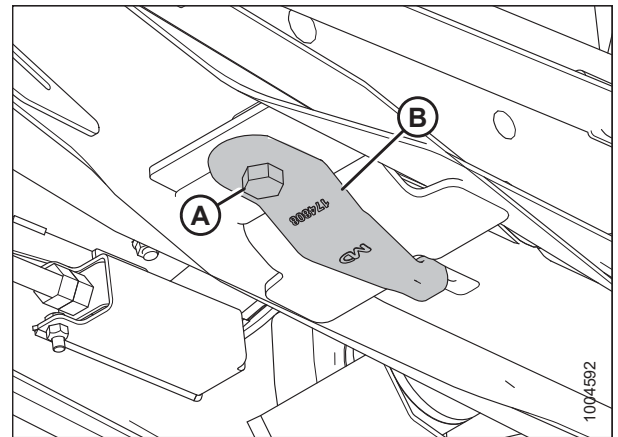
Figura 4.169: Parte inferior del módulo de flotación
