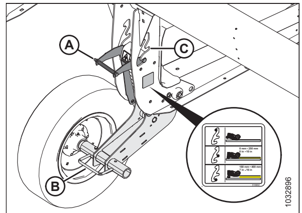
Figura 3.34: Rueda estabilizadora
