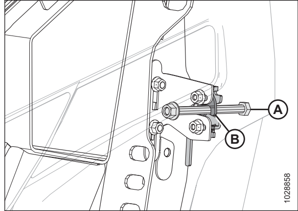
Figura 3.19: Pestillo de dos etapas
