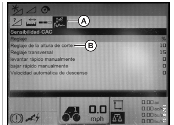
Figura 3.332: Pantalla de la cosechadora CLAAS
