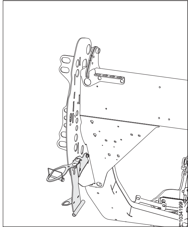
Figura 6.3: Kit de soporte de almacenamiento de abresurcos: MD n.º B7030
