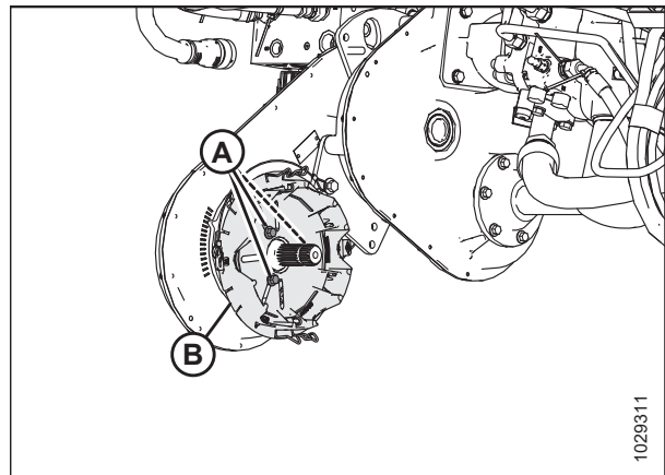
Figura 5.62: Cubierta del tensor de la cadena de la caja de engranajes de completión
