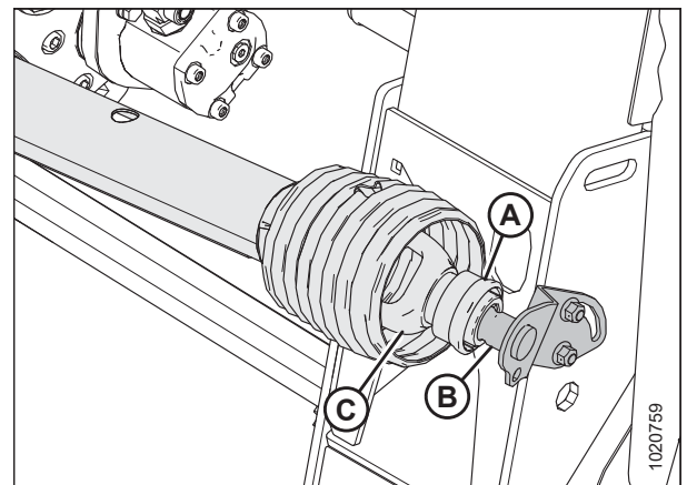
Figura 5.46: Extremo del mando de la cosechadora
