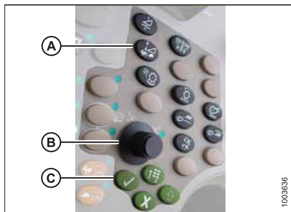
Figura 3.429: Consola de control de la cosechadora John Deere
