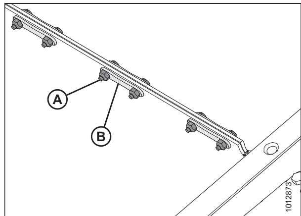
Figura 5.176: Conector de la lona
