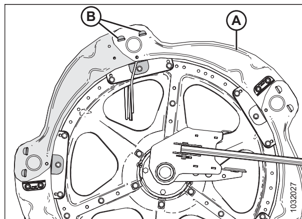
Figura 5.331: Tapas laterales del molinete: sección final exterior
