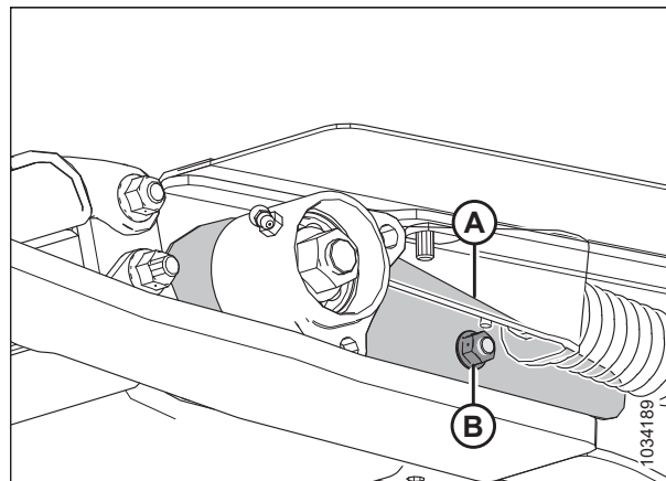
Figura 5.208: Cubierta tensora: lado izquierdo
