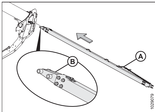
Figura 3.585: Final del enganche
