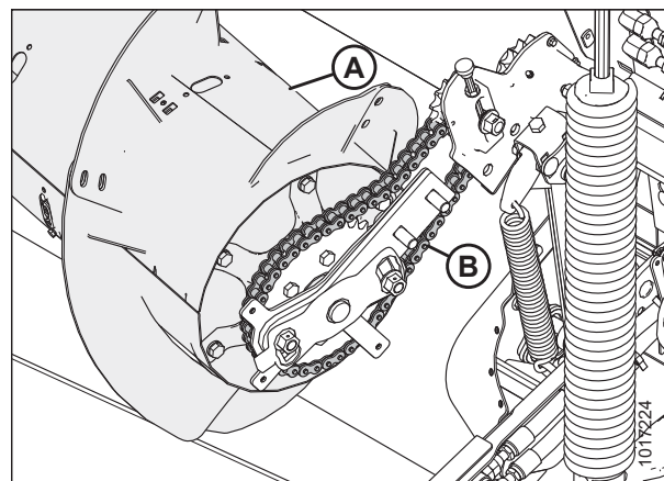
Figura 5.79: Mando del sinfín
