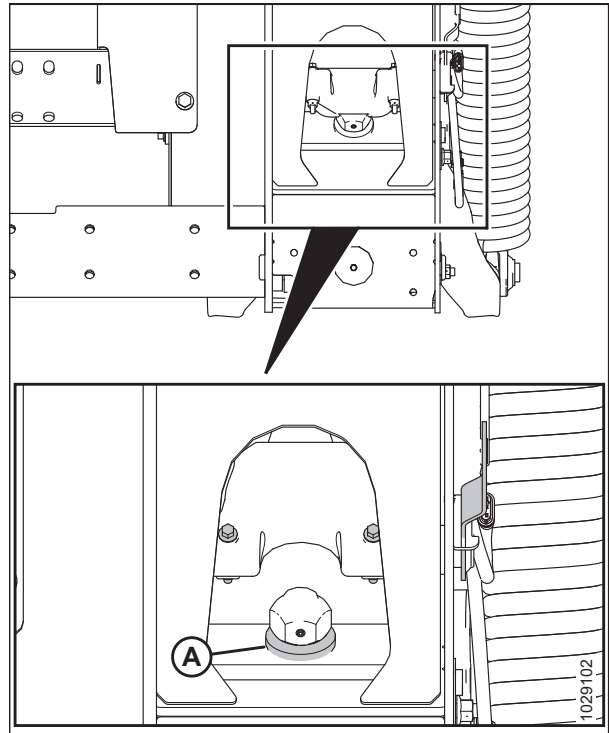
Figura 3.197: Arandela del amortiguador de parada
