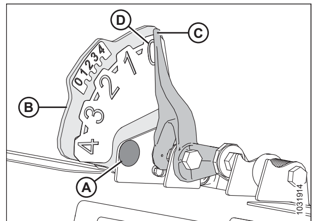
Figura 3.417: Indicador de flotación
