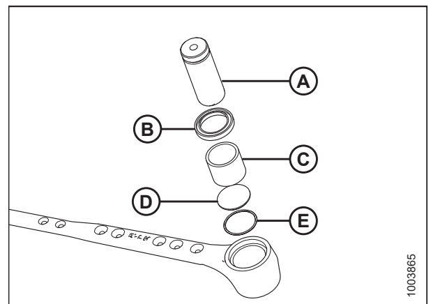
Figura 5.116: Ensamblaje del rodamiento de la cabeza de la cuchilla
