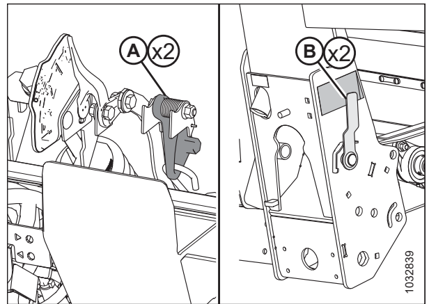
Figura 3.100: Ensamblaje de la placa de verificación
