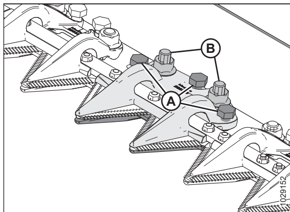
Figura 5.166: Sujetador central
