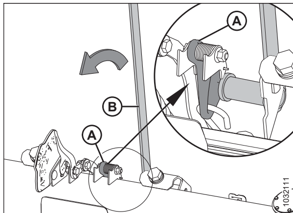
Figura 3.55: Ensamblaje de ajuste de flotación: izquierdo
