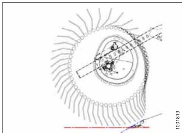
Figura 3.160: Perfil del diente: posición 1
