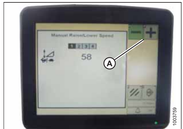
Figura 3.440: Pantalla de la cosechadora John Deere
