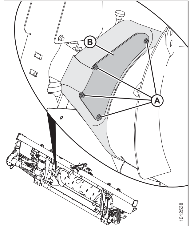
Figura 5.20: Panel de inspección del mando del sinfín
