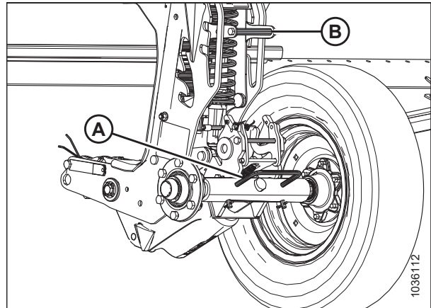
Figura 3.591: Ruedas de transporte izquierdas en la posición de almacenamiento más alta
