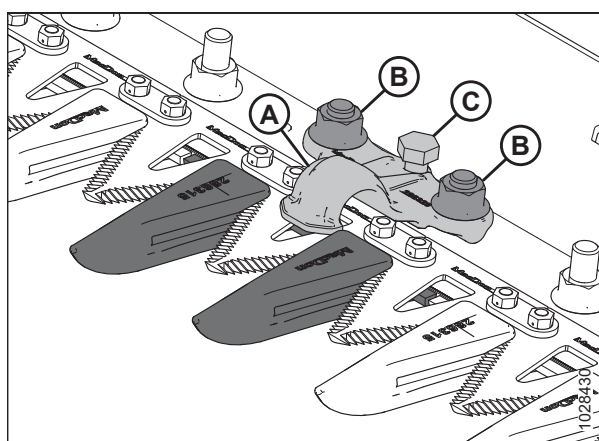
Figura 5.138: Puntones de cuchilla puntiagudos
