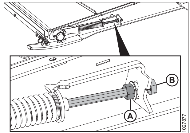
Figura 5.193: Tensor de la lona de alimentación
