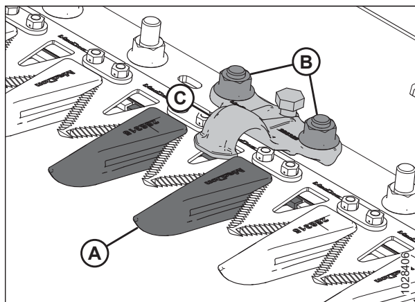
Figura 5.136: Puntones de cuchilla puntiagudos
