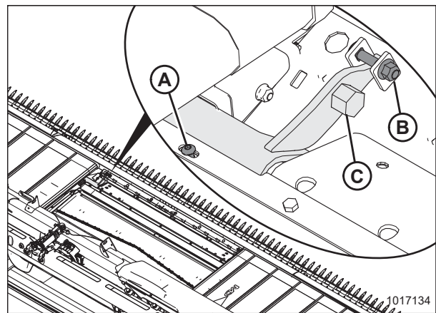
Figura 4.172: Pestillo del módulo de flotación
