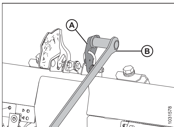
Figura 3.56: Ensamblaje de ajuste de flotación: izquierdo
