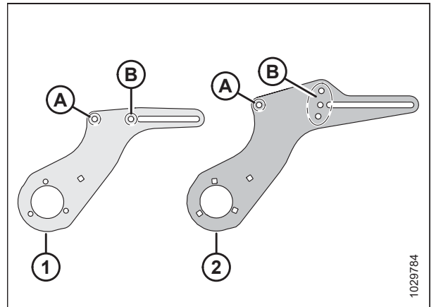
Figura 3.170: Detalles de montaje ajustables
