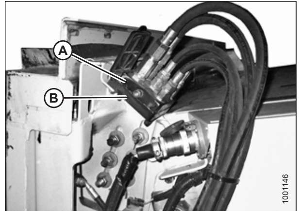
Figura 4.146: Acoplador de la cosechadora
