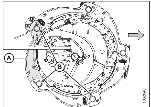
Figura 5.322: Tapas laterales del molinete: extremo de leva exterior
