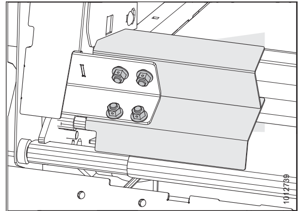
Figura 6.11: Kit del esquinero de alimentación
