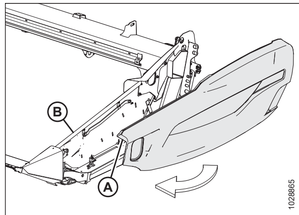
Figura 3.12: Tapa lateral de la plataforma izquierda
