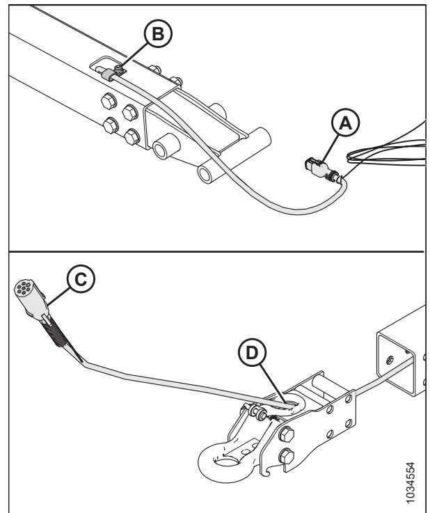
Figura 5.382: Extracción del adaptador de remolque de pivote
