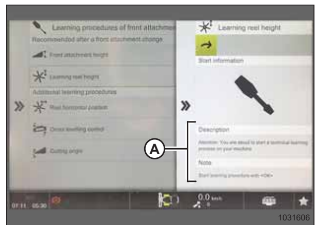
Figura 3.366: Página de aprendizaje de altura del molinete
