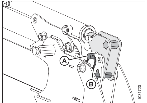
Figura 3.145: Cilindro del brazo derecho: Posición de retroceso
