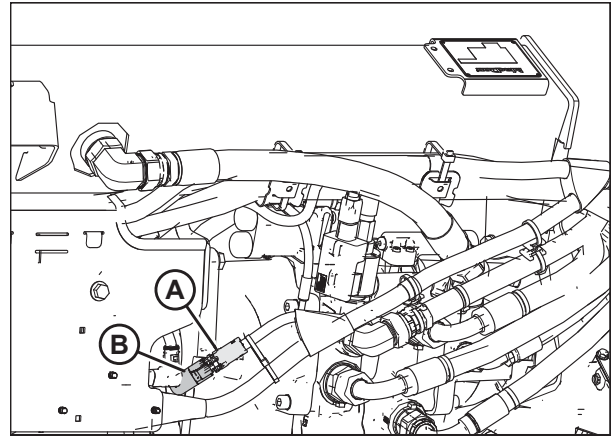
Figura 3.198: Indicador de flotación izquierdo: vista desde atrás
