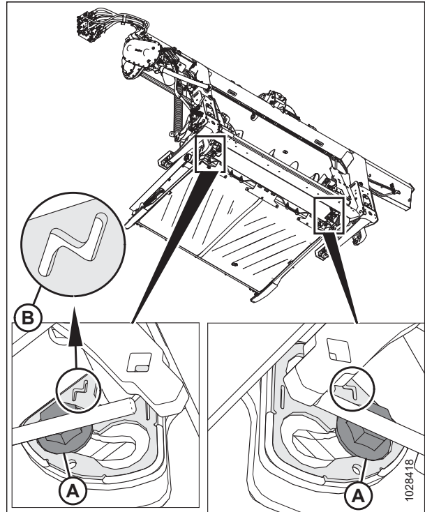
Figura 5.64: Posición de flotación
