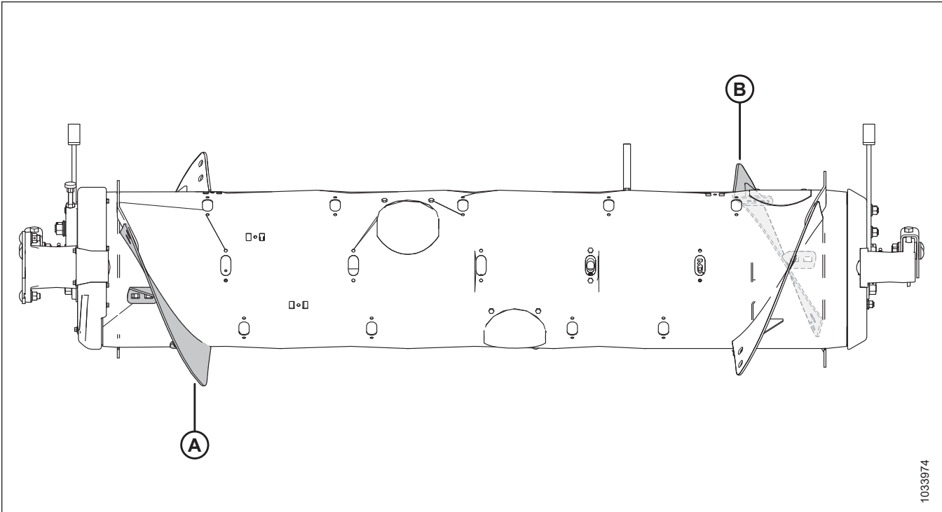
Figura 4.16: Configuración ancha
