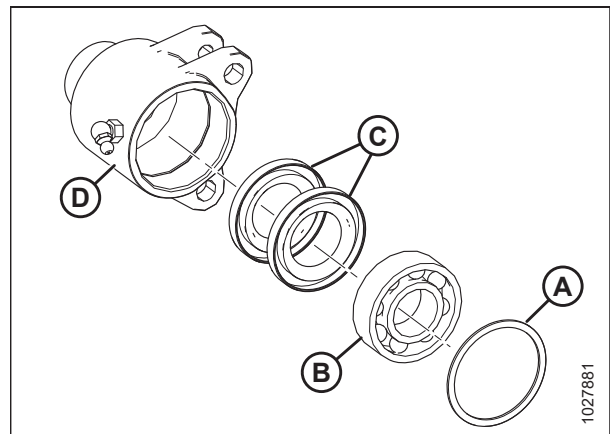
Figura 5.218: Montaje del rodamiento
