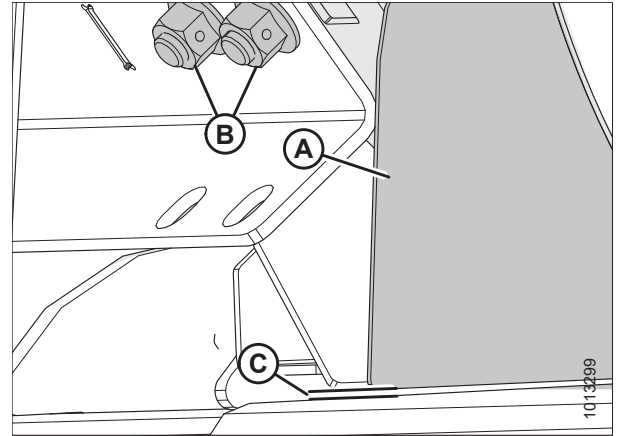
Figura 5.235: Distancia de la batea y el deflector
