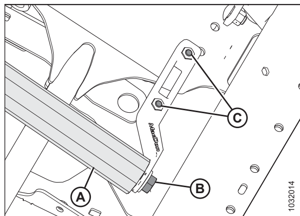
Figura 5.263: Rodillo de mando
