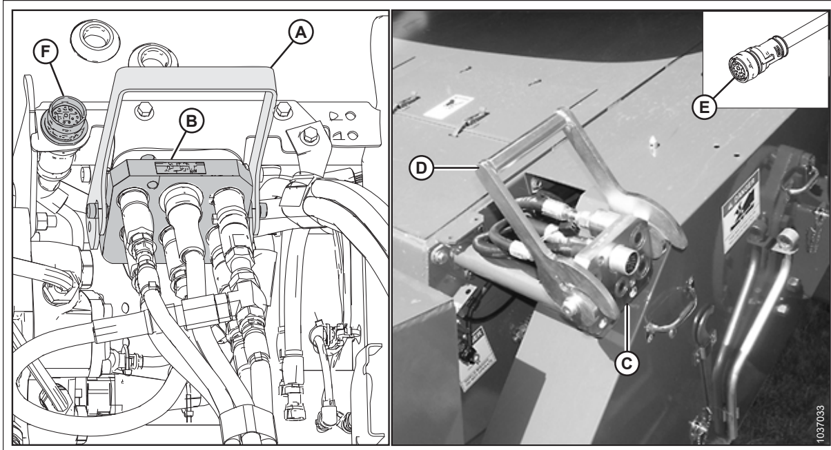
Figura 4.62: Hidráulica y acoplamiento múltiple eléctrico
