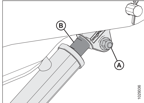
Figura 5.277: Cilindro del brazo exterior
