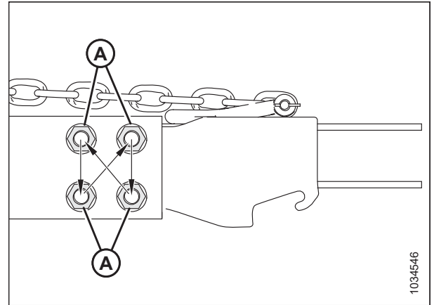
Figura 5.385: Secuencia de par de torsión
