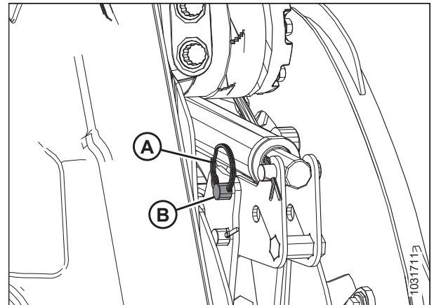
Figura 3.150: Cilindro del brazo central izquierdo: Posición de avance
