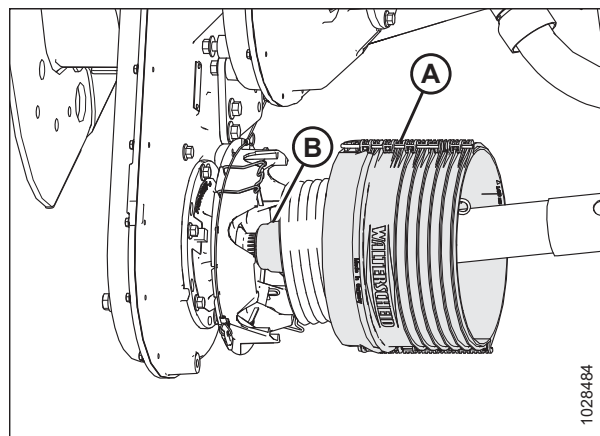
Figura 5.41: Escudo del cardán para cosechadora
