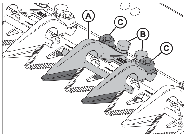
Figura 5.156: Puntón de cuchilla corto
