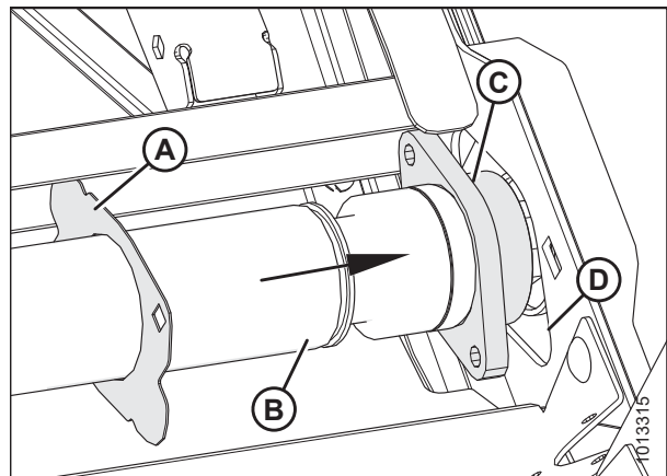
Figura 5.190: Rodillo de mando: extremo del rodamiento
