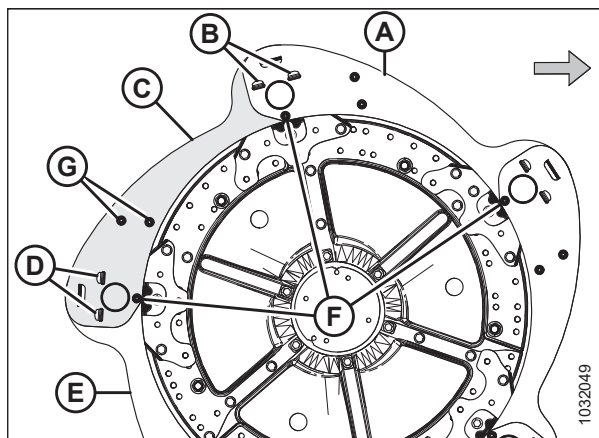
Figura 5.329: Tapas laterales del molinete: extremo de leva interior
