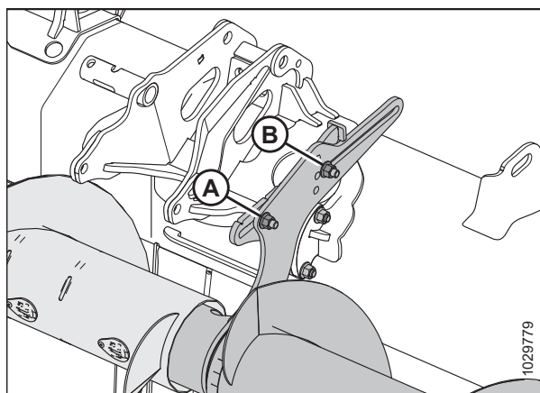
Figura 3.171: Posición inicial de los montajes ajustables: sinfín de tres piezas
