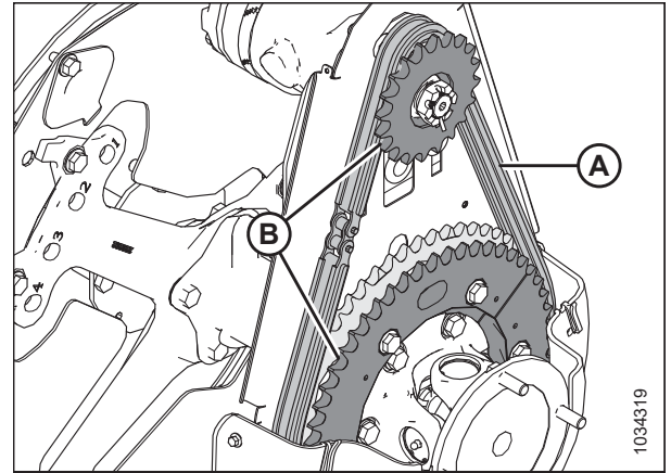
Figura 5.353: Piñón del mando del molinete
