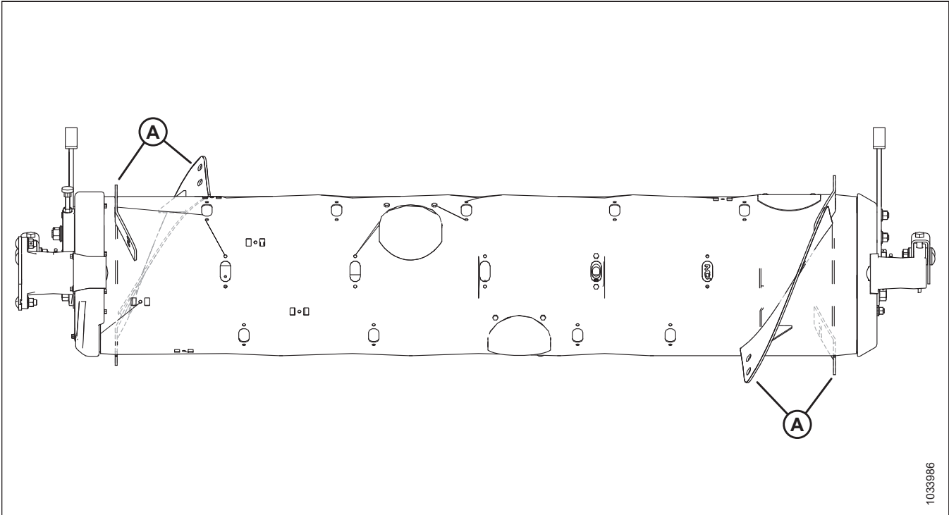
Figura 4.26: Configuración ultraancha
