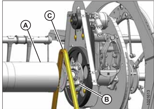
Figura 5.370: Reemplazo de la cadena
