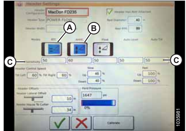
Figura 3.219: Controles automáticos y configuraciones de sensibilidad
