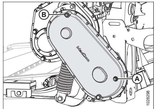
Figura 5.27: Caja de engranajes de compleción del mando de la plataforma
