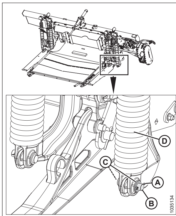
Figura 3.70: Se muestra el resorte de flotación izquierdo externo
