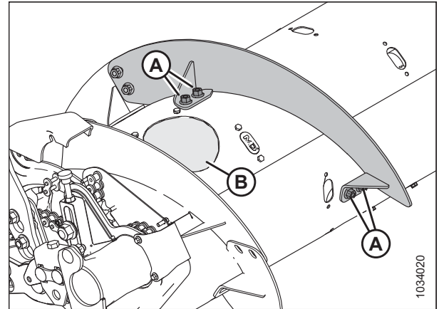
Figura 4.47: Lado izquierdo del sinfín
