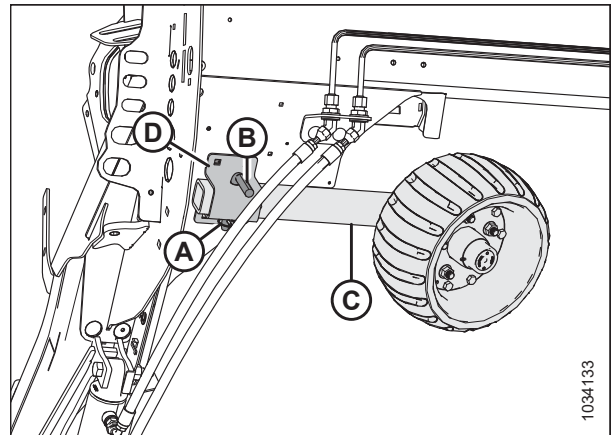
Figura 3.571: Ensamble de la rueda izquierda
