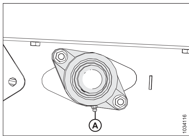
Figura 5.3: Rodillo de mando de la lona de alimentación
