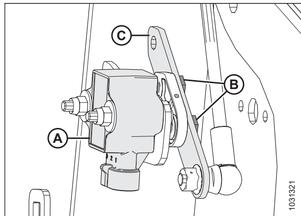
Figura 3.134: Sensor de altura del molinete-Brazo del molinete derecho
