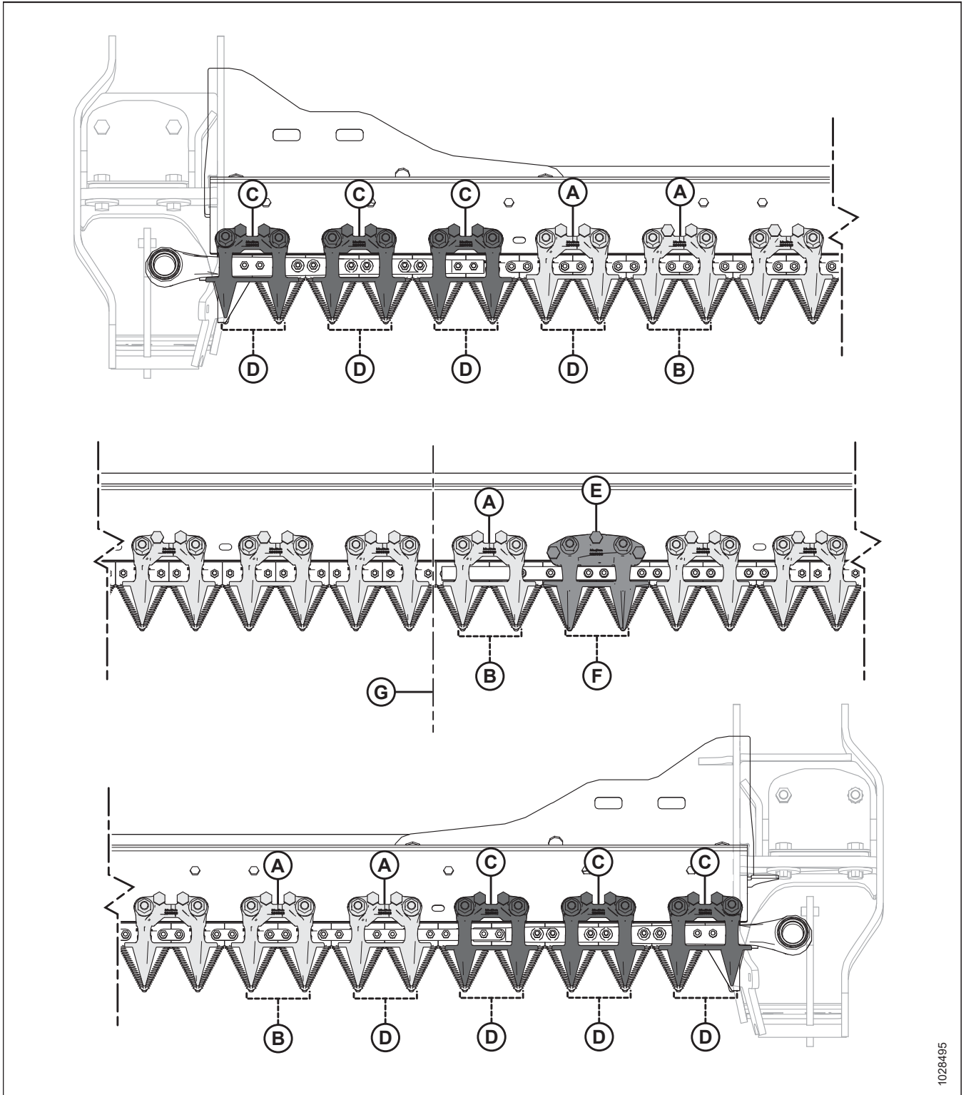
Figura 5.151: Puntón de cuchilla corto y ubicaciones del sujetador: plataformas de doble cuchilla
