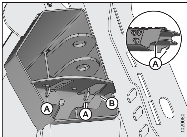
Figura 3.586: Ganchos de retención del final de horquilla
