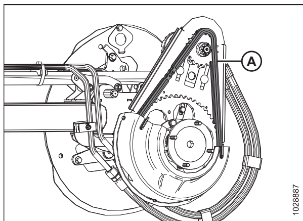
Figura 5.19: Cadena del mando
