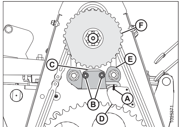
Figura 5.374: Conjunto del mando del molinete: sensor de velocidad
