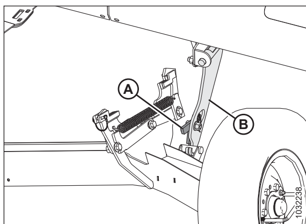
Figura 3.604: Soporte de suelo derecho
