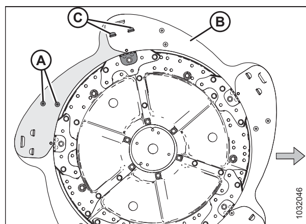
Figura 5.327: Tapas laterales del molinete: extremo de leva interior
