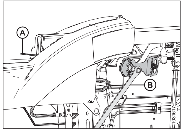
Figura 3.99: Ala en posición desbloqueada
