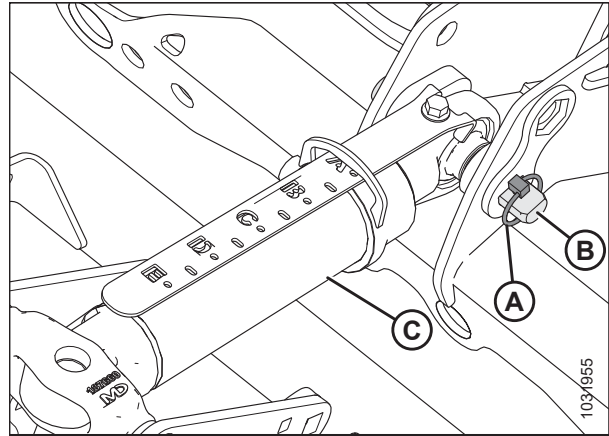
Figura 4.162: Unión central hidráulica
