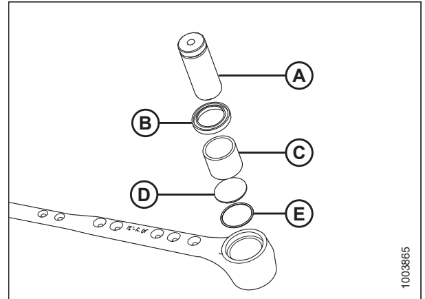
Figura 5.115: Ensamblaje del rodamiento de la cabeza de la cuchilla
