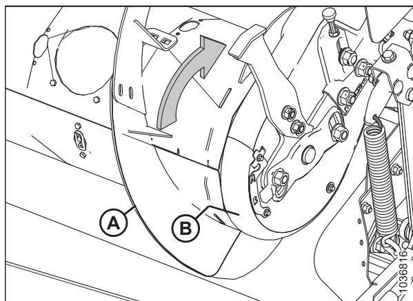
Figura 5.67: Mando del sinfín de alimentación
