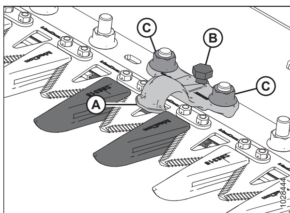
Figura 5.140: Sujetador puntiagudo
