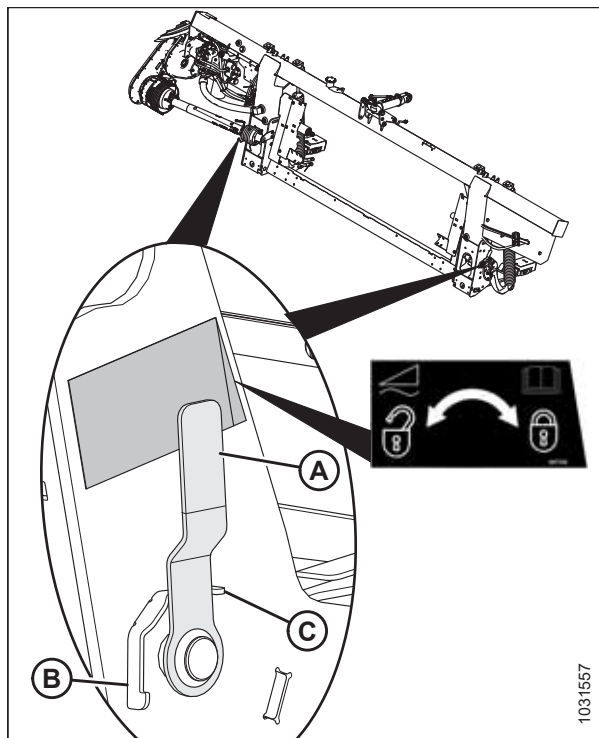
Figura 3.72: Traba de flotación: en posición de bloqueo
