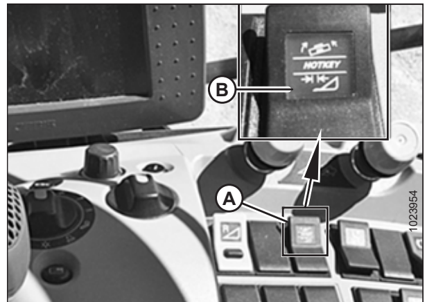
Figura 3.116: Consola CLAAS 700
