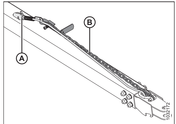
Figura 3.618: Arnés de cableado de la barra de remolque
