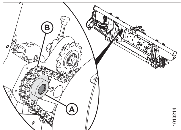
Figura 5.78: Mando del sinfín
