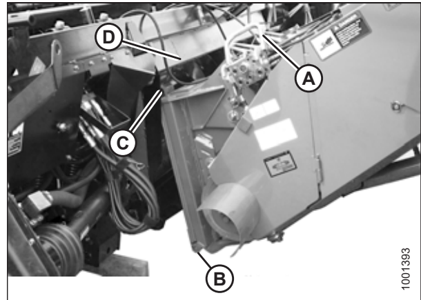
Figura 4.116: Cosechadora y módulo de flotación
