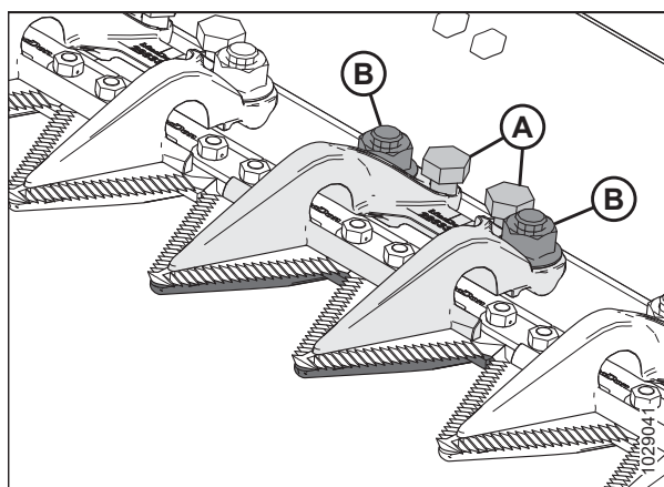
Figura 5.158: Sujetador del puntón de cuchilla corto
