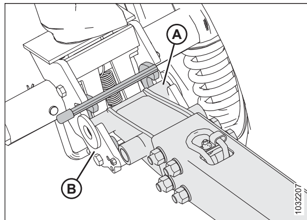
Figura 3.582: Barra de remolque y pivote de transporte
