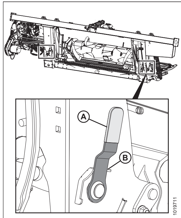
Figura 4.65: Manija de bloqueo de flotación: se muestra el lado derecho en detalle, opuesto al lado izquierdo
