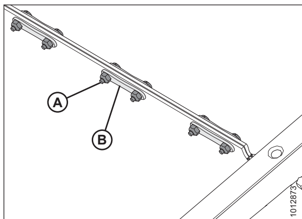
Figura 5.213: Conector de la lona
