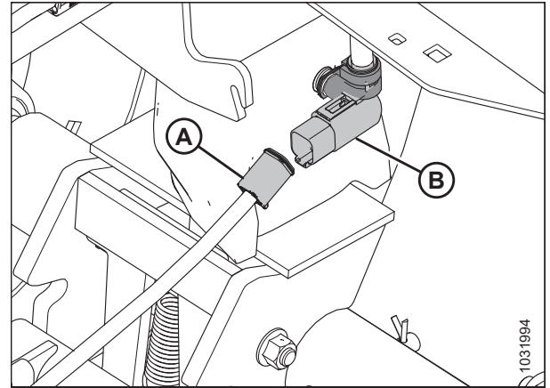
Figura 3.617: Conexión eléctrica de la barra de remolque
