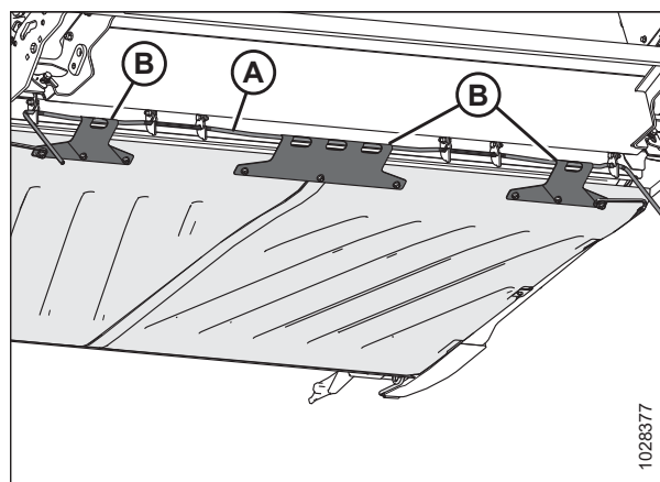
Figura 5.227: Parte inferior de la batea de la plataforma de alimentación
