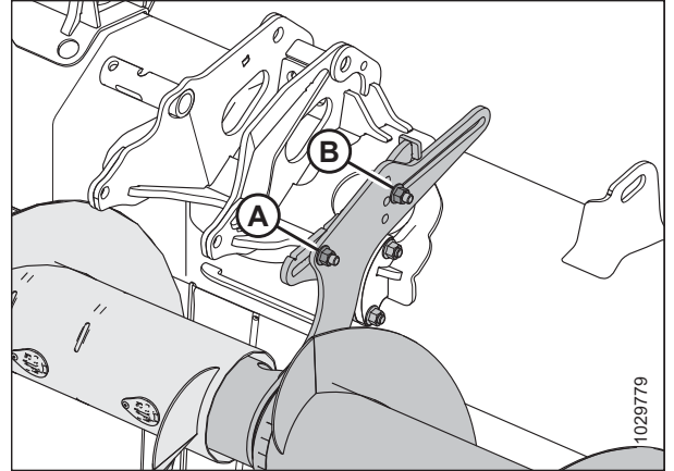
Figura 3.169: Posición inicial de los montajes ajustables: sinfín de tres piezas
