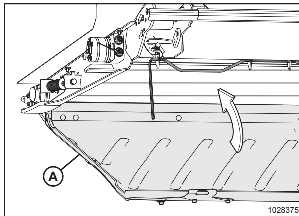
Figura 5.226: Bandeja de la plataforma de alimentación
