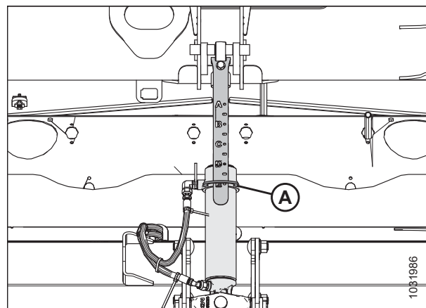
Figura 3.195: Unión central
