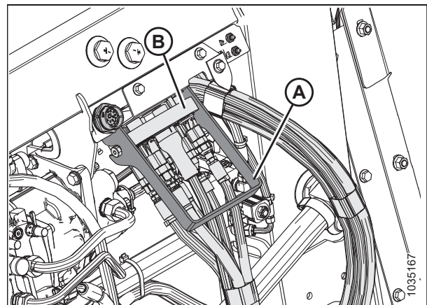
Figura 4.117: Almacenamiento del acoplamiento múltiple
