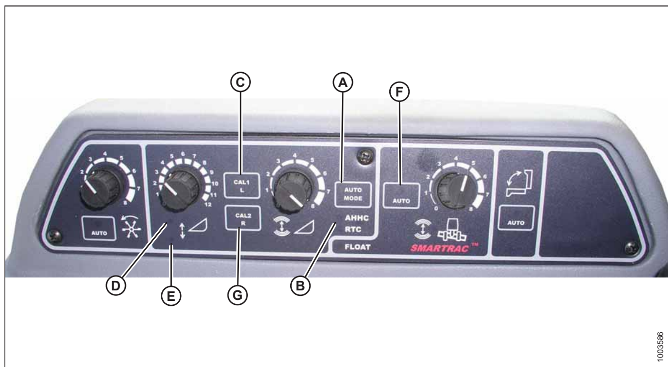
Figura 3.374: Controles automáticos de altura de la plataforma de cosechadora
