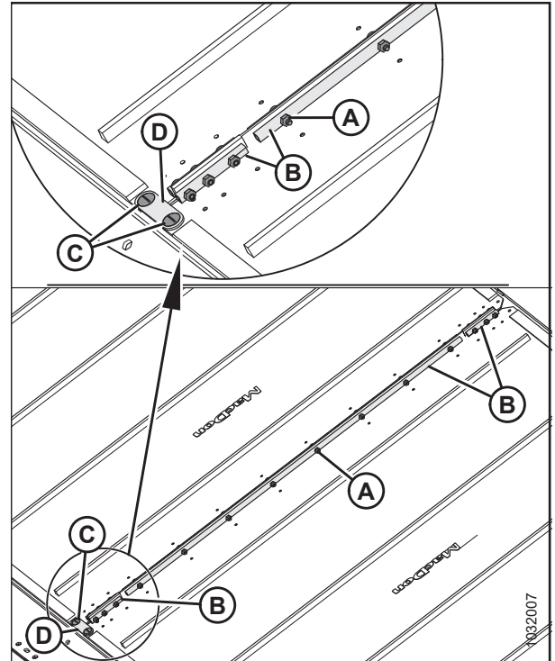
Figura 5.236: Conectores de la lona
