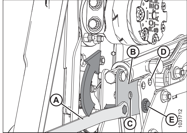
Figura 3.141: Cilindro del brazo central: Posición de avance
