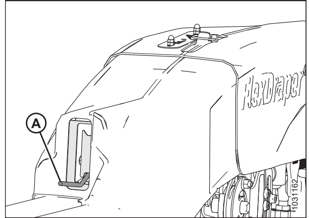
Figura 3.80: Ala en posición desbloqueada
