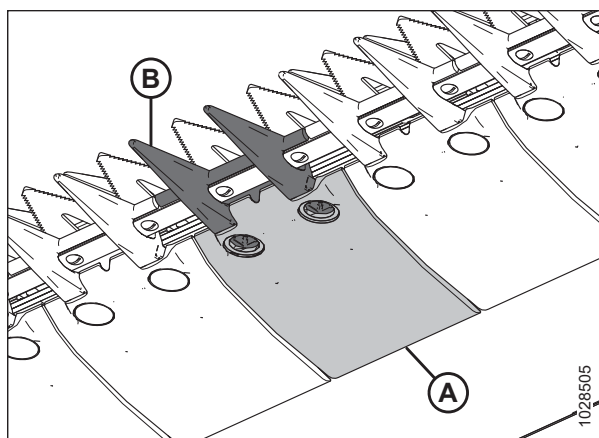
Figura 5.155: Puntón de cuchilla corto y placa de desgaste
