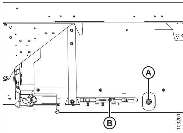
Figura 5.256: Tensor de la lona
