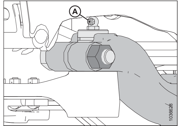
Figura 5.120: Cabeza de la cuchilla
