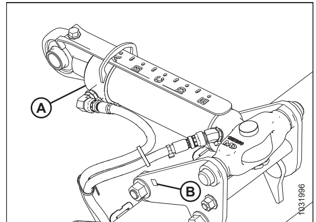
Figura 4.164: Unión central
