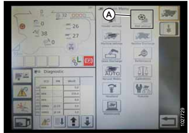
Figura 3.215: Ajustes del molinete en el menú principal de la cosechadora
