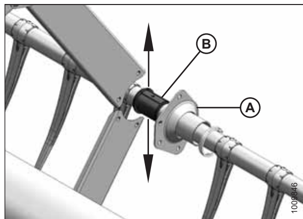
Figura 5.301: Soporte del kit de refuerzo de la barra de dientes: opcional
