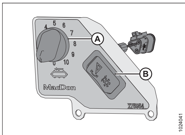
Figura 3.126: Control de velocidad de la lona lateral en cabina
