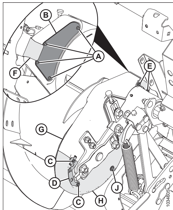
Figura 5.74: Mando del sinfín
