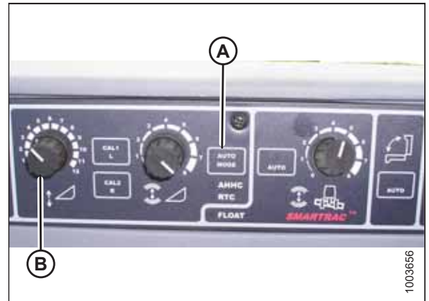
Figura 3.378: Consola de AHHC
