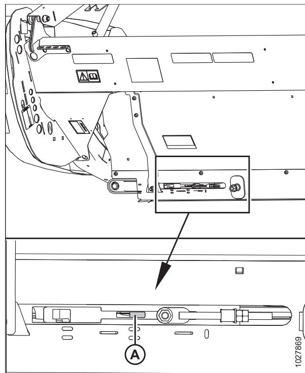
Figura 5.238: Comprobación del ajustador de tensión: se muestra el lado izquierdo; opuesto al lado derecho
