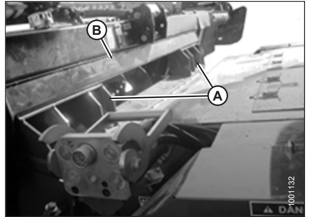
Figura 4.71: Módulo de flotación en la cosechadora
