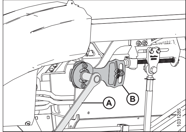
Figura 3.77: Mecanismo de bloqueo del ala
