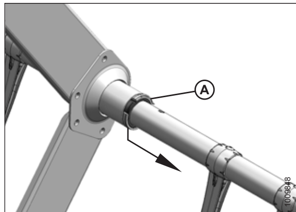
Figura 5.300: Abrazadera del buje del kit de refuerzo de la barra de dientes: opcional
