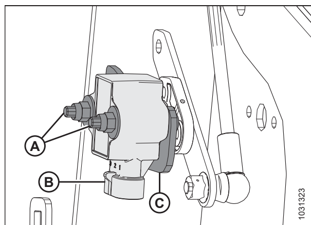
Figura 3.135: Sensor de altura del molinete-Brazo del molinete derecho
