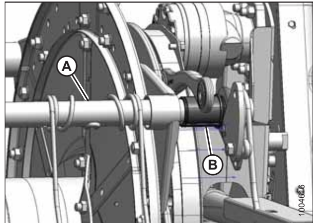
Figura 5.314: Extremo de leva
