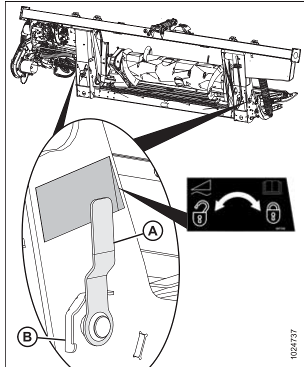
Figura 4.89: Manija de bloqueo de flotación
