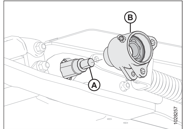
Figura 5.219: Rodamiento de rodillo tensor: lado izquierdo
