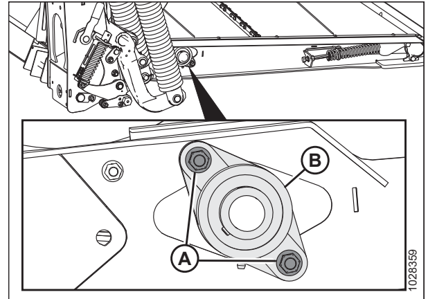
Figura 5.192: Rodamiento del rodillo de mando
