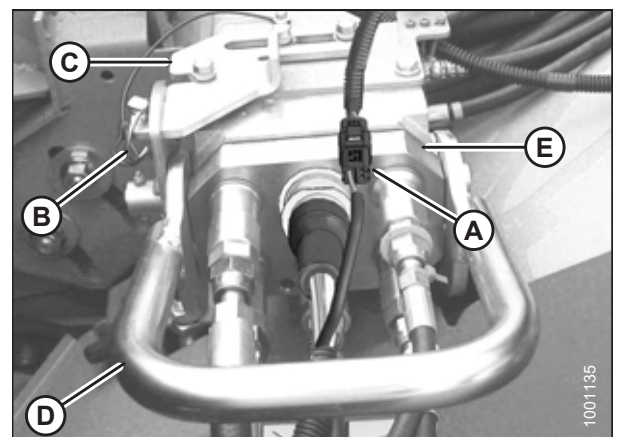
Figura 4.129: Acoplador múltiple
