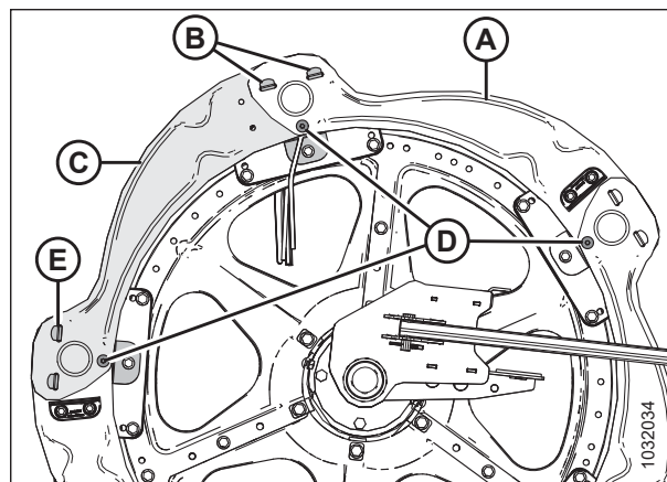
Figura 5.333: Tapas laterales del molinete: sección final exterior
