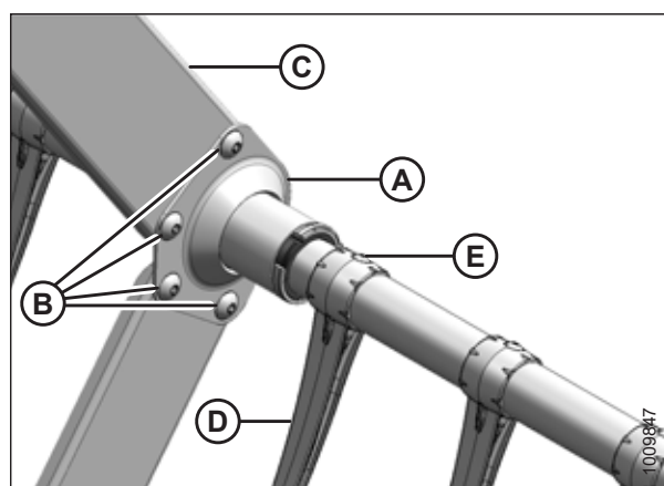
Figura 5.319: Soporte del kit de refuerzo de la barra de dientes: opcional
