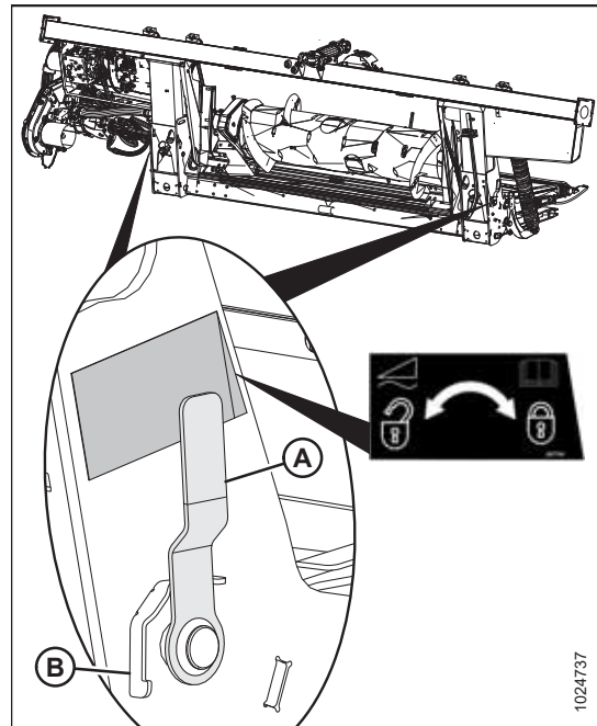
Figura 4.61: Manija de bloqueo de flotación
