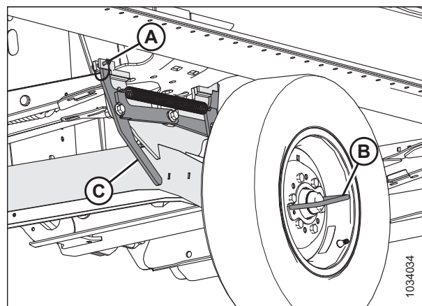
Figura 3.593: Eje de transporte derecho enganchado en la posición de transporte
