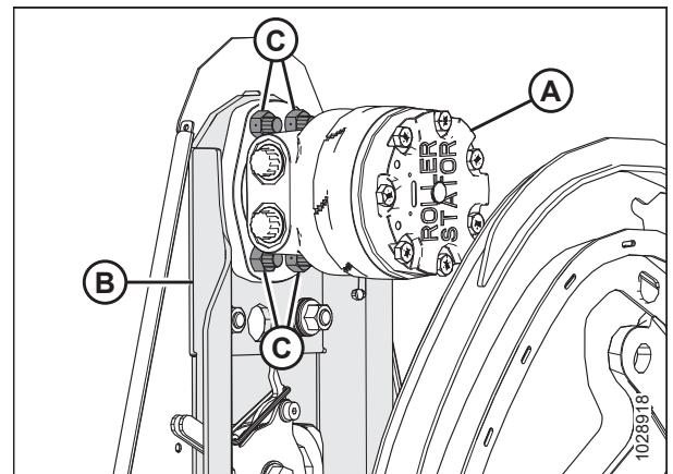
Figura 5.363: Motor del mando del molinete
