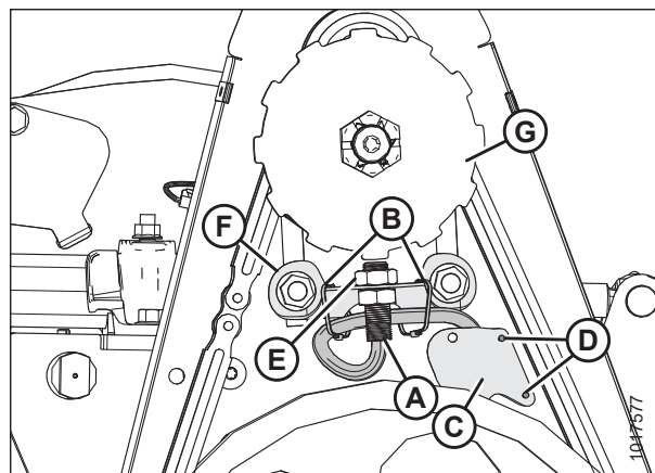
Figura 5.377: Sensor de velocidad
