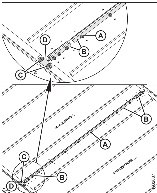
Figura 5.265: Conector de la lona
