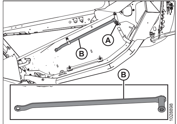
Figura 3.81: Parte final izquierda
