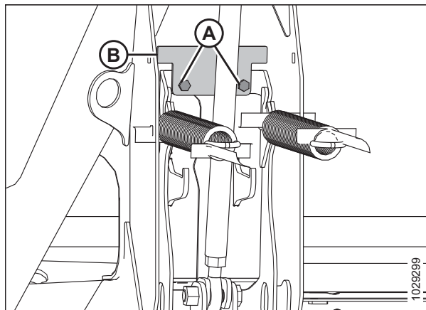
Figura 3.91: Placa limitadora de "cara triste" de flexión
