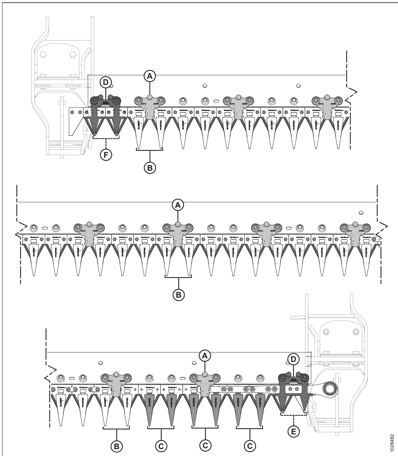
Figura 5.124: Puntones de cuchilla puntiagudos y ubicaciones de los sujetadores: plataformas de cuchilla simple
