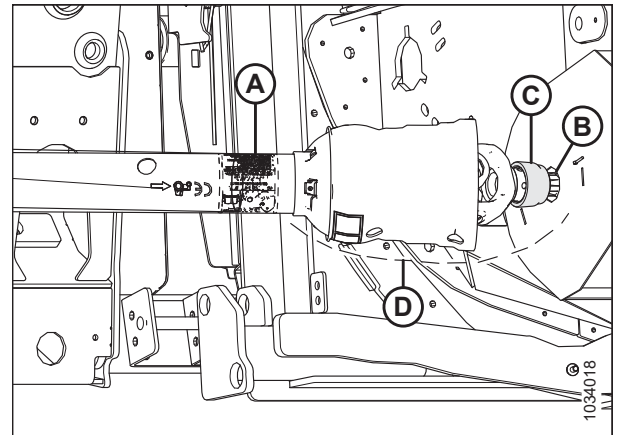
Figura 4.177: Cardán de inclinación lateral
