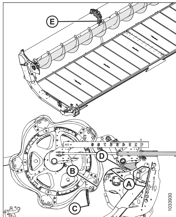
Figura 3.172: Ubicaciones de verificación de separación del UCA
