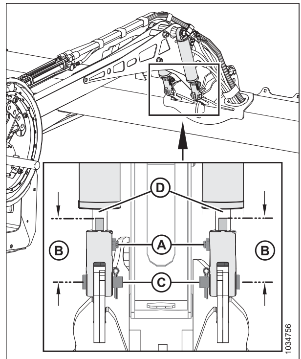
Figura 5.276: Cilindro del brazo central
