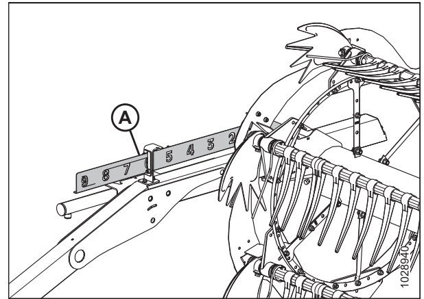
Figura 3.94: Posición avance-retroceso
