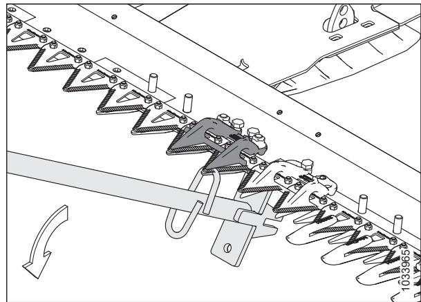
Figura 5.133: Ajuste hacia abajo: puntón de cuchilla corto
