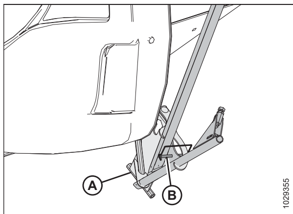
Figura 3.185: Almacenamiento de la varilla abresurcos para arroz
