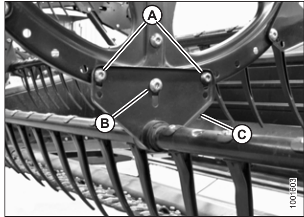
Figura 5.280: Disco del molinete central
