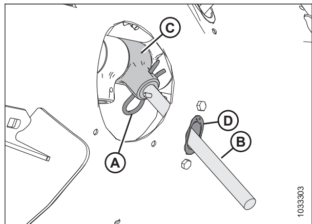
Figura 4.49: Dedo del sinfín
