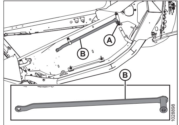
Figura 3.104: Parte final izquierda
