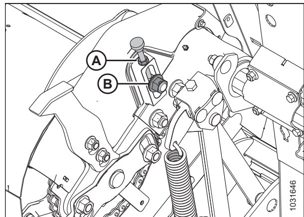
Figura 5.91: Cadena del sinfín de alimentación: vista delantera
