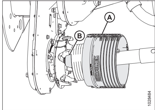
Figura 5.37: Escudo del cardán para cosechadora
