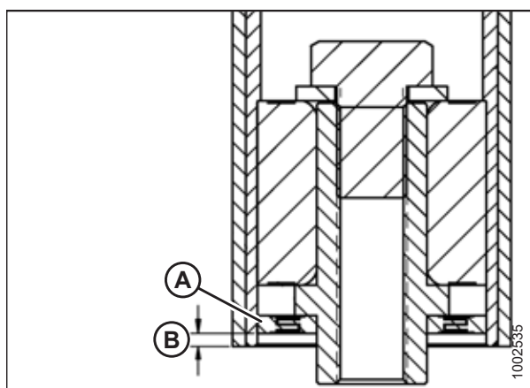
Figura 5.252: Rodamiento del rodillo tensor
