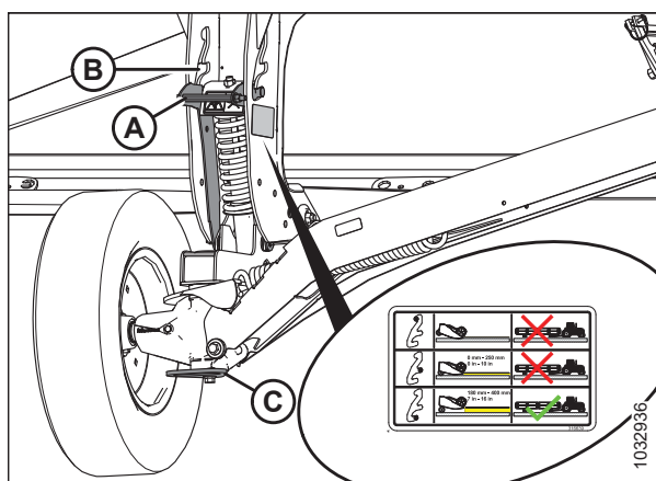
Figura 3.35: Rueda derecha
