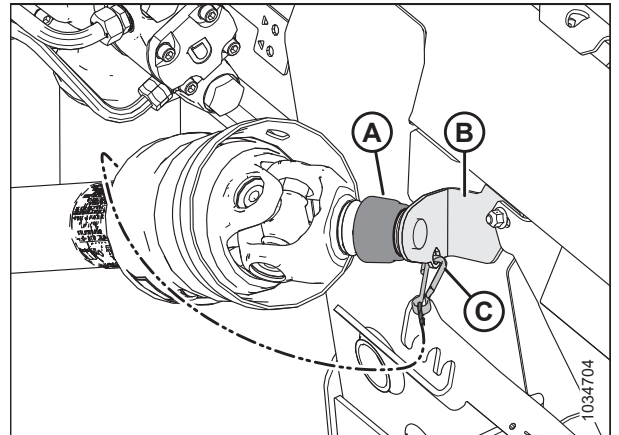
Figura 4.105: Cardán en posición de almacenamiento: cardán Sidehill/Hillside MD n.º B7180, MD n.º B7181, o MD n.º B7182
