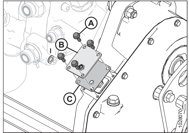
Figura 5.59: Cubierta del tensor de la cadena de la caja de engranajes principal
