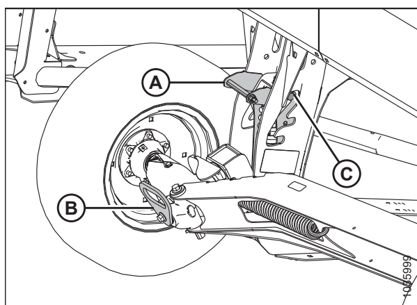
Figura 3.596: Ruedas de transporte derechas en la posición de almacenamiento más alta
