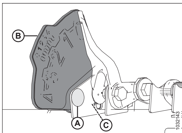
Figura 3.201: Indicador de configuración de flotación: izquierdo
