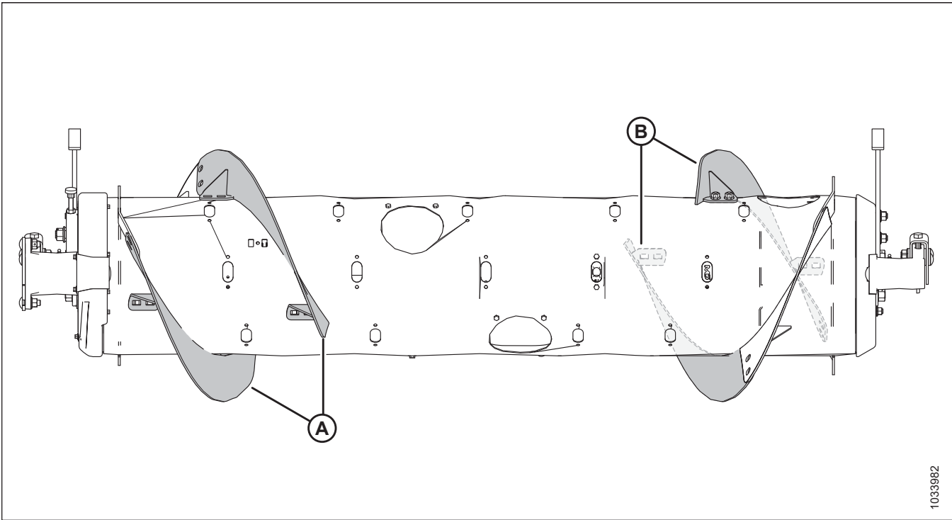
Figura 4.6: Configuración estrecha
