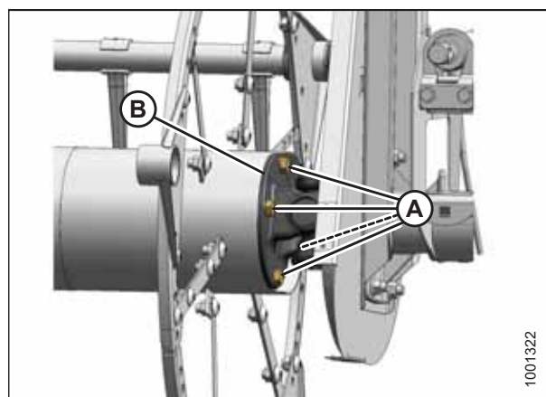
Figura 5.369: Cruceta
