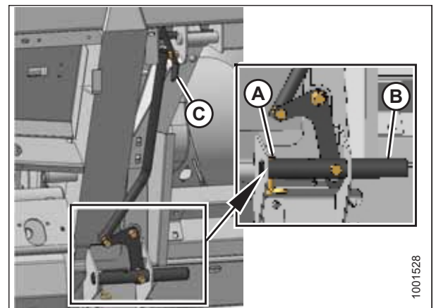
Figura 4.114: Trabas del alimentador
