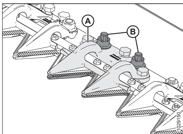
Figura 5.164: Puntón de cuchilla central
