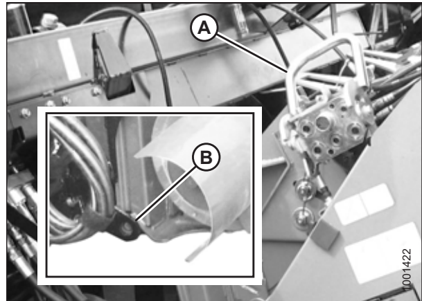
Figura 4.131: Trabas del embocador
