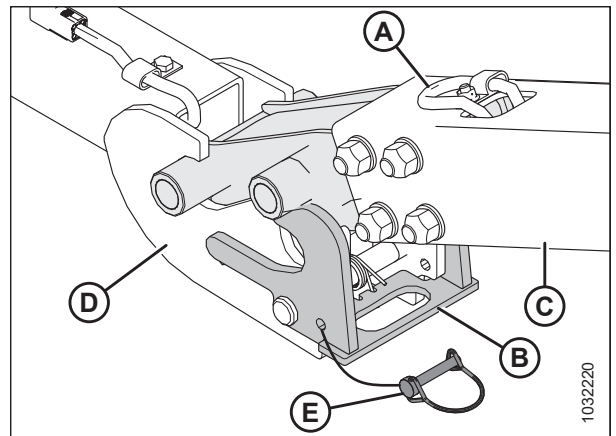
Figura 3.613: Barra de remolque a la extensión
