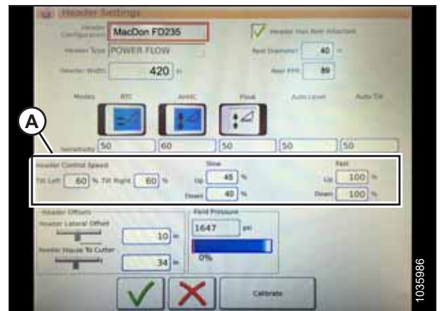
Figura 3.397: Configuraciones de control de la velocidad de la plataforma
