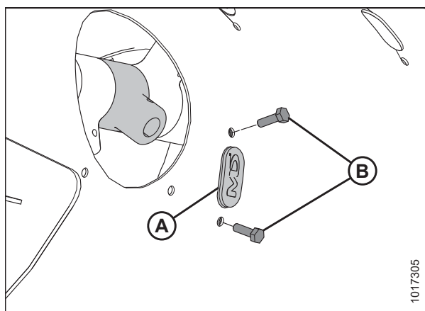
Figura 5.96: Tapón
