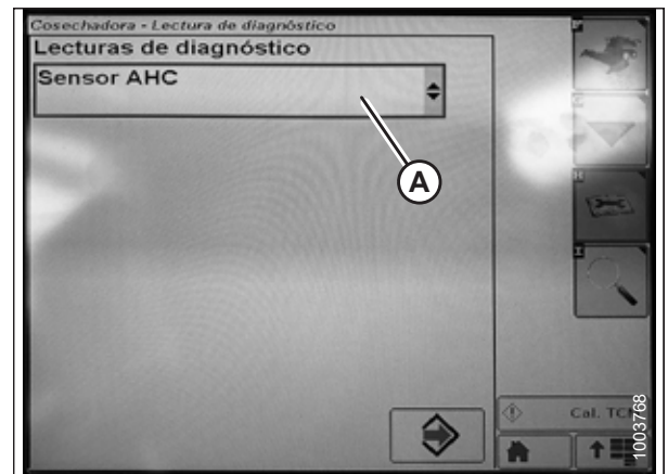
Figura 3.435: Pantalla de la cosechadora John Deere
