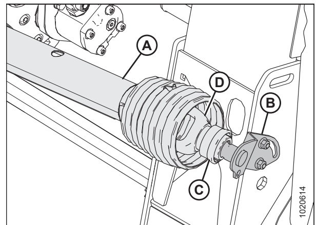
Figura 5.55: Extremo del mando de la cosechadora
