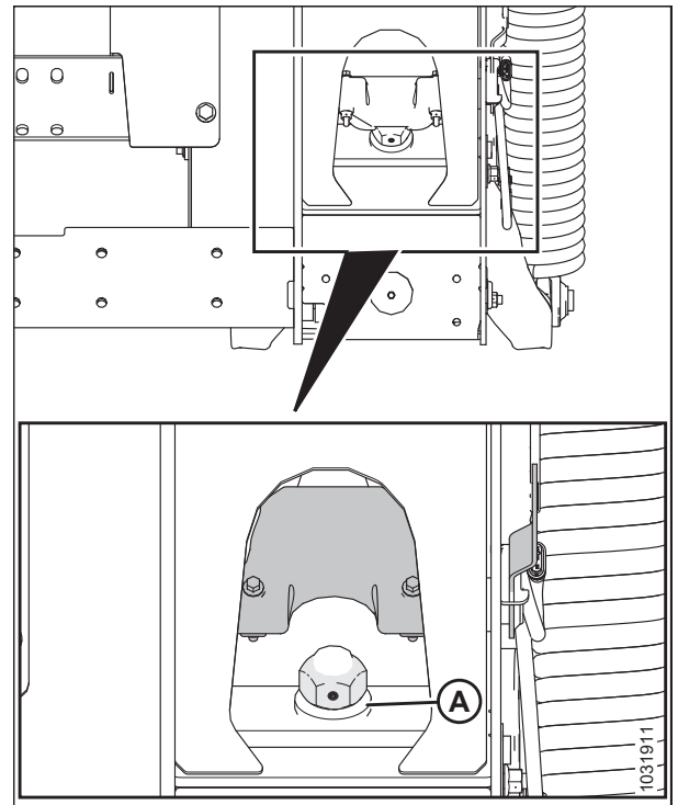
Figura 3.416: Traba de flotación
