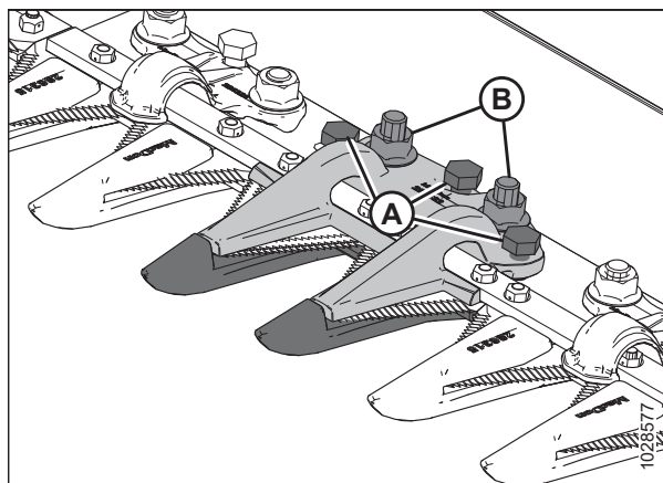
Figura 5.148: Sujetador central puntiagudo
