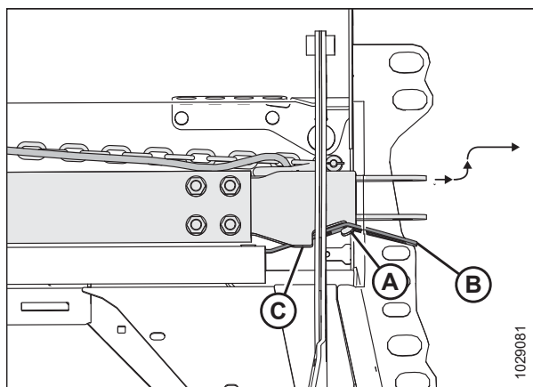
Figura 3.609: Barra de remolque en almacenamiento
