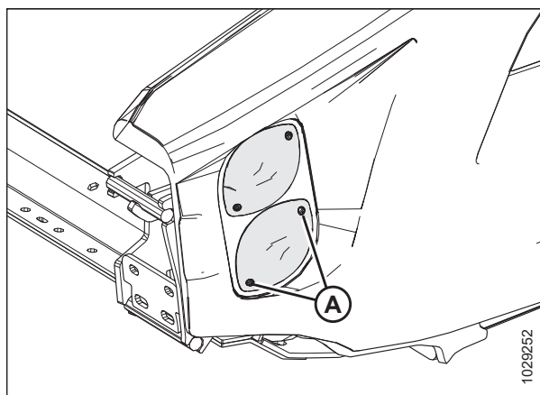
Figura 5.34: Transporte de auto-tráiler opcional (luces roja y ámbar)
