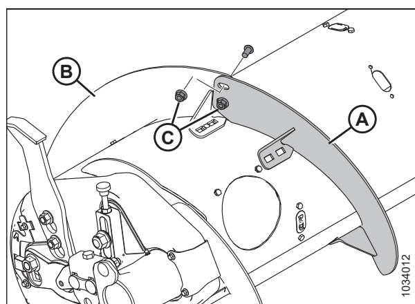
Attēls 3.121: Gliemežtransportiera kreisā puse
