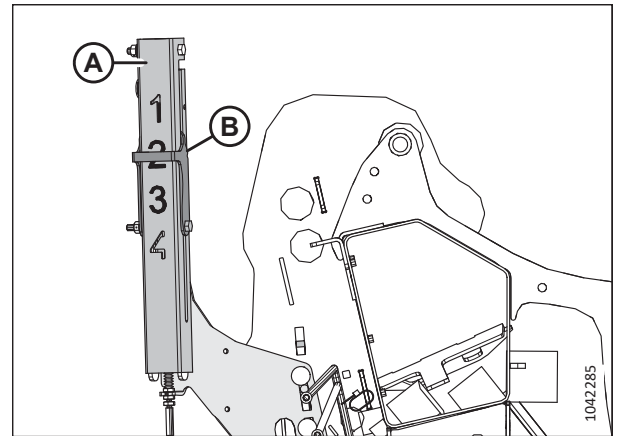
Attēls 3.144: Augstuma indikators — aizmugurējais kreisais gals
