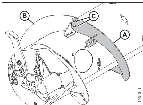
Attēls 3.119: Gliemežtransportiera kreisā puse
