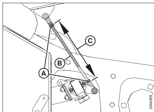
Attēls 3.207: Tītavu augstuma sensors — nolaišta labās puses tītavu svira
