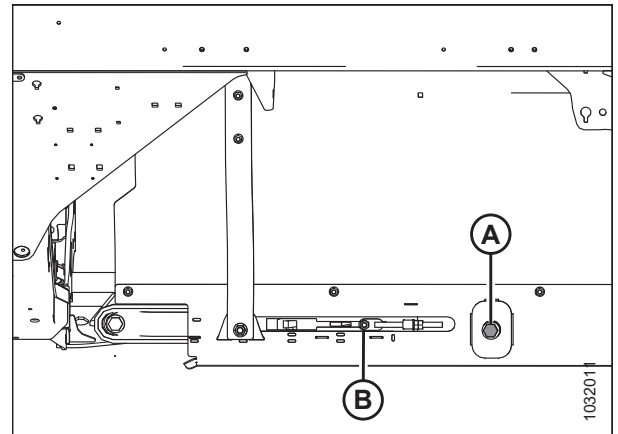
Attēls 4.246: Stiebru pacēlāja spriegotājs
