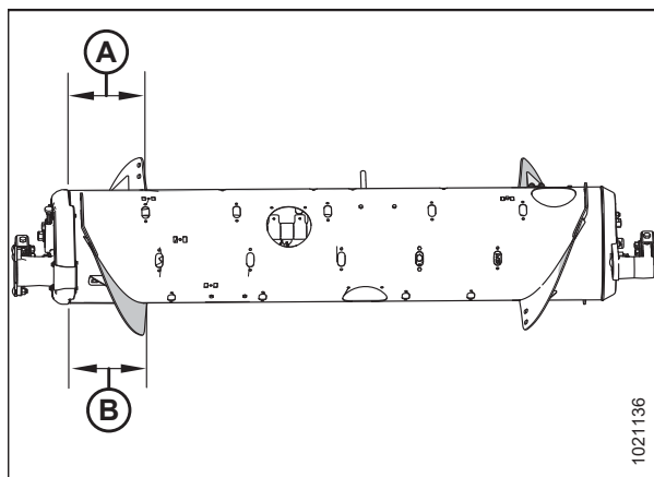
Attēls 3.81: Plata konfigurācija — skats no aizmugures
