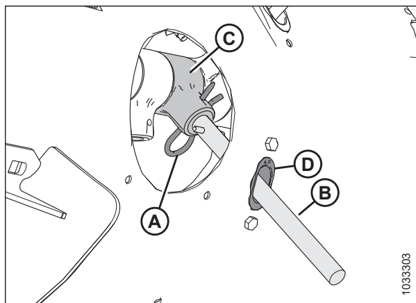
Attēls 3.126: Gliemežtransportiera pirksts
