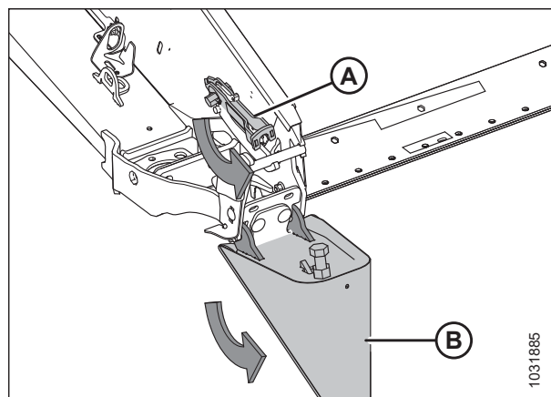
Attēls 3.242: Kultūraugu dalītājs ar aizdaru
