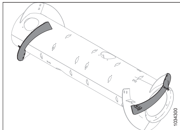
Attēls 5.14: Augstas nodiluma pakāpes spirālveida lāpstiņu pagarinājuma komplekts padeves gliemežtransportierim
