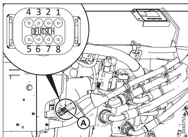
Attēls 3.264: Savienotājs
