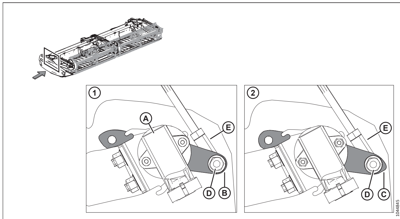
Attēls 3.204: Tītavu augstuma sensora novietojums
