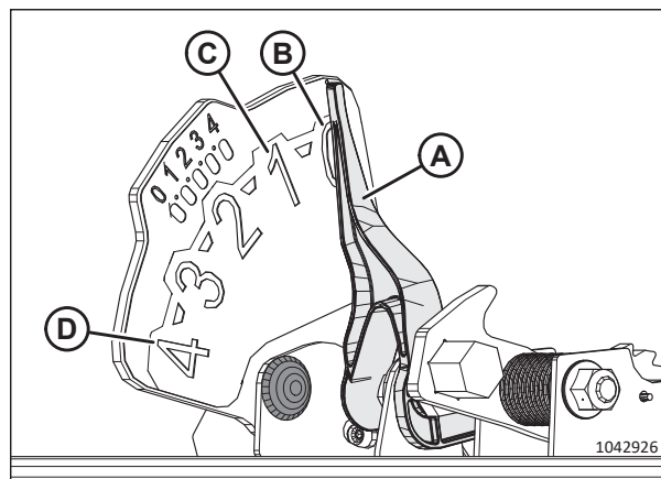
Attēls 3.288: Reljefa kopēšanas indikators
