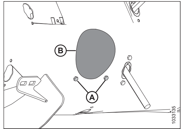
Attēls 4.86: Gliemežtransportiera piekļuves atveres pārsegs
