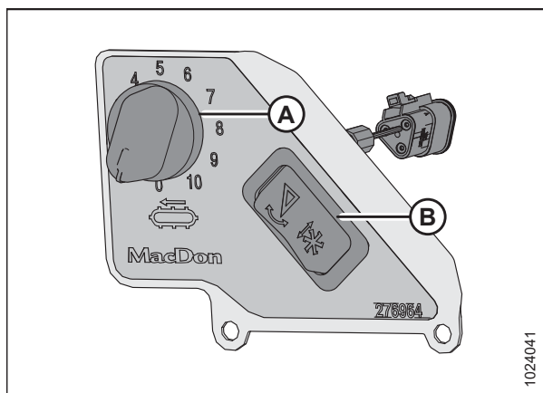
Attēls 3.200: Sānu stiebru pacēlāja ātruma vadības ierīce kabīnē
