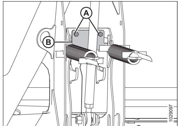
Attēls 3.181: Locīšanas izvērsuma ierobežotāja plāksne
