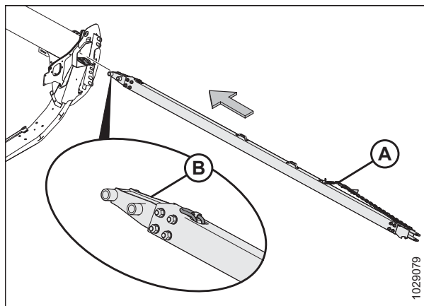
Attēls 3.348: Sakabes gals
