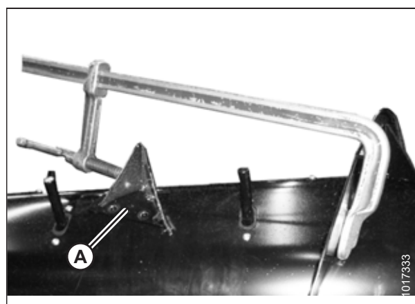
Attēls 3.122: Spirālveida lāpstiņu aksiāls novietojums
