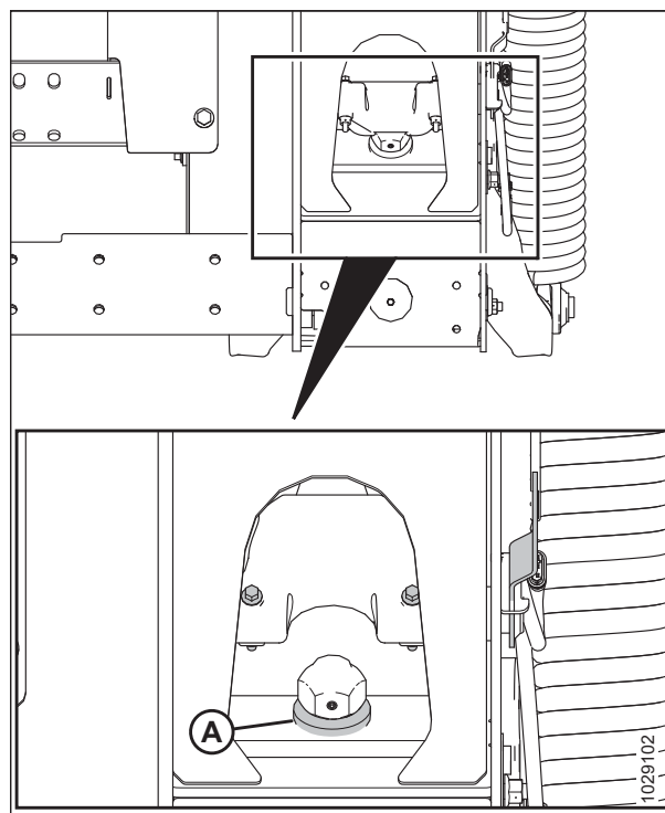
Attēls 3.295: Paplāksne aizturēm uz leju
