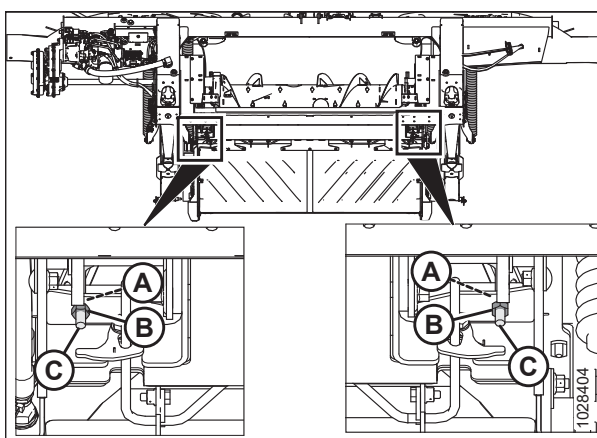
Attēls 3.138: Atsperu spriegotājs
