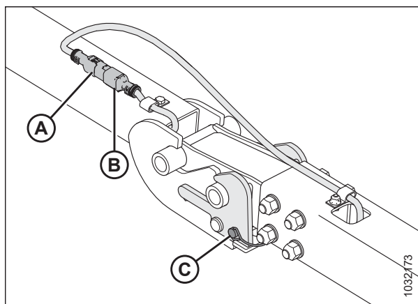
Attēls 3.377: Jūgstieņa / pagarinājuma stiprinājums
