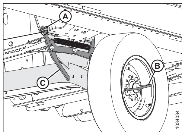
Attēls 3.356: Labā transportēšanas ass fiksēta transportēšanas stāvoklī
