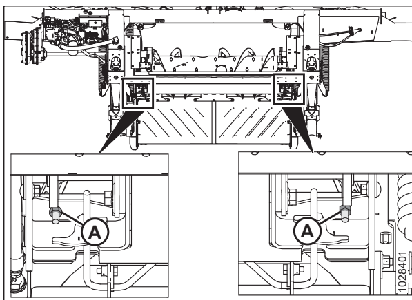
Attēls 3.137: Atsperu spriegotājs
