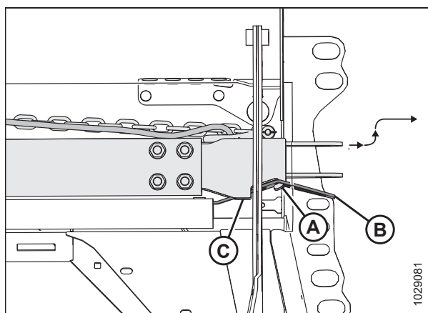
Attēls 3.372: Jūgstienis uzglabāšanā
