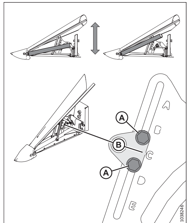
Attēls 3.254: Sānu deflektora augstuma regulēšana
