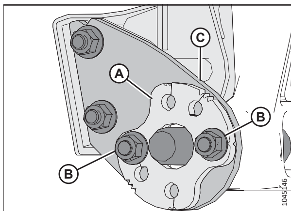
Attēls 3.64: AF11 padeves tvertnes aizturtaņas
