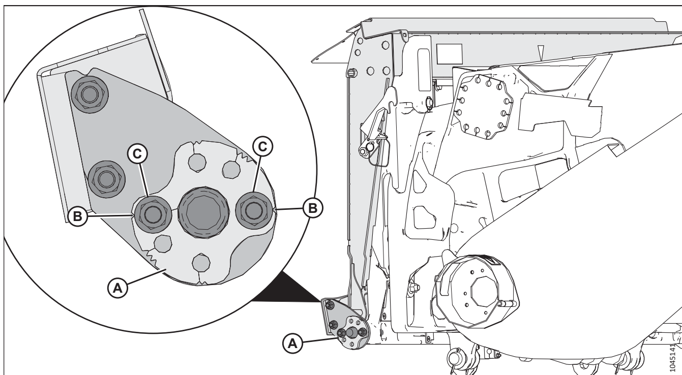
Attēls 3.61: Kombains un reljefa kopēšanas modulis
