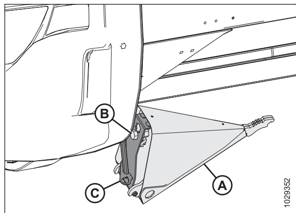
Attēls 3.240: Papildu kultūraugu dalītājs
