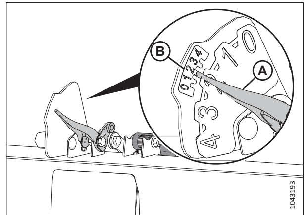
Attēls 3.145: Automātiskā hedera augstuma indikators
