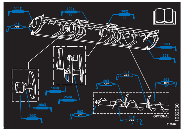
Attēls 4.22: FD2 sērijas eļļošanas punktu izkārtojuma uzlīme
