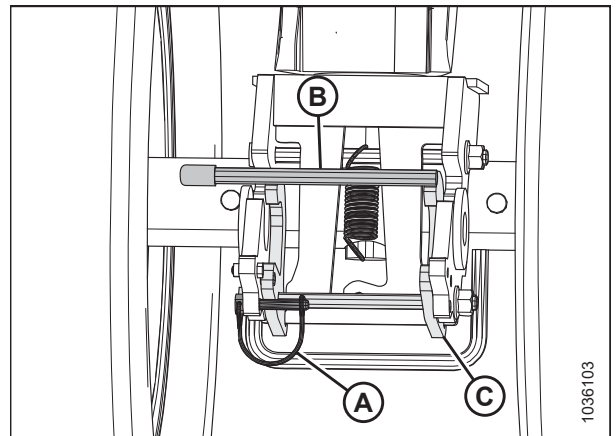
Attēls 3.351: Kreisie transportēšanas riteņi — griešanās bloķēšanas fiksators ir atvienots
