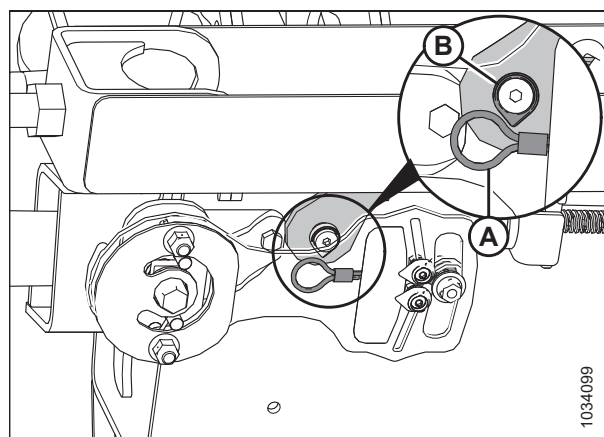
Attēls 3.188: Kreisās puses locīšanas kontrolierīces kabeļa bloķētājs
