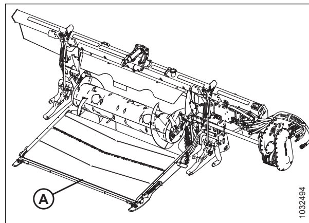
Attēls 3.202: FM200 reljefa kopēšanas modulis
