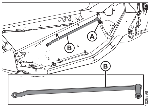
Attēls 3.179: Kreisā gala loksne
