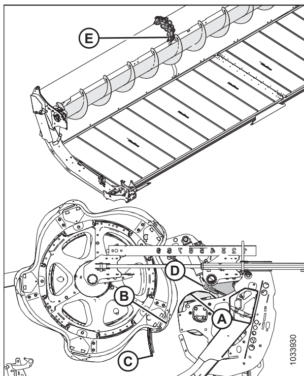
Attēls 3.236: AKG klīrensa pārbaudes vieta
