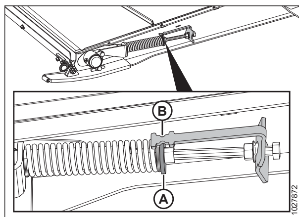
Attēls 4.167: Padeves stiebru pacelāja spriegotājs
