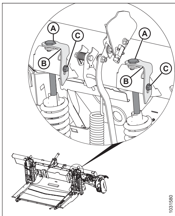
Attēls 3.166: Reljefa kopēšanas moduļa regulēšana kreisajā pusē
