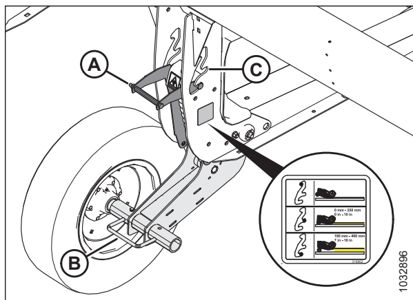
Attēls 3.139: Stabilizatora ritenis
