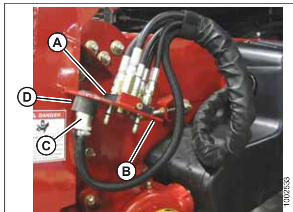
Attēls 3.75: Multisavienotāja uzglabāšana
