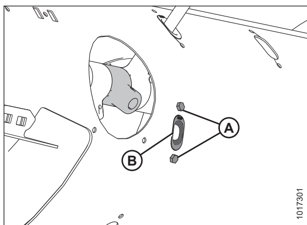
Attēls 3.127: Gliemežtransportiera pirksta caurums
