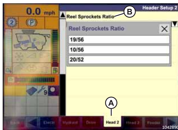
Attēls 3.333: Case IH kombaina displejs
