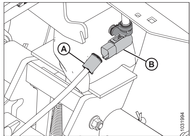
Attēls 3.340: Jūgstieņa elektriskais savienojums
