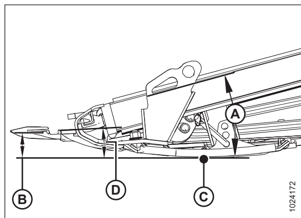
Attēls 3.151: Hedera leņķis
