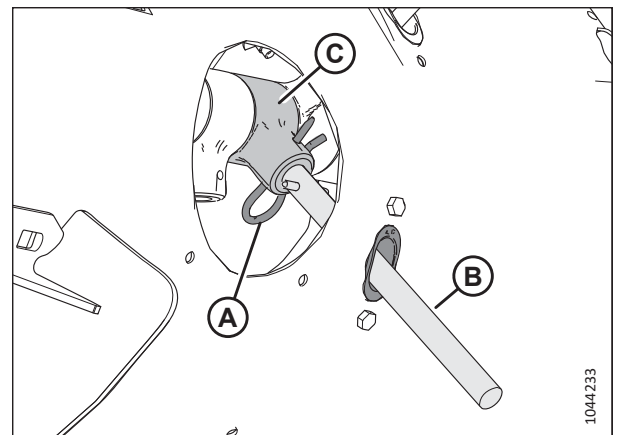
Attēls 4.87: Gliemežtransportiera pirksts
