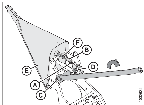
Attēls 3.246: Uzstādīts kultūraugu dalītājs
