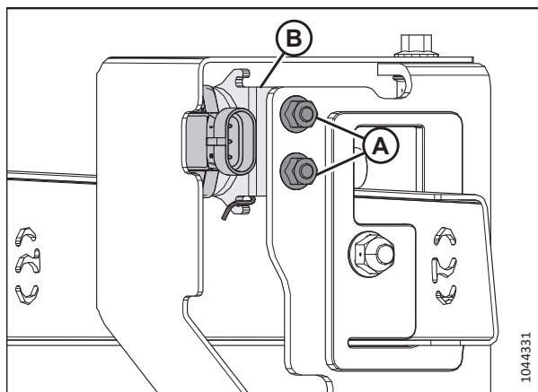
Attēls 3.220: Atgāzuma sensors
