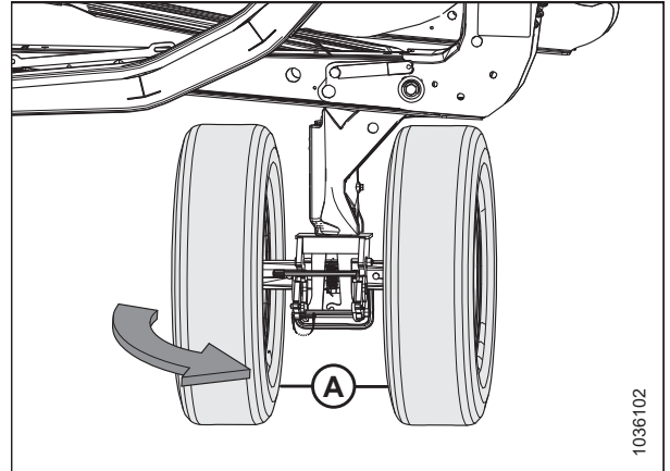
Attēls 3.350: Kreisie transportēšanas riteņi transportēšanas režīmā
