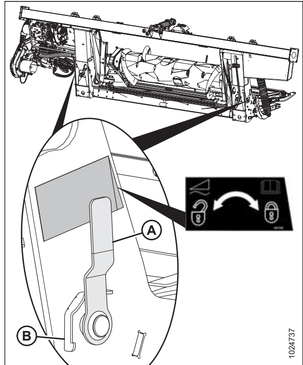
Attēls 3.162: Hedera reljefa kopēšanas bloķējums bloķētā stāvoklī
