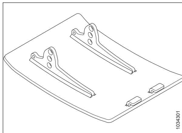
Attēls 5.27: Tērauda sliežu uzliku komplekts
