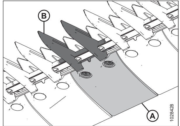
Attēls 4.125: Smails naža aizsargs un nodilumplāksne
