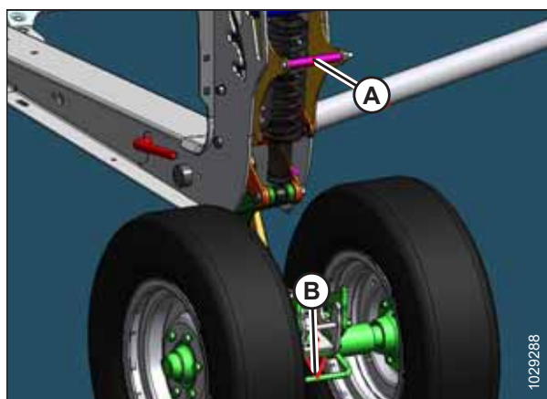
Attēls 3.362: Priekšējie transportēšanas riteņi
