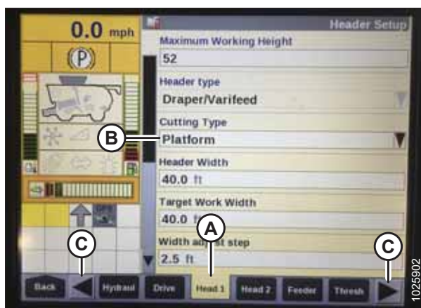
Attēls 3.279: Case IH kombaina displejs
