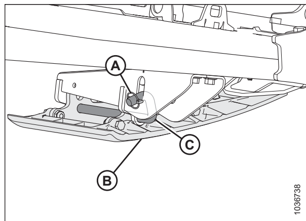
Attēls 3.150: Ārējā sliežu uzlika
