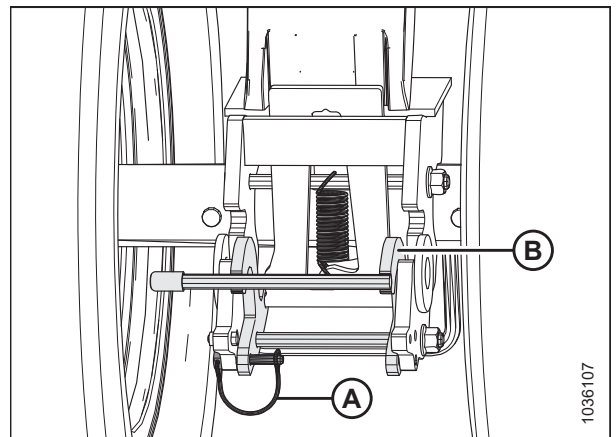
Attēls 3.352: Kreisie transportēšanas riteņi — rotācijas bloķēšanas fiksators ir saslēgts
