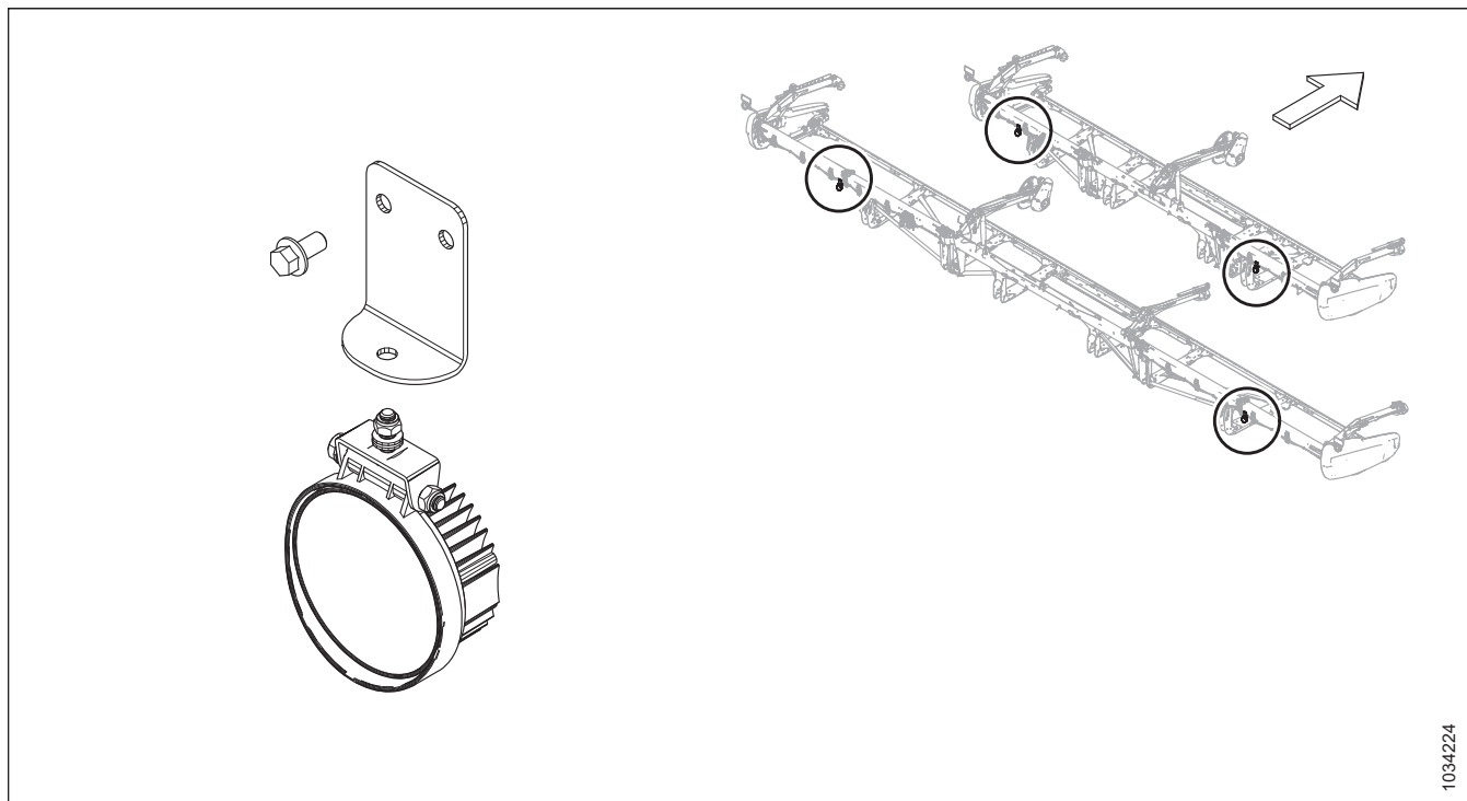
Attēls 5.28: Rugāju lukturu komplekts
