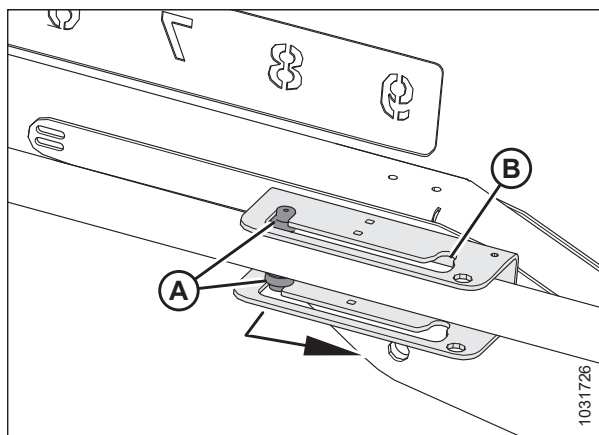
Attēls 3.216: Atgāzuma cilindra regulēšanas 2. tips — pozīcija uz priekšu
