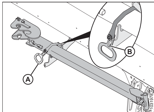
Attēls 3.347: Jūgstieņa pagarinājuma uzglabāšana
