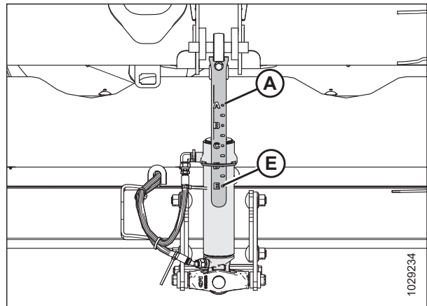
Attēls 3.153: Vidējā atsaite
