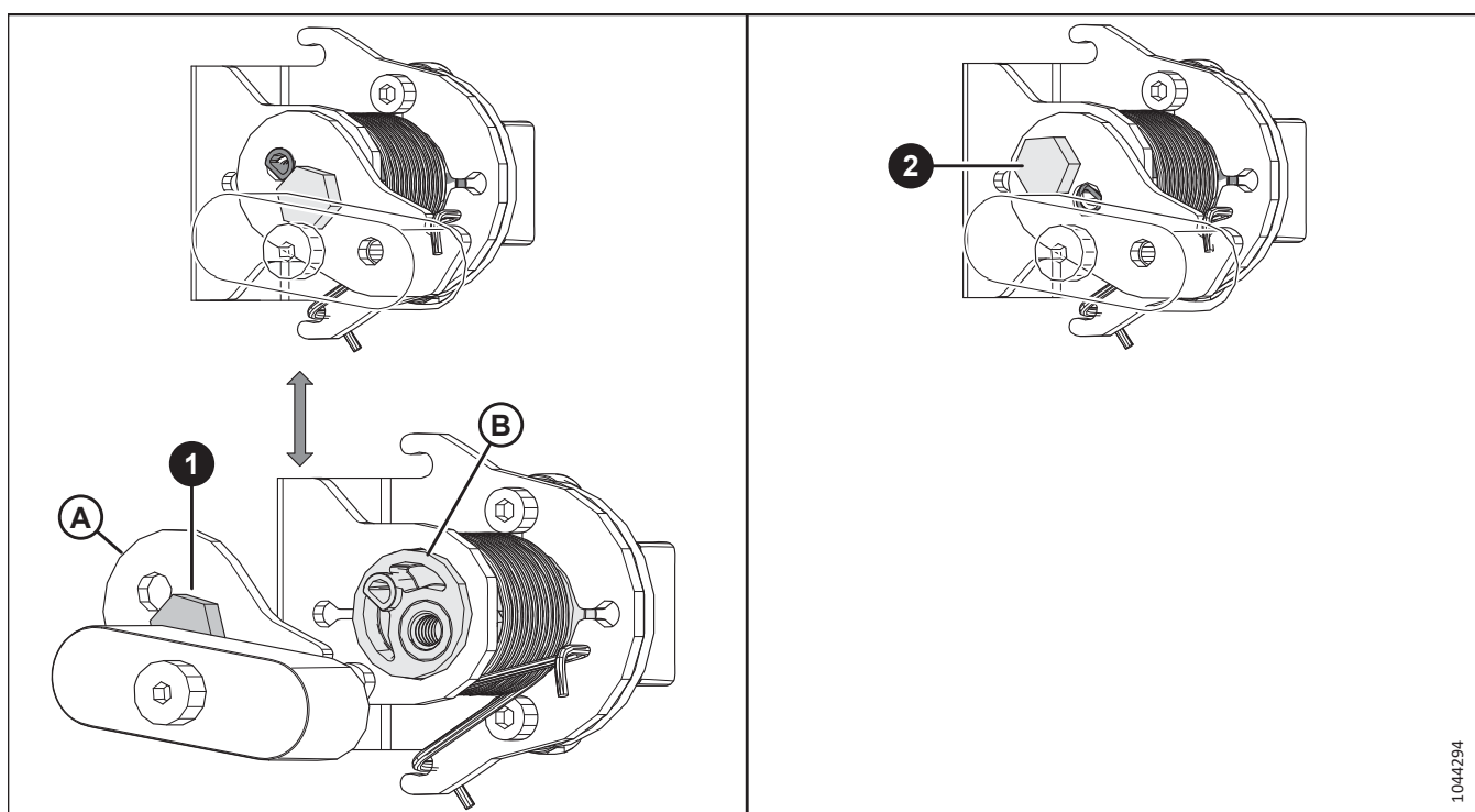
Attēls 3.222: Senora sviras pozīcija
