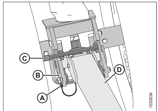
Attēls 3.341: Jūgstieņa pagarinājums un transportēšanas šarnīrs
