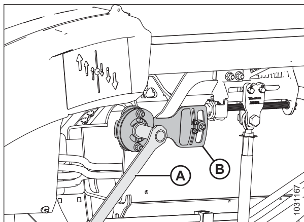
Attēls 3.180: Spārns bloķētā stāvoklī
