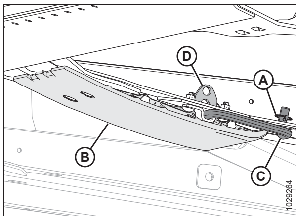
Attēls 3.149: Iekšējā sliežu uzlika
