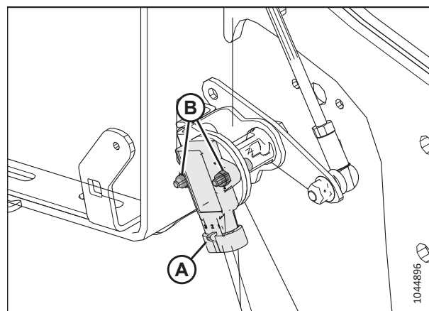
Attēls 3.205: Tītavu augstuma sensors — labās puses tītavu svira
