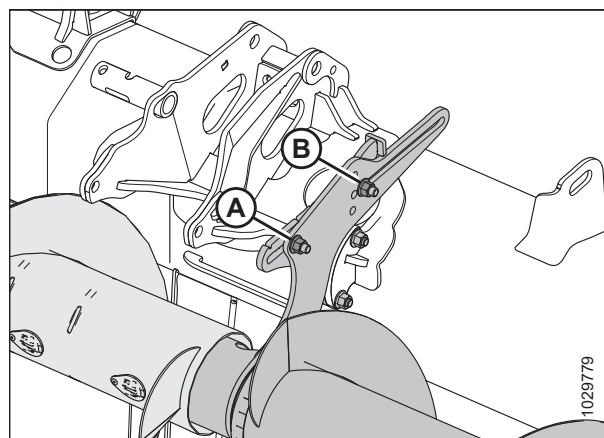
Attēls 3.235: Regulējamo stiprinājumu sākotnējā pozīcija — trīsdaļīgs gliemežtransportieris
