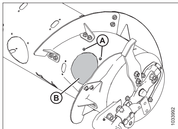
Attēls 3.105: Gliemežtransportiera piekļuves pārsegs — labā puse
