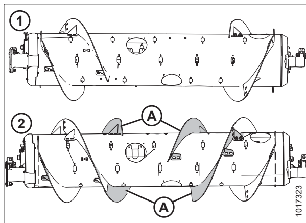
Attēls 3.84: Gliemežtransportiera konfigurācijas — skats no aizmugures
