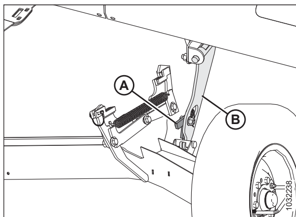
Attēls 3.367: Lauka balsts labajā pusē
