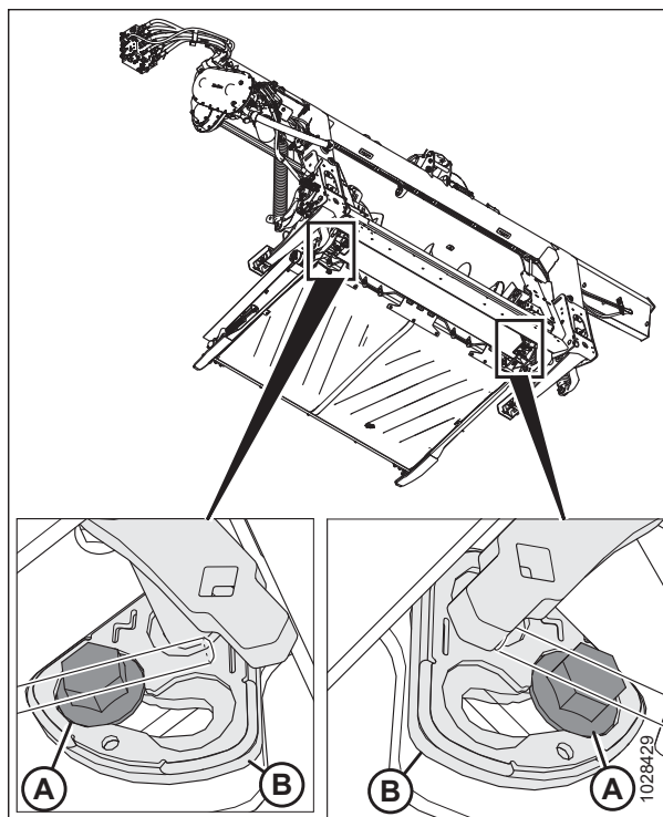
Attēls 3.135: Padeves gliemežtransportiera reljefa kopēšanas regulēšana
