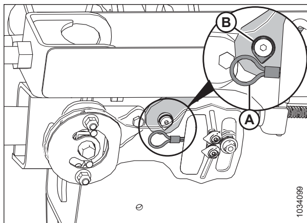
Attēls 3.195: Kreisās puses locīšanas kontrolierīces kabeļa bloķētājs
