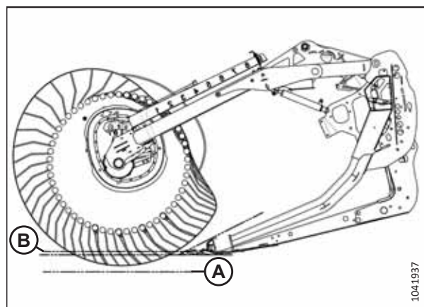
Attēls 3.227: Pirksta profils — izciļņa 4. pozīcija, maksimālais hedera leņķis
