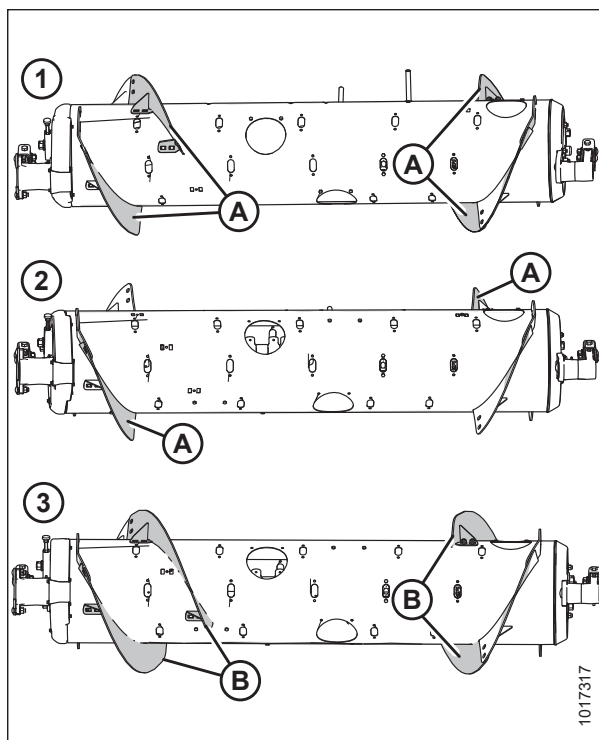
Attēls 3.90: Gliemežtransportiera konfigurācijas — skats no aizmugures
