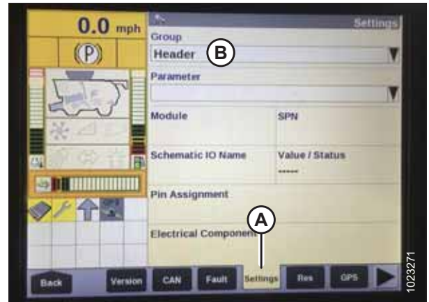
Attēls 3.275: Case IH kombaina displejs
