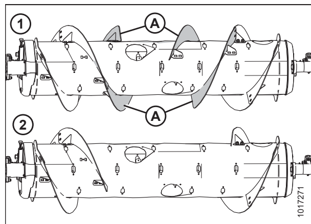
Attēls 3.89: Gliemežtransportiera konfigurācijas — skats no aizmugures
