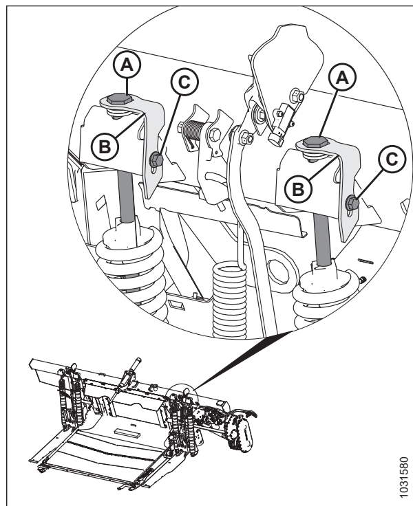
Attēls 3.168: Reljefa kopēšanas moduļa regulēšana kreisajā pusē
