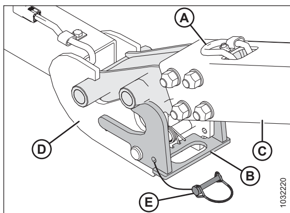
Attēls 3.376: Jūgstienis pie pagarinājuma
