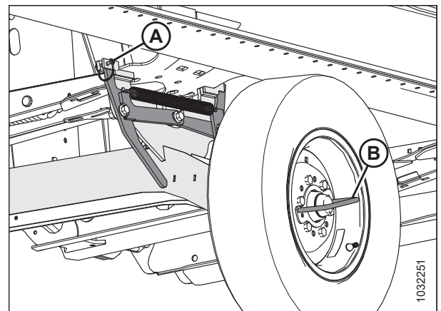
Attēls 3.370: Labā transportēšanas ass
