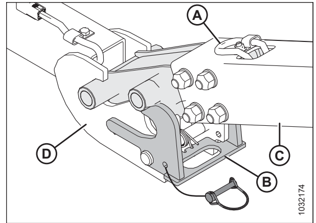
Attēls 3.339: Jūgstieņa / pagarinājuma savienojums
