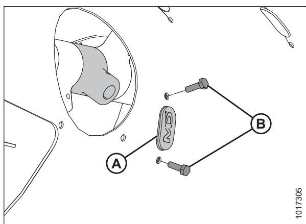
Attēls 3.128: Noslēgs
