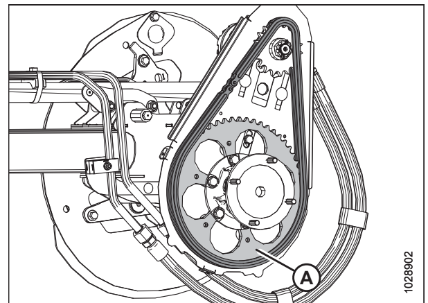
Attēls 4.321: Tītavu piedziņa
