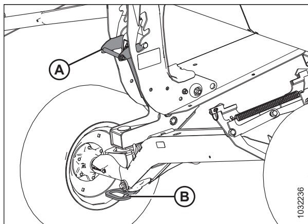
Attēls 3.366: Atbalsta riteņi
