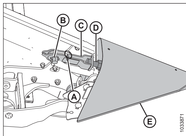
Attēls 3.237: Kultūraugu dalītājs ar aizdari
