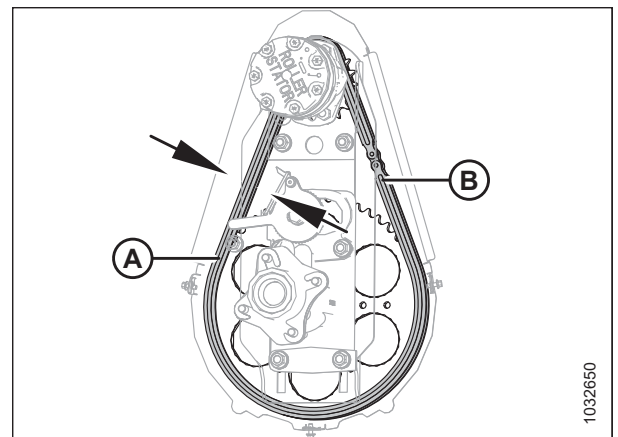
Attēls 4.320: Tītavu piedziņa
