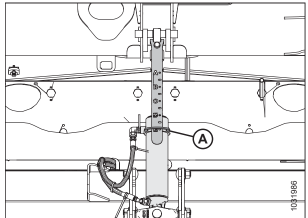
Attēls 3.270: Vidējā atsaite
