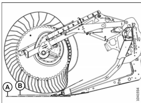
Attēls 3.223: Pirksta profils — izciļņa 1. pozīcija
