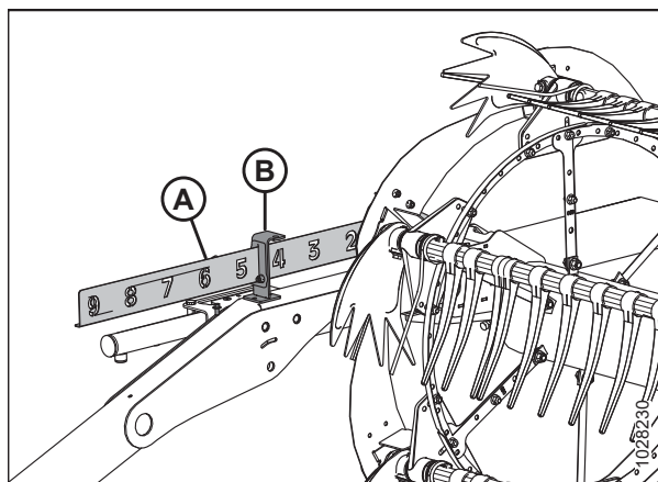
Attēls 3.209: Atgāzuma indikators
