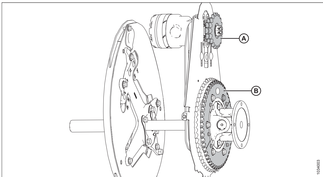
Attēls 3.197: Tītavu piedziņa ar papildu ķēdesratiem
