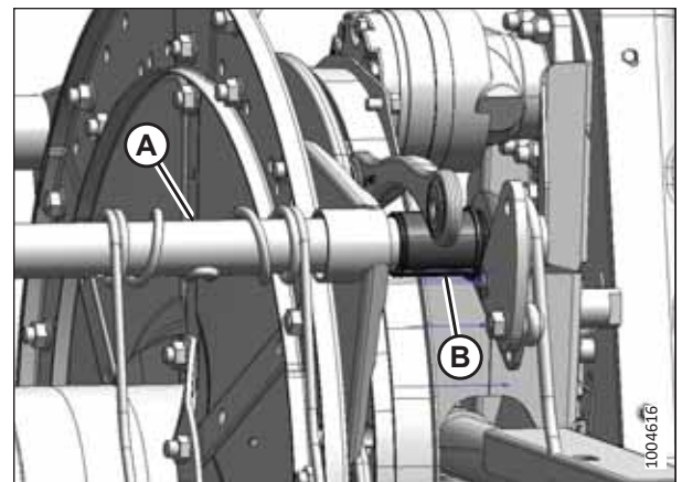
Attēls 4.284: Izcilņa gals
