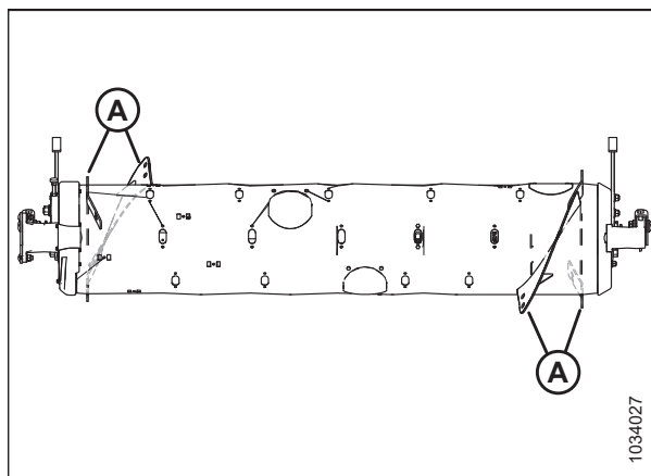
Attēls 3.91: Īpaši plata konfigurācija
