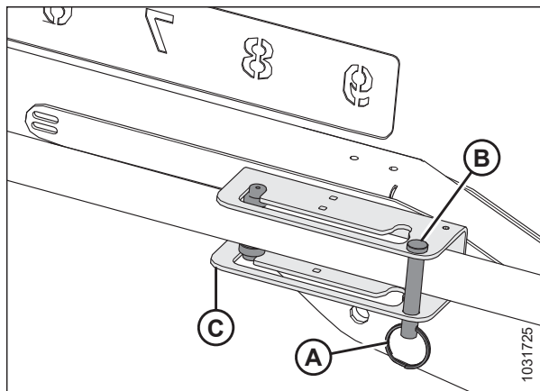
Attēls 3.215: Atgāzuma cilindra regulēšanas 2. tips — pozīcija uz priekšu
