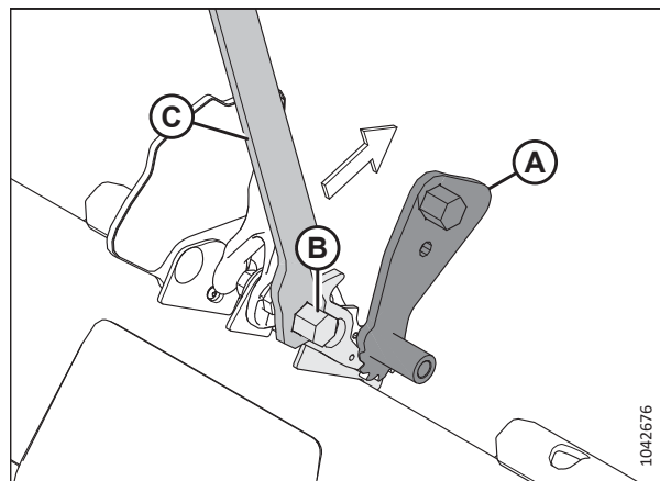
Attēls 3.169: Universālais darbarīks, kas aktivizēts ar kreiso sprūdu
