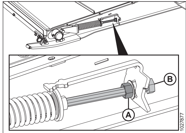
Attēls 4.177: Padeves stiebru pacēlāja spriegotājs
