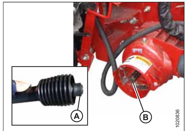
Attēls 3.68: Kombaina izvades vārpsta
