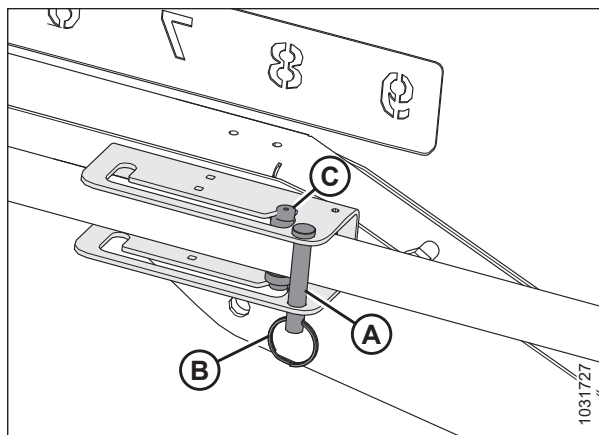
Attēls 3.217: Atgāzuma cilindra regulēšanas 2. tips — pozīcija uz aizmuguri
