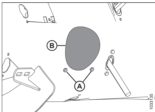
Attēls 3.132: Gliemežtransportiera piekļuves atveres pārsegs
