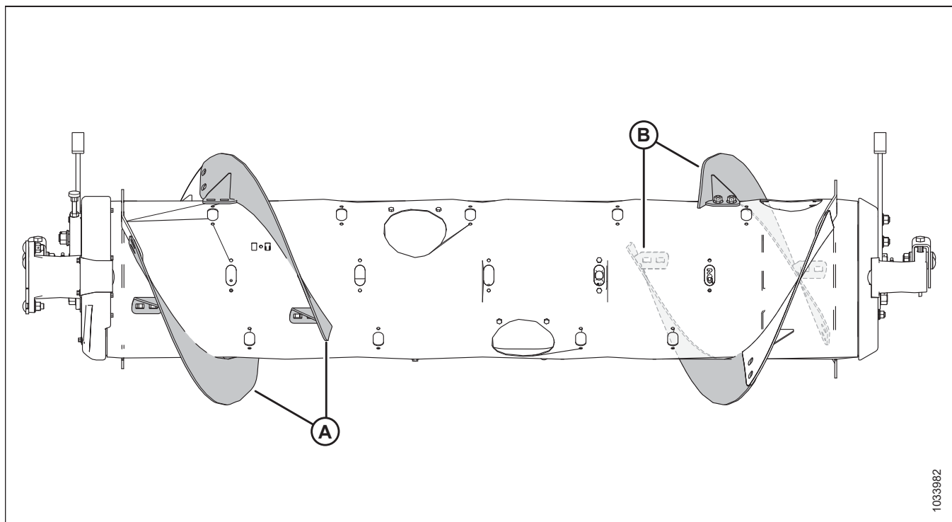
Attēls 3.88: Šaura konfigurācija
