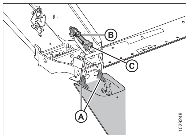
Attēls 3.241: Kultūraugu dalītājs ar aizdaru
