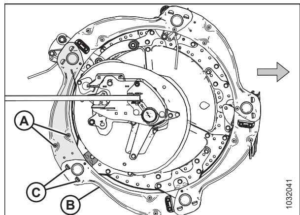
Attēls 4.296: Tītavu gala vairogis — ārējais izciļņa gals
