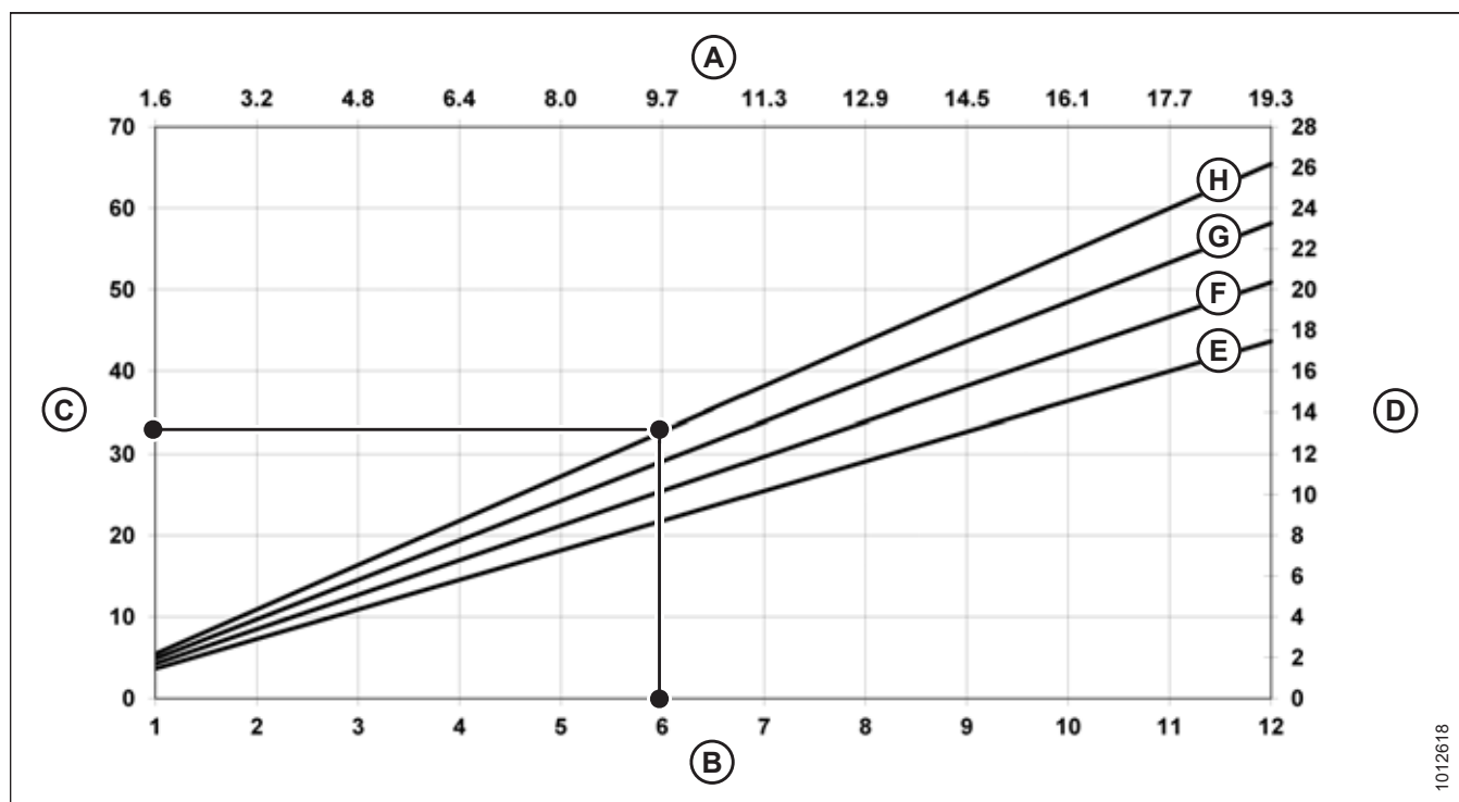
Attēls 3.198: Zemes ātrums un platība akros
