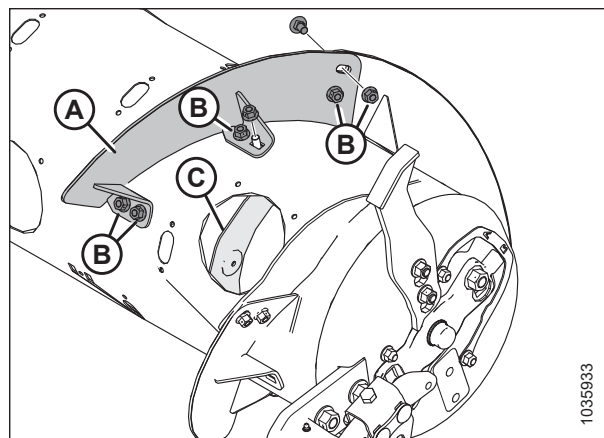
Attēls 3.106: Īsa spirālveida lāpstiņa — labā puse
