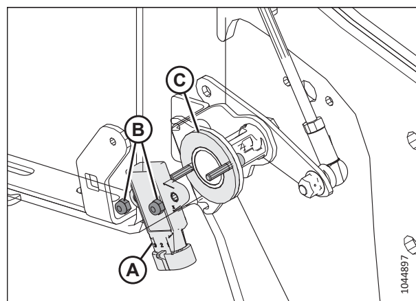
Attēls 3.206: Tītavu augstuma sensors — labās puses tītavu svira
