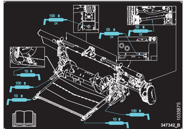
Attēls 4.21: FM200 eļļošanas punktu izkārtojuma uzlīme
