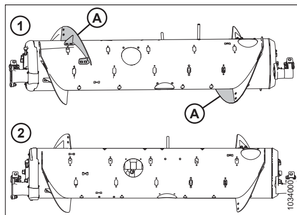
Attēls 3.99: Gliemežtransportiera konfigurācijas — skats no aizmugures
