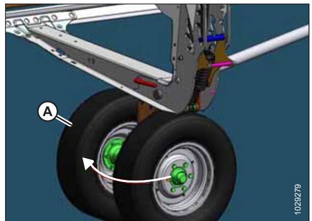
Attēls 3.365: Priekšējie transportēšanas riteņi
