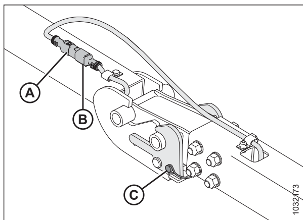
Attēls 3.338: Jūgstieņa / pagarinājuma stiprinājums
