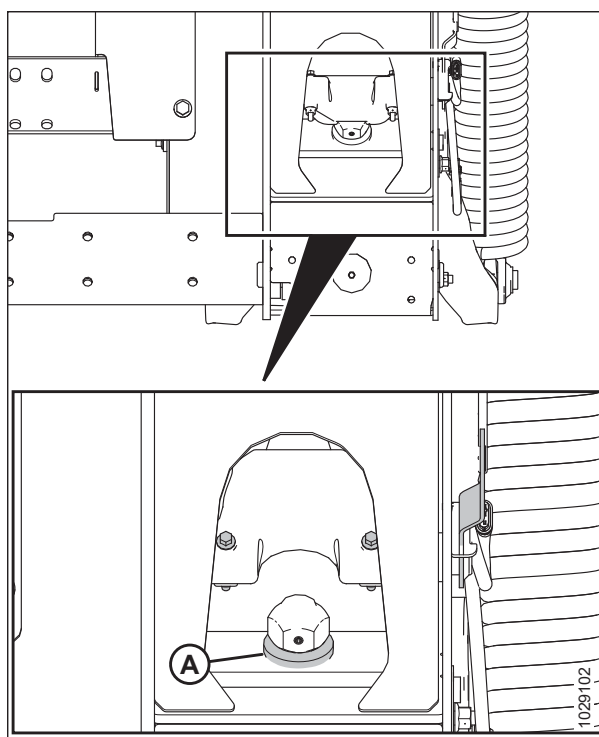
Attēls 3.272: Paplāksne aizturēm uz leju
