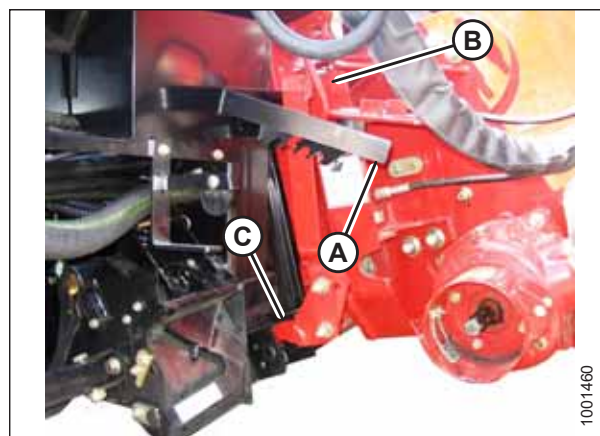
Attēls 3.77: Padeves tvertnes bloķētāji
