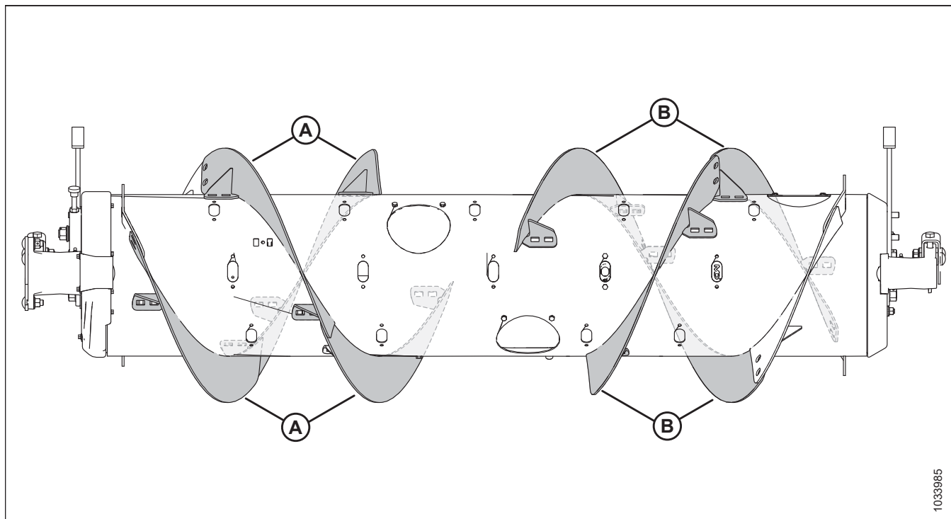
Attēls 3.83: Īpaši šaura konfigurācija
