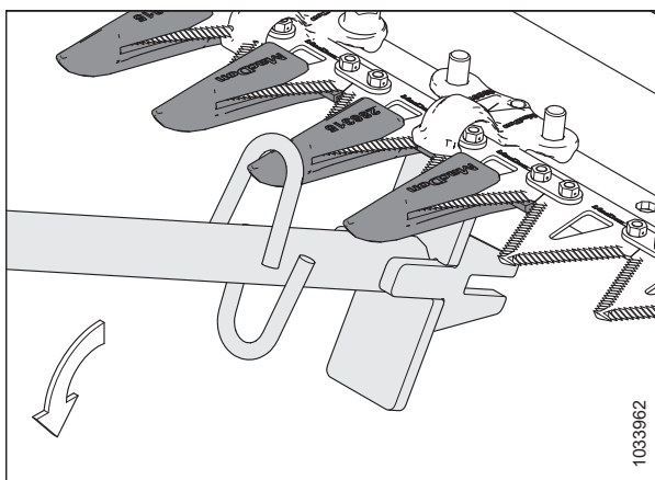
Attēls 4.120: Regulēšana uz leju — smails aizsargs
