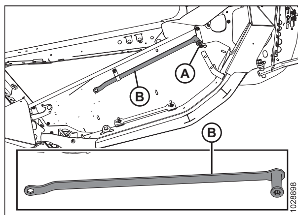
Attēls 3.189: Kreisais gala vairogs
