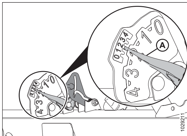
Attēls 3.157: Pļaušana pie zemes
