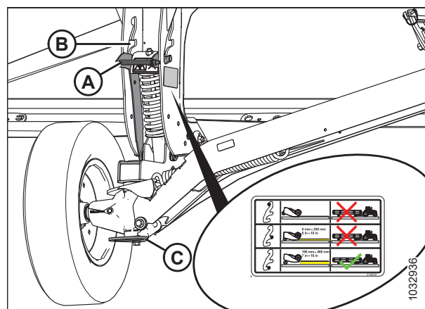
Attēls 3.140: Labais ritenis
