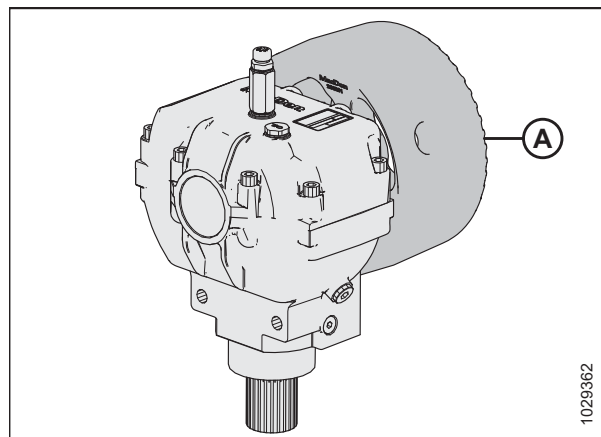
Attēls 3.203: Spararats
