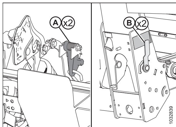
Attēls 3.190: Kontrolierīces plāksnes mezgls
