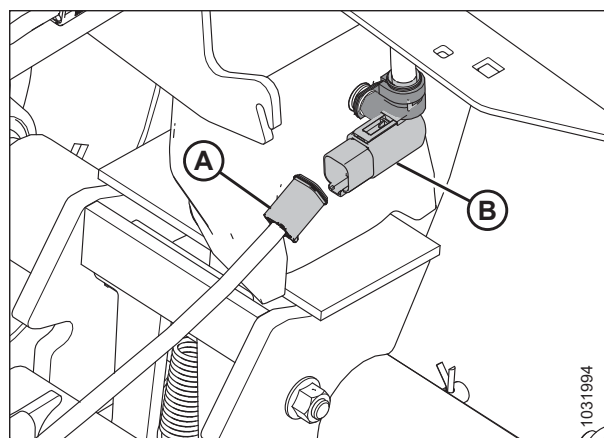
Attēls 3.380: Jūgstieņa elektriskais savienojums
