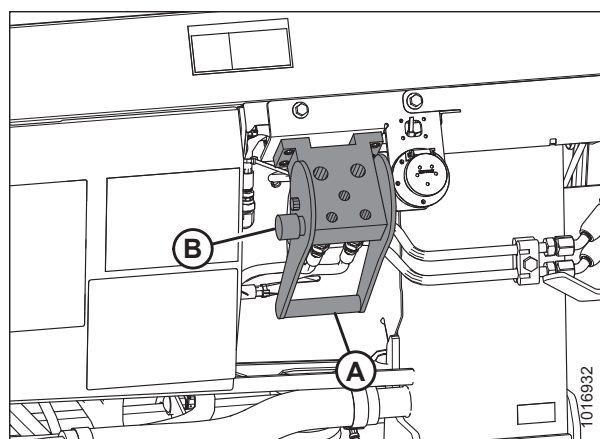
Attēls 3.76: Reljefa kopēšanas moduļa kontaktligzda
