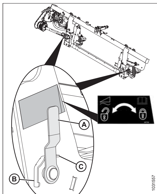
Attēls 3.171: Reljefa kopēšanas bloķējums — bloķētā stāvoklī
