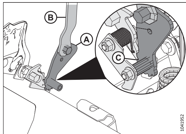
Attēls 3.164: Universālais darbarīks, kas savienots ar kreisās puses reljefa kopēšanas moduļa iestatīšanas mezglu
