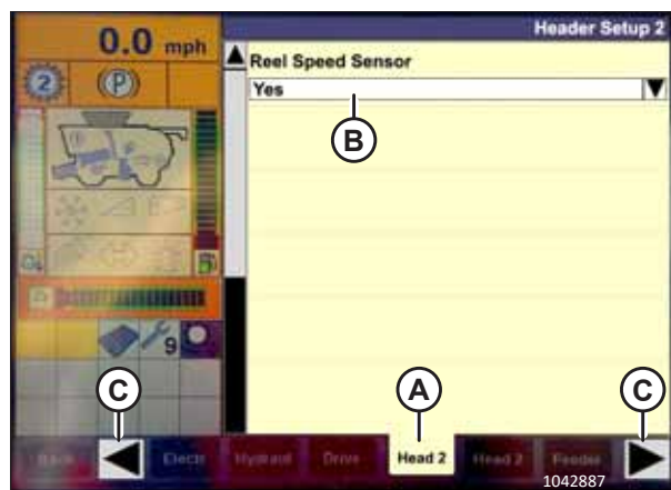
Attēls 3.332: Case IH kombaina displejs
