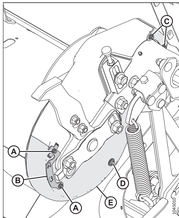
Attēls 4.76: Padeves gliemežtransportiera piedziņa — skats no priekšas
