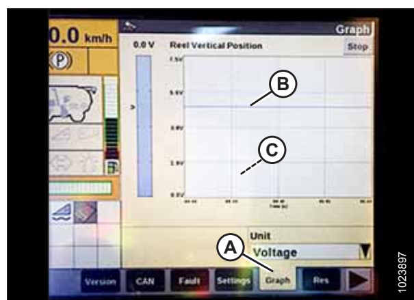
Attēls 3.328: Case IH kombaina displejs
