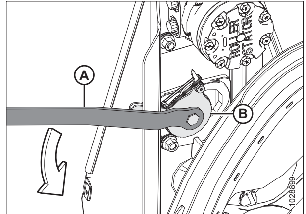
Attēls 4.319: Tītavu piedziņa
