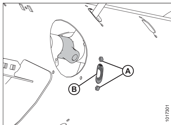
Attēls 3.130: Gliemežtransportiera pirksta caurums
