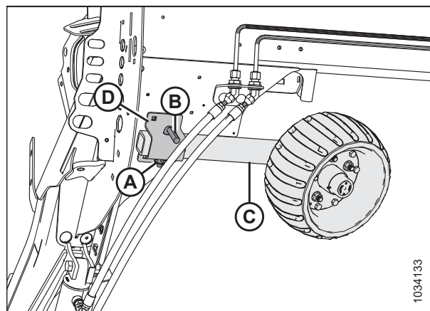
Attēls 3.361: Kreisā riteņa komplekts
