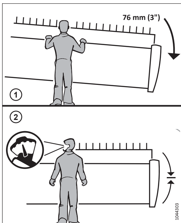
Attēls 3.167: Reljefa kopēšanas pārbaude
