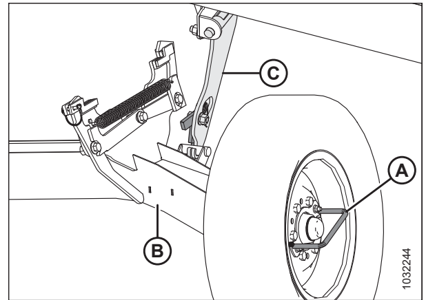
Attēls 3.368: Lauka balsts labajā pusē
