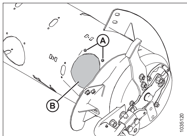
Attēls 3.111: Gliemežtransportiera piekļuves pārsegs — labā puse
