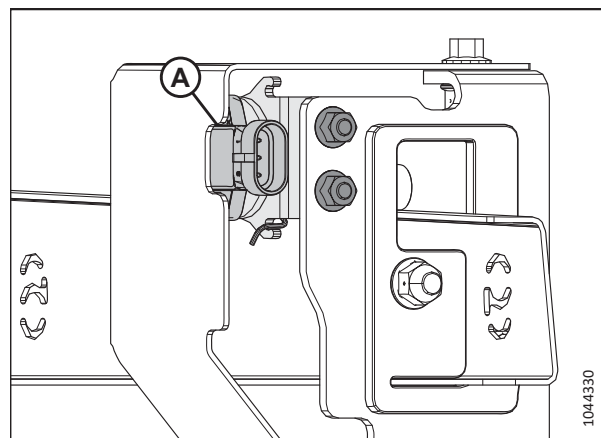
Attēls 3.218: Atgāzuma sensors
