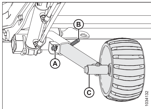
Attēls 3.335: Kreisā riteņa komplekts
