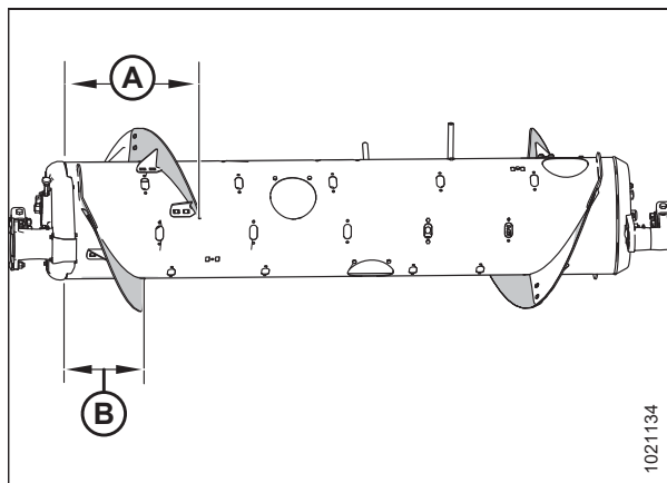
Attēls 3.80: Vidēja konfigurācija — skats no aizmugures
