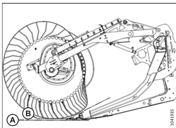
Attēls 3.224: Pirksta profils — izciļņa 2. pozīcija
