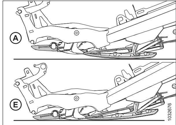
Attēls 3.152: Aizsargu leņķi
