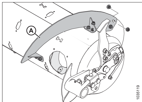
Attēls 3.115: Gara spirālveida lāpstiņa — labā puse
