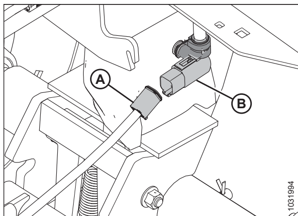
Attēls 3.343: Jūgstieņa elektriskais savienojums
