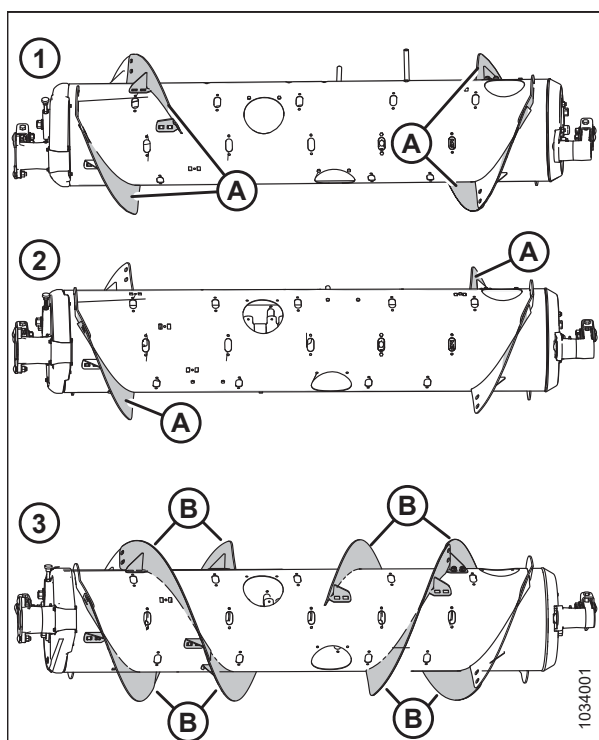
Attēls 3.85: Gliemežtransportiera konfigurācijas — skats no aizmugures
