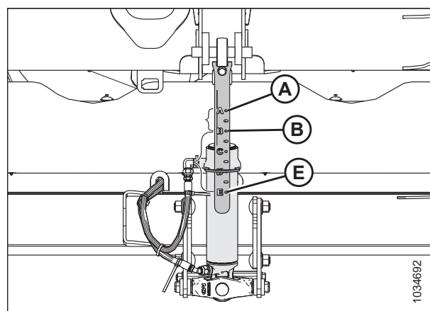
Attēls 3.142: Hedera leņķa indikators
