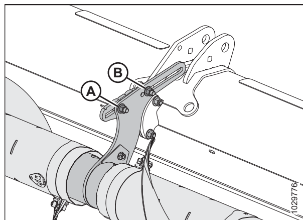
Attēls 3.234: Regulējamo stiprinājumu sākotnējā pozīcija — divdaļīgs gliemežtransportieris
