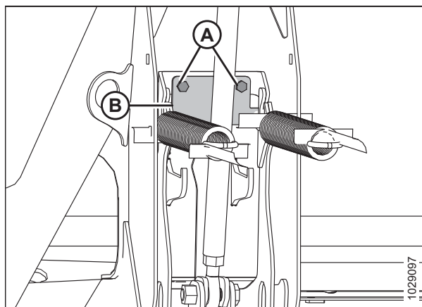
Attēls 3.182: Locīšanas izvērsuma ierobežotāja plāksne
