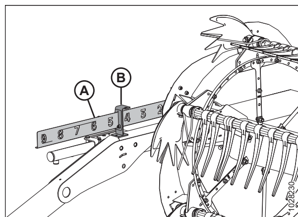
Attēls 3.208: Atgāzuma indikators
