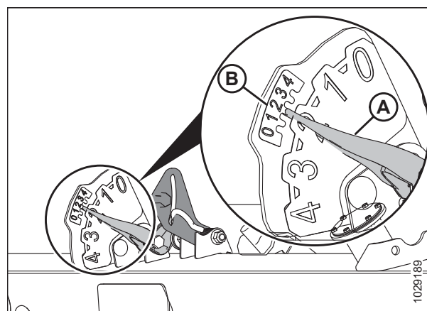
Attēls 3.165: Kreisās puses reljefa kopēšanas iestatījums un AHC indikators
