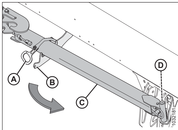
Attēls 3.371: Jūgstieņa pagarinājums uzglabāšanā
