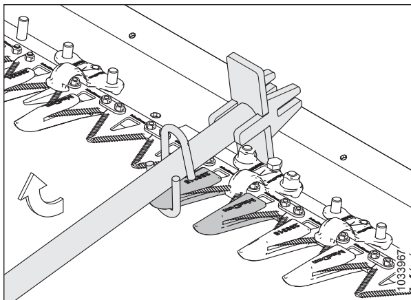
Attēls 4.118: Regulēšana uz augšu — smails aizsargs
