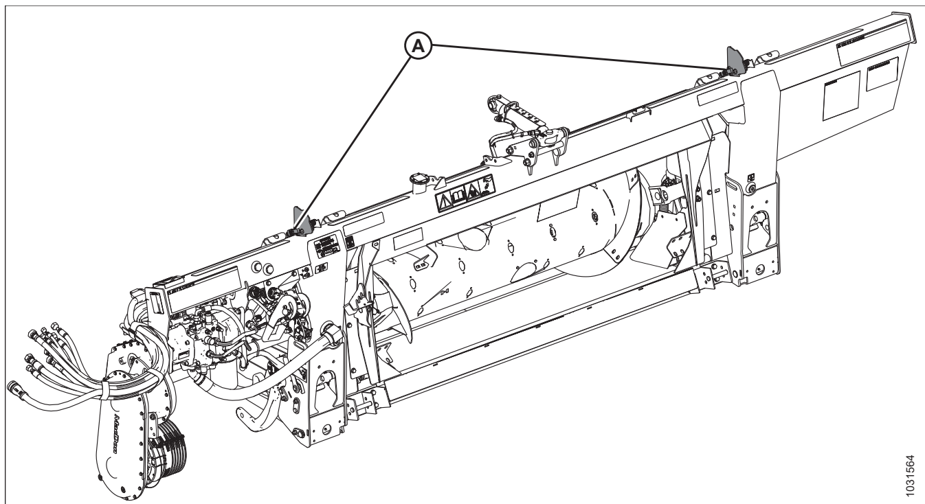
Attēls 3.263: FM200 reljefa kopēšanas modulis
