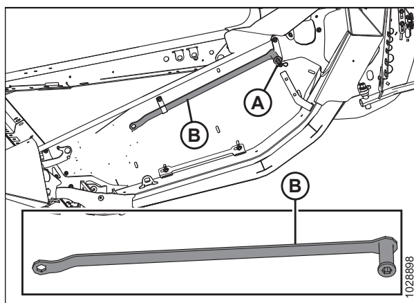
Attēls 3.196: Universālais darbarīks
