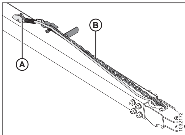
Attēls 3.337: Jūgstieņa uzstādīšana
