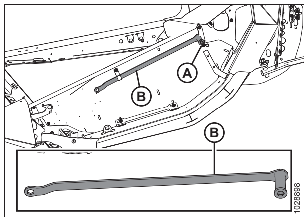
Attēls 3.163: Universālā darbarīka atrašanās vieta
