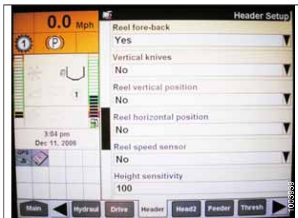
Attēls 3.306: Case IH kombaina displejs
