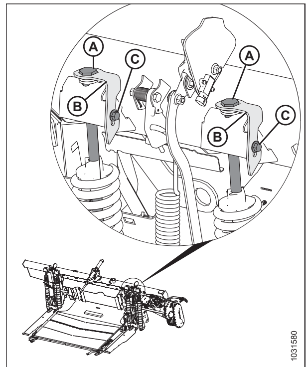
Фигура 3.170: Регулиране на плаващото положение отляво
