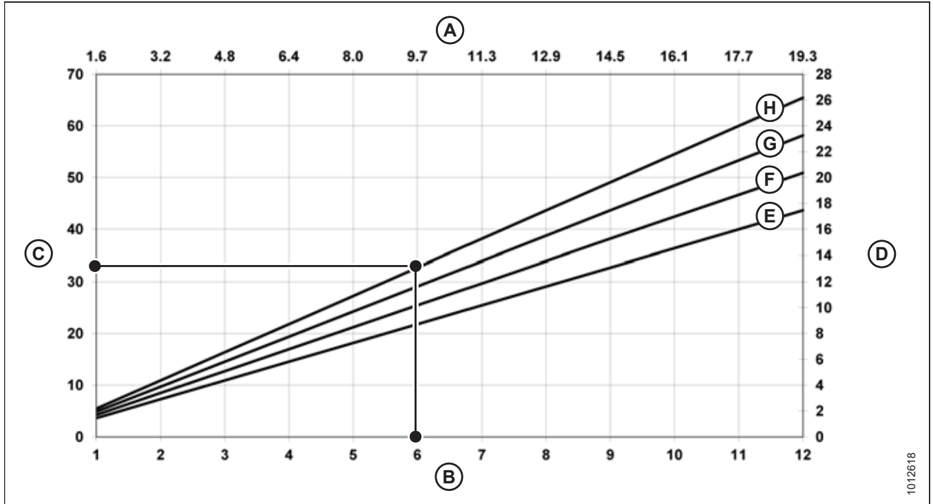
Фигура 3.202: Скорост на движение спрямо акри
