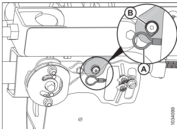
Фигура 3.180: Ключалка на жилото на контролното устройство на гъвкавата връзка – лява страна
