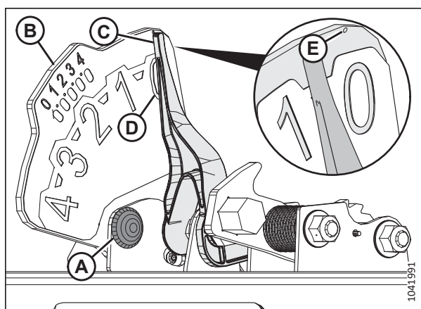
Фигура 3.165: Индикатор за плаващо положение
