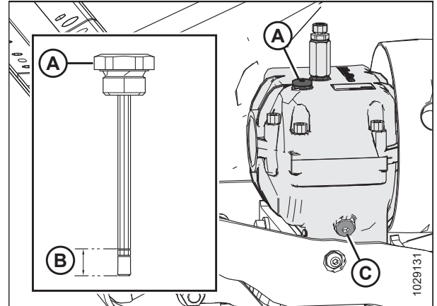
Фигура 4.159: Кутия за задвижване на ножовете
