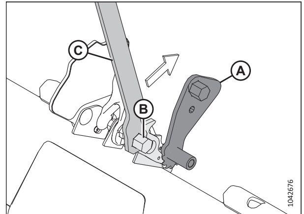
Фигура 3.173: Многофункционален инструмент, зацепен с ляв палец
