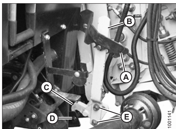
Фигура 3.61: Ключалки на подаващата камера
