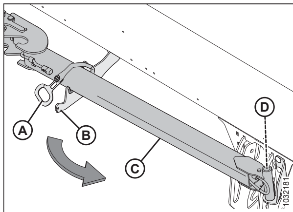
Фигура 3.376: Удължител на теглича в положение за съхранение
