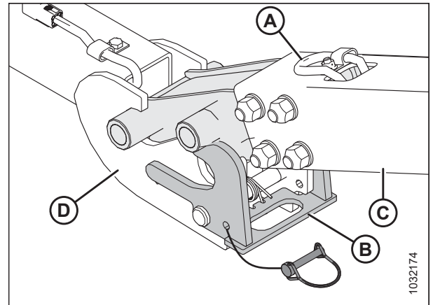
Фигура 3.344: Съединение теглич/удължител
