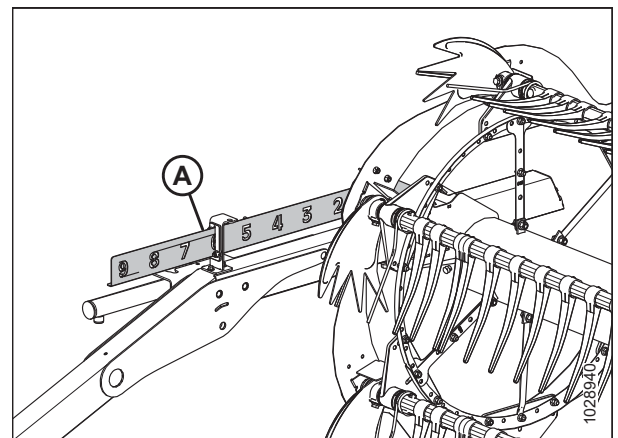
Фигура 3.163: Надлъжно положение
