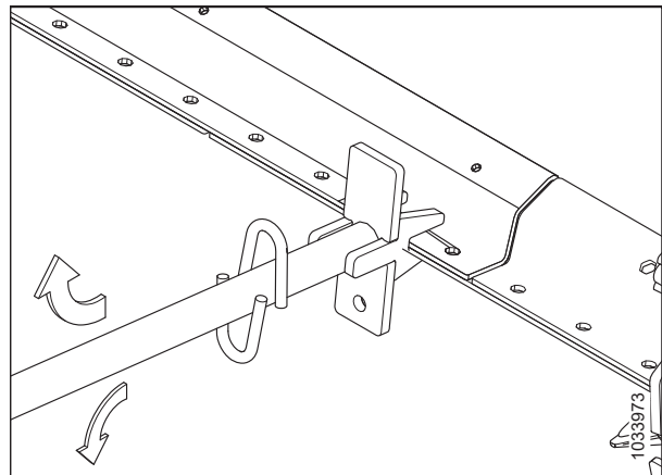
Фигура 4.122: Регулиране на гредата на предпазителите – без предпазители
