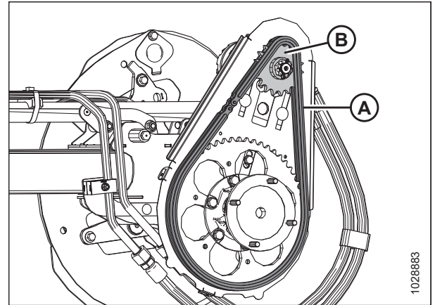
Фигура 4.325: Единично верижно зъбно колело
