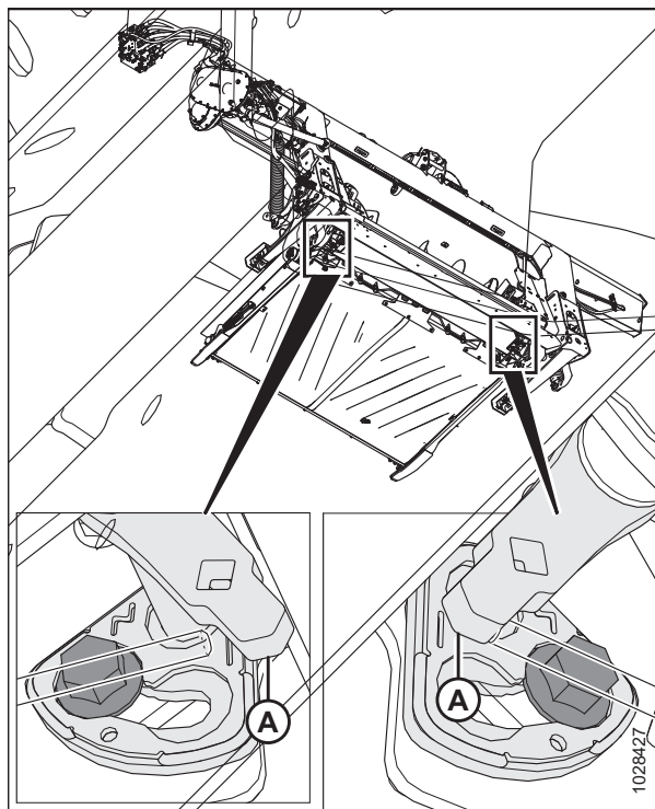
Фигура 3.137: Рамена за регулиране на плаващото положение на шнека
