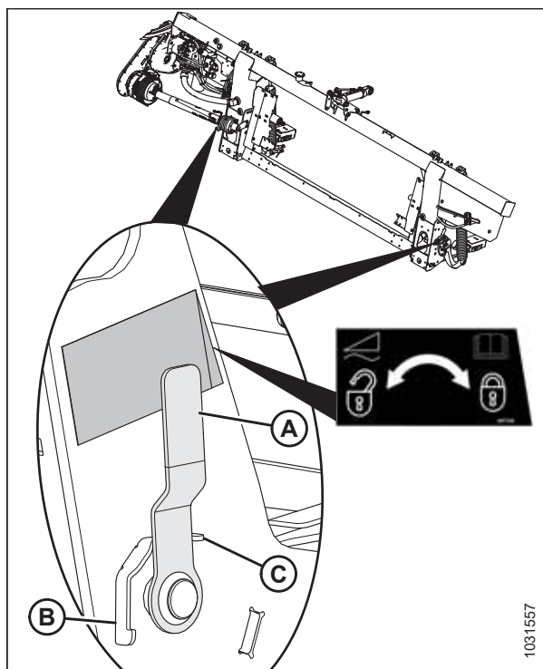
Фигура 3.175: Ключалка на плаващото положение – в заключено положение
