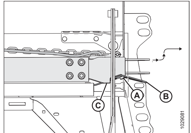
Фигура 3.377: Теглич в положение за съхранение
