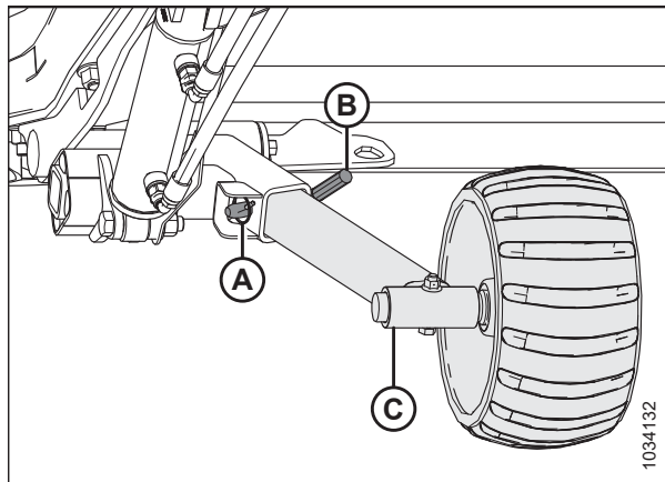
Фигура 3.365: Възел на лявото колело
