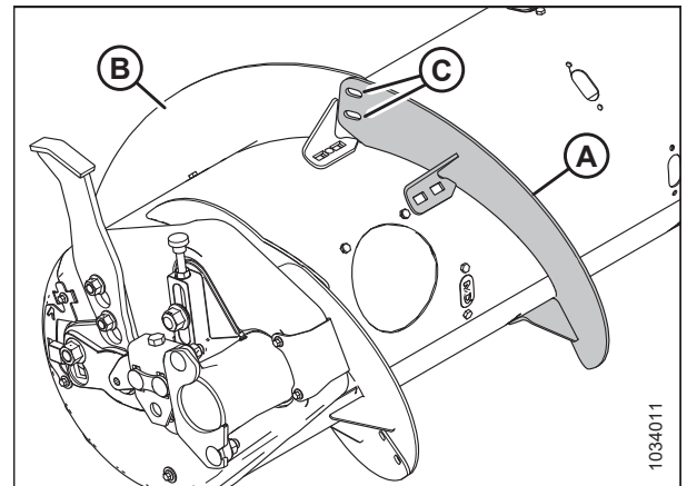
Фигура 3.123: Лява страна на шнека
