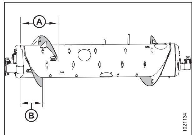
Фигура 3.84: Средна конфигурация – изглед отзад
