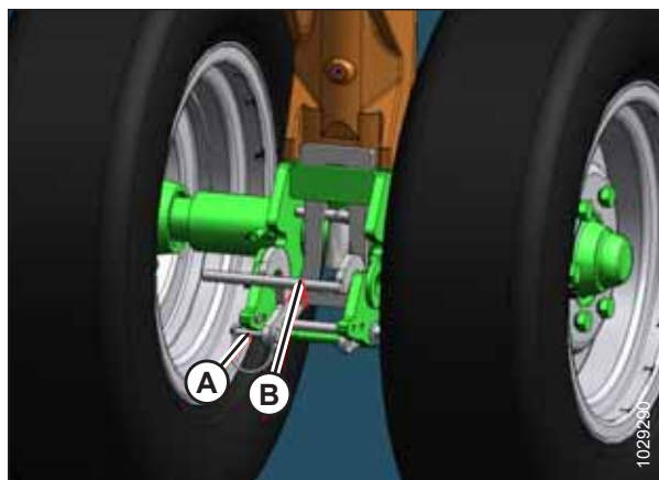
Фигура 3.369: Предни транспортни колела
