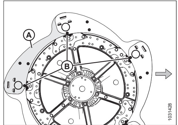
Фигура 4.299: Крайни щитове на мотовилото – вътрешен край с ексцентрик
