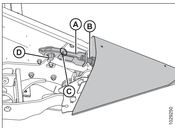
Фигура 3.247: Разделител на култура с ключалка
