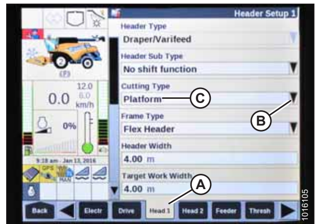
Фигура 3.304: Дисплей на комбайн New Holland
