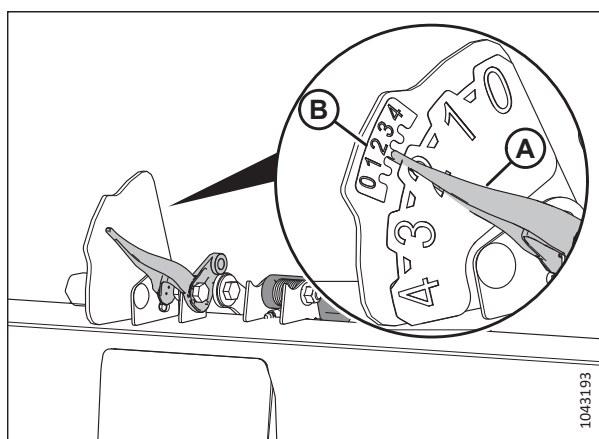
Фигура 3.152: Автоматичен индикатор за височината на хедера
