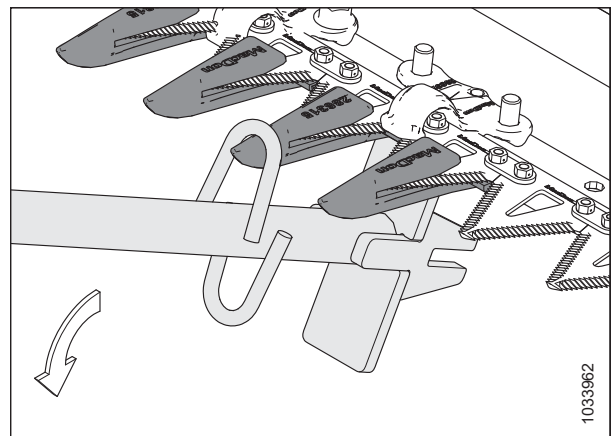
Фигура 4.120: Регулиране надолу – заострен предпазител
