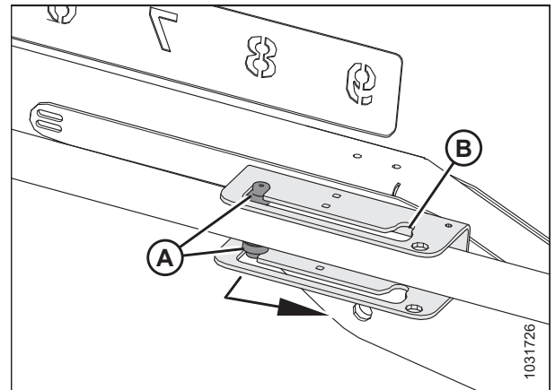
Фигура 3.220: Регулиране на цилиндър за надлъжно положение тип 2 – предно положение
