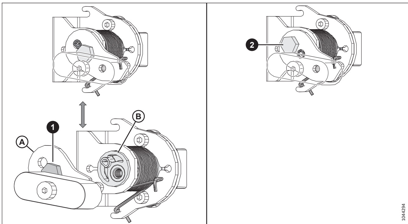
Фигура 3.226: Положение на рамото на датчика
