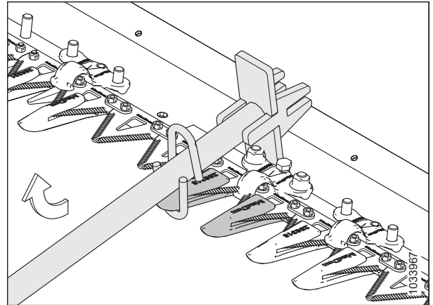
Фигура 4.118: Регулиране нагоре – заострен предпазител
