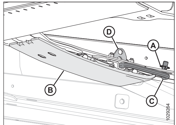
Фигура 3.153: Вътрешна опорна пета
