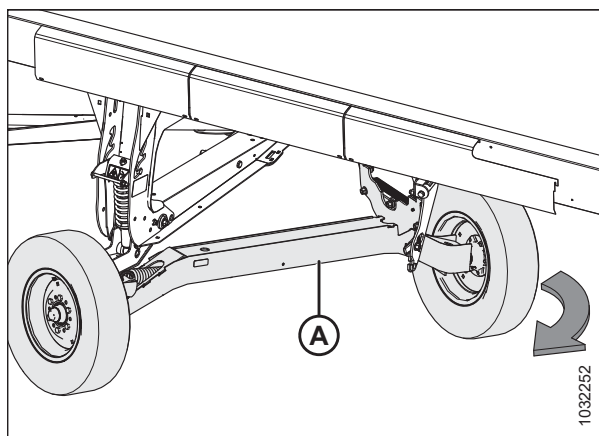
Фигура 3.362: Завъртане на дясната транспортна ос
