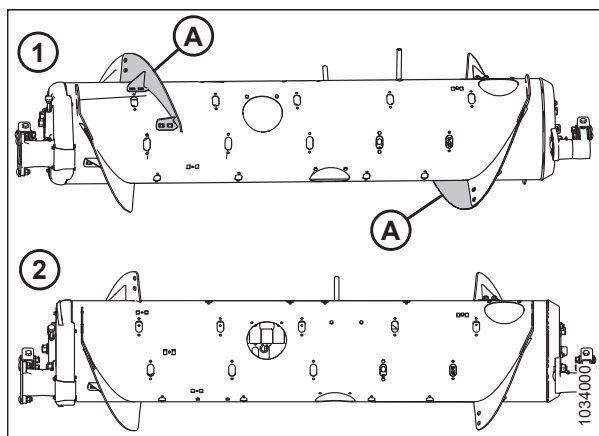
Фигура 3.103: Шнекови конфигурации – изглед отзад
