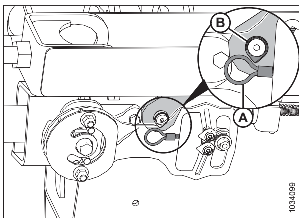
Фигура 3.199: Лева ключалка на жилото на контролното устройство на гъвкавата връзка
