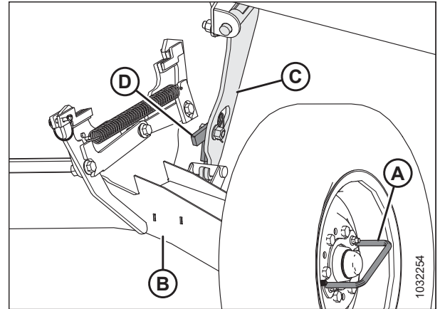
Фигура 3.363: Дясна транспортна ос, заключена в полево положение
