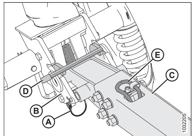
Фигура 3.384: Теглич и лев транспортен шарнир
