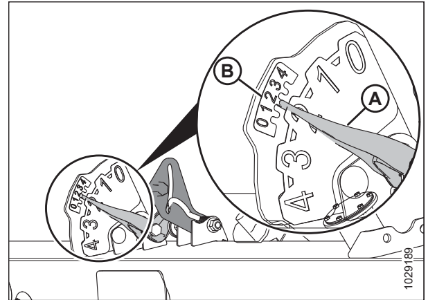
Фигура 3.169: Настройка на плаващото движение отляво и индикатор за АННС
