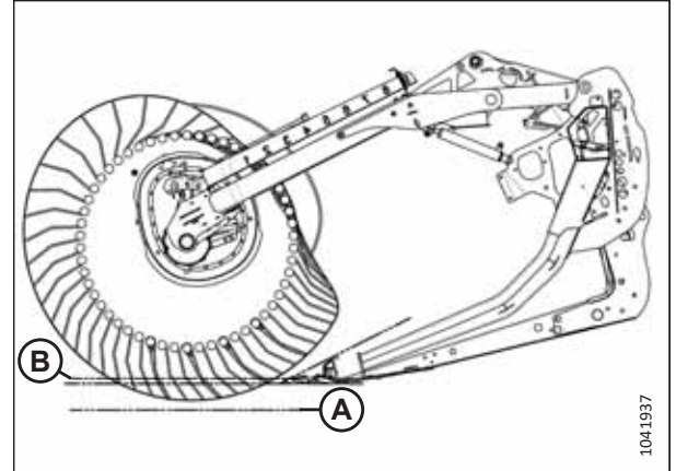
Фигура 3.231: Профил на зъбите – положение на ексцентрика 4, максимален ъгъл на хедера
