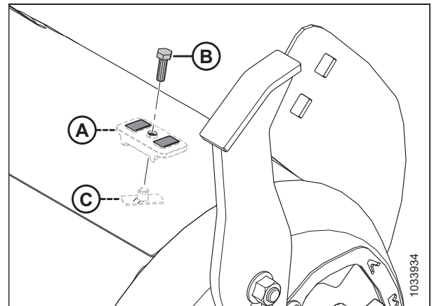
Фигура 3.112: Монтиране на тапи за слотове
