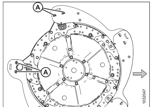
Фигура 4.301: Отстранен краен щит на мотовилото – вътрешен край с ексцентрик
