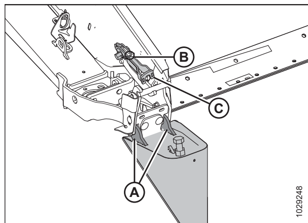
Фигура 3.245: Разделител на култура с ключалка
