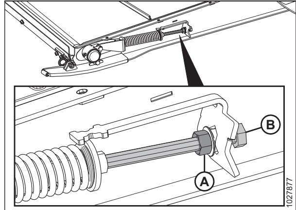
Фигура 4.182: Обтегач на подаващата лента
