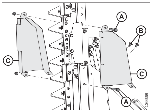
Фигура 4.374: Външни капаци на ножовата глава
