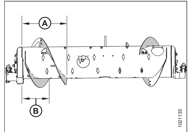
Фигура 3.83: Тясна конфигурация – изглед отзад
