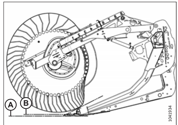
Фигура 3.227: Профил на зъба – положение на ексцентрика 1
