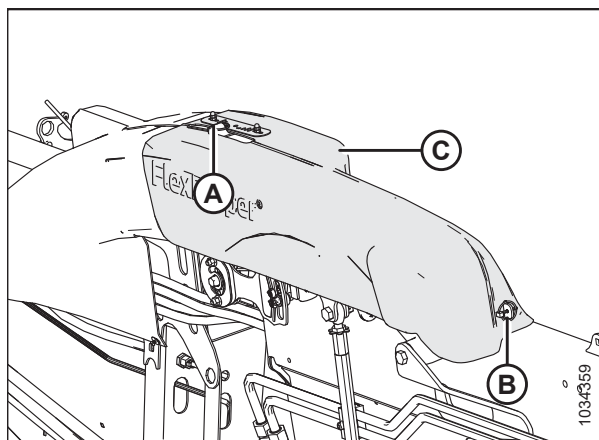
Фигура 3.32: Вътрешен капак на гъвката връзка – лява страна
