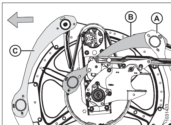
Фигура 4.308: Крайни щитове на мотовилото – вътрешен заден край
