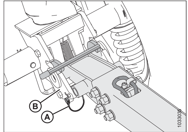
Фигура 3.349: Теглич и ляв транспортен шарнир
