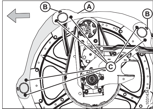
Фигура 4.312: Крайни щитове на мотовилото – вътрешен заден край
