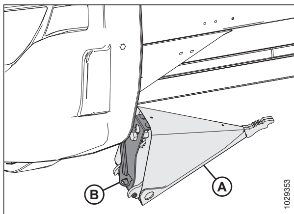
Фигура 3.243: Опционална конзола за съхранение на разделителя на култура
