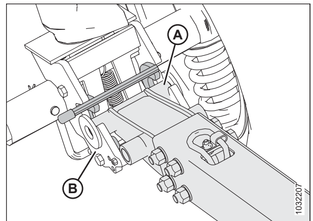
Фигура 3.350: Теглич и ляв транспортен шарнир
