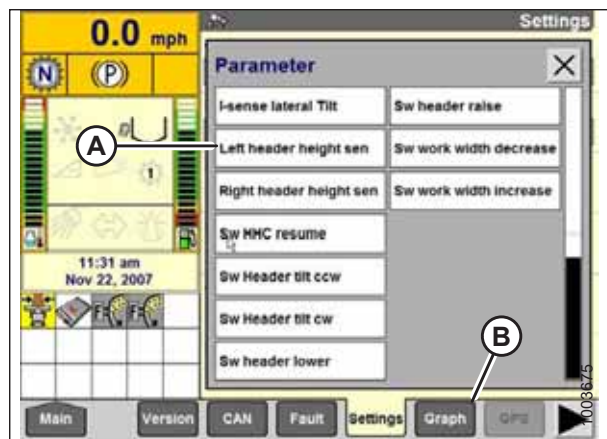
Фигура 3.282: Дисплей на комбайн New Holland
