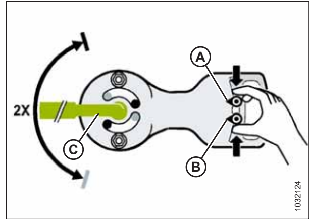
Фигура 3.196: Индикатори за баланс на лявото крило
