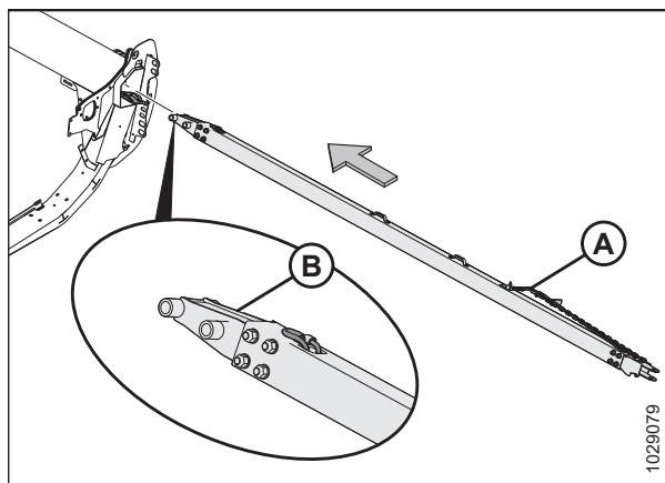
Фигура 3.353: Край на навесната система
