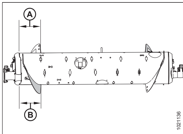
Фигура 3.85: Широка конфигурация – изглед отзад
