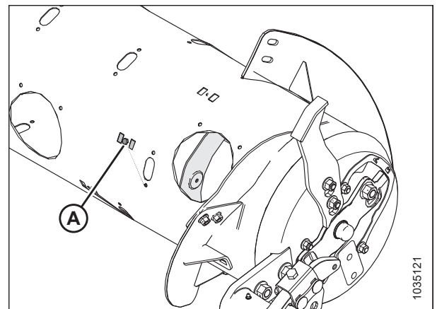
Фигура 3.117: Дясна страна на шнека
