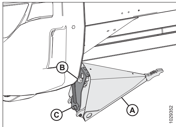
Фигура 3.244: Опционален разделител на култура
