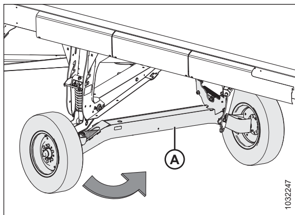
Фигура 3.374: Дясна транспортна ос
