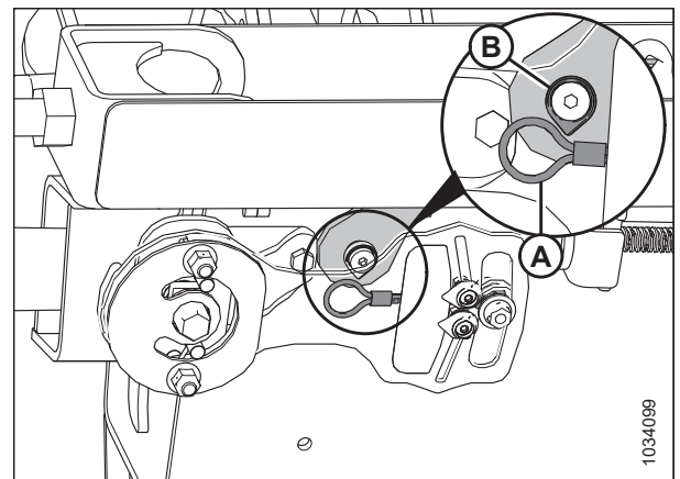
Фигура 3.178: Ключалка на жилото на контролното устройство на гъвкавата връзка – лява страна
