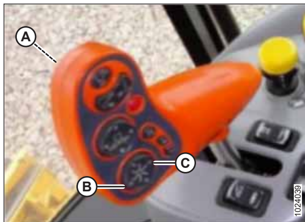
Фигура 3.158: Органи за управление при New Holland CR/CX
