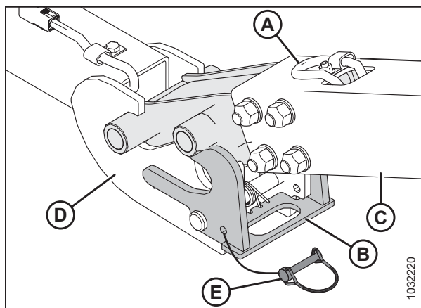
Фигура 3.381: Теглич към удължител
