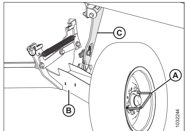
Фигура 3.373: Дясна полева опора
