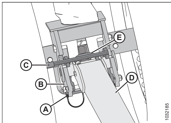
Фигура 3.379: Удължител на теглича към левия транспортен шарнир
