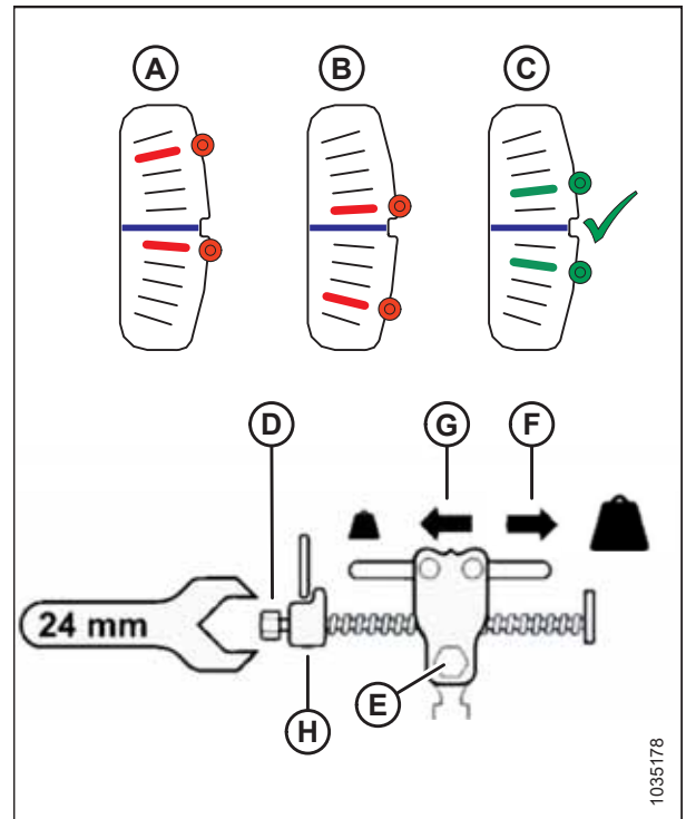
Фигура 3.197: Планка на контролното устройство за регулиране на баланса на лявото крило
