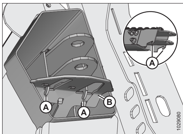
Фигура 3.354: Куки за задържане от страната на вилката
