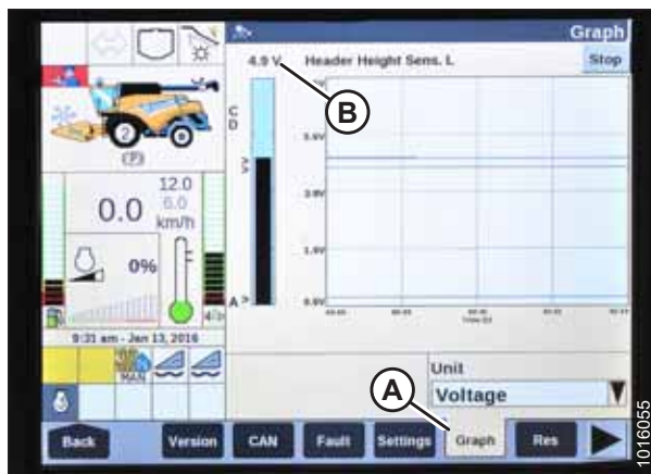
Фигура 3.302: Дисплей на комбайн New Holland
