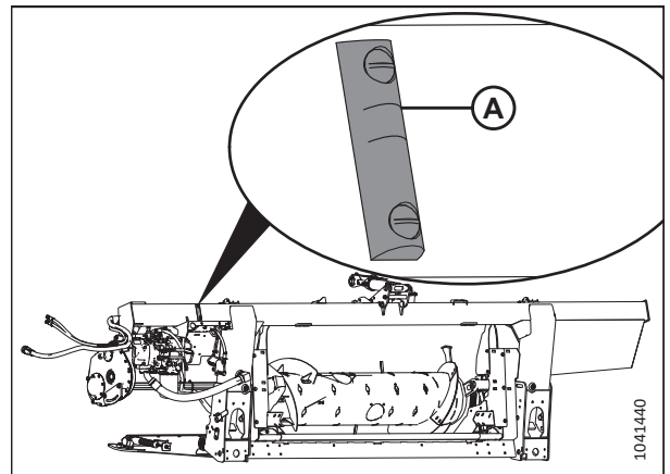
Фигура 4.33: Контролно прозорче за нивото на маслото
