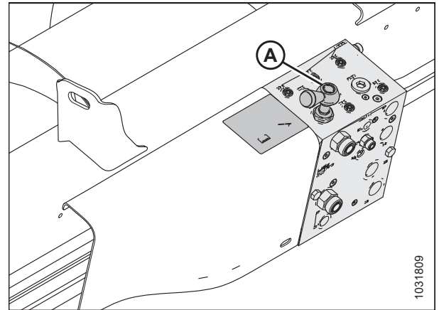
Фигура 3.234: Спирателен клапан
