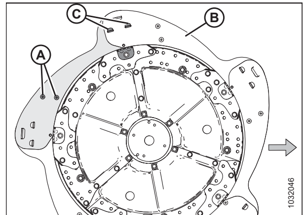
Фигура 4.300: Крайни щитове на мотовилото – вътрешен край с ексцентрик
