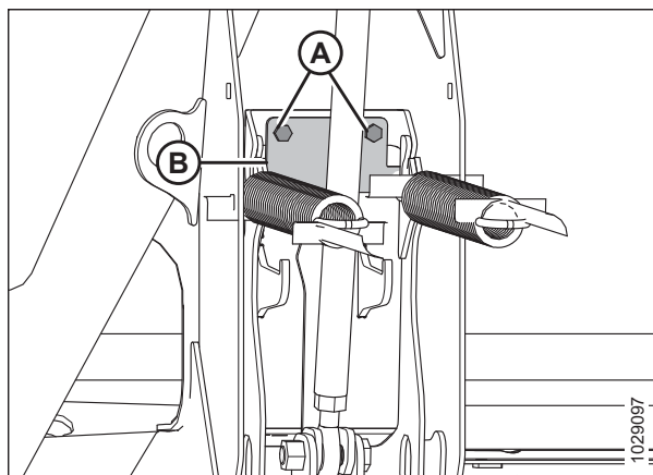
Фигура 3.186: Планка на ограничителя на огъването надолу
