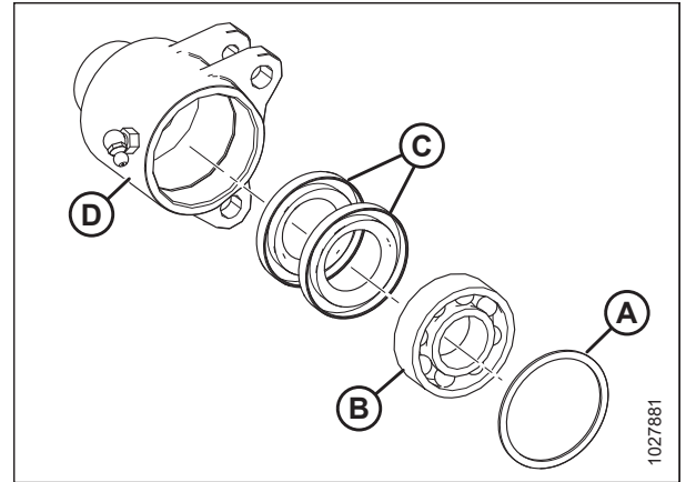
Фигура 4.200: Възел на лагера
