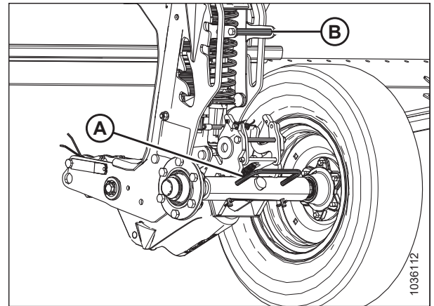
Фигура 3.359: Леви транспортни колела в най-високо положение за съхранение
