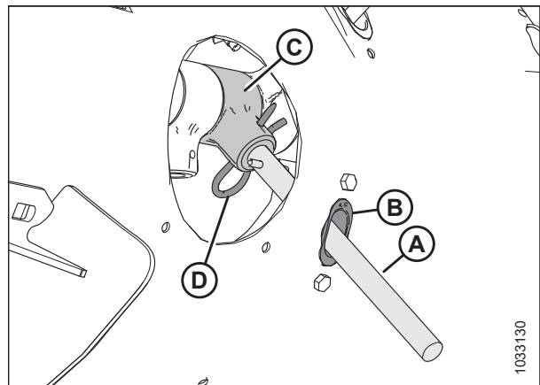
Фигура 3.135: Зъб на шнека
