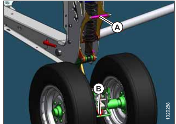
Фигура 3.367: Предни транспортни колела
