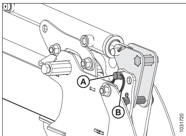
Фигура 3.218: Регулиране на цилиндър за надлъжно положение тип 1 – задно положение
