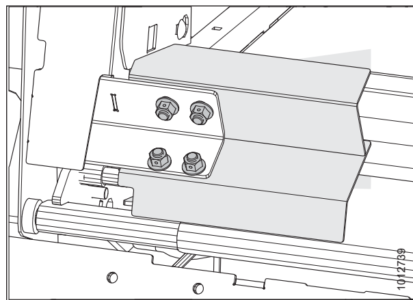
Фигура 5.19: Стрипер
