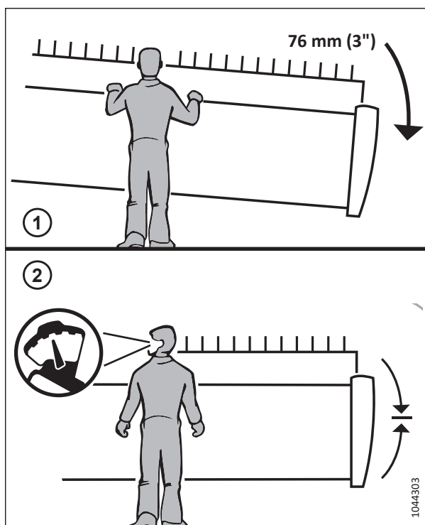
Фигура 3.171: Проверка на плаващото положение
