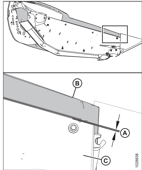
Фигура 3.15: Хлабина между крайния щит и страницата
