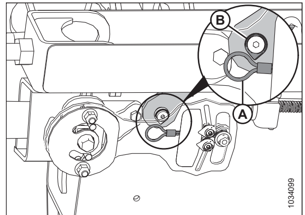
Фигура 3.192: Лева ключалка на жилото на контролното устройство на гъвкавата връзка
