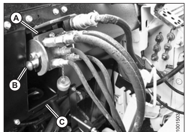
Фигура 3.74: Връзки на плаващия модул
