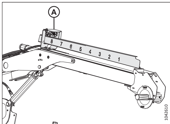
Фигура 3.225: Датчик за надлъжно положение
