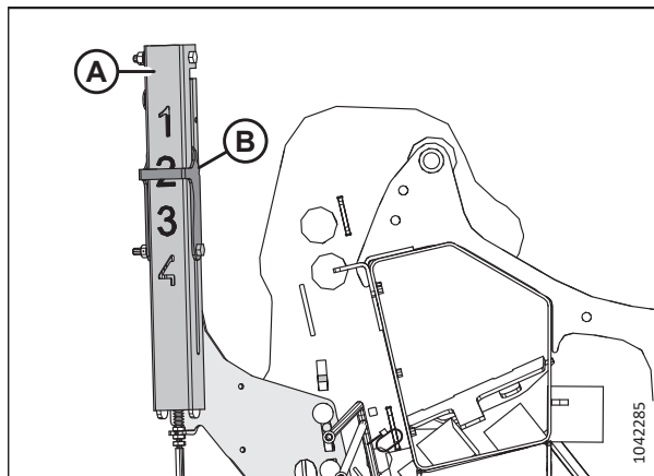
Фигура 3.148: Индикатор за височина – заден ляв край
