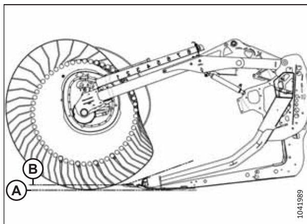
Фигура 3.230: Профил на зъбите – положение на ексцентрика 4, минимален ъгъл на хедера
