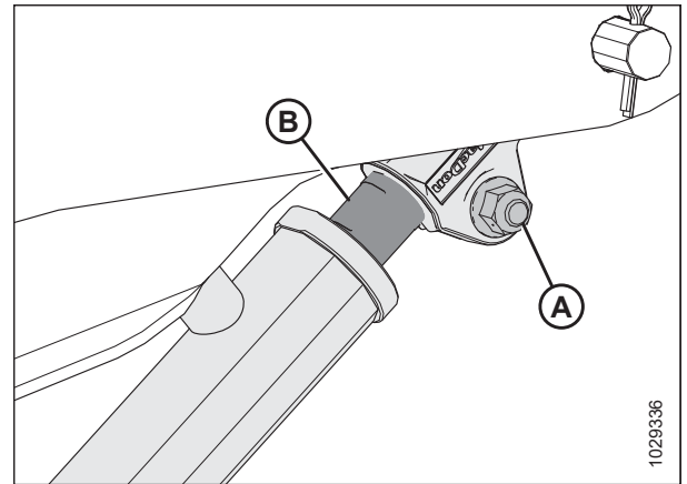
Фигура 4.265: Цилиндър на външното рамо
