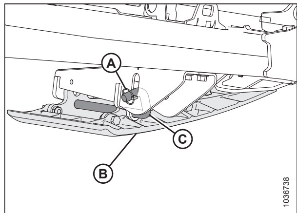
Фигура 3.154: Външна опорна пета
