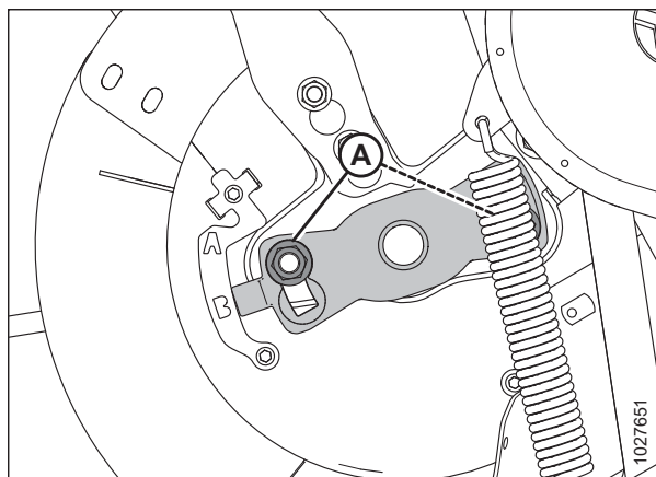
Фигура 4.100: Индикатор за синхронизация на зъбите на шнека
