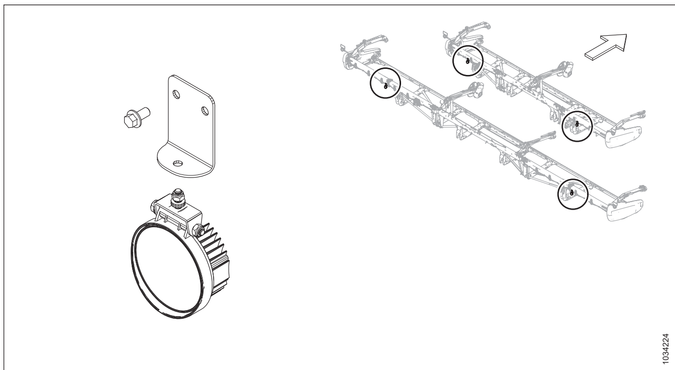
Фигура 5.29: Комплект светлини за стърнището
