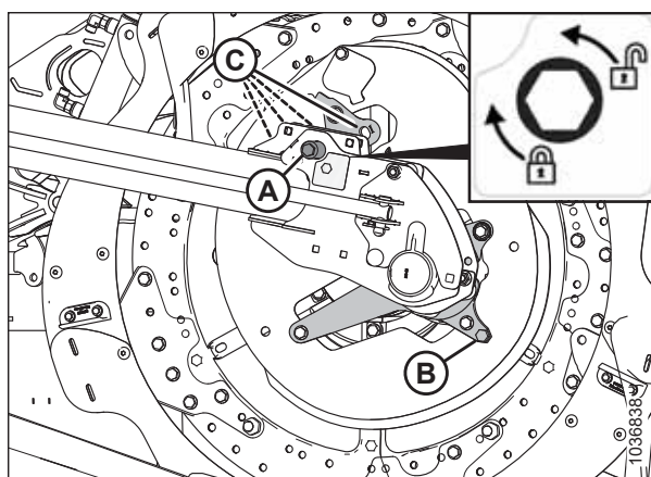
Фигура 3.233: Положения на диска на ексцентрика
