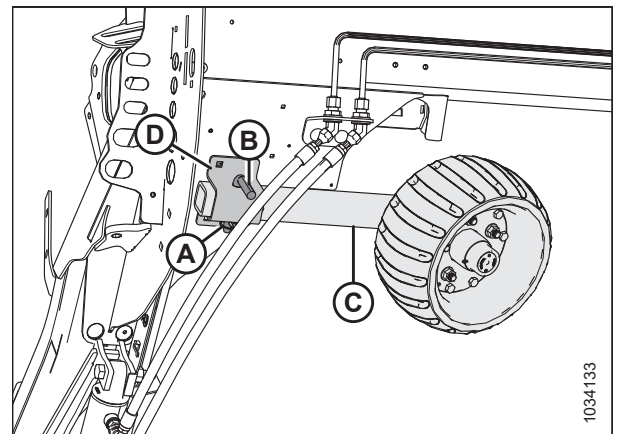
Фигура 3.339: Възел на лявото колело
