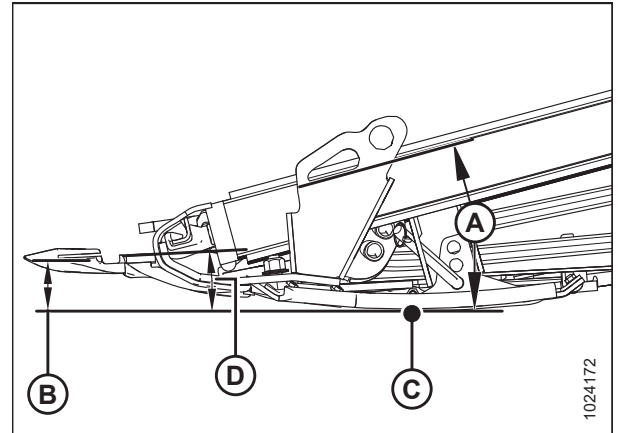
Фигура 3.155: Ъгъл на хедера
