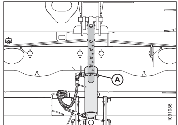
Фигура 3.274: Централна връзка
