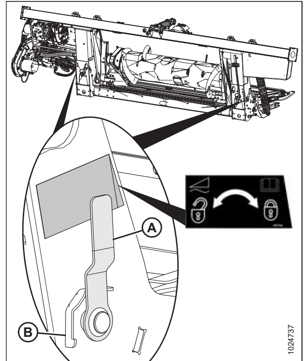
Фигура 3.166: Ключалка за плаващото положение на хедера в заключено положение
