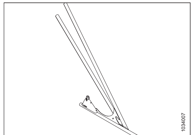
Фигура 3.265: Опционален прът на разделителя на ориз
