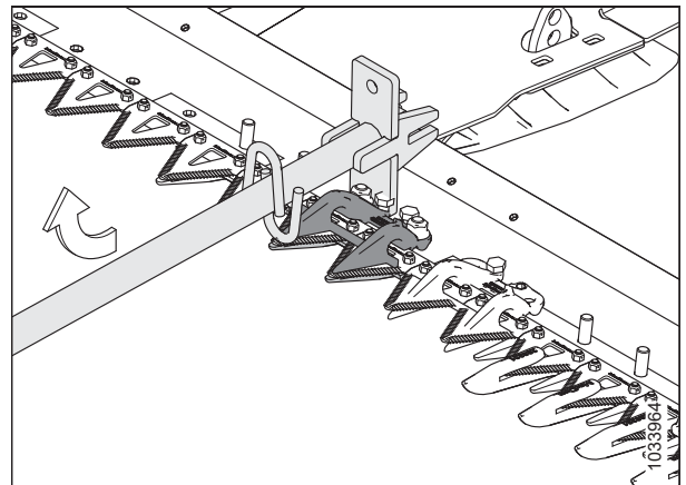
Фигура 4.119: Регулиране нагоре – къс предпазител за ножове
