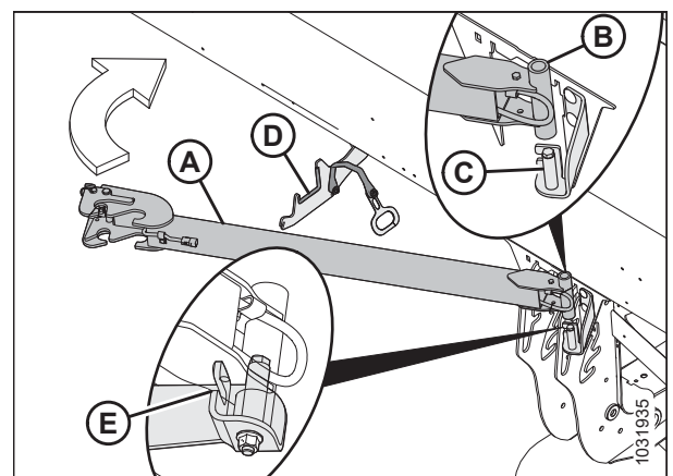
Фигура 3.351: Съхранение на удължителя на теглича
