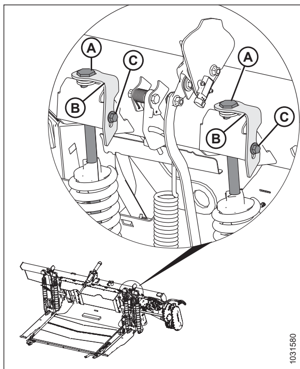
Фигура 3.172: Регулиране на плаващото положение отляво
