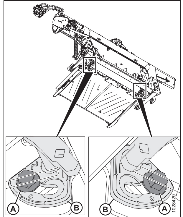
Фигура 3.139: Регулиране на плаващото положение на подаващия шнек
