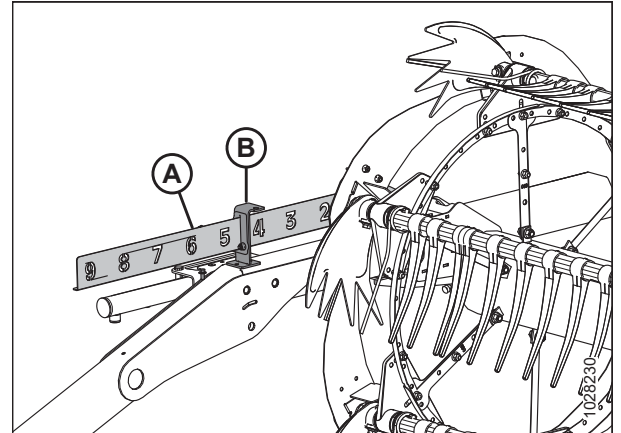
Фигура 3.213: Индикатор за надлъжно положение
