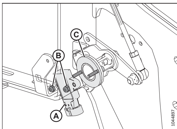
Фигура 3.210: Датчик за височината на мотовилото – дясно рамо на мотовилото
