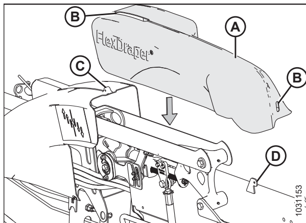
Фигура 3.31: Вътрешен капак на гъвката връзка – лява страна
