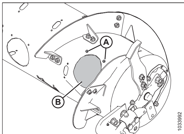
Фигура 3.109: Капак за достъп до шнека – дясна страна
