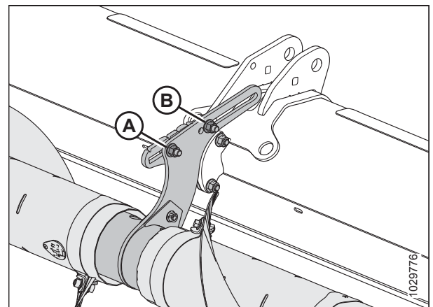
Фигура 3.238: Първоначално положение на регулируемите стойки – двукомпонентен шнек
