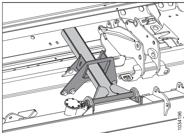
Фигура 5.26: Комплект за стабилизиране на страничен наклон
