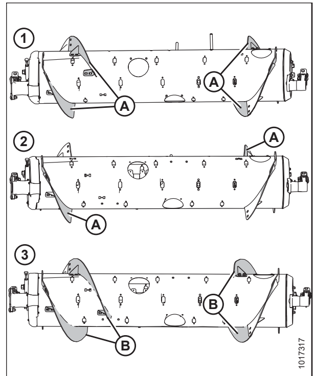
Фигура 3.94: Шнекови конфигурации – изглед отзад
