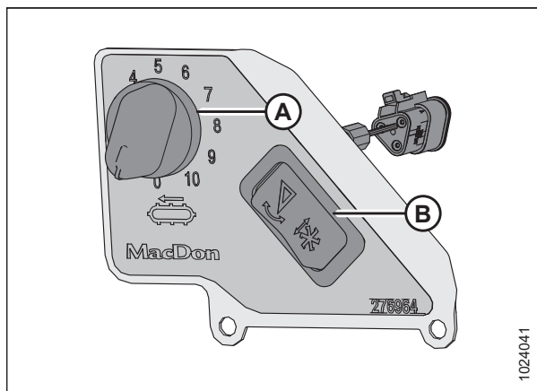
Фигура 3.204: Орган за управление на скоростта на страничните ленти от кабината
