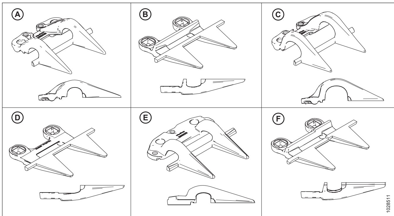
Фигура 4.137: Видове предпазители и държачи, използвани в конфигурации с къси предпазители на ножа
