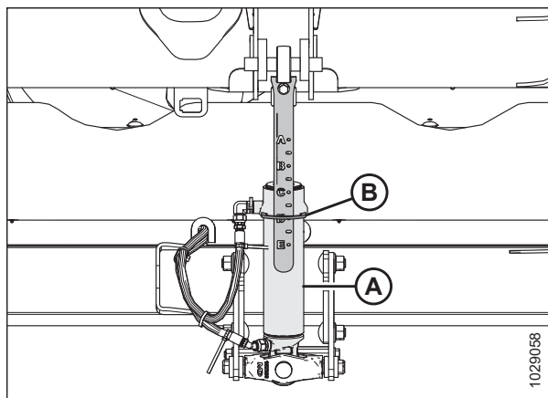
Фигура 3.164: Централна връзка
