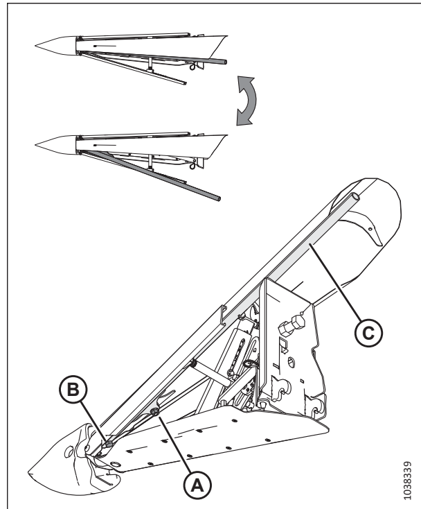
Фигура 3.259: Регулиране на страничния прът на горния дефлектор
