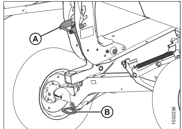
Фигура 3.371: Копирни колела
