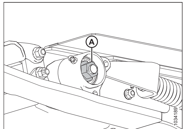
Фигура 4.202: Лагер на паразитната ролка – лява страна
