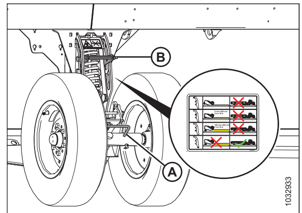
Фигура 3.145: Ляво колело
