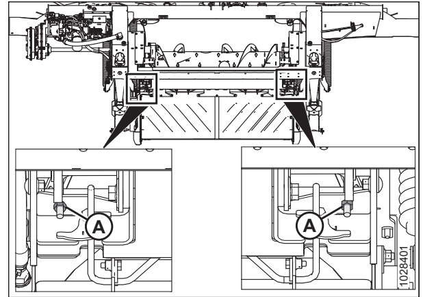
Фигура 3.141: Обтегач на пружината
