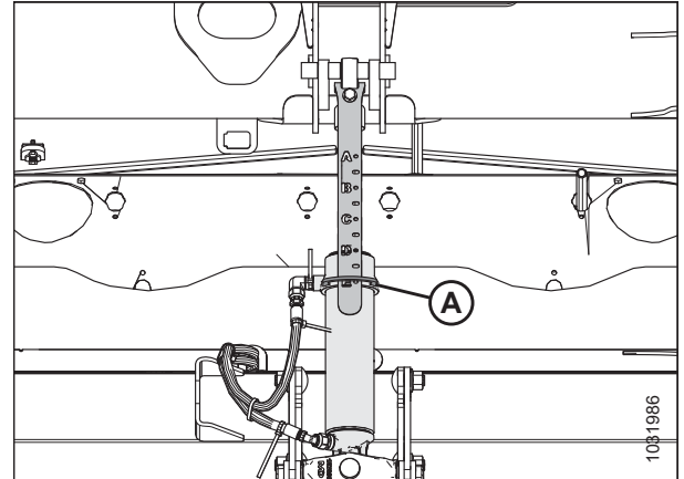
Фигура 3.269: Централна връзка
