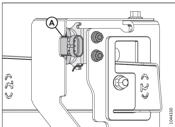
Фигура 3.222: Датчик за надлъжно положение
