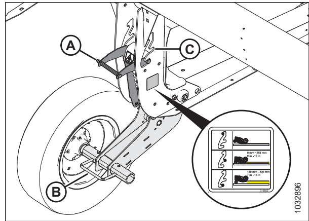
Фигура 3.143: Стабилизиращо колело
