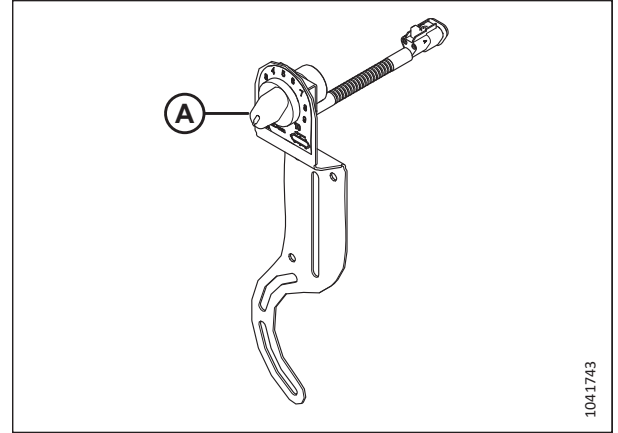
Фигура 3.205: Управление на скоростта на страничната лента от кабината при New Holland
