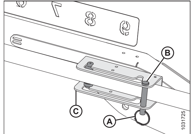
Фигура 3.219: Регулиране на цилиндър за надлъжно положение тип 2 – предно положение
