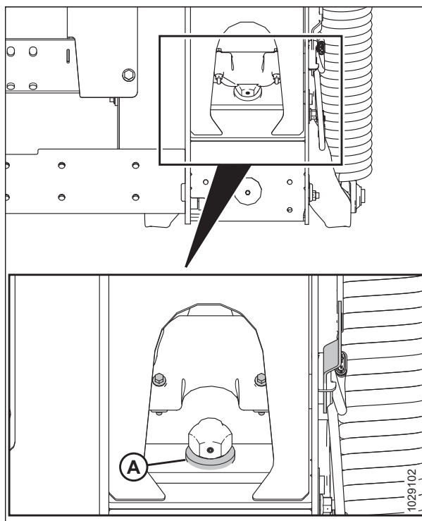
Фигура 3.277: Шайба на долния ограничител
