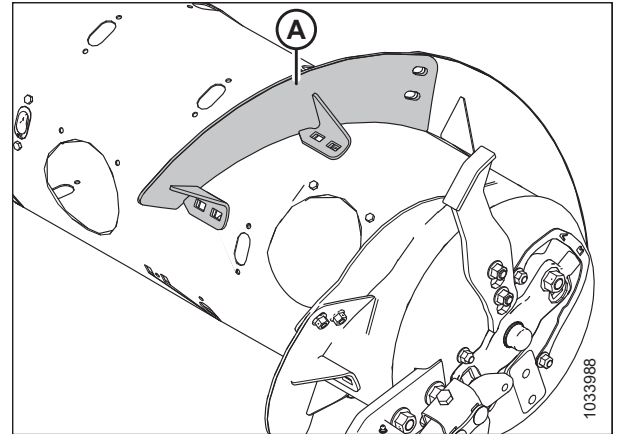
Фигура 3.116: Дясна страна на шнека
