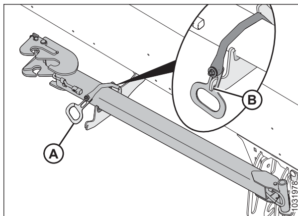
Фигура 3.352: Съхранение на удължителя на теглича
