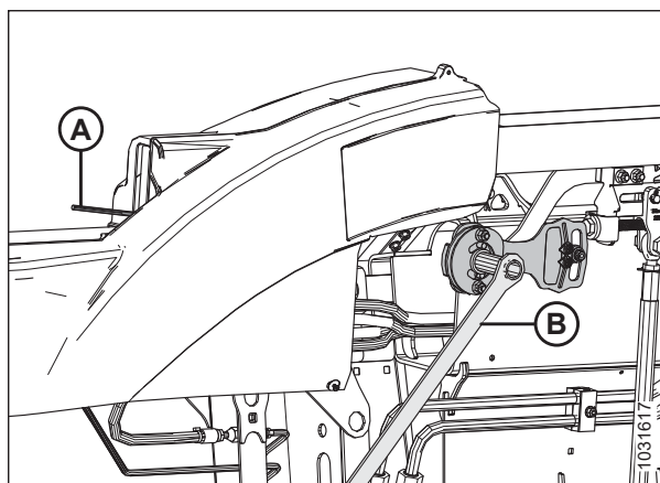
Фигура 3.195: Крило в отключено положение
