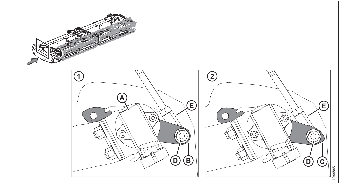
Фигура 3.208: Местоположение на датчика за височина на мотопилото
