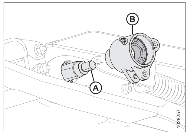
Фигура 4.201: Лагер на паразитната ролка – лява страна
