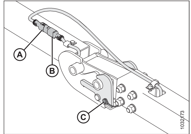
Фигура 3.382: Кабелен сноп на теглича/удължителя
