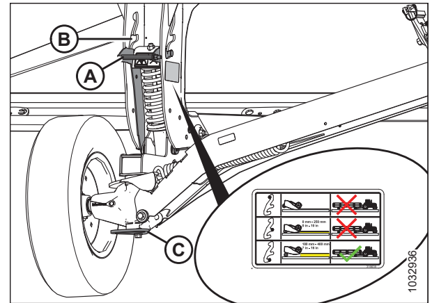
Фигура 3.144: Дясно колело
