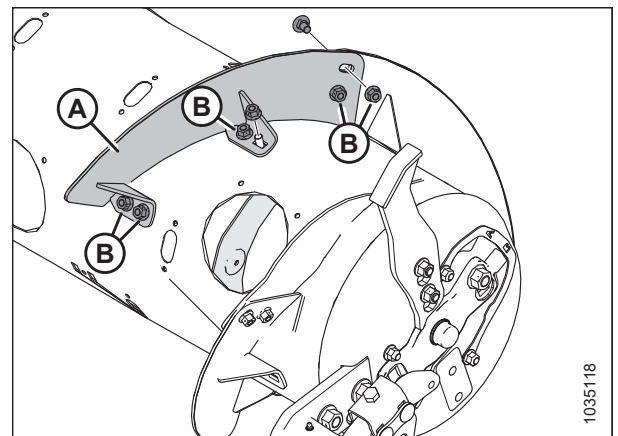
Фигура 3.118: Къса спирала – дясна страна
