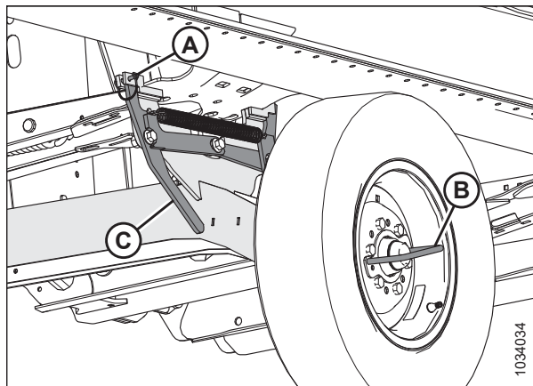
Фигура 3.361: Дясна транспортна ос, заключена в транспортно положение
