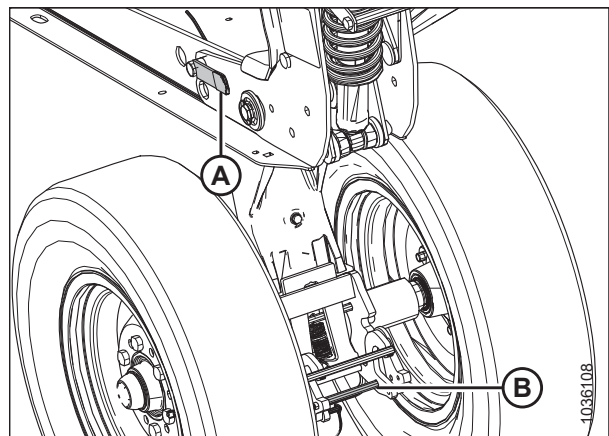
Фигура 3.358: Леви транспортни колела – освободен шарнир
