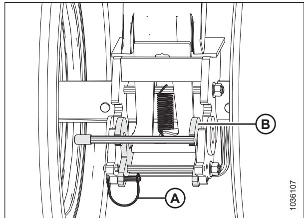
Фигура 3.357: Леви транспортни колела – ключалката за блокиране на въртенето е включена
