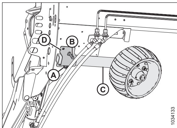
Фигура 3.366: Възел на лявото колело
