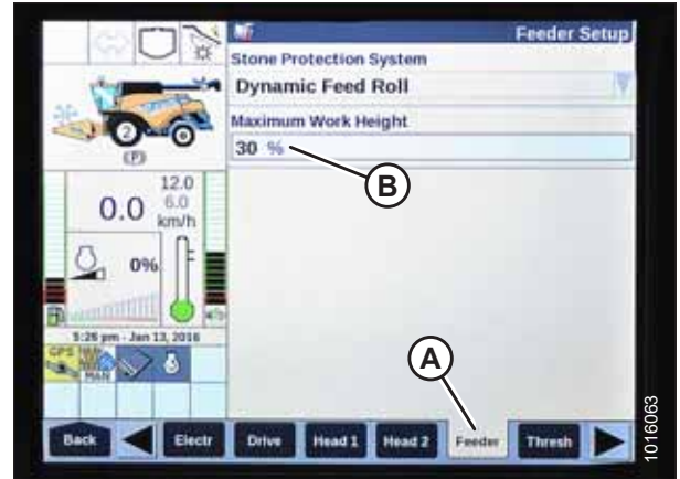
Фигура 3.334: Дисплей на комбайн New Holland
