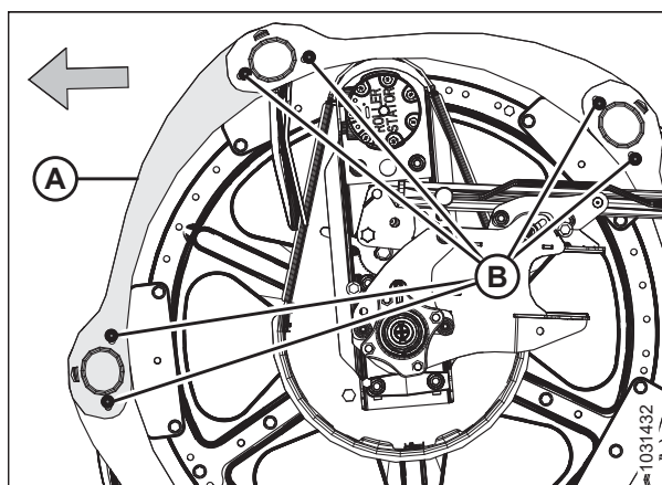
Фигура 4.307: Крайни щитове на мотовилото – вътрешен заден край
