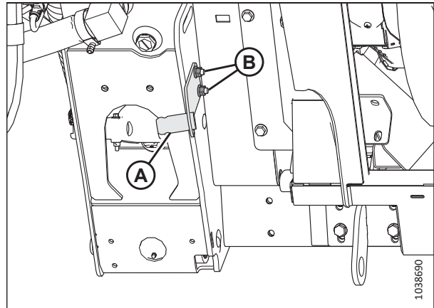
Фигура 4.46: Опорна конзола на карданната предавка
