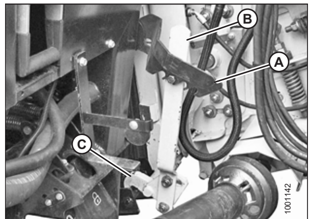
Фигура 3.80: Ключалки на подаващата камера
