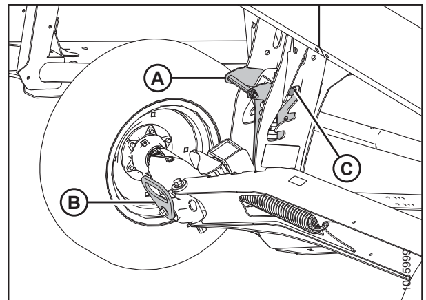
Фигура 3.364: Десни транспортни колела в най-високо положение за съхранение
