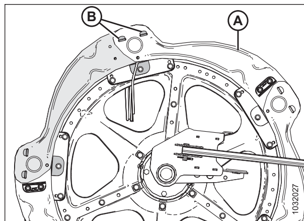
Фигура 4.304: Крайни щитове на мотовилото – външен заден край
