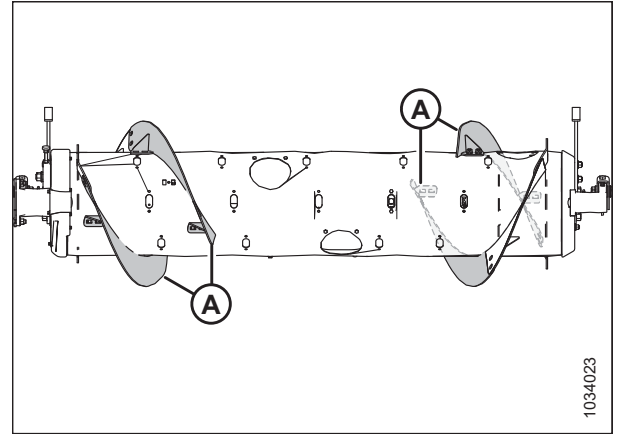
Фигура 3.122: Тясна конфигурация
