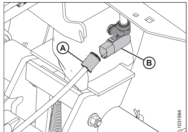
Фигура 3.345: Електрическа връзка на теглича
