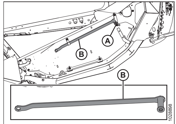
Фигура 3.183: Лява страница
