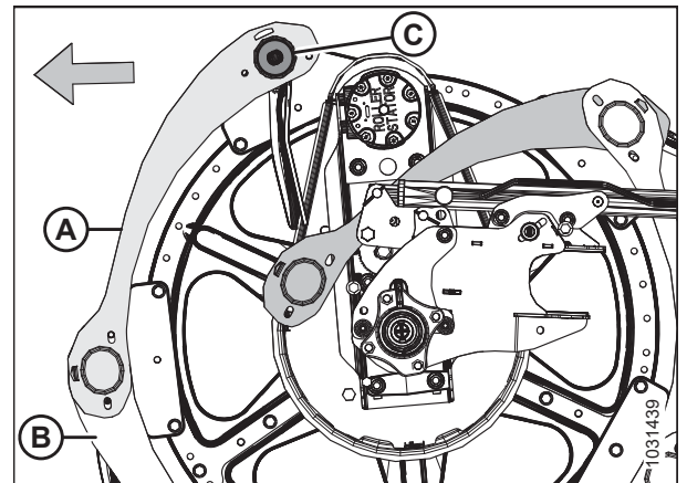
Фигура 4.310: Крайни щитове на мотовилото – вътрешен заден край
