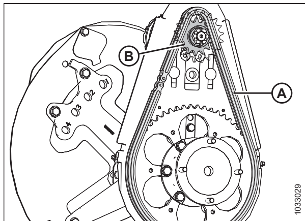
Фигура 4.327: Двойно верижно зъбно колело в конфигурацията за висок въртящ момент
