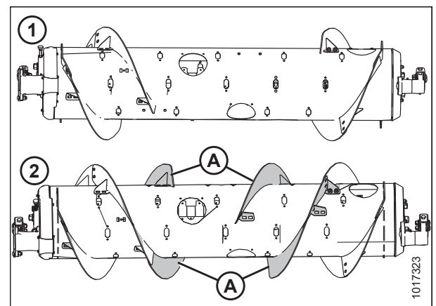
Фигура 3.88: Шнекови конфигурации – изглед отзад
