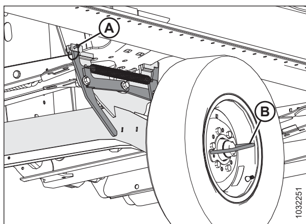
Фигура 3.375: Дясна транспортна ос
