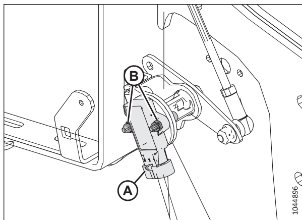
Фигура 3.209: Датчик за височината на мотовилото – дясно рамо на мотовилото
