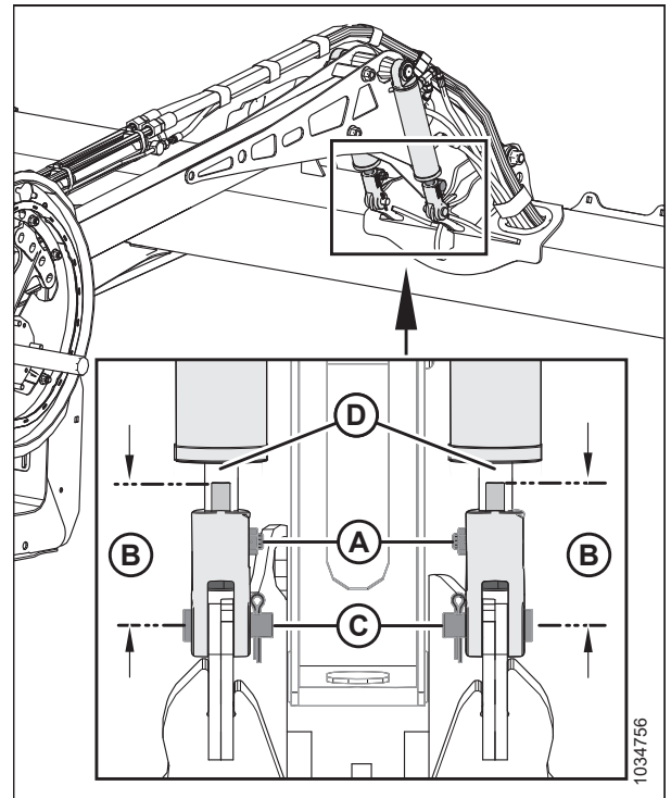
Фигура 4.266: Цилиндри на централното рамо
