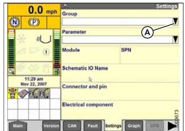
Фигура 3.280: Дисплей на комбайн New Holland
