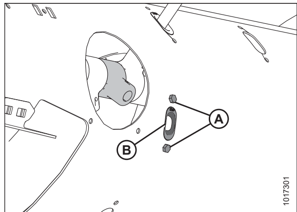
Фигура 3.134: Отвор за зъб на шнека
