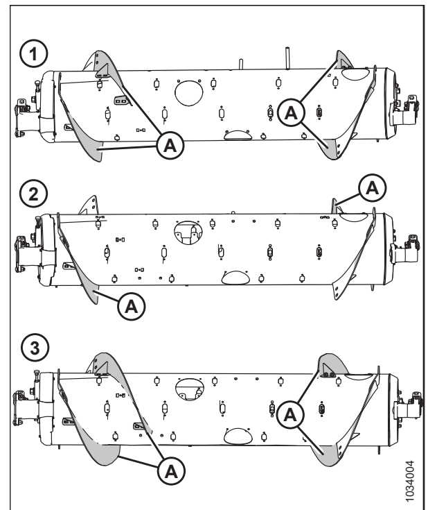
Фигура 3.108: Шнекови конфигурации – изглед отзад
