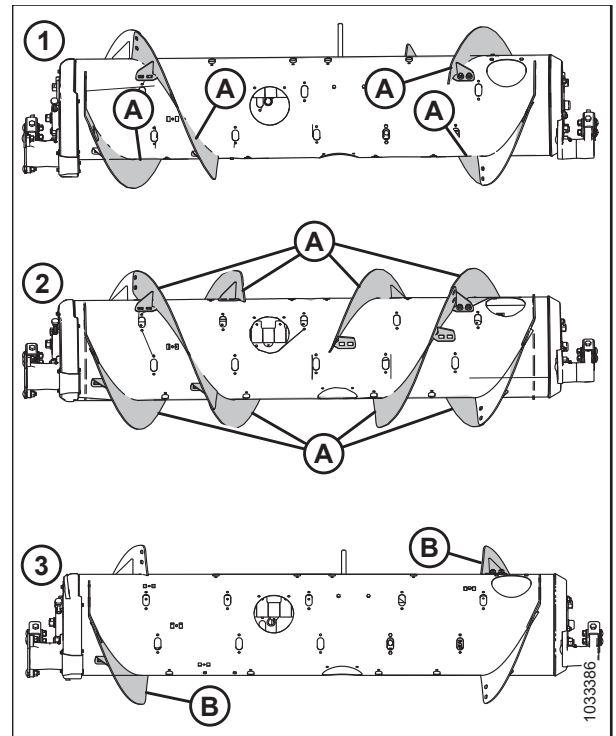
Фигура 3.105: Шнекови конфигурации – изглед отзад
