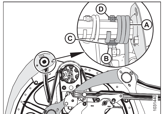
Фигура 4.311: Крайни щитове на мотовилото – вътрешен заден край
