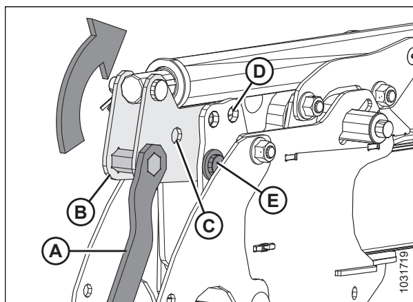
Фигура 3.217: Регулиране на цилиндър за надлъжно положение тип 1 – предно положение
