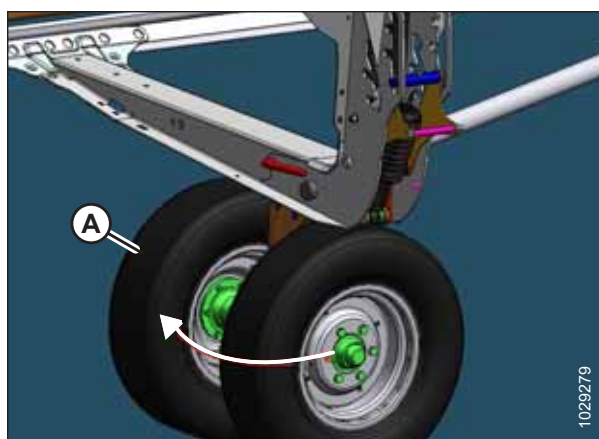
Фигура 3.370: Предни транспортни колела
