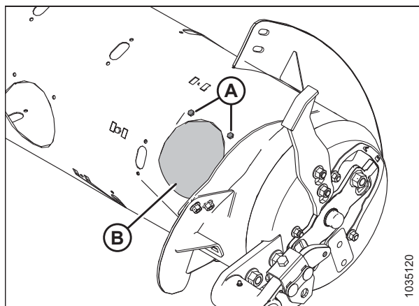
Фигура 3.115: Капак за достъп до шнека – дясна страна
