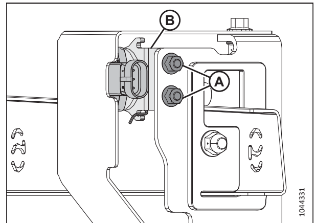
Фигура 3.224: Датчик за надлъжно положение
