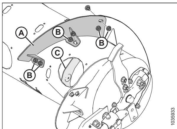
Фигура 3.110: Къса спирала – дясна страна
