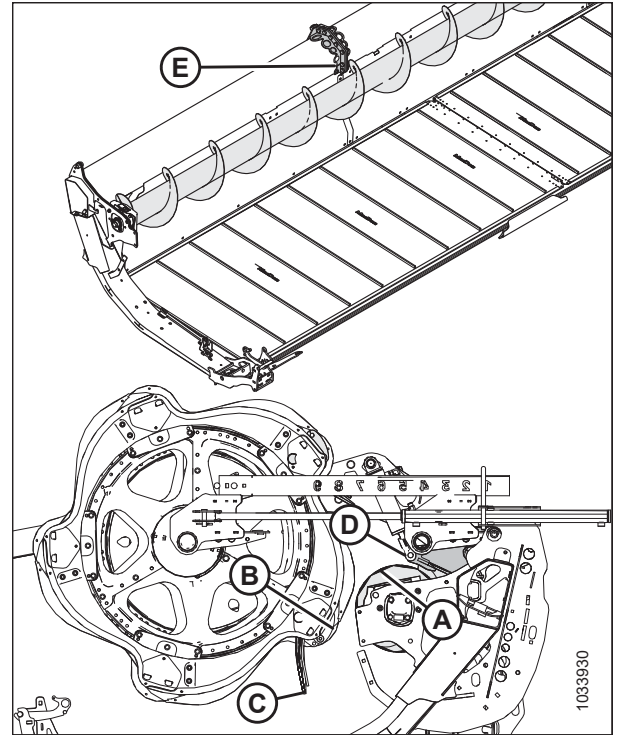
Фигура 3.240: Местоположения за проверка на хлабината на UCA
