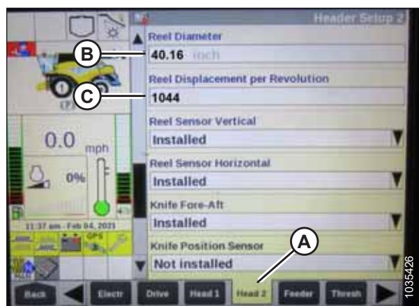
Фигура 3.311: Дисплей на комбайн New Holland
