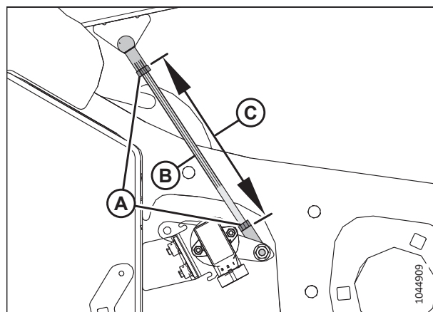
Фигура 3.211: Датчик за височина на мотовилото – спуснато дясно рамо на мотовилото
