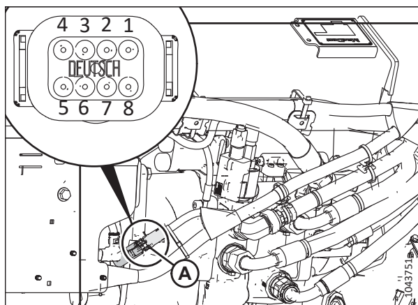
Фигура 3.268: Конектор
