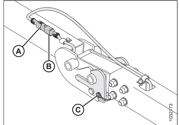
Фигура 3.343: Кабелен сноп на теглича/ удължителя
