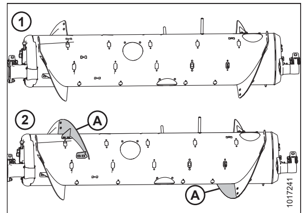
Фигура 3.98: Шнекови конфигурации – изглед отзад
