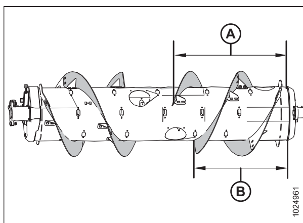
Фигура 3.82: Много тясна конфигурация – изглед отзад
