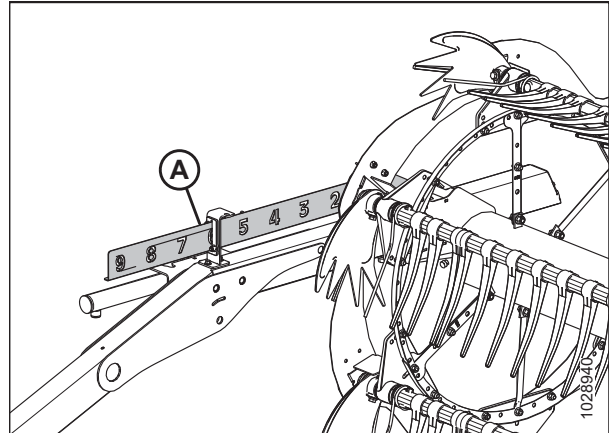
Фигура 3.189: Надлъжно положение
