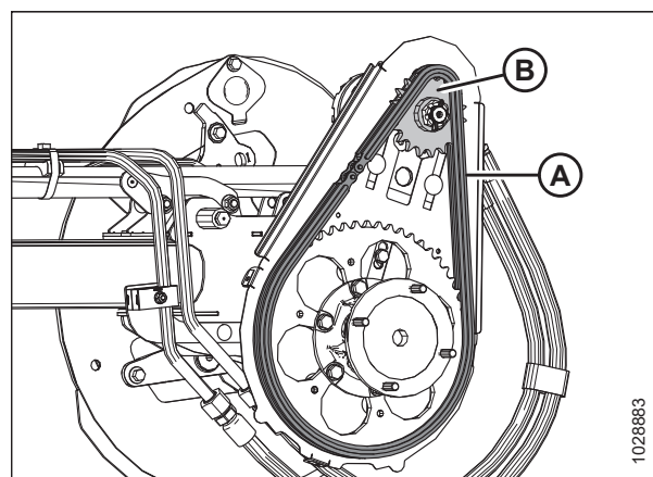
Рисунок 5.215: Одиночная звездочка
