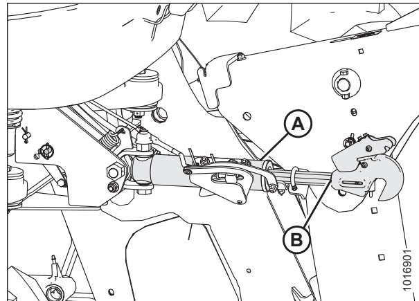
Рисунок 4.92: Гидравлическое центральное соединение
