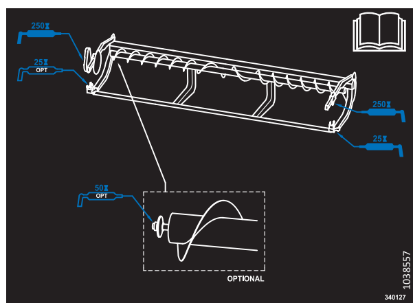
Рисунок 5.14: Наклейка с указанием точки смазки для жатки с одинарным приводом ножа с односоставным верхним поперечным шнеком
