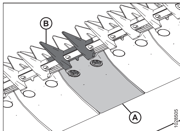
Рисунок 5.71: Укороченный противорежущий палец и износная пластина
