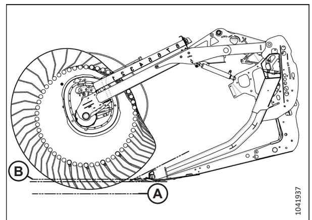
Рисунок 3.63: Профиль пальцев — положение эксцентрика 4, максимальный угол жатки
