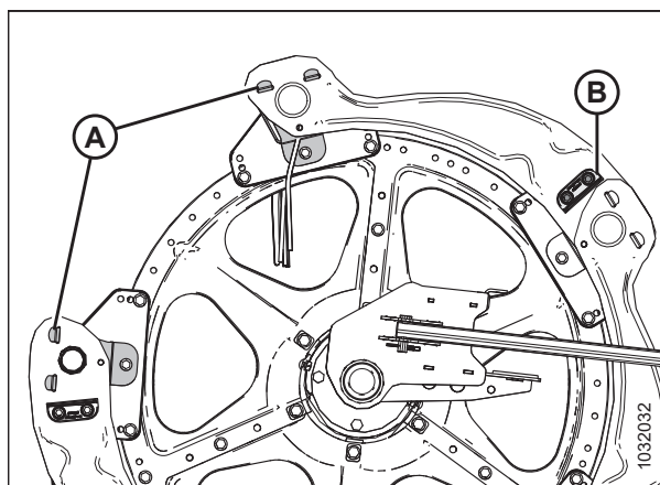
Рисунок 5.195: Боковой щиток мотовила снят — внешняя сторона хвостовика
