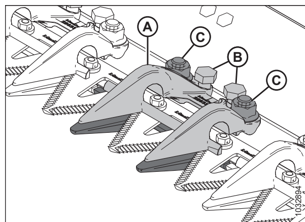
Рисунок 5.72: Укороченный противорежущий палец
