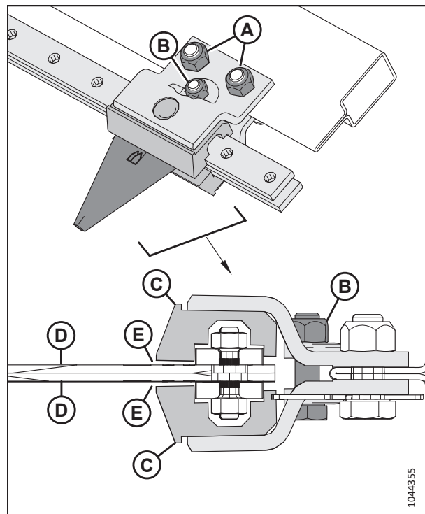
Рисунок 5.240: Вертикальный нож (вид сверху)
