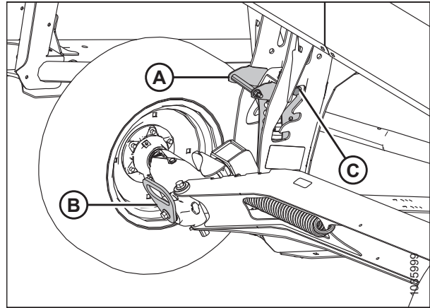
Рисунок 3.117: Правые транспортные колеса в самом высоком положении хранения
