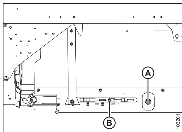
Рисунок 5.113: Натяжитель полотна
