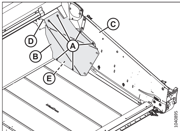
Рисунок 5.128: Задний широкий дефлектор — показана левая сторона
