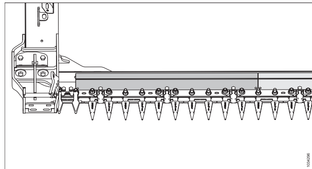
Рисунок 6.12: Комплект камнеуловителей
