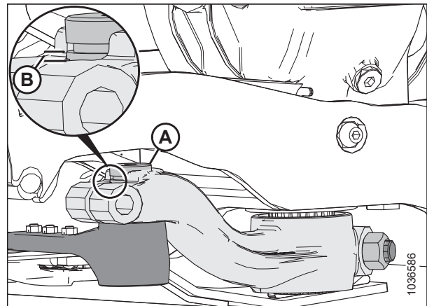
Рисунок 5.38: Головка ножа
