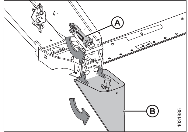
Рисунок 3.76: Делитель с опцией замка
