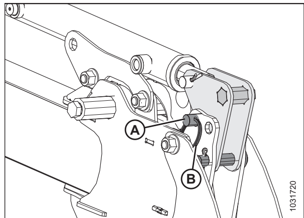
Рисунок 3.52: Регулировка цилиндра перемещения вперед/назад, тип 1 — заднее положение
