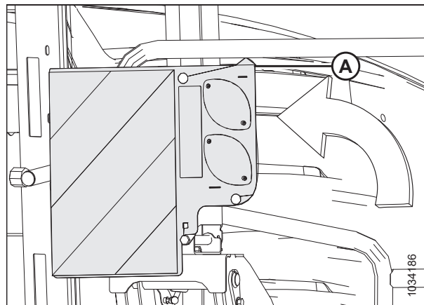
Рисунок 4.143: Левое сигнальное световое табло
