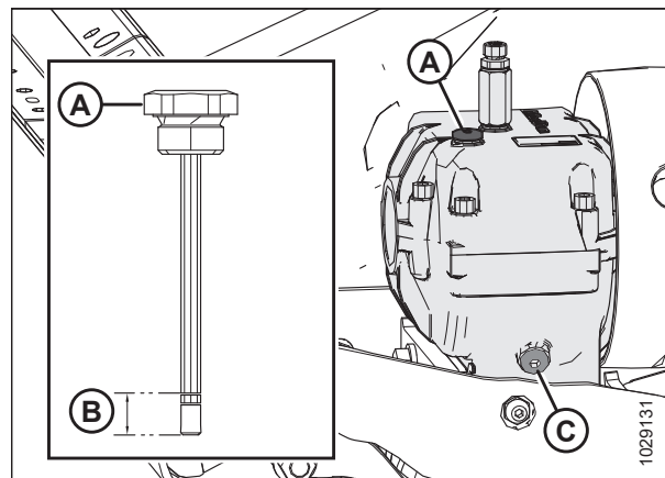
Рисунок 5.87: Редуктор привода ножа
