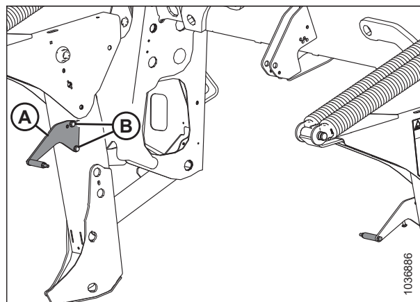
Рисунок 4.124: Кронштейн формовочного щитка — серия R2
