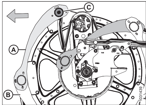
Рисунок 5.200: Боковые щитки мотовила — внутренняя сторона хвостовика
