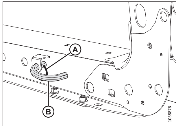
Рисунок 4.6: Опора жатки
