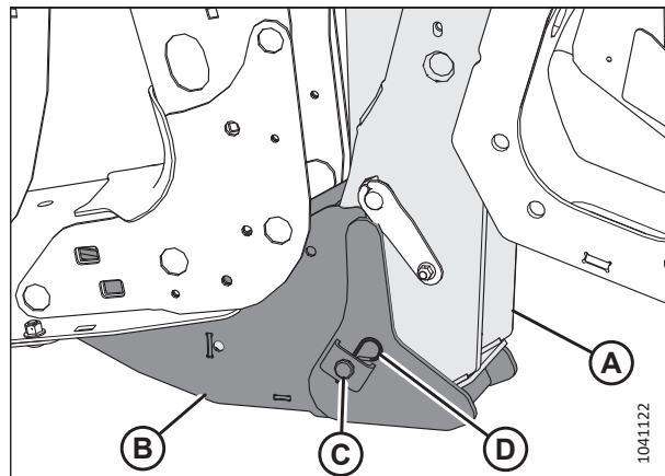
Рисунок 4.118: Лапа жатки и подъемное соединение косилки, соединенные опорой жатки
