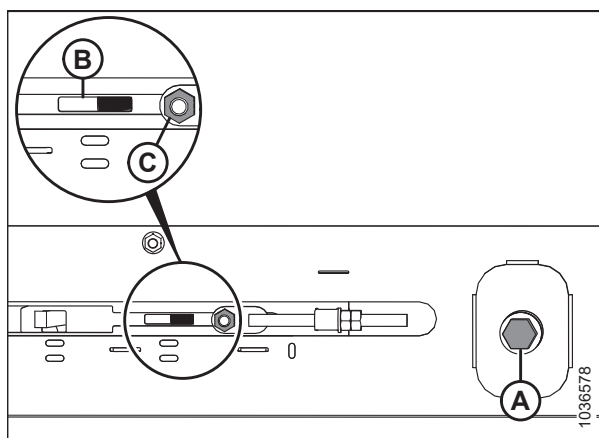
Рисунок 5.99: Регулировка левого натяжителя
