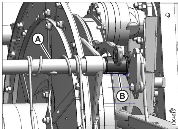
Рисунок 5.160: Сторона эксцентрика
