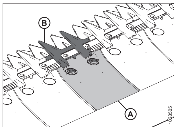
Рисунок 5.78: Центральный противорежущий палец и износная пластина
