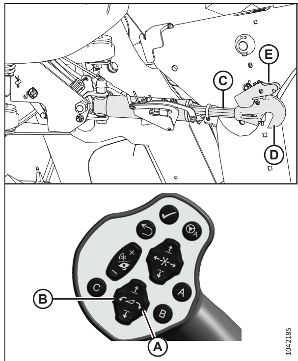
Рисунок 4.132: Гидравлическое центральное звено
