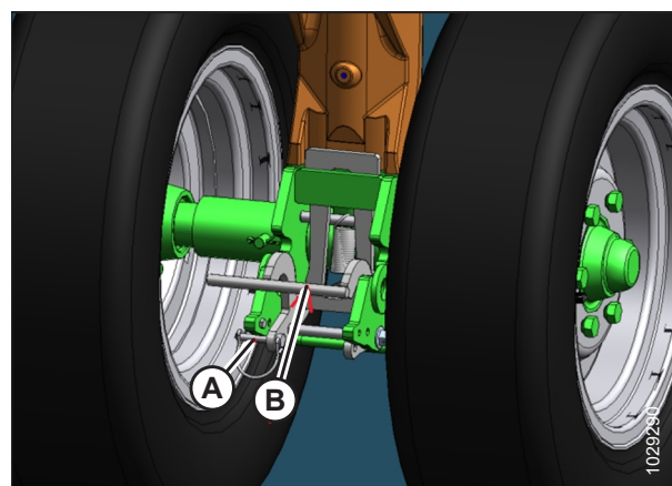
Рисунок 3.120: Передние транспортные колеса
