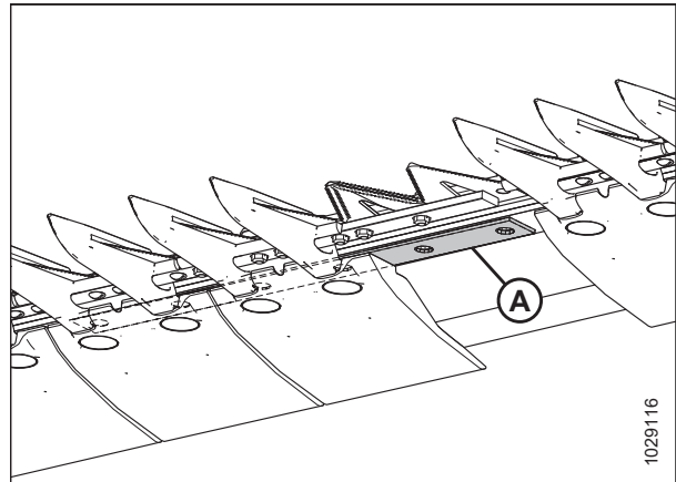
Рисунок 5.59: Ножевой брус
