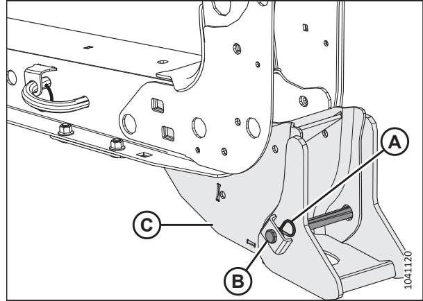
Рисунок 4.5: Опора жатки — показана левая сторона
