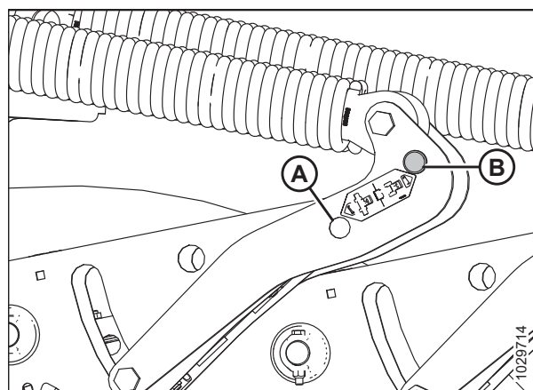
Рисунок 4.20: Рычаги флотации жатки
