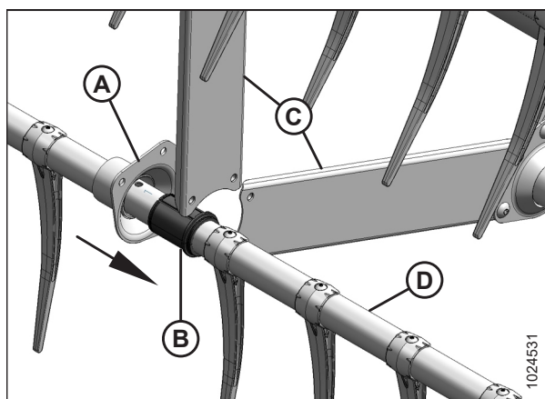
Рисунок 5.179: Противоположная опора комплекта усиления граблин мотовила (опция)
