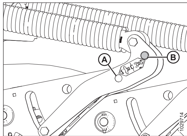
Рисунок 4.1: Соединение флотации жатки — серия M
