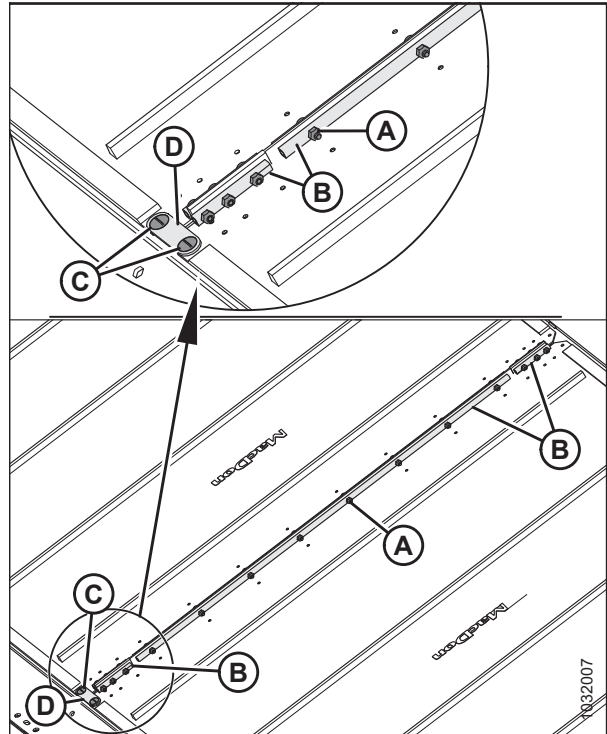
Рисунок 5.114: Стыковочные планки полотна
