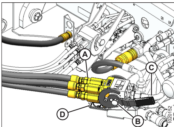
Рисунок 4.105: Многоканальная муфта ножа/ мотвила
