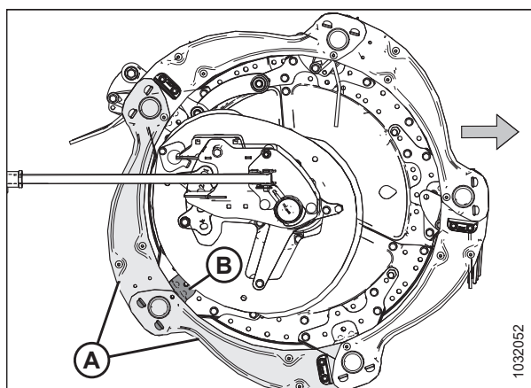
Рисунок 5.204: Опоры боковых щитков мотовила
