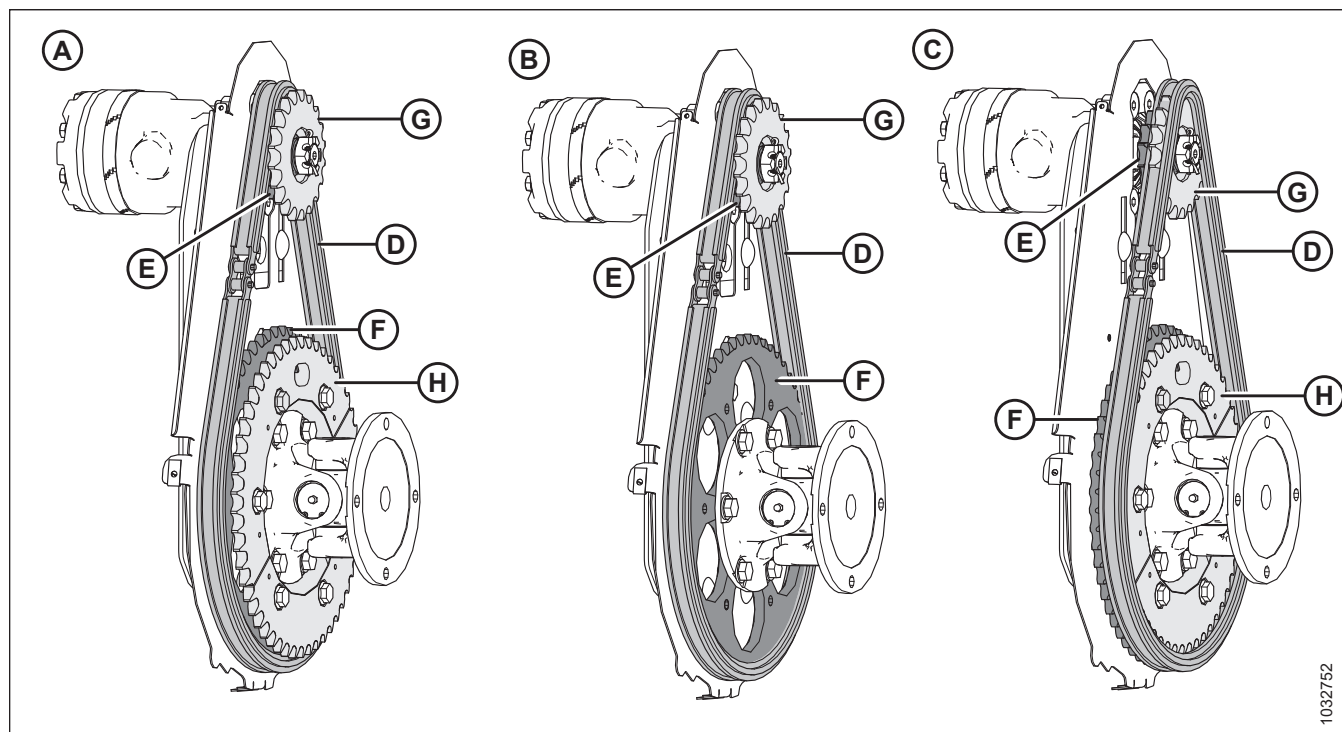
Рисунок 5.219: Конфигурации привода мотовила — дополнительные двойные звездочки
