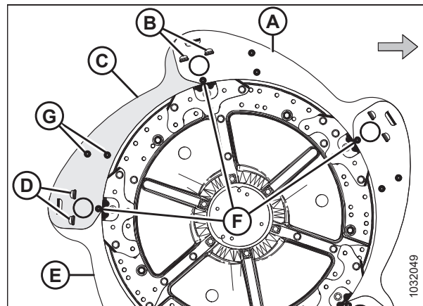
Рисунок 5.192: Боковые щитки мотовила — внутренняя сторона эксцентрика
