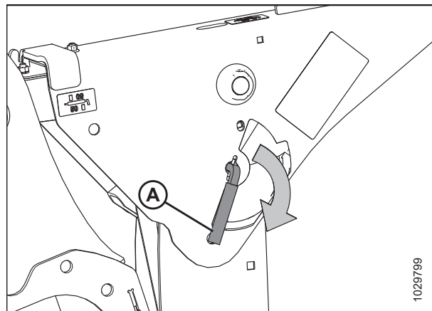
Рисунок 4.120: Рычаг предохранительного упора
