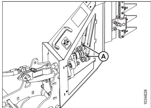
Рисунок 5.243: Тавотницы на толкателях вертикальных ножей
