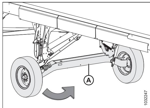
Рисунок 3.125: Правая транспортная ось
