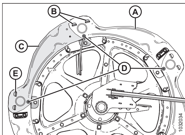
Рисунок 5.196: Боковые щитки мотовила — внешняя сторона хвостовика
