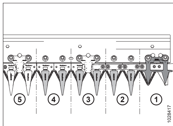
Рисунок 5.51: Заостренные противорежущие пальцы на приводной стороне
