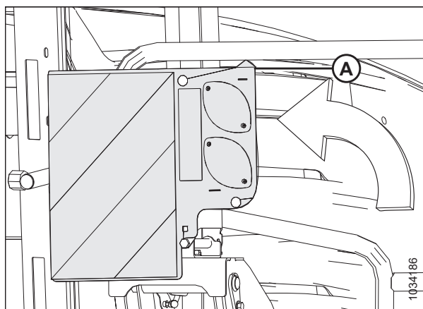
Рисунок 4.126: Левое сигнальное световое табло
