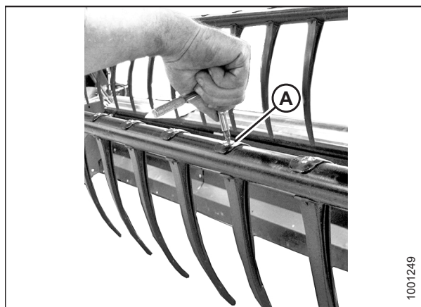
Рисунок 5.151: Установка пластмассового пальца
