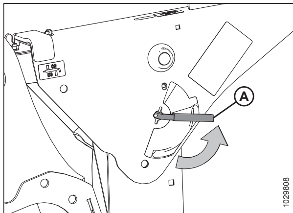
Рисунок 4.151: Рычаг предохранительного упора
