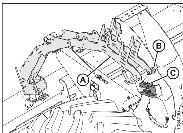
Рисунок 4.142: Левая наружная опора косилки
