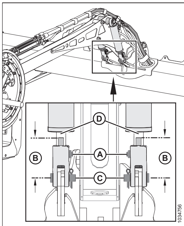
Рисунок 5.140: Гидроцилиндры центрального рычага
