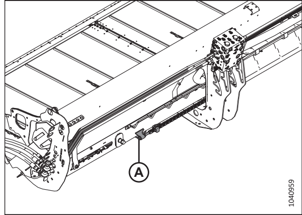
Рисунок 3.85: Болт регулировки цепи — показан левый, правый — аналогичный
