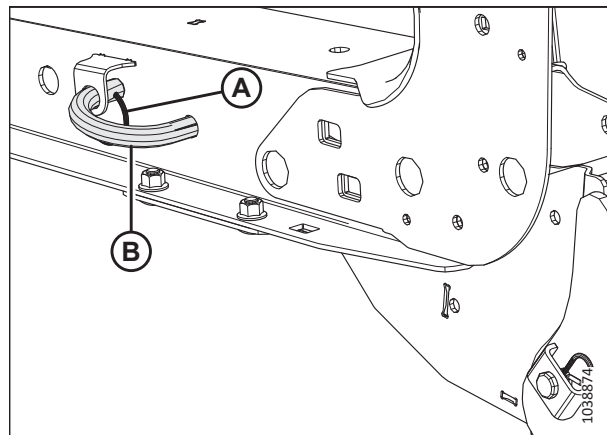
Рисунок 4.96: Опора жатки
