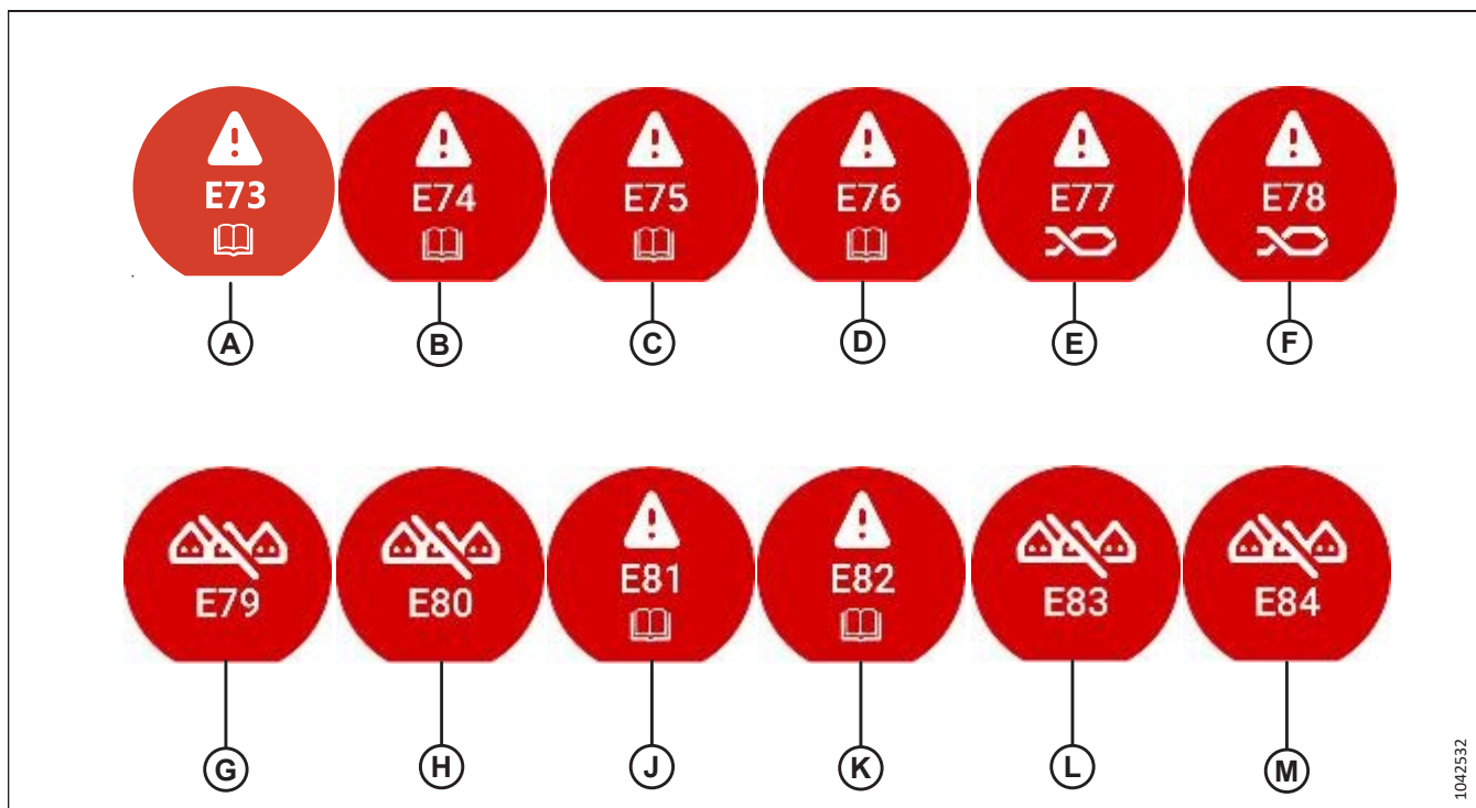
Рисунок 5.22: Символ кодов неисправностей — дисплей сенсорного кодирующего устройства
