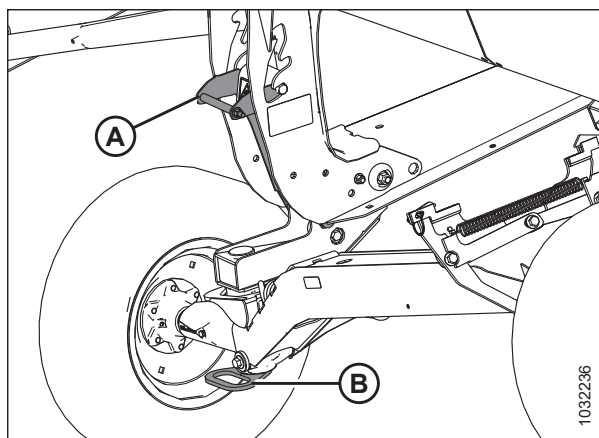
Рисунок 3.122: Копирующие колеса
