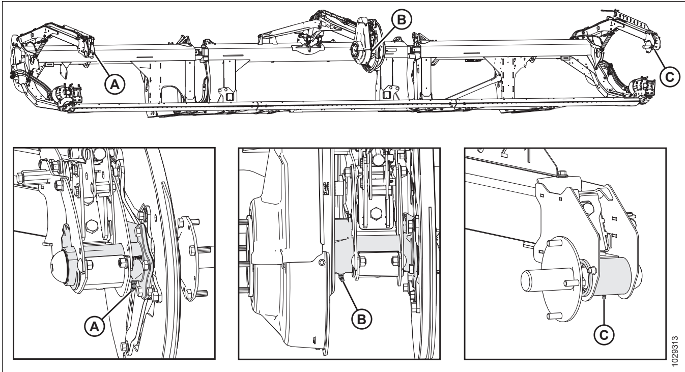
Рисунок 5.11: Мотовило
