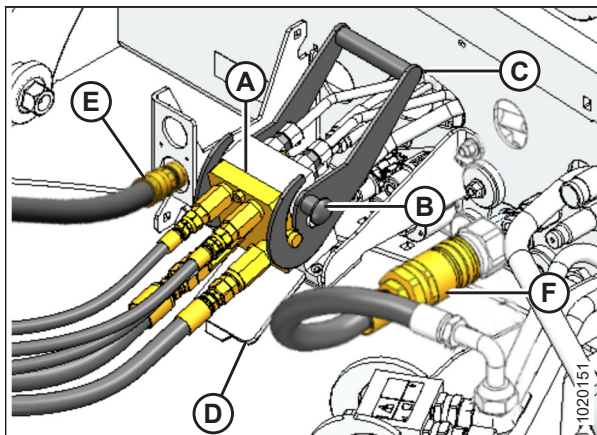
Рисунок 4.104: Многоканальная муфта полотна/ мотвила
