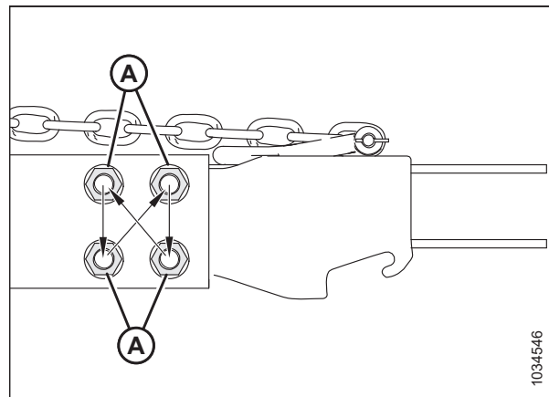
Рисунок 5.230: Последовательность затяжки
