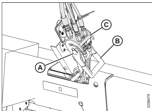
Рисунок 4.57: Гидравлическая система мотовила
