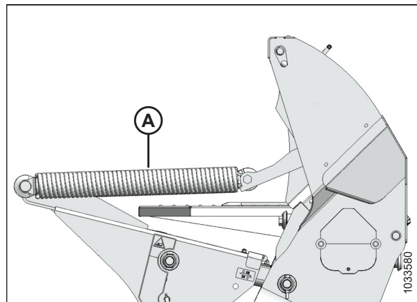
Рисунок 4.85: Пружины флотации жатки
