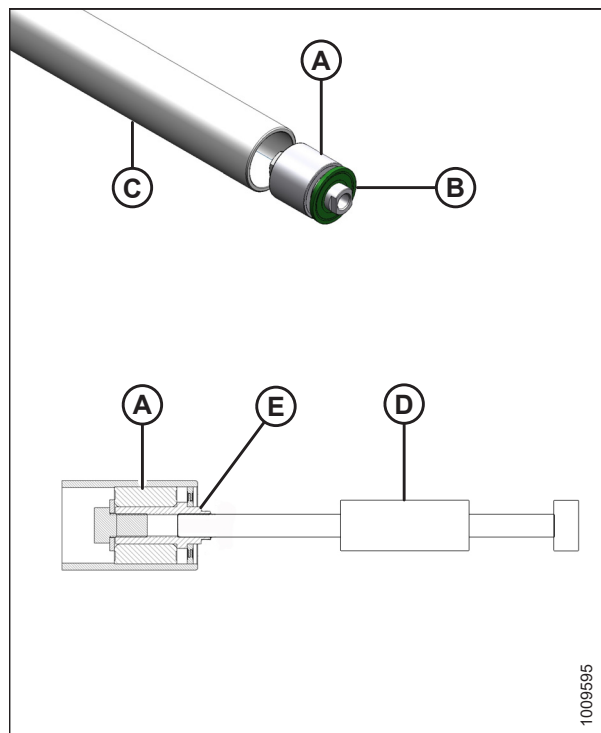
Рисунок 5.118: Роликовый подшипник
