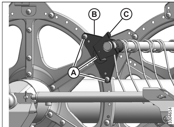
Рисунок 5.171: Хвостовик
