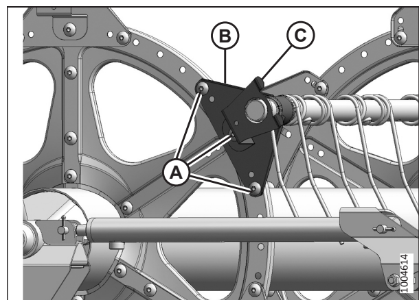
Рисунок 5.156: Хвостовик
