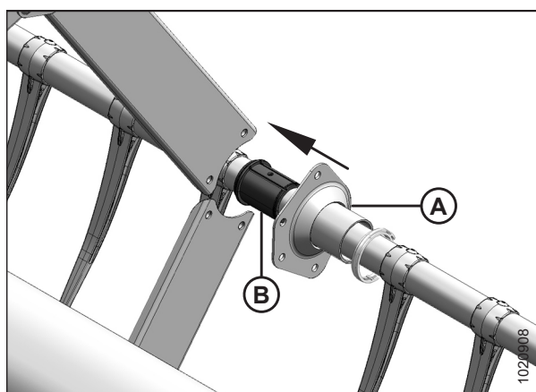
Рисунок 5.178: Опора комплекта усиления граблин мотовила (опция)
