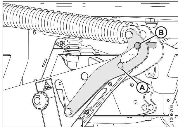
Рисунок 4.76: Рычаги флотации жатки
