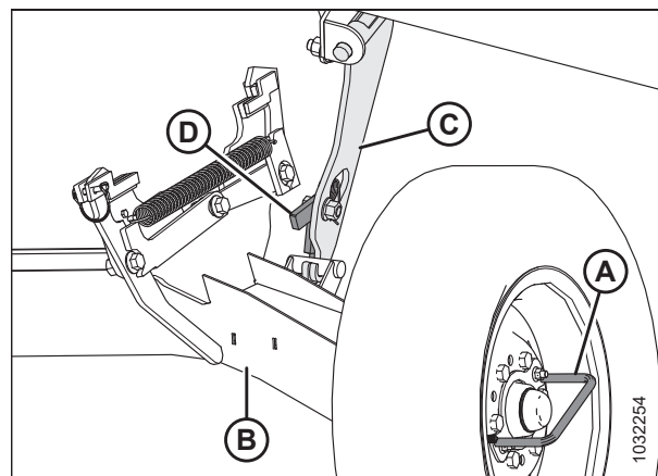
Рисунок 3.116: Правая транспортная ось зафиксирована в рабочем положении
