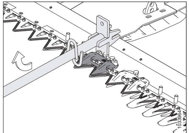
Рисунок 5.47: Регулировка смещением вверх — укороченный противорезающий палец
