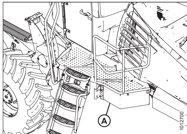
Рисунок 4.149: Левая платформа
