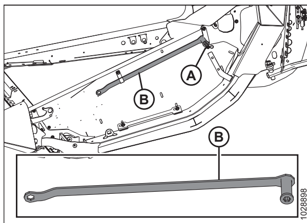
Рисунок 5.208: Место хранения универсального инструмента — левая сторона
