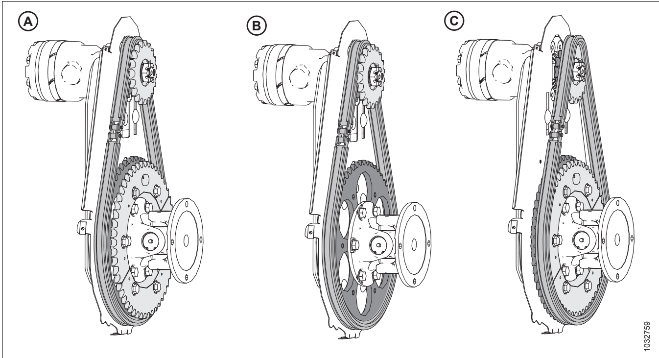
Рисунок 5.216: Конфигурации привода мотовила — дополнительные двойные звездочки
