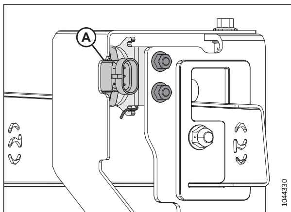
Рисунок 3.56: Датчик продольного перемещения
