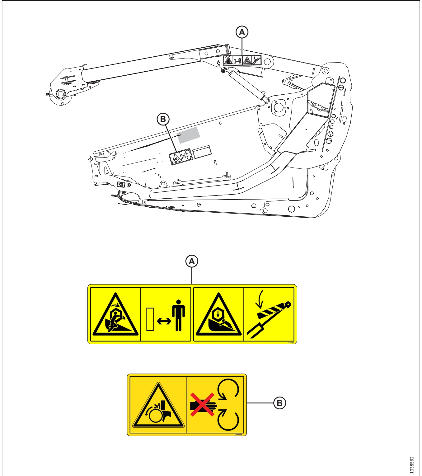
Рисунок 1.21: Боковины жатки и опоры мотовила
