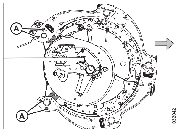
Рисунок 5.187: Боковой щиток мотовила снят — внешняя сторона эксцентрика
