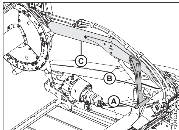
Рисунок 5.143: Рычаг центровки одинарного мотовила
