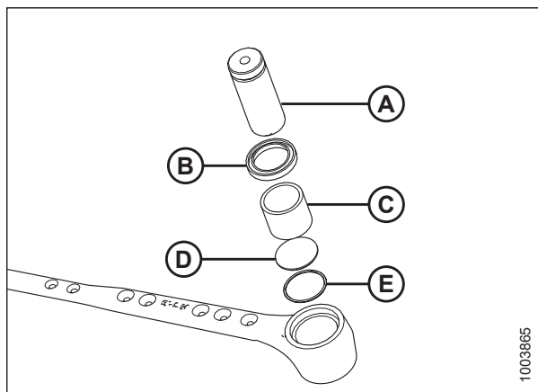
Рисунок 5.35: Подшипник головки ножа в сборе
