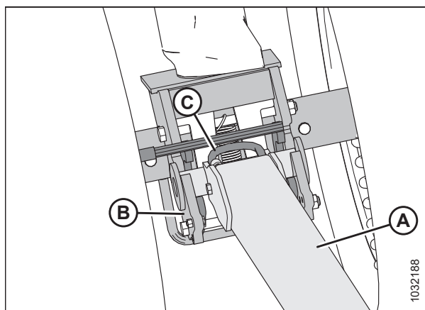
Рисунок 3.100: Защелка после отсоединения от удлинителя
