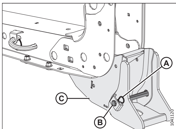
Рисунок 4.72: Лапа и опора жатки
