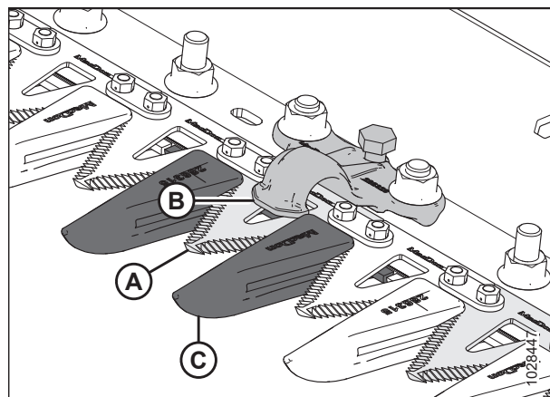
Рисунок 5.55: Прижим острого противорежущего пальца
