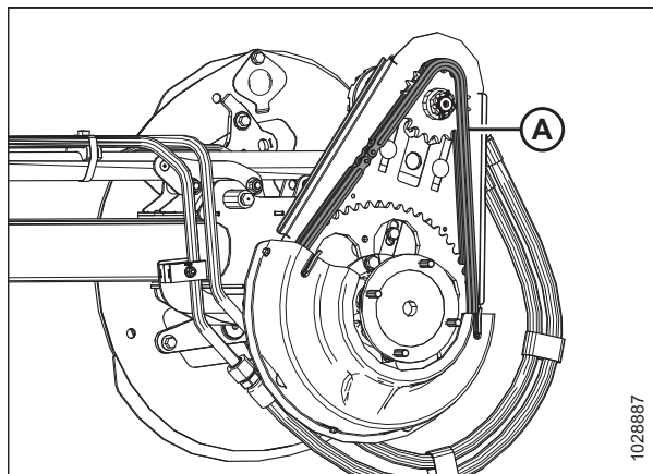
Рисунок 5.17: Приводная цепь — показан привод сдвоенного мотовила
