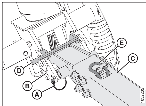
Рисунок 3.135: Буксирная тяга и левый транспортный шарнир
