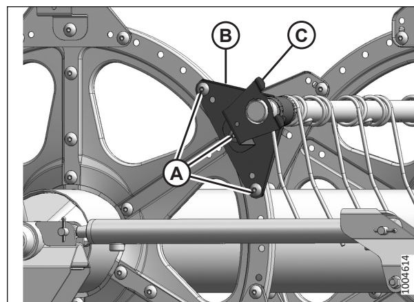
Рисунок 5.176: Хвостовик
