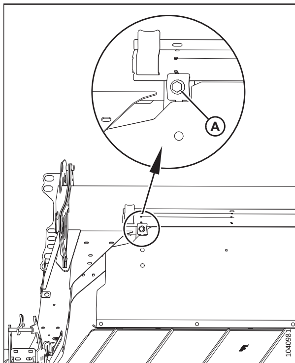
Рисунок 3.91: Изображение правой деки
