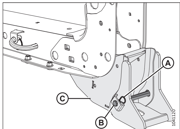
Рисунок 4.168: Стойка жатки
