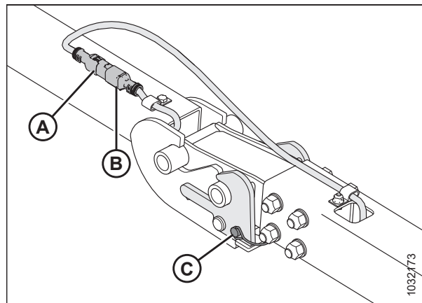
Рисунок 3.133: Жгут проводов буксирной тяги/удлинителя
