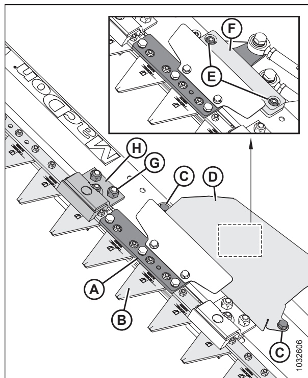
Рисунок 5.238: Вертикальный нож — противорежущий палец снят
