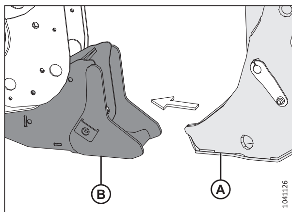
Рисунок 4.40: Лапа и опора жатки
