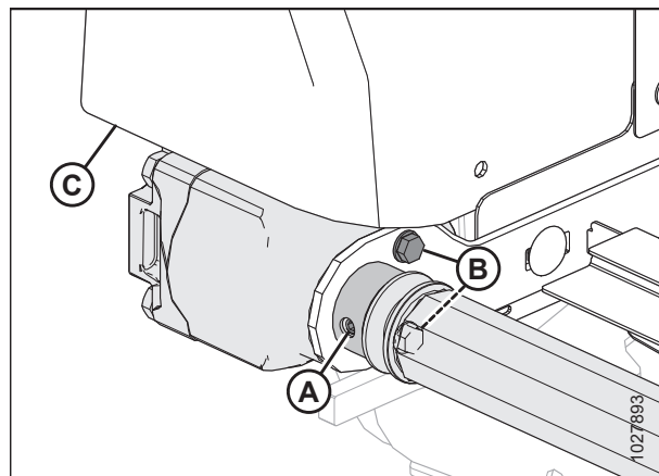
Рисунок 5.115: Приводной ролик
