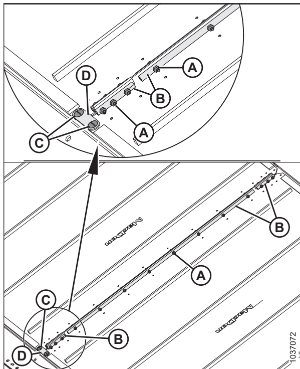
Рисунок 5.94: Стыковочные планки полотна
