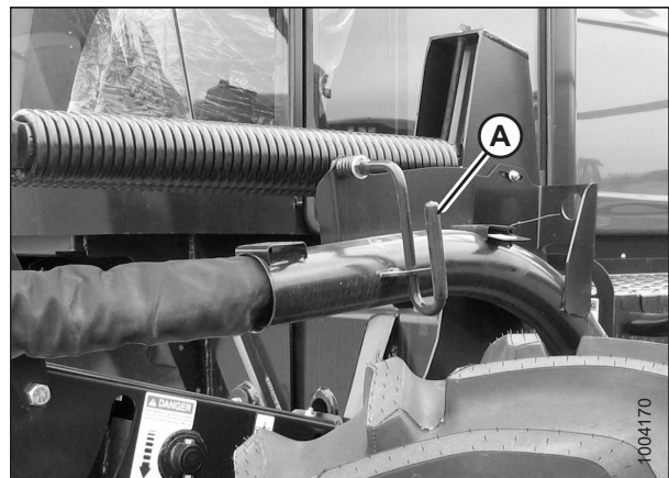
Рисунок 4.53: Место хранения шлангов
