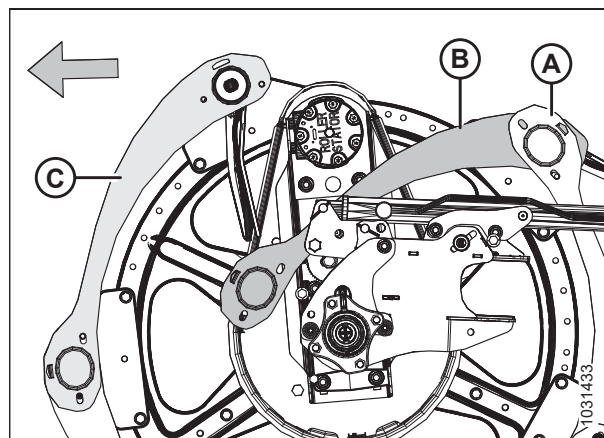
Рисунок 5.198: Боковые щитки мотовила — внутренняя сторона хвостовика
