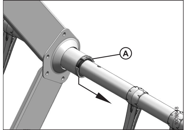
Рисунок 5.163: Хомут втулки комплекта усиления граблей
