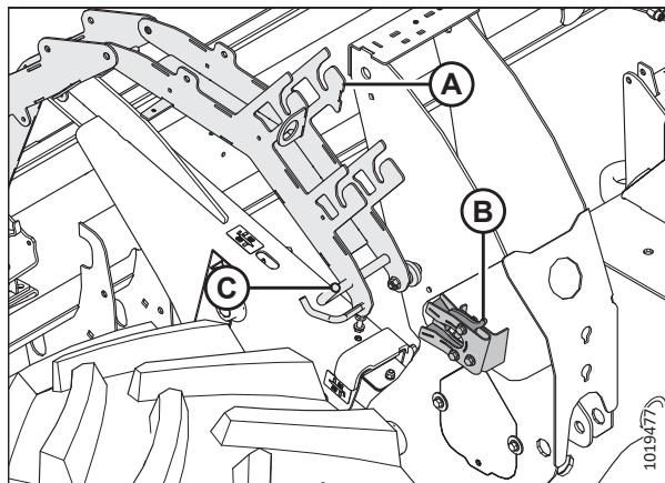
Рисунок 4.115: Система укладки гидравлических шлангов
