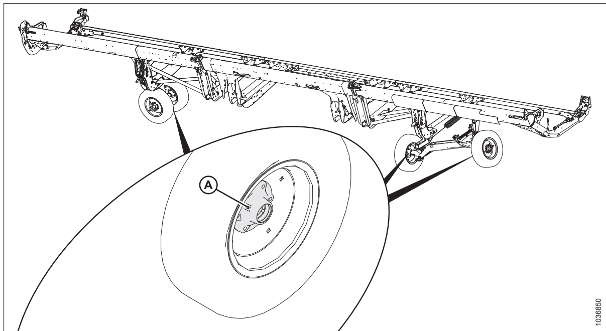
Рисунок 5.12: Подшипники колес
