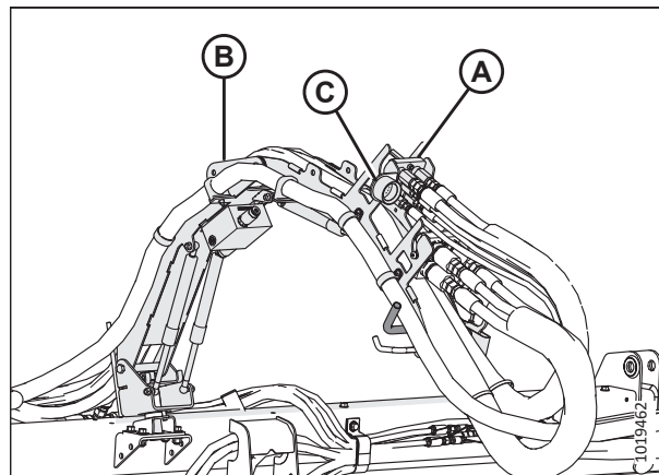
Рисунок 4.163: Система укладки гидравлических шлангов
