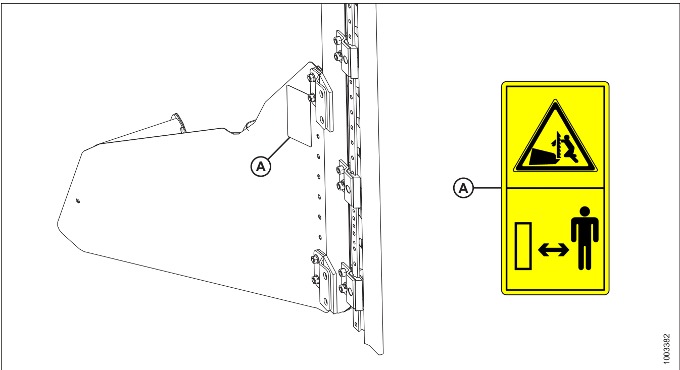
Рисунок 1.33: Вертикальный нож (дополнительное оборудование)
