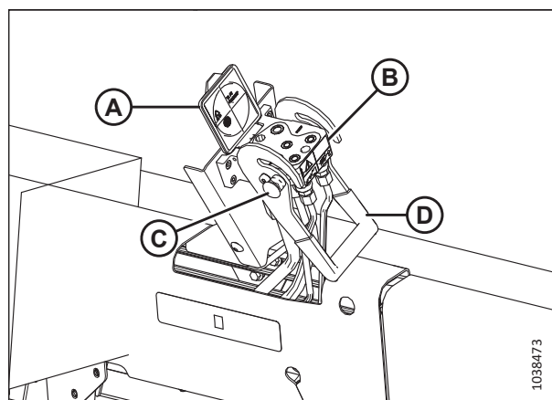
Рисунок 4.55: Гнездо гидравлики мотовила
