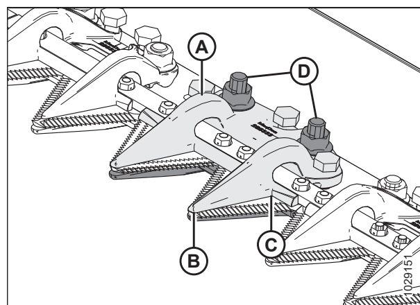
Рисунок 5.81: Прижим центрального противорежущего пальца
