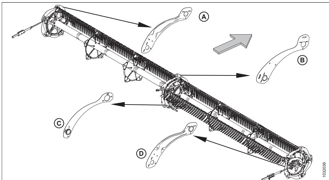
Рисунок 5.184: Боковые щитки мотовила
