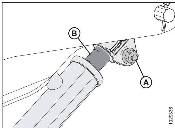
Рисунок 5.139: Гидроцилиндр внешнего рычага
