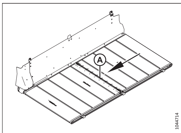
Рисунок 5.88: Стыковочная планка полотна
