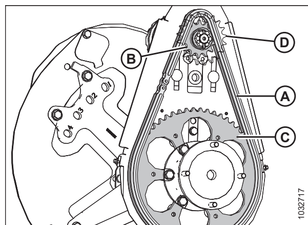
Рисунок 5.221: Двойная звездочка — конфигурация с высоким крутящим моментом
