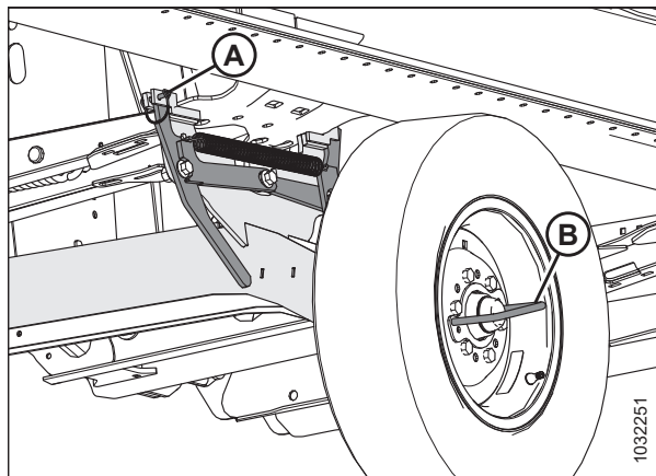
Рисунок 3.126: Правая транспортная ось
