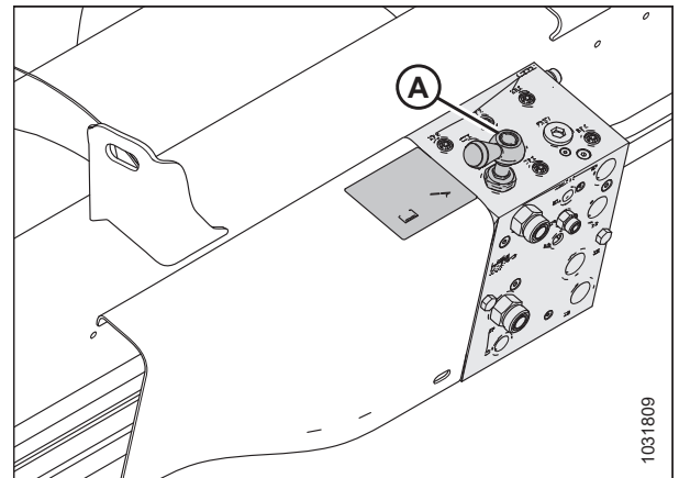
Рисунок 3.66: Отсечной клапан
