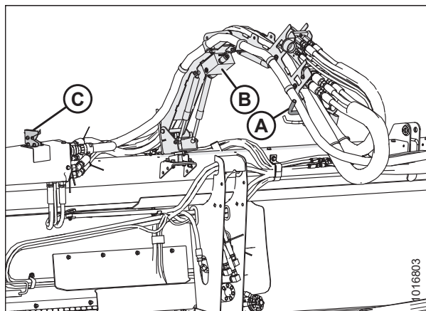
Рисунок 4.141: Система укладки гидравлических шлангов
