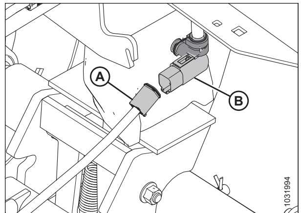
Рисунок 3.98: Электрическое соединение буксирной тяги
