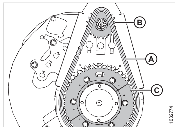
Рисунок 5.222: Двойная звездочка — конфигурация с высокой скоростью вращения
