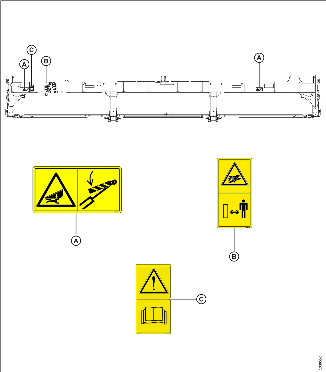
Рисунок 1.24: Задняя труба — Полотняная жатка D225
