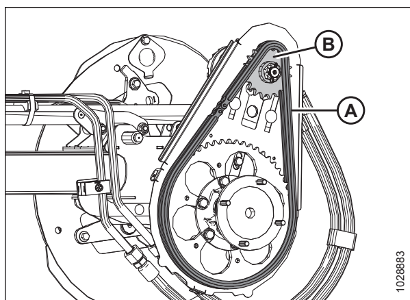
Рисунок 5.212: Одиночная звездочка
