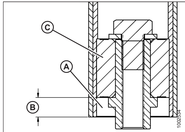
Рисунок 5.108: Подшипник натяжного ролика
