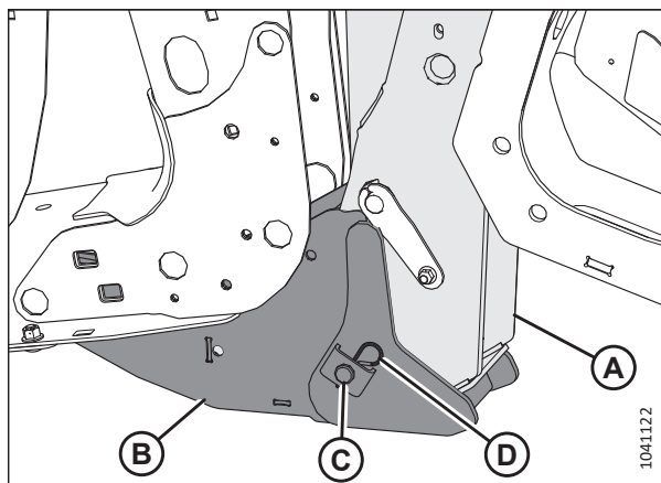
Рисунок 4.95: Подъемное соединение косилки и лапа жатки
