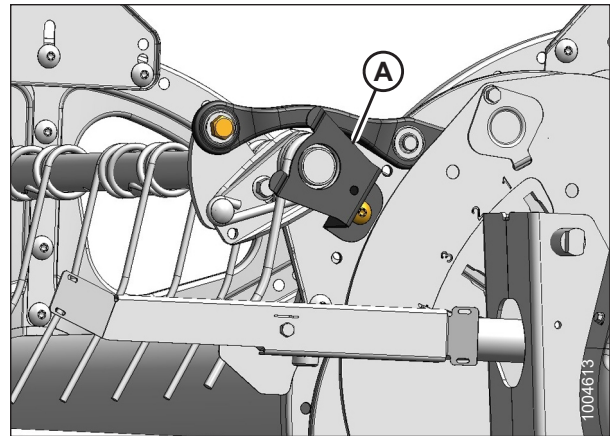
Рисунок 5.155: Сторона эксцентрика
