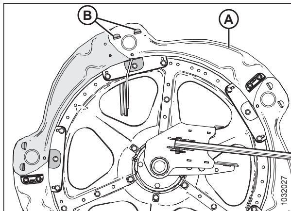
Рисунок 5.194: Боковые щитки мотовила — внешняя сторона хвостовика
