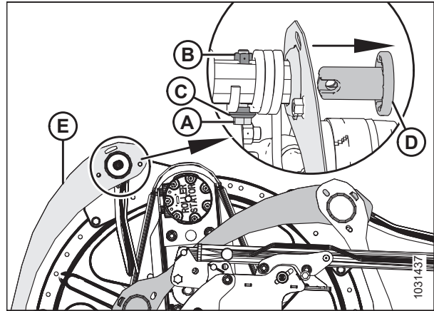
Рисунок 5.199: Боковые щитки мотовила — внутренняя сторона хвостовика
