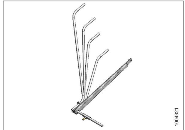
Рисунок 6.8: Стержни формирования валков
