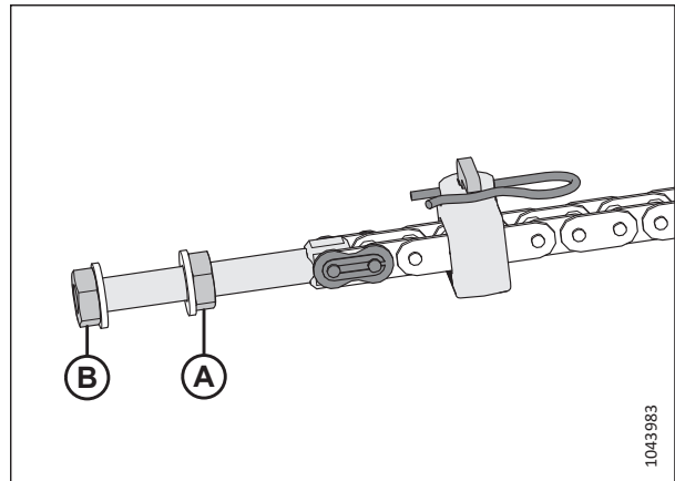
Рисунок 3.86: Левый болт регулировки цепи — правый аналогичен
