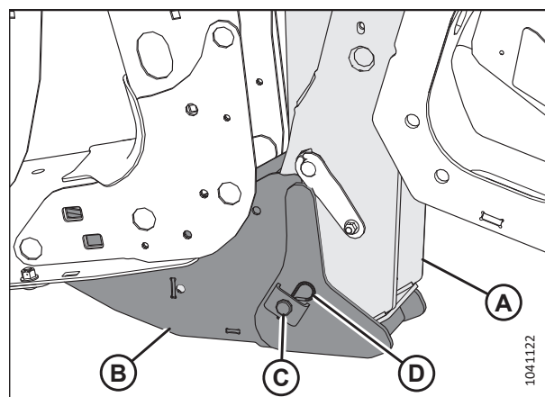
Рисунок 4.15: Подъемное соединение косилки и лапа жатки
