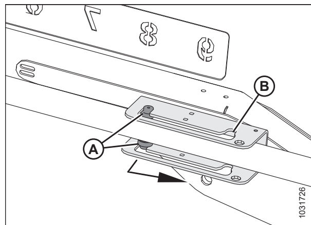
Рисунок 3.54: Регулировка цилиндра перемещения вперед/назад, тип 2 — переднее положение
