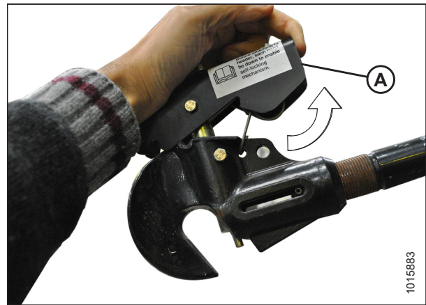
Рисунок 4.66: Центральное соединение
