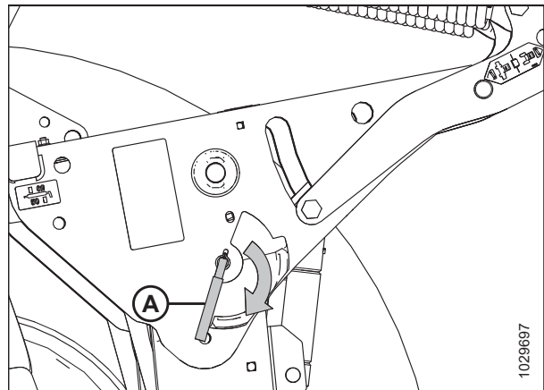
Рисунок 4.48: Рычаг предохранительного упора
