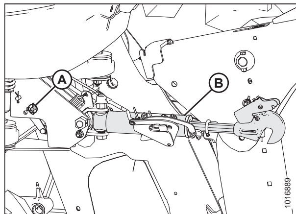
Рисунок 4.81: Центральное соединение без функции самовыравнивания
