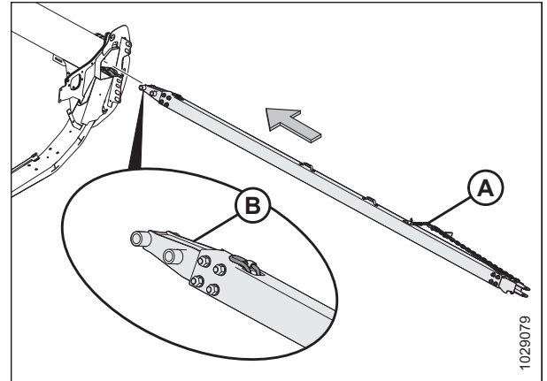
Рисунок 3.106: Сторона сцепки
