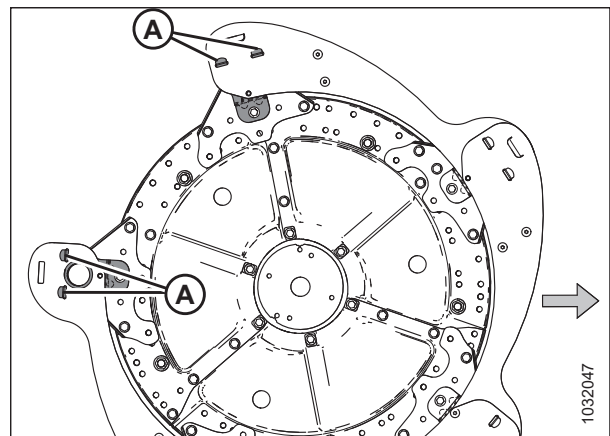
Рисунок 5.191: Боковой щиток мотовила снят — внутренняя сторона эксцентрика
