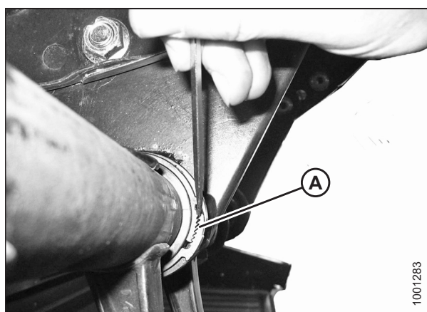
Рисунок 5.162: Хомут втулки
