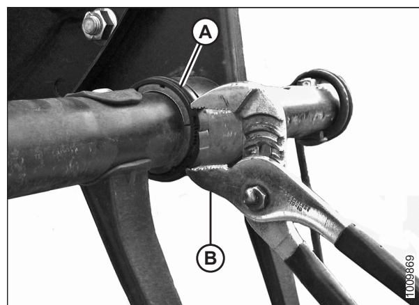
Рисунок 5.181: Установка хомута
