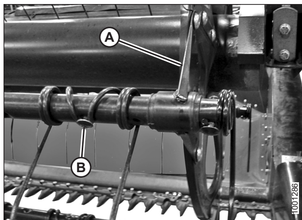
Рисунок 5.147: Граблина
