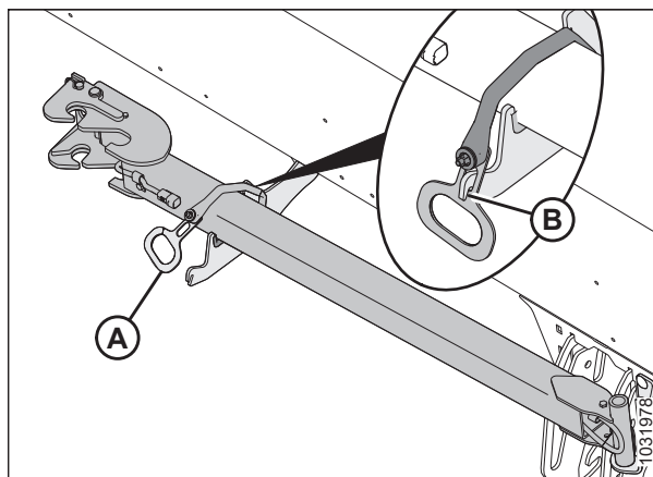
Рисунок 3.105: Место хранения удлиннителя буксирной тяги
