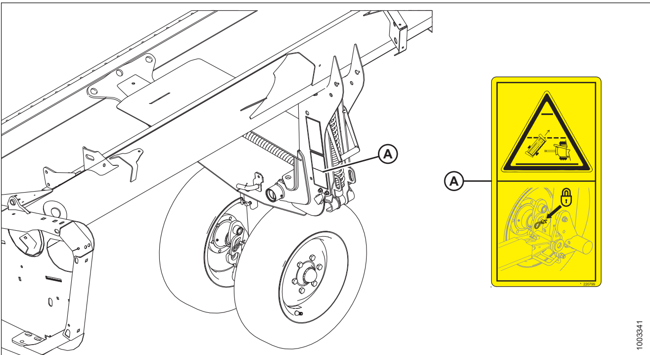
Рисунок 1.29: Транспортное средство EasyMove™ (опция)
