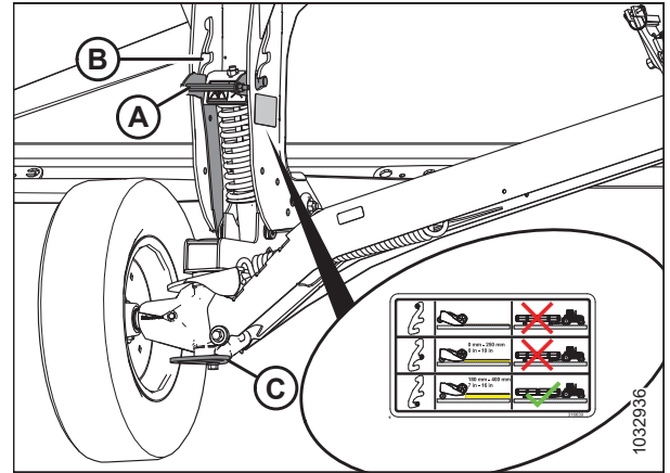
Рисунок 3.34: Правое колесо
