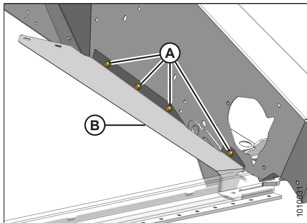
Рисунок 5.132: Передний дефлектор
