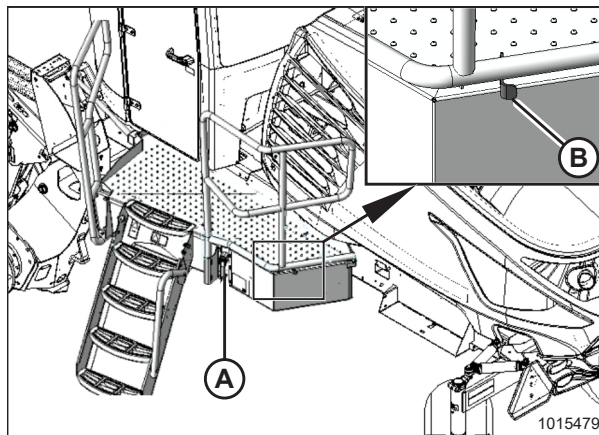
Рисунок 4.109: Левая платформа
