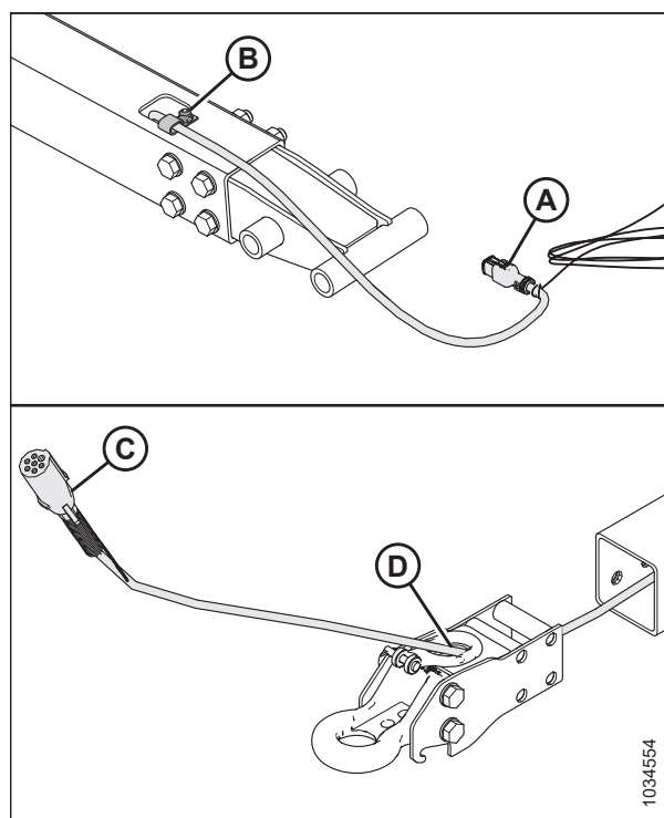
Рисунок 5.227: Снятие кольцевого буксирного переходника
