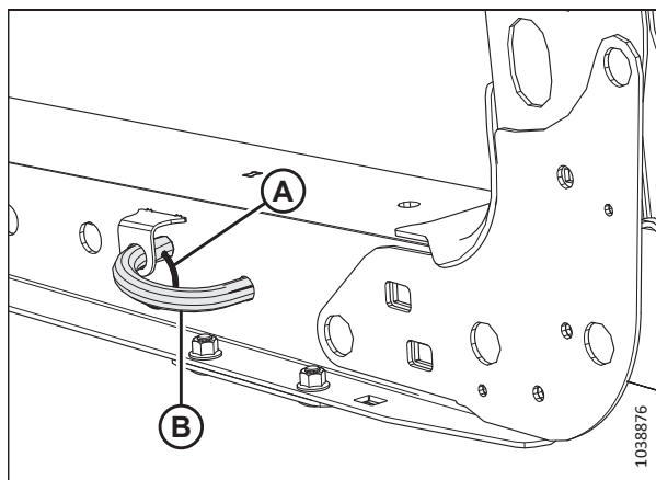
Рисунок 4.84: Опора жатки
