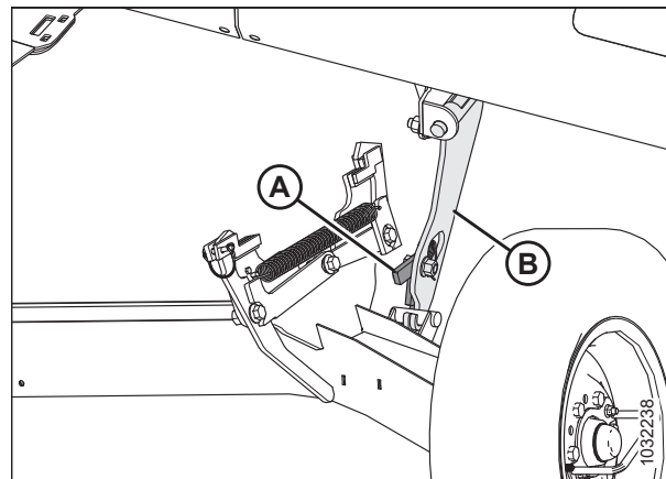
Рисунок 3.123: Правая рабочая опора
