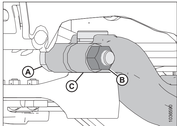
Рисунок 5.39: Головка ножа
