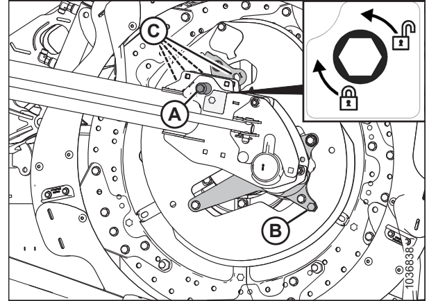
Рисунок 3.65: Положения диска эксцентрика
