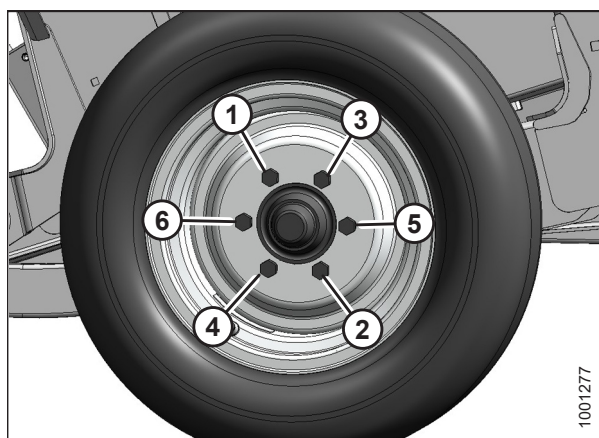
Рисунок 5.223: Последовательность затяжки болтов
