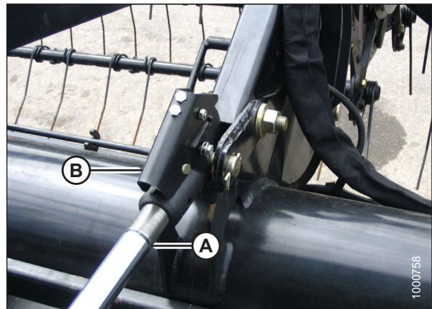
Рисунок 4.122: Гидравлическое центральное звено
