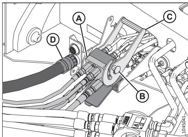
Рисунок 4.162: Многоканальная муфта полотна/мотовила
