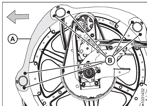
Рисунок 5.197: Боковые щитки мотовила — внутренняя сторона хвостовика
