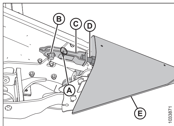
Рисунок 3.71: Делитель с опцией замка
