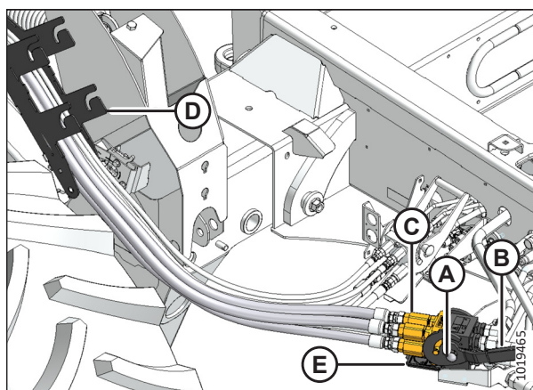
Рисунок 4.110: Многоканальная муфта ножа/мотовила
