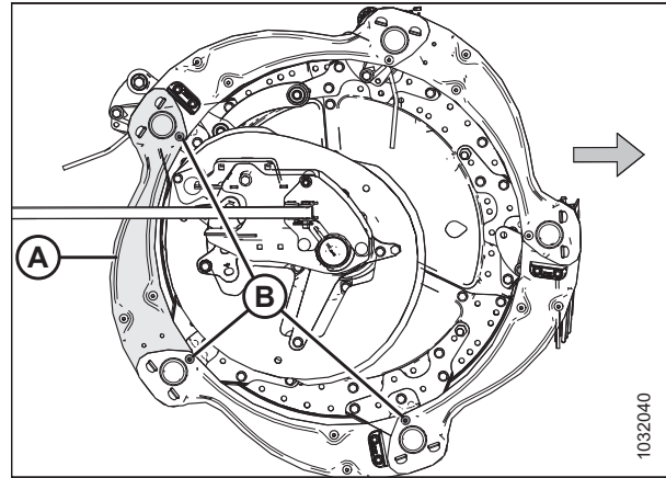
Рисунок 5.185: Боковые щитки мотовила — внешняя сторона эксцентрика
