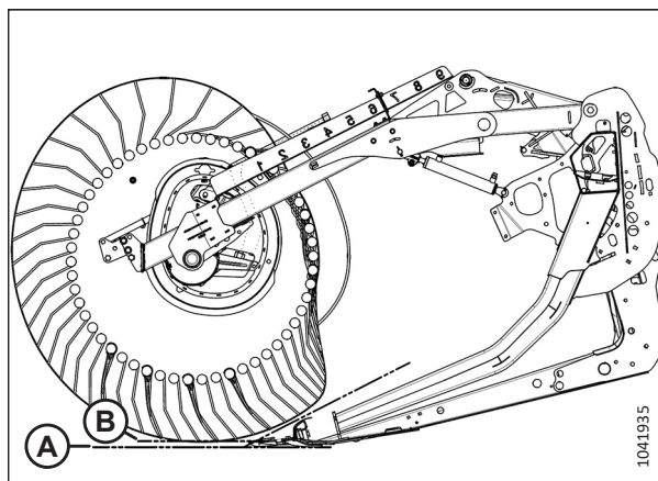
Рисунок 3.60: Профиль пальцев — положение эксцентрика 2
