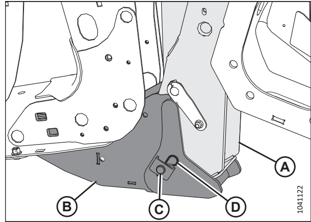
Рисунок 4.65: Лапа жатки и подъемное соединение косилки, соединенные опорой жатки
