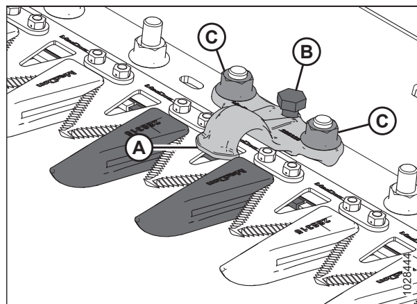
Рисунок 5.56: Заостренный прижим
