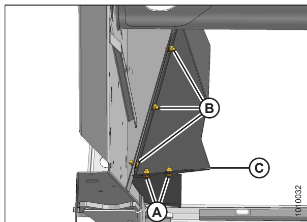
Рисунок 5.134: Задний дефлектор
