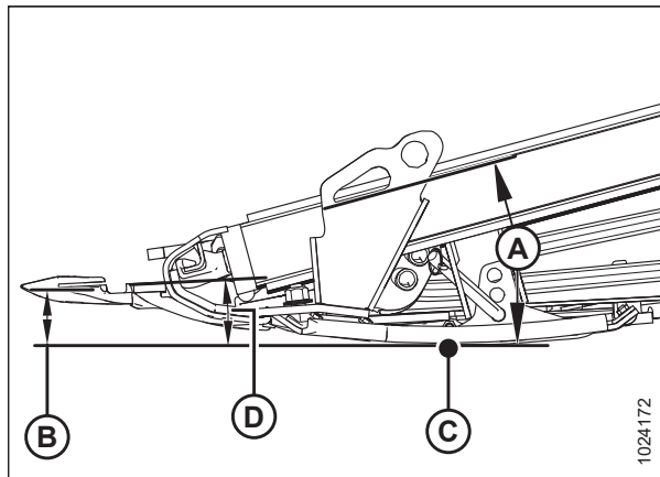
Рисунок 3.38: Угол атаки жатки
