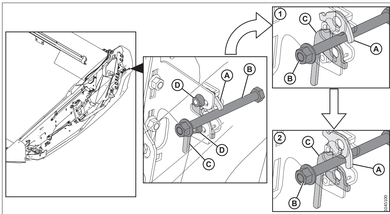
Рисунок 3.19: Защелка двухэтапной фиксации бокового щитка
