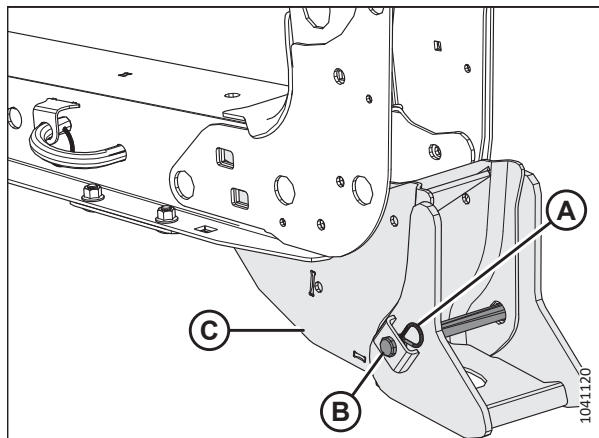
Рисунок 4.80: Лапа и опора жатки
