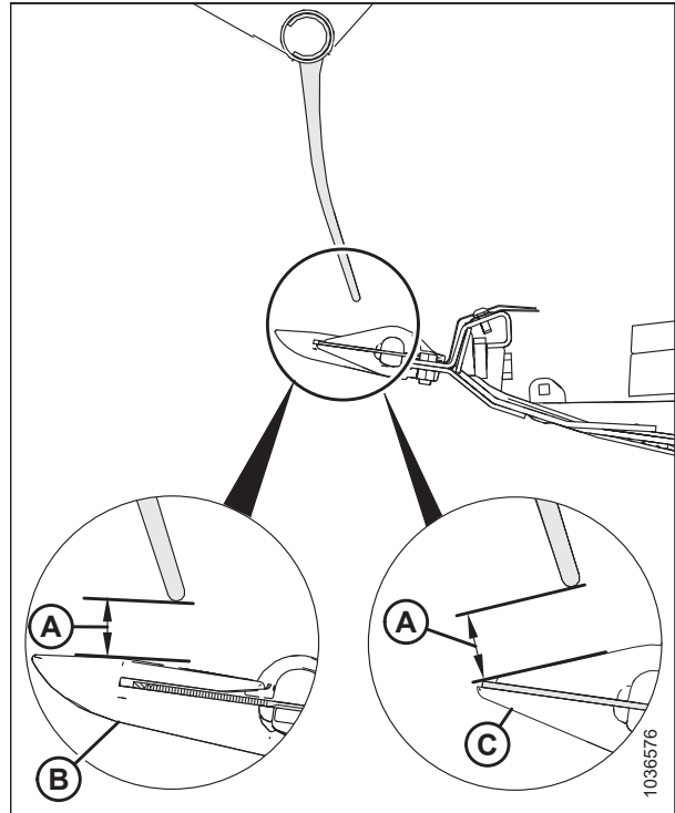
Рисунок 5.136: Измерение расстояния от конца пальца до противорежущего пальца
