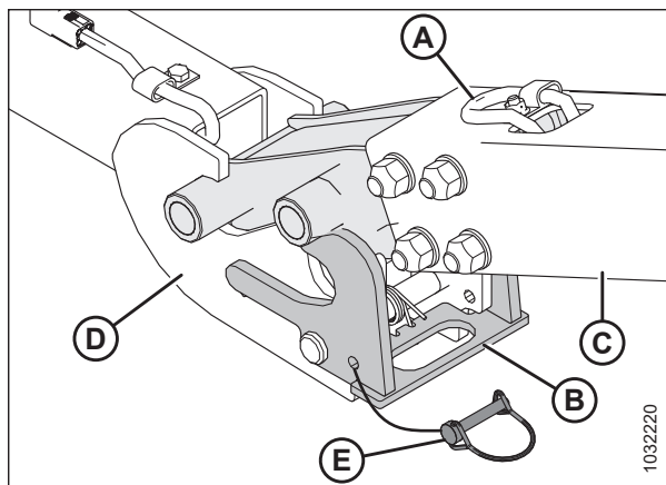
Рисунок 3.132: Буксирная тяга к удлинителю
