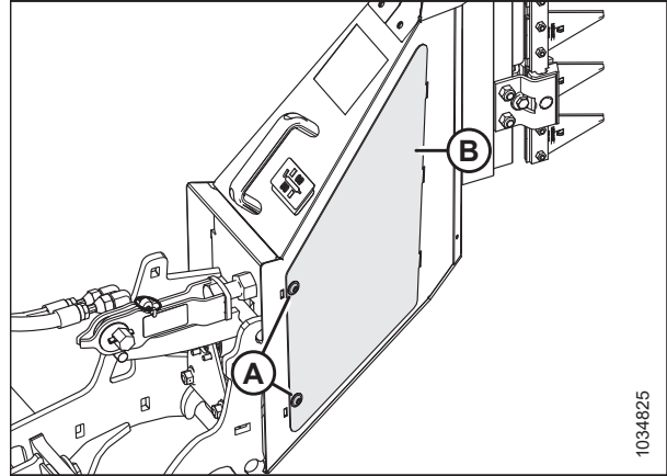
Рисунок 5.242: Крышка доступа к вертикальному ножу
