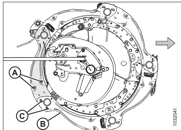
Рисунок 5.186: Боковые щитки мотовила — внешняя сторона эксцентрика
