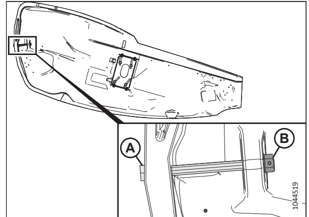
Рисунок 3.20: Болт бокового щитка
