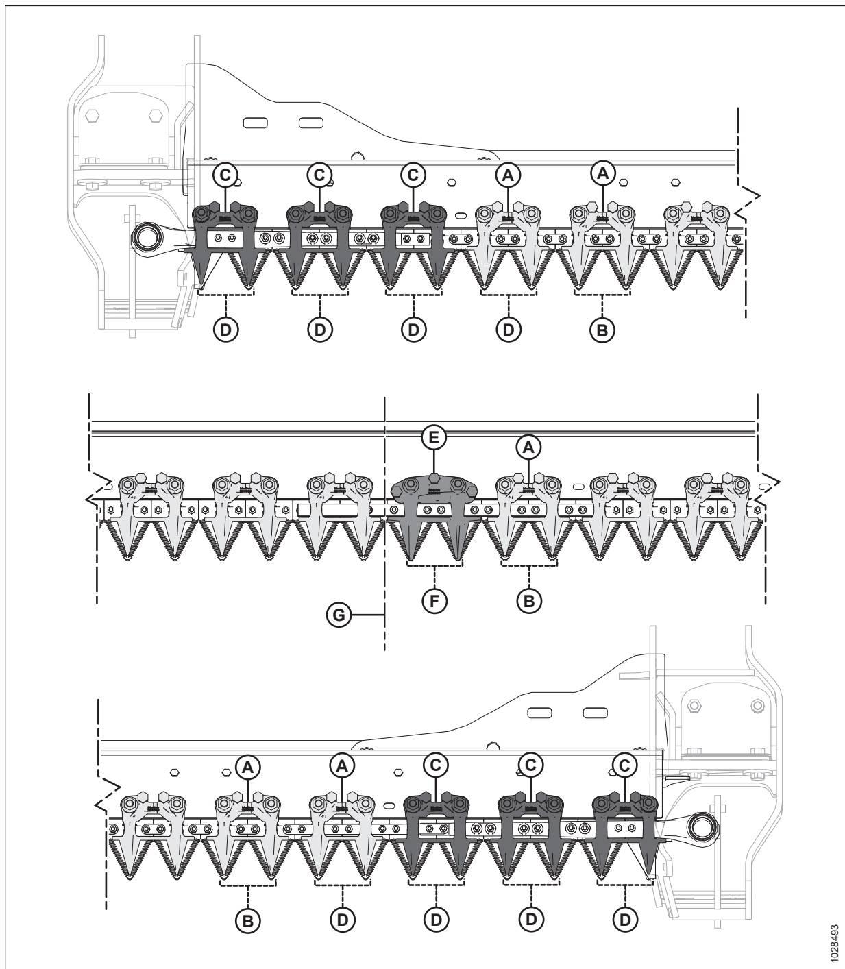
Рисунок 5.68: Расположение укороченных противорежущих пальцев и прижимов
