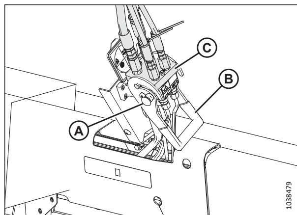
Рисунок 4.56: Подключение гидравлики мотовила
