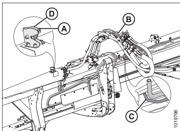
Рисунок 4.100: Система укладки гидравлических шлангов — все жатки, кроме D215
