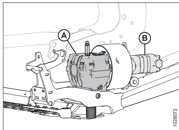
Рисунок 5.84: Показан левый редуктор привода ножа (правый аналогичен левому)
