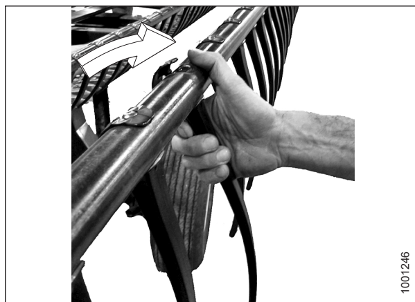
Рисунок 5.150: Установка пластмассового пальца
