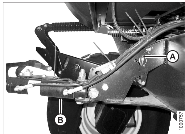
Рисунок 4.24: Гидравлическое центральное соединение без комплекта самовыравнивания
