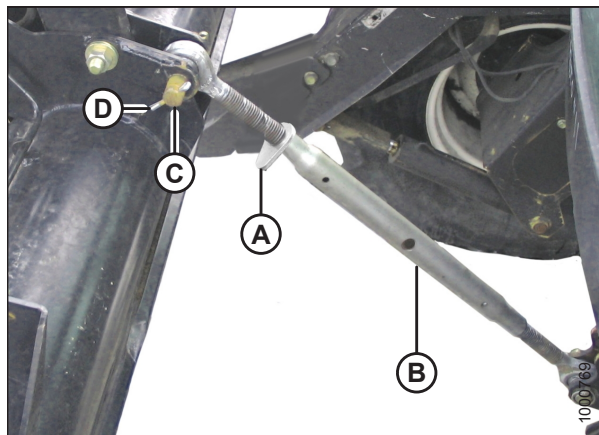
Рисунок 4.42: Механическое центральное соединение
