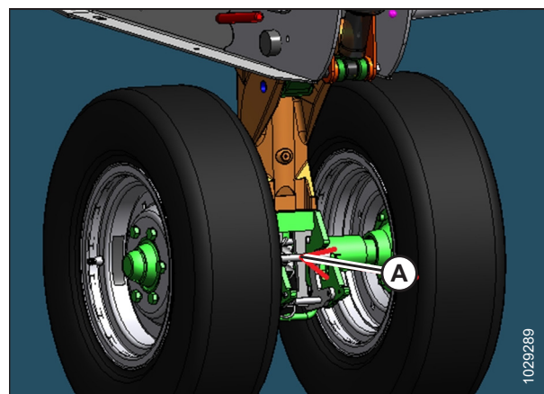
Рисунок 3.119: Передние транспортные колеса
