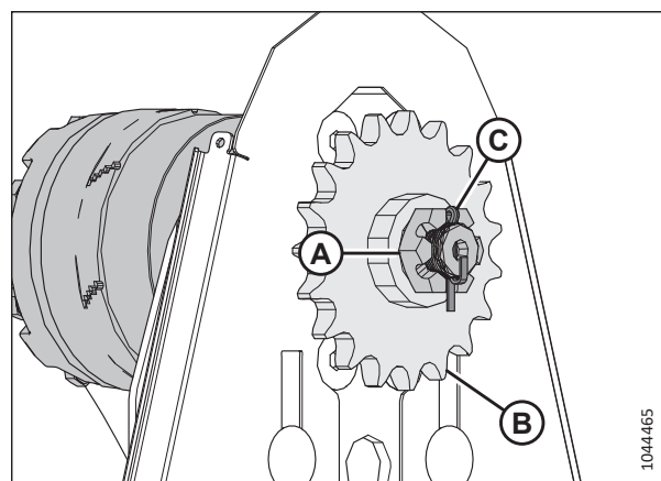
Рисунок 5.214: Одиночная звездочка
