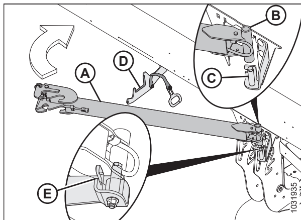
Рисунок 3.104: Место хранения удлиннителя буксирной тяги
