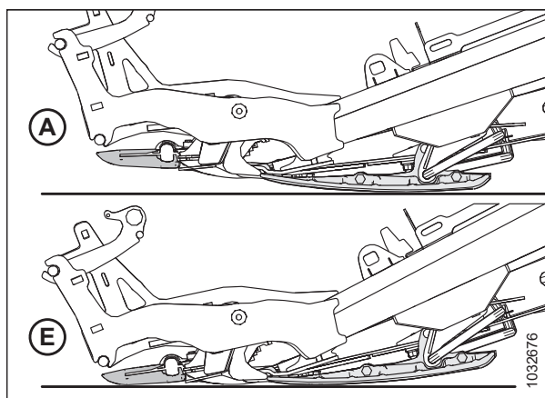
Рисунок 3.39: Углы противорезающих пальцев
