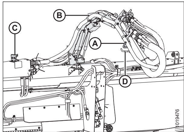
Рисунок 4.167: Система укладки гидравлических шлангов
