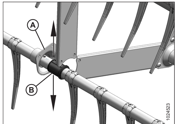
Рисунок 5.165: Противоположная опора комплекта усиления граблей
