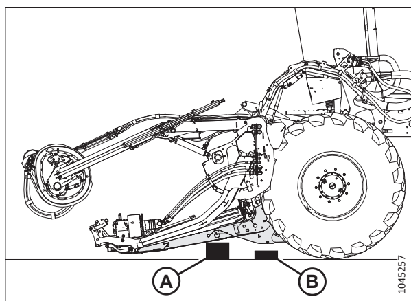
Рисунок 4.152: Установка жатки на грунт
