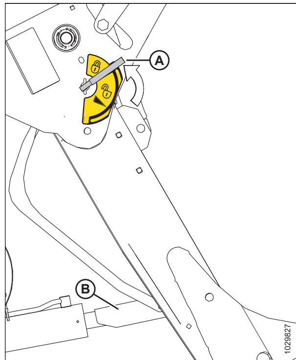
Рисунок 4.14: Предохранительный упор
