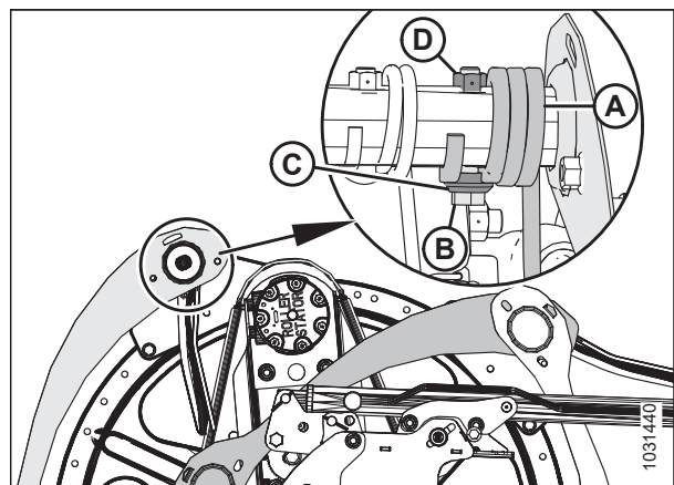
Рисунок 5.201: Боковые щитки мотовила — внутренняя сторона хвостовика
