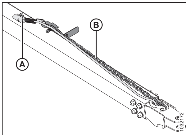
Рисунок 3.95: Сборка буксирной тяги
