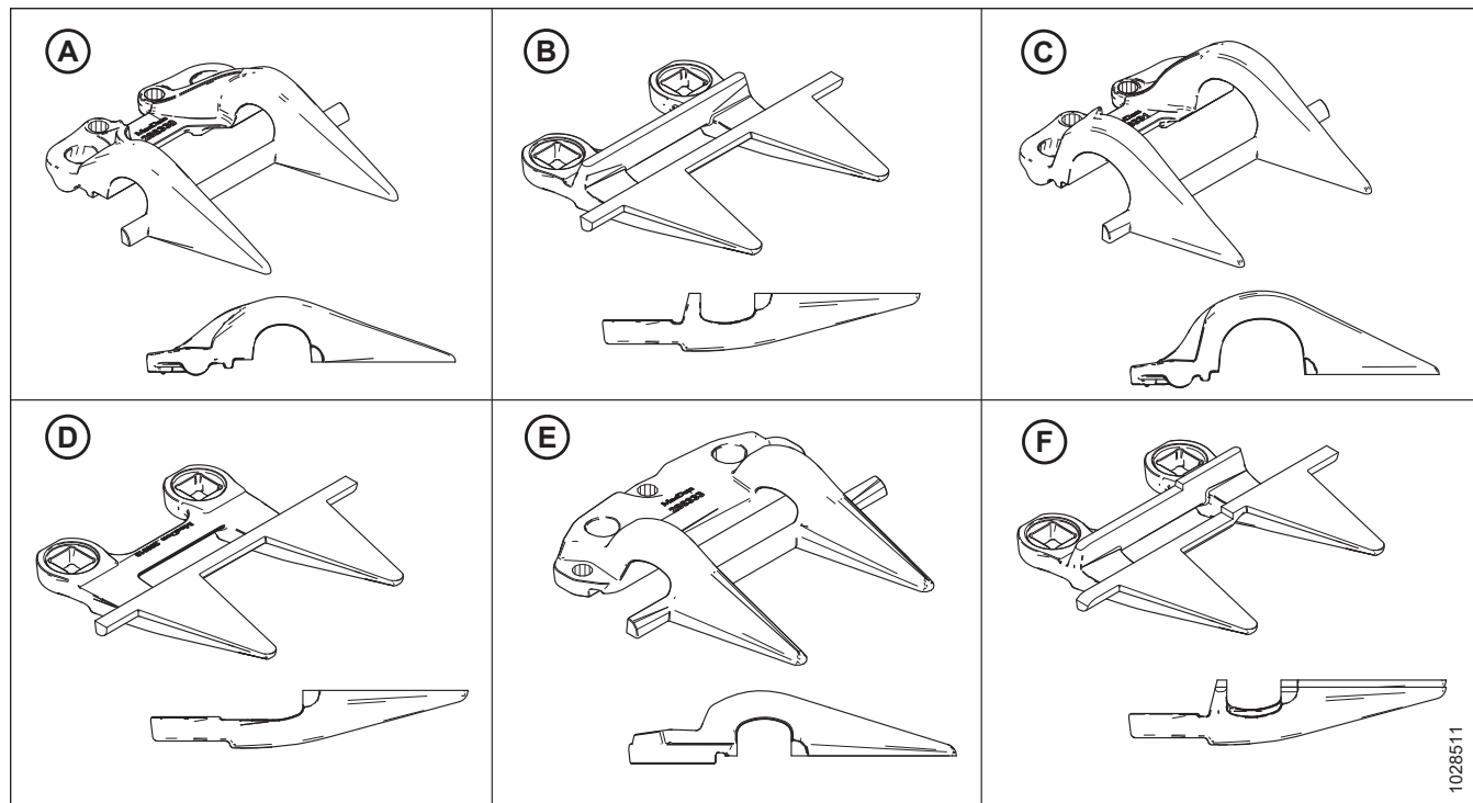
Рисунок 5.65: Типы противорезущих пальцев и прижимов, используемых в укороченных конфигурациях
