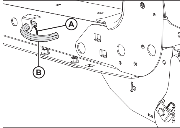
Рисунок 4.16: Опора жатки
