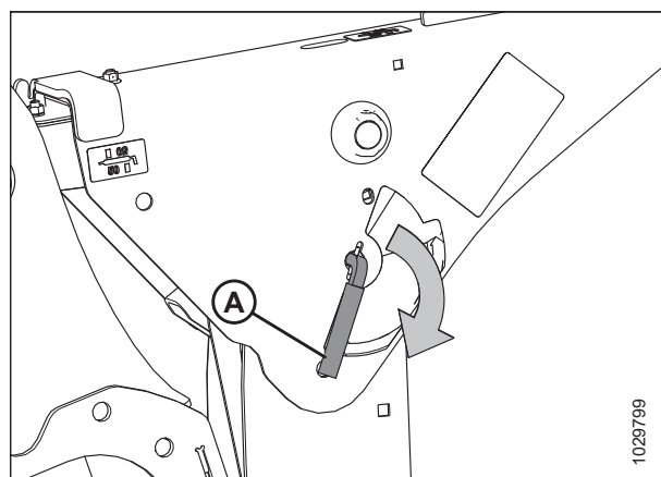
Рисунок 4.97: Рычаг предохранительного упора
