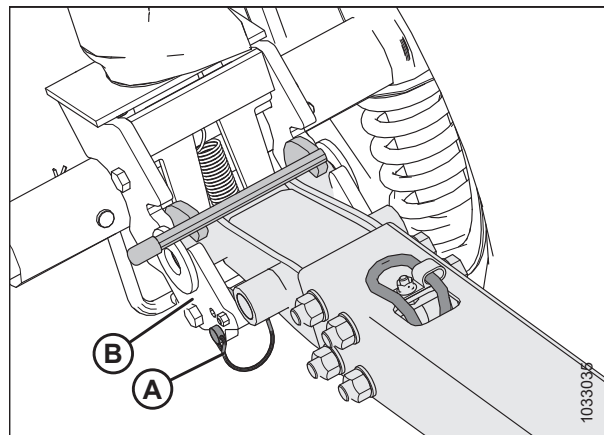
Рисунок 3.102: Буксирная тяга и левый транспортный шарнир
