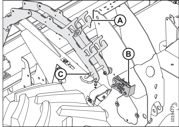
Рисунок 4.166: Система укладки гидравлических шлангов
