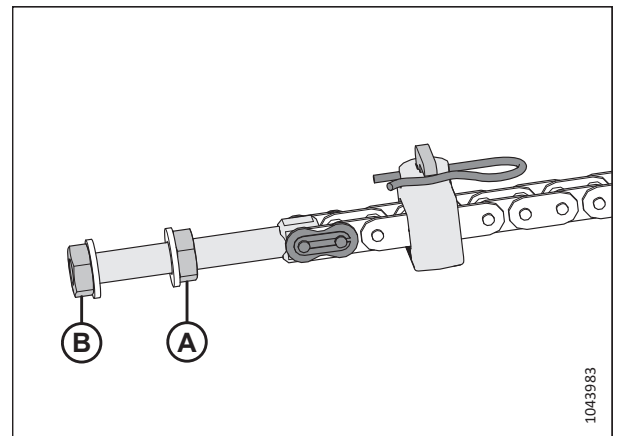
Рисунок 3.88: Левый болт регулировки цепи — правый аналогичен
