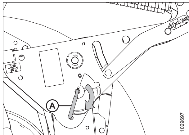
Рисунок 4.77: Предохранительный упор
