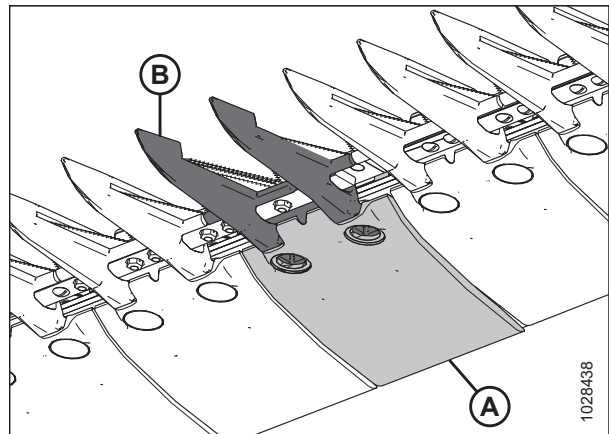
Рисунок 5.60: Заостренный центральный противорежущий палец и износная пластина
