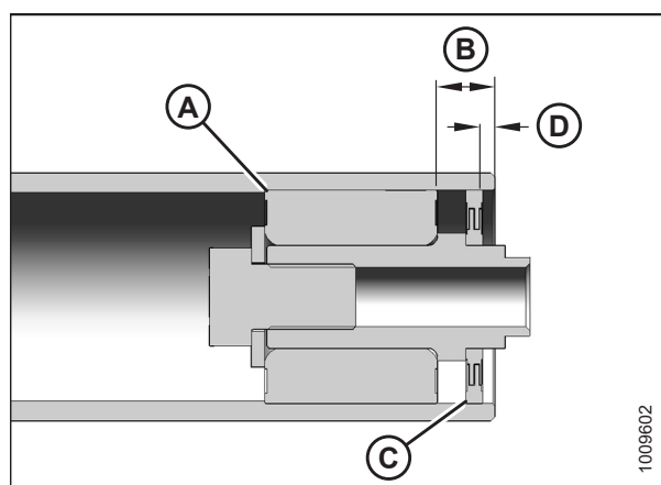
Рисунок 5.119: Роликовый подшипник
