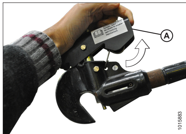
Рисунок 4.119: Центральное соединение
