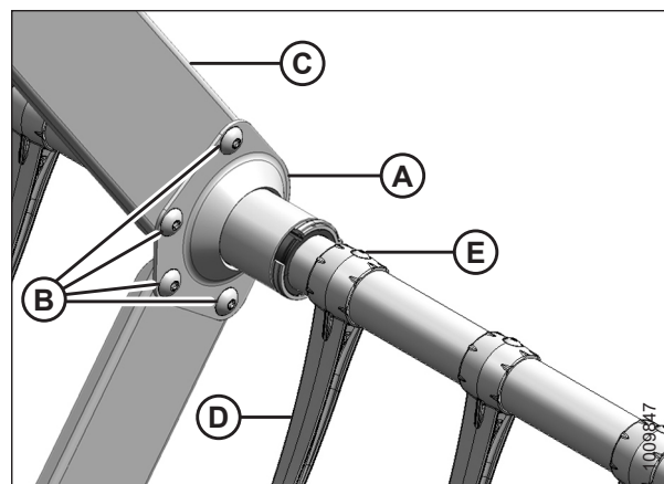
Рисунок 5.182: Опора комплекта усиления граблин мотовила (опция)
