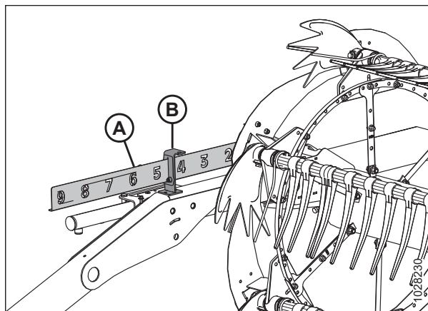
Рисунок 3.45: Индикатор продольного перемещения
