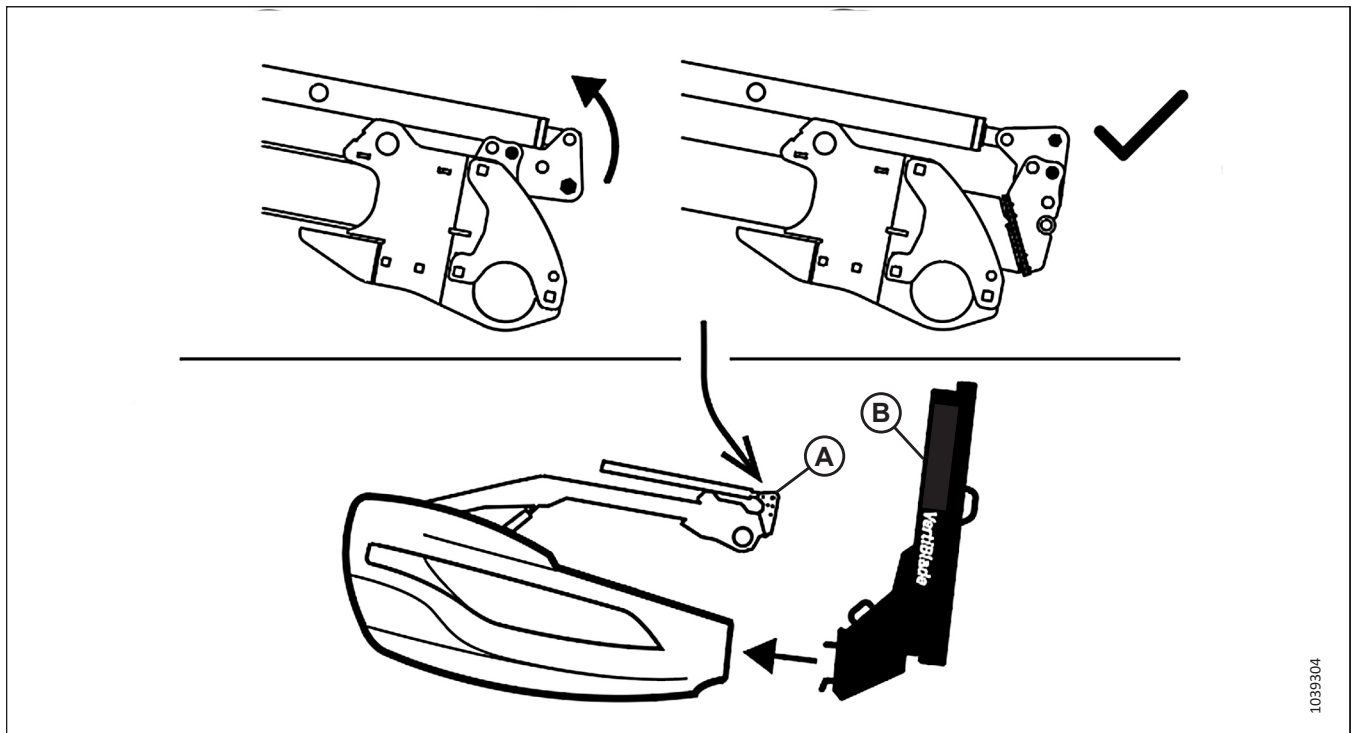
Рисунок 3.47: Положение мотовила с установленной опцией вертикального ножа
