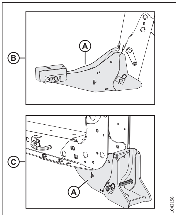
Рисунок 4.125: Монтаж опор жатки
