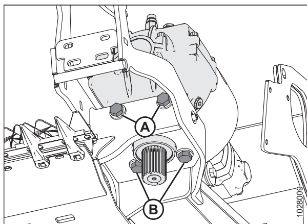
Рисунок 5.86: Редуктор привода ножа — вид снизу
