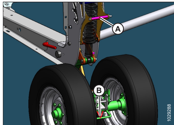
Рисунок 3.118: Передние транспортные колеса
