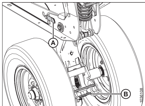
Рисунок 3.111: Левые транспортные колеса — шарнир освобожден
