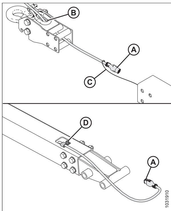
Рисунок 5.233: Установка кольцевого буксирного переходника
