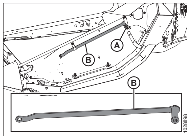
Рисунок 5.206: Место хранения универсального инструмента
