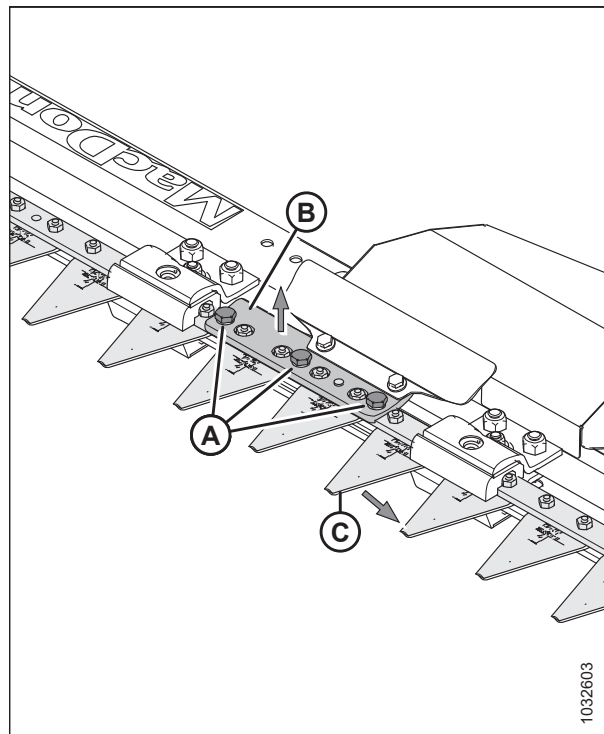
Рисунок 5.237: Вертикальный нож — противорежущий палец снят
