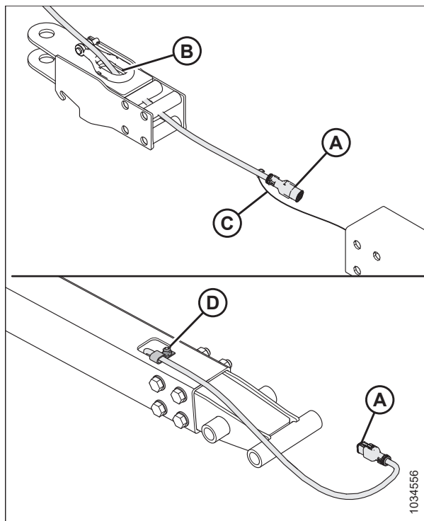
Рисунок 5.228: Установка вилочного буксирного переходника
