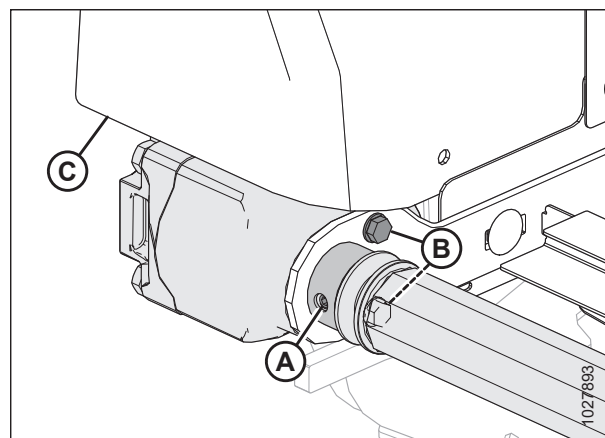
Рисунок 5.121: Приводной ролик
