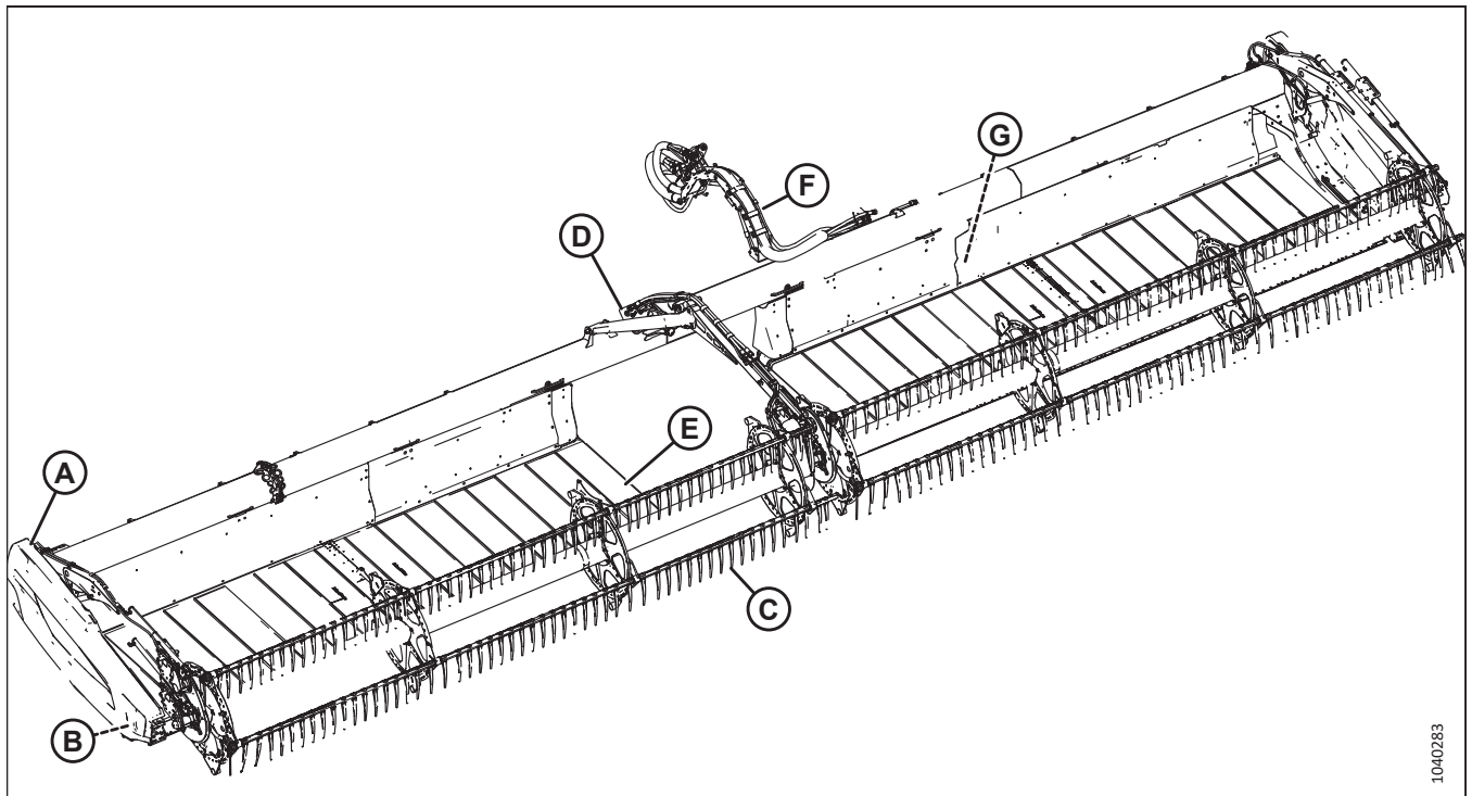
Рисунок 2.2: Полотняная жатка серии D2 — показано двойное мотовило
