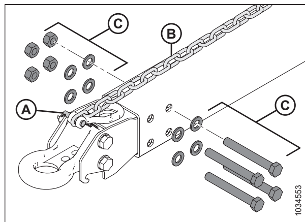
Рисунок 5.226: Снятие кольцевого буксирного переходника
