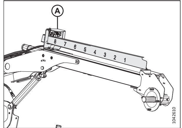
Рисунок 3.57: Датчик положения вперед/назад
