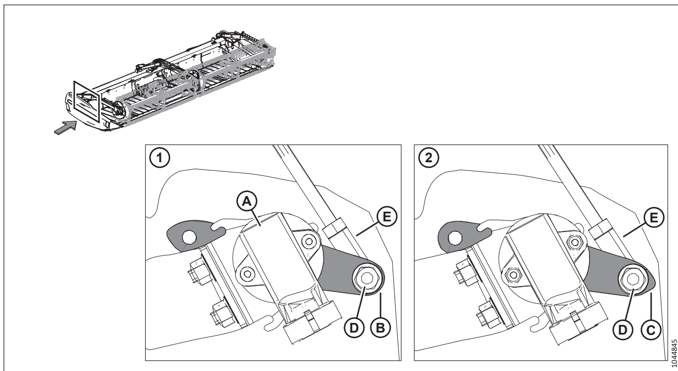
Рисунок 3.42: Расположение датчика высоты мотовила
