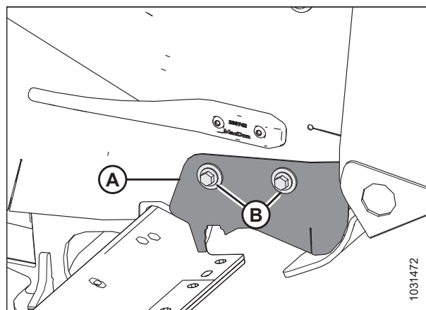
Рисунок 5.83: Защита головки ножа
