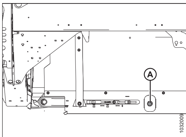
Рисунок 5.112: Натяжитель полотна
