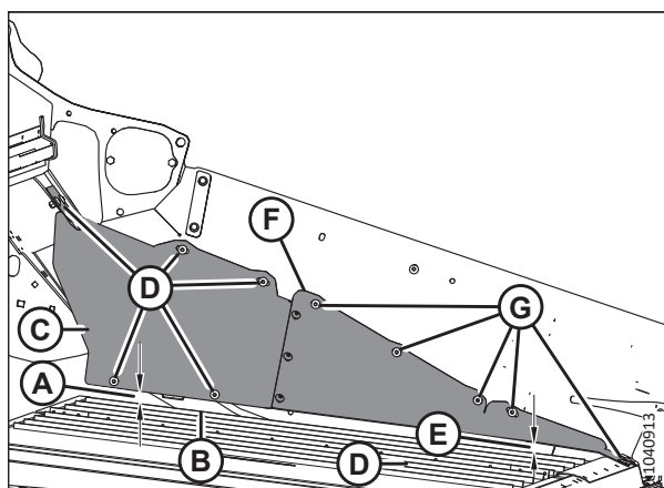
Рисунок 5.130: Дефлекторы — показана левая сторона
