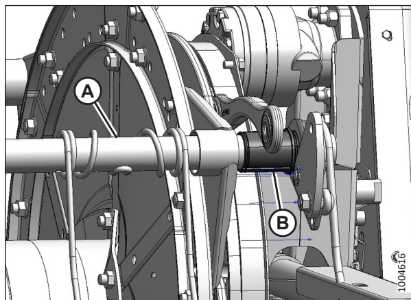
Рисунок 5.167: Сторона эксцентрика
