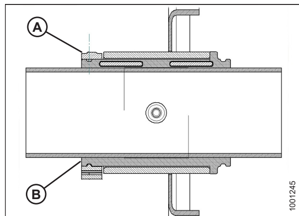
Рисунок 5.174: Втулка
