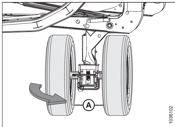
Рисунок 3.108: Левые транспортные колеса в транспортном режиме
