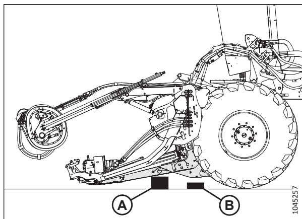
Рисунок 4.117: Установка жатки на грунт
