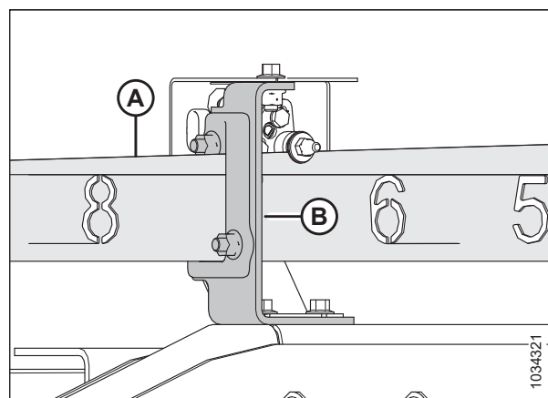
Рисунок 5.135: Продольное положение
