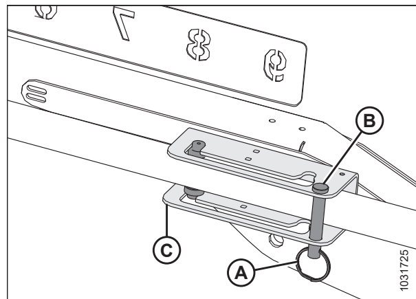
Рисунок 3.53: Регулировка цилиндра перемещения вперед/назад, тип 2 — переднее положение
