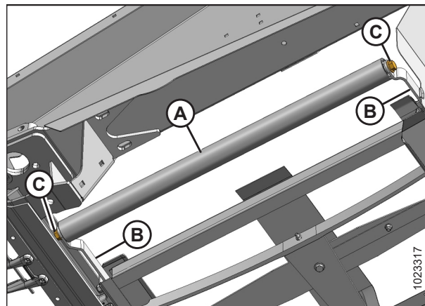
Рисунок 5.110: Натяжной ролик
