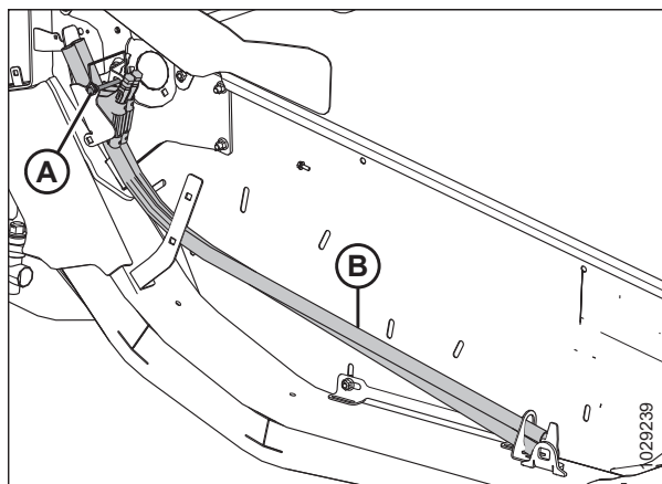
Рисунок 3.79: Правая боковина
