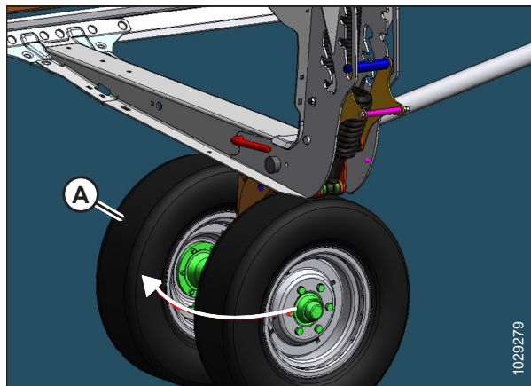
Рисунок 3.121: Передние транспортные колеса
