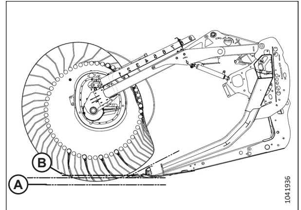
Рисунок 3.61: Профиль пальцев — положение эксцентрика 3
