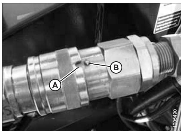
Рисунок 4.60: Быстроразъемное соединение
