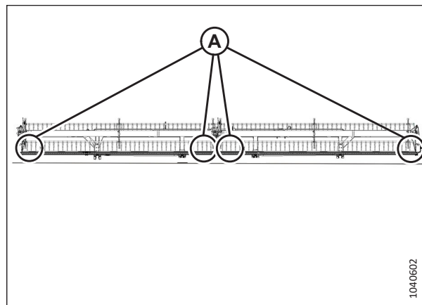
Рисунок 5.138: Расположение точек замера для жатки со сдвоенным мотовилом
