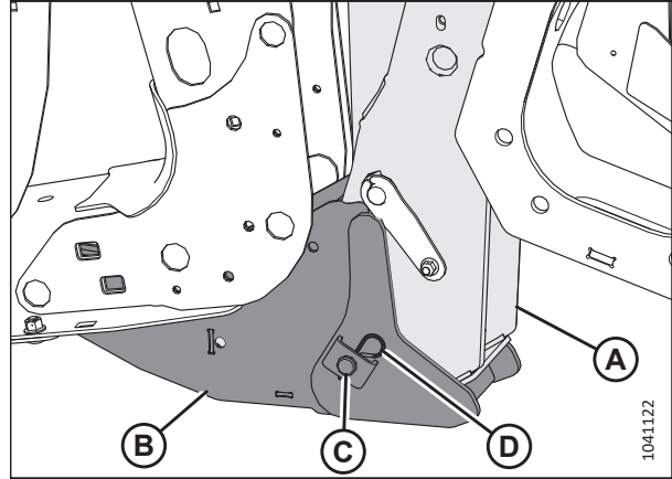
Рисунок 4.75: Лапа жатки и подъемное соединение косилки, соединенные опорой жатки
