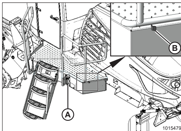
Рисунок 4.99: Левая платформа
