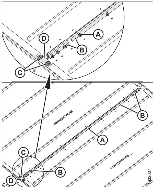
Рисунок 5.122: Стыковочная планка полотна
