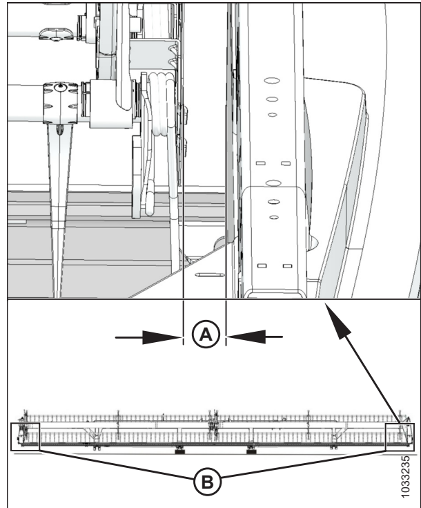
Рисунок 5.144: Зазор между мотовилом и боковиной жатки
