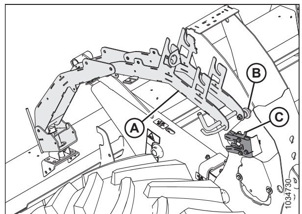
Рисунок 4.103: Левая наружная опора косилки
