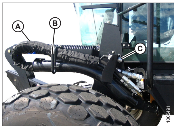
Рисунок 4.61: Место хранения шлангов
