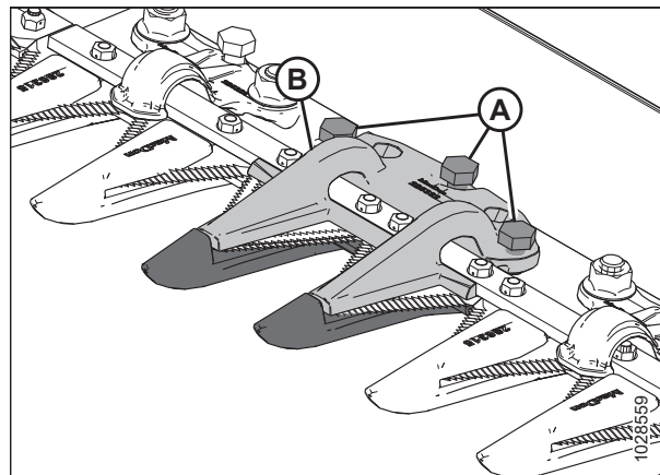
Рисунок 5.61: Заостренный центральный противорежущий палец
