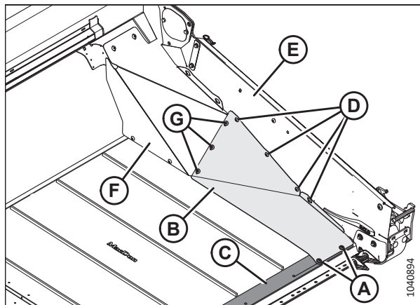
Рисунок 5.124: Широкие дефлекторы — показана левая сторона
