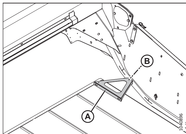
Рисунок 5.127: Накладка — показана левая сторона
