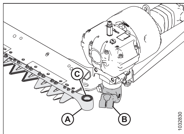
Рисунок 5.34: Левая головка ножа
