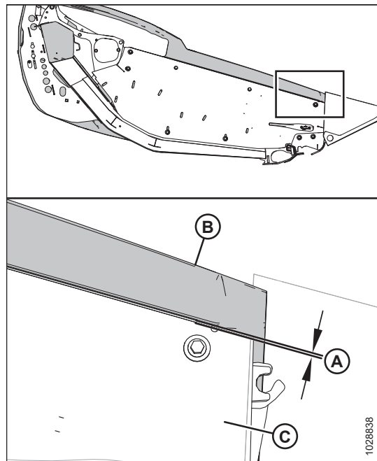
Рисунок 3.14: Зазор между боковым щитком и боковиной
