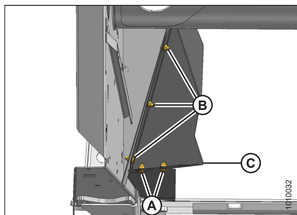
Рисунок 5.131: Задний дефлектор
