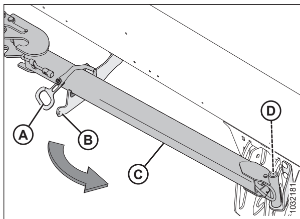
Рисунок 3.127: Удлинитель буксирной тяги в месте для хранения
