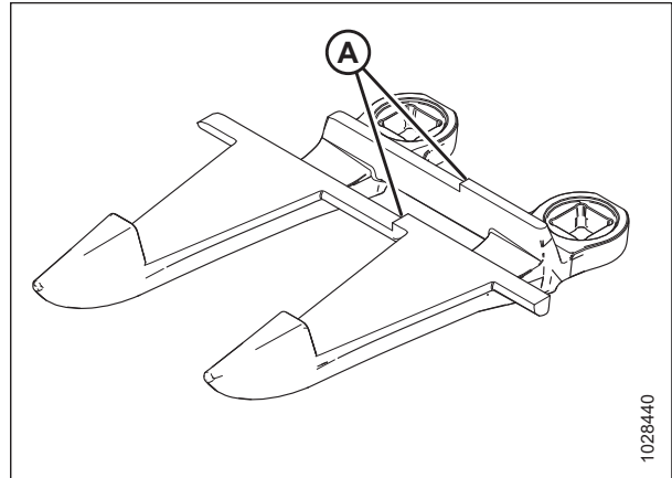
Рисунок 5.58: Заостренный центральный противорежущий палец
