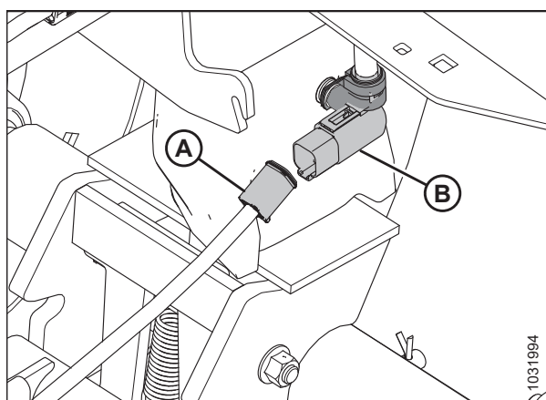
Рисунок 3.101: Электрическое соединение буксирной тяги
