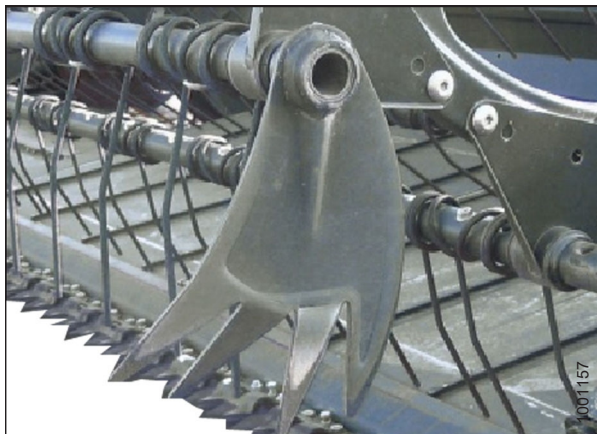
Рисунок 6.6: Палец для полеглых культур
