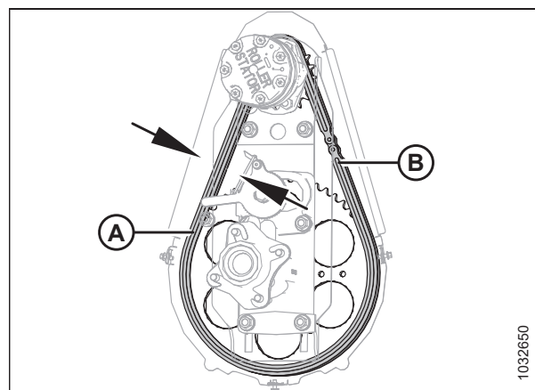
Рисунок 5.210: Привод мотопила
