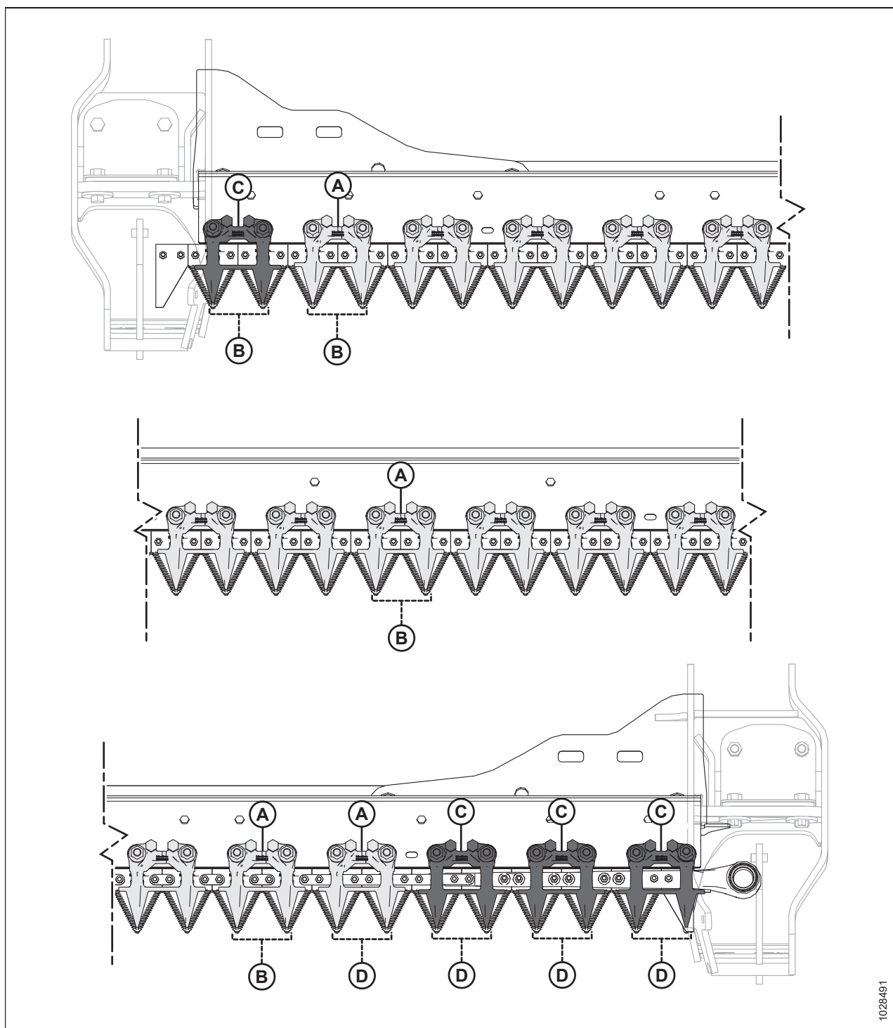
Рисунок 5.66: Местоположение укороченных противорезущих пальцев и прижимов — жатки с одинарными ножами
