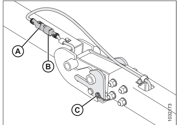
Рисунок 3.96: Жгут проводов буксирной тяги/ удлинителя
