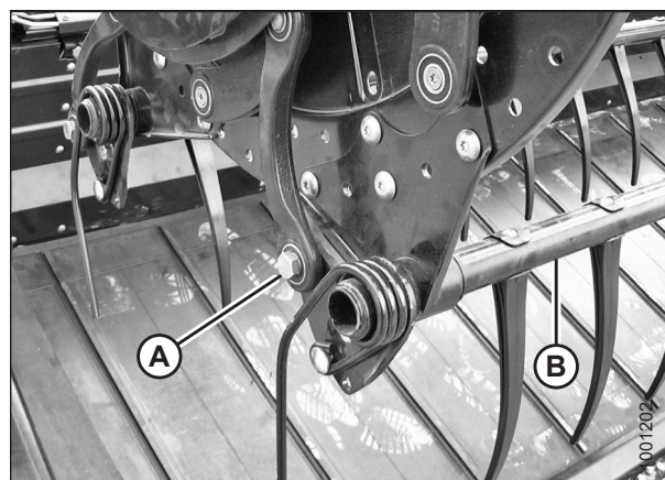
Рисунок 5.158: Сторона эксцентрика
