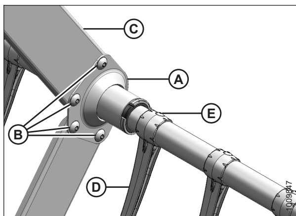
Рисунок 5.161: Опора граблины
