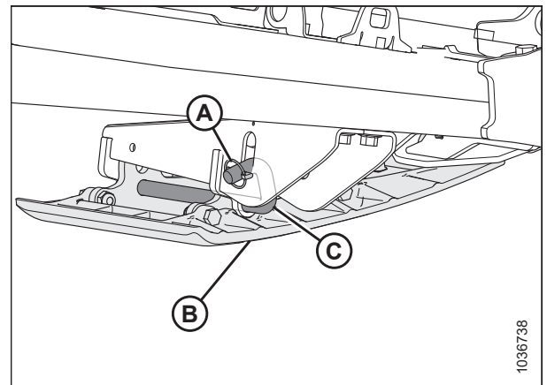
Рисунок 3.37: Внешний копирующий башмак
