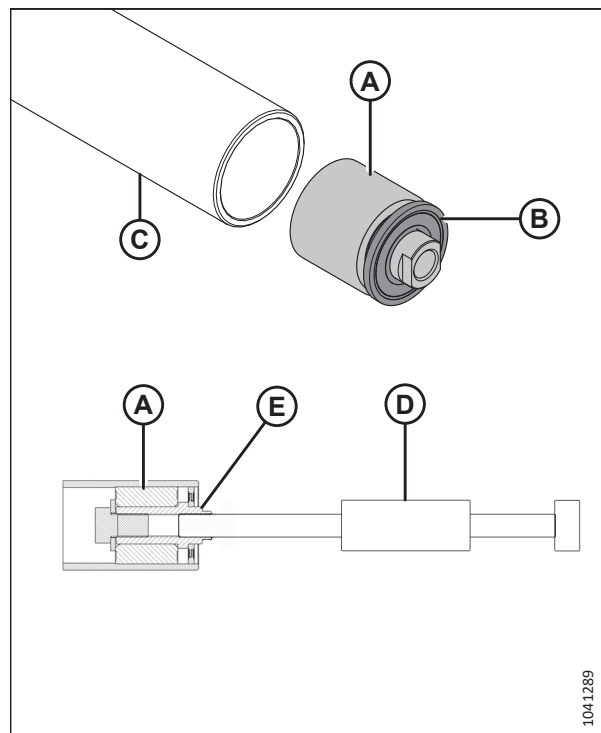
Рисунок 5.105: Подшипник и уплотнение натяжного ролика
