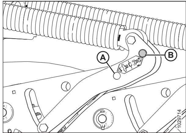
Рисунок 4.36: Рычаги флотации жатки
