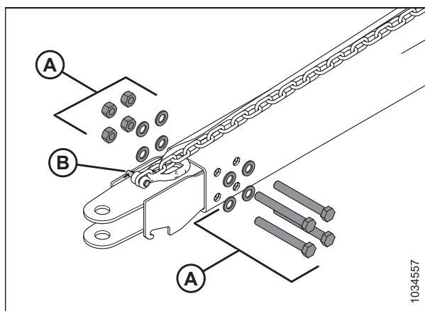
Рисунок 5.229: Установка вилочного буксирного переходника
