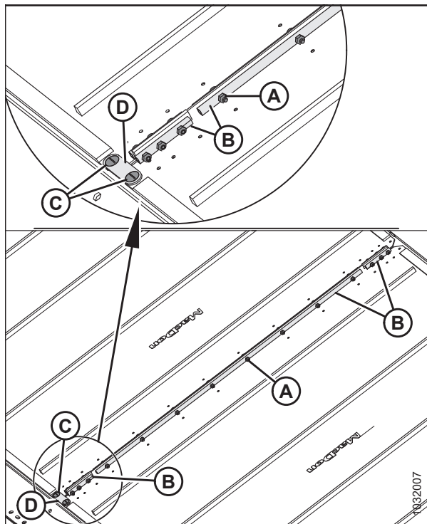
Рисунок 5.91: Стыковочные планки полотна
