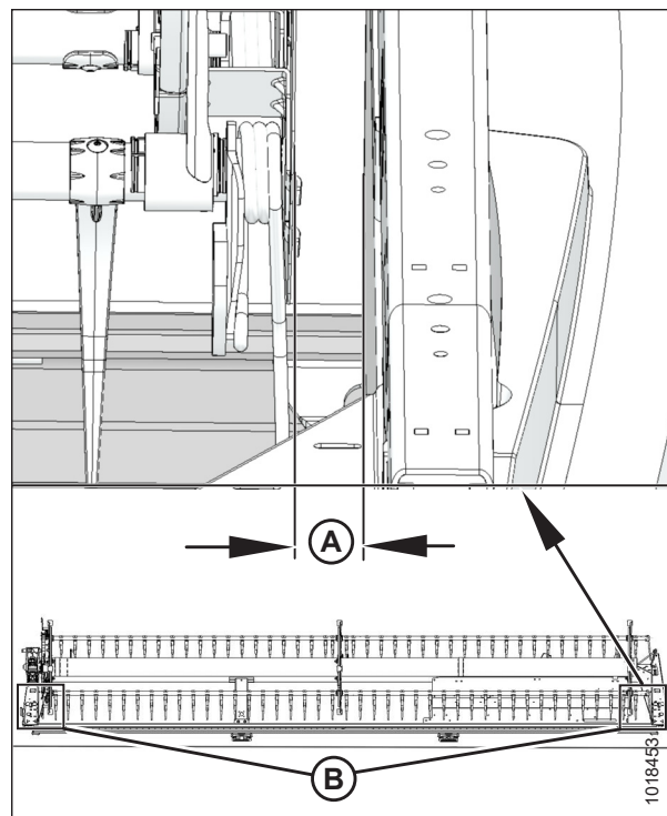
Рисунок 5.142: Зазор между мотовилом и боковиной жатки
