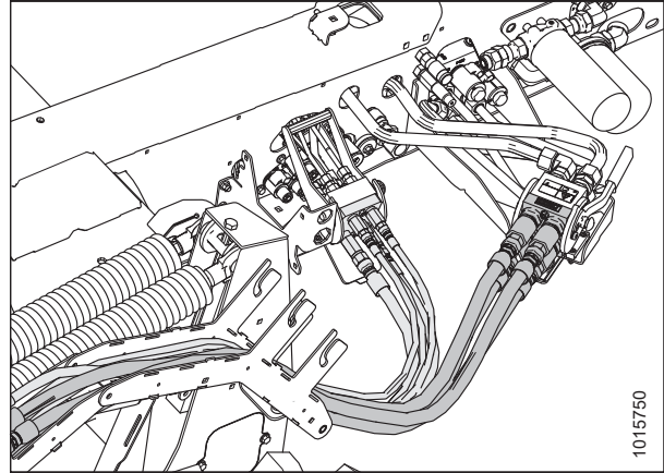
Рисунок 4.146: Гидравлические многоканальные муфты и прокладка шлангов
