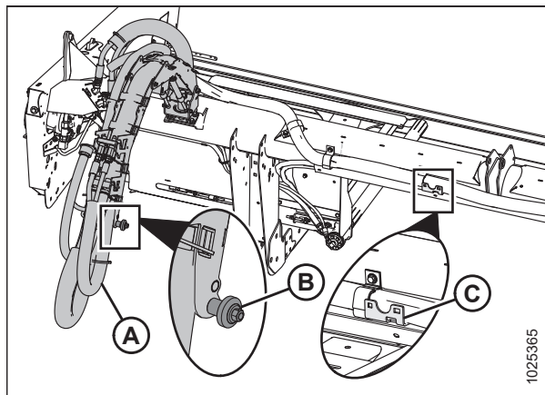
Рисунок 4.140: Система укладки гидравлических шлангов — полотняная жатка D215
