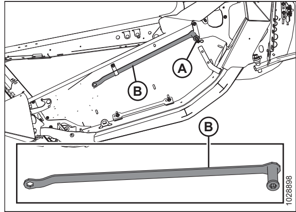
Рисунок 3.48: Левая торцевая обшивка
