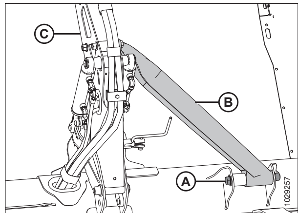
Рисунок 5.145: Центральный опорный рычаг сдвоенного мотовила
