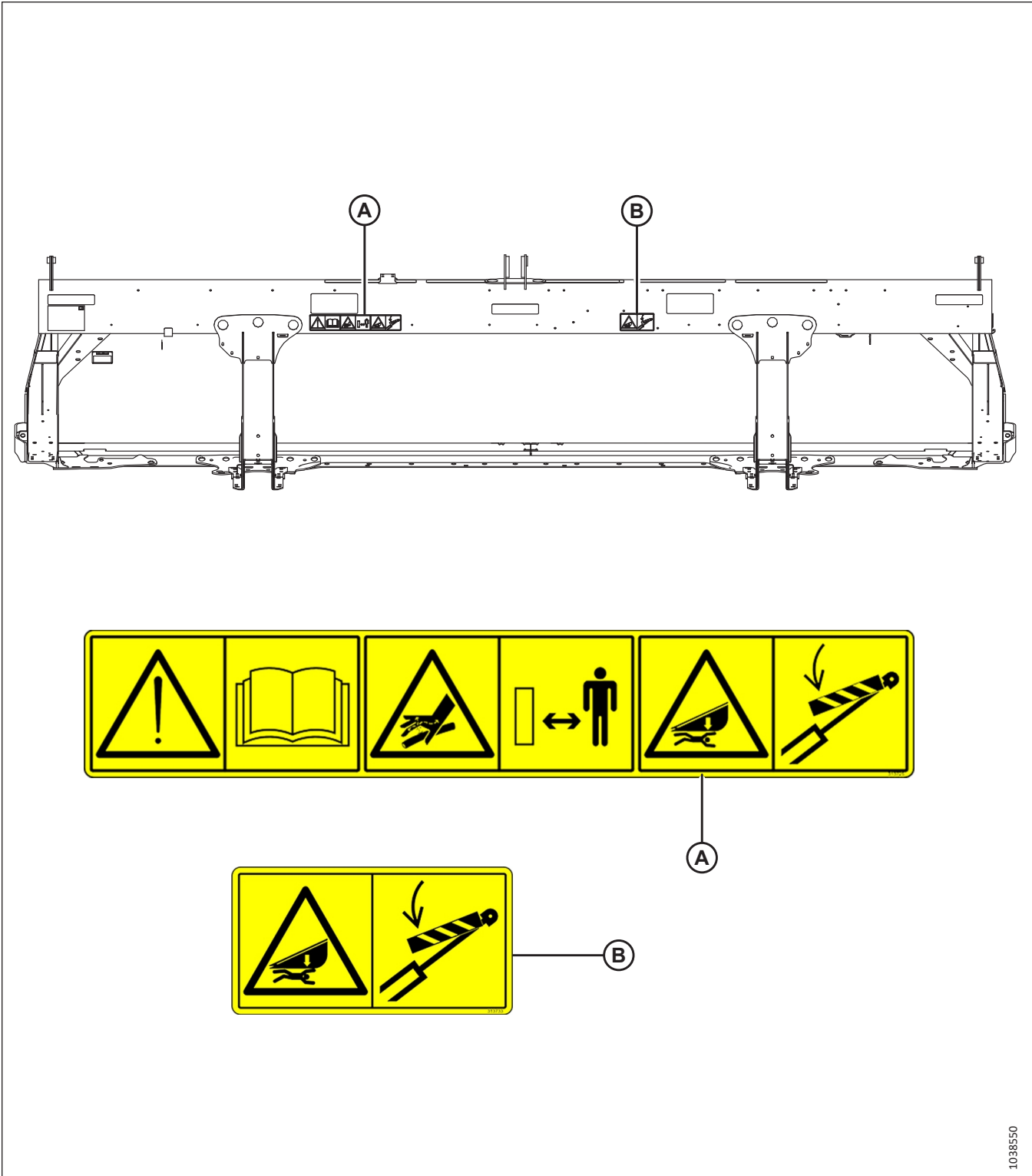
Рисунок 1.22: Задняя труба — Полотняная жатка D215
