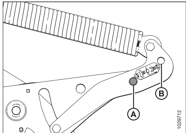
Рисунок 4.33: Рычаги флотации жатки
