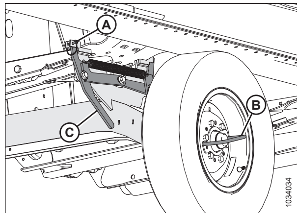
Рисунок 3.114: Правая транспортная ось зафиксирована в транспортном положении
