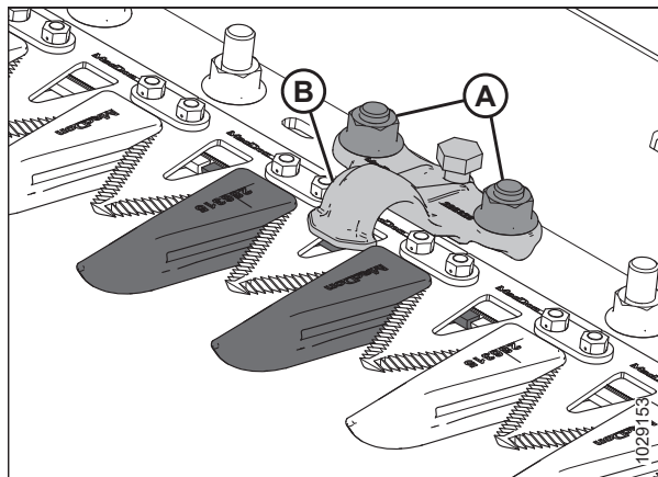
Рисунок 5.31: Ножевой брус
