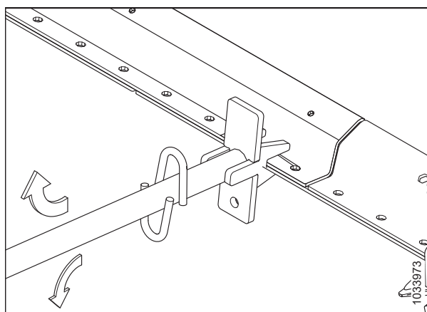
Рисунок 5.50: Регулировка пальцевого бруса — без противорежущих пальцев
