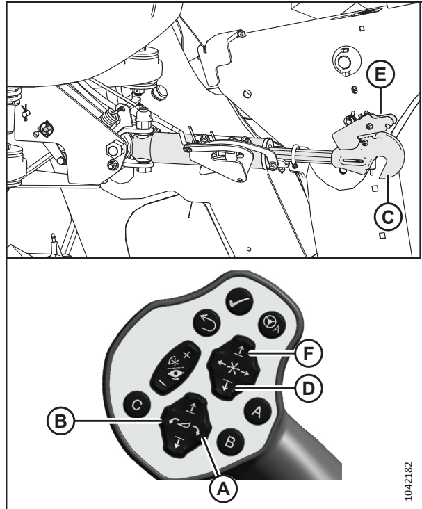
Рисунок 4.131: Гидравлическое центральное звено
