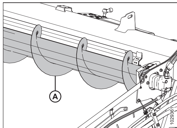
Рисунок 6.5: Верхний поперечный шнек
