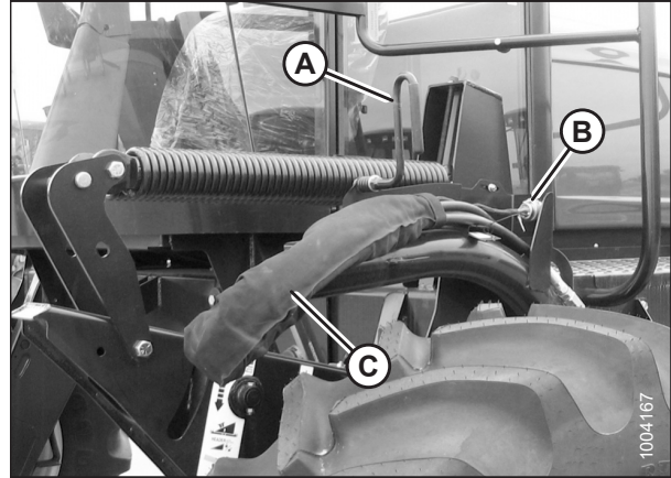
Рисунок 4.51: Шланги привода жатки
