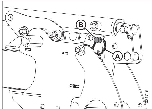
Рисунок 3.50: Регулировка цилиндра перемещения вперед/назад, тип 1 — переднее положение
