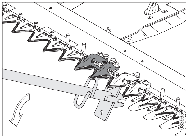
Рисунок 5.49: Регулировка смещением вниз — укороченный противорежущий палец
