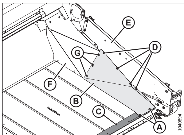
Рисунок 5.129: Широкие дефлекторы — показана левая сторона
