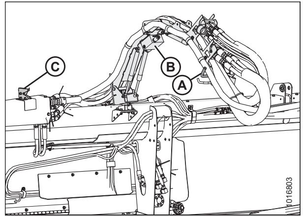
Рисунок 4.102: Система укладки гидравлических шлангов
