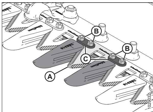
Рисунок 5.32: Ножевой брус
