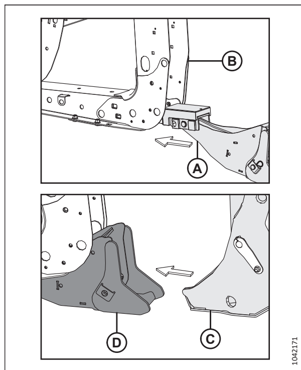
Рисунок 4.130: Лапа и опора жатки
