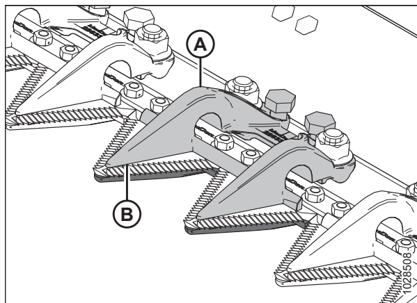
Рисунок 5.73: Укороченные противорежущие пальцы
