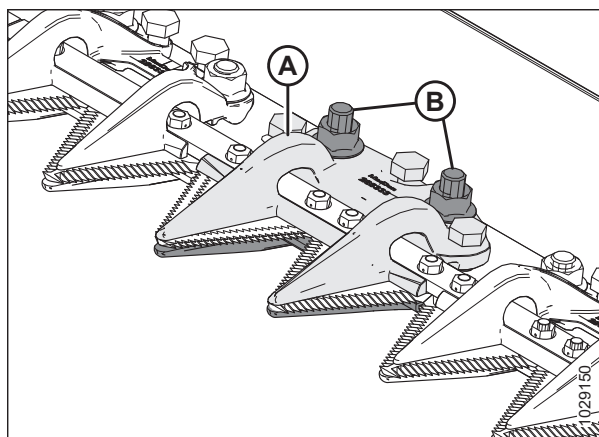
Рисунок 5.80: Центральный противорежущий палец
