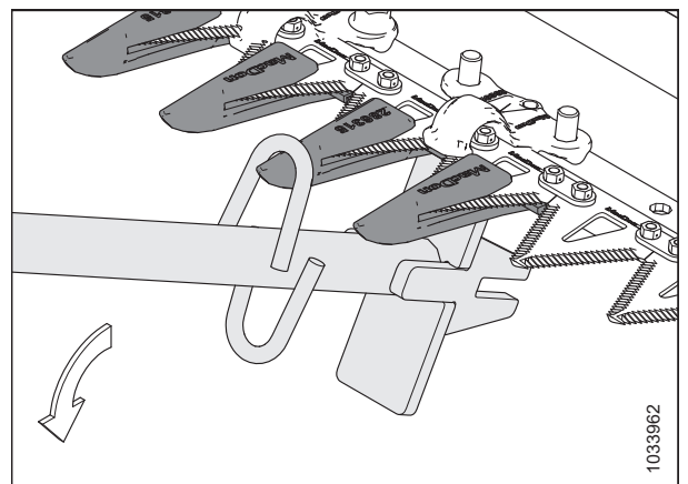
Рисунок 5.48: Регулировка смещением вниз — заостренный противорезающий палец
