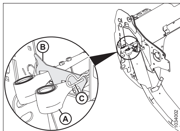
Рисунок 5.41: Запасные ножи
