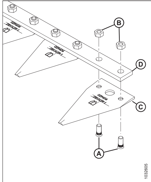
Рисунок 5.239: Узел секции ножа
