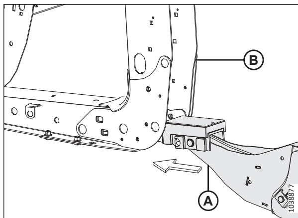
Рисунок 4.90: Лапа и опора жатки
