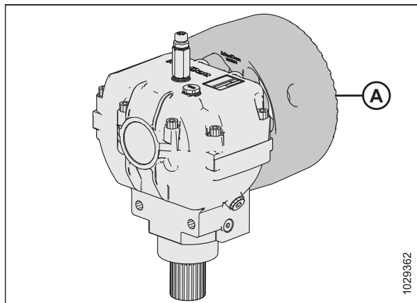
Рисунок 3.41: Маховик
