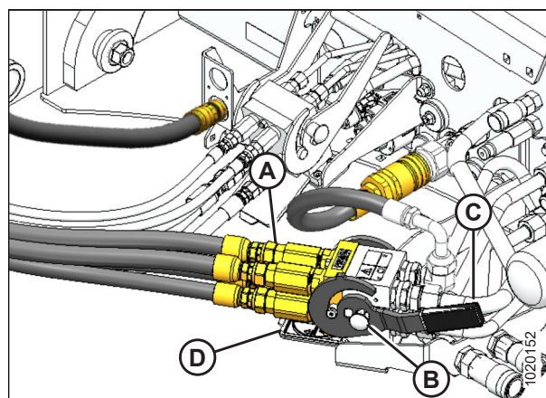
Рисунок 4.145: Многоканальная муфта ножа/ мотовила
