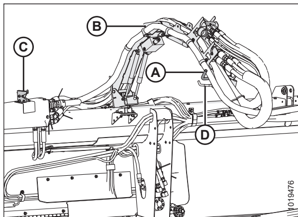
Рисунок 4.116: Система укладки гидравлических шлангов
