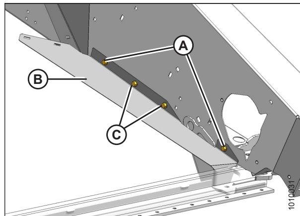
Рисунок 5.133: Передний дефлектор
