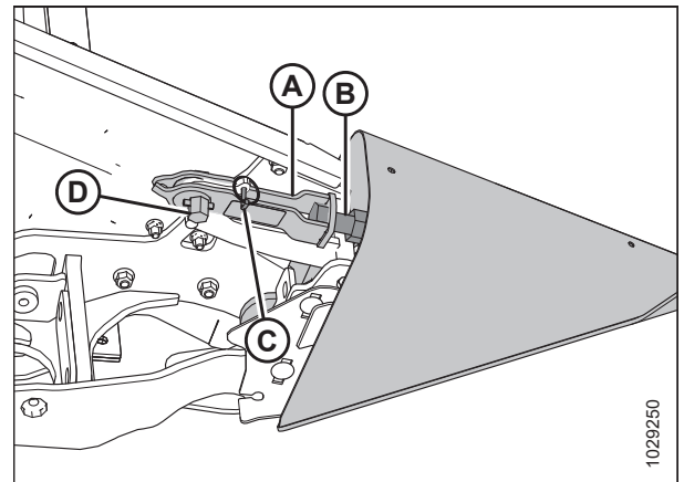
Рисунок 3.77: Делитель с опцией замка
