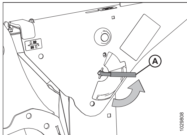
Рисунок 4.134: Рычаг предохранительного упора
