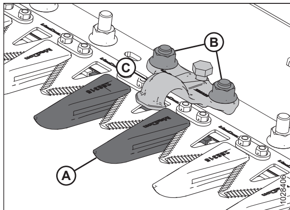
Рисунок 5.52: Заостренные противорежущие пальцы
