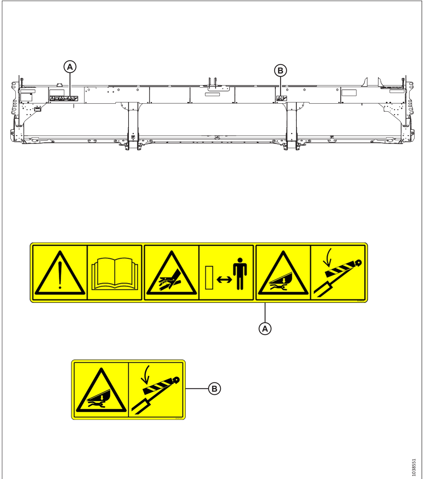
Рисунок 1.23: Задняя труба — Полотняная жатка D220
