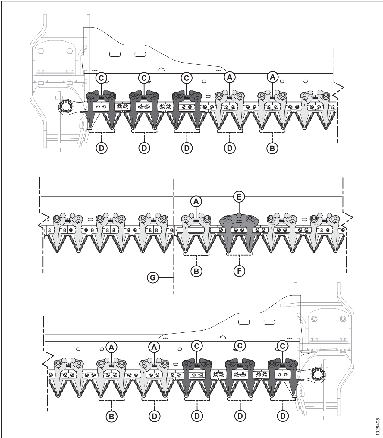
Рисунок 5.67: Местоположение укороченных противорежущих пальцев и прижимов — жатки с двойными ножами
