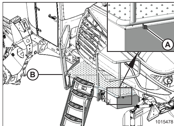
Рисунок 4.164: Левая платформа
