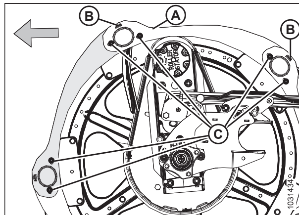
Рисунок 5.202: Боковые щитки мотовила — внутренняя сторона хвостовика
