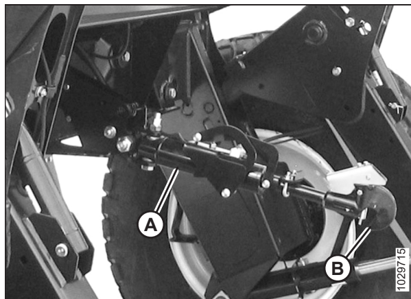
Рисунок 4.12: Гидравлическое центральное соединение
