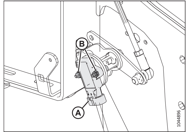
Рисунок 3.43: Датчик высоты мотовила: правый рычаг мотовила
