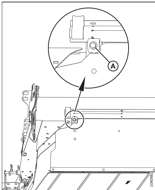
Рисунок 3.89: Механизм перемещения столов вручную
