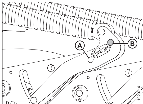
Рисунок 4.4: Рычаги флотации жатки
