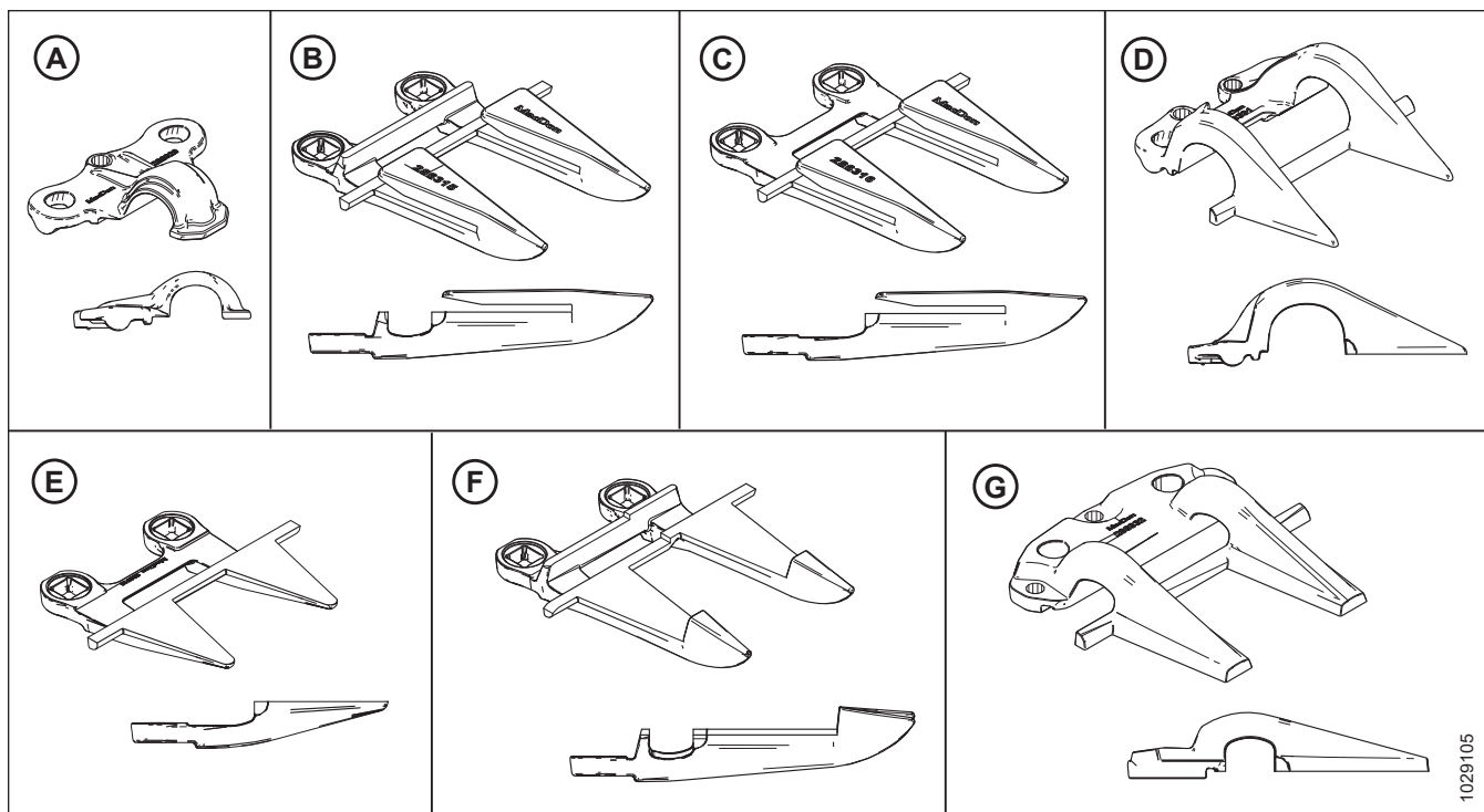
Рисунок 5.42: Типы противорезающих пальцев и прижимов, используемых в заостренных конфигурациях
