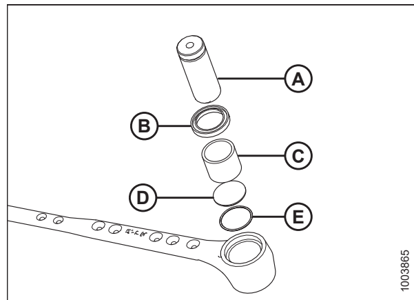
Рисунок 5.36: Подшипник головки ножа в сборе
