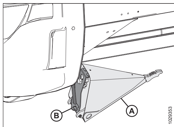
Рисунок 3.73: Дополнительное место для хранения делителей
