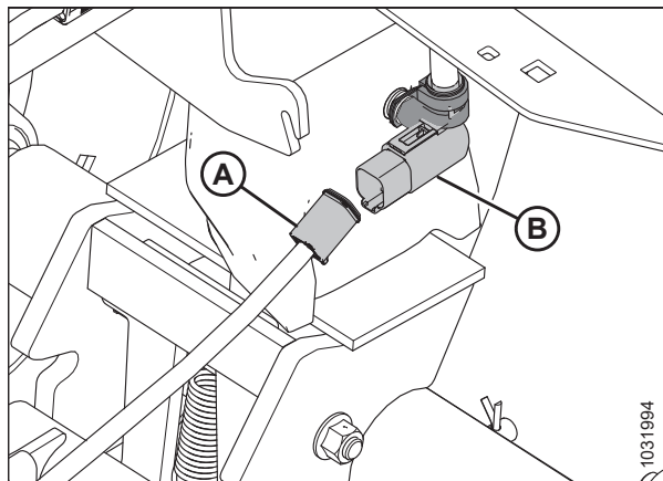
Рисунок 3.136: Электрическое соединение буксирной тяги
