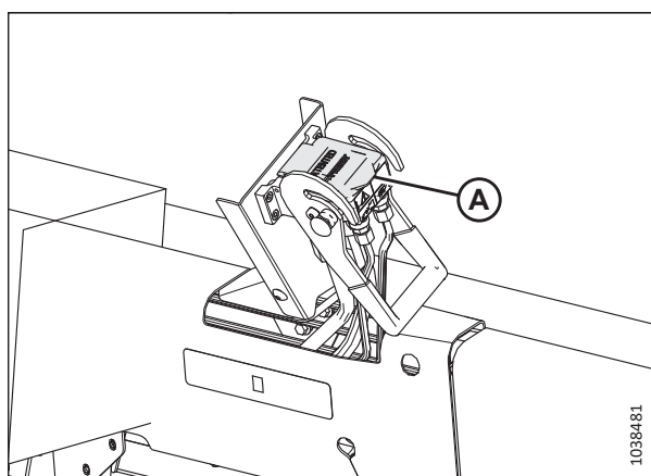
Рисунок 4.58: Закрытая крышка гнезда
