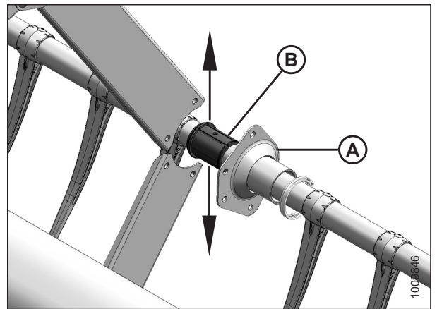
Рисунок 5.164: Опора комплекта усиления граблей
