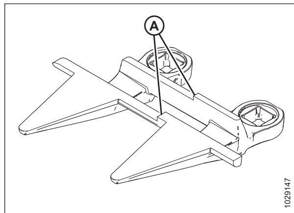
Рисунок 5.76: Центральный противорежущий палец
