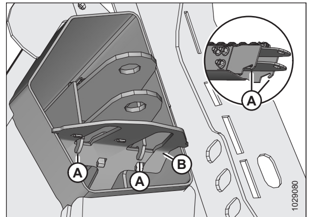
Рисунок 3.107: Удерживающие крюки на стороне вилки
