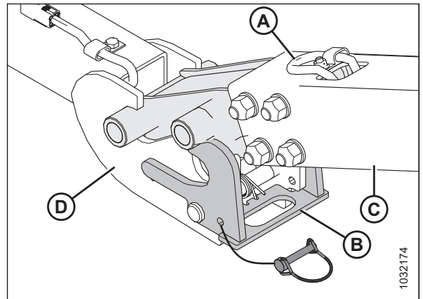
Рисунок 3.97: Буксирная тяга/место соединения удлинителя
