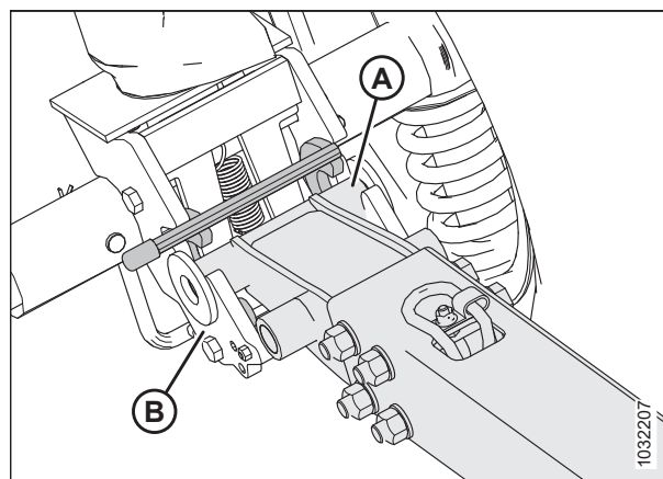
Рисунок 3.103: Буксирная тяга и левый транспортный шарнир
