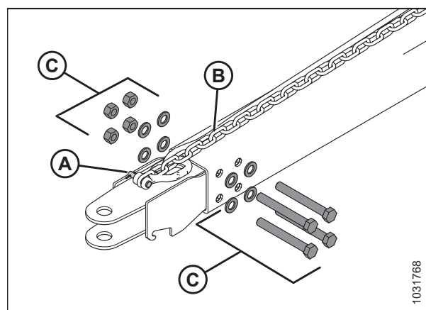
Рисунок 5.231: Снятие вилочного переходника
