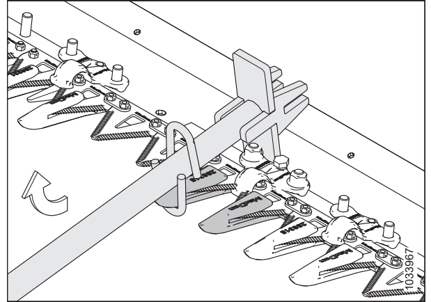
Рисунок 5.46: Регулировка смещением вверх — заостренный противорезающий палец
