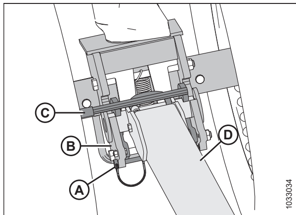
Рисунок 3.99: Удлинитель буксирной тяги и транспортный шарнир
