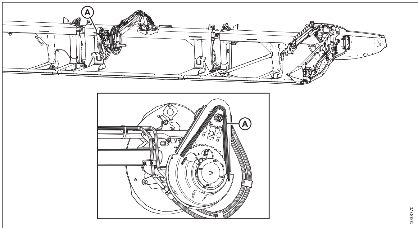
Рисунок 5.7: Мотовило
