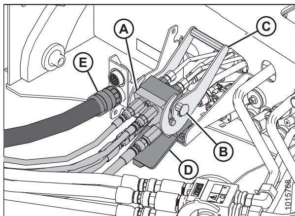
Рисунок 4.111: Многоканальная муфта полотна/мотовила
