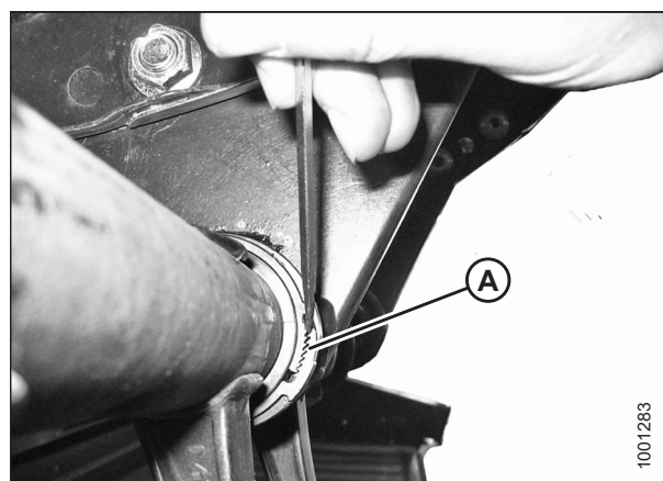
Рисунок 5.159: Хомут втулки
