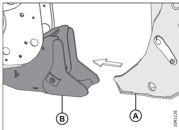
Рисунок 4.25: Лапа и опора жатки
