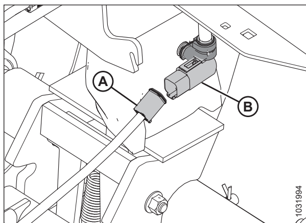
Рисунок 3.131: Электрическое соединение буксирной тяги
