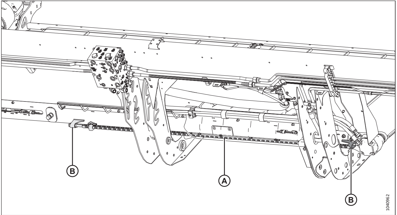
Рисунок 3.87: Цепь гидравлического механизма перемещения столов — показана левая, правая — аналогична
