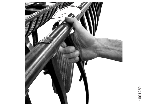
Рисунок 5.149: Снятие пластмассового пальца
