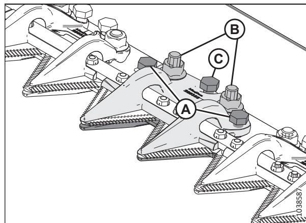
Рисунок 5.82: Центральный прижим
