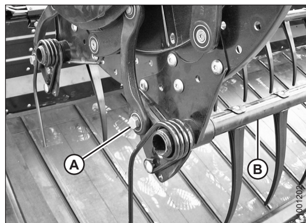
Рисунок 5.170: Сторона эксцентрика
