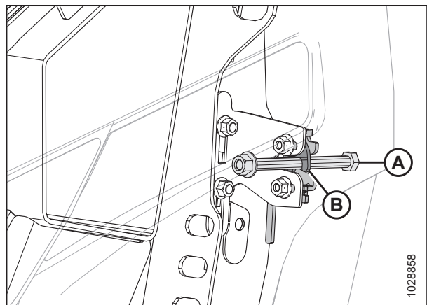
Рисунок 3.13: Двухступенчатая защелка
