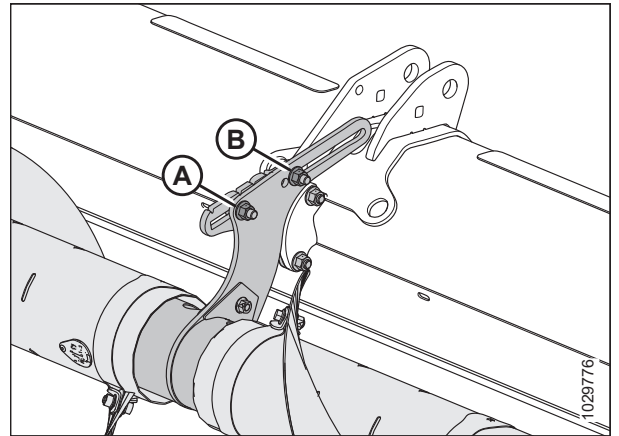
Рисунок 3.69: Первоначальное положение регулируемых креплений — двухсоставной шнек
