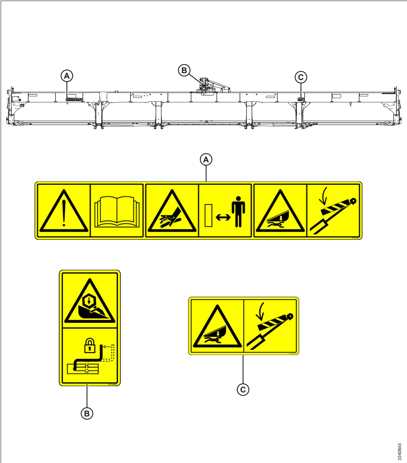
Рисунок 1.26: Задняя труба — Полотняная жатка D235
