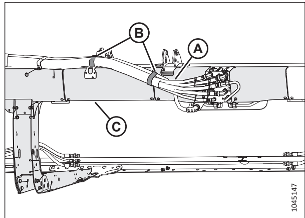
Рисунок 4.147: Положение шланга на жатке D215/ D220
