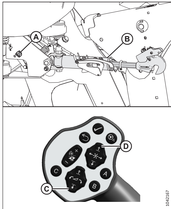
Рисунок 4.129: Центральное соединение без функции самовыравнивания
