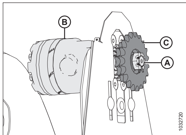
Рисунок 5.218: Двойная звездочка
