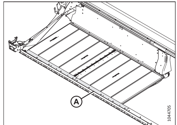
Рисунок 5.90: Уплотнения ножевого бруса
