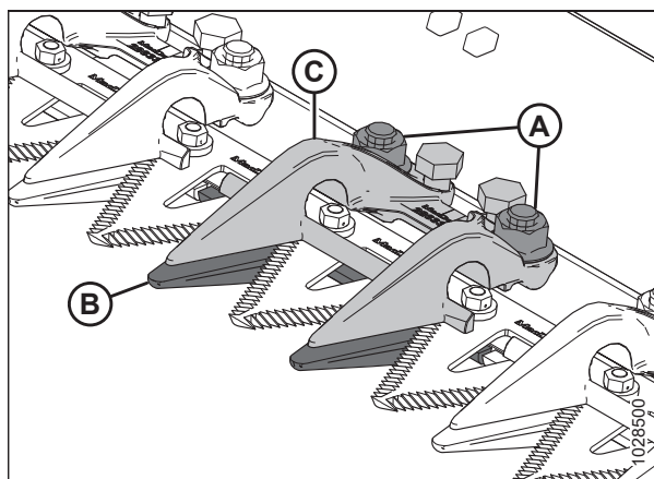
Рисунок 5.69: Укороченные противорежущие пальцы
