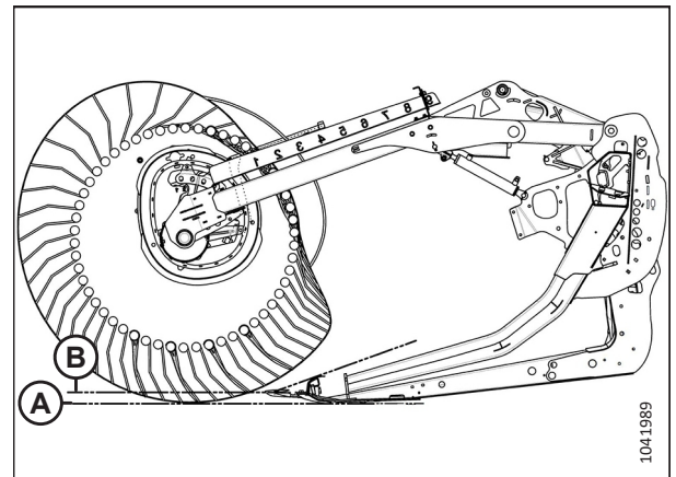
Рисунок 3.62: Профиль пальцев — положение эксцентрика 4, минимальный угол атаки жатки
