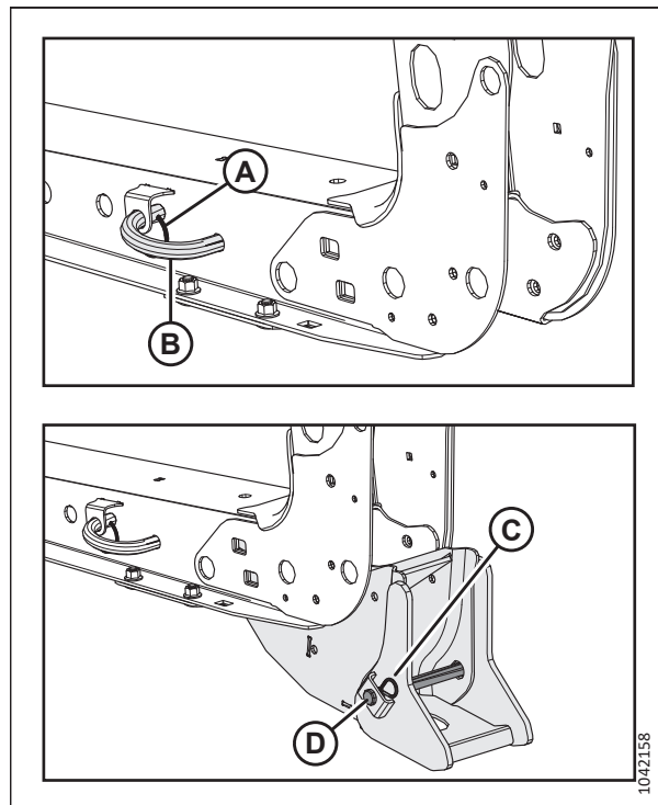
Рисунок 4.127: Лапа жатки — показана левая сторона
