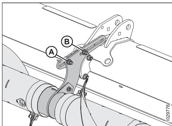
Рисунок 3.67: Первоначальное положение регулируемых креплений — двухсоставной шнек
