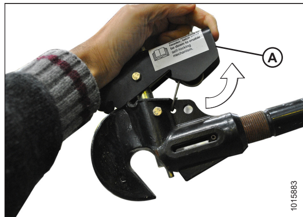
Рисунок 4.154: Центральное соединение
