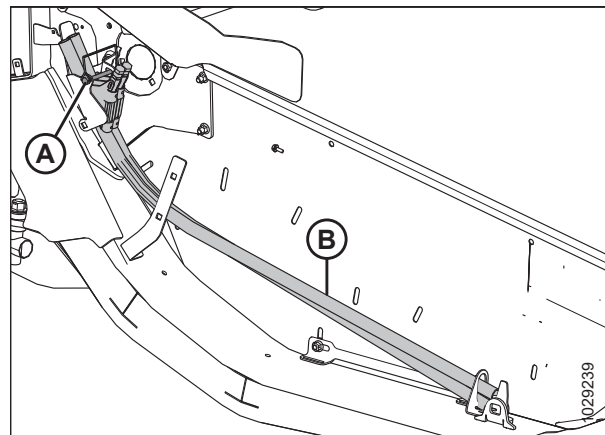
Рисунок 3.80: Пруты делителя
