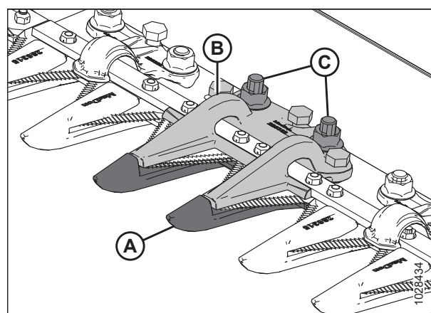
Рисунок 5.57: Заостренный центральный противорежущий палец
