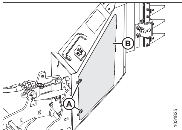
Рисунок 5.244: Крышка доступа к вертикальному ножу
