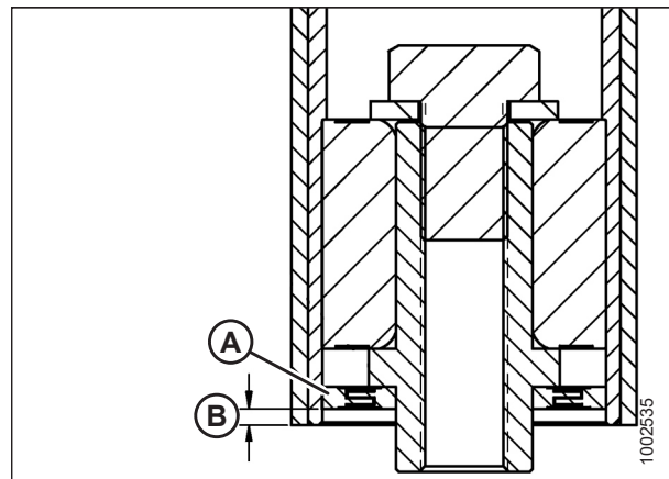
Рисунок 5.109: Подшипник натяжного ролика
