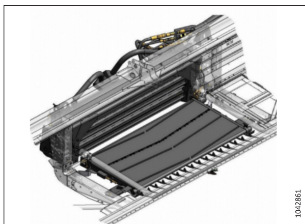
Рисунок 6.15: Сенная плющилка HC20
