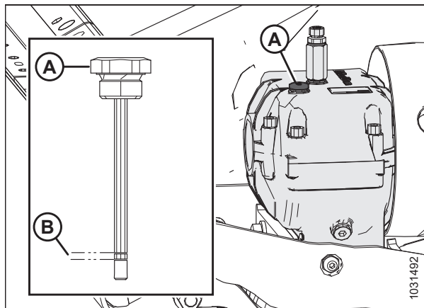
Рисунок 5.85: Редуктор привода ножа
