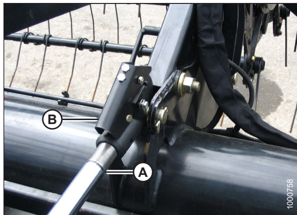
Рисунок 4.71: Гидравлическое центральное звено
