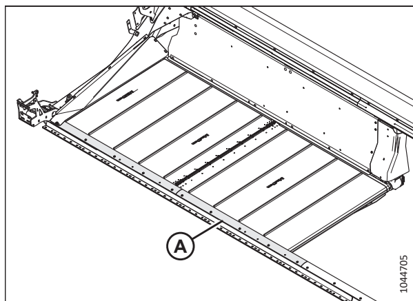
Рисунок 5.95: Уплотнения ножевого бруса
