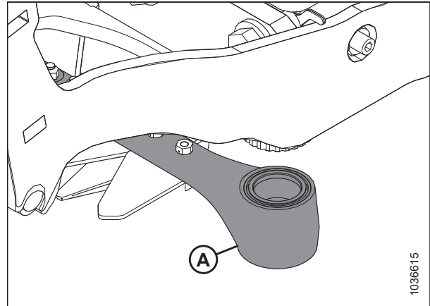
Рисунок 5.37: Головка ножа
