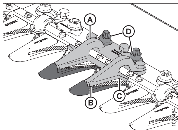
Рисунок 5.63: Заостренный центральный прижим
