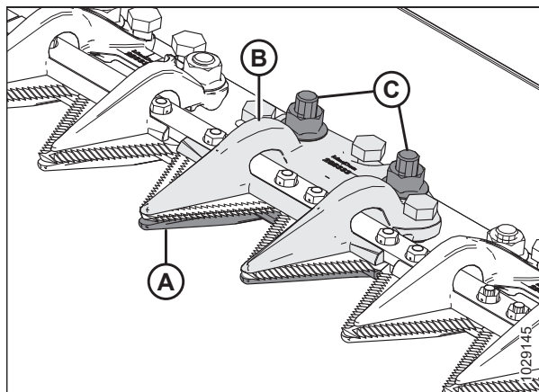
Рисунок 5.75: Центральный противорежущий палец
