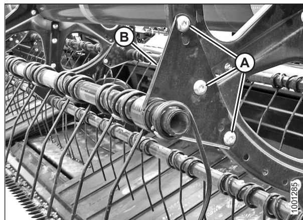
Рисунок 5.146: Рычаг граблины
