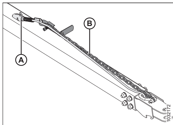
Рисунок 3.134: Жгут проводов буксирной тяги
