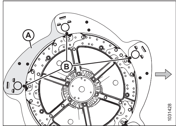
Рисунок 5.189: Боковые щитки мотовила — внутренняя сторона эксцентрика
