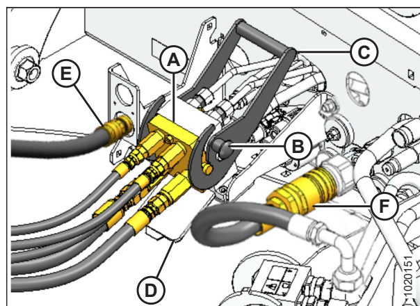
Рисунок 4.144: Многоканальная муфта полотна/ мотовила
