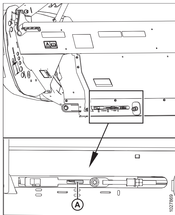
Рисунок 5.96: Проверка левого натяжителя
