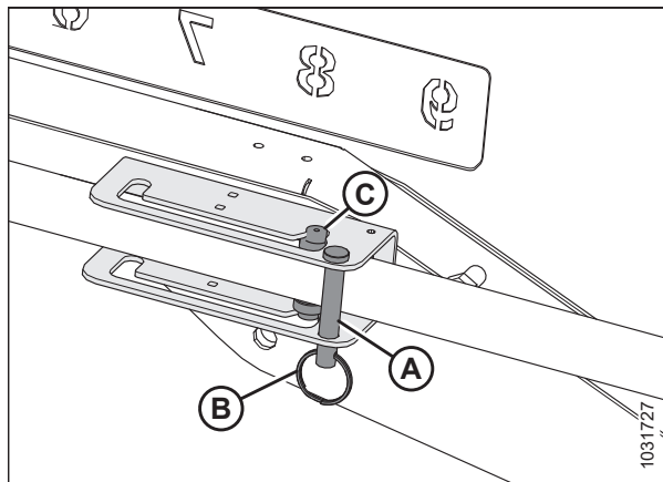
Рисунок 3.55: Регулировка цилиндра перемещения вперед/назад, тип 2 — заднее положение
