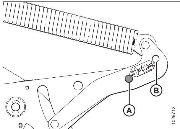
Рисунок 4.17: Рычаги флотации жатки
