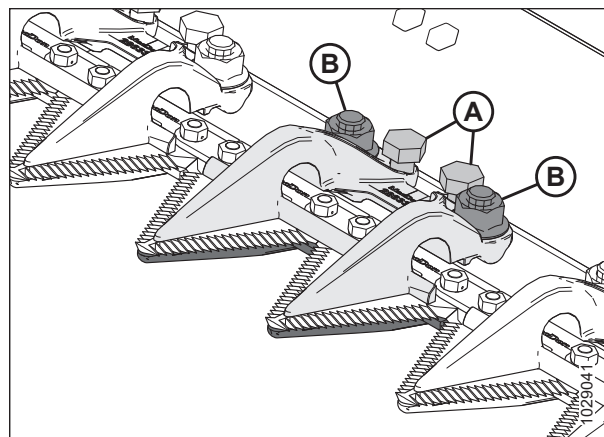
Рисунок 5.74: Прижим укороченного противорежущего пальца
