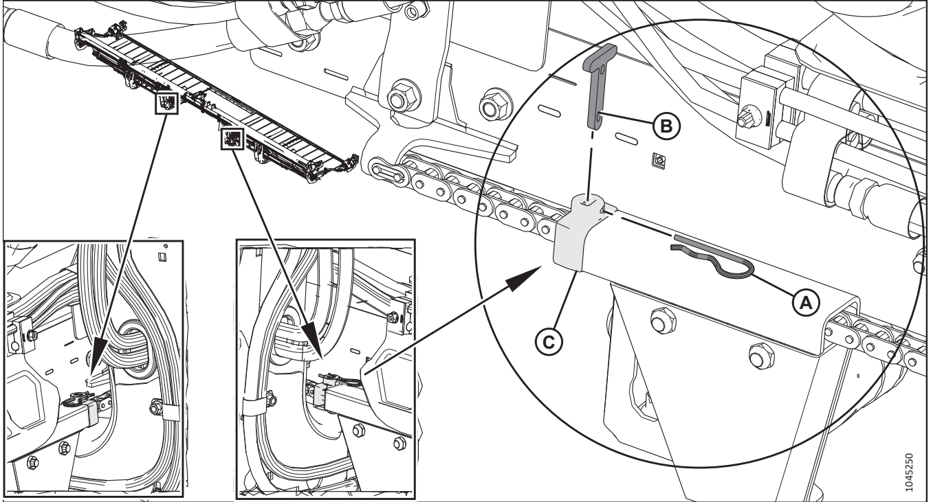
Рисунок 3.84: Внутренний упор перемещения дек
