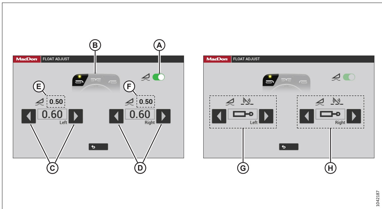
Рисунок 4.138: Регулировка флотации
