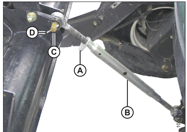
Рисунок 4.79: Механическое центральное соединение
