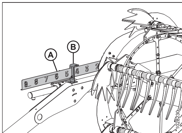
Рисунок 3.46: Индикатор продольного перемещения
