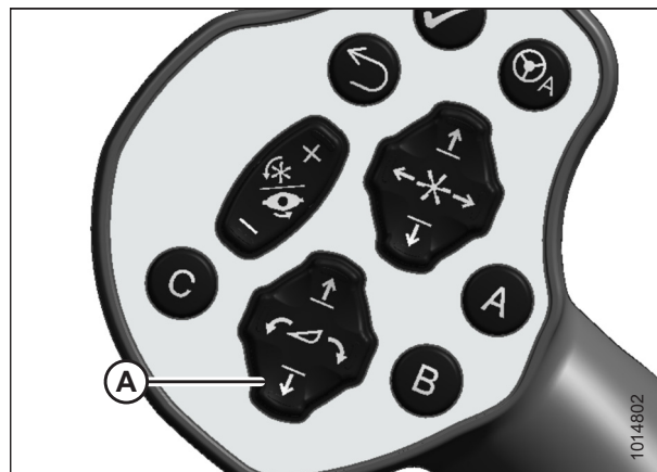
Рисунок 4.137: Рычаг путевой скорости (GSL)
