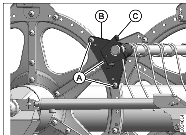
Рисунок 5.152: Хвостовик
