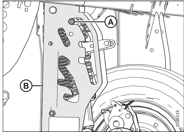
Рисунок 3.113: Штифт шарнира левого транспортного колеса в самом высоком положении хранения
