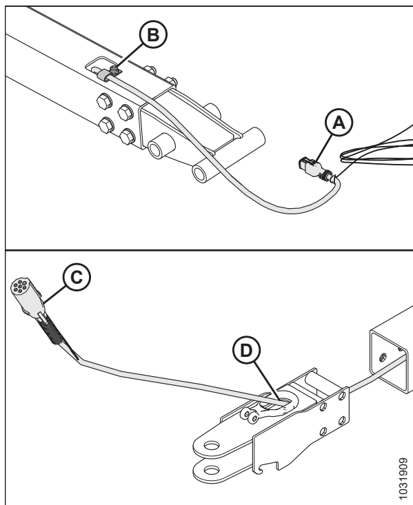
Рисунок 5.232: Снятие вилочного буксирного переходника
