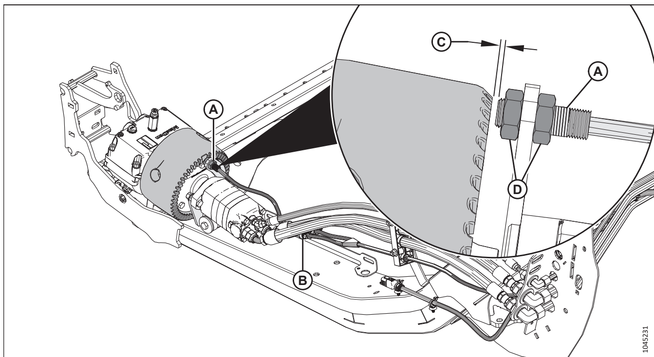
Рисунок 5.20: Левый датчик скорости — положение на косилках серии M1/M2
