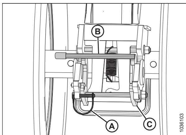
Рисунок 3.109: Левые транспортные колеса — защелка, препятствующая вращению, открыта
