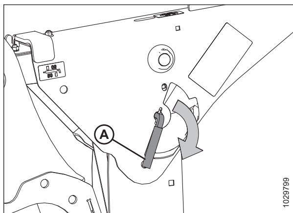
Рисунок 4.136: Рычаг предохранительного упора
