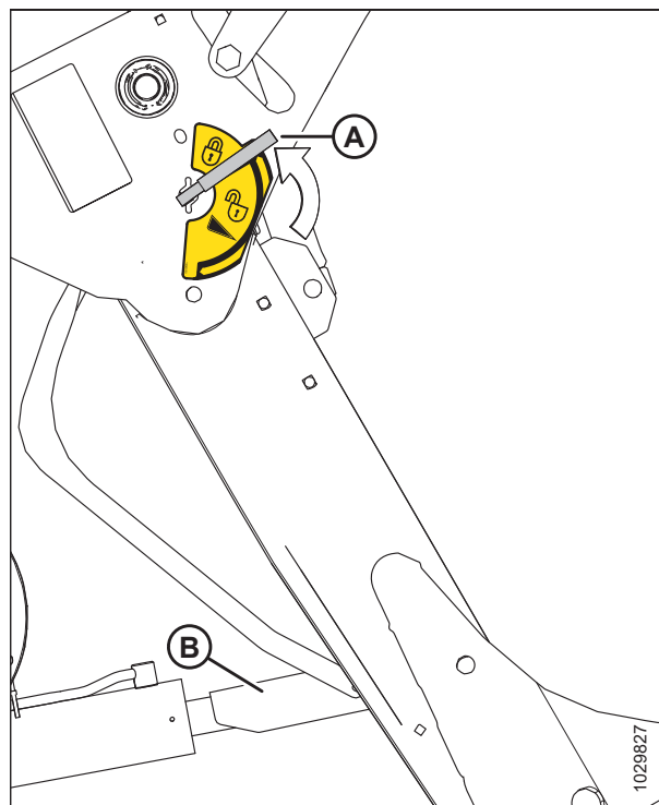
Рисунок 4.74: Предохранительный упор
