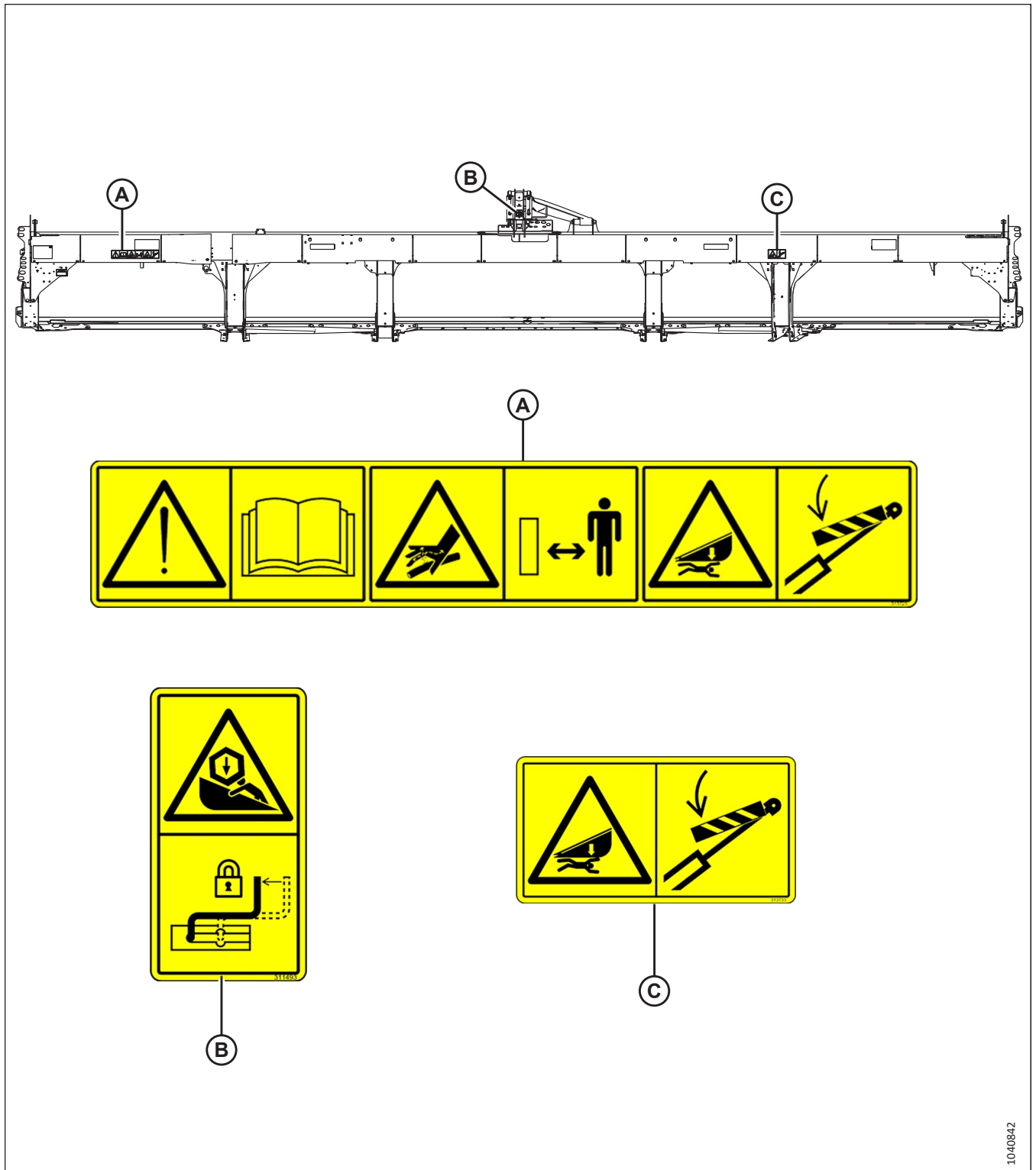
Рисунок 1.25: Задняя труба — Полотняная жатка D230
