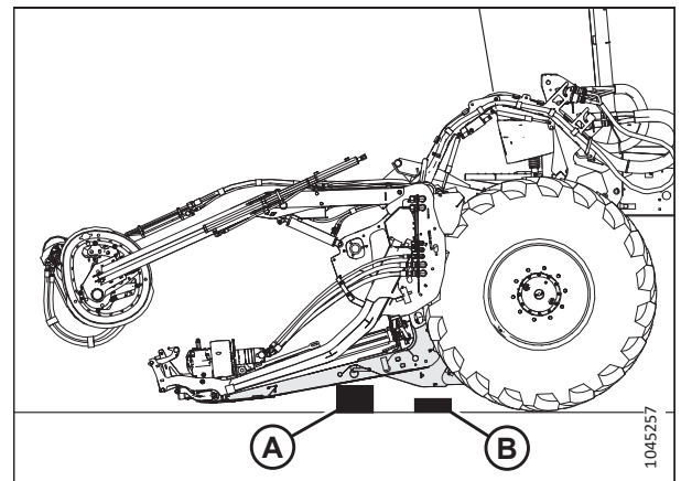
Рисунок 4.64: Установка жатки на грунт
