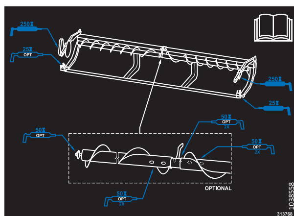
Рисунок 5.15: Наклейка для жатки с одинарным приводом ножа с двухсоставным верхним поперечным шнеком
