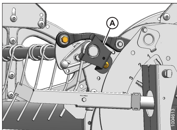
Рисунок 5.172: Сторона эксцентрика
