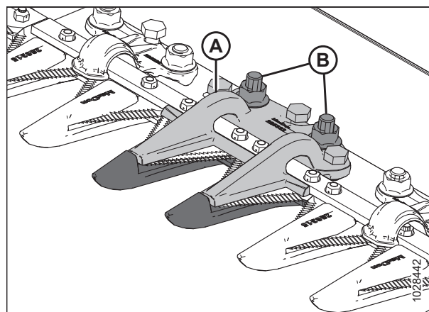
Рисунок 5.62: Заостренный центральный противорежущий палец
