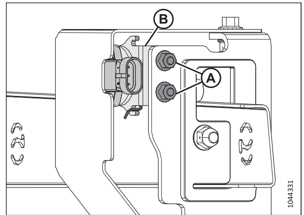
Рисунок 3.58: Датчик продольного перемещения
