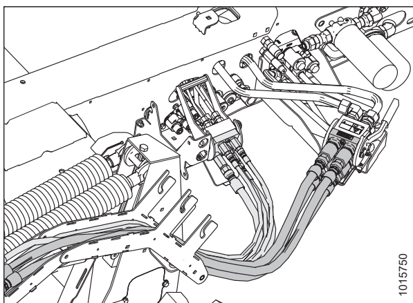
Рисунок 4.106: Гидравлические многоканальные муфты и прокладка шлангов
