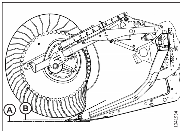
Рисунок 3.59: Профиль пальцев — положение эксцентрика 1
