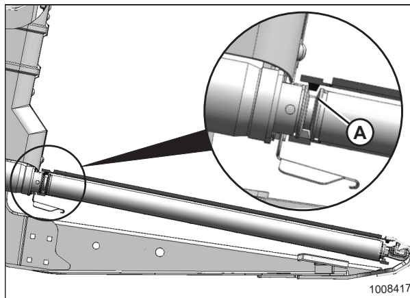
Рисунок 5.97: Приводной ролик
