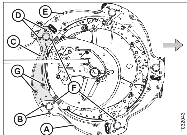
Рисунок 5.188: Боковые щитки мотовила — внешняя сторона эксцентрика
