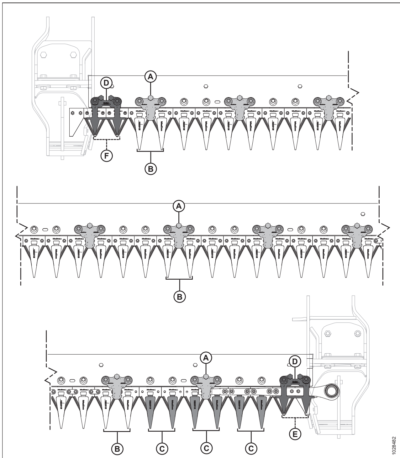
Рисунок 5.43: Местоположение заостренных противорезущих пальцев и прижимов — жатки с одинарными ножами
