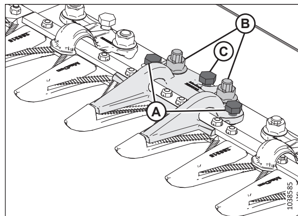
Рисунок 5.64: Заостренный центральный прижим
