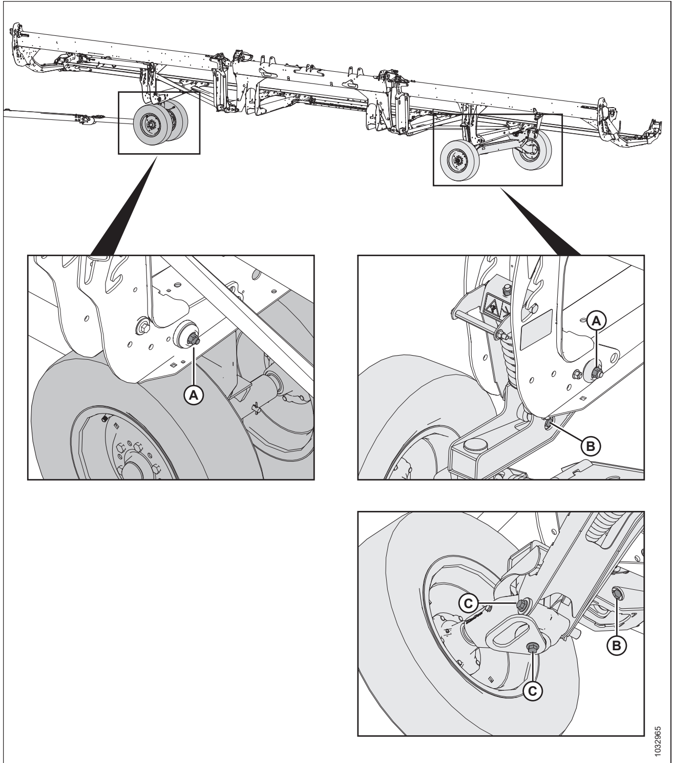
Рисунок 5.224: Болты узла транспортировочной системы
