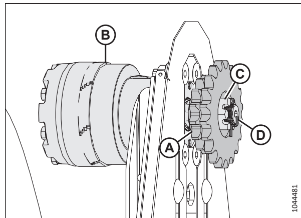
Рисунок 5.220: Двойная звездочка
