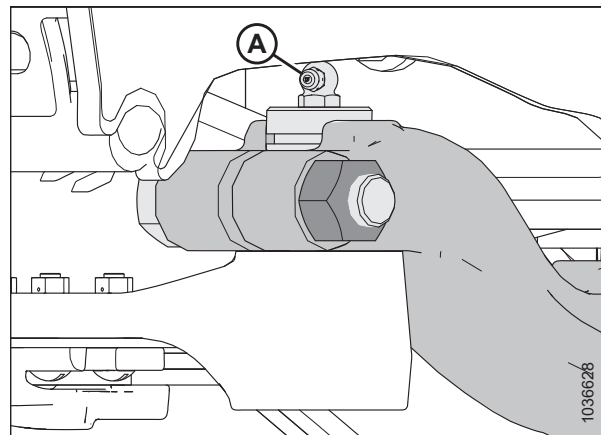
Рисунок 5.40: Головка ножа
