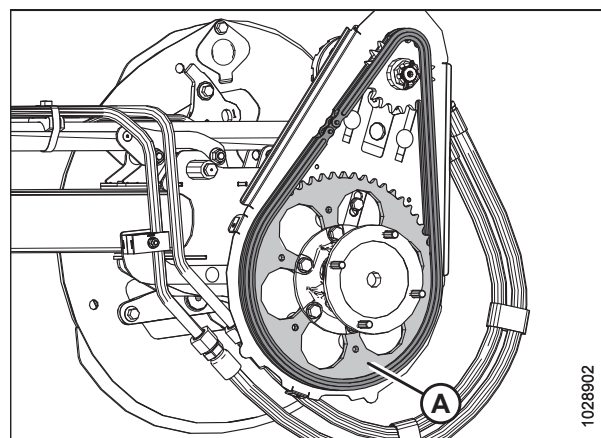
Рисунок 5.211: Привод мотопила
