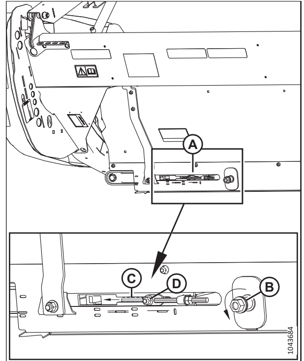
Рисунок 5.89: Регулировка левого натяжителя
