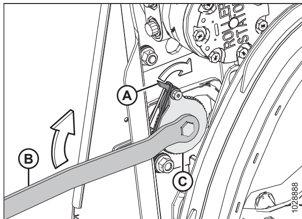
Рисунок 5.207: Привод мотовила
