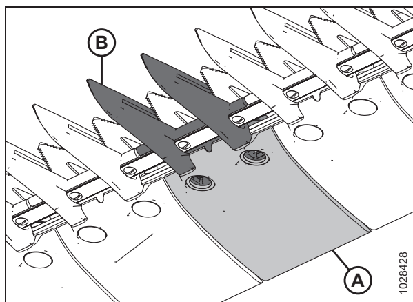
Рисунок 5.53: Заостренный противорежущий палец и износная пластина
