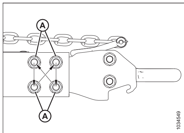
Рисунок 5.235: Последовательность затяжки
