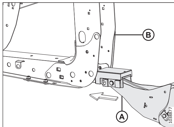
Рисунок 4.10: Лапа и опора жатки
