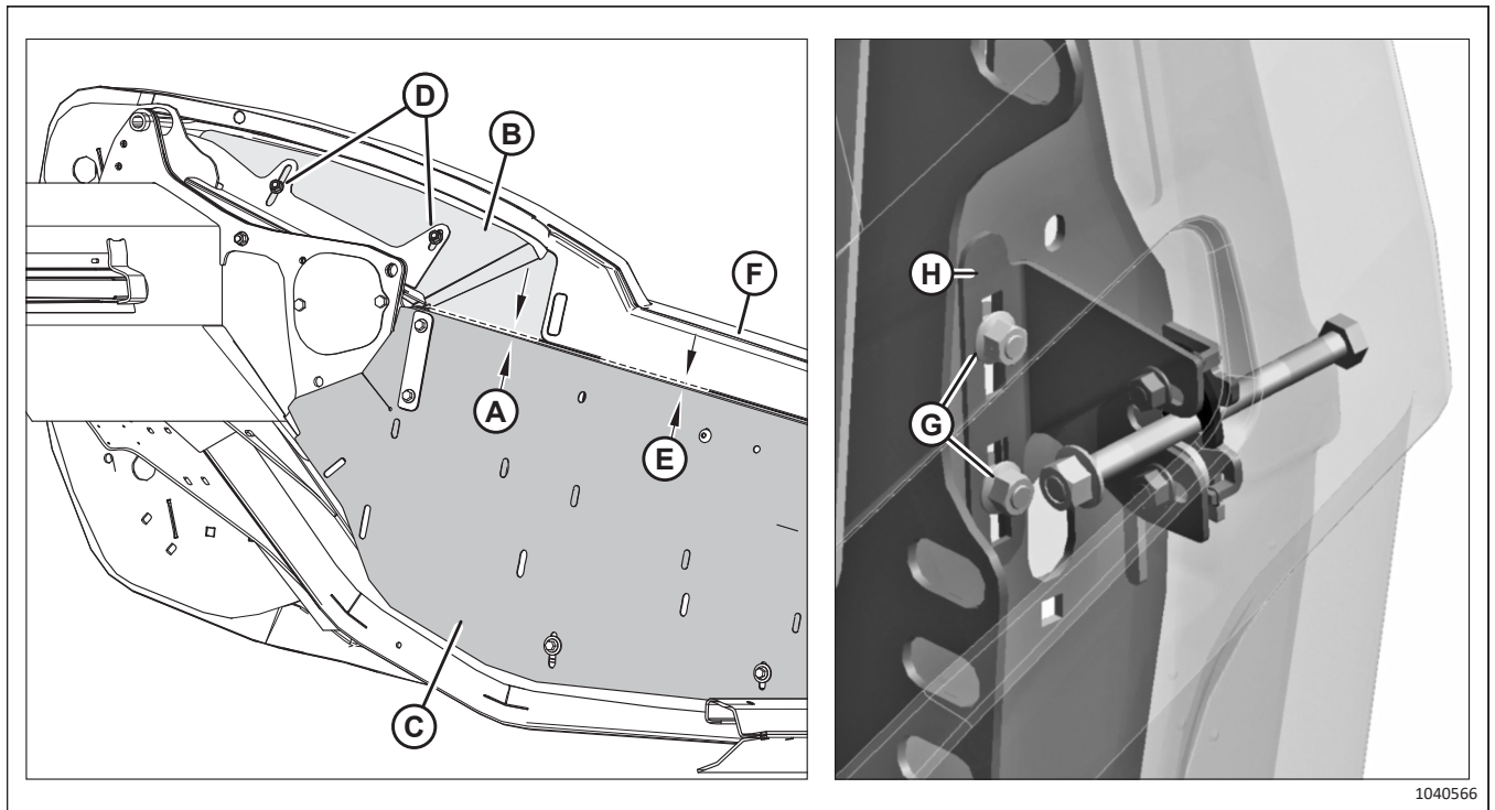
Рисунок 3.18: Величина зазора между подголовником и боковой панелью
