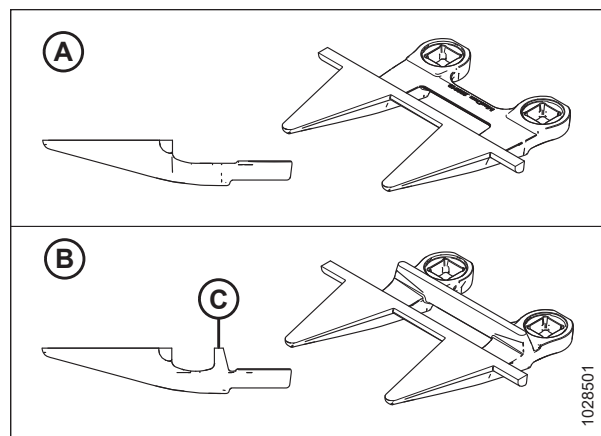
Рисунок 5.70: Концевой противорежущий палец и укороченный противорежущий палец
