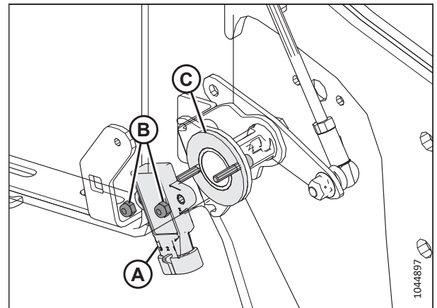
Рисунок 3.44: Датчик высоты мотовила: правый рычаг мотовила
