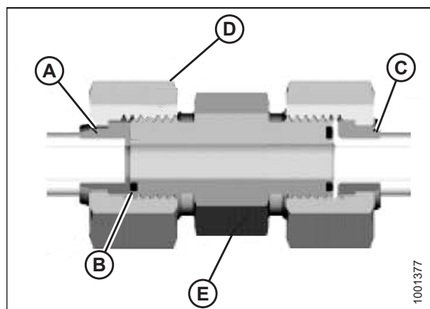
Рисунок 8.10: Гидравлический фитинг
