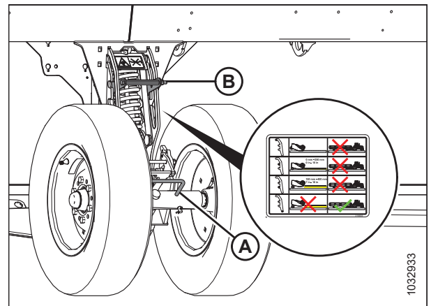
Рисунок 3.35: Левое колесо
