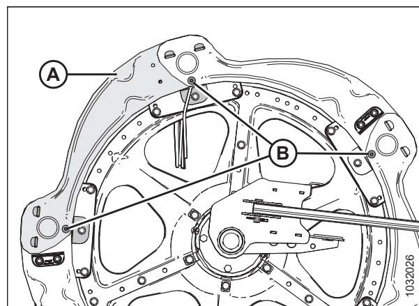
Рисунок 5.193: Боковые щитки мотовила — внешняя сторона хвостовика
