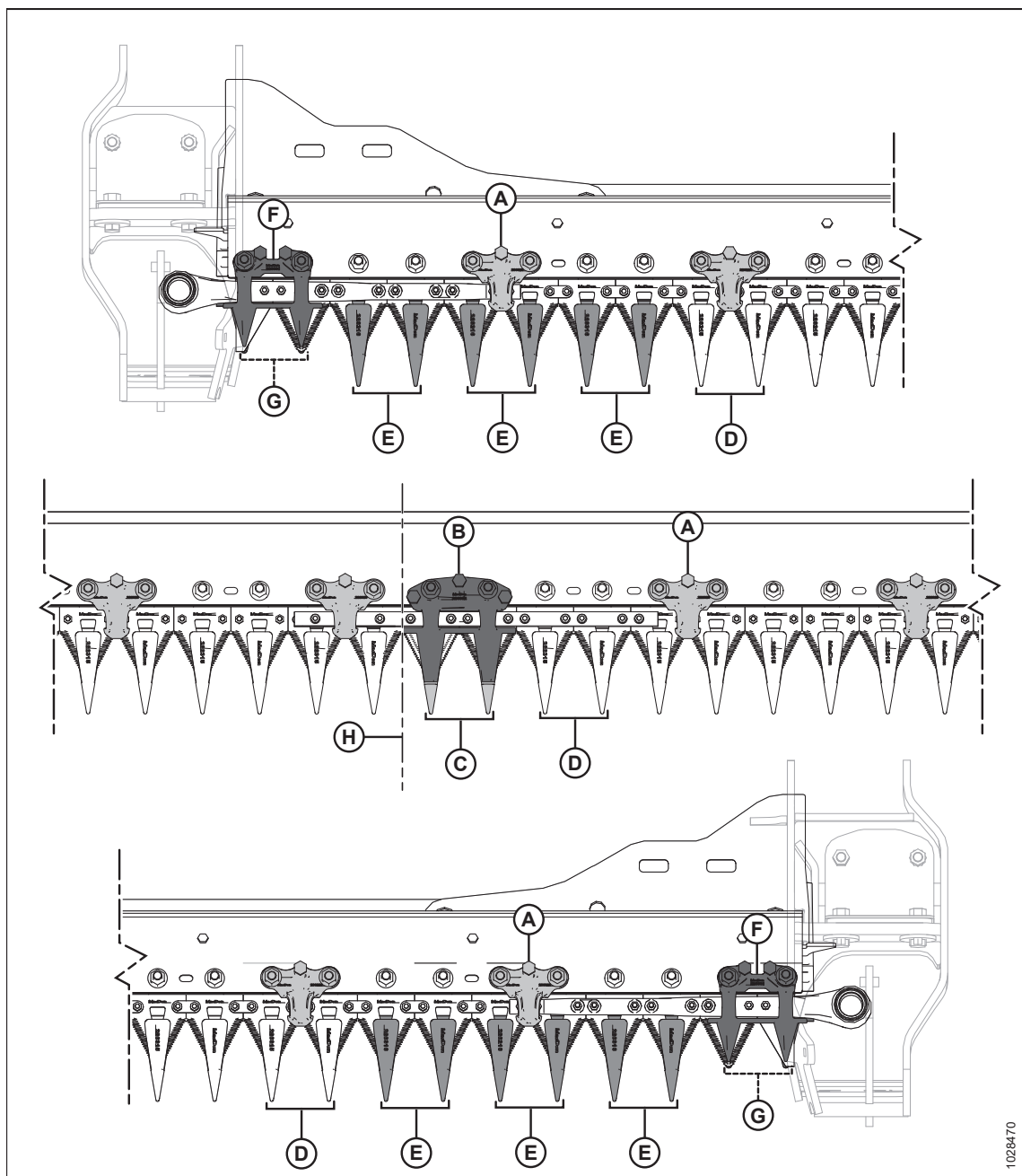
Рисунок 5.45: Расположение заостренных противорежущих пальцев и прижимов
