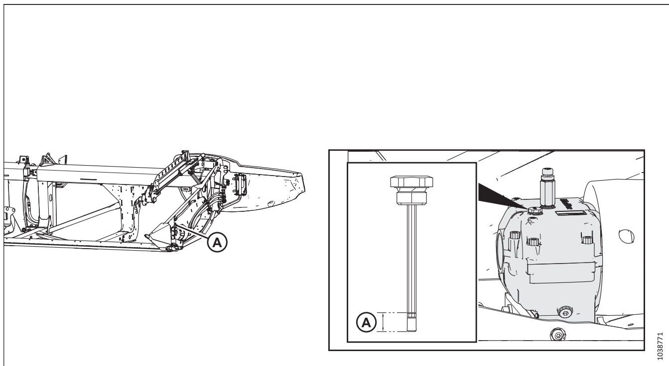
Рисунок 5.10: Редуктор привода ножа
