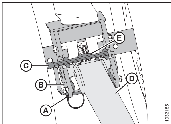
Рисунок 3.130: Удлинитель буксирной тяги к левому транспортному шарниру
