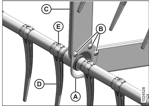
Рисунок 5.183: Противоположная опора комплекта усиления граблин мотовила (опция)
