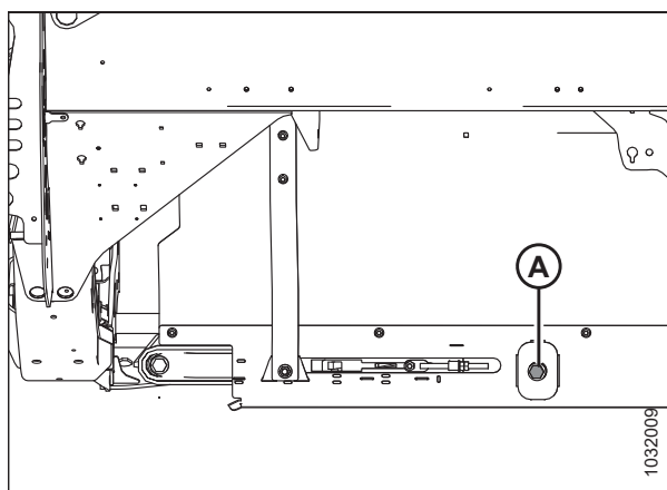
Рисунок 5.123: Натяжитель полотна — показана левая сторона
