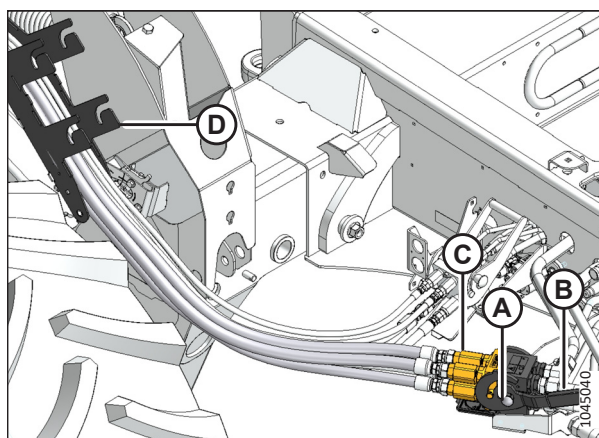
Рисунок 4.161: Многоканальная муфта ножа/мотовила
