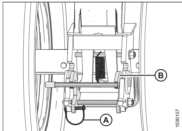
Рисунок 3.110: Левые транспортные колеса — защелка, препятствующая вращению, закрыта
