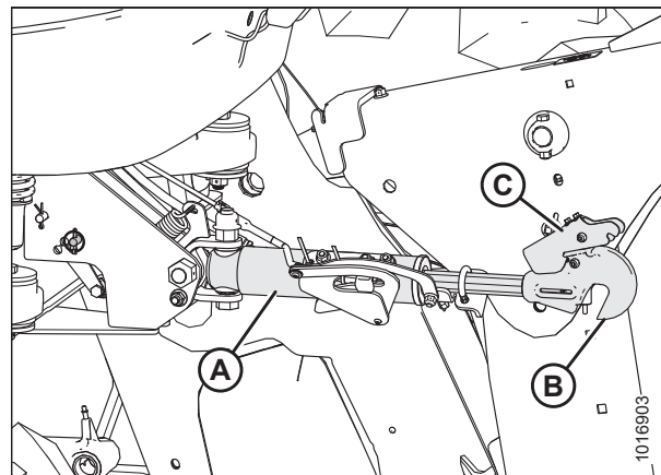
Рисунок 4.91: Гидравлическое центральное соединение
