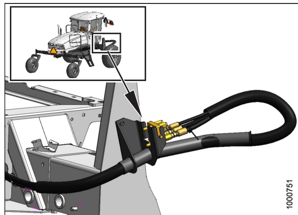
Рисунок 4.54: Место хранения шлангов мотовила
