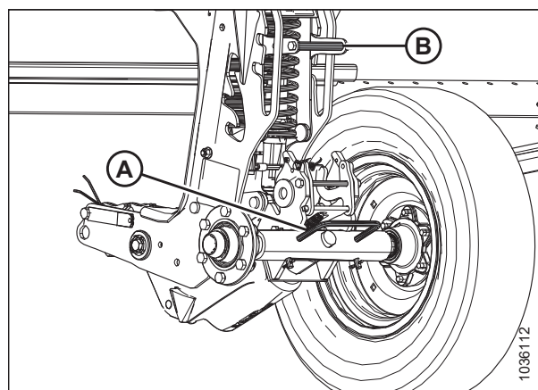
Рисунок 3.112: Левые транспортные колеса в самом высоком положении хранения
