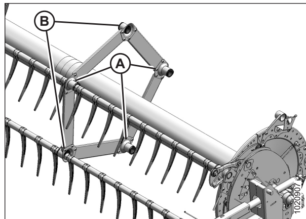
Рисунок 5.157: Опоры граблины
