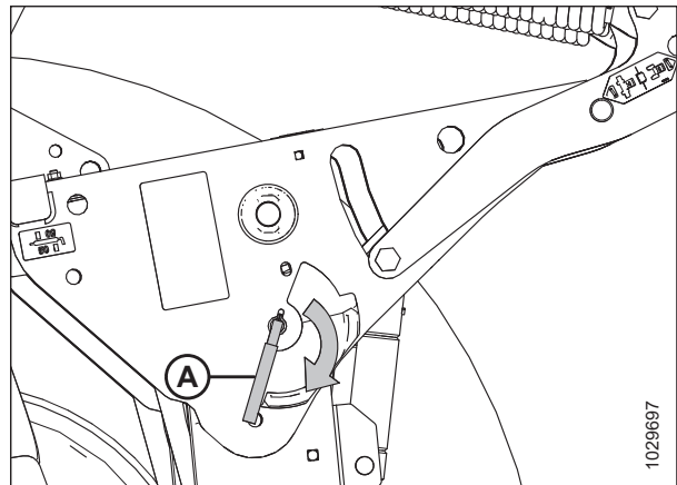
Рисунок 4.18: Рычаг предохранительного упора
