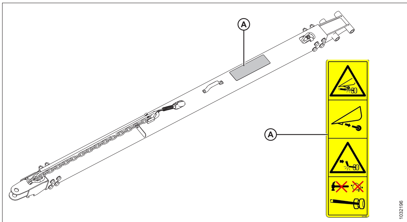
Рисунок 1.30: Транспортировочная система EasyMove™ Transport — дышло (на рисунке показано короткое дышло; длинное дышло выглядит аналогично) (дополнительное оборудование)
