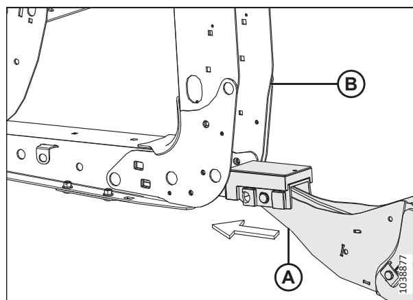
Рисунок 4.41: Лапа и опора жатки
