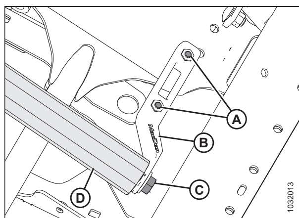
Рисунок 5.117: Приводной ролик
