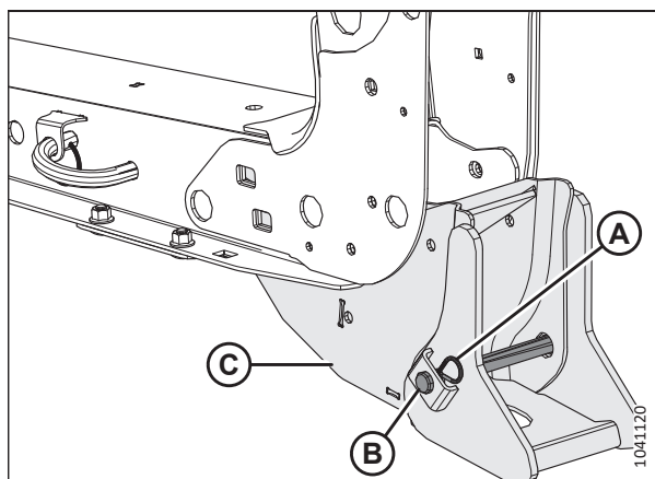
Рисунок 4.83: Опора жатки — показана левая сторона
