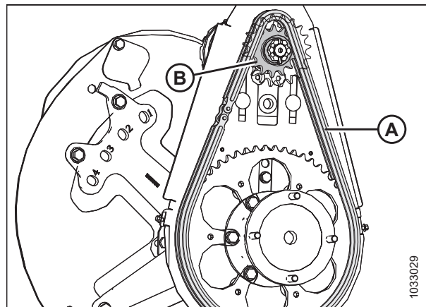
Рисунок 5.217: Двойная звездочка в конфигурации с высоким крутящим моментом
