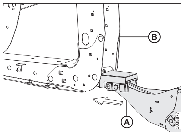
Рисунок 4.26: Лапа и опора жатки
