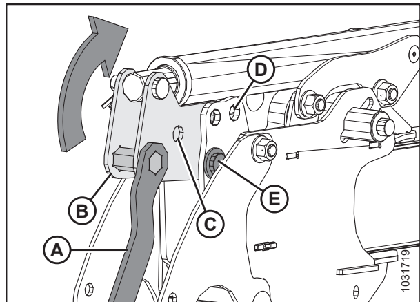
Рисунок 3.51: Регулировка цилиндра перемещения вперед/назад, тип 1 — заднее положение
