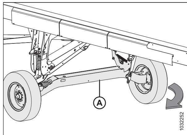
Рисунок 3.115: Вращение правой транспортной оси
