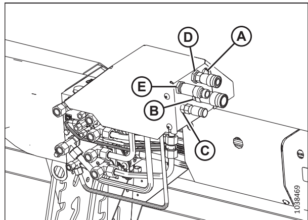
Рисунок 4.52: Гнезда подключения на жатке
