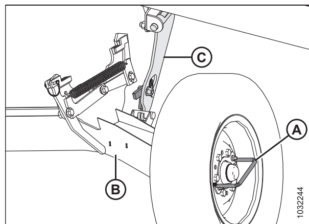
Рисунок 3.124: Правая рабочая опора
