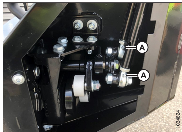
Рисунок 5.241: Тавотницы на толкателях вертикальных ножей
