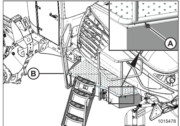
Рисунок 4.107: Левая платформа
