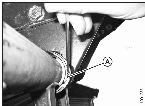
Рисунок 5.153: Хомут втулки
