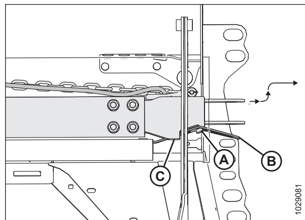
Рисунок 3.128: Буксирная тяга в месте для хранения
