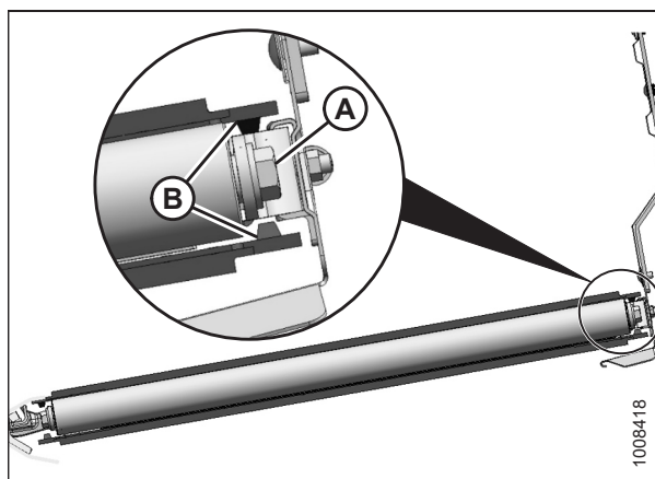
Рисунок 5.98: Натяжной ролик
