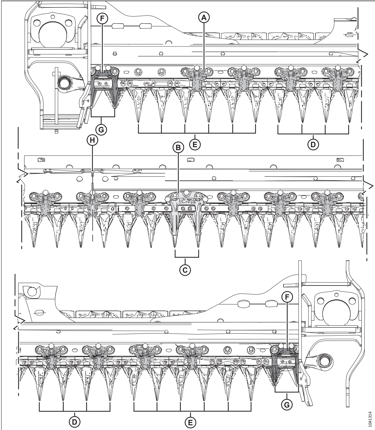
Рисунок 5.44: Расположение заостренных противорежущих пальцев и прижимов
