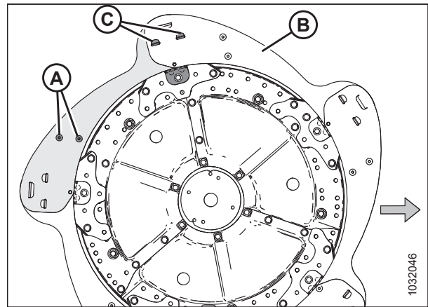
Рисунок 5.190: Боковые щитки мотовила — внутренняя сторона эксцентрика
