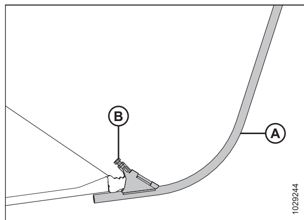
Рисунок 3.81: Стержень на делителе
