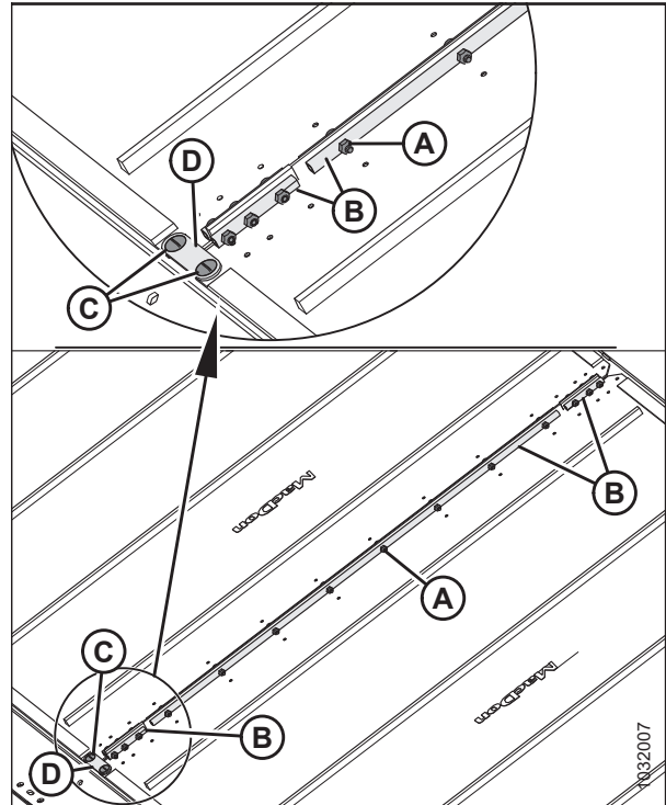
Рисунок 5.103: Стыковочные планки полотна
