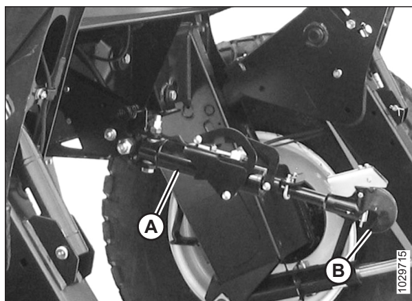
Рисунок 4.28: Гидравлическое центральное соединение
