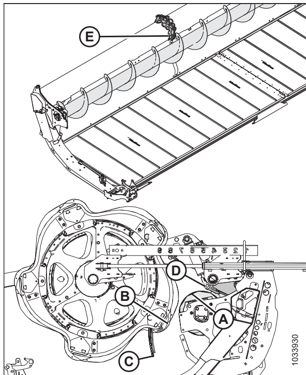
Рисунок 3.70: Места проверки зазора верхнего поперечного шнека
