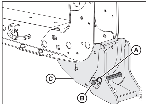
Рисунок 4.123: Опора жатки
