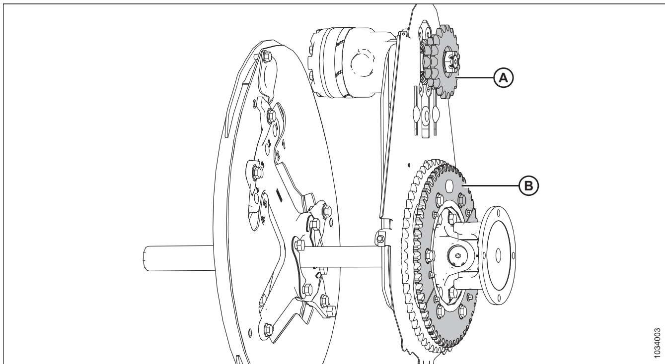
Рисунок 3.40: Привод мотвила с дополнительными звездочками
