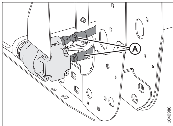
Рисунок 3.92: Гидромотор правой деки
