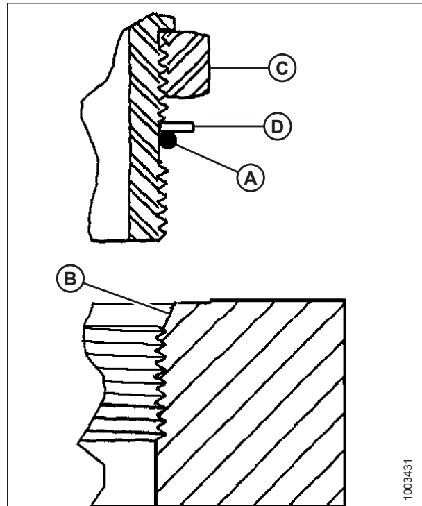
Рисунок 8.6: Гидравлический фитинг
