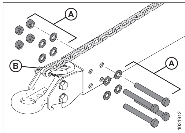
Рисунок 5.234: Установка кольцевого буксирного переходника
