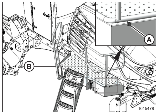
Рисунок 4.148: Левая платформа
