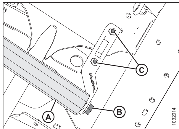
Рисунок 5.120: Приводной ролик
