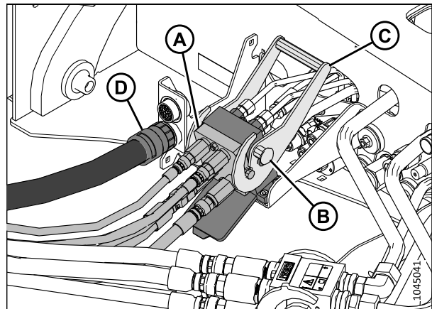
Figure 4.162: Multicoupleur du tapis/rabatteur
