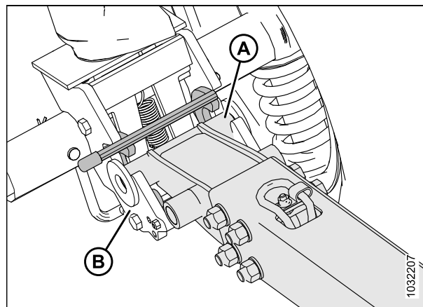
Figure 3.103: Barre de remorquage et pivot de transport gauche
