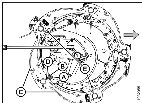
Figure 5.205: Supports des blindages du rabatteur
