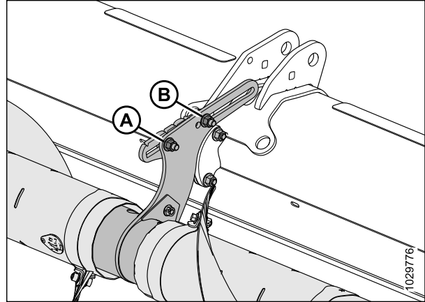
Figure 3.67: Position initiale des supports réglables - Vis en deux parties
