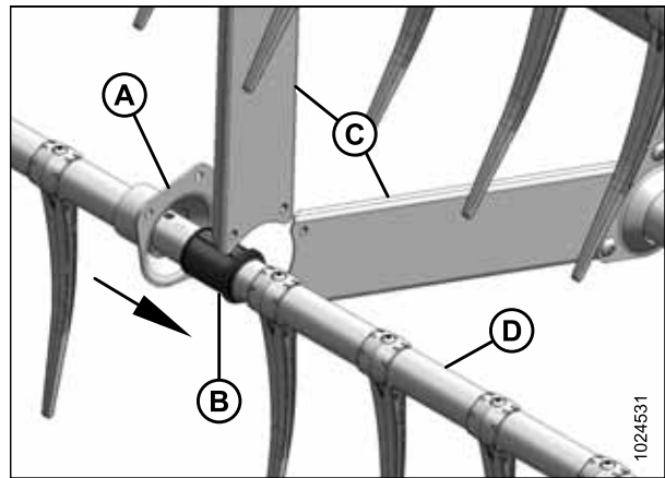
Figure 5.179: Support opposé du kit de renforcement des tubes à doigts en option
