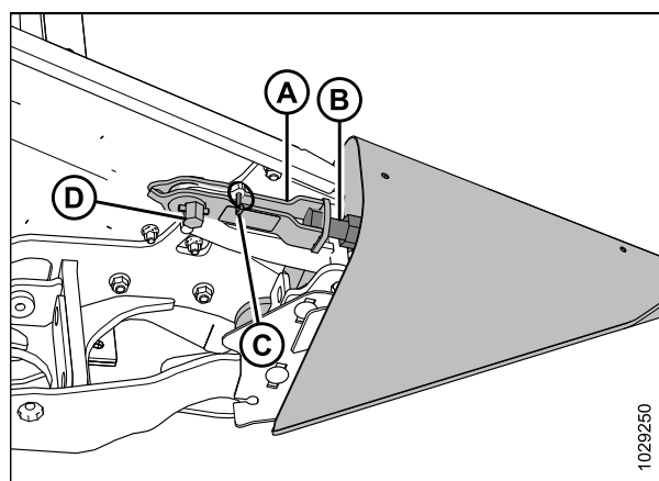
Figure 3.77: Diviseur de récolte avec verrouillage
