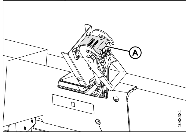
Figure 4.58: Couvercle du connecteur fermé
