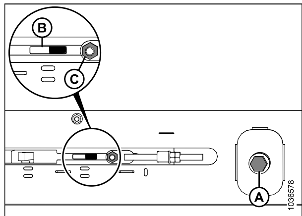
Figure 5.99: Réglage du tendeur gauche
