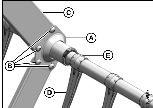
Figure 5.161: Support du tube à doigts
