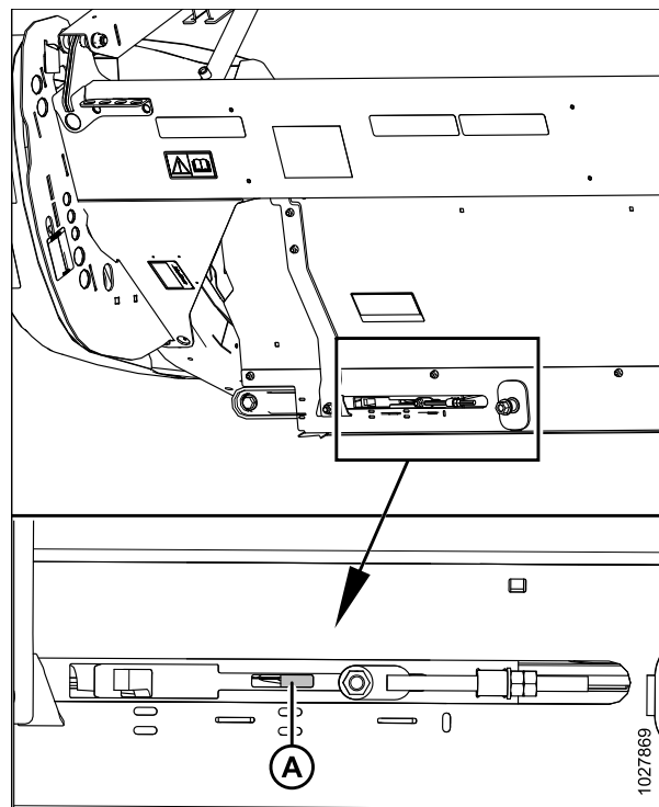
Figure 5.96: Vérification du dispositif de réglage de la tension à gauche
