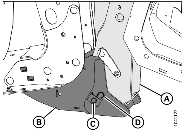
Figure 4.153: Patte de la plateforme et articulation de levage de l'andaineuse reliées par le support de la plateforme
