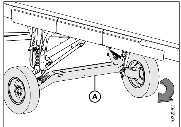
Figure 3.115: Rotation de l'essieu de transport droit
