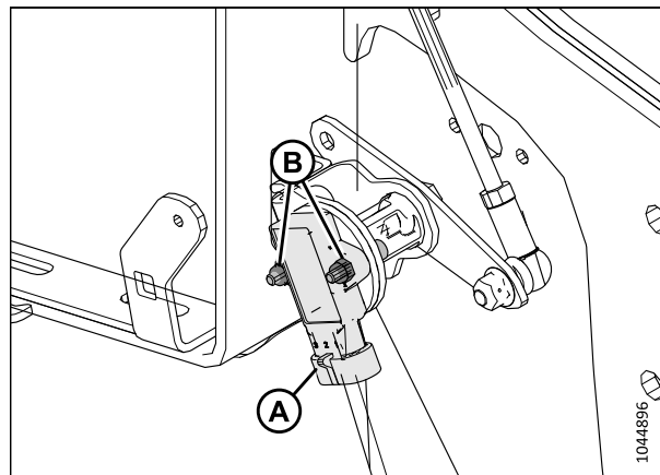
Figure 3.43: Capteur de hauteur du rabatteur – Bras droit du rabatteur
