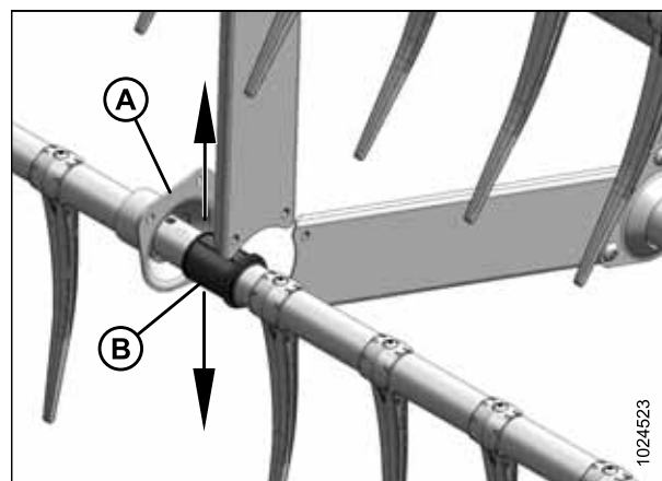
Figure 5.165: Support opposé de kit de renforcement de tubes à doigts
