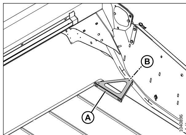
Figure 5.127: Gousset – Côté gauche illustré
