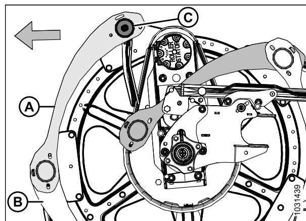
Figure 5.200: Boucliers des rabatteurs - Extrémité arrière intérieure
