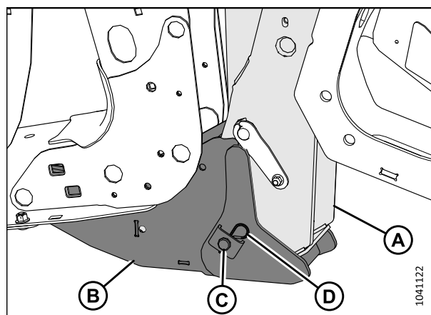
Figure 4.15: Articulation de levage de l'andaineuse et étau de la plateforme
