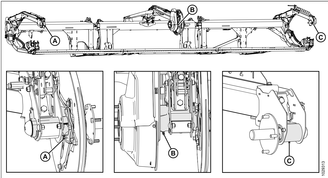
Figure 5.11: Rabatteur
