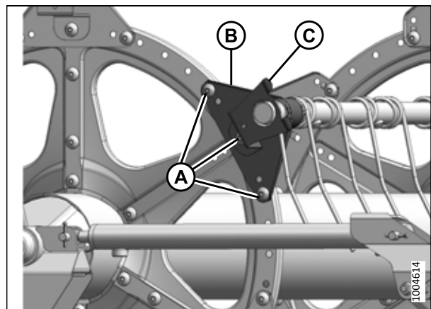
Figure 5.156: Extrémité arrière
