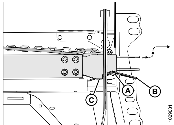
Figure 3.128: Rangement de la barre de remorquage
