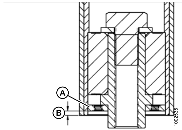
Figure 5.109: Roulement de rouleau libre
