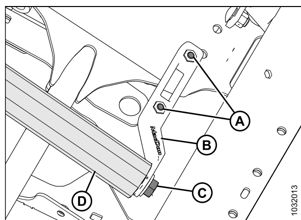
Figure 5.117: Rouleau d'entraînement
