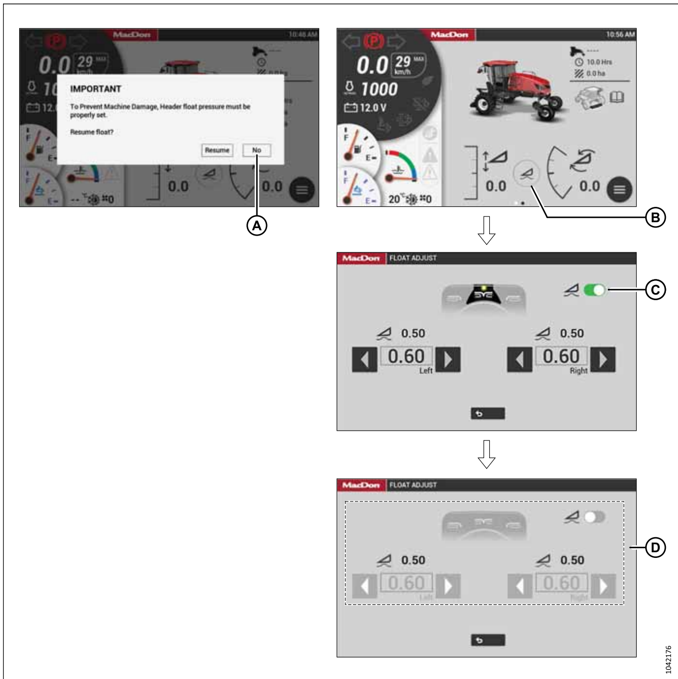
Figure 4.156: Retrait du flottement
