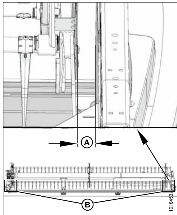
Figure 5.142: Écartement entre le rabatteur et la tôle d'extrémité
