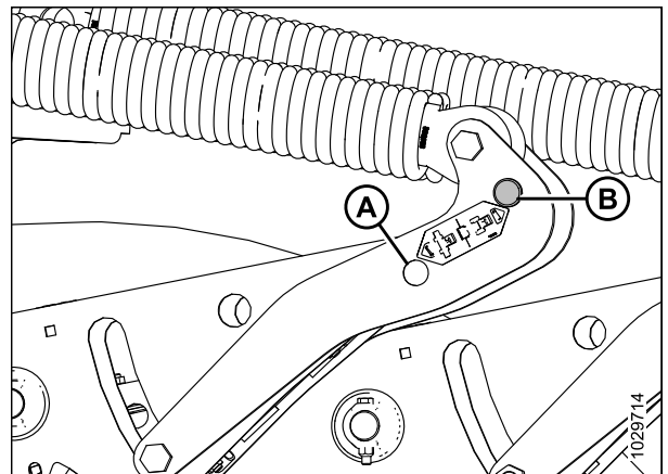
Figure 4.36: Articulation de flottement de la plateforme
