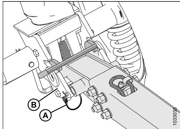
Figure 3.102: Barre de remorquage et pivot de transport gauche
