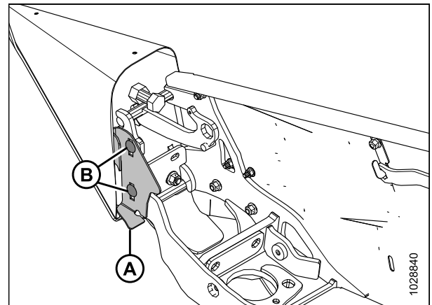
Figure 3.15: Support du capot de la plateforme
