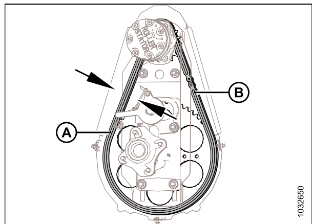
Figure 5.210: Entraînement du rabatteur
