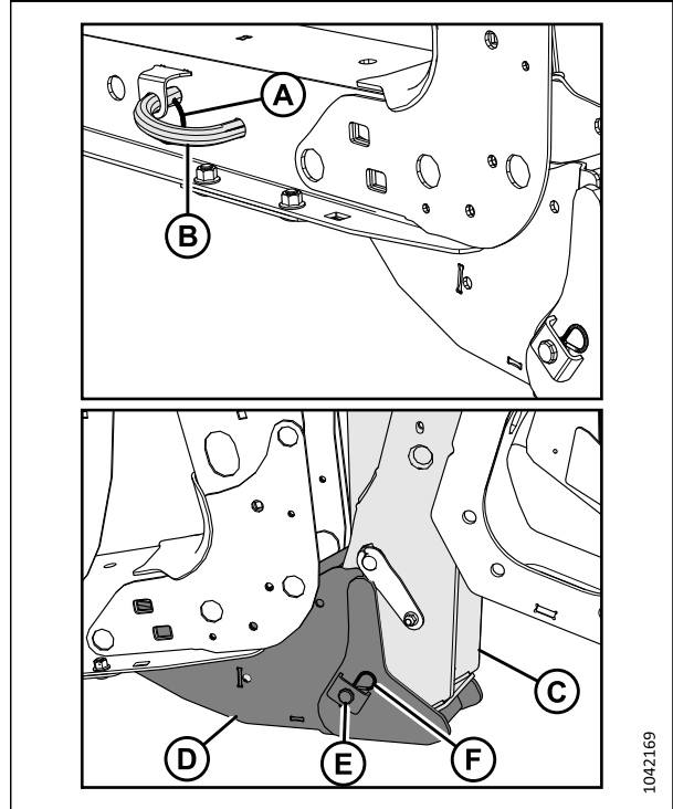
Figure 4.135: Articulation de levage de l'andaineuse et étau de la plateforme
