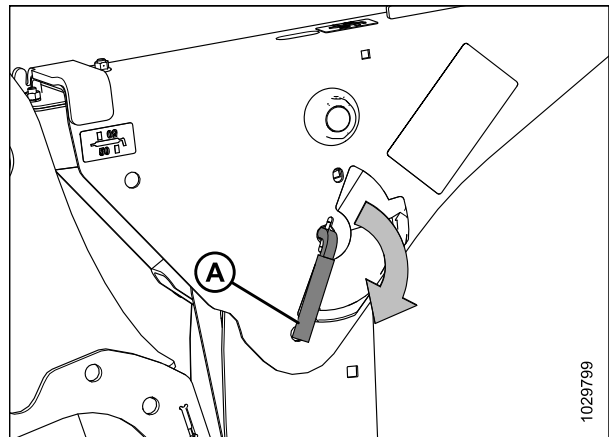
Figure 4.136: Levier du support de sécurité
