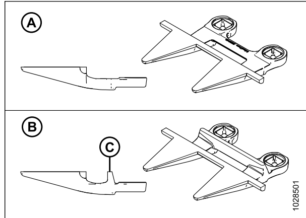
Figure 5.70: Doigts de couteau d'extrémité et doigts de couteau court
