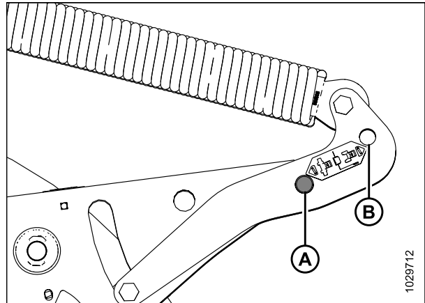
Figure 4.17: Articulation de flottement de la plateforme
