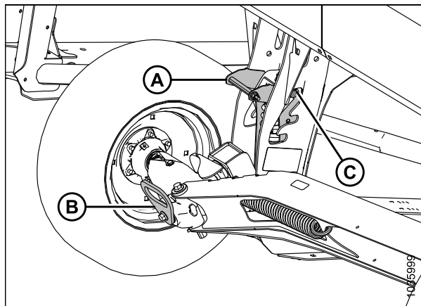
Figure 3.117: Roues de transport droites dans la position de rangement la plus haute
