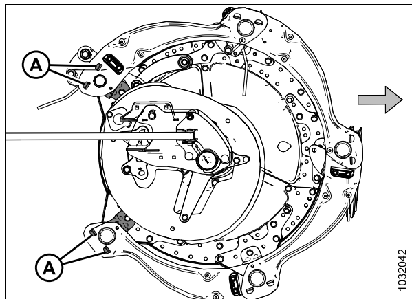
Figure 5.187: Bouclier du rabatteur enlevé - Extrémité de came extérieure
