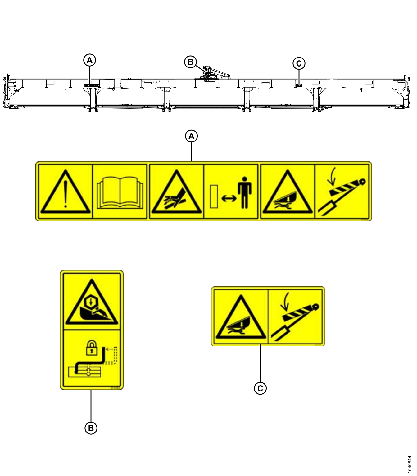
Figure 1.27: Tube arrière – Plateforme de coupe à tapis D241
