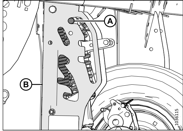
Figure 3.113: Goupille pivotante des roues de transport gauches dans la position de rangement la plus haute
