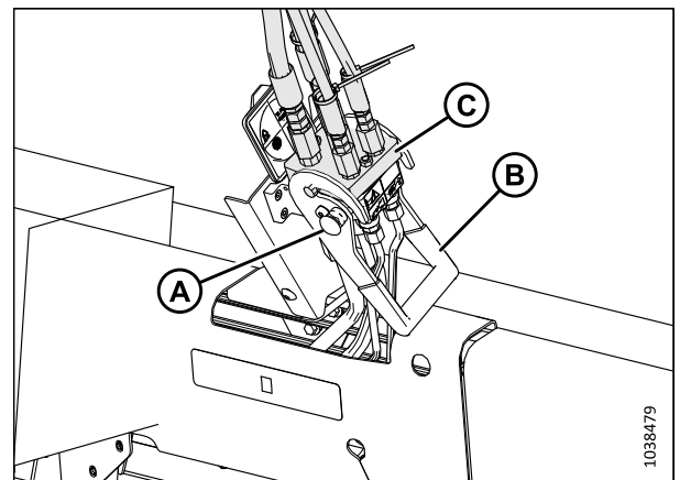
Figure 4.57: Système hydraulique du rabatteur
