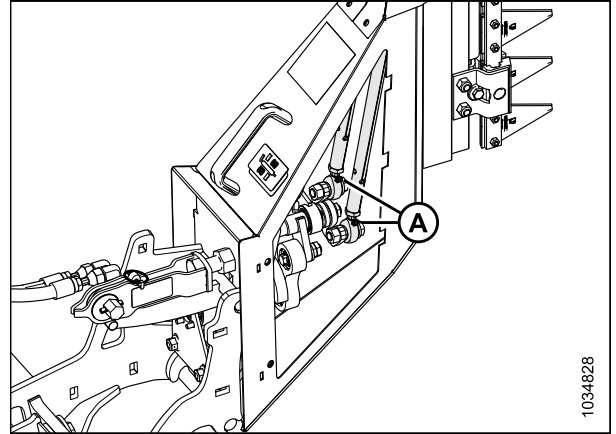
Figure 5.243: Graissage des embouts sur les tiges-poussoirs des couteaux verticaux
