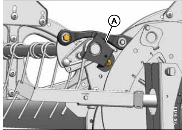
Figure 5.172: Extrémité de la came
