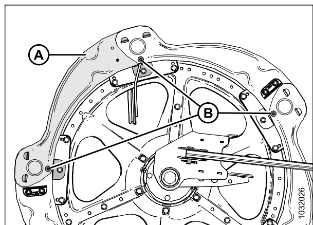
Figure 5.193: Boucliers des rabatteurs - Extrémité arrière extérieure
