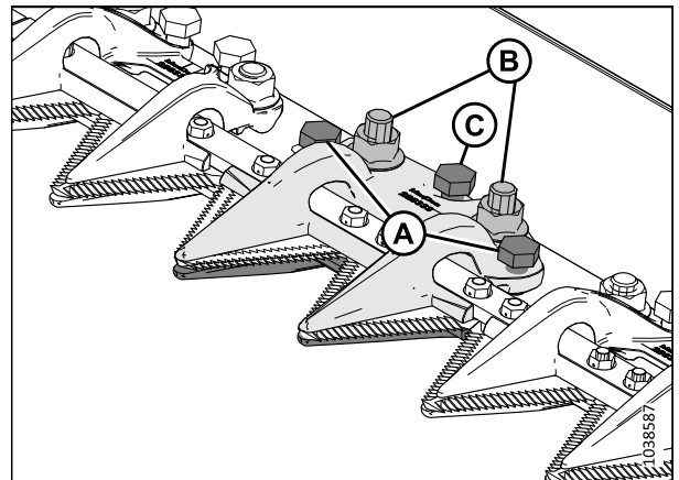
Figure 5.82: Rabatteur central
