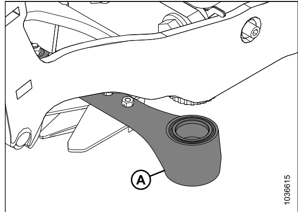
Figure 5.37: Tête de couteau
