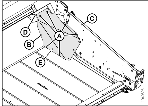
Figure 5.128: Déflecteur arrière large – Côté gauche illustré
