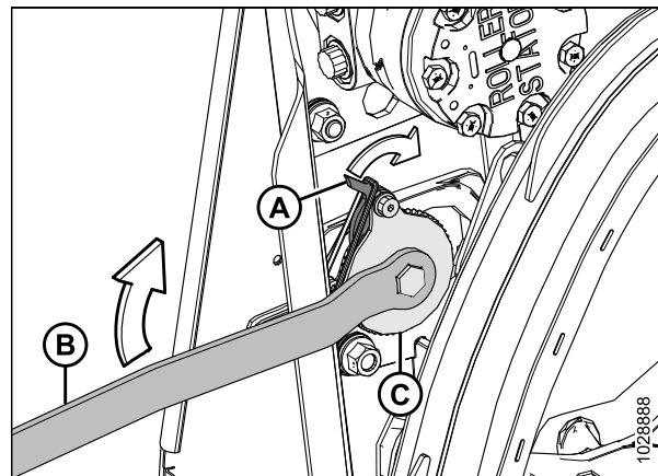
Figure 5.207: Entraînement du rabatteur
