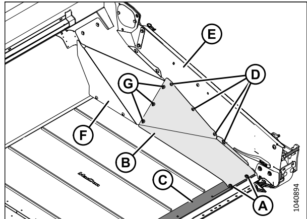
Figure 5.129: Déflecteur large – Côté gauche illustré
