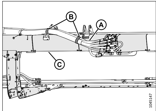
Figure 4.147: Position des flexibles des plateformes de coupe à tapis D215/D220
