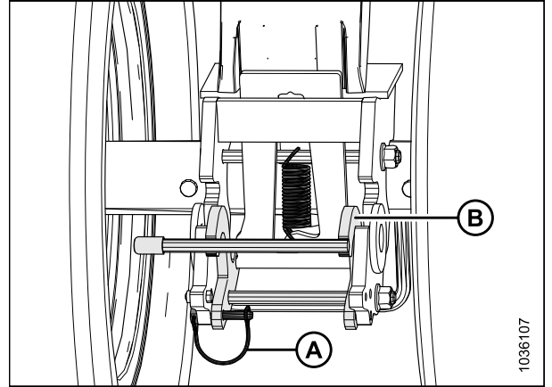
Figure 3.110: Roues de transport gauches – Loquet de verrouillage de rotation enclenché
