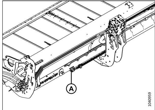
Figure 3.85: Boulons de réglage de la chaîne – Côté gauche représenté, côté droit similaire
