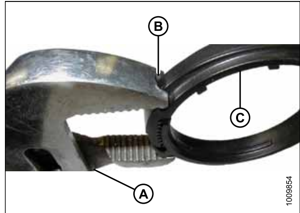
Figure 5.166: Pince multiprise modifiée
