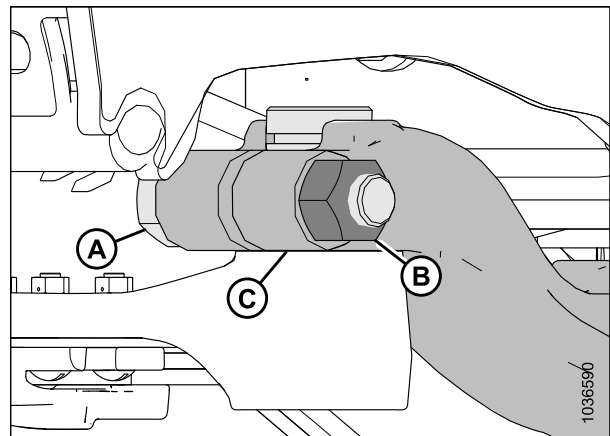
Figure 5.39: Tête de couteau
