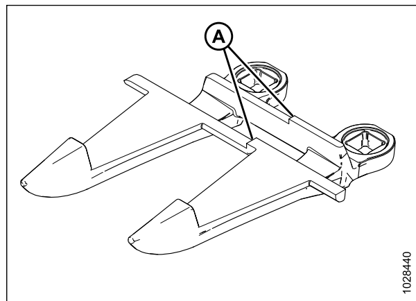
Figure 5.58: Doigt de couteau central pointus
