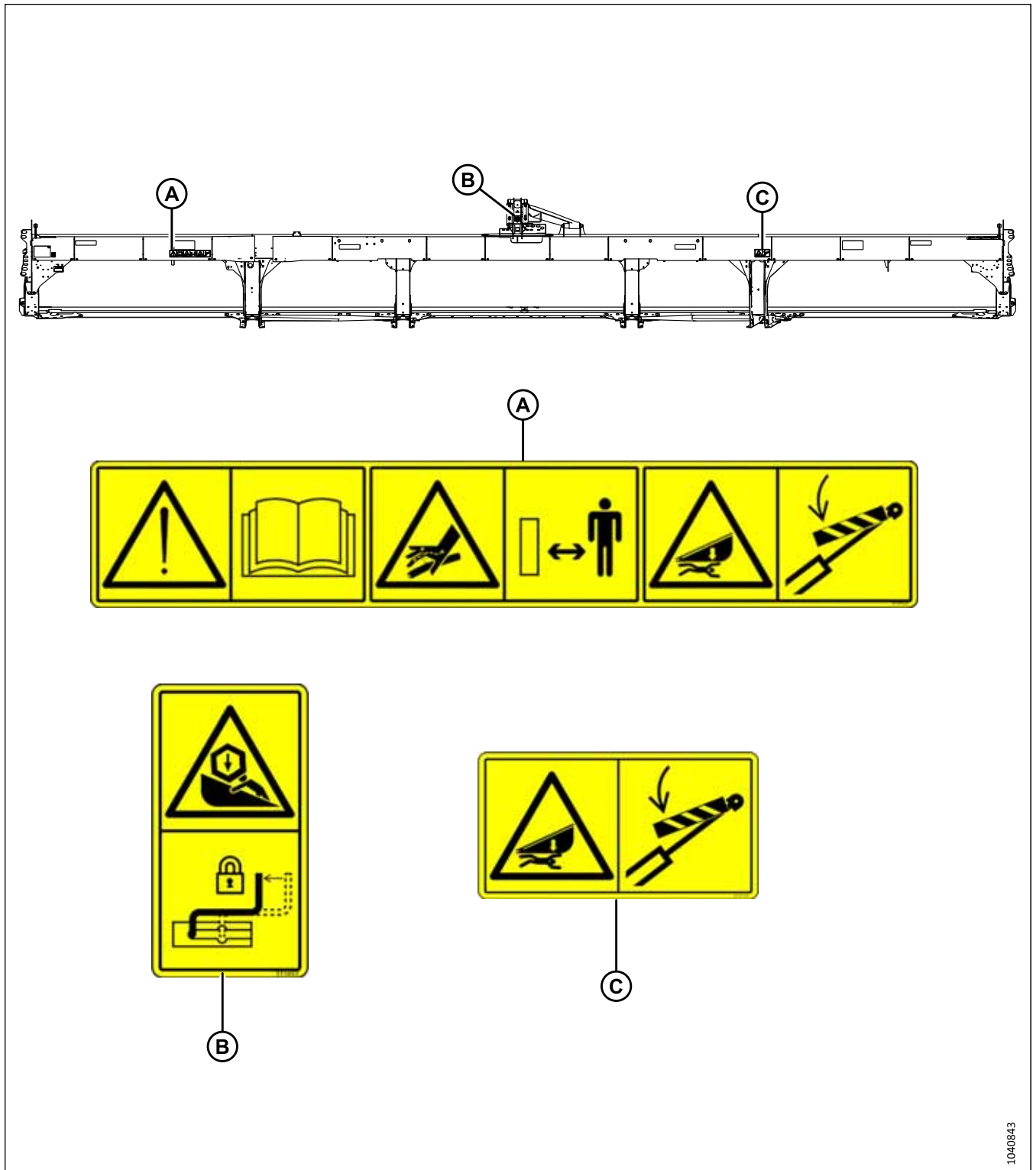
Figure 1.26: Tube arrière – Plateforme de coupe à tapis D235
