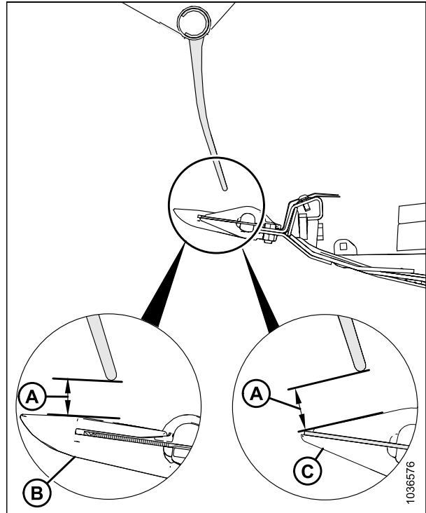
Figure 5.136: La mesure du bout du doigt à la protection
