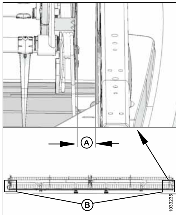
Figure 5.144: Écartement entre le rabatteur et la tôle d'extrémité
