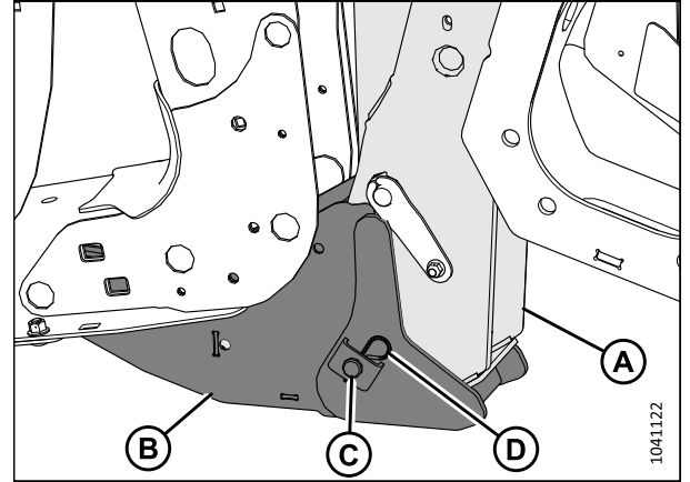
Figure 4.45: Articulation de levage de l'andaineuse et étau de la plateforme
