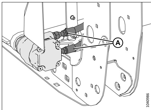
Figure 3.92: Moteur du tablier de droite
