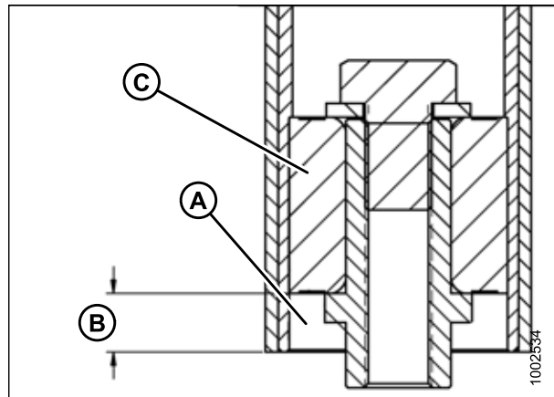
Figure 5.108: Roulement de rouleau libre
