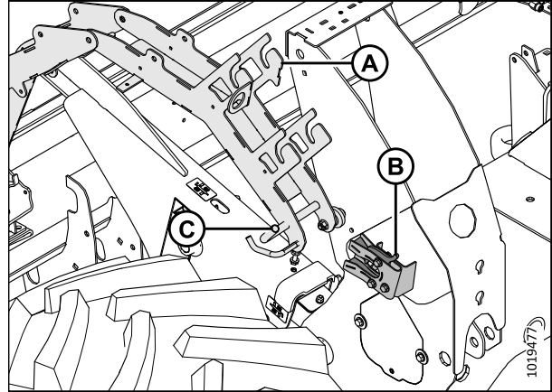
Figure 4.166: Système de gestion des flexibles hydrauliques
