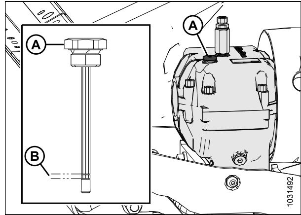
Figure 5.85: Boîtier d'entraînement de couteau
