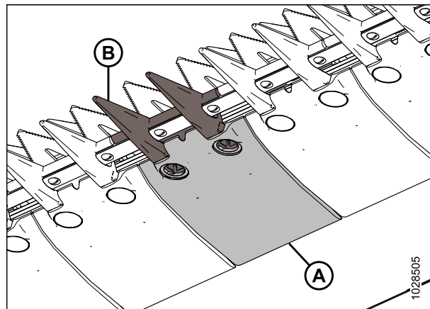
Figure 5.71: Doigts de couteau court et plaque d'usure
