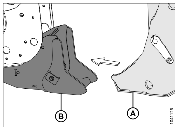
Figure 4.89: Étauçon de la plateforme et support
