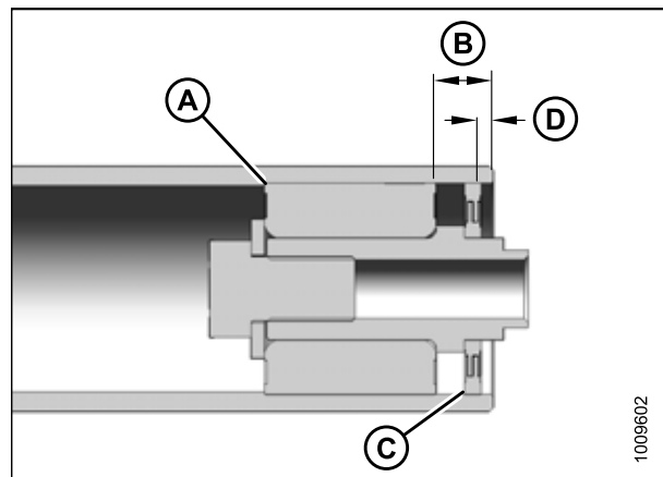
Figure 5.119: Roulement de rouleau
