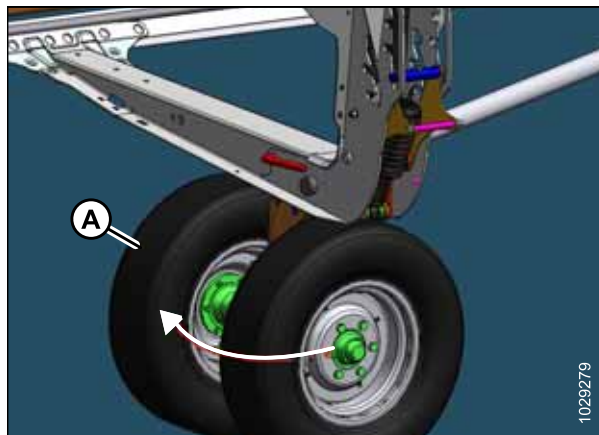
Figure 3.121: Roues de transport avant
