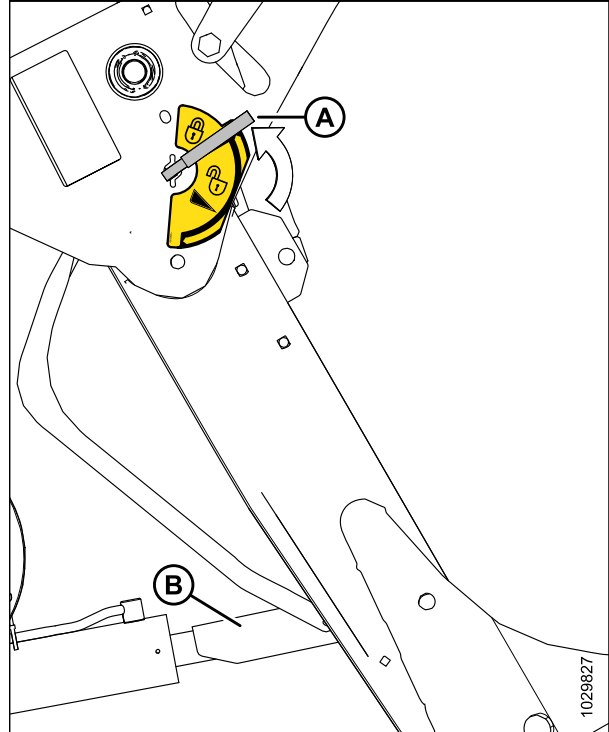
Figure 4.63: Levier du support de sécurité
