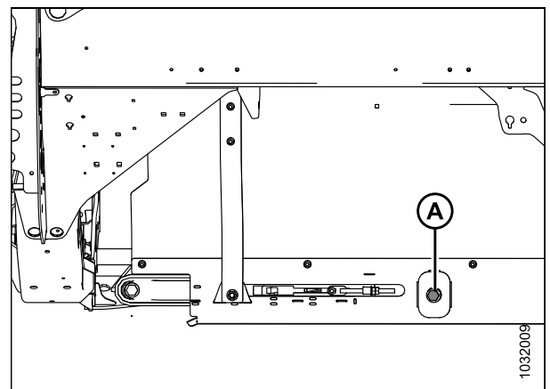
Figure 5.102: Tendeur - Côté gauche illustré
