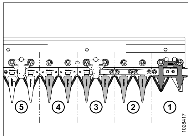
Figure 5.51: Doigt de couteaux pointus du côté de la conduite
