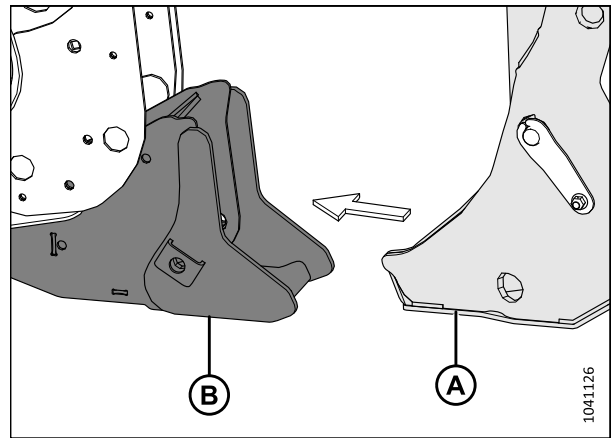
Figure 4.25: Étançon de la plateforme et support
