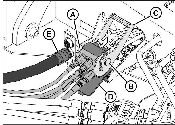
Figure 4.111: Multicoupleur du tapis/rabatteur
