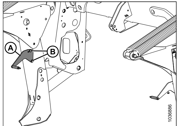
Figure 4.124: Support du blindage de formage – Série R2
