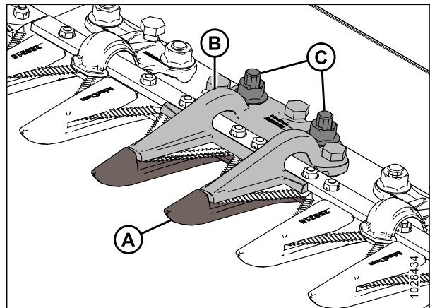
Figure 5.57: Doigt de couteau central pointus
