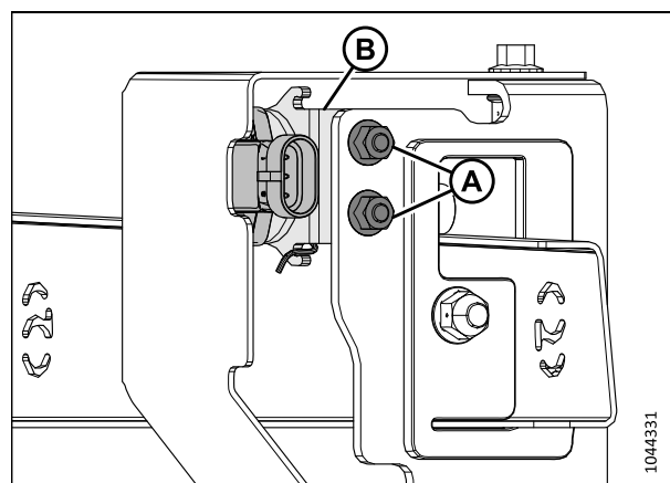
Figure 3.58: Capteur avant-arrière
