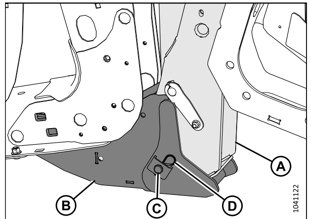
Figure 4.31: Articulation de levage de l'andaineuse et étau de la plateforme
