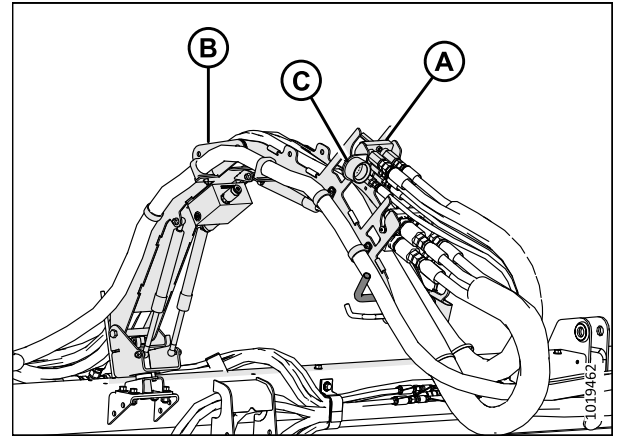
Figure 4.163: Système de gestion des flexibles hydrauliques
