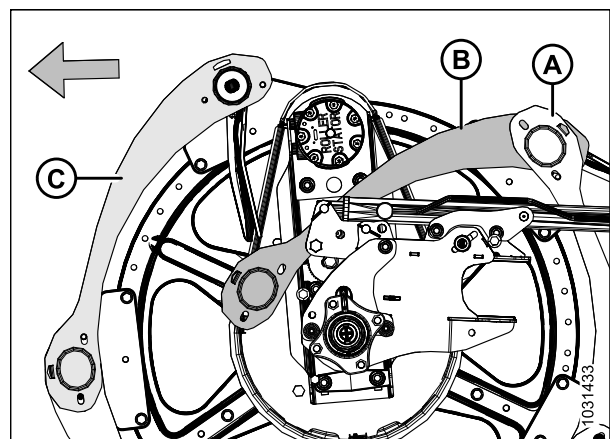
Figure 5.198: Boucliers des rabatteurs - Extrémité arrière intérieure
