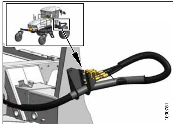
Figure 4.54: Rangement des flexibles du rabatteur
