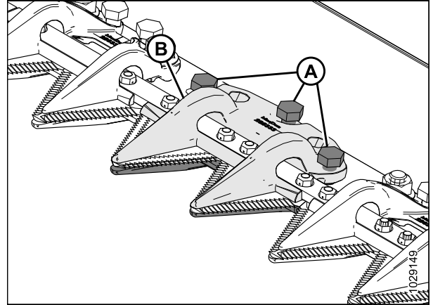
Figure 5.79: Doigt de couteau central
