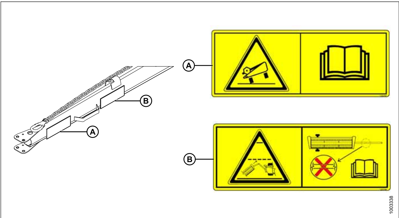
Figure 1.31: Barre de remorquage EasyMove MC pour transport (en option)
