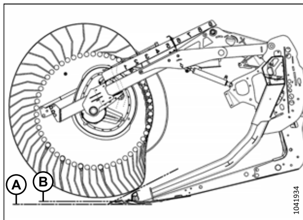
Figure 3.59: Profil des doigts – Position 1 de la came
