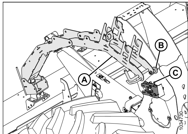
Figure 4.142: Étauçon extérieur gauche de l'andaineuse
