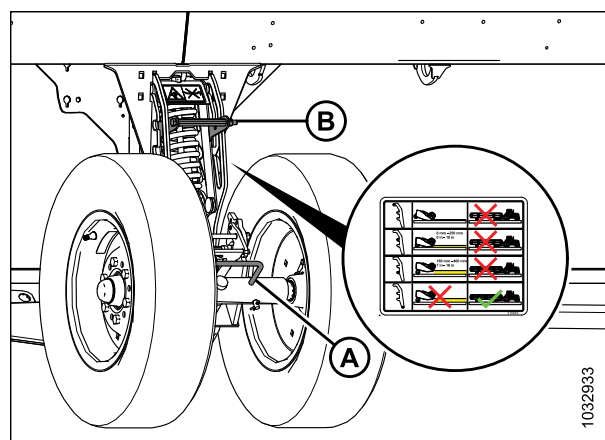
Figure 3.35: Roue gauche
