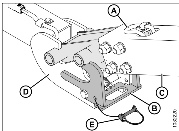
Figure 3.132: Extension de la barre de remorquage
