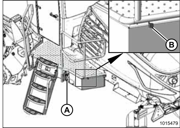
Figure 4.160: Plateforme de gauche
