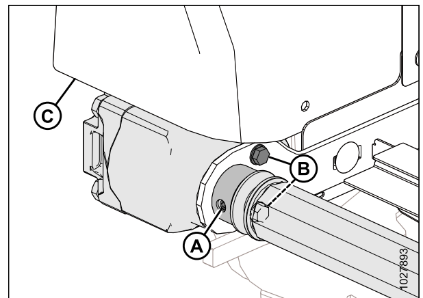
Figure 5.121: Rouleau d'entraînement
