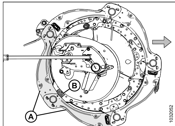
Figure 5.204: Supports des blindages du rabatteur
