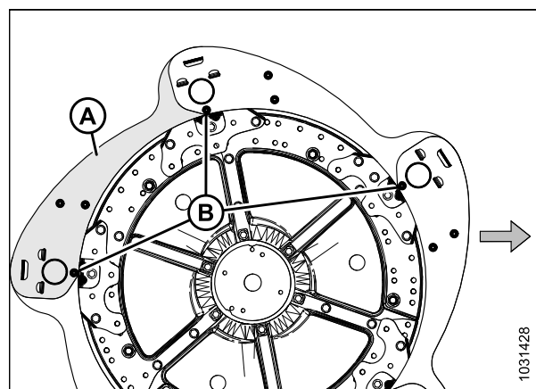
Figure 5.189: Boucliers des rabatteurs - Extrémité de came intérieure
