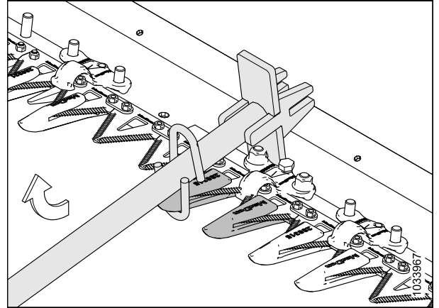
Figure 5.46: Réglage vers le haut - Doigt pointu
