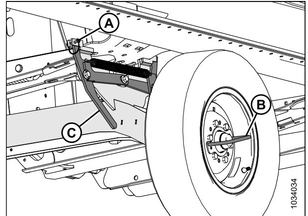
Figure 3.114: Essieu de transport droit verrouillé dans la position de transport
