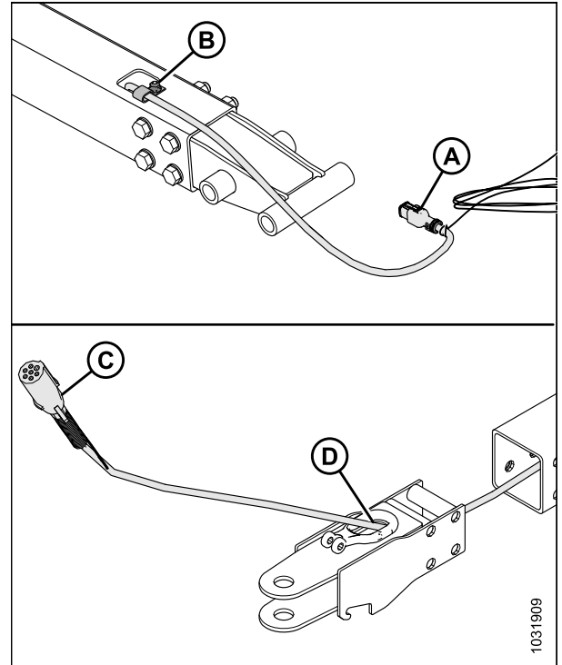
Figure 5.232: Démontage de l'adaptateur de remorquage de la chape
