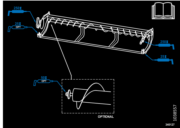
Figure 5.14: Autocollant indiquant le point de graissage pour les plateformes à couteau unique avec vis transversale supérieure à une pièce
