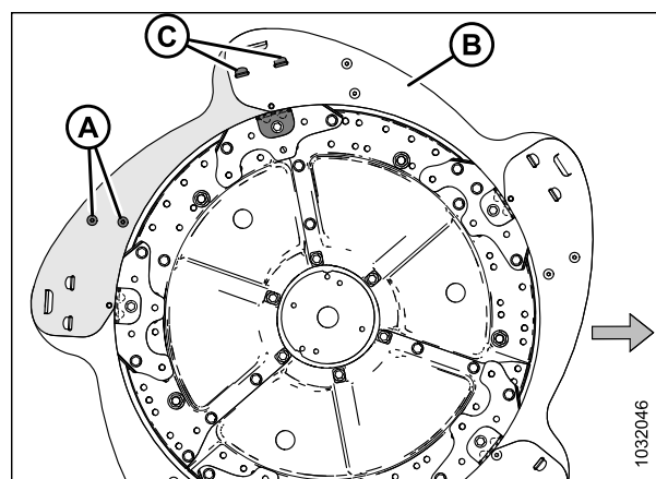
Figure 5.190: Boucliers des rabatteurs - Extrémité de came intérieure
