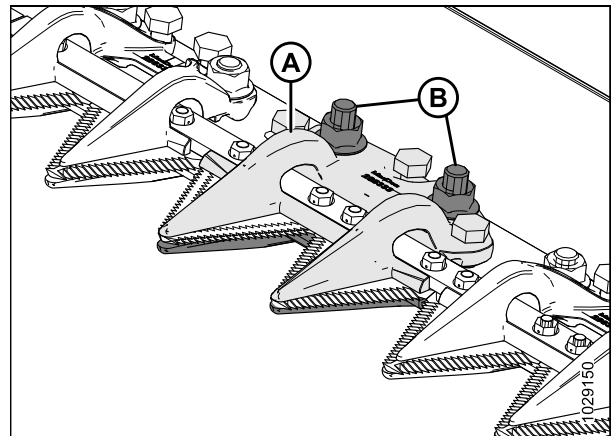
Figure 5.80: Doigt de couteau central
