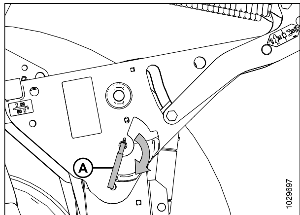
Figure 4.34: Support de sécurité du levier
