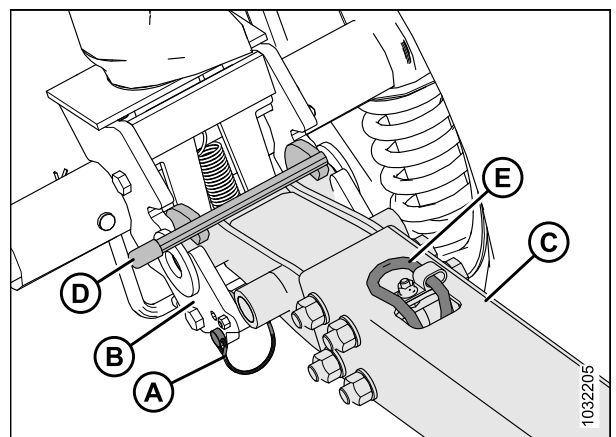
Figure 3.135: Barre de remorquage et pivot de transport gauche
