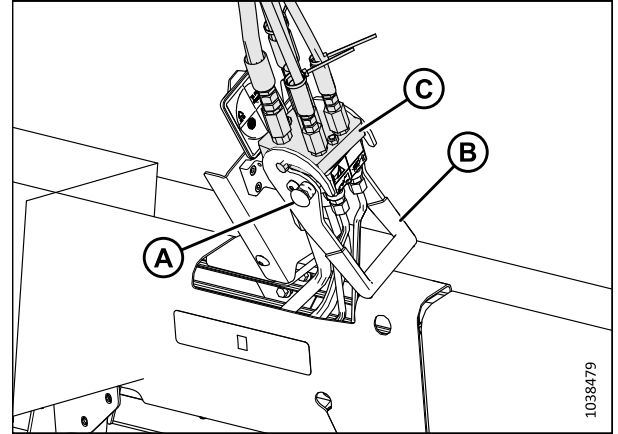
Figure 4.56: Attelage des flexibles du rabatteur
