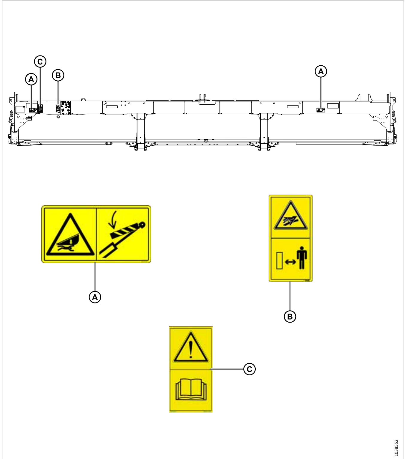
Figure 1.24: Tube arrière – Plateforme de coupe à tapis D225
