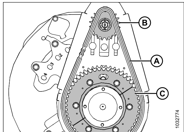
Figure 5.222: Pignon double – Configuration à grande vitesse
