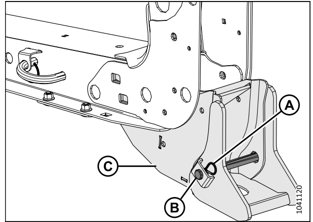
Figure 4.80: Étançon de la plateforme et support
