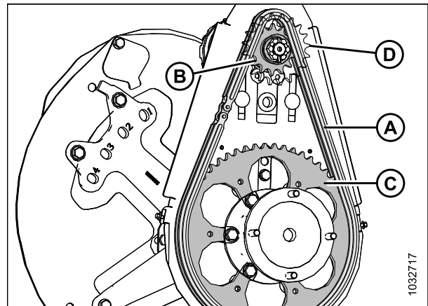
Figure 5.221: Pignon double – Configuration à couple élevé
