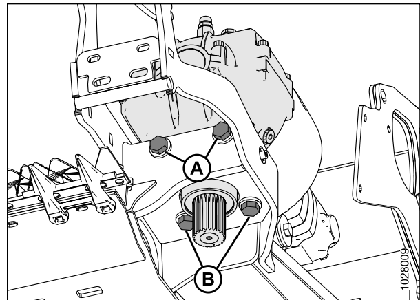
Figure 5.86: Boîtier d'entraînement du couteau - Vue d'en bas
