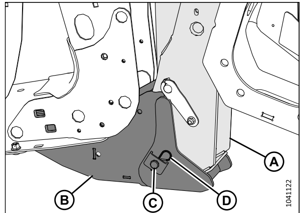
Figure 4.95: Articulation de levage de l'andaineuse et étau de la plateforme
