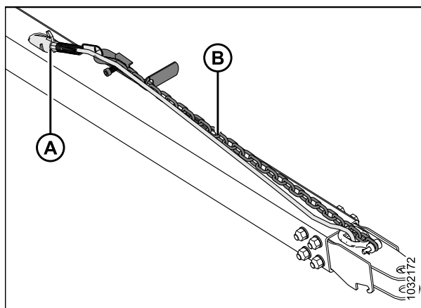
Figure 3.95: Assemblage de la barre de remorquage
