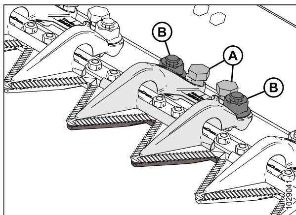
Figure 5.74: Doigt de couteau court, rabatteur
