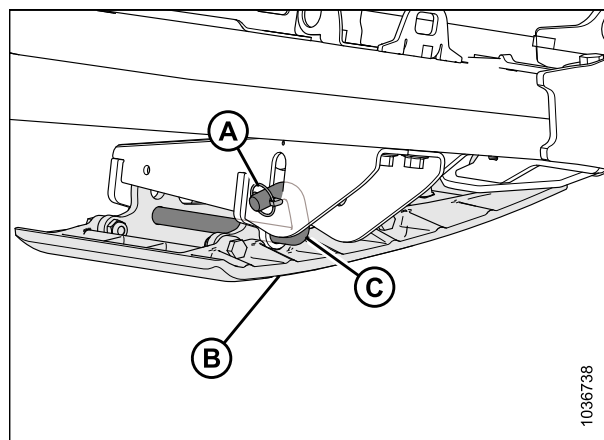
Figure 3.37: Patin extérieur
