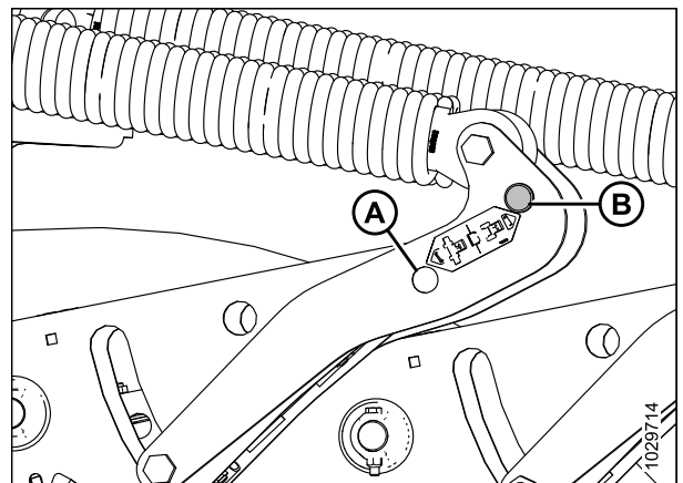
Figure 4.20: Articulation de flottement de la plateforme
