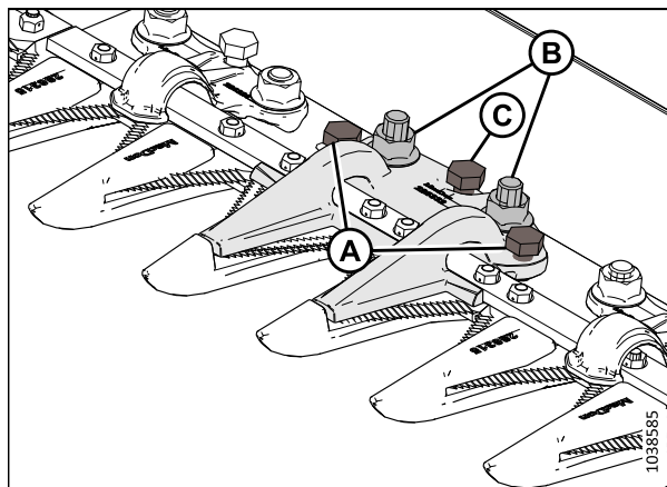
Figure 5.64: Rabatteur pointu central
