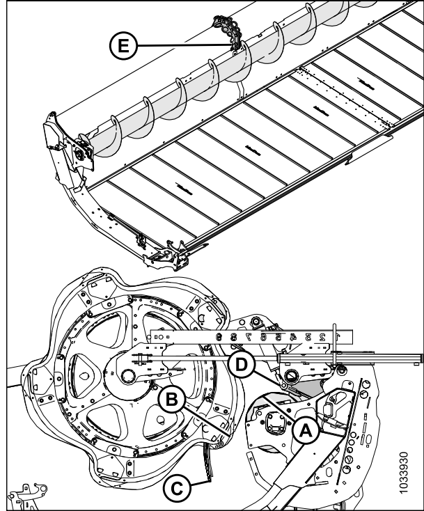
Figure 3.70: Lieux de contrôle de l'UCA
