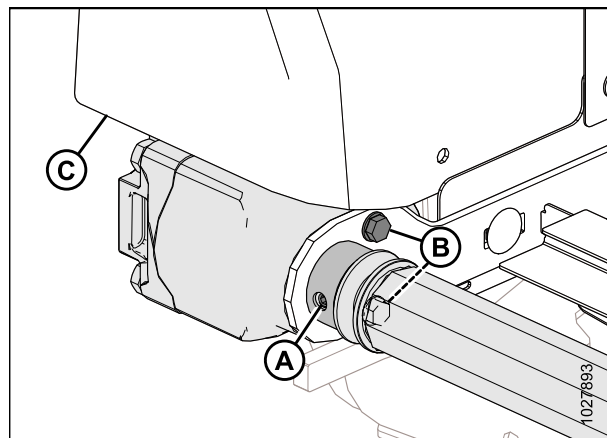
Figure 5.115: Rouleau d'entraînement
