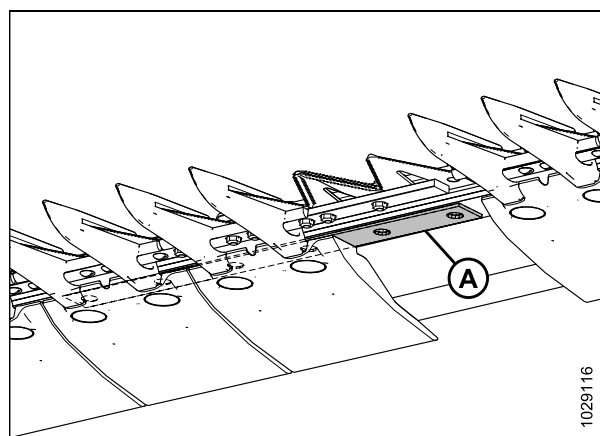
Figure 5.59: Barre de coupe
