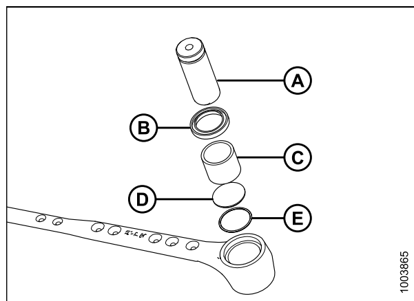
Figure 5.35: Assemblage du roulement de la tête de couteau
