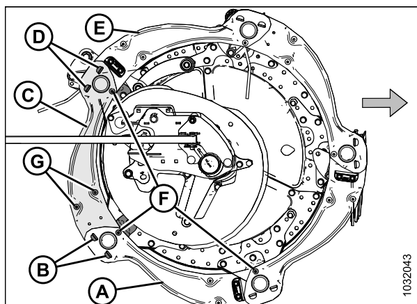
Figure 5.188: Boucliers des rabatteurs - Extrémité de came extérieure
