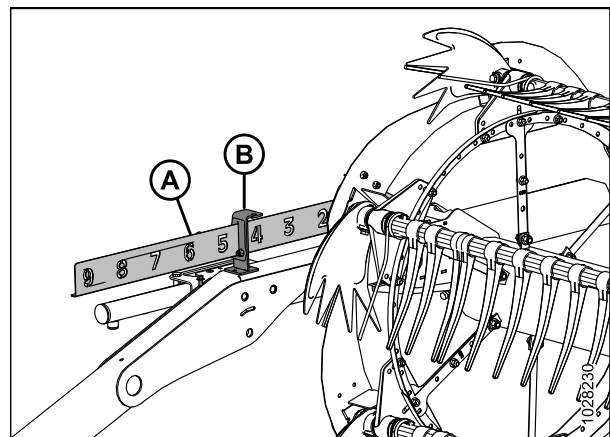
Figure 3.46: Indicateur d'avant-arrière
