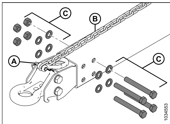
Figure 5.226: Démontage de l'adaptateur de remorquage de l'anneau d'attelage
