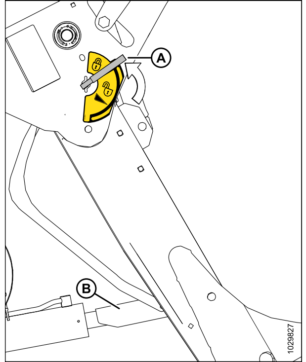
Figure 4.30: Support de sécurité
