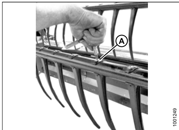
Figure 5.151: Installation des doigts en plastique
