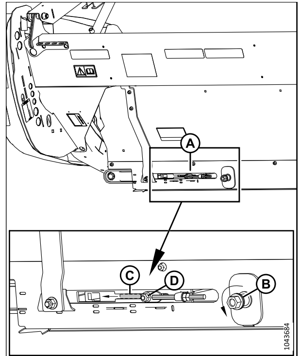
Figure 5.89: Réglage du tendeur gauche
