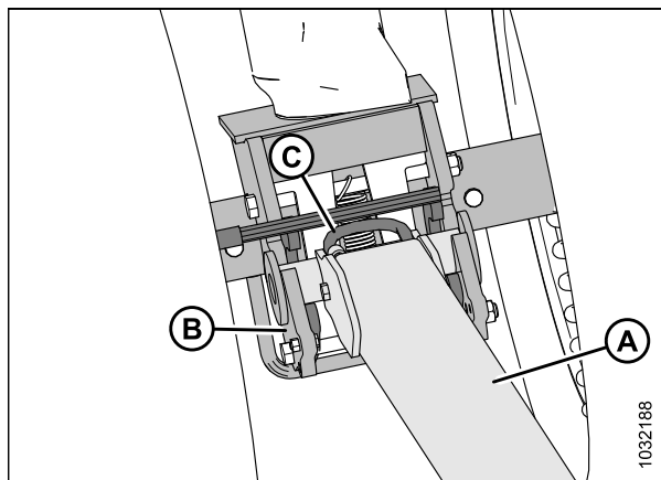
Figure 3.100: Verrou désengagé de l'extension
