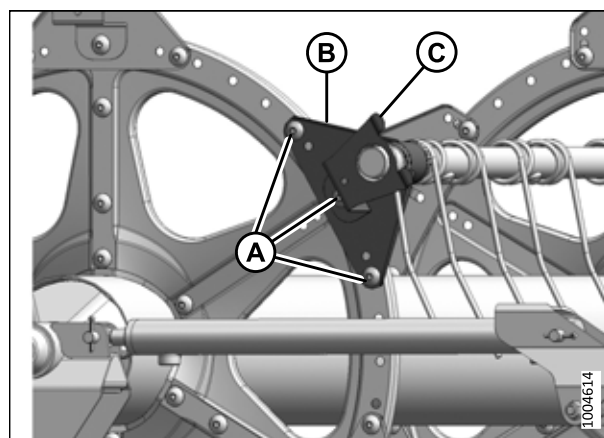
Figure 5.176: Extrémité arrière
