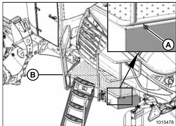
Figure 4.148: Plateforme de gauche
