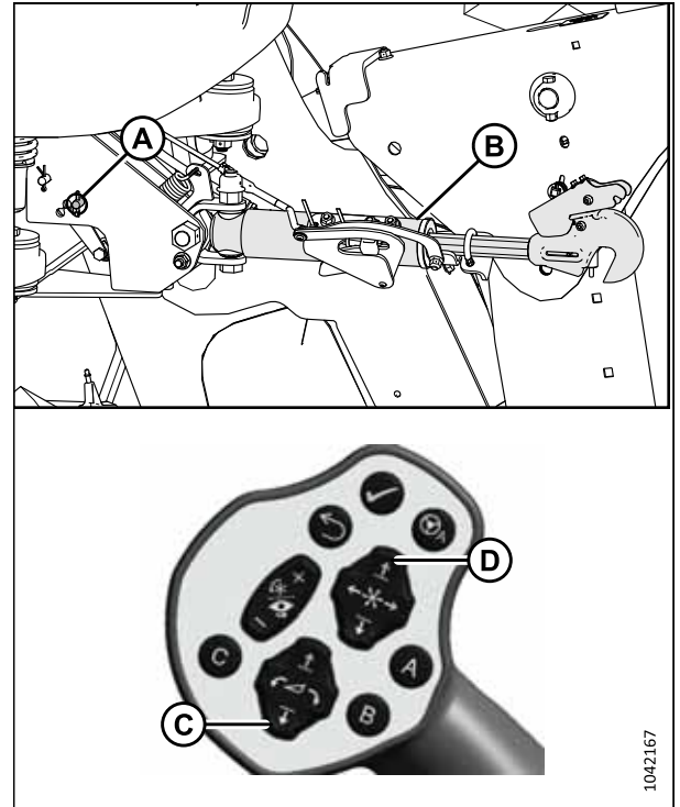
Figure 4.129: Vérin d'inclinaison à alignement automatique
