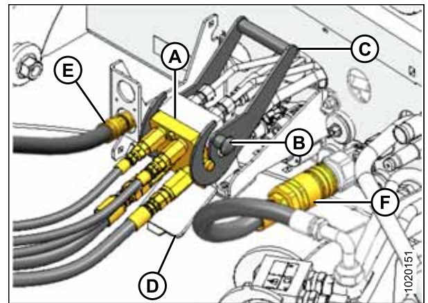
Figure 4.144: Multicoupleur du tapis/rabatteur
