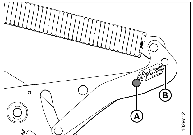
Figure 4.47: Articulation de flottement de la plateforme
