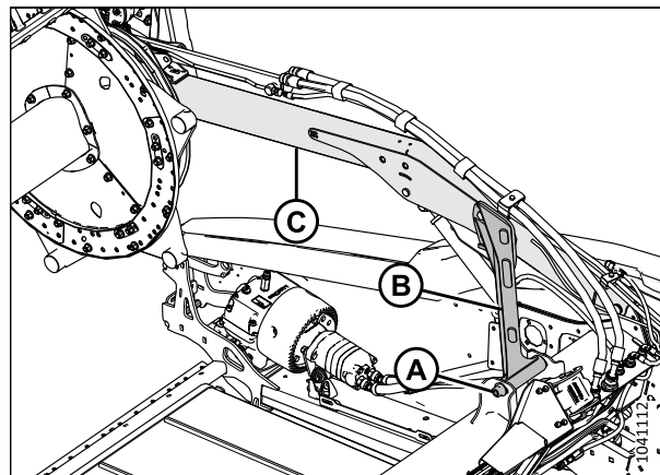
Figure 5.143: Bras de support de rabatteur unique
