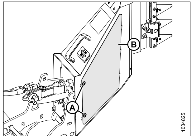
Figure 5.244: Capot d'accès aux couteaux verticaux
