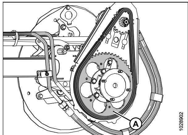
Figure 5.211: Entraînement du rabatteur
