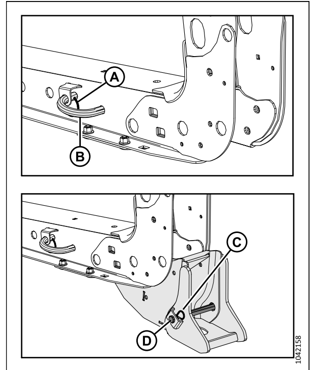
Figure 4.127: Étauçon de la plateforme de coupe – Côté gauche illustré
