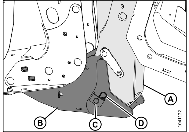
Figure 4.75: Patte de la plateforme et articulation de levage de l'andaineuse reliées par le support de la plateforme
