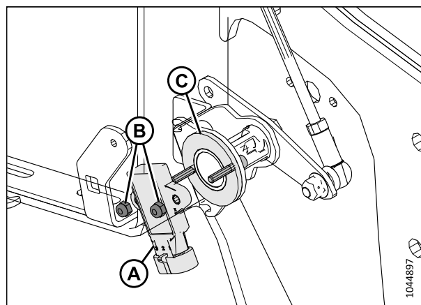
Figure 3.44: Capteur de hauteur du rabatteur – Bras droit du rabatteur
