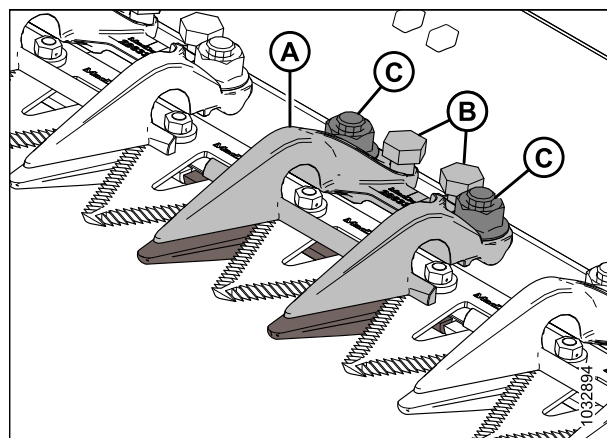
Figure 5.72: Doigt de couteau court
