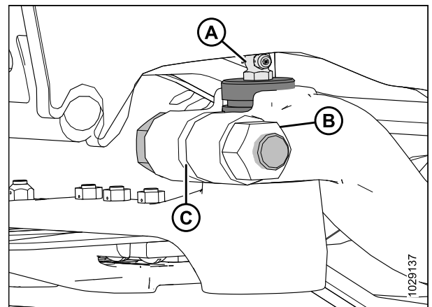
Figure 5.33: Tête de couteau
