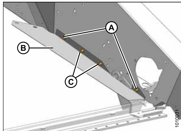
Figure 5.133: Déflecteur avant
