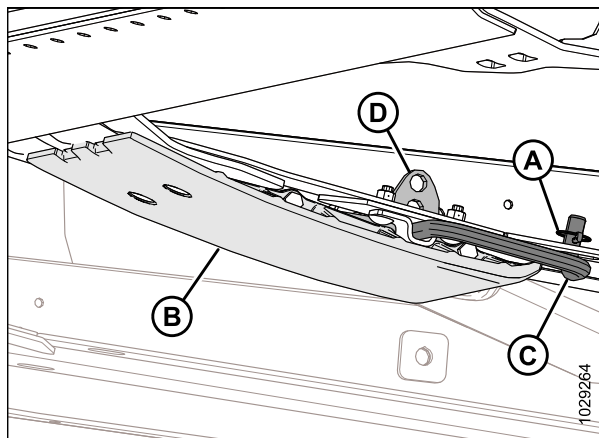
Figure 3.36: Patin intérieur
