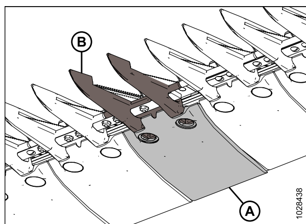
Figure 5.60: Doigt du couteau central pointu et plaque d'usure
