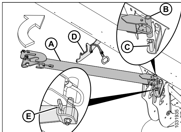
Figure 3.104: Stockage de l'extension de la barre de remorquage
