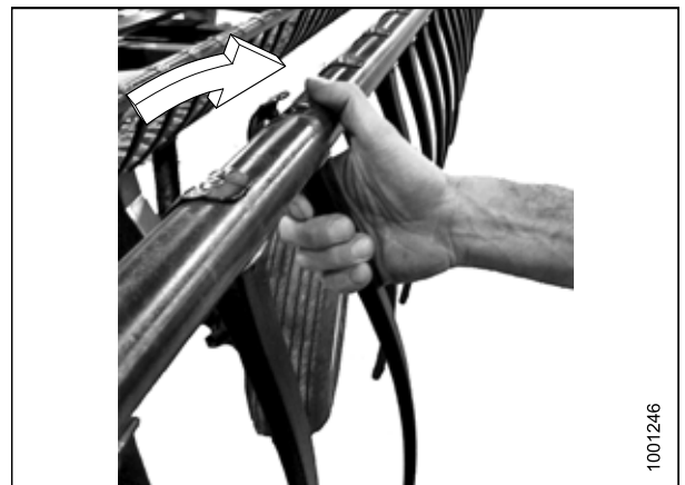
Figure 5.150: Installation des doigts en plastique
