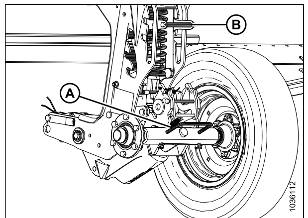
Figure 3.112: Roues de transport gauches dans la position de rangement la plus haute
