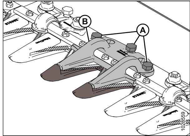
Figure 5.61: Doigt de couteau central pointus
