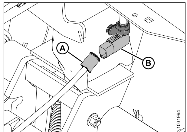
Figure 3.98: Connexion électrique de la barre de remorquage
