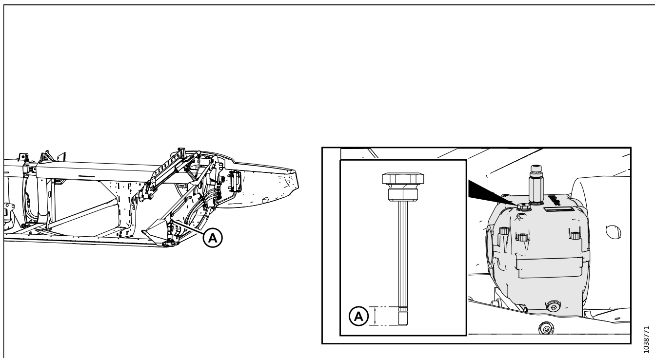
Figure 5.10: Boîtier d'entraînement de couteau
