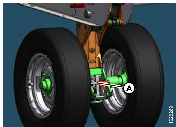
Figure 3.119: Roues de transport avant
