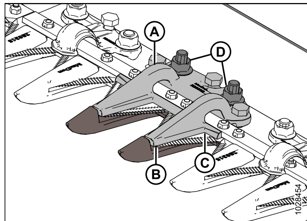
Figure 5.63: rabatteur pointu central
