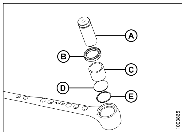
Figure 5.36: Assemblage du roulement de la tête de couteau
