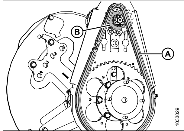
Figure 5.217: Pignon double en configuration à couple élevé
