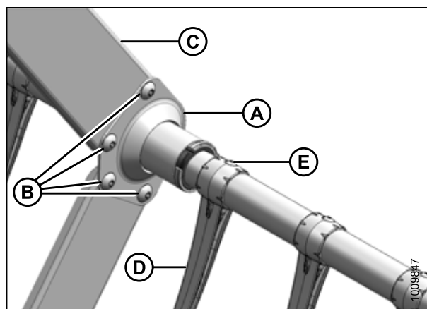
Figure 5.182: Support du kit de renforcement des tubes à doigts en option
