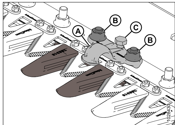
Figure 5.54: Doigts de couteau pointus
