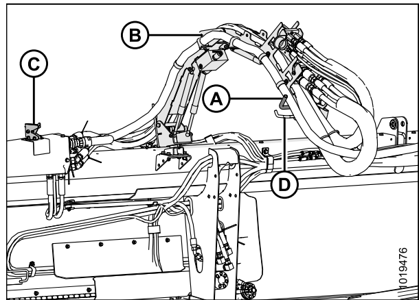
Figure 4.167: Système de gestion des flexibles hydrauliques
