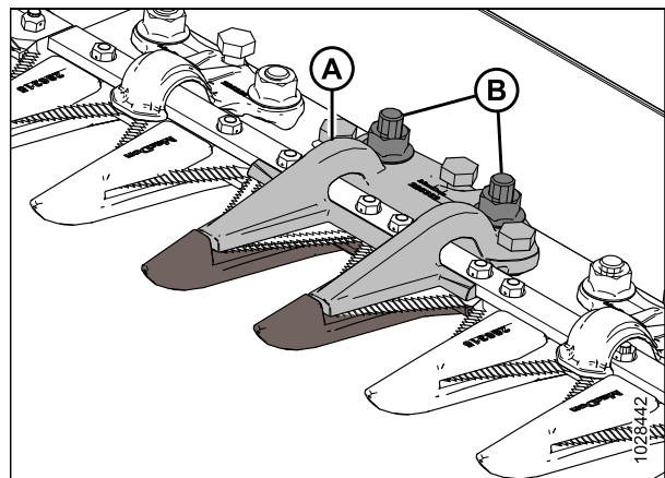
Figure 5.62: Doigt de couteau central pointus
