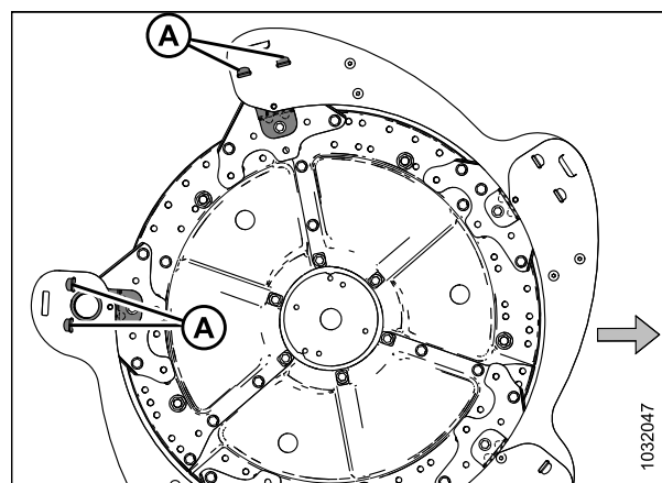
Figure 5.191: Bouclier du rabatteur enlevé - Extrémité de came intérieure
