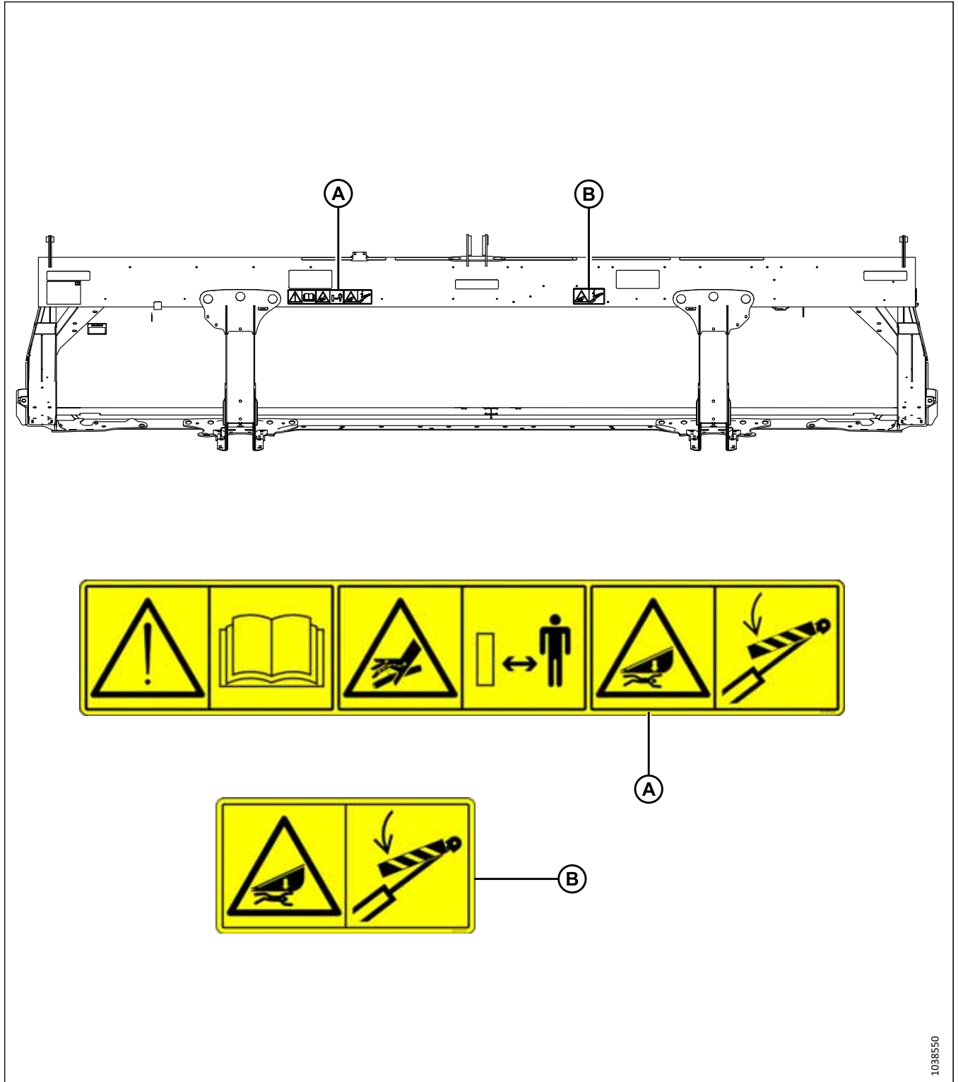
Figure 1.22: Tube arrière – Plateforme de coupe à tapis D215
