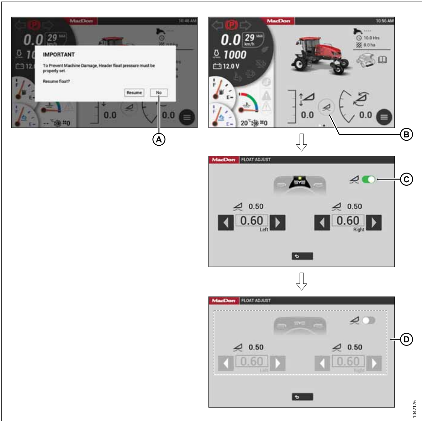
Figure 4.128: Retrait du flottement
