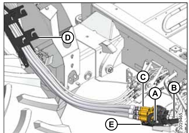
Figure 4.110: Multicoupleur de l'entraînement de couteau/rabatteur
