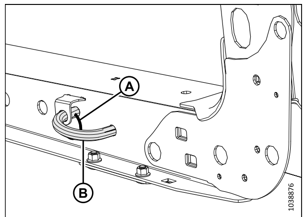
Figure 4.84: Étauçon de la plateforme
