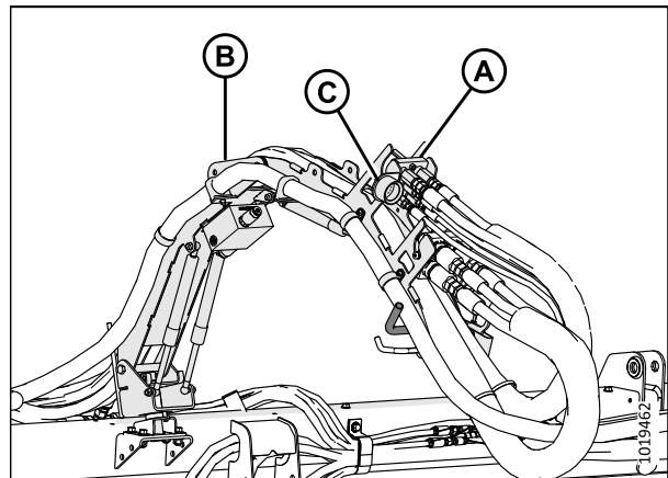
Figure 4.112: Système de gestion des flexibles hydrauliques
