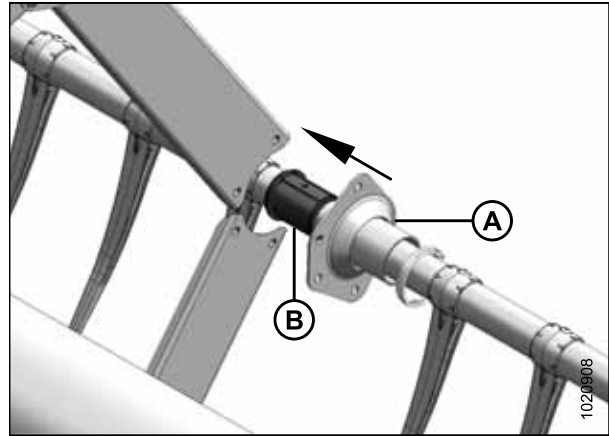
Figure 5.178: Support du kit de renforcement des tubes à doigts en option
