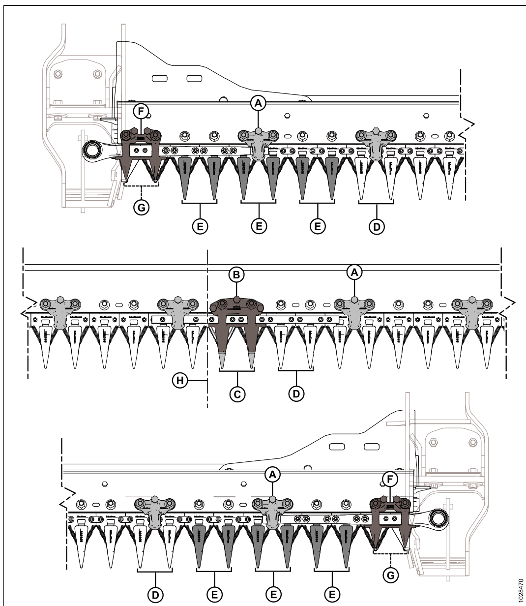
Figure 5.45: Emplacement des doigts de couteaux pointus et mécanismes de retenue
