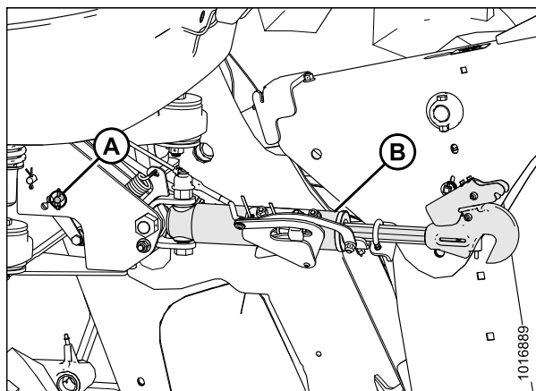
Figure 4.81: Vérin d'inclinaison à alignement automatique
