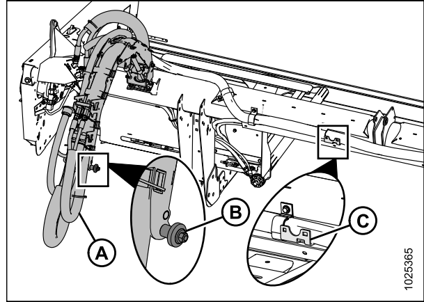
Figure 4.140: Système de gestion des tuyaux hydrauliques – Plateformes de coupe à tapis D215
