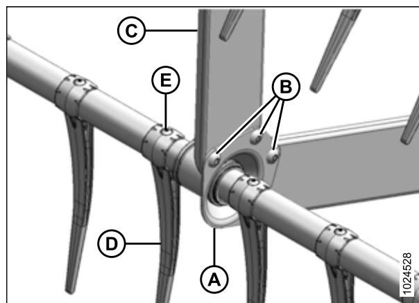
Figure 5.183: Support opposé du kit de renforcement des tubes à doigts en option
