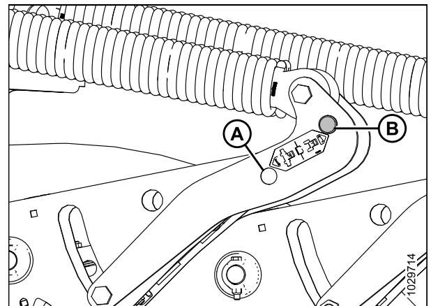
Figure 4.4: Articulation de flottement de la plateforme
