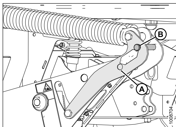
Figure 4.67: Articulation de flottement de la plateforme
