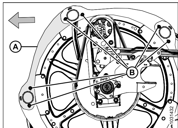
Figure 5.197: Boucliers des rabatteurs - Extrémité arrière intérieure
