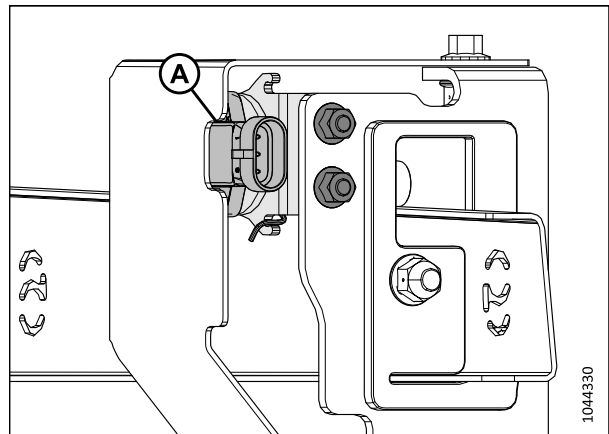
Figure 3.56: Capteur avant-arrière
