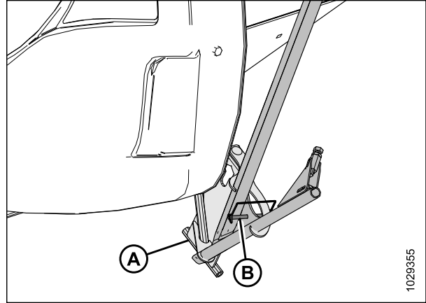
Figure 3.83: Stockage de la tige de diviseur à riz
