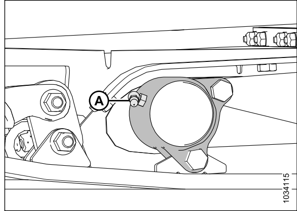
Figure 5.5: Rouleau libre du tapis d'alimentation
