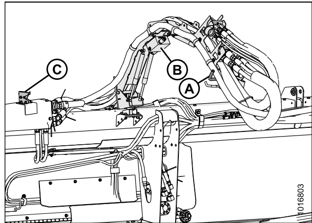
Figure 4.141: Système de gestion des flexibles hydrauliques
