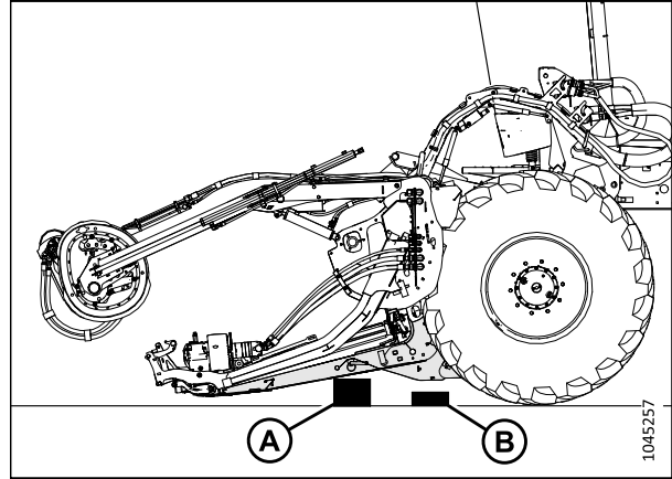
Figure 4.117: Réglage de la plateforme au sol
