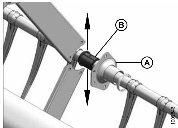
Figure 5.164: Support de kit de renforcement de tubes à doigts
