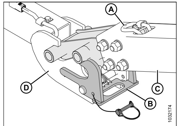
Figure 3.97: Barre de remorquage/Articulation de l'extension
