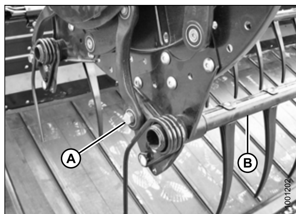
Figure 5.170: Extrémité de la came
