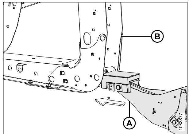
Figure 4.10: Étançon de la plateforme et support
