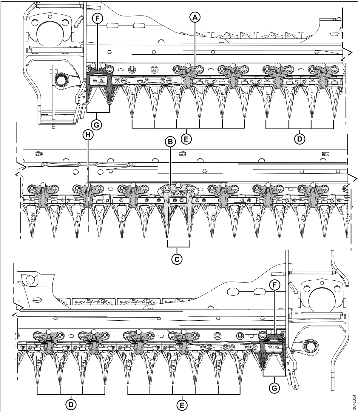
Figure 5.44: Emplacement des doigts pointus et mécanismes de retenue
