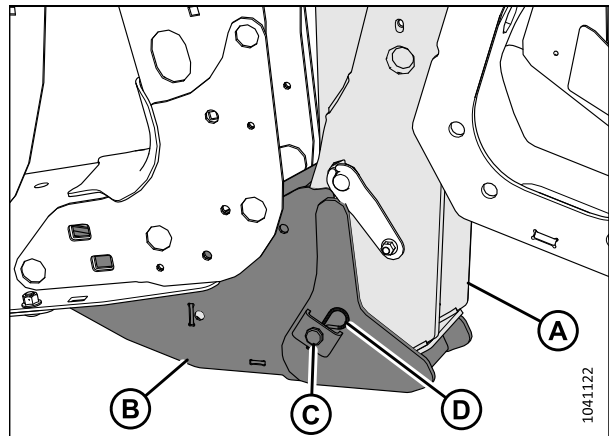
Figure 4.118: Patte de la plateforme et articulation de levage de l'andaineuse reliées par le support de la plateforme
