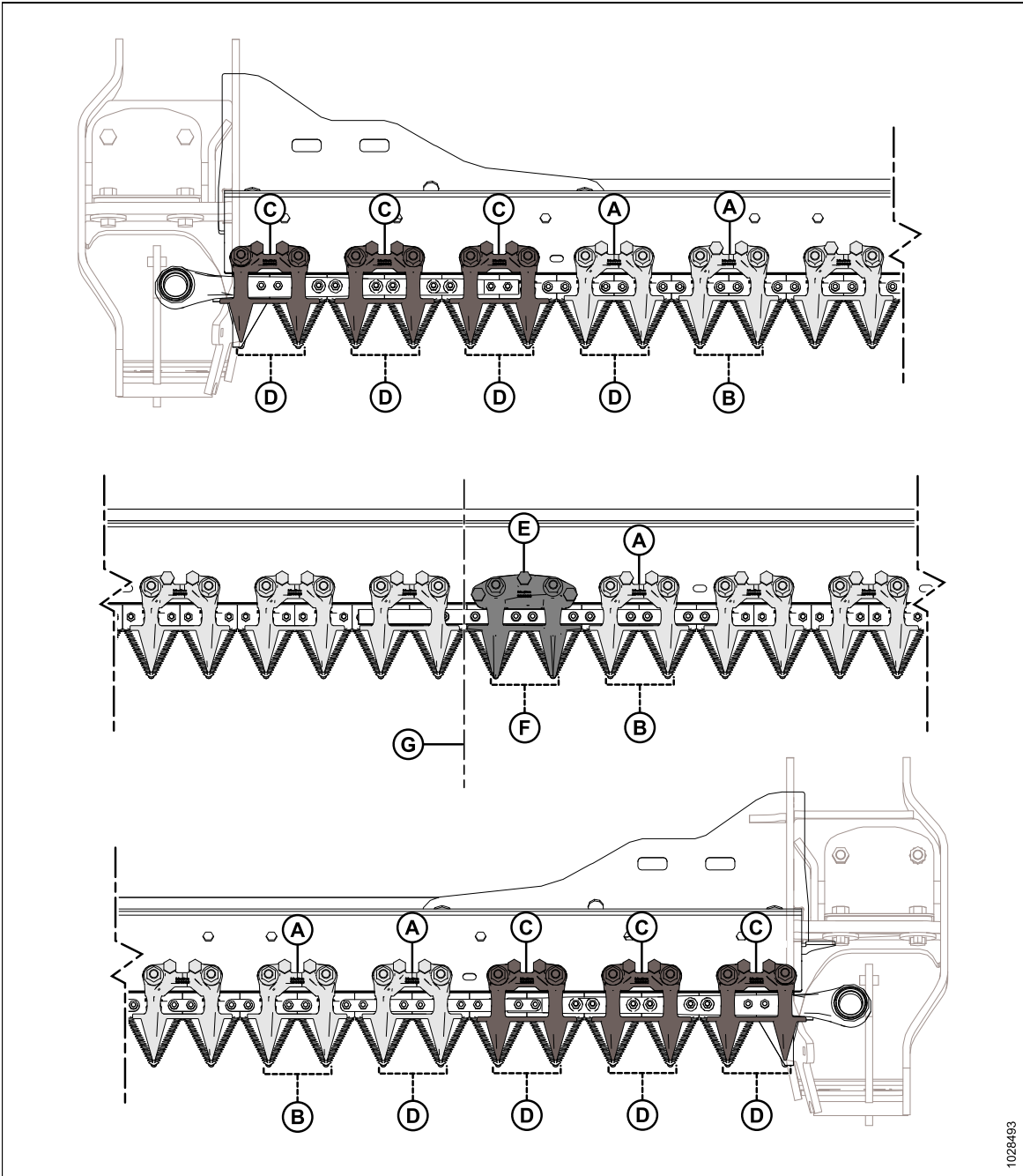
Figure 5.68: Emplacement des doigts de couteaux courts et mécanismes de retenue
