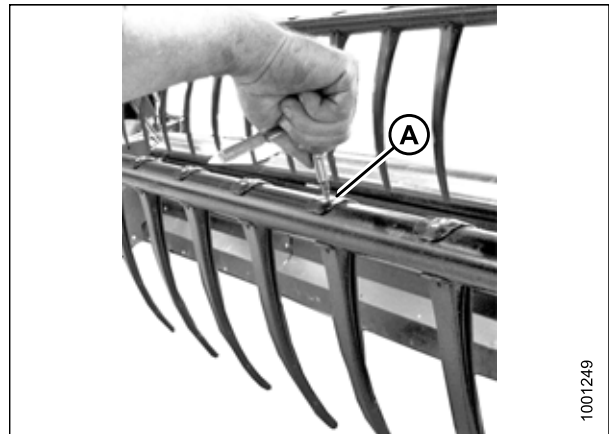
Figure 5.148: Retrait des doigts en plastique
