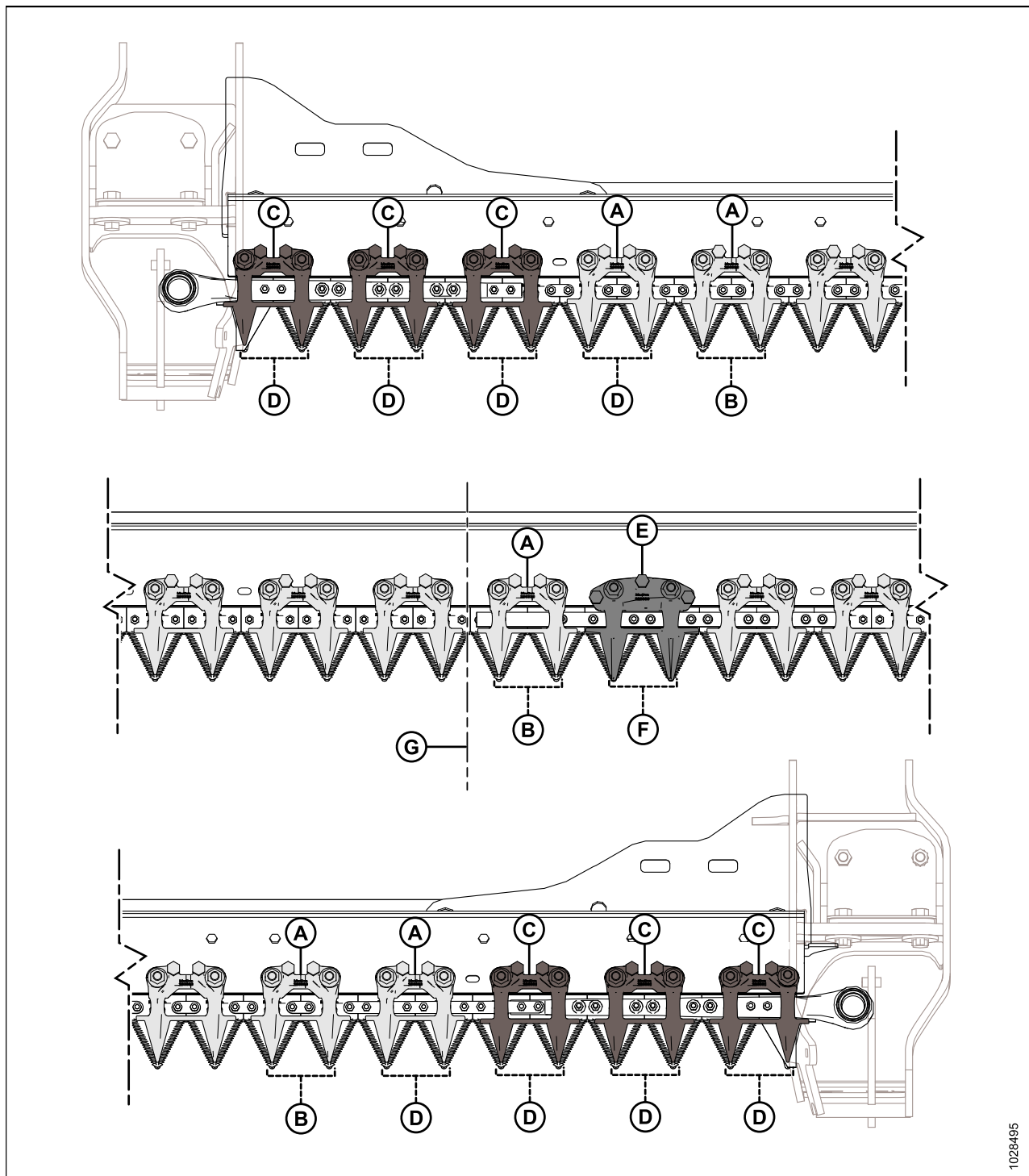
Figure 5.67: Emplacement des doigts de couteau court et rabatteurs – Plateformes à couteau double
