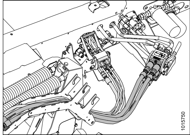
Figure 4.146: Acheminement des coupleurs et flexibles hydrauliques
