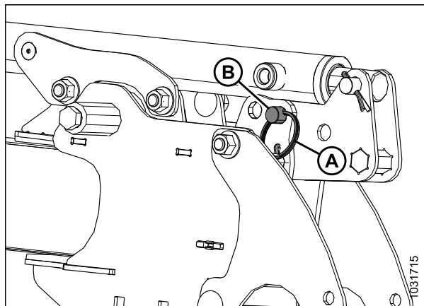
Figure 3.50: Réglage des vérins avant-arrière de type 1 – Position avant
