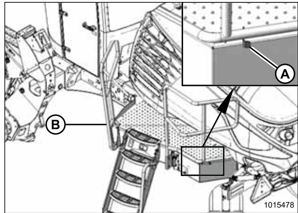
Figure 4.107: Plateforme de gauche
