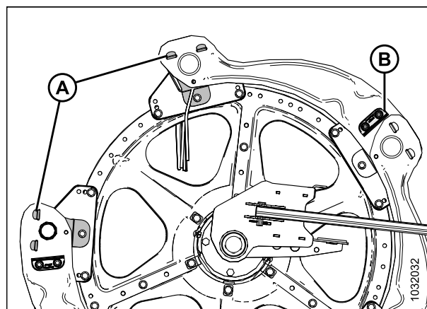
Figure 5.195: Bouclier du rabatteur enlevé - Extrémité arrière extérieure
