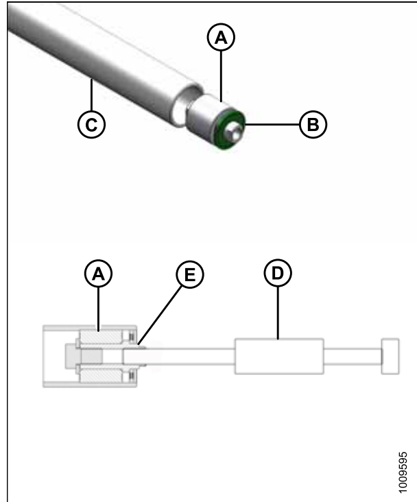
Figure 5.118: Roulement de rouleau
