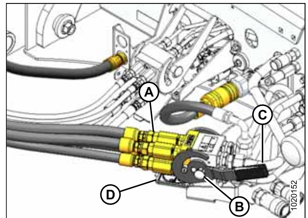
Figure 4.145: Multicoupleur de l'entraînement de couteau/rabatteur
