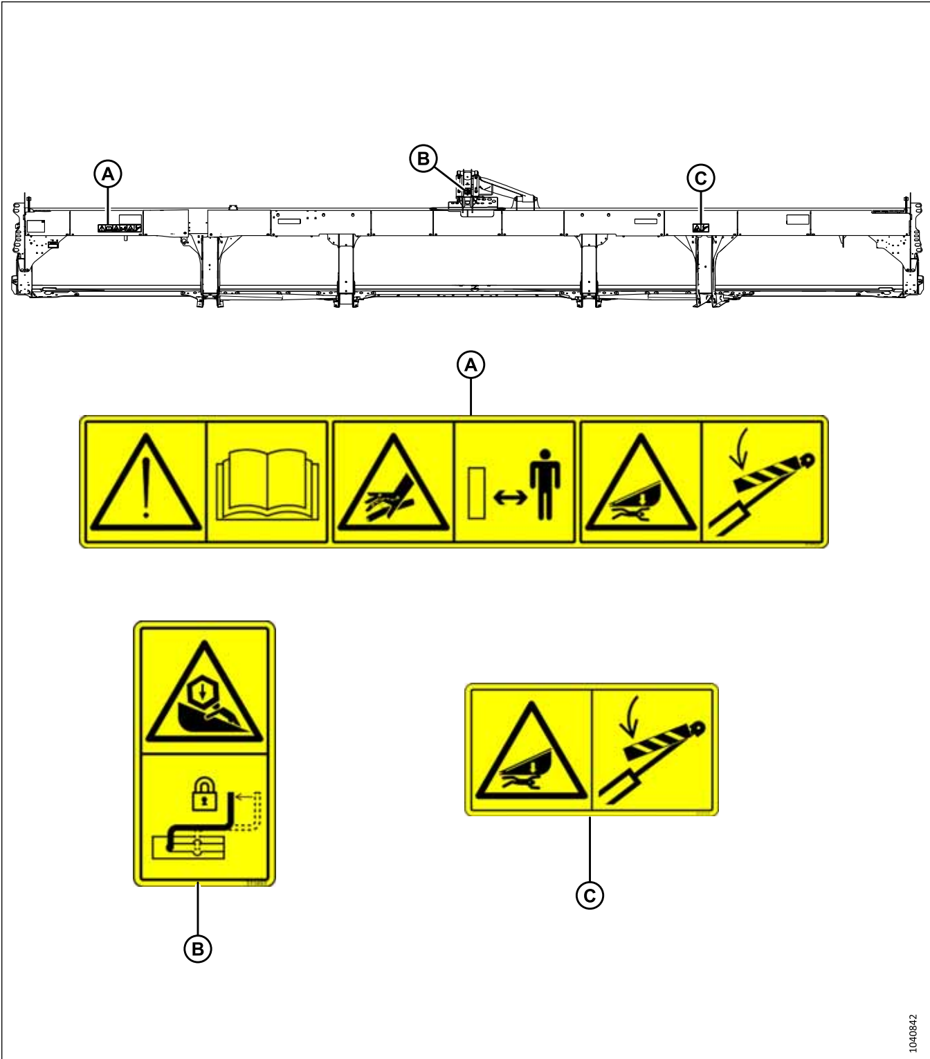
Figure 1.25: Tube arrière – Plateforme de coupe à tapis D230
