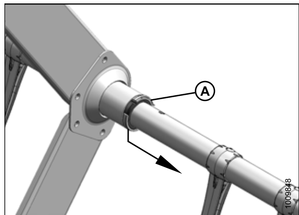
Figure 5.163: Collier de bague de kit de renforcement de tubes à doigts
