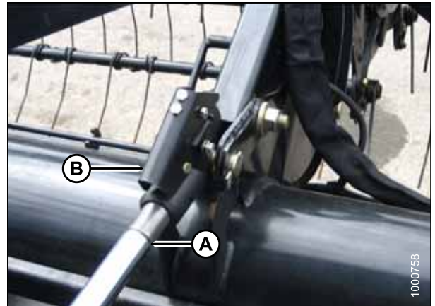
Figure 4.122: Vérin d'inclinaison hydraulique
