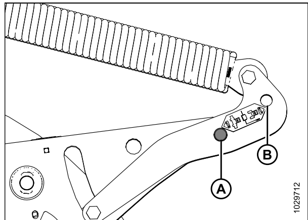
Figure 4.33: Articulation de flottement de la plateforme
