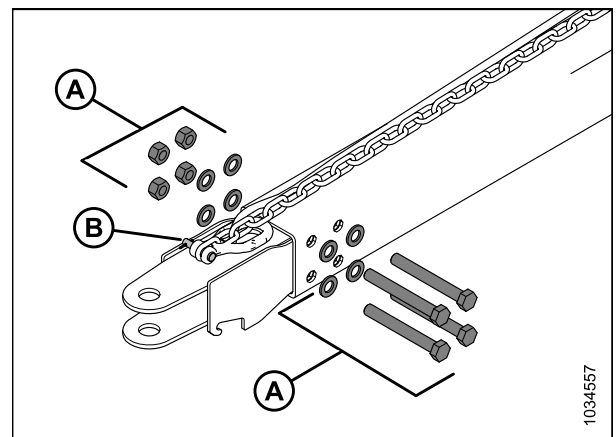
Figure 5.229: Installation de l'adaptateur d'anneau de chape
