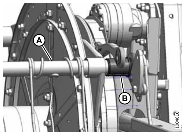
Figure 5.160: Extrémité de la came
