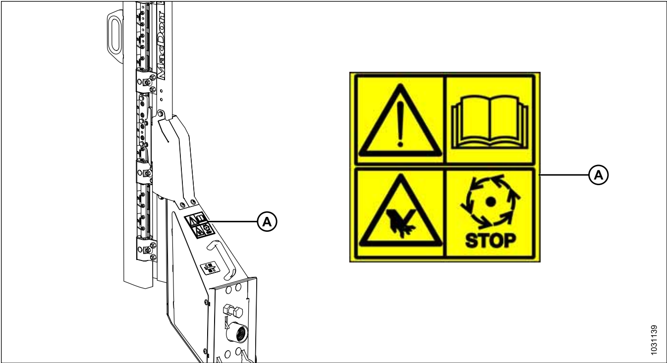
Figure 1.34: Scie verticale (en option)
