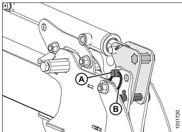
Figure 3.52: Réglage des vérins avant-arrière de type 1 – Position arrière
