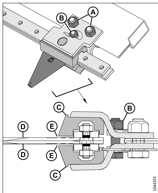
Figure 5.240: Couteau vertical (vue du dessus)
