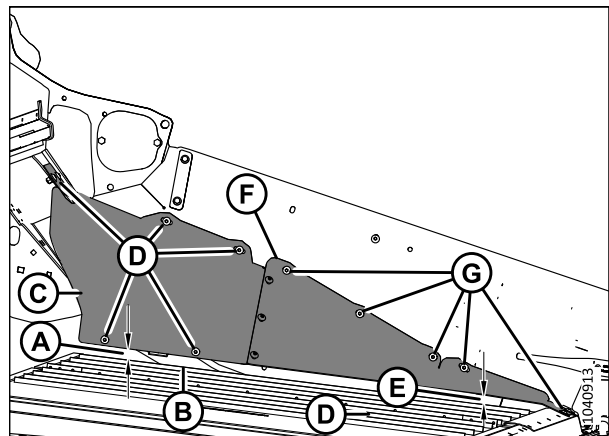
Figure 5.130: Déflecteur – Côté gauche illustré
