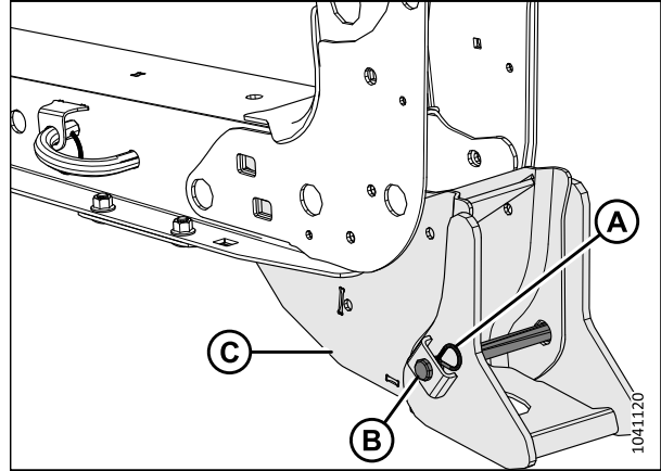
Figure 4.21: Support de la plateforme de coupe – Côté gauche illustré
