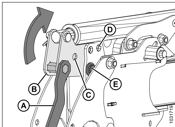
Figure 3.51: Réglage des vérins avant-arrière de type 1 – Position avant
