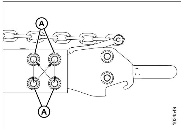
Figure 5.235: Séquence de couple
