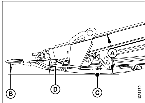
Figure 3.38: Angle de la plateforme
