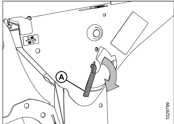
Figure 4.97: Levier du support de sécurité
