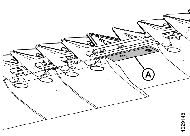
Figure 5.77: Barre de coupe
