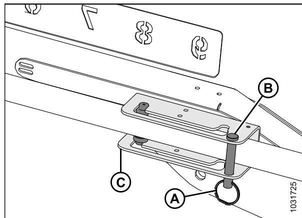
Figure 3.53: Réglage des vérins avant-arrière de type 2 – Position avant
