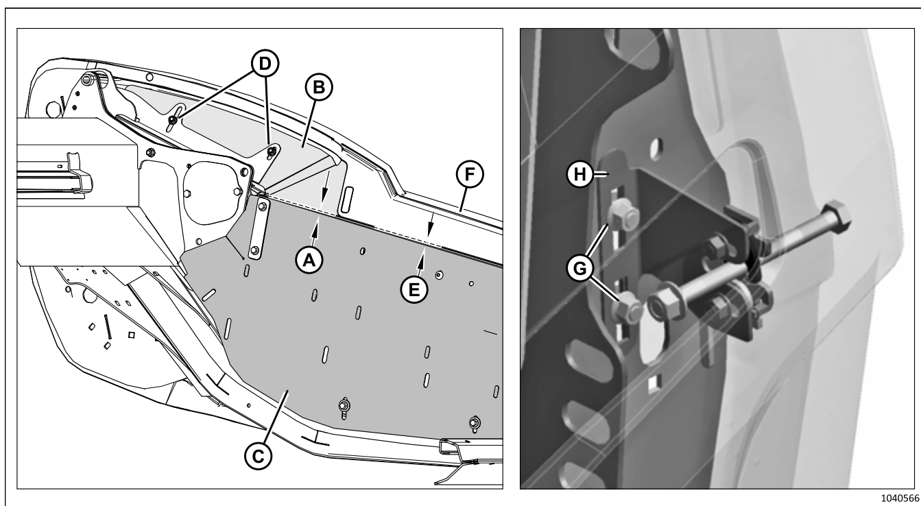
Figure 3.18: Spécification relative à l'écartement entre le blindage du cou et le panneau d'extrémité
