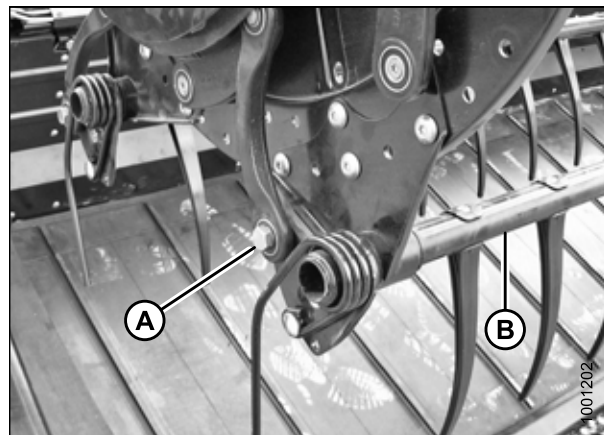
Figure 5.158: Extrémité de la came
