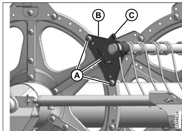
Figure 5.152: Extrémité arrière
