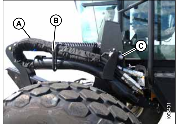
Figure 4.61: Rangement des flexibles
