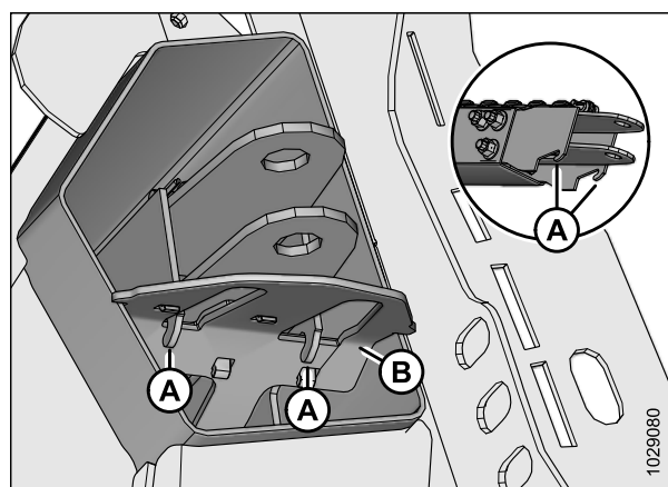
Figure 3.107: Crochets de retenue de l'extrémité de la chape
