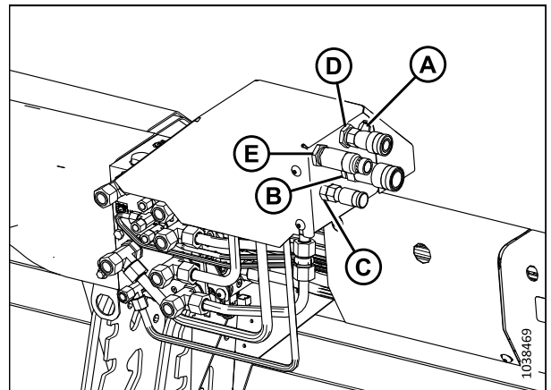
Figure 4.52: Connecteurs d'accouplement de la plateforme
