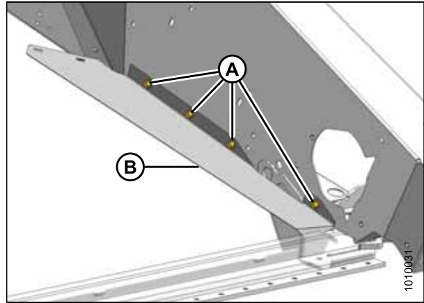
Figure 5.132: Déflecteur avant
