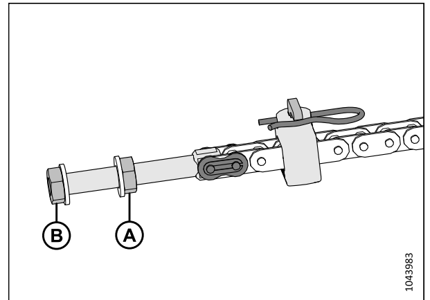
Figure 3.88: Boulon de réglage de la chaîne gauche – côté droit identique
