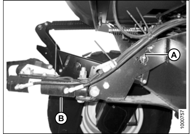
Figure 4.24: Vérin d'inclinaison hydraulique sans kit d'alignement automatique
