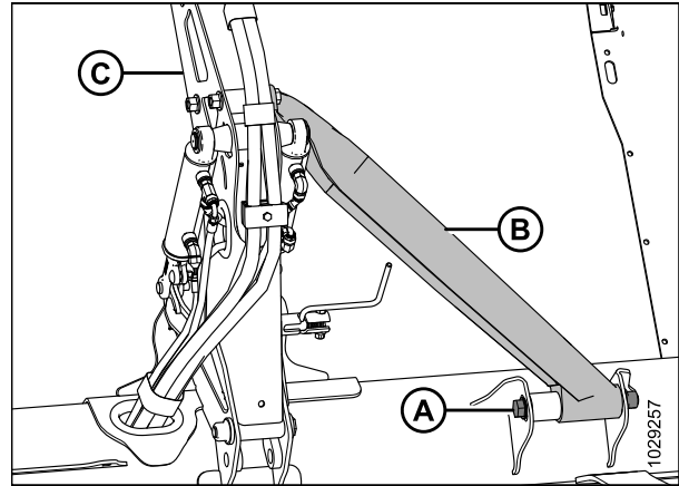
Figure 5.145: Bras de support central du rabatteur double
