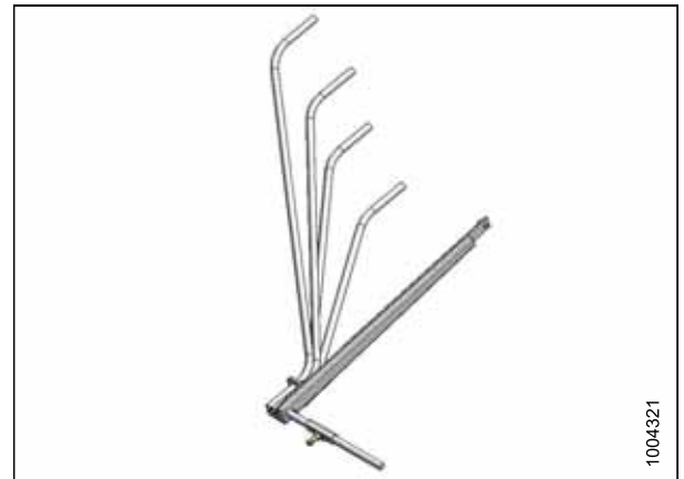
Figure 6.8: Tiges de formage d'andains
