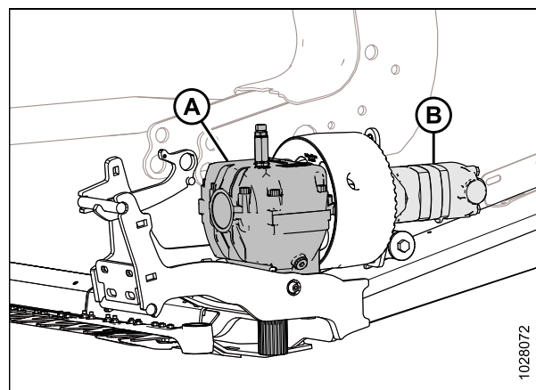
Figure 5.84: Illustration du boîtier d'entraînement de couteaux côté gauche – similaire du côté droit
