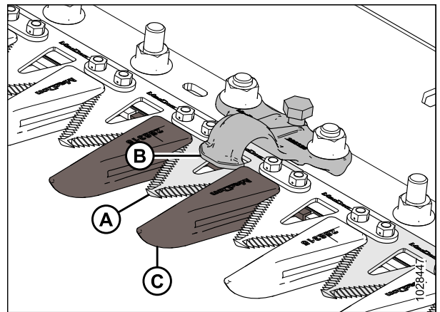
Figure 5.55: Rabatteurs des doigts pointus
