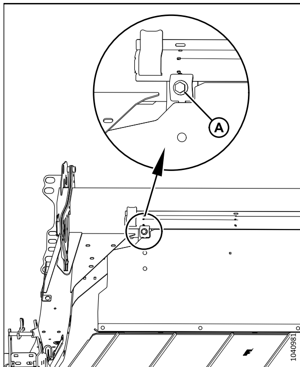
Figure 3.91: Tablier de droite représenté
