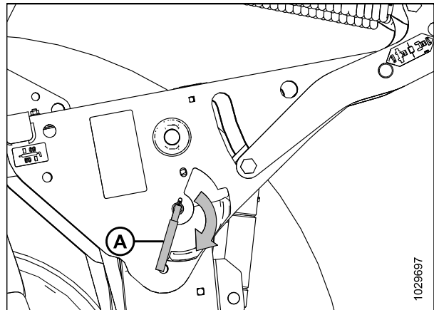
Figure 4.18: Support de sécurité du levier
