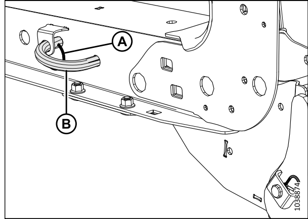
Figure 4.96: Étançon de la plateforme
