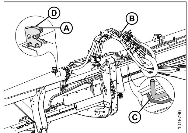
Figure 4.100: Système de gestion des tuyaux hydrauliques – Toutes les plateformes sauf D215
