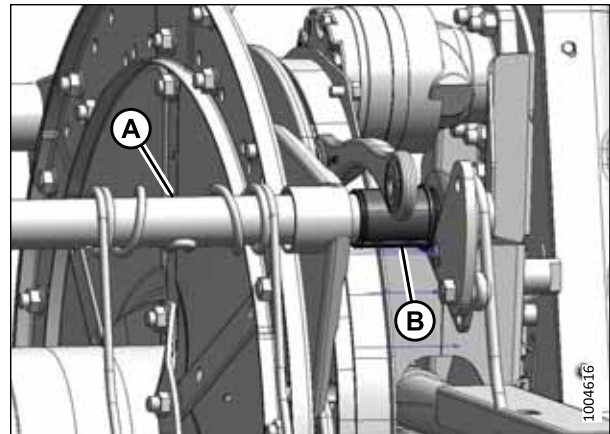
Figure 5.167: Extrémité de la came
