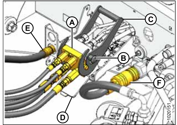
Figure 4.104: Multicoupleur du tapis/rabatteur
