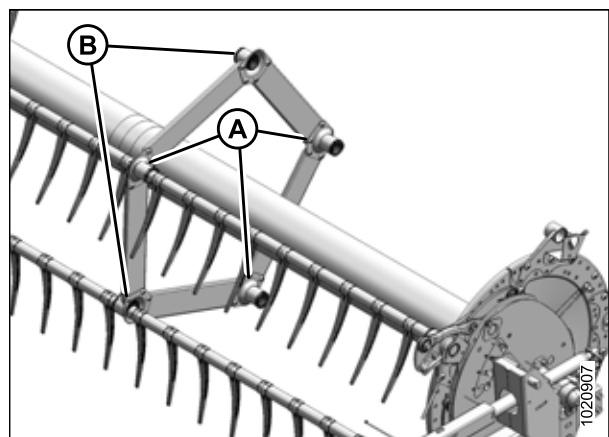
Figure 5.157: Supports du tube à doigts
