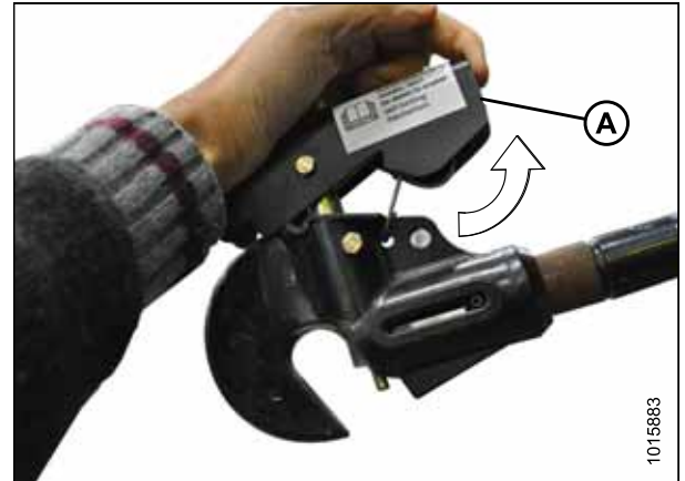
Figure 4.154: Vérin d'inclinaison
