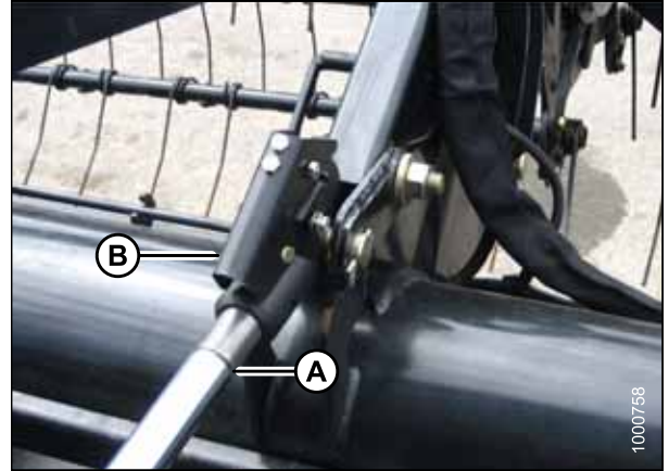
Figure 4.71: Vérin d'inclinaison hydraulique
