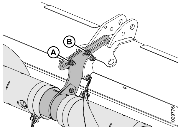
Figure 3.69: Position initiale des supports réglables - Vis en deux parties
