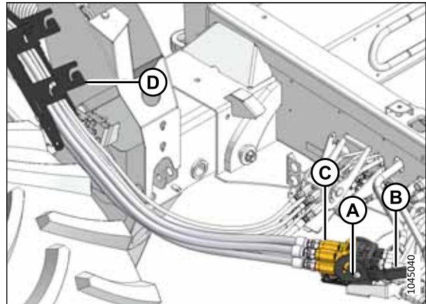
Figure 4.161: Multicoupleur de l'entraînement de couteau/rabatteur
