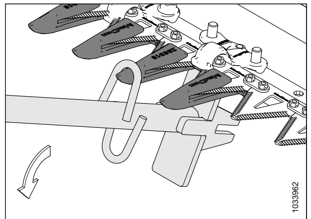
Figure 5.48: Réglage vers le bas - Doigt pointu
