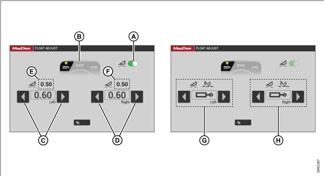
Figure 4.138: Réglage du flottement
