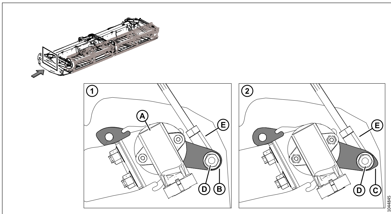
Figure 3.42: Emplacement du capteur de hauteur du rabatteur
