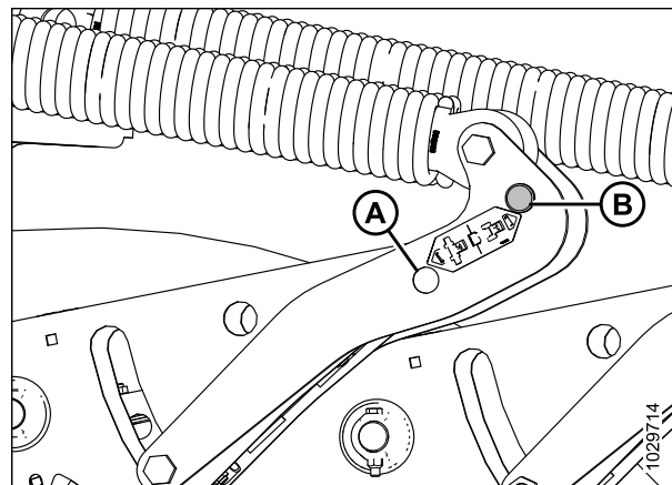
Figure 4.1: Articulation de flottement de la plateforme – série M
