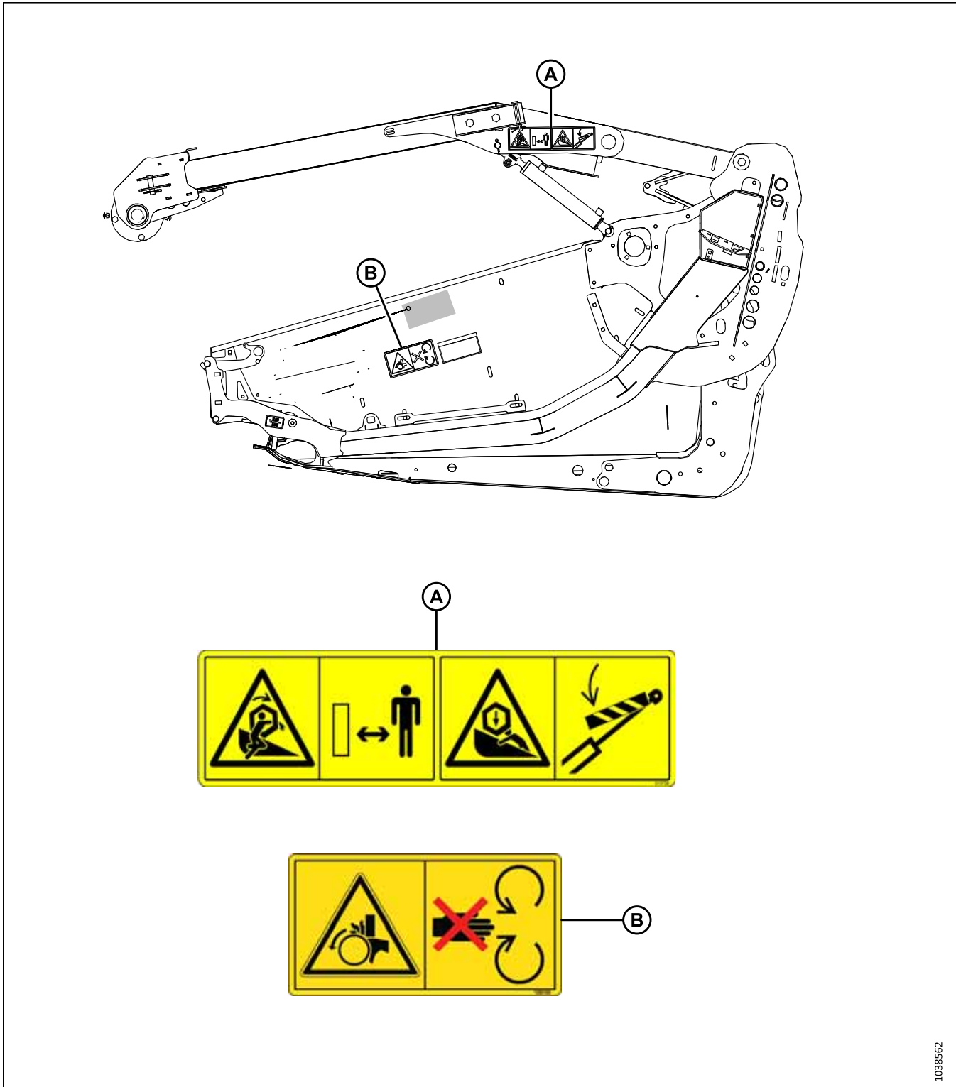
Figure 1.21: Tôles d'extrémité et bras de rabatteur
