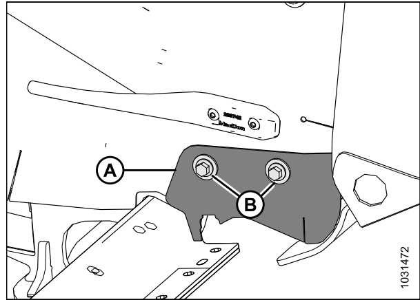
Figure 5.83: Blindage de la tête de couteau
