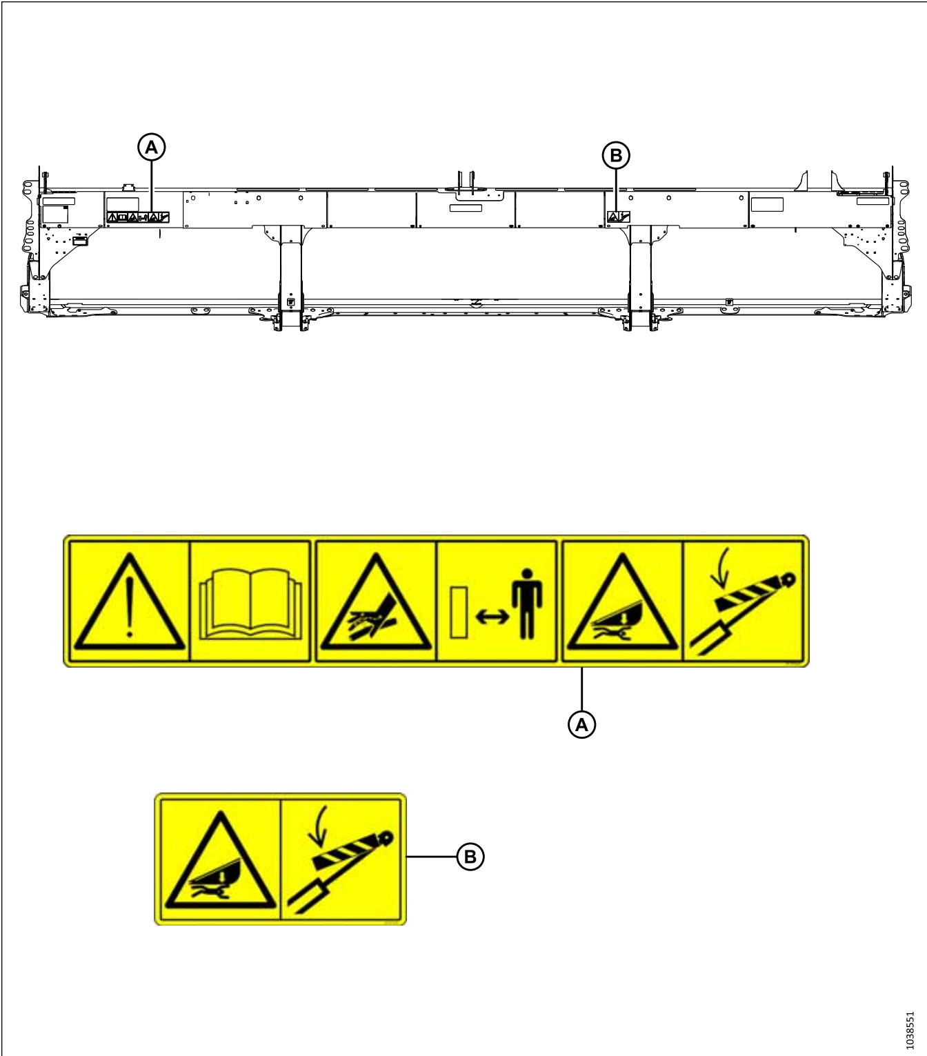
Figure 1.23: Tube arrière – Plateforme de coupe à tapis D220
