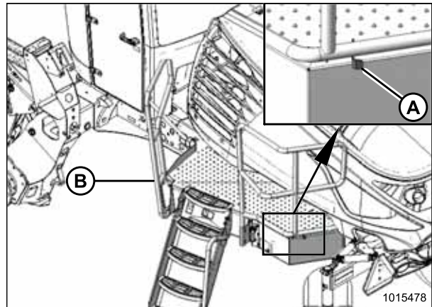
Figure 4.113: Plateforme de gauche
