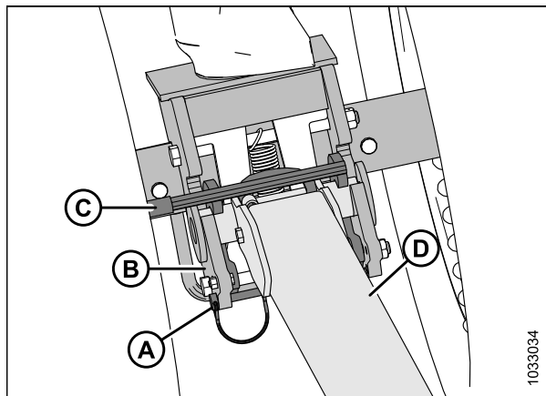
Figure 3.99: Extension de la barre de remorquage et du pivot de transport
