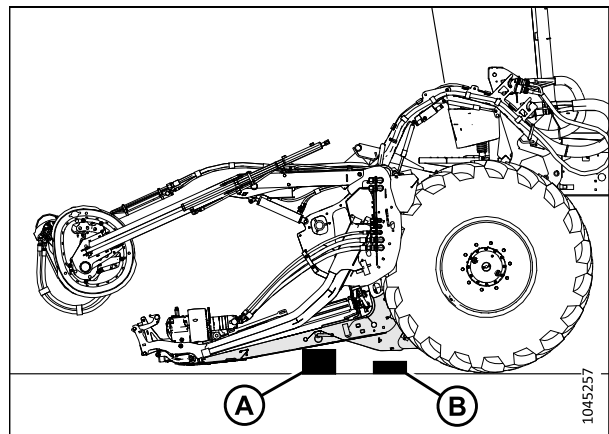
Figure 4.64: Réglage de la plateforme au sol
