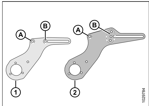
Figure 3.68: Détails du montage ajustable
