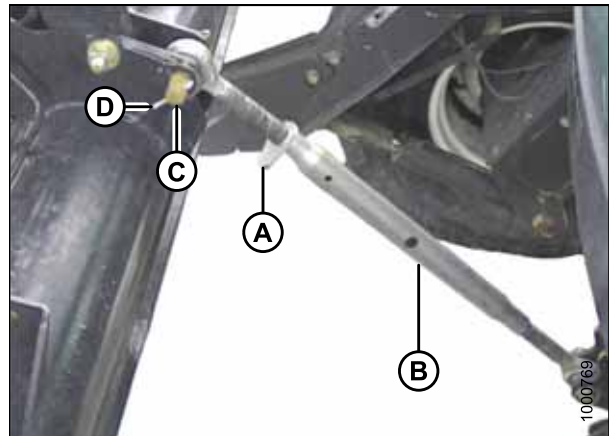
Figure 4.79: Vérin d'inclinaison mécanique
