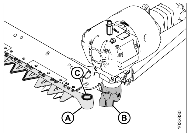
Figure 5.34: Tête de couteau gauche
