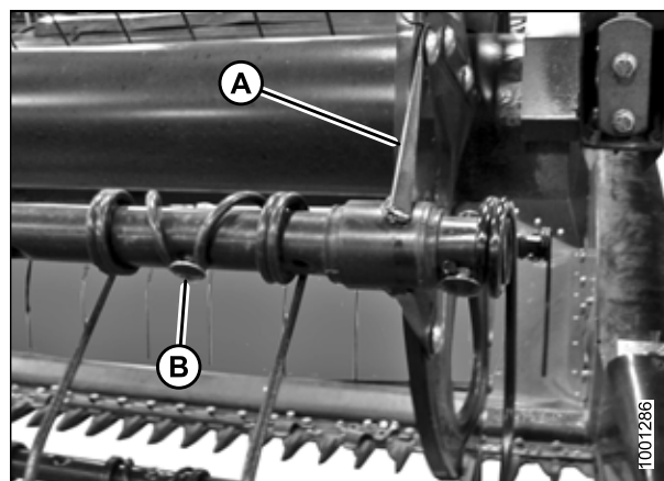
Figure 5.147: Tube à doigts
