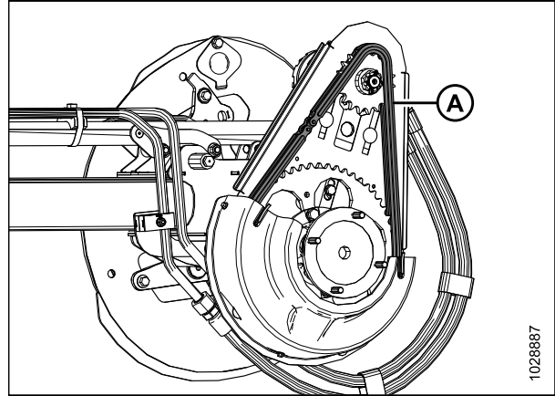
Figure 5.17: Chaîne d'entraînement – Entraînement de rabatteur double illustré
