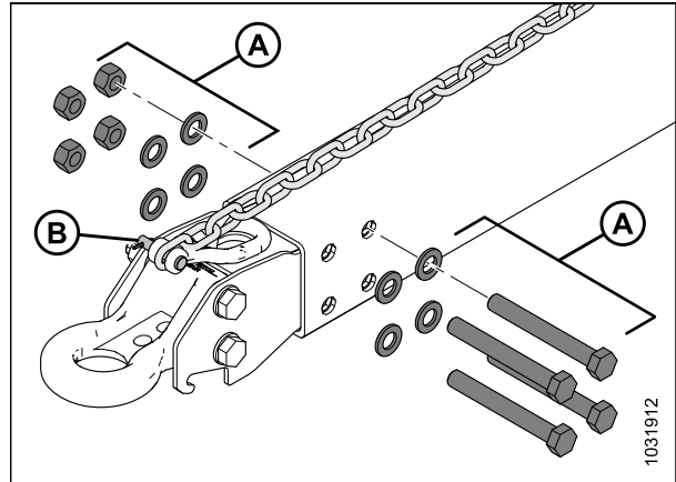
Figure 5.234: Installation de l'adaptateur pour anneau d'attelage
