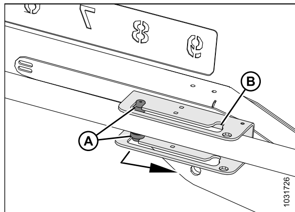
Figure 3.54: Réglage des vérins avant-arrière de type 2 – Position avant
