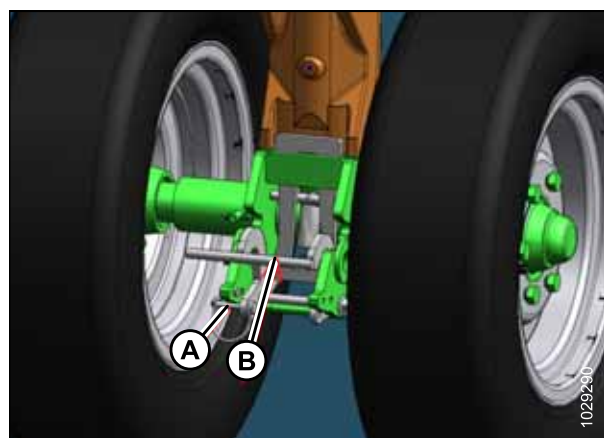
Figure 3.120: Roues de transport avant
