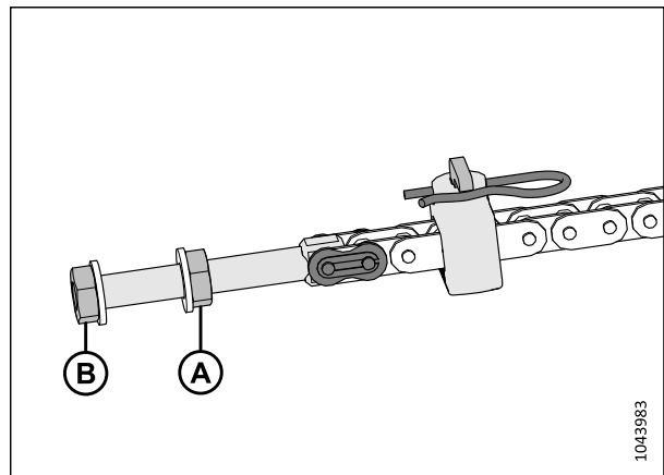
Figure 3.86: Boulon de réglage de la chaîne gauche – côté droit identique
