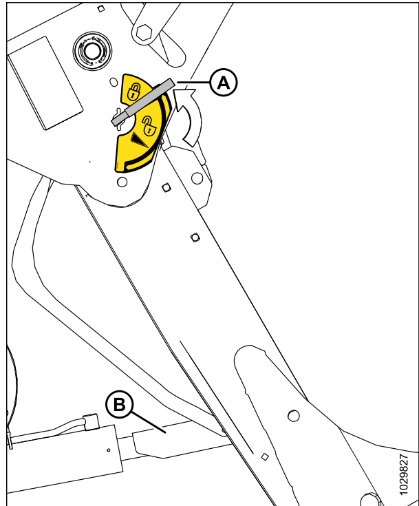
Figure 4.44: Support de sécurité
