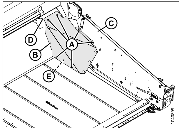
Figure 5.125: Déflecteur arrière large – Côté gauche illustré
