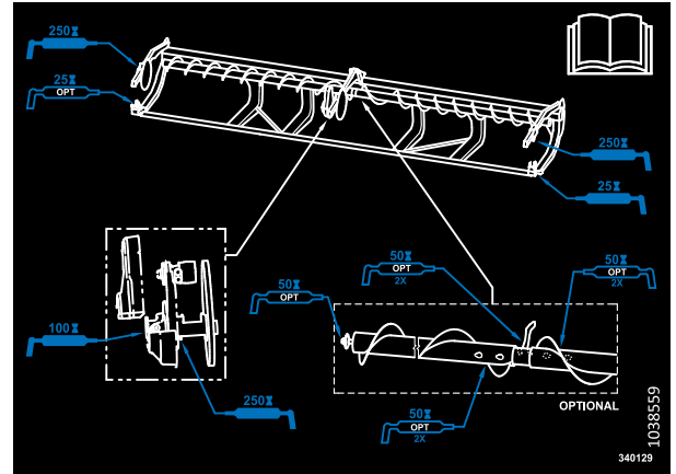
Figure 5.16: Autocollant pour les plateformes à couteau double avec vis transversale supérieure à deux pièces
