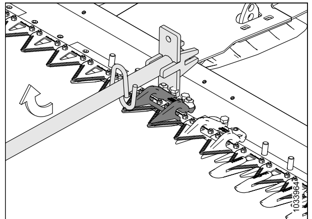
Figure 5.47: Réglage vers le haut – Doigt court
