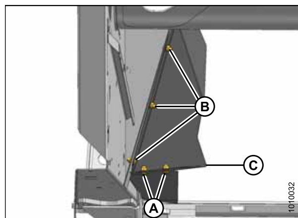
Figure 5.131: Déflecteur arrière
