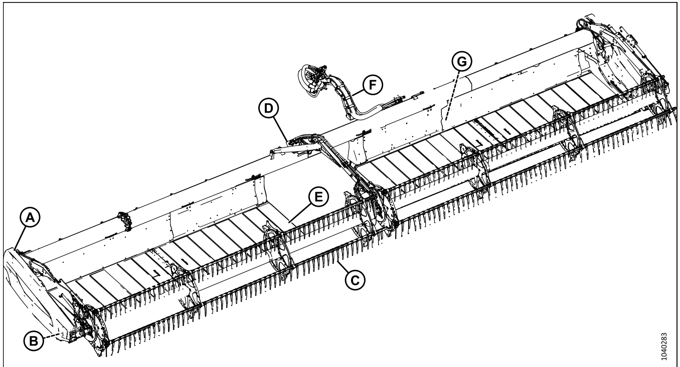
Figure 2.2: Plateforme de coupe à tapis de série D2 – rabatteur double illustré
