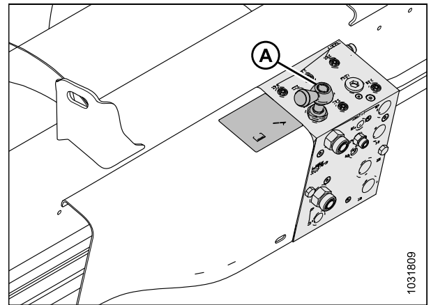
Figure 3.66: Vanne d'arrêt
