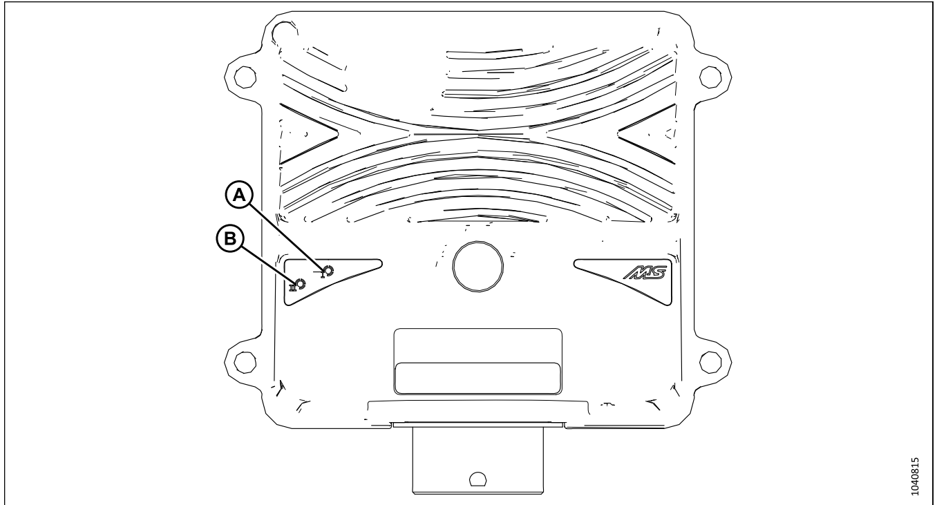
Figure 5.28: Module de réglage électronique de la synchronisation des couteaux doubles (ETDK)
