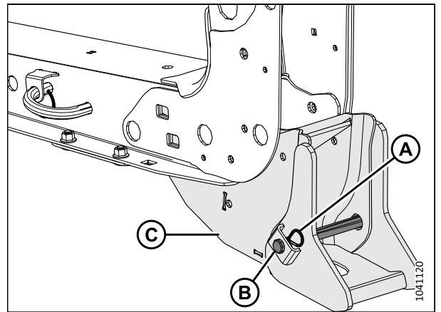
Figure 4.83: Support de la plateforme de coupe – Côté gauche illustré
