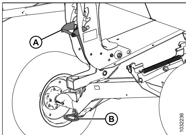
Figure 3.122: Roues de jauge
