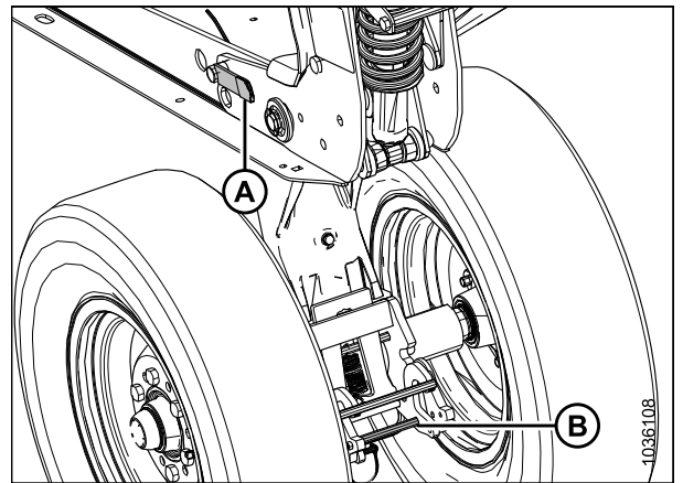
Figure 3.111: Roues de transport gauches – Pivot dégagé
