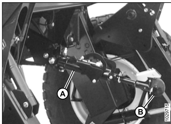
Figure 4.28: Vérin d'inclinaison hydraulique
