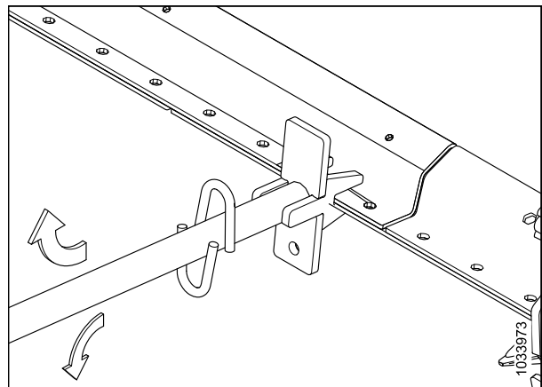
Figure 5.50: Ajustement des barres de protection - Pas de protection
