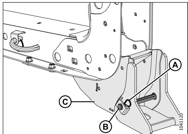
Figure 4.168: Chandelle de la plateforme
