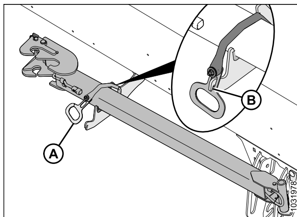
Figure 3.105: Stockage de l'extension de la barre de remorquage
