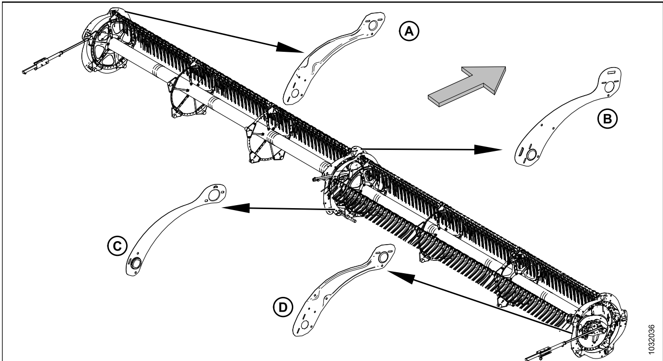
Figure 5.184: Blindages du rabatteur
