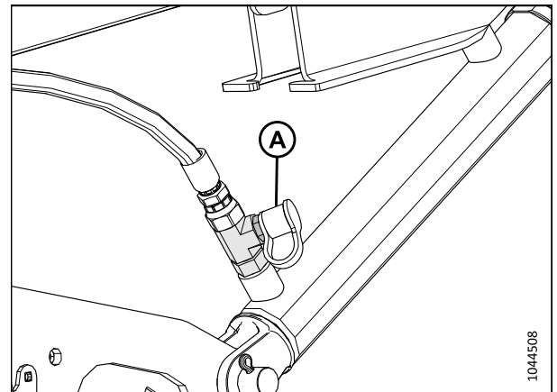
Figure 5.141: Déclencheur pneumatique de levage du rabatteur pneumatique
