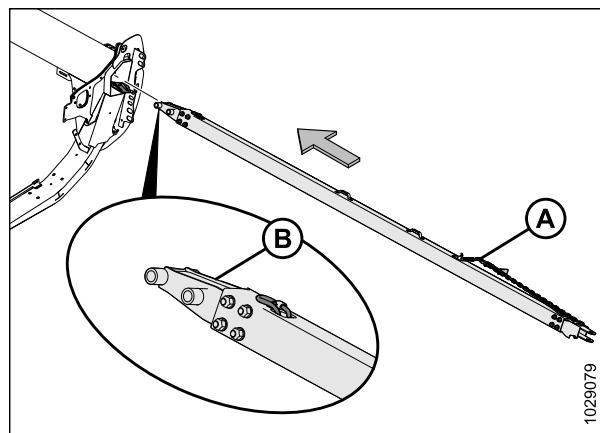
Figure 3.106: Extrémité de l'attelage
