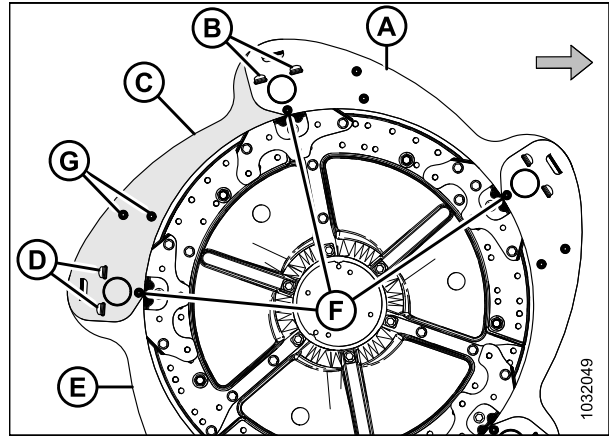
Figure 5.192: Boucliers des rabatteurs - Extrémité de came intérieure
