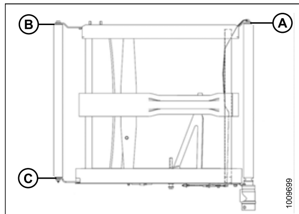
Figure 5.101: Bras de rouleaux
