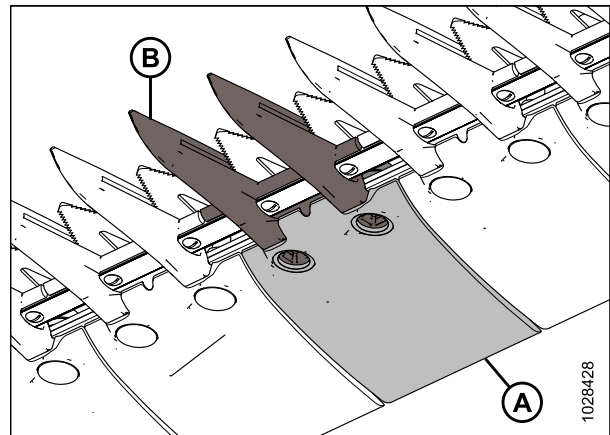
Figure 5.53: Doigts de couteau pointus et plaque d'usure
