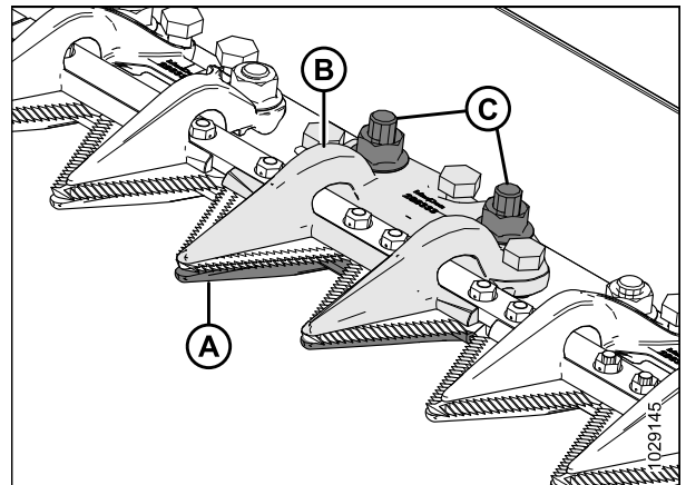
Figure 5.75: Doigt de couteau central
