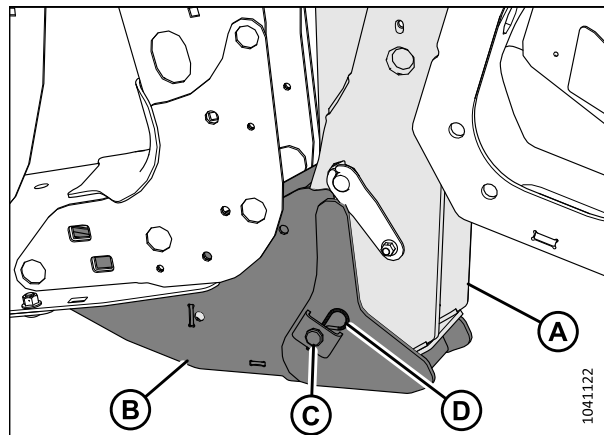
Figure 4.65: Patte de la plateforme et articulation de levage de l'andaineuse reliées par le support de la plateforme
