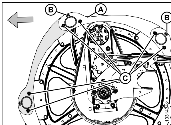
Figure 5.202: Boucliers des rabatteurs - Extrémité arrière intérieure
