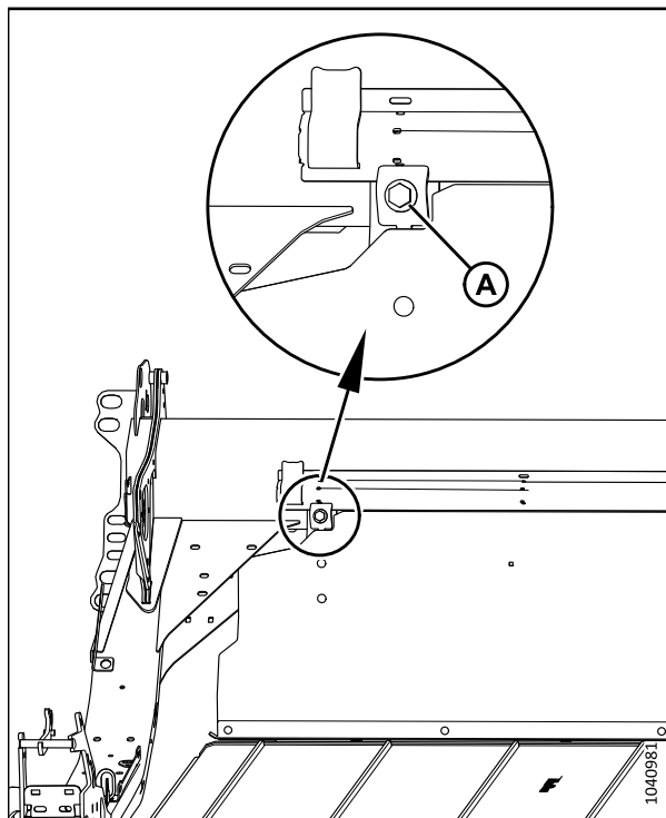
Figure 3.89: Décalage manuel du tablier
