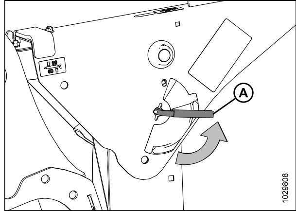
Figure 4.151: Levier du support de sécurité
