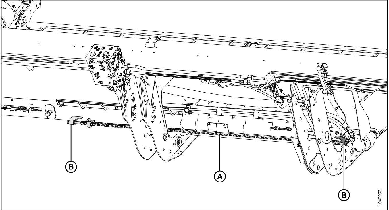
Figure 3.87: Chaîne de décalage hydraulique du tablier – Côté gauche représenté, côté droit similaire
