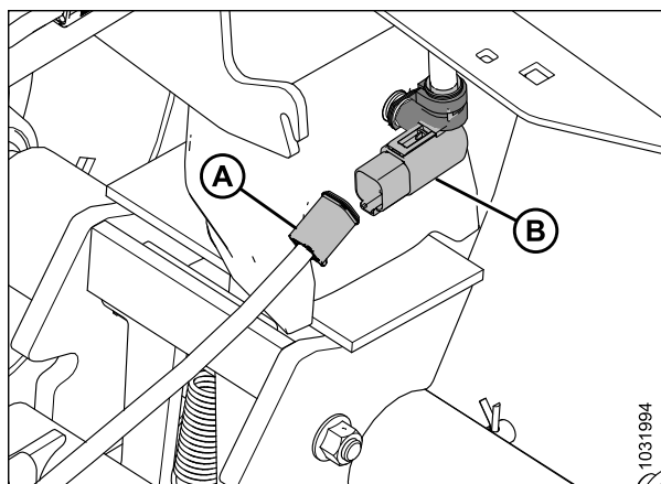
Figure 3.101: Connexion électrique de la barre de remorquage
