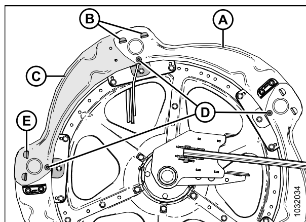
Figure 5.196: Boucliers des rabatteurs - Extrémité arrière extérieure
