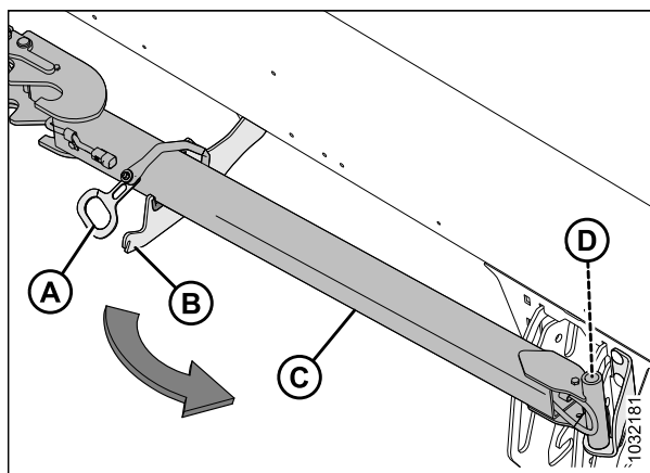
Figure 3.127: Stockage de l'extension de la barre de remorquage
