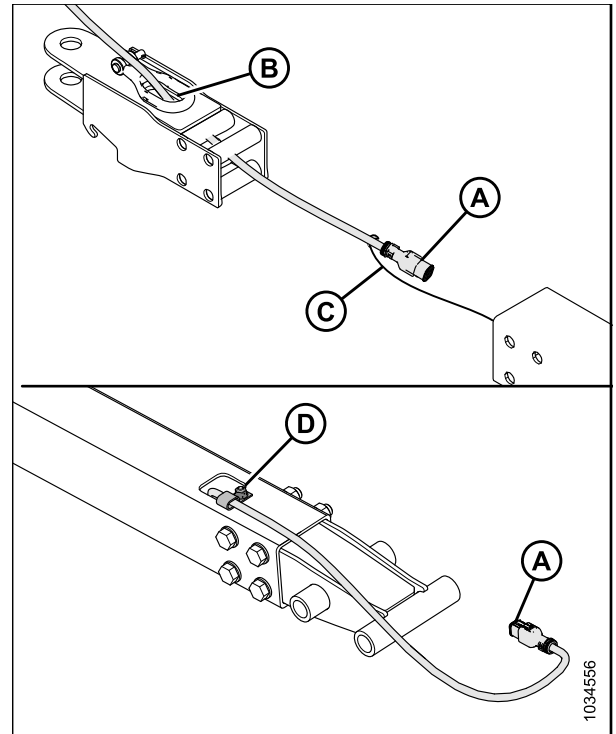
Figure 5.228: Installation de l'adaptateur d'anneau de chape
