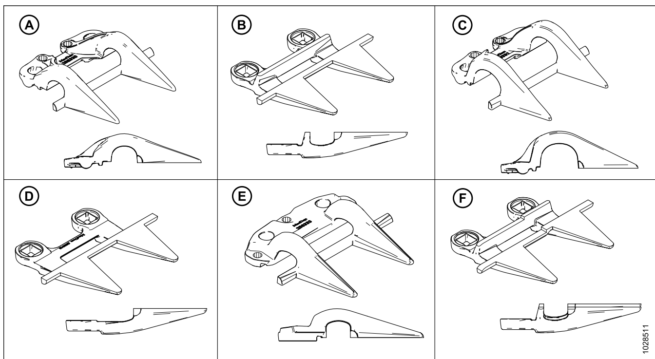
Figure 5.65: Types de doigts et de retenue utilisés dans les configurations de doigts de couteau court
