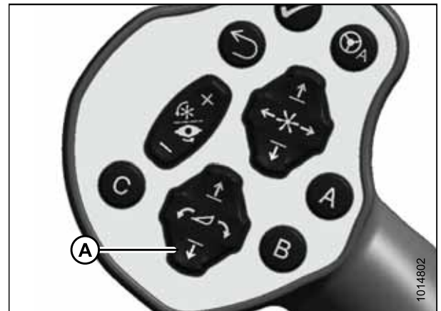
Figure 4.137: Levier de vitesse au sol (LVS)
