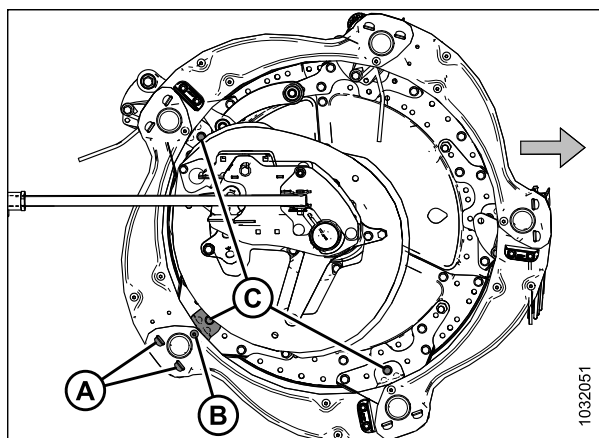
Figure 5.203: Supports des blindages du rabatteur
