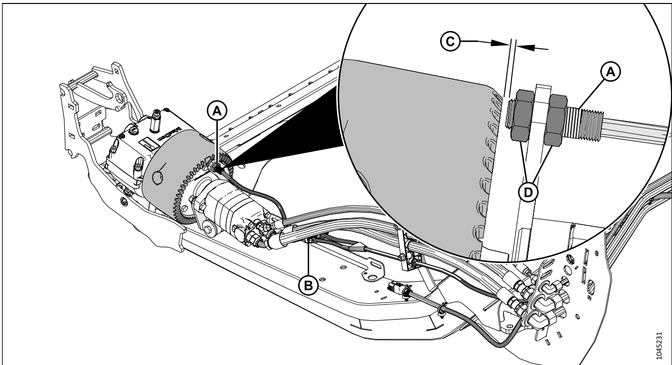
Figure 5.20: Capteur de vitesse gauche – position pour les modèles de série M1/M2
