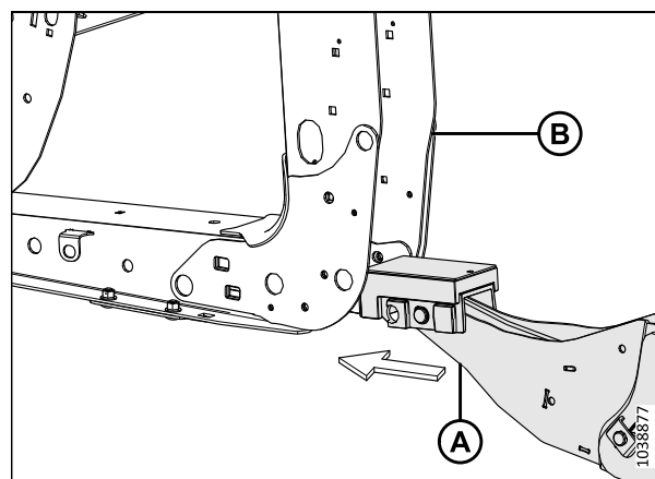
Figure 4.90: Étauçon de la plateforme et support
