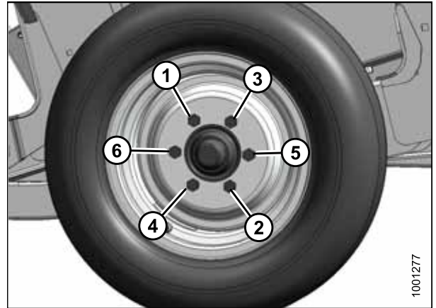
Figure 5.223: Séquence de serrage des boulons
