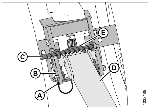
Figure 3.130: Extension de la barre de remorquage au pivot de transport gauche
