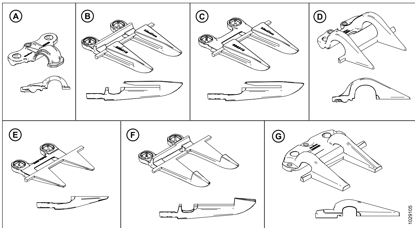
Figure 5.42: Types de protection et de rabatteur utilisés dans les configurations de doigts de lamier pointu
