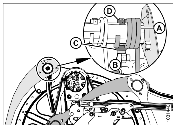
Figure 5.201: Boucliers des rabatteurs - Extrémité arrière intérieure
