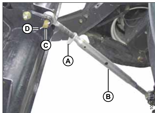
Figure 4.42: Vérin d'inclinaison mécanique
