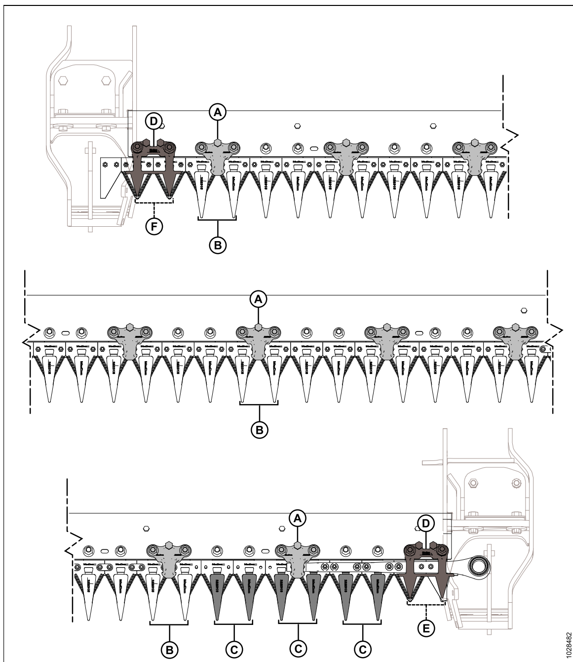
Figure 5.43: Emplacement des doigts et mécanismes de retenue – Plateformes à couteau unique
