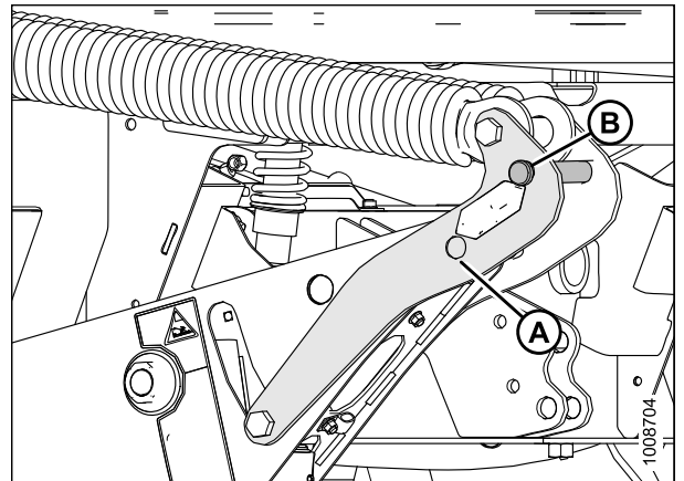
Figure 4.76: Articulation de flottement de la plateforme
