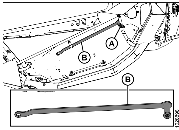
Figure 3.64: Plateau d'extrémité gauche
