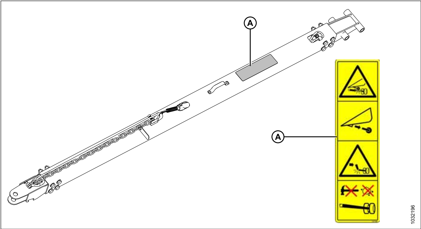
Figure 1.30: Système de transport EasyMove MC – Barre de remorquage (courte barre représentée, longue barre similaire) (en option)
