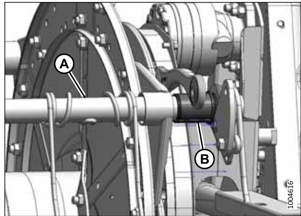
Figure 5.173: Extrémité de la came
