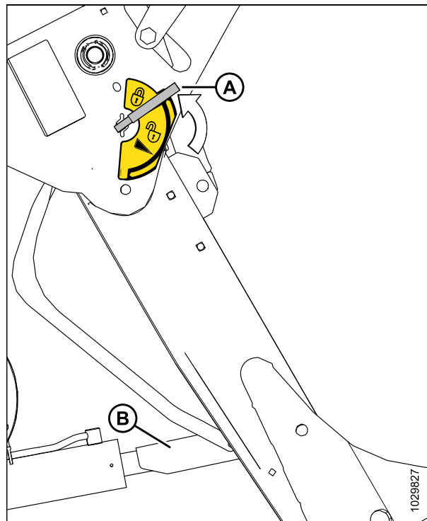
Figure 4.14: Support de sécurité
