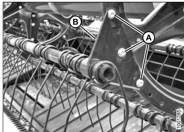
Figure 5.146: Bras du tube à doigts
