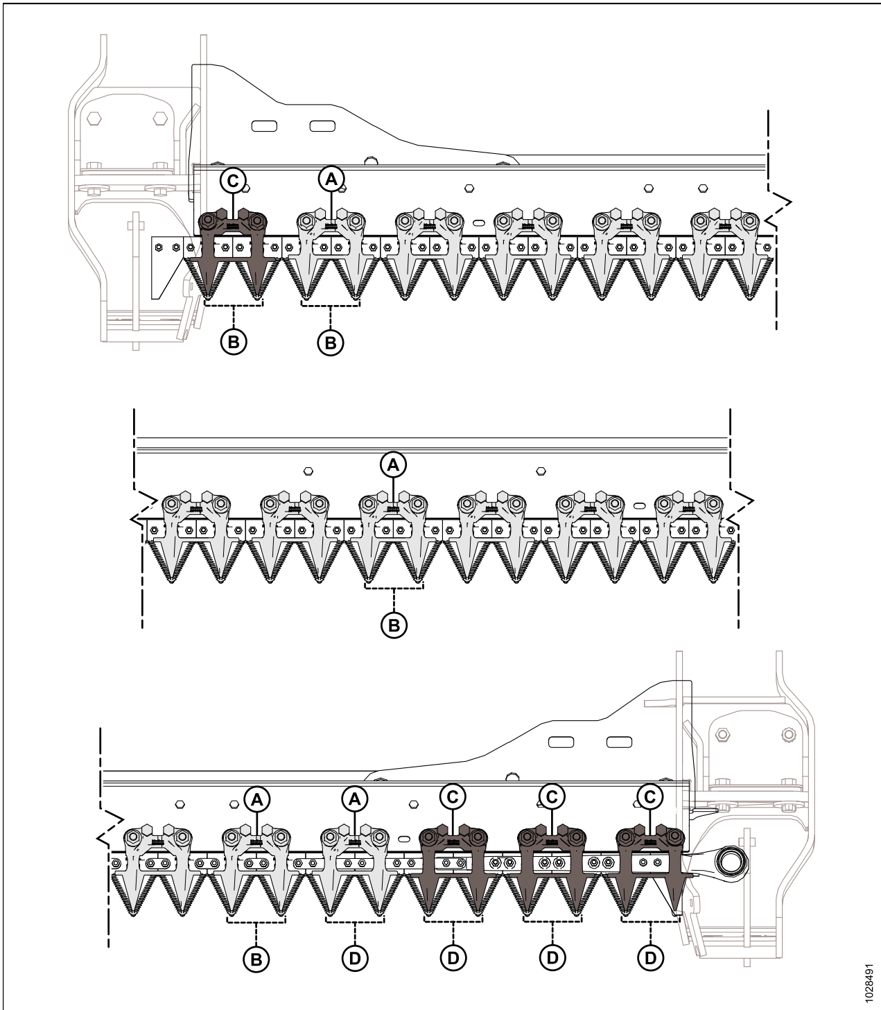
Figure 5.66: Emplacement des doigts de couteau court et rabatteurs – Plateformes à couteau unique
