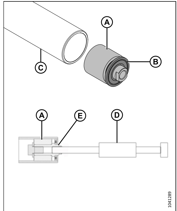
Figure 5.105: Roulement du rouleau libre et joint
