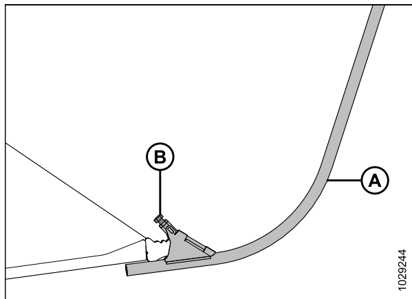
Figure 3.78: Tige de division de récolte
