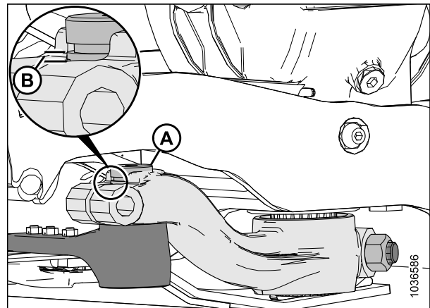
Figure 5.38: Tête de couteau
