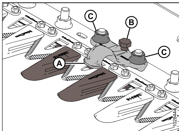
Figure 5.56: Rabatteurs pointus
