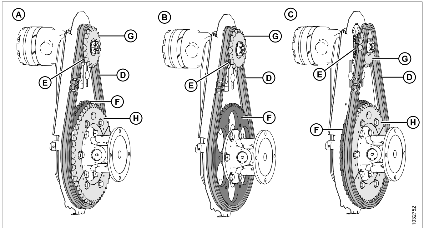
Figure 5.219: Configurations du rabatteur – Pignons doubles optionnels
