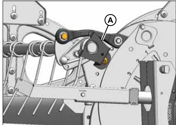
Figure 5.155: Extrémité de la came
