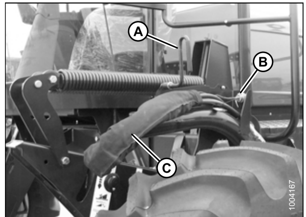
Figure 4.51: Flexibles d'entraînement de la plateforme
