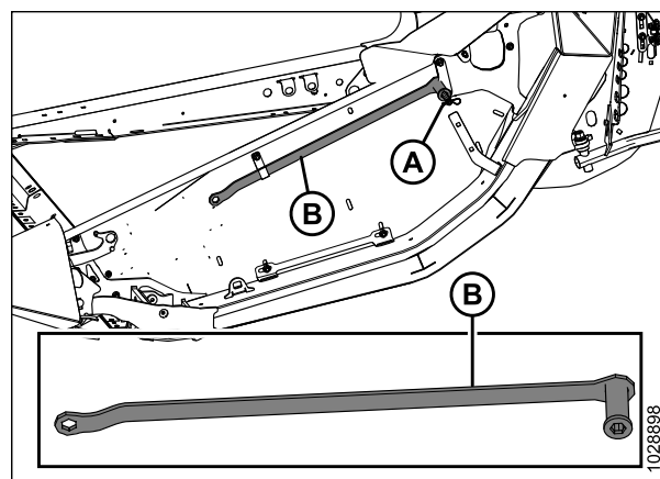
Figure 5.208: Emplacement de rangement de l'outil polyvalent – Côté gauche
