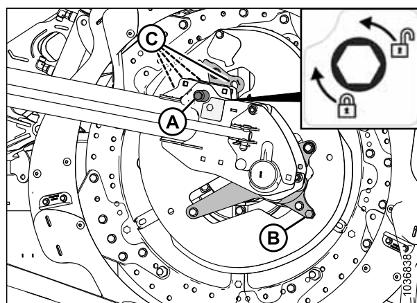
Figure 3.65: Positions du disque à came
