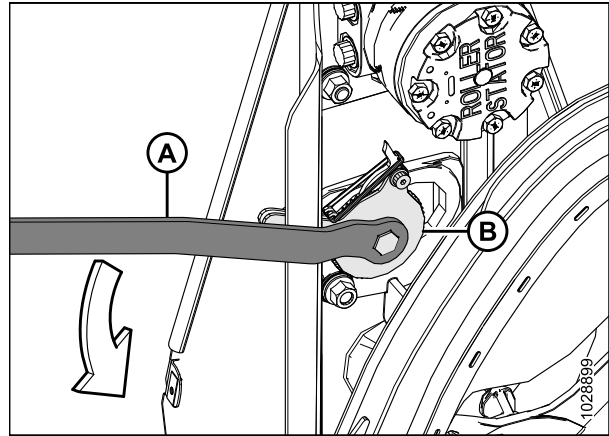
Figure 5.209: Entraînement du rabatteur
