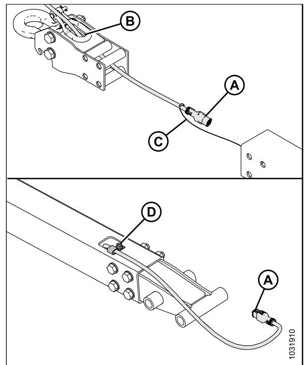
Figure 5.233: Installation de l'adaptateur pour anneau d'attelage
