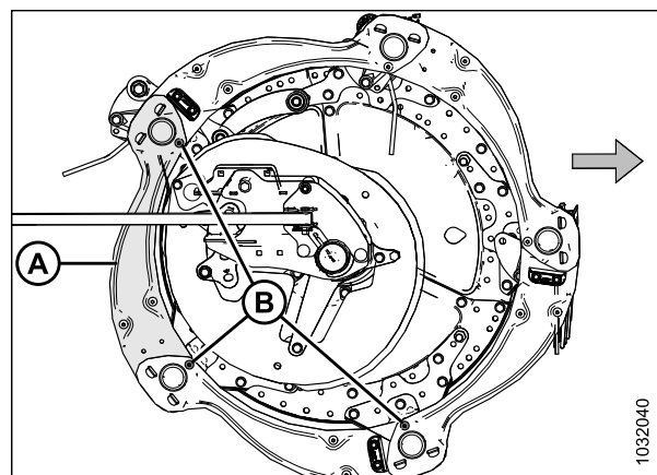
Figure 5.185: Boucliers des rabatteurs - Extrémité de came extérieure
