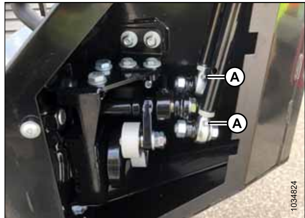
Figure 5.241: Graissage des embouts sur les tiges-poussoirs des couteaux verticaux
