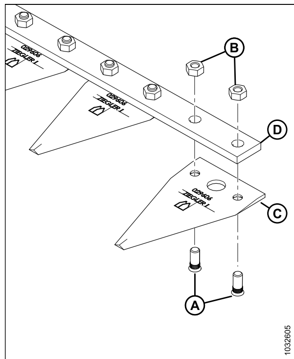
Figure 5.239: Assemblage de la section de couteau
