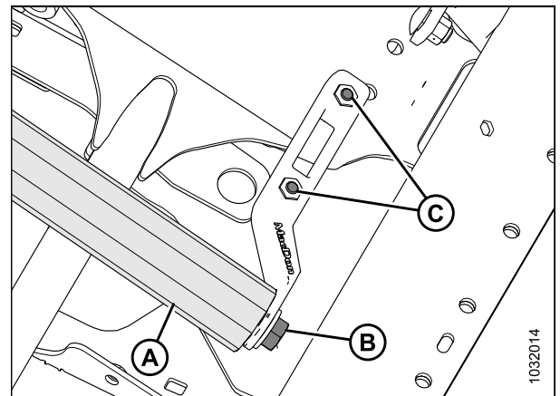
Figure 5.120: Rouleau d'entraînement
