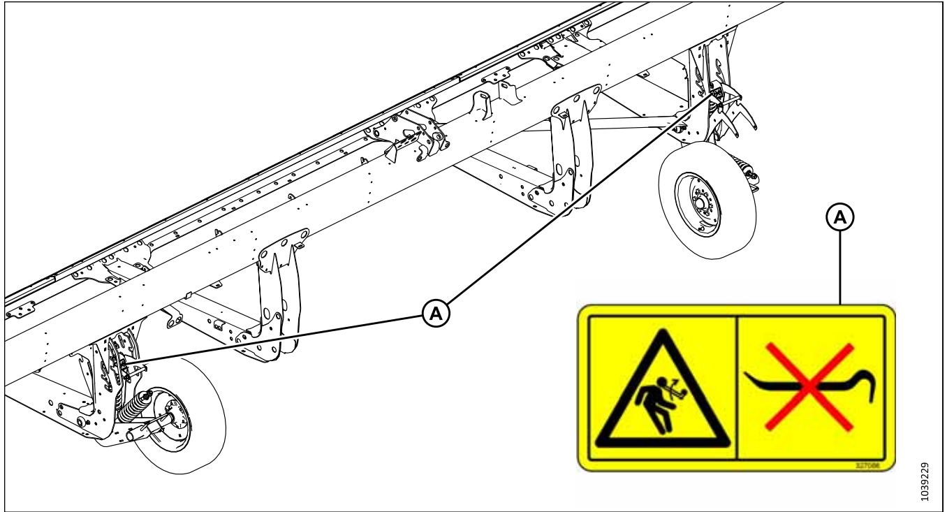
Figure 1.32: Roues stabilisatrices (en option)
