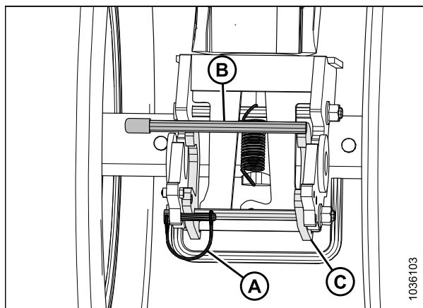
Figure 3.109: Roues de transport gauches – Loquet de verrouillage de rotation désengagé
