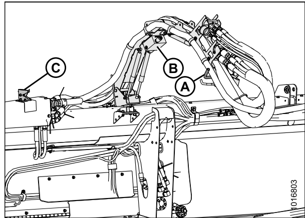
Figure 4.102: Système de gestion des flexibles hydrauliques
