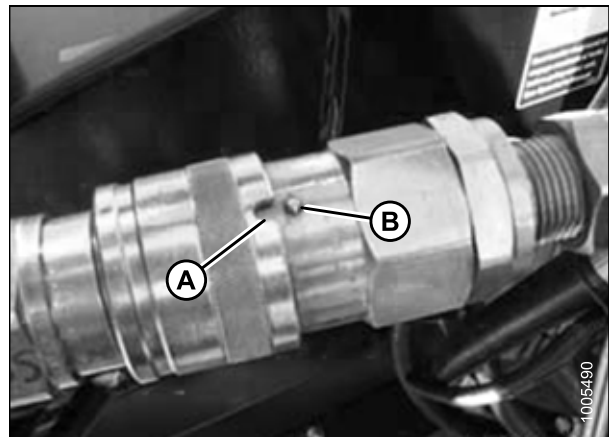
Figure 4.60: Déconnexion des connecteurs rapides
