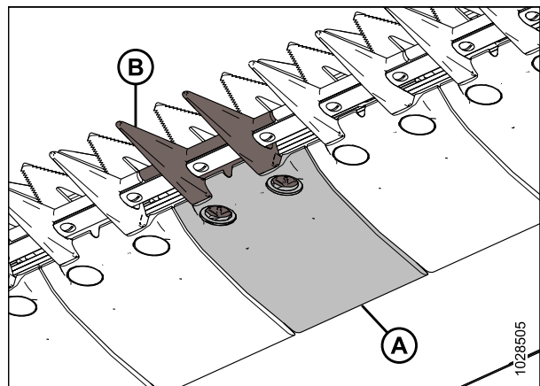
Figure 5.78: Doigt du couteau central et plaque d'usure
