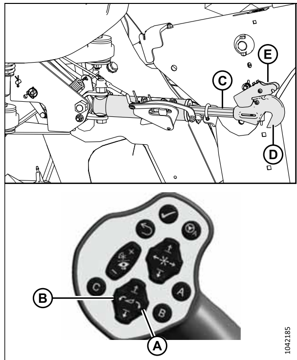
Figure 4.132: Vérin d'inclinaison hydraulique
