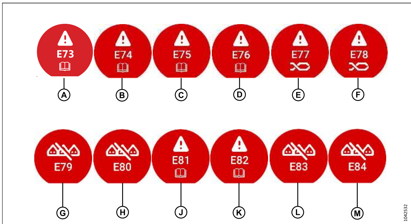
Figure 5.22: Symbole des codes de défaut – Écran TE
