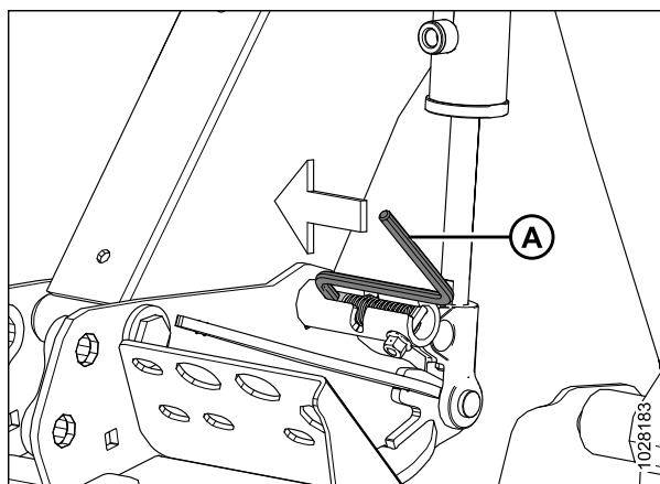
Figure 3.4: Support de sécurité du rabatteur enclenché – Bras central
