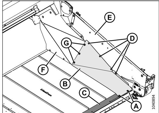
Figure 5.124: Déflecteur large – Côté gauche illustré
