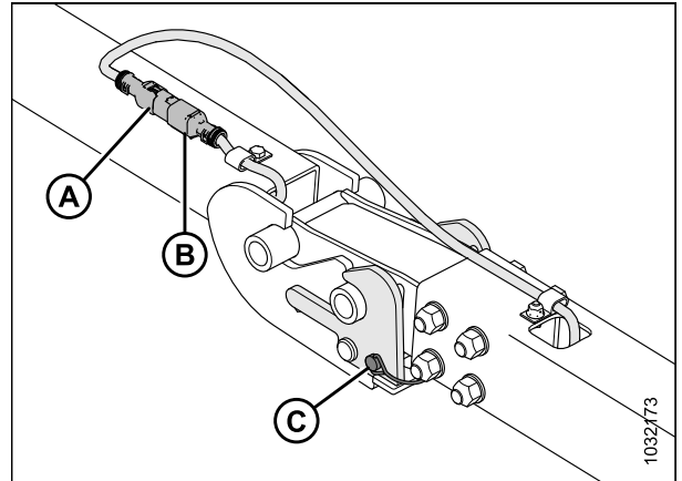
Figure 3.133: Barre de remorquage/Rallonge de harnais
