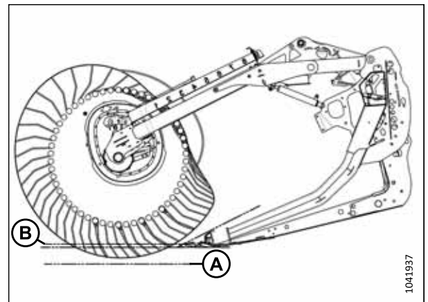
Figure 3.63: Profil des doigts – Came en position 4, angle de la plateforme au maximum
