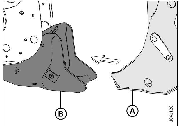
Figure 4.9: Étançon de la plateforme et support
