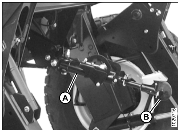
Figure 4.12: Vérin d'inclinaison hydraulique
