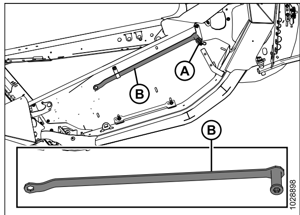
Figure 5.206: Emplacement de rangement de l'outil polyvalent
