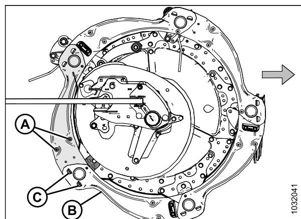
Figure 5.186: Boucliers des rabatteurs - Extrémité de came extérieure
