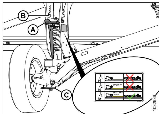
Figure 3.34: Roue droite
