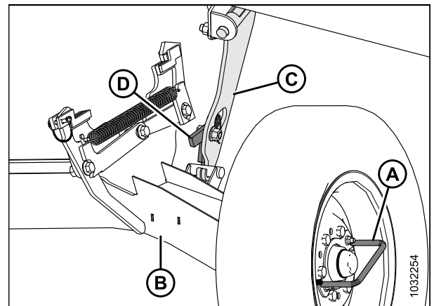
Figure 3.116: Essieu de transport droit verrouillé dans la position de travail
