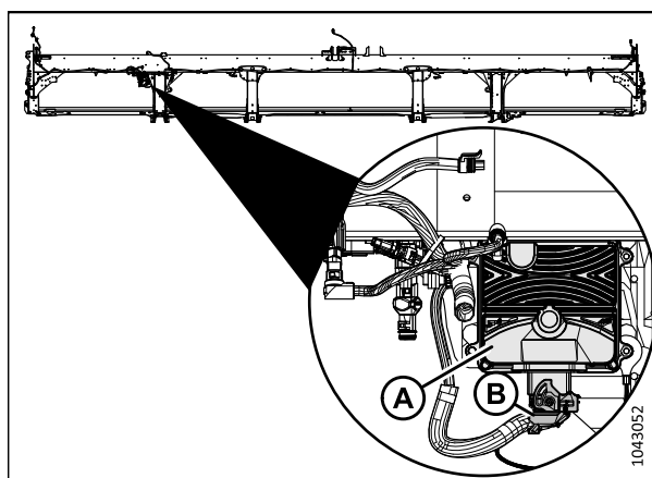
Figure 1.16: Module de commande du ETDK
