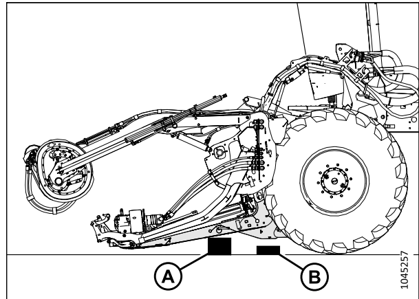
Figure 4.152: Réglage de la plateforme au sol
