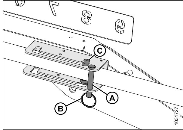
Figure 3.55: Réglage des vérins avant-arrière de type 2 – Position arrière
