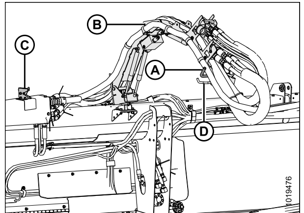
Figure 4.116: Système de gestion des flexibles hydrauliques
