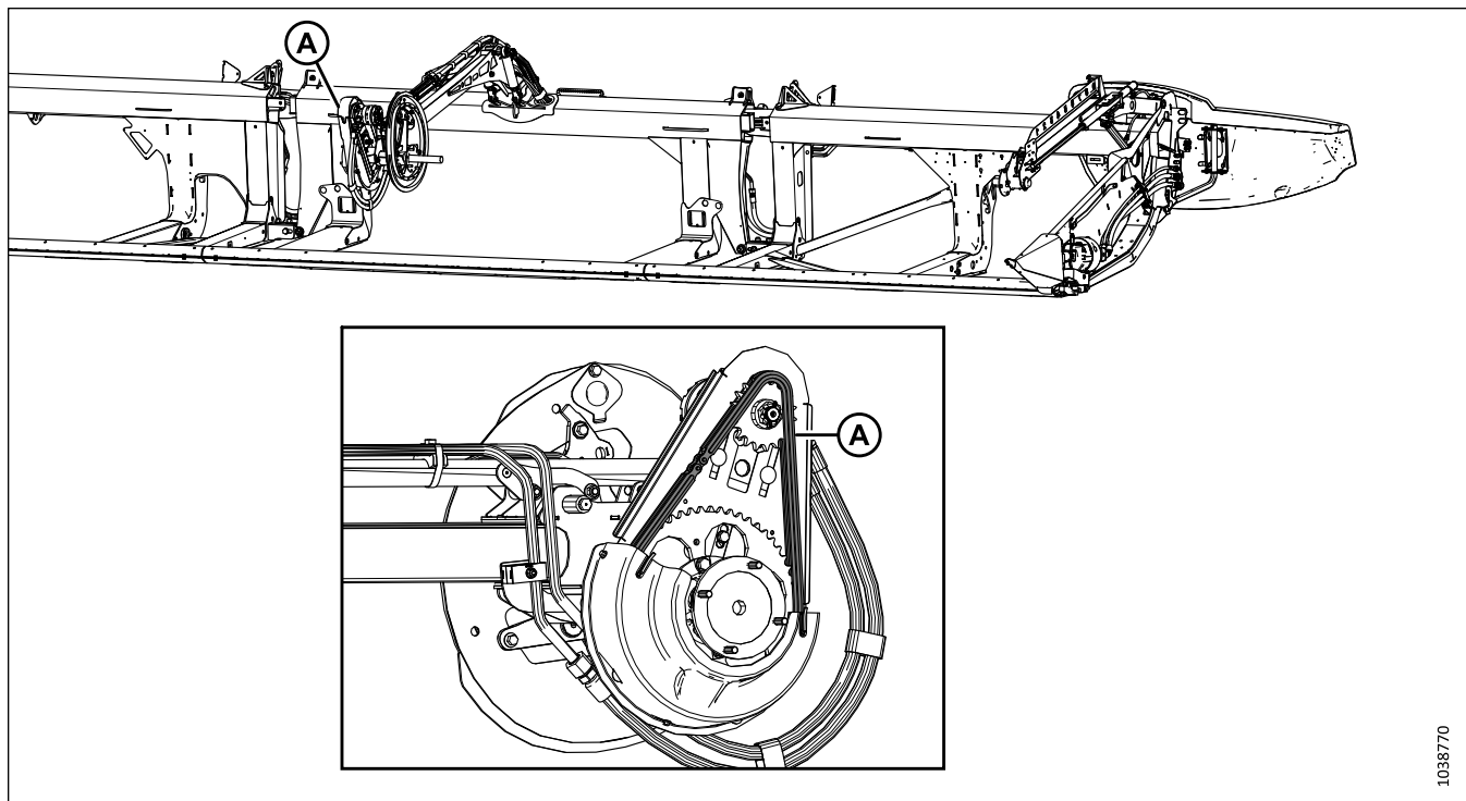
Figure 5.7: Rabatteur
