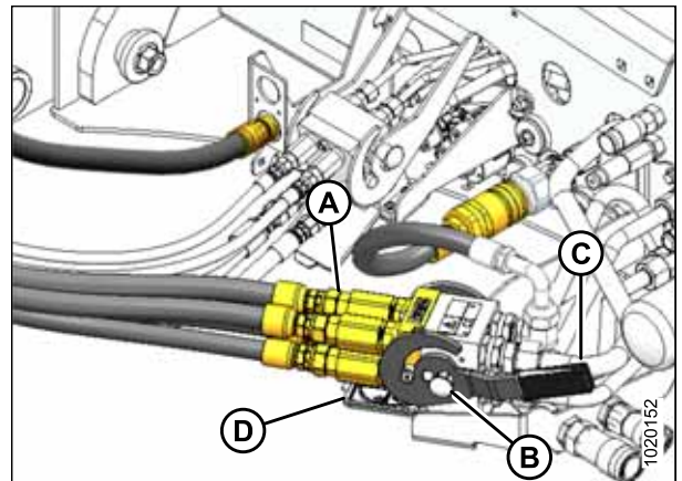
Figure 4.105: Multicoupleur de l'entraînement de couteau/rabatteur
