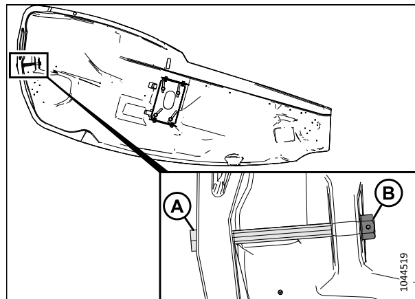
Figure 3.20: Boulon du capot du diviseur
