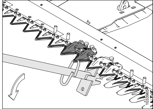
Figure 5.49: Réglage vers le bas – Doigt de lamier court
