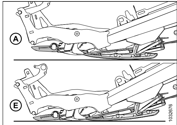
Figure 3.39: Angles de la coiffe de protection
