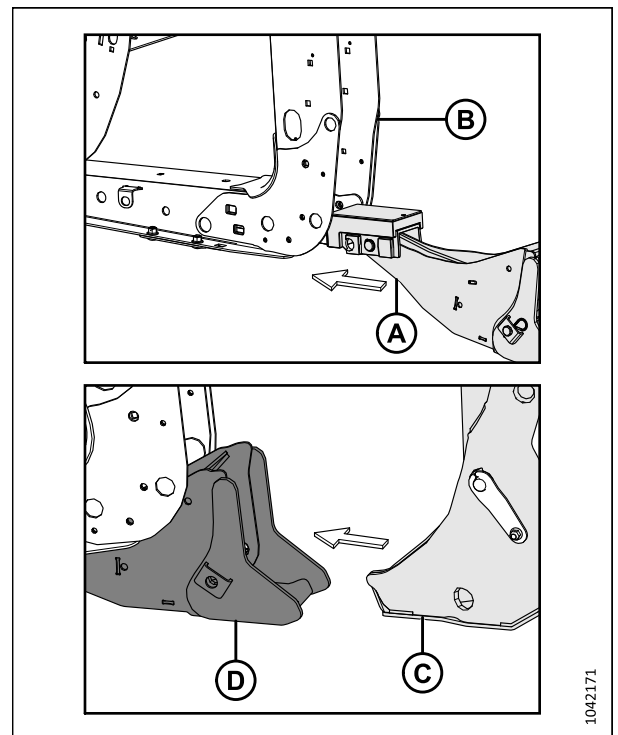
Figure 4.130: Étauçon de la plateforme et support
