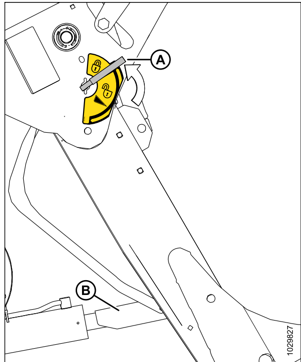
Figure 4.74: Levier du support de sécurité
