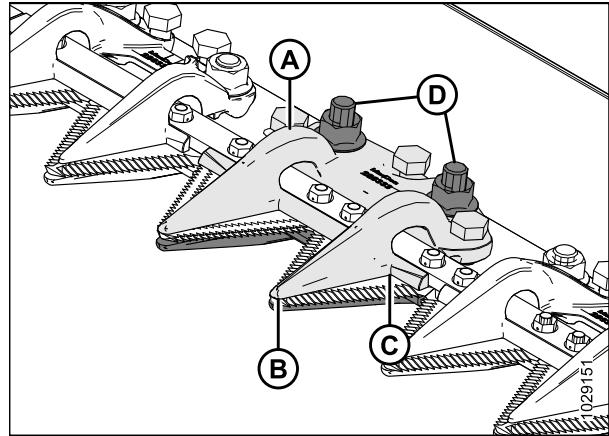
Figure 5.81: Rabatteur du doigt de couteau central
