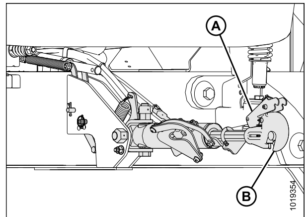
Figure 4.159: Vérin d'inclinaison hydraulique
