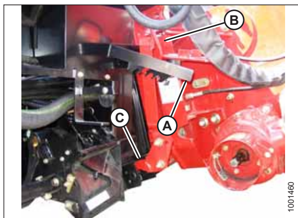
Рисунок 3.70: Блокировки наклонной камеры
