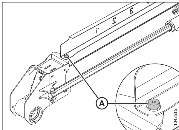
Рисунок 3.184: Индикаторный болт
