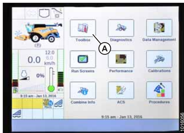
Рисунок 3.44: Приборная панель комбайнов New Holland
