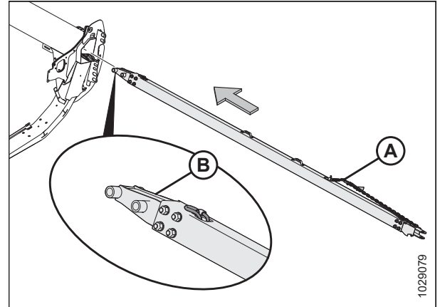
Рисунок 3.308: Сторона сцепки
