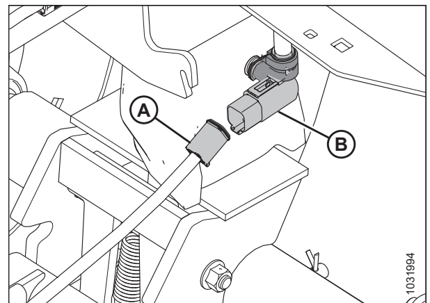
Рисунок 3.300: Электрическое соединение буксирной тяги
