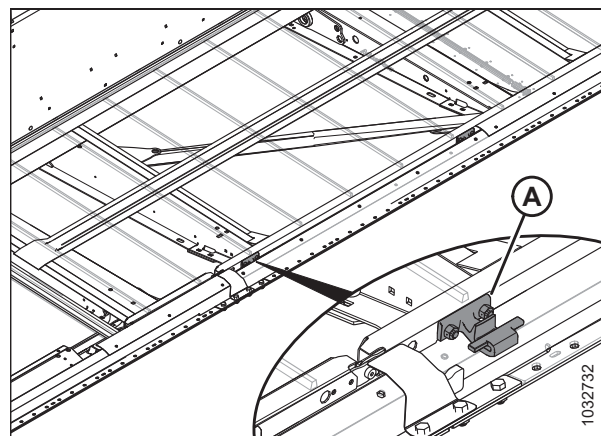
Рисунок 4.239: Опоры деки полотна
