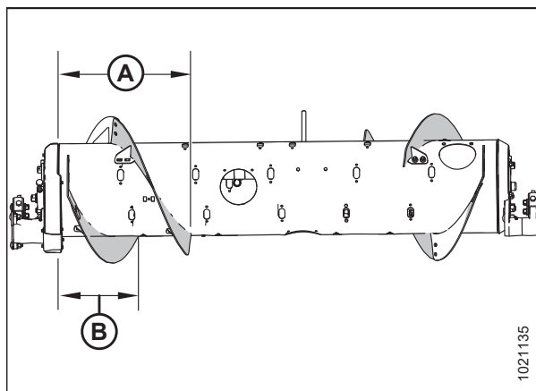
Рисунок 3.72: Узкая конфигурация: вид сзади
