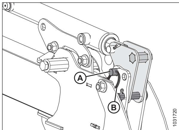
Рисунок 3.177: Регулировка цилиндра перемещения вперед/назад, тип 1 — заднее положение
