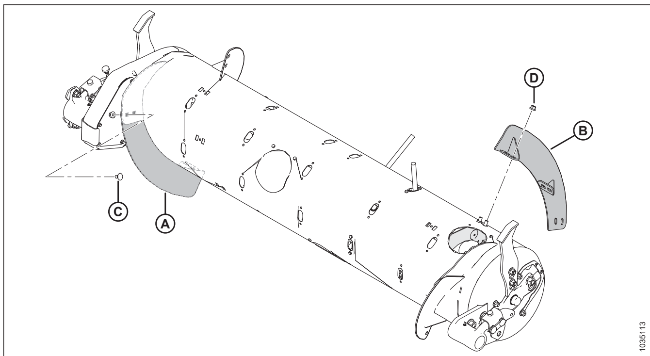
Рисунок 3.95: Широкая конфигурация
