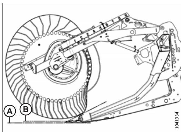
Рисунок 3.185: Профиль пальцев — положение эксцентрика 1
