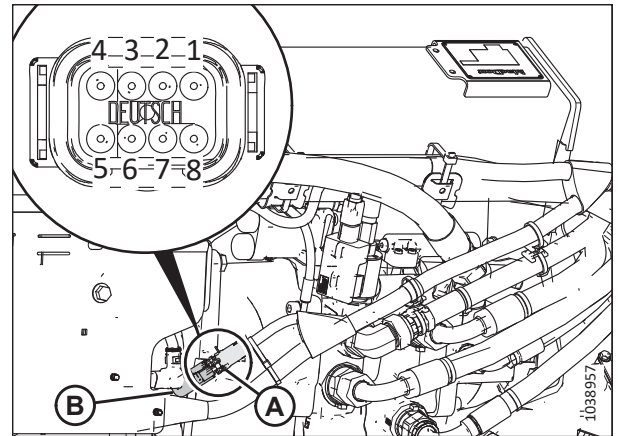
Рисунок 3.230: Соединитель Р600 — вид сзади
