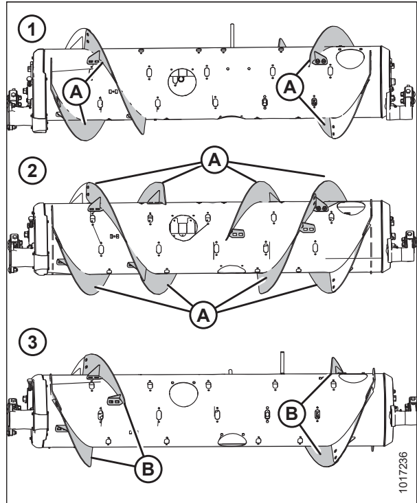
Рисунок 3.88: Конфигурации шнека: вид сзади
