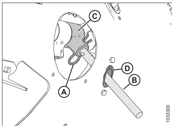
Рисунок 3.119: Палец шнека
