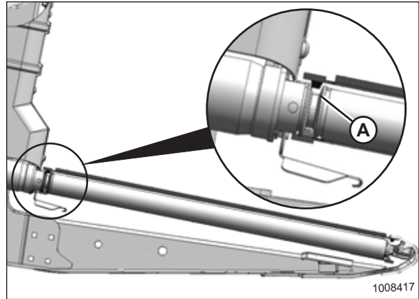
Рисунок 4.245: Приводной ролик
