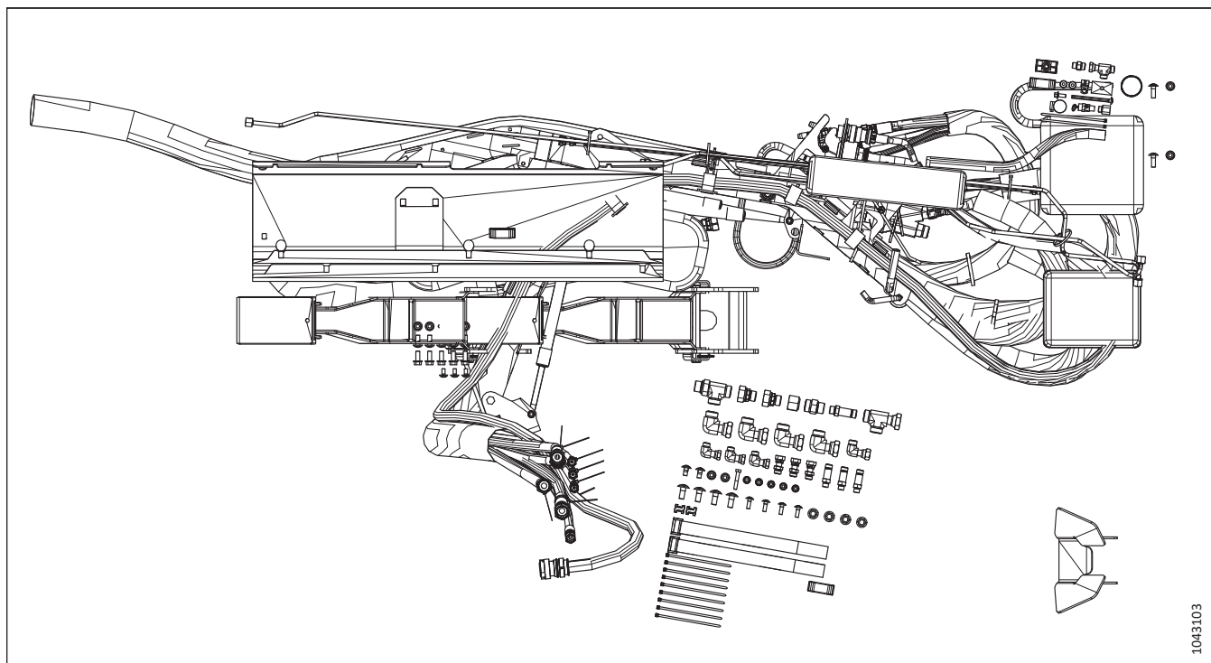
Рисунок 5.19: Комплект двойного назначения для использования сконфигурированных под комбайн жаток D2 на косилках M1/M2
