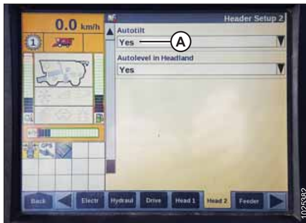
Рисунок 3.246: Приборная панель комбайна Case IH
