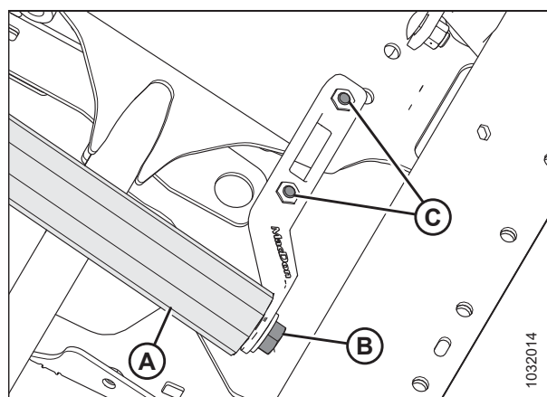
Рисунок 4.268: Приводной ролик
