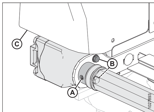
Рисунок 4.269: Приводной ролик
