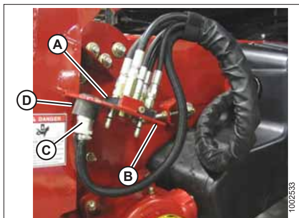
Рисунок 3.68: Хранение многоканальной муфты
