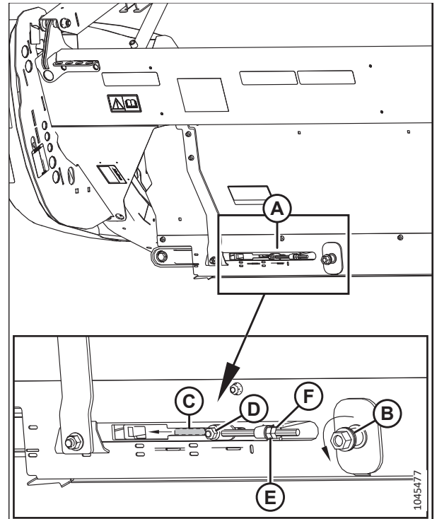
Рисунок 4.232: Регулировка левого натяжителя
