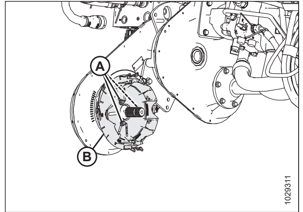
Рисунок 4.68: Крышка натяжителя цепи комплектного редуктора
