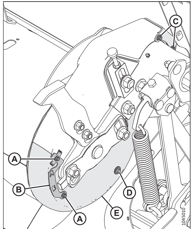
Рисунок 4.81: Привод подающего шнека — вид спереди
