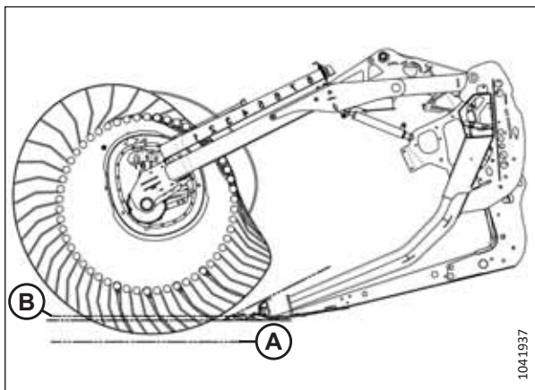
Рисунок 3.189: Профиль пальцев — положение эксцентрика 4, максимальный угол жатки
