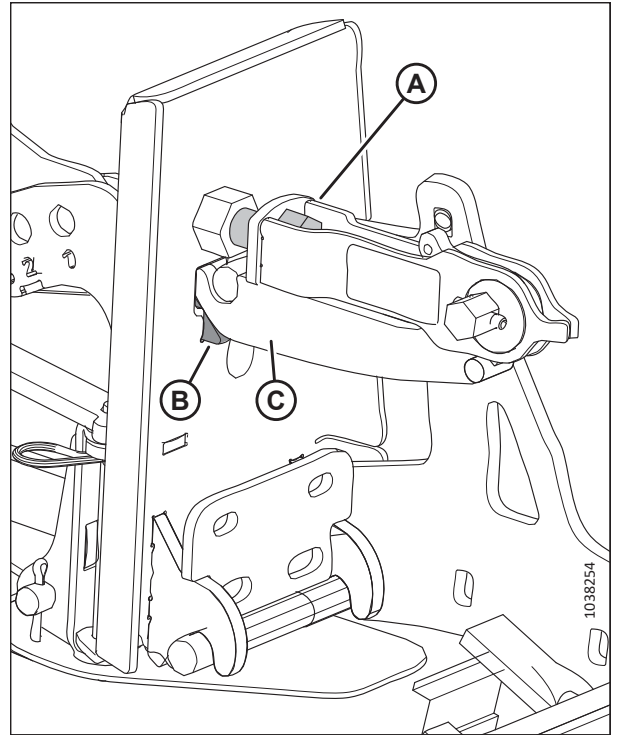
Рисунок 3.211: Делитель культуры зафиксирован на жатке
