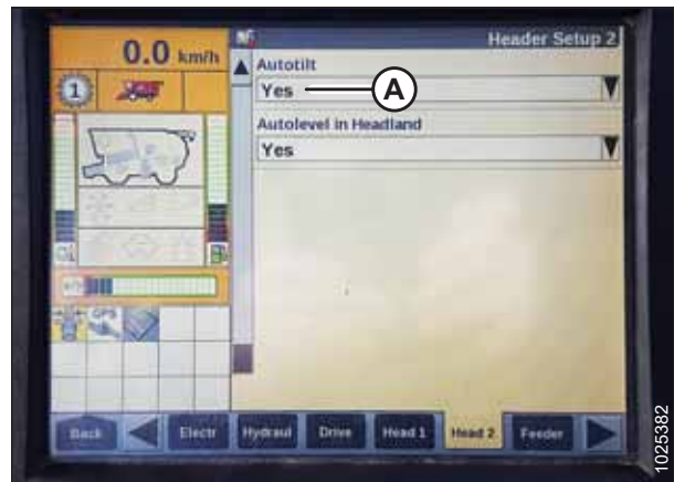
Рисунок 3.273: Приборная панель комбайна Case IH
