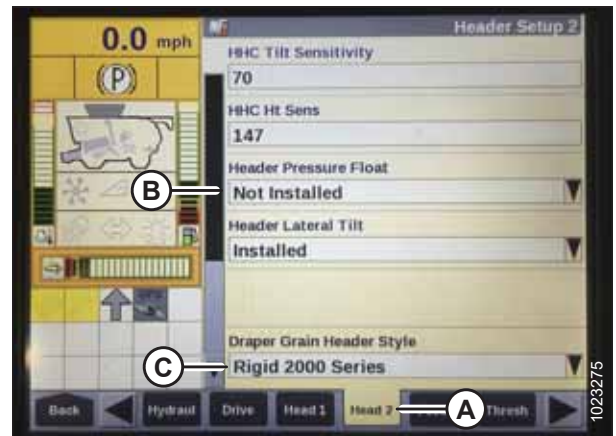
Рисунок 3.242: Приборная панель комбайна Case IH
