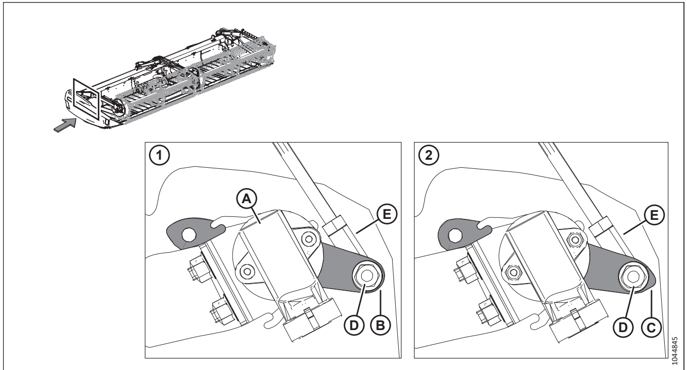
Рисунок 3.166: Расположение датчика высоты мотовила
