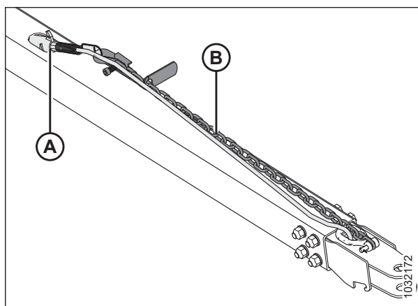
Рисунок 3.297: Сборка буксирной тяги
