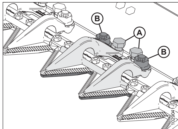
Рисунок 4.162: Прижим укороченного противорезающего пальца
