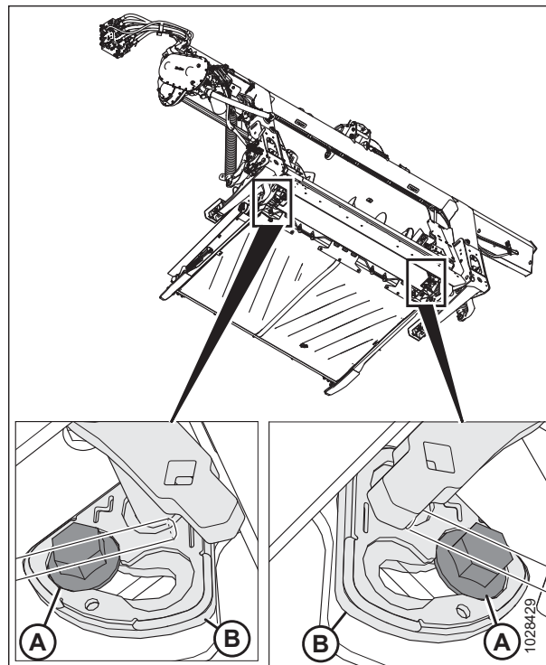
Рисунок 3.128: Регулировка флотации подающего шнека
