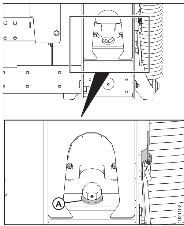
Рисунок 3.275: Шайба нижнего упора
