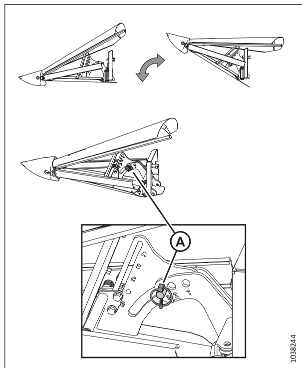
Рисунок 3.213: Регулировка нижнего упора
