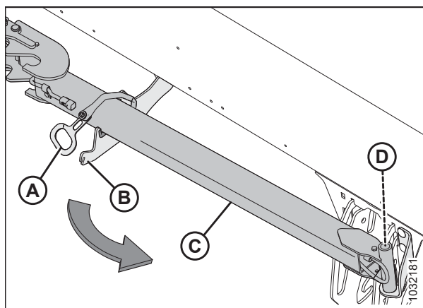
Рисунок 3.329: Удлинитель буксирной тяги в месте для хранения
