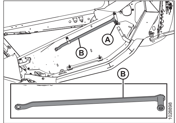
Рисунок 3.151: Местонахождение универсального инструмента
