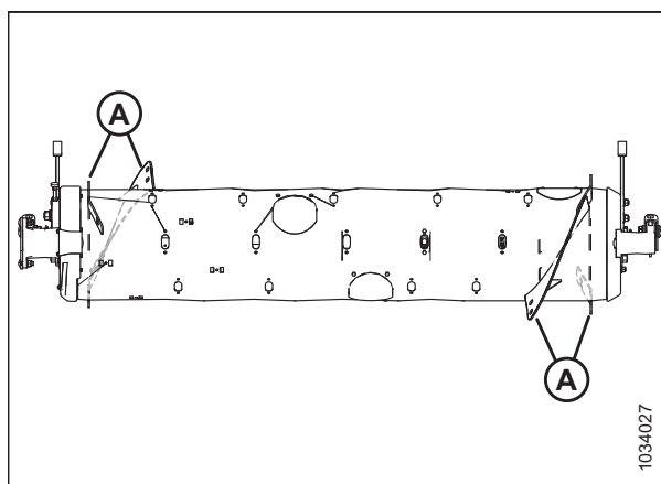
Рисунок 3.75: Сверхширокая конфигурация: вид сзади
