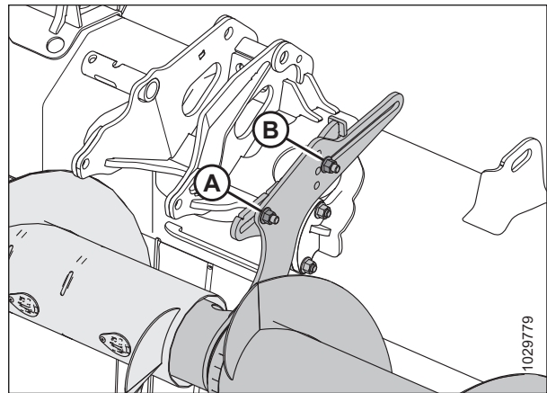
Рисунок 3.194: Первоначальное положение регулируемых креплений — трехсоставной шнек
