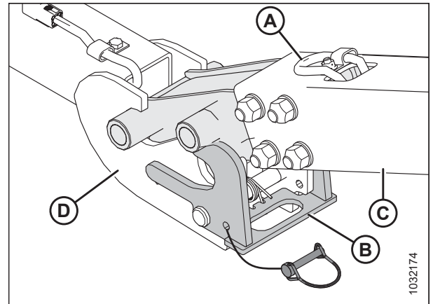
Рисунок 3.299: Буксирная тяга/место соединения удлинителя
