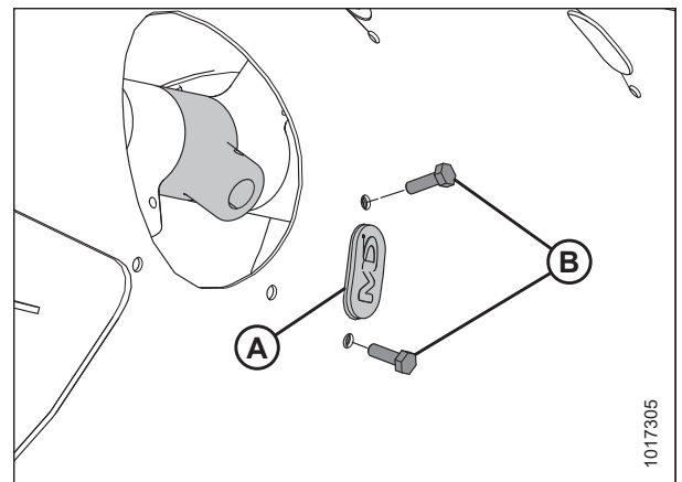
Рисунок 3.121: Заглушка
