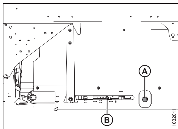
Рисунок 4.261: Натяжитель полотна
