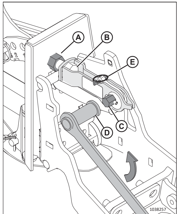
Рисунок 3.212: Регулировка защелки
