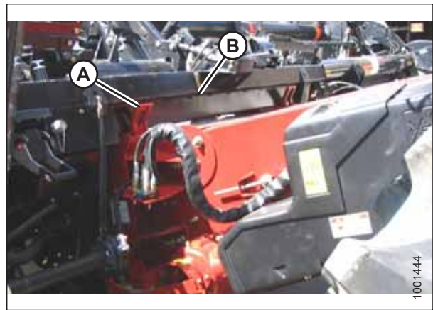
Рисунок 3.53: Комбайн и копирующий модуль
