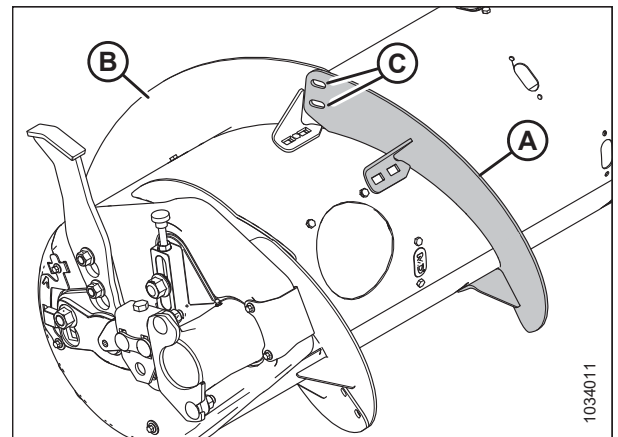
Рисунок 3.112: Левая сторона шнека
