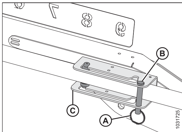
Рисунок 3.178: Регулировка цилиндра перемещения вперед/назад, тип 2 — переднее положение
