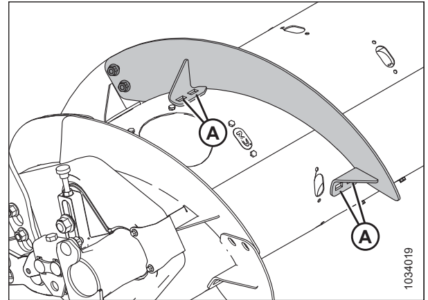
Рисунок 3.116: Витки на левой стороне шнека
