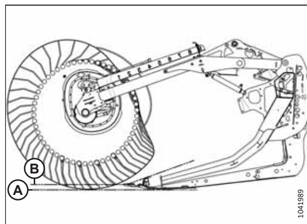
Рисунок 3.188: Профиль пальцев — положение эксцентрика 4, минимальный угол атаки жатки
