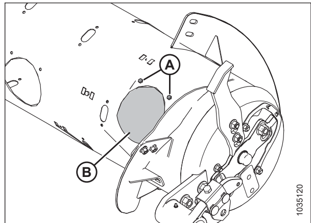
Рисунок 3.104: Технологическая крышка шнека: правая сторона
