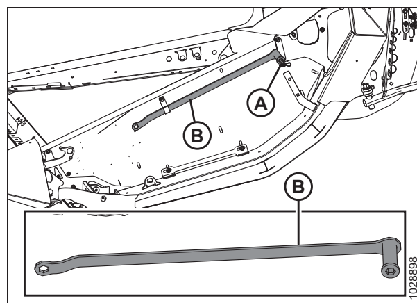
Рисунок 3.144: Местонахождение универсального инструмента
