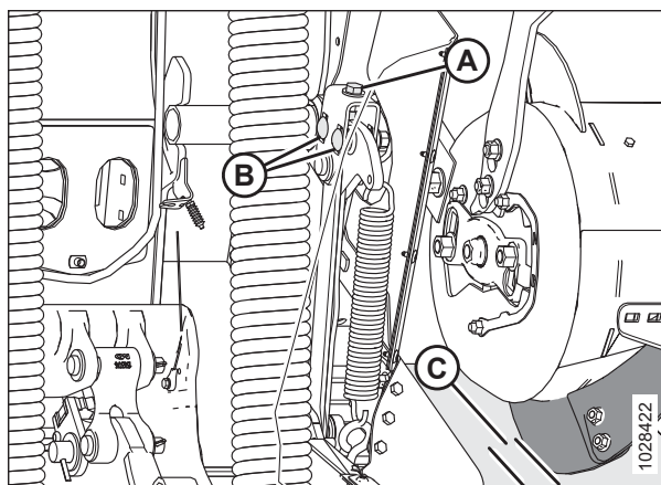
Рисунок 4.74: Зазор шнека
