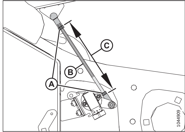
Рисунок 3.169: Датчик высоты мотовила — правая опора мотовила опущена
