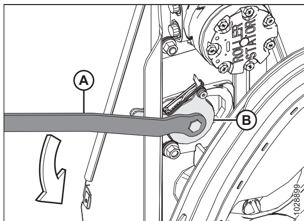
Рисунок 4.332: Привод мотвила
