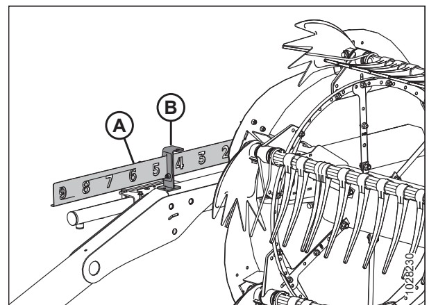
Рисунок 3.171: Индикатор продольного перемещения
