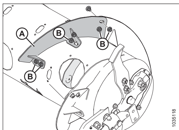
Рисунок 3.107: Короткий виток: правая сторона
