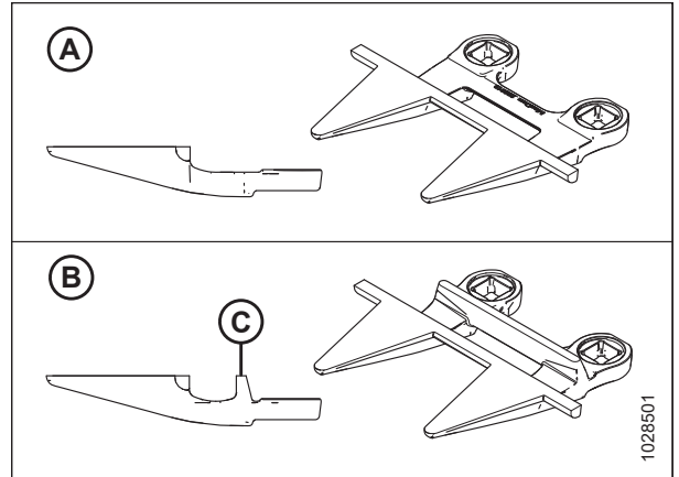
Рисунок 4.158: Концевой противорежущий палец и укороченный противорежущий палец
