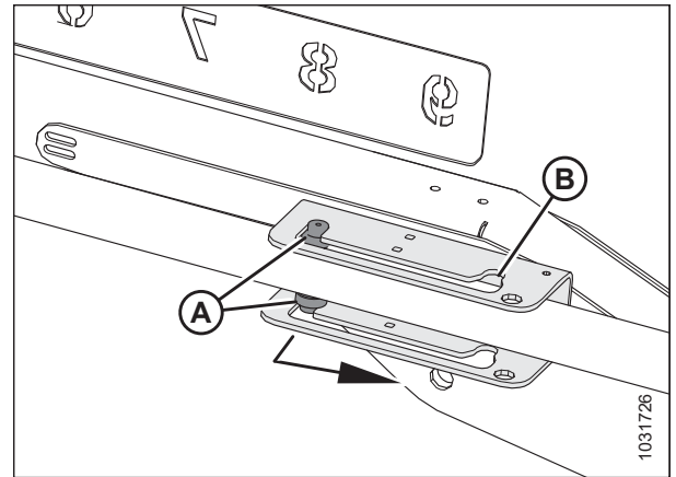
Рисунок 3.179: Регулировка цилиндра перемещения вперед/назад, тип 2 — переднее положение
