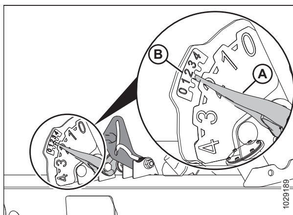
Рисунок 3.146: Левый индикатор настроек флотации и индикатор системы автоматического контроля высоты жатки (АННС)
