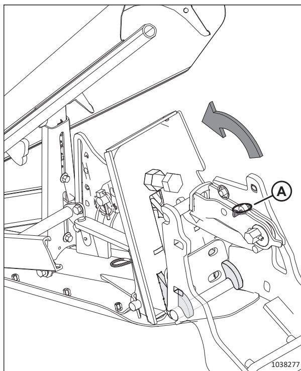
Рисунок 3.207: Защелка отсоединена
