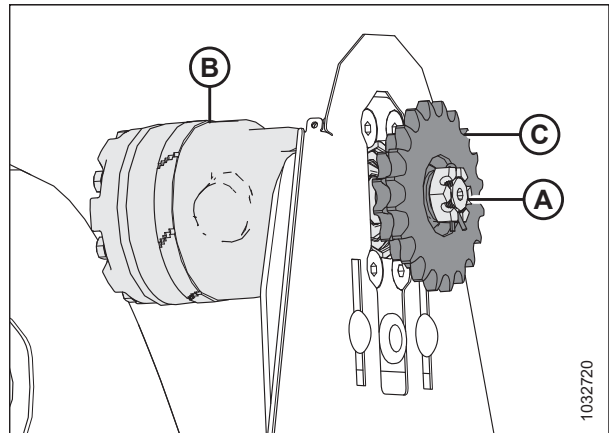
Рисунок 4.341: Двойная звездочка
