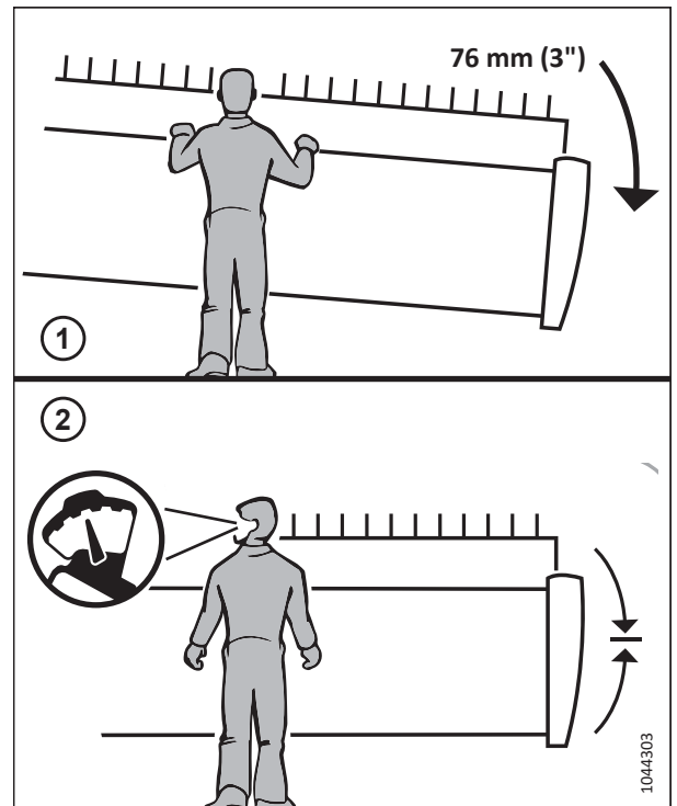
Рисунок 3.148: Проверка флотации
