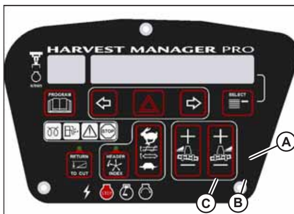
Рисунок 3.292: Органы управления комбайна Case
