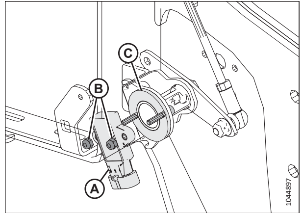
Рисунок 3.168: Датчик высоты мотовила: правый рычаг мотовила
