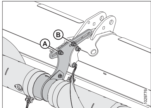
Рисунок 3.193: Первоначальное положение регулируемых креплений — двухсоставной шнек
