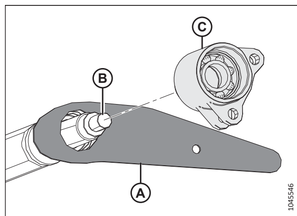
Рисунок 4.203: Натяжной ролик
