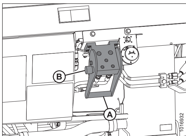
Рисунок 3.69: Гнездо копирующего модуля
