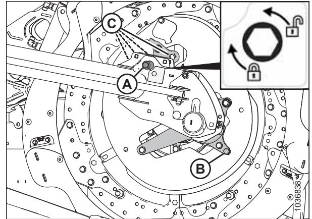
Рисунок 3.191: Положения диска эксцентрика
