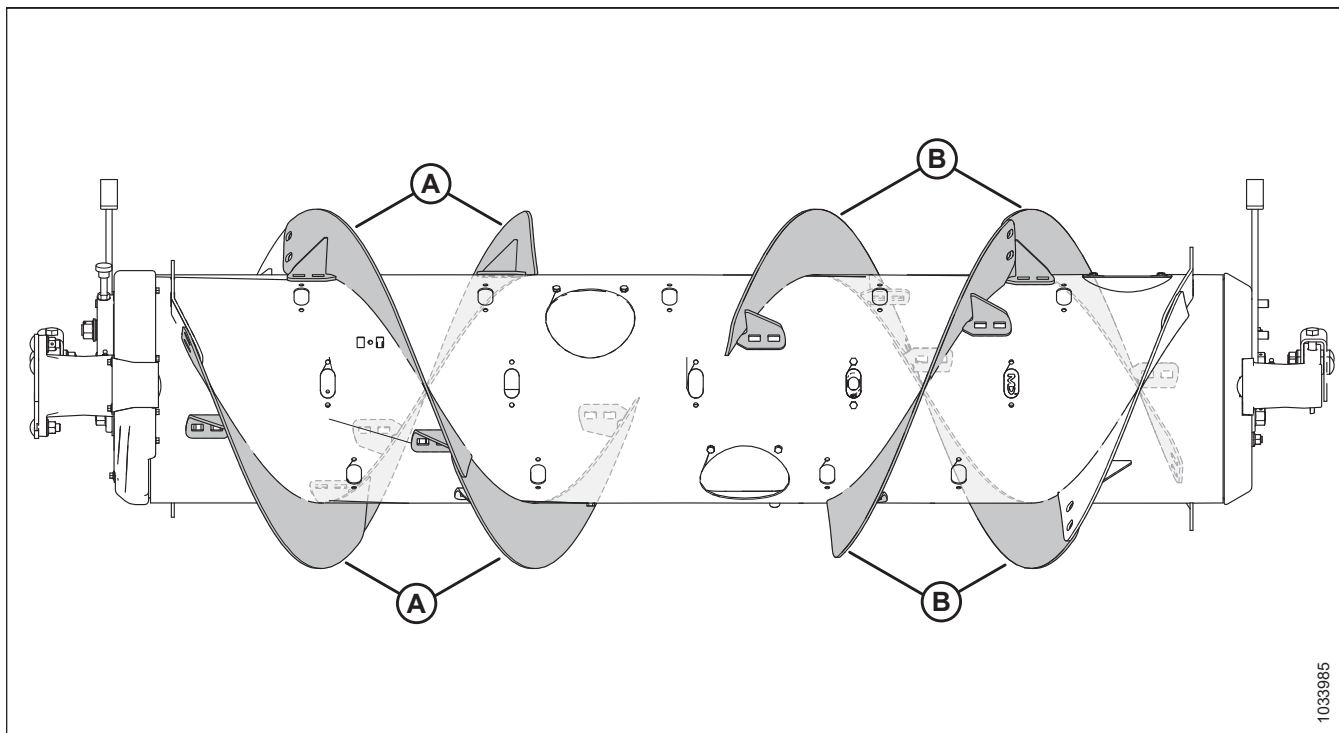
Рисунок 3.76: Сверхузкая конфигурация
