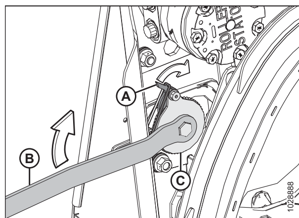
Рисунок 4.330: Привод мотовила
