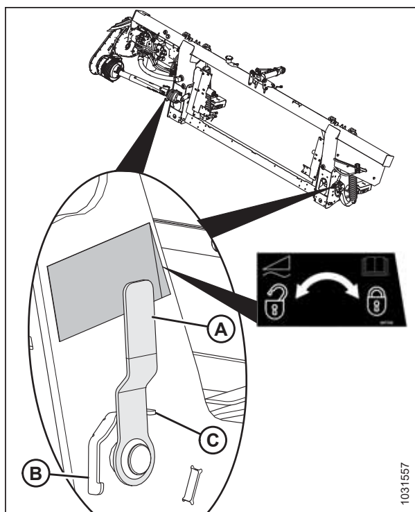
Рисунок 3.153: Замок флотации в запертом положении
