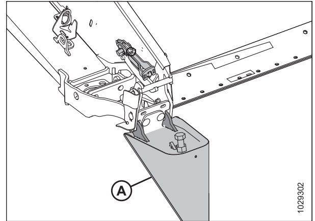
Рисунок 3.200: Делитель с опцией замка
