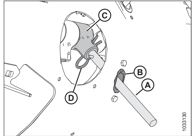
Рисунок 3.124: Палец шнека
