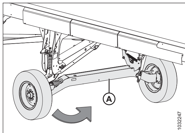
Рисунок 3.327: Правая транспортная ось
