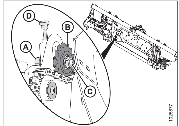
Рисунок 4.94: Привод шнека
