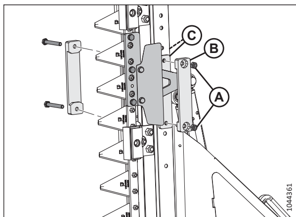
Рисунок 4.372: Направляющие головок ножа
