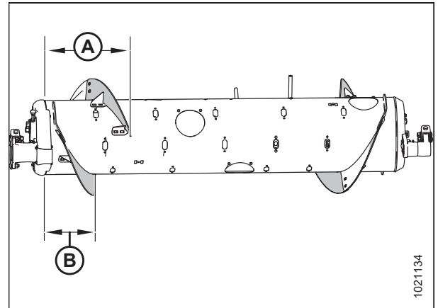
Рисунок 3.73: Средняя конфигурация: вид сзади
