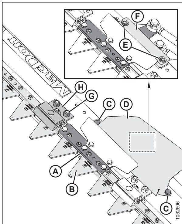
Рисунок 4.363: Вертикальный нож — противорежущий палец снят
