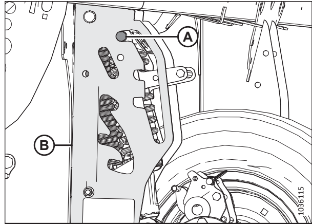
Рисунок 3.315: Штифт шарнира левого транспортного колеса в самом высоком положении хранения
