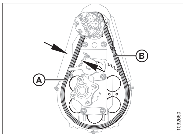
Рисунок 4.333: Привод мотвила
