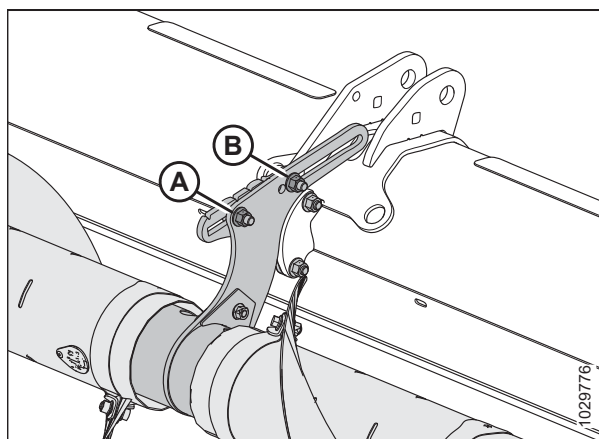
Рисунок 3.196: Первоначальное положение регулируемых креплений — двухсоставной шнек
