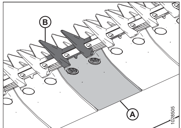
Рисунок 4.166: Центральный противорежущий палец и износная пластина
