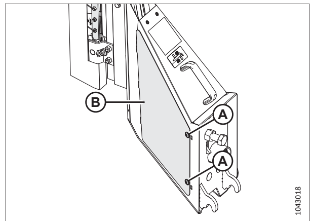
Рисунок 4.375: Снятие крышки
