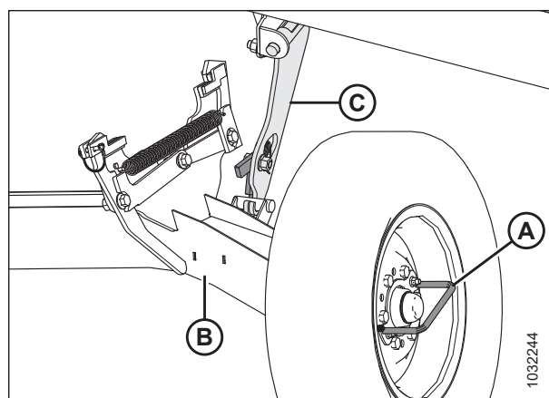
Рисунок 3.326: Правая рабочая опора
