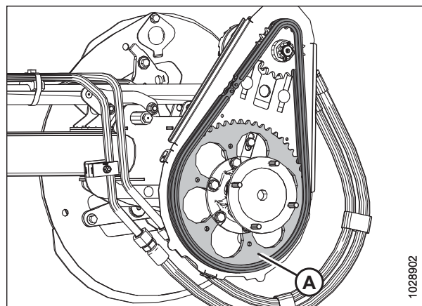
Рисунок 4.334: Привод мотовила
