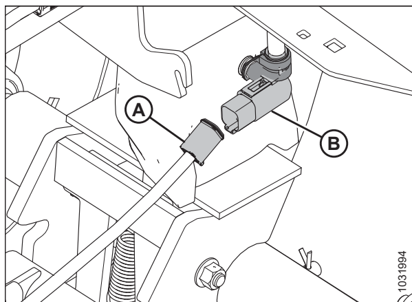
Рисунок 3.303: Электрическое соединение буксирной тяги
