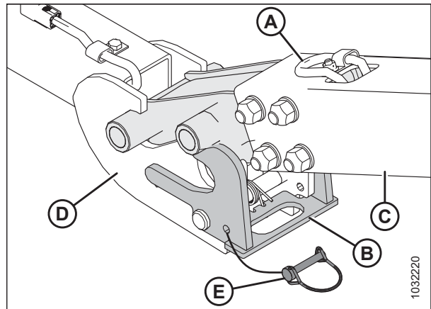
Рисунок 3.334: Буксирная тяга к удлинителю
