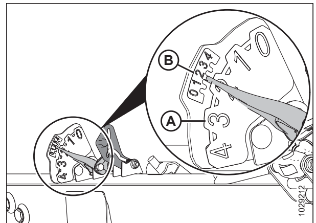
Рисунок 3.137: Индикатор флотации — левая сторона
