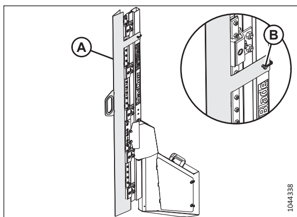
Рисунок 4.370: Вертикальный нож
