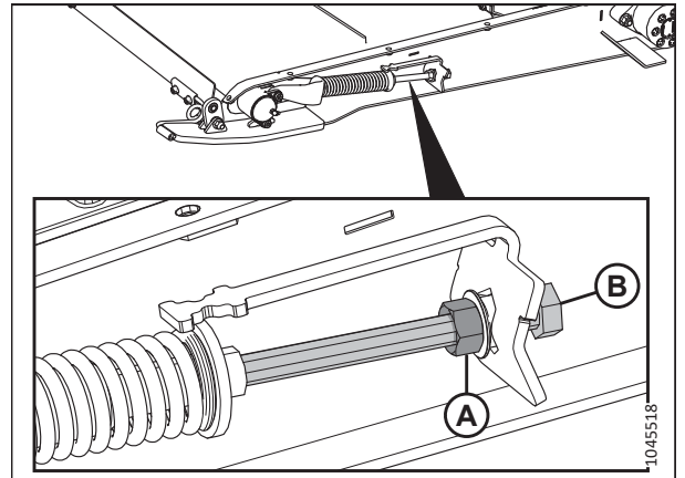
Рисунок 4.184: Натяжитель подающего полотна
