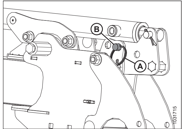
Рисунок 3.175: Регулировка цилиндра перемещения вперед/назад, тип 1 — переднее положение
