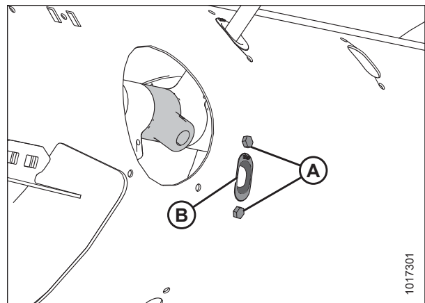
Рисунок 3.123: Отверстие пальца шнека
