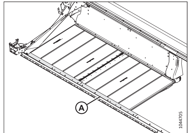
Рисунок 4.233: Уплотнения ножевого бруса
