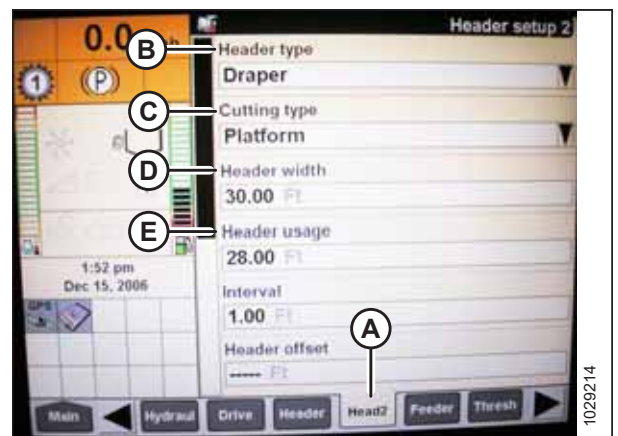
Рисунок 3.271: Приборная панель комбайна Case IH
