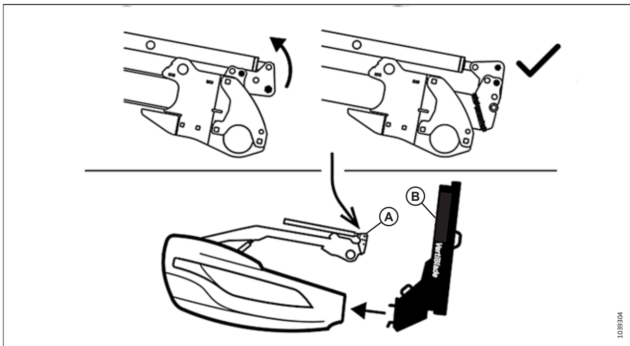
Рисунок 4.360: Положение цилиндра перемещения мотовила вперед/назад для вертикальных ножей
