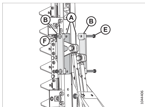
Рисунок 4.379: Направляющие головок ножа
