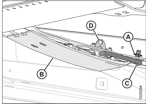
Рисунок 3.135: Внутренний копирующий башмак
