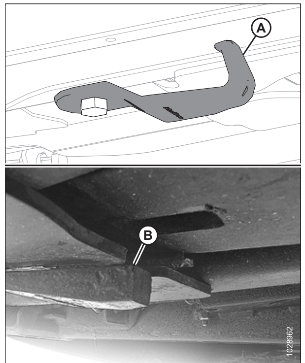
Рисунок 4.227: Крюки расцепного предохранителя соединения
