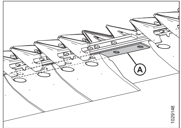
Рисунок 4.165: Ножевой брус
