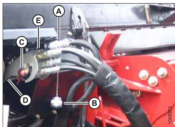
Рисунок 3.67: Многоканальная муфта
