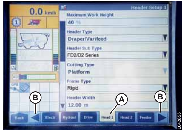
Рисунок 3.38: Приборная панель комбайна Case IH
