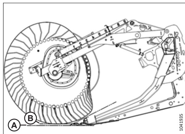
Рисунок 3.186: Профиль пальцев — положение эксцентрика 2
