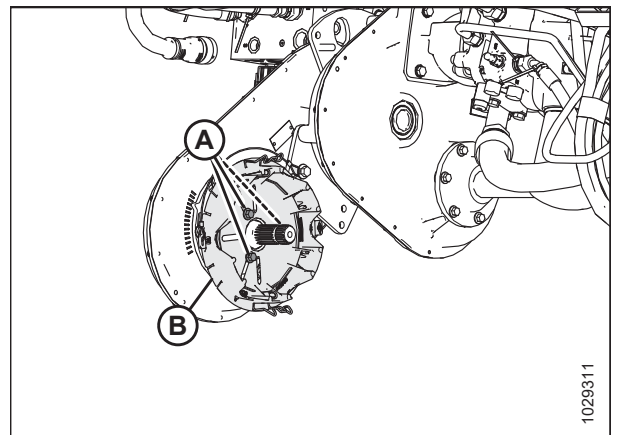
Рисунок 4.70: Крышка натяжителя цепи комплектного редуктора
