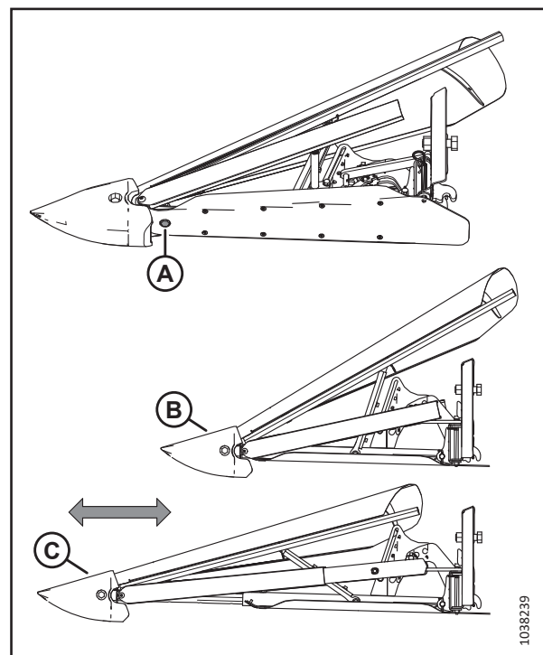
Рисунок 3.214: Продольная регулировка носового конуса
