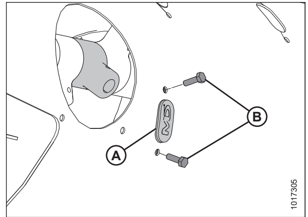
Рисунок 4.109: Отверстие пальца шнека
