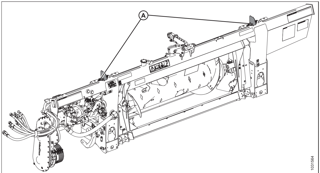
Рисунок 3.225: Копирующий модуль FM200
