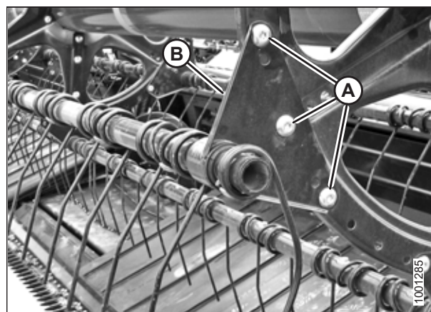
Рисунок 4.285: Рычаг граблины
