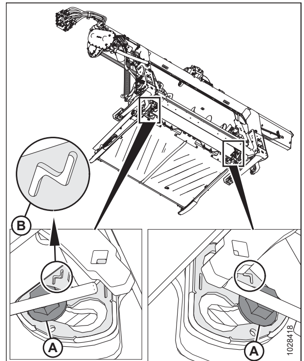
Рисунок 4.72: Положение флотации
