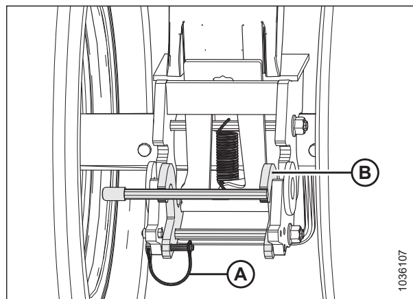
Рисунок 3.312: Левые транспортные колеса — защелка, препятствующая вращению, закрыта
