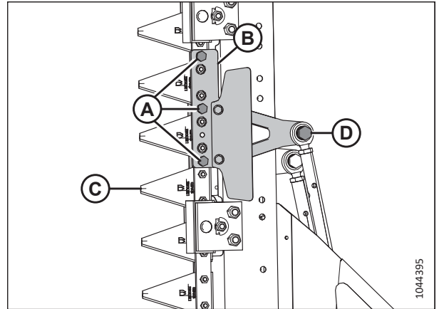
Рисунок 4.373: Наружная головка ножа
