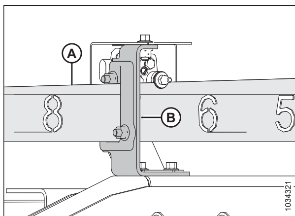
Рисунок 4.272: Продольное положение
