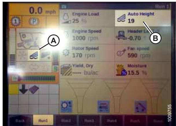
Рисунок 3.287: Приборная панель комбайна Case IH
