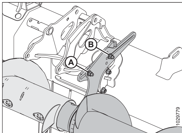
Рисунок 3.197: Первоначальное положение регулируемых креплений — трехсоставной шнек
