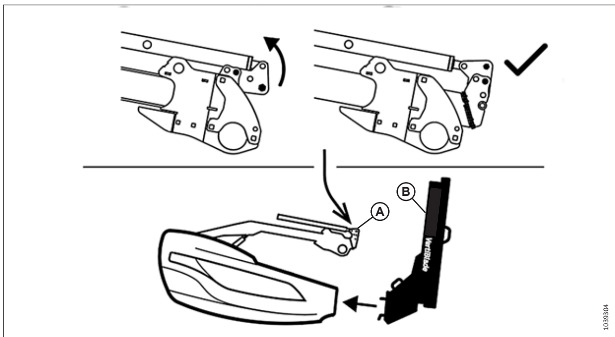
Рисунок 3.172: Положение мотовила с установленной опцией вертикального ножа
