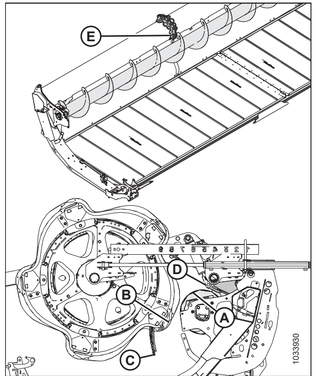
Рисунок 3.198: Места проверки зазора верхнего поперечного шнека
