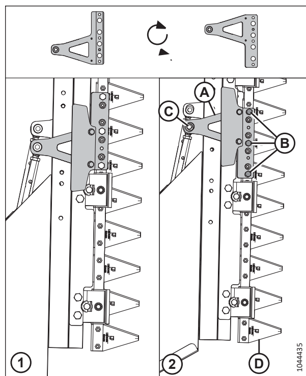
Рисунок 4.378: Внутренняя головка ножа
