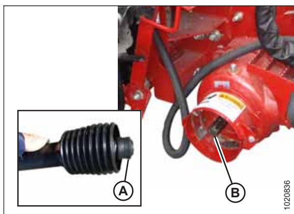
Рисунок 3.61: Выходной вал комбайна
