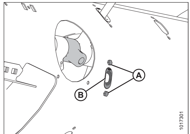
Рисунок 4.110: Отверстие пальца шнека
