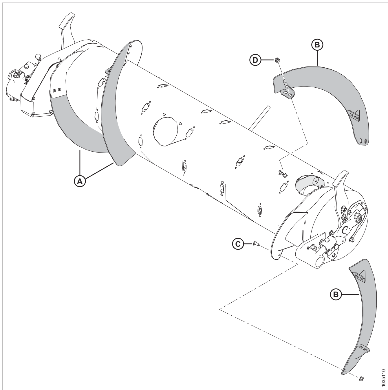
Рисунок 3.85: Узкая конфигурация
