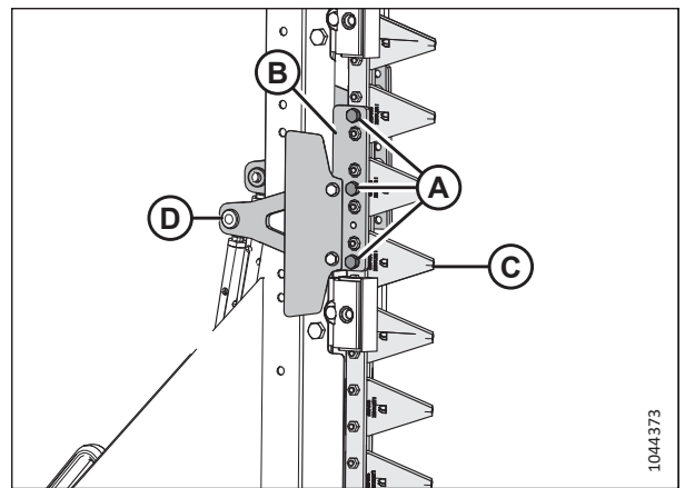
Рисунок 4.374: Внутренняя головка ножа
