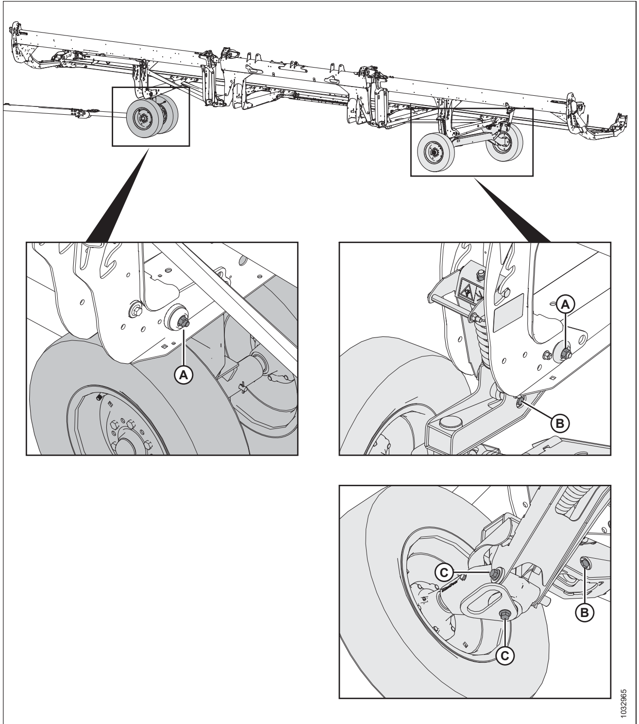
Рисунок 4.348: Болты узла транспортировочной системы
