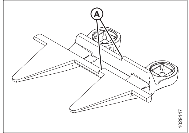
Рисунок 4.164: Центральный противорежущий палец
