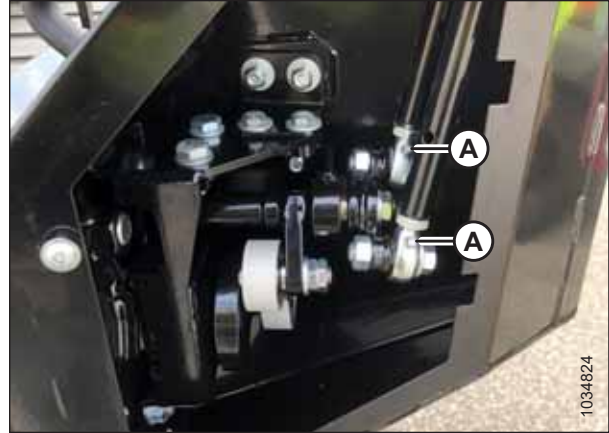
Рисунок 4.366: Тавотницы на толкателях вертикальных ножей
