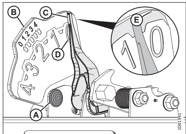
Рисунок 3.142: Индикатор флотации
