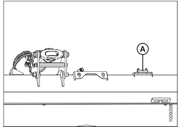
Рисунок 3.274: Спиртовой уровень
