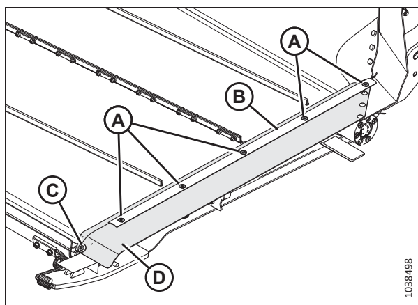
Рисунок 4.176: Зазор между лентой и ножевым брусом подающего полотна
