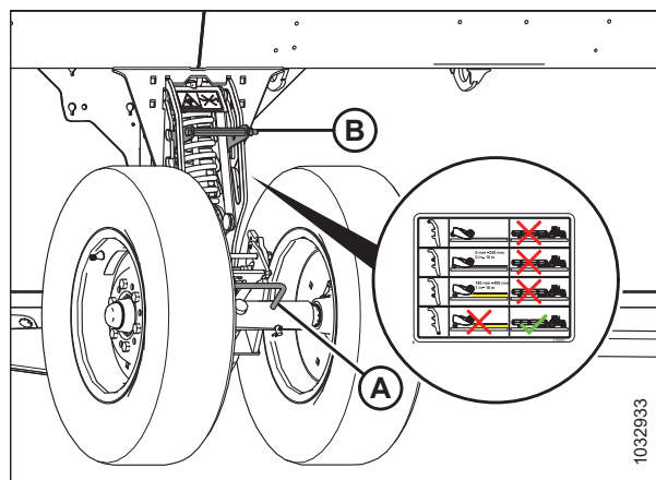
Рисунок 3.134: Левое колесо
