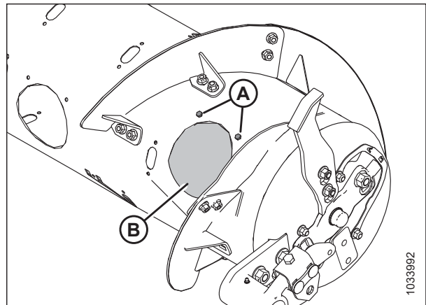
Рисунок 3.98: Технологическая крышка шнека: правая сторона
