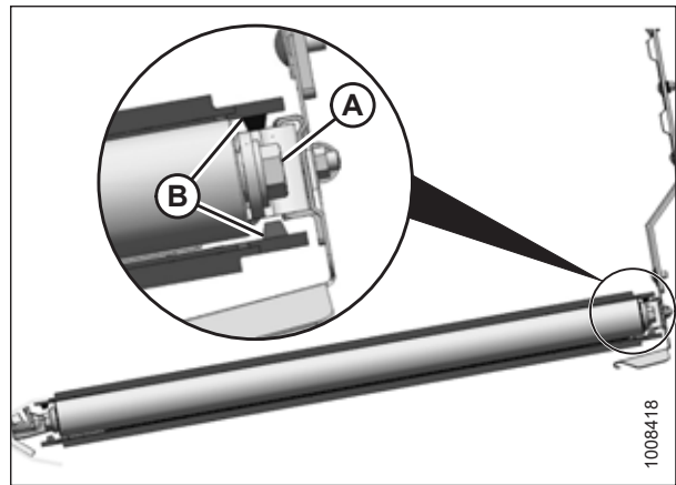
Рисунок 4.246: Натяжной ролик
