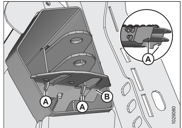
Рисунок 3.309: Удерживающие крюки на стороне вилки
