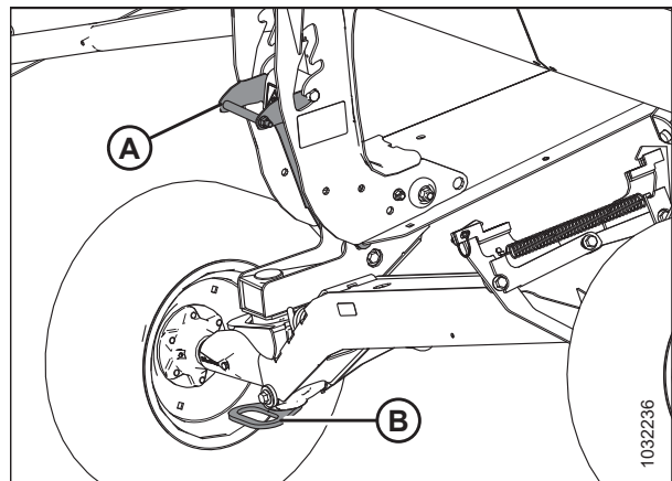
Рисунок 3.324: Копирующие колеса
