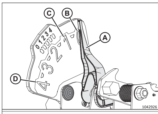
Рисунок 3.291: Индикатор флотации
