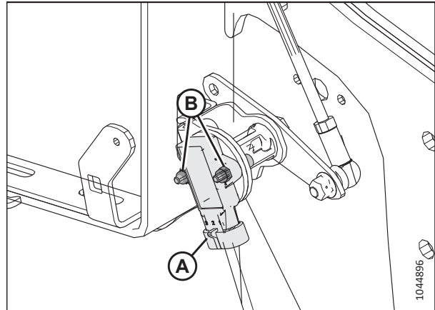
Рисунок 3.167: Датчик высоты мотовила: правый рычаг мотовила
