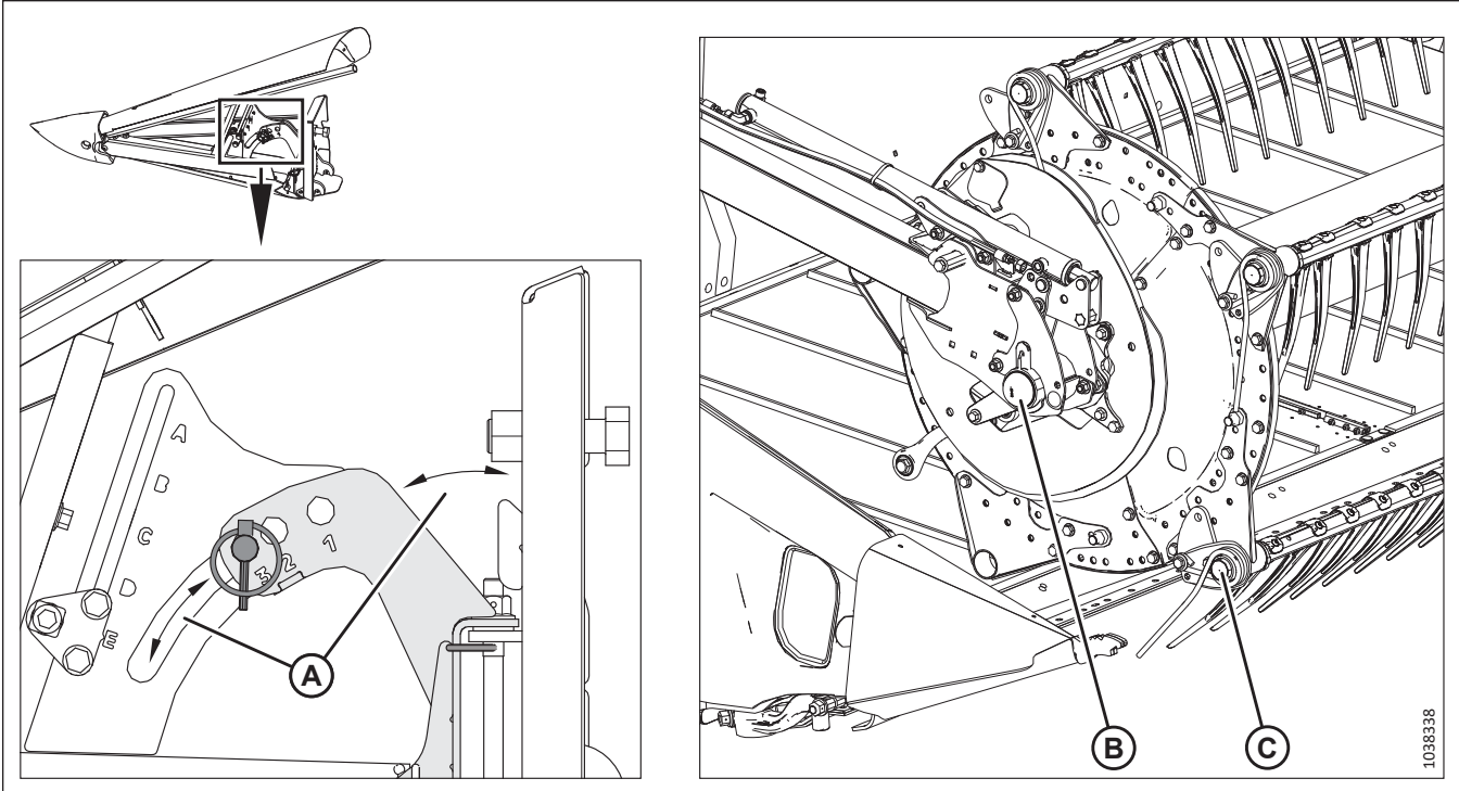
Рисунок 3.218: Диапазон движения копирующего делителя культуры
