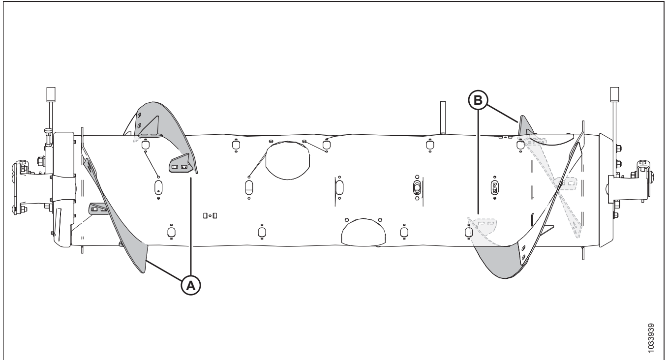
Рисунок 3.86: Средняя конфигурация
