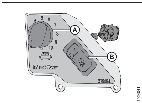
Рисунок 3.161: Органы управления скоростью бокового полотна в кабине
