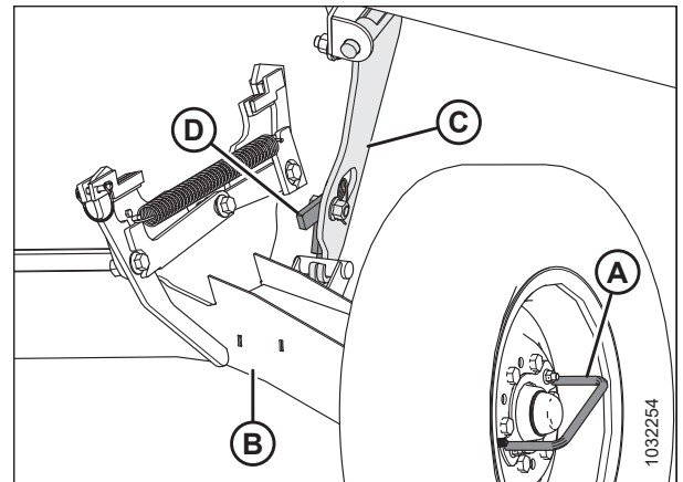
Рисунок 3.318: Правая транспортная ось зафиксирована в рабочем положении
