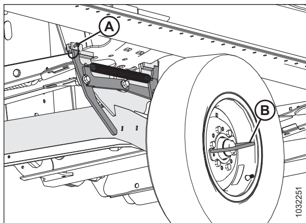
Рисунок 3.328: Правая транспортная ось
