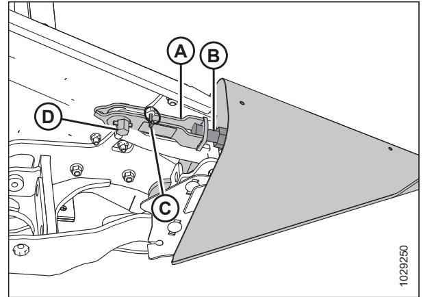
Рисунок 3.205: Делитель с опцией замка
