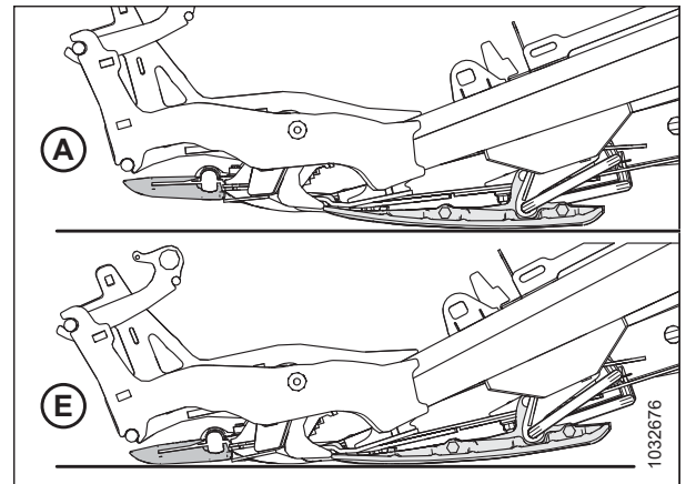
Рисунок 3.155: Углы противорежущих пальцев
