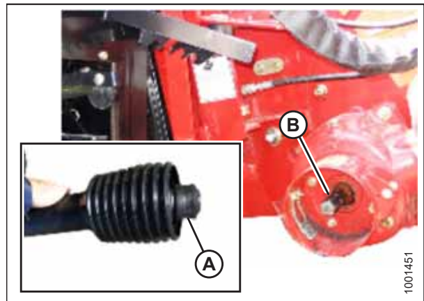
Рисунок 3.64: Кардан привода жатки
