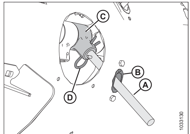
Рисунок 4.111: Палец шнека
