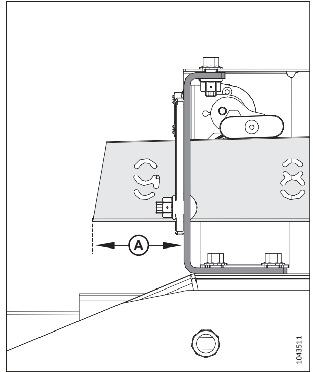
Рисунок 3.182: Скоба продольного перемещения
