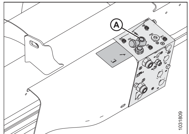
Рисунок 3.192: Отсечной клапан
