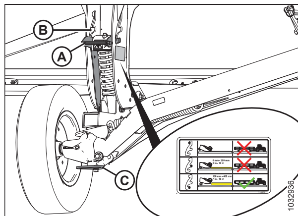
Рисунок 3.133: Правое колесо
