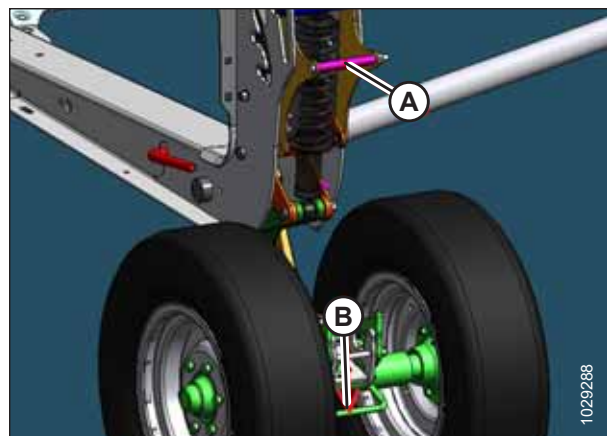
Рисунок 3.320: Передние транспортные колеса
