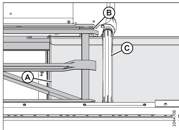
Рисунок 4.235: Полотно
