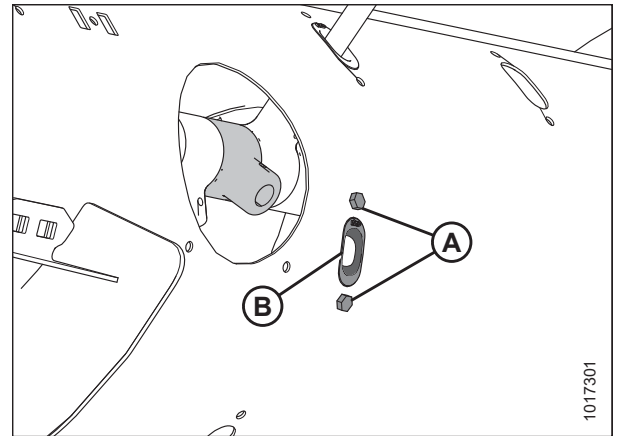
Рисунок 3.120: Отверстие пальца шнека
