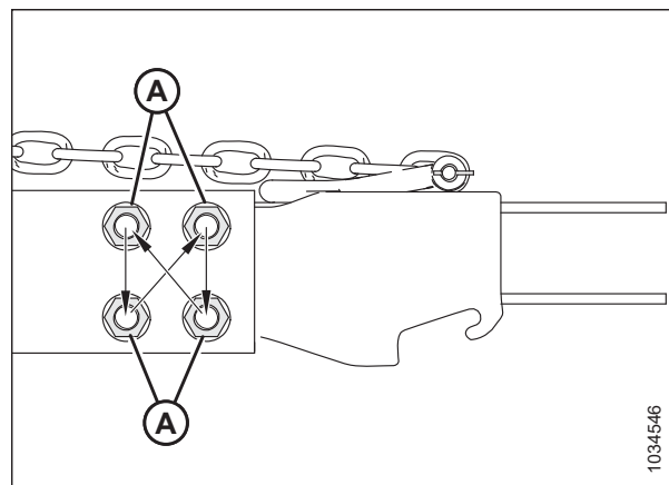
Рисунок 4.354: Последовательность затяжки
