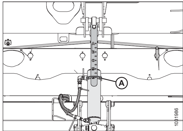
Рисунок 3.232: Центральное соединение
