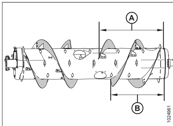
Рисунок 3.71: Сверхузкая конфигурация: вид сзади
