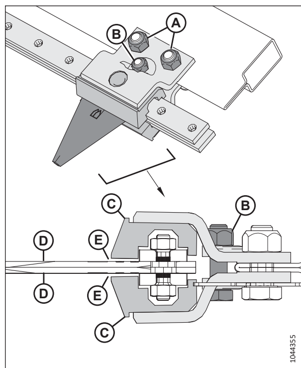
Рисунок 4.365: Вертикальный нож (вид сверху)
