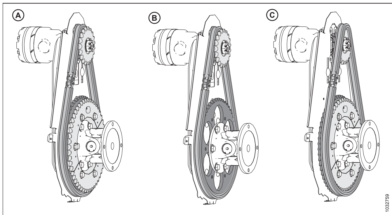
Рисунок 4.339: Конфигурации привода мотвила — дополнительные двойные звездочки
