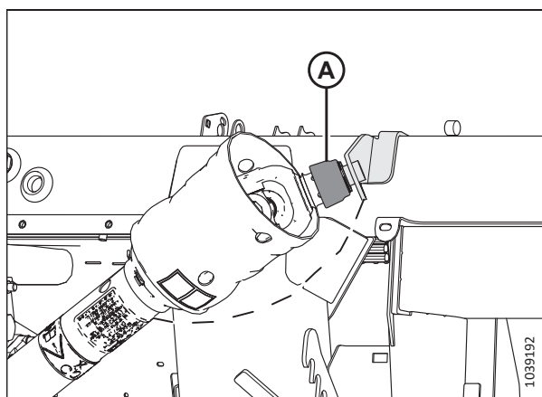
Рисунок 3.60: Карданный вал в положении хранения — карданный вал для работы на холмистой местности В7180, В7181 или В7326
