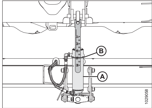
Рисунок 3.141: Центральное соединение
