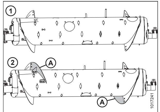
Рисунок 3.87: Конфигурации шнека: вид сзади
