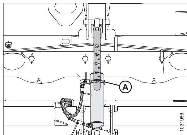
Рисунок 3.227: Центральное соединение
