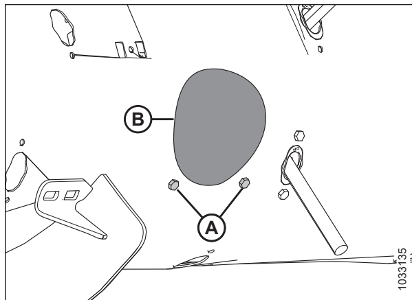
Рисунок 3.118: Крышка отверстия доступа к шнеку
