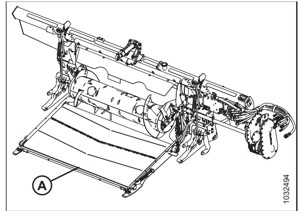
Рисунок 3.163: Копирующий модуль FM200
