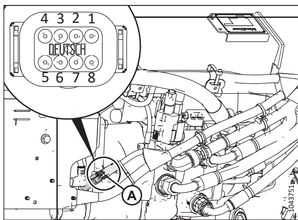
Рисунок 3.226: Разъем
