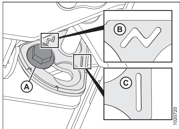
Рисунок 3.127: Положения флотации шнека
