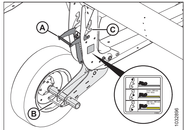
Рисунок 3.132: Стабилизирующее колесо
