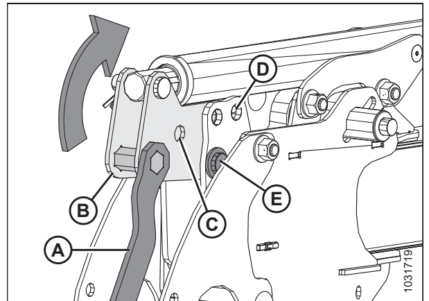
Рисунок 3.176: Регулировка цилиндра перемещения вперед/назад, тип 1 — переднее положение
