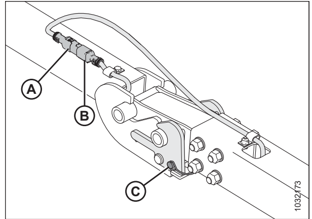
Рисунок 3.335: Жгут проводов буксирной тяги/удлинителя
