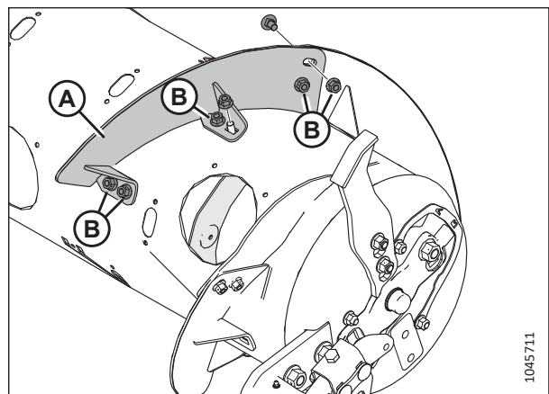
Рисунок 3.99: Короткий виток: правая сторона
