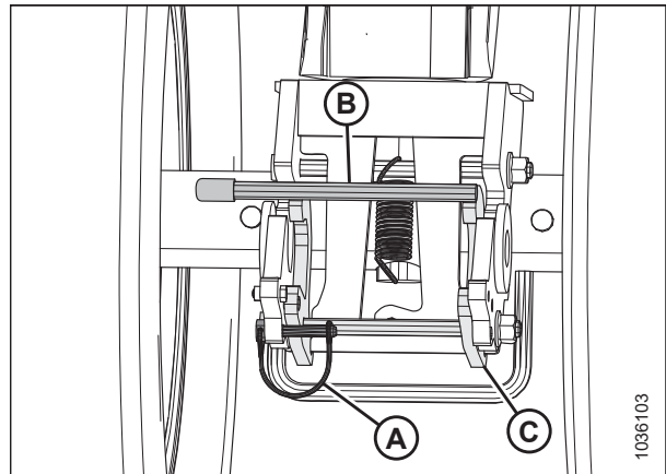
Рисунок 3.311: Левые транспортные колеса — защелка, препятствующая вращению, открыта
