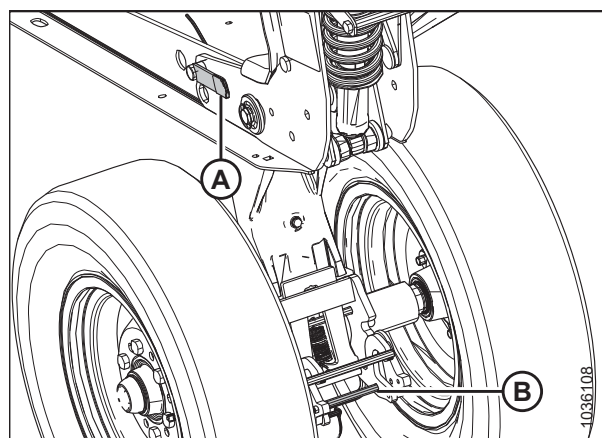
Рисунок 3.313: Левые транспортные колеса — шарнир освобожден
