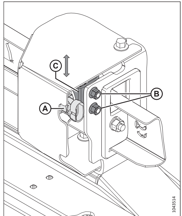
Рисунок 3.183: Датчик продольного перемещения
