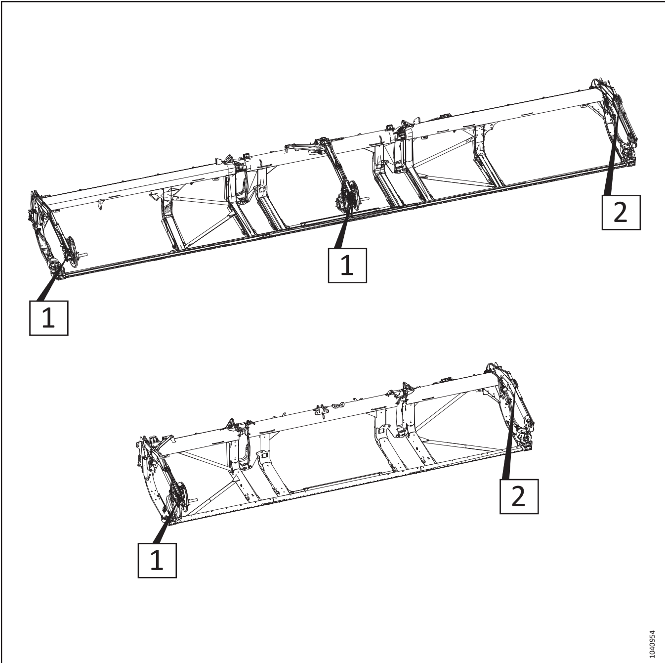
Рисунок 3.174: Регулируемые цилиндры перемещения вперед/назад — цифры для обозначения процедур
