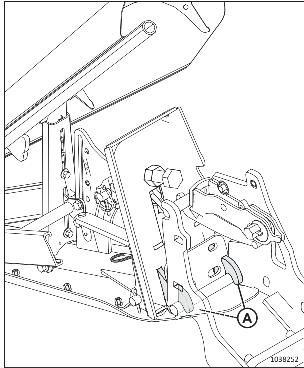
Рисунок 3.209: Установка делителя
