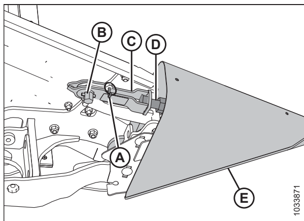
Рисунок 3.199: Делитель с опцией замка
