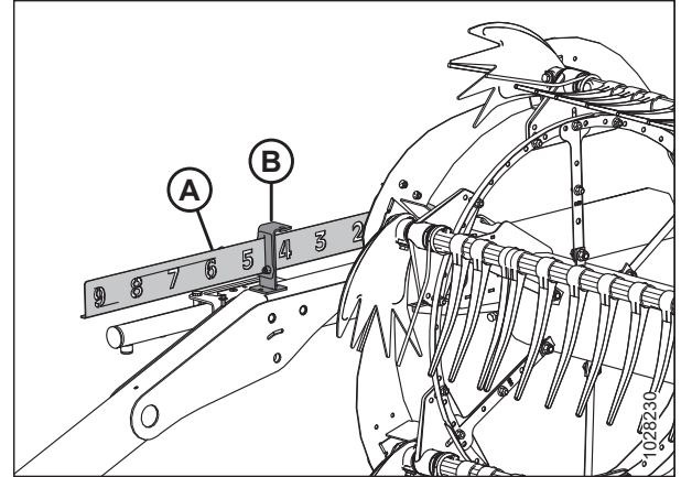
Рисунок 3.170: Индикатор продольного перемещения
