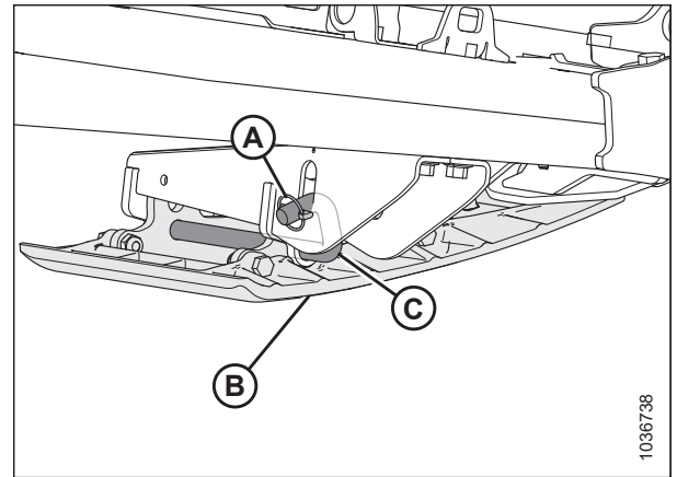
Рисунок 3.136: Внешний копирующий башмак
