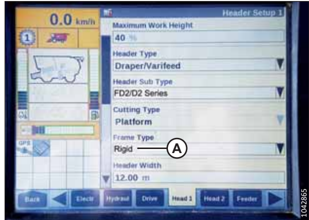
Рисунок 3.280: Приборная панель комбайна Case IH
