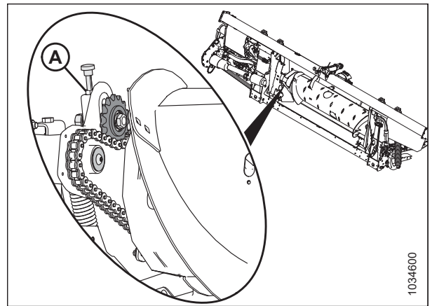
Рисунок 4.95: Привод шнека
