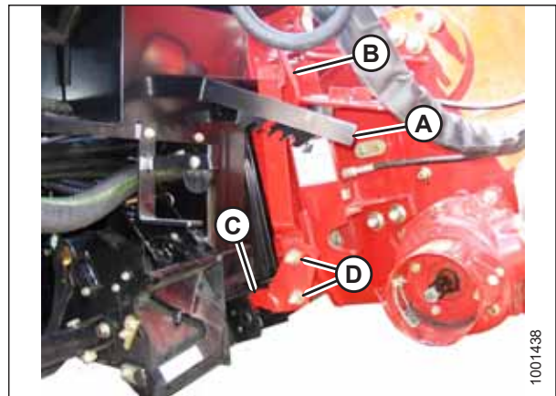
Рисунок 3.54: Комбайн и копирующий модуль
