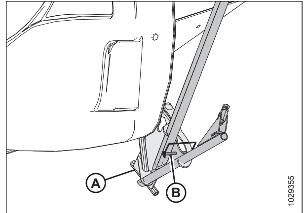
Рисунок 3.224: Место хранения делителей для скашивания риса
