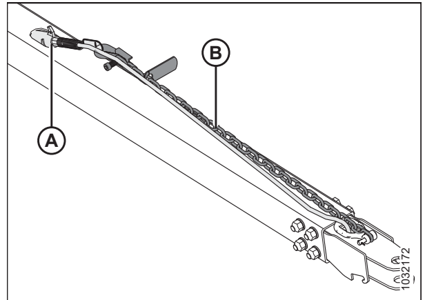
Рисунок 3.336: Жгут проводов буксирной тяги
