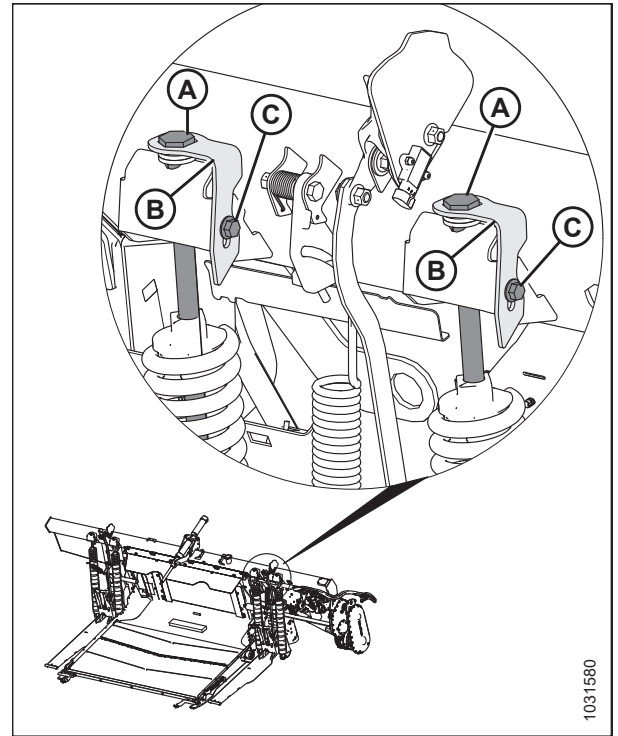
Рисунок 3.147: Регулировка флотации слева
