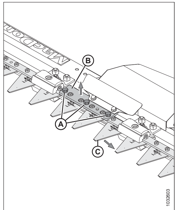
Рисунок 4.362: Вертикальный нож — противорежущий палец снят
