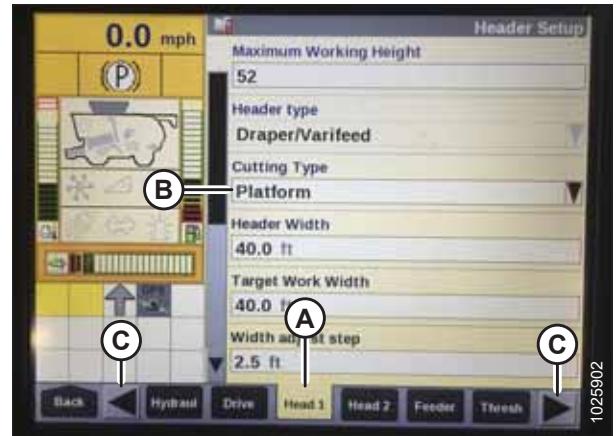
Рисунок 3.241: Приборная панель комбайна Case IH
