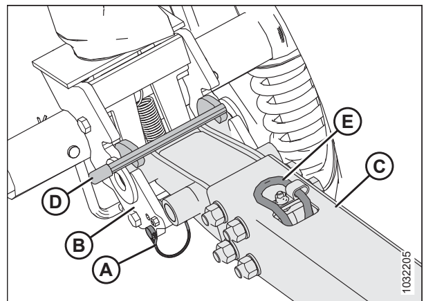
Рисунок 3.337: Буксирная тяга и левый транспортный шарнир
