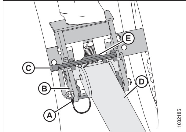
Рисунок 3.332: Удлинитель буксирной тяги к левому транспортному шарниру
