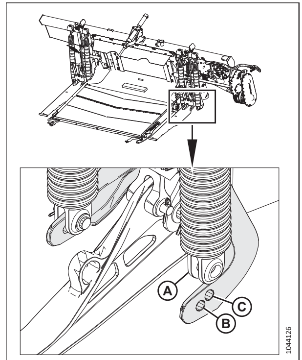
Рисунок 3.152: Пружина флотации, отсоединенная от рычага флотации
