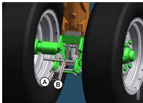
Рисунок 3.322: Передние транспортные колеса
