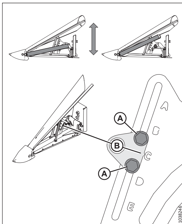
Рисунок 3.216: Регулировка высоты бокового дефлектора
