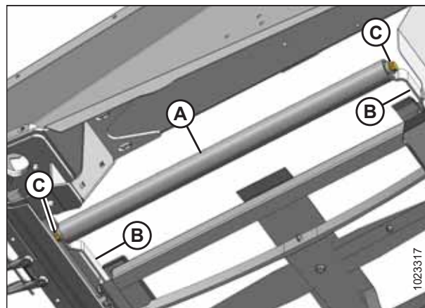
Рисунок 4.258: Натяжной ролик
