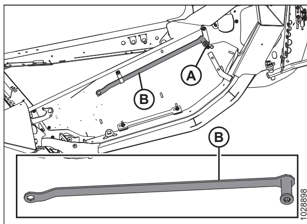
Рисунок 3.190: Левая торцевая обшивка
