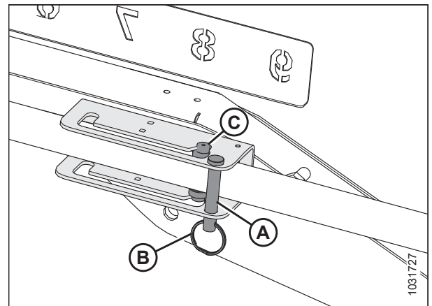
Рисунок 3.180: Регулировка цилиндра перемещения вперед/назад, тип 2 — заднее положение
