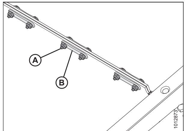
Рисунок 4.185: Стыковочная планка полотна
