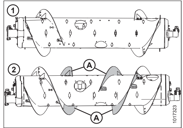
Рисунок 3.77: Конфигурации шнека: вид сзади
