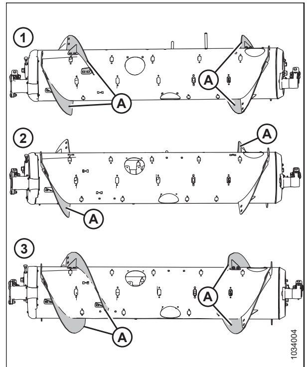
Рисунок 3.97: Конфигурации шнека: вид сзади
