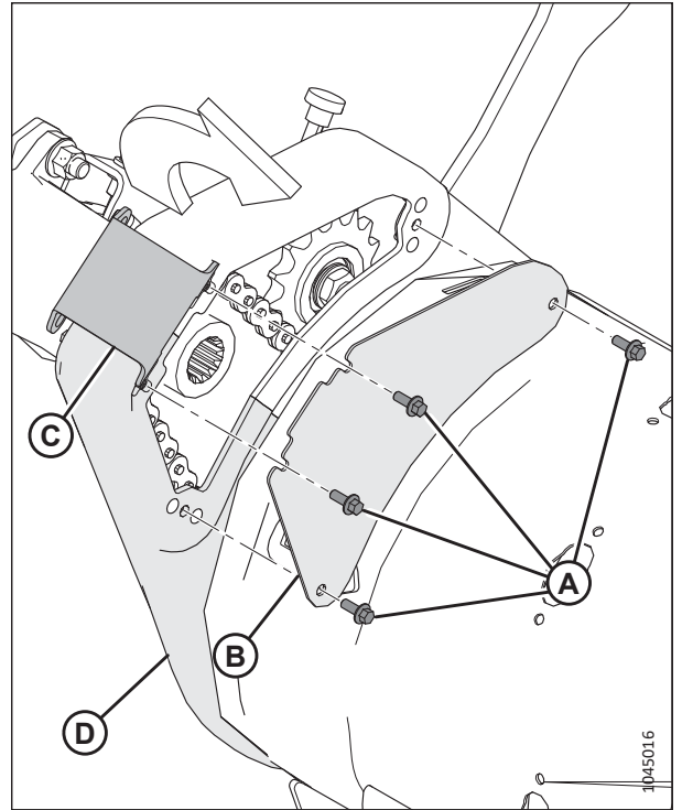
Рисунок 4.80: Привод подающего шнека - вид сзади
