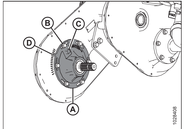
Рисунок 4.69: Крышка натяжителя цепи комплектного редуктора
