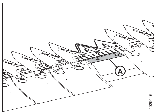
Рисунок 4.147: Ножевой брус
