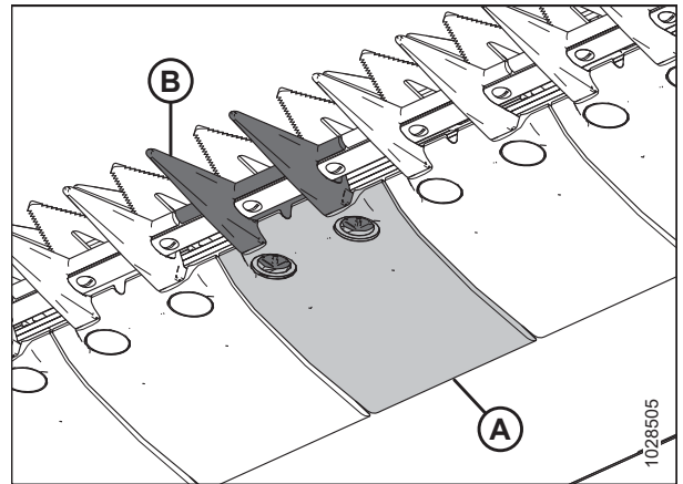
Рисунок 4.159: Укороченный противорежущий палец и износная пластина
