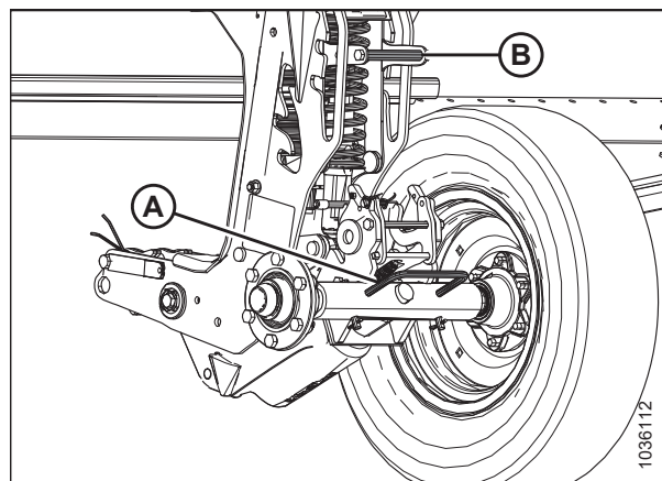
Рисунок 3.314: Левые транспортные колеса в самом высоком положении хранения
