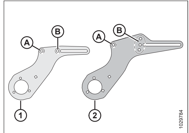
Рисунок 3.195: Сведения о регулируемых креплениях
