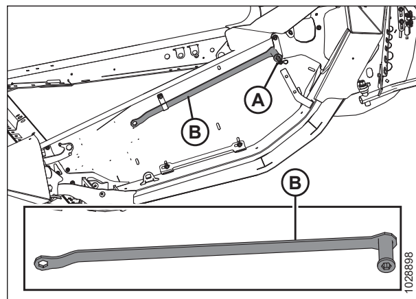
Рисунок 3.173: Левая торцевая обшивка
