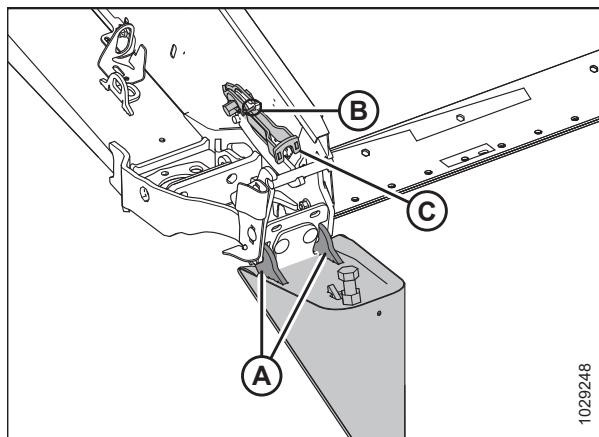
Рисунок 3.203: Делитель с опцией замка
