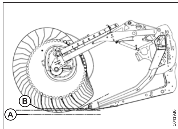
Рисунок 3.187: Профиль пальцев — положение эксцентрика 3
