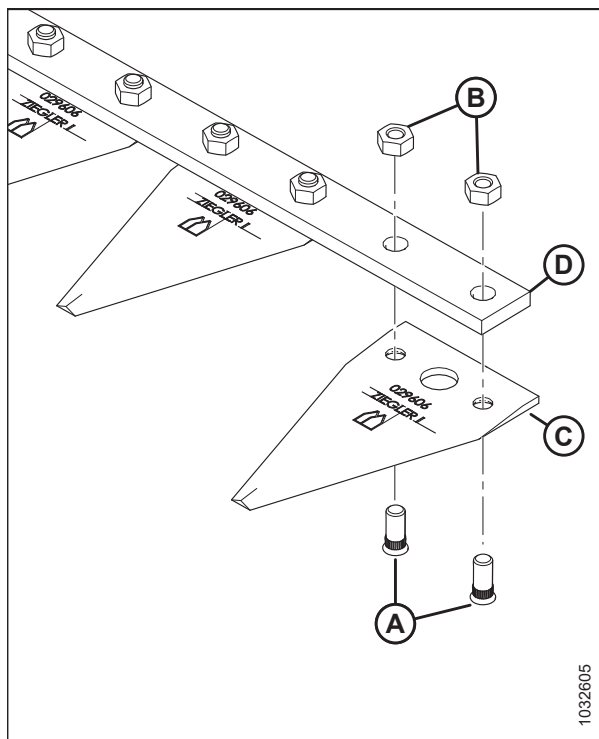
Рисунок 4.364: Узел секции ножа
