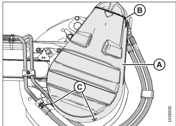
Рисунок 3.28: Крышка привода
