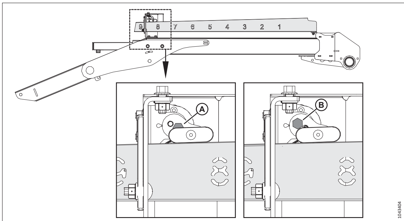
Рисунок 3.181: Конфигурации рычага датчика
