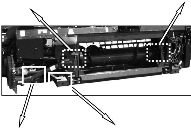
AUGER PIVOT
