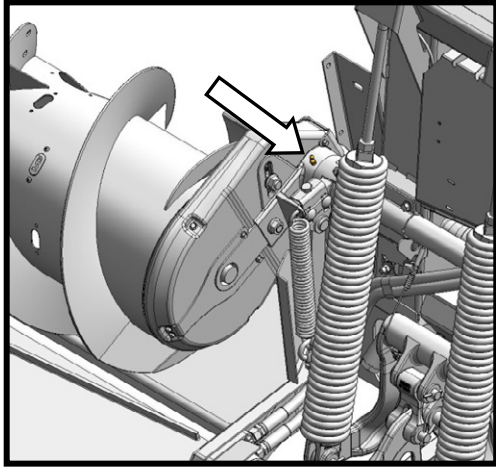
AUGER PIVOT
